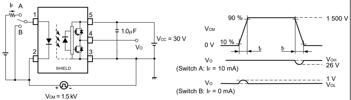
図9 CMR測定回路と波形
