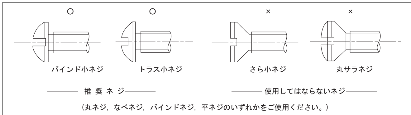
図8 推奨のネジ, 使用してはならないネジの種類
