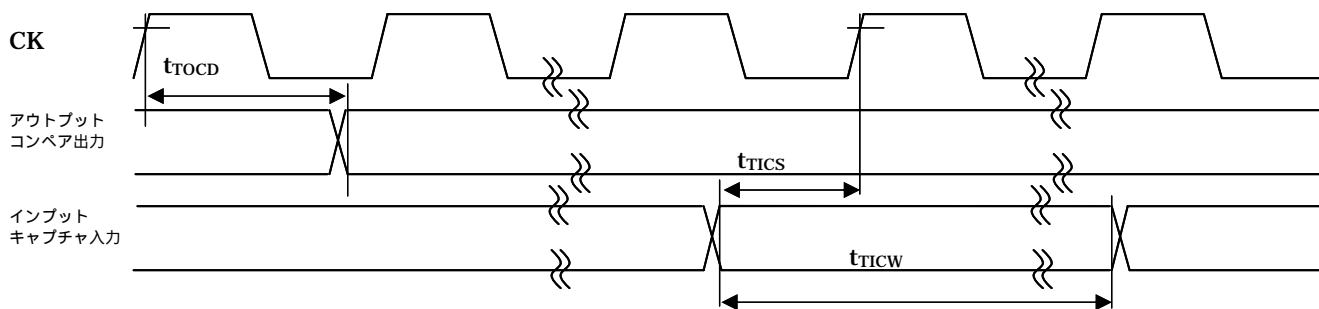
図 31.40(1) MTU2 入出力タイミング
