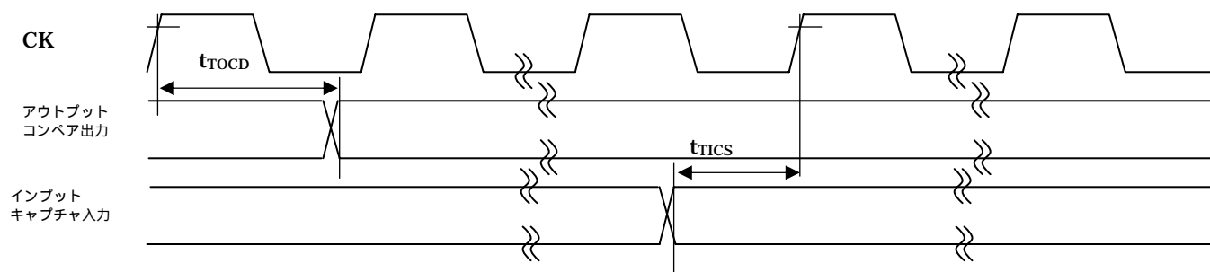
図 31.40 MTU2、MTU2S 入出力タイミング
