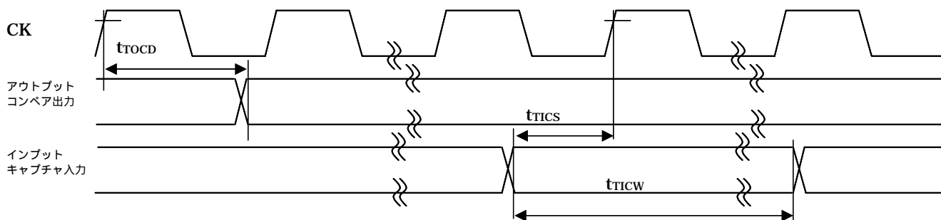
図 31.40(2) MTU2S 入出力タイミング
