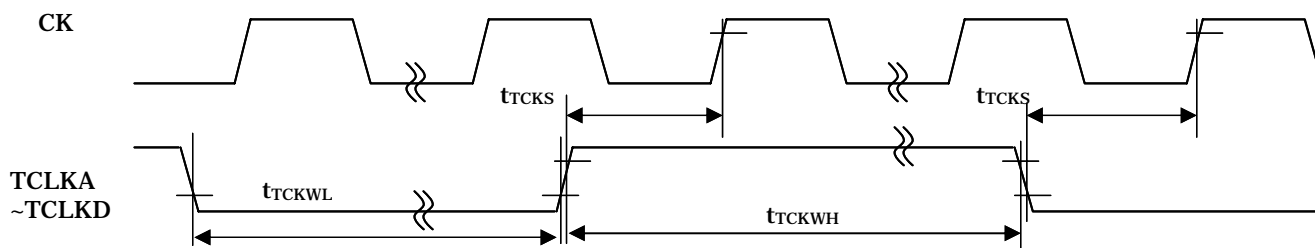
図 31.41 MTU2、MTU2S クロック入力タイミング
