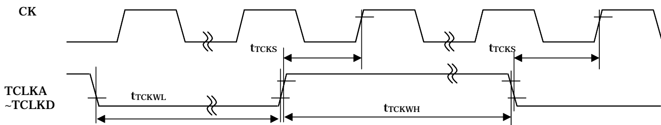
図 31.41(1) MTU2 クロック入力タイミング
