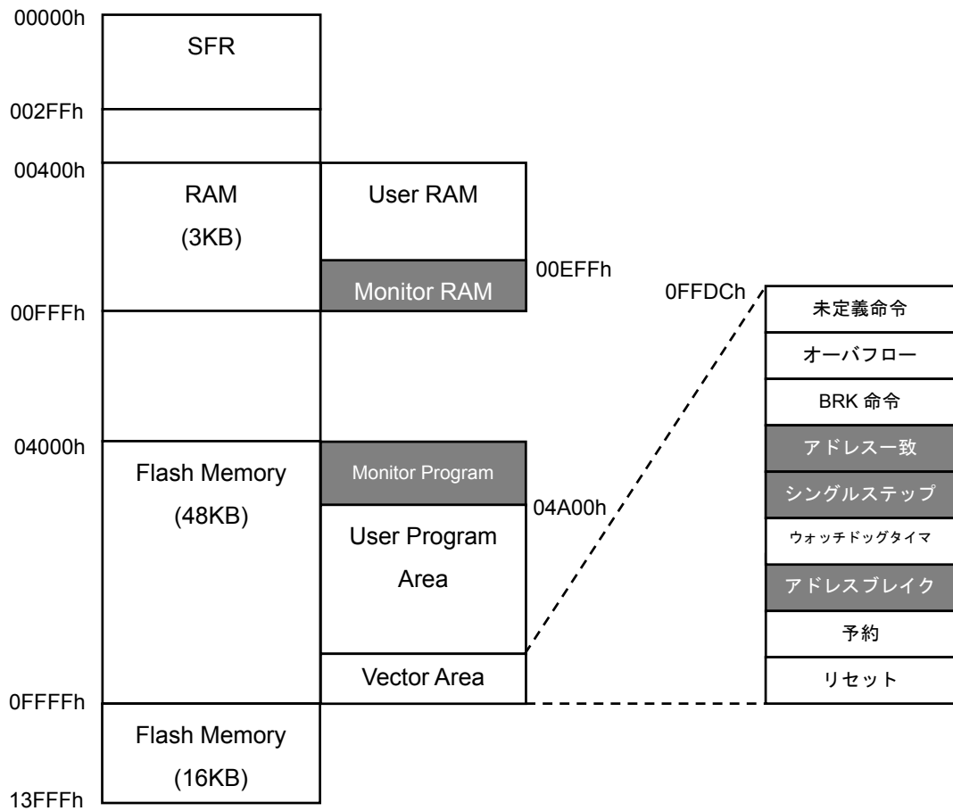
図 4にR8C/Tinyフラッシュメモリ 64KB内蔵版のメモリマップを示します。
