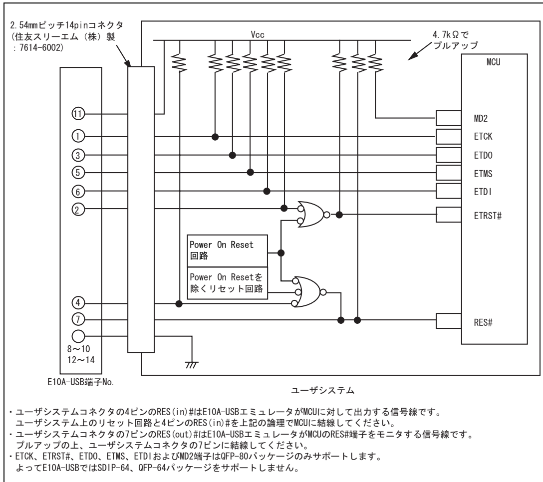
図 1.3 E10A-USB との接続例
