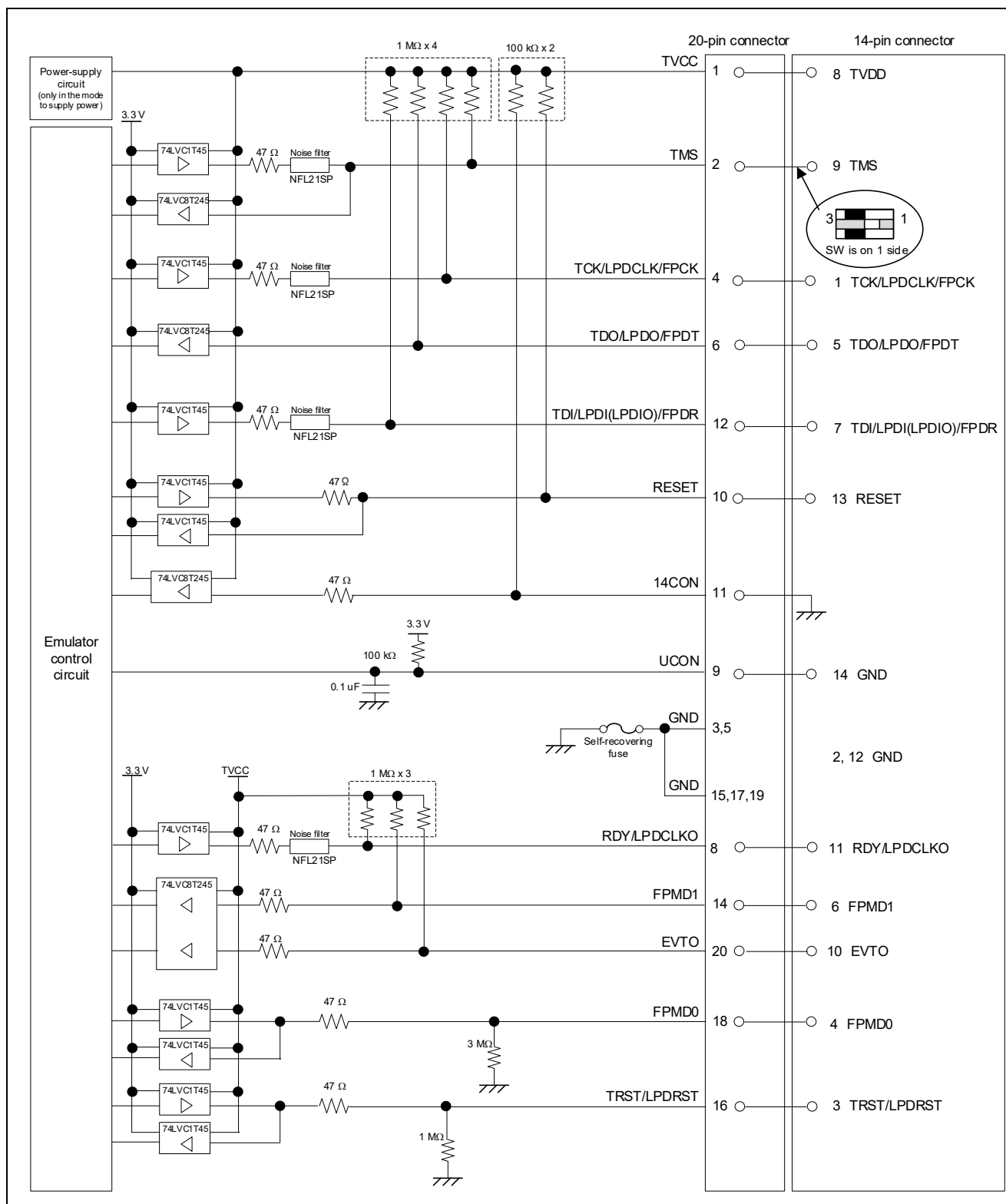
図 5-3 E2 エミュレータ (Rev.C) 内インタフェース回路 (LPD 4pin、JTAG、1wireUART、2wireUART、CSI)
