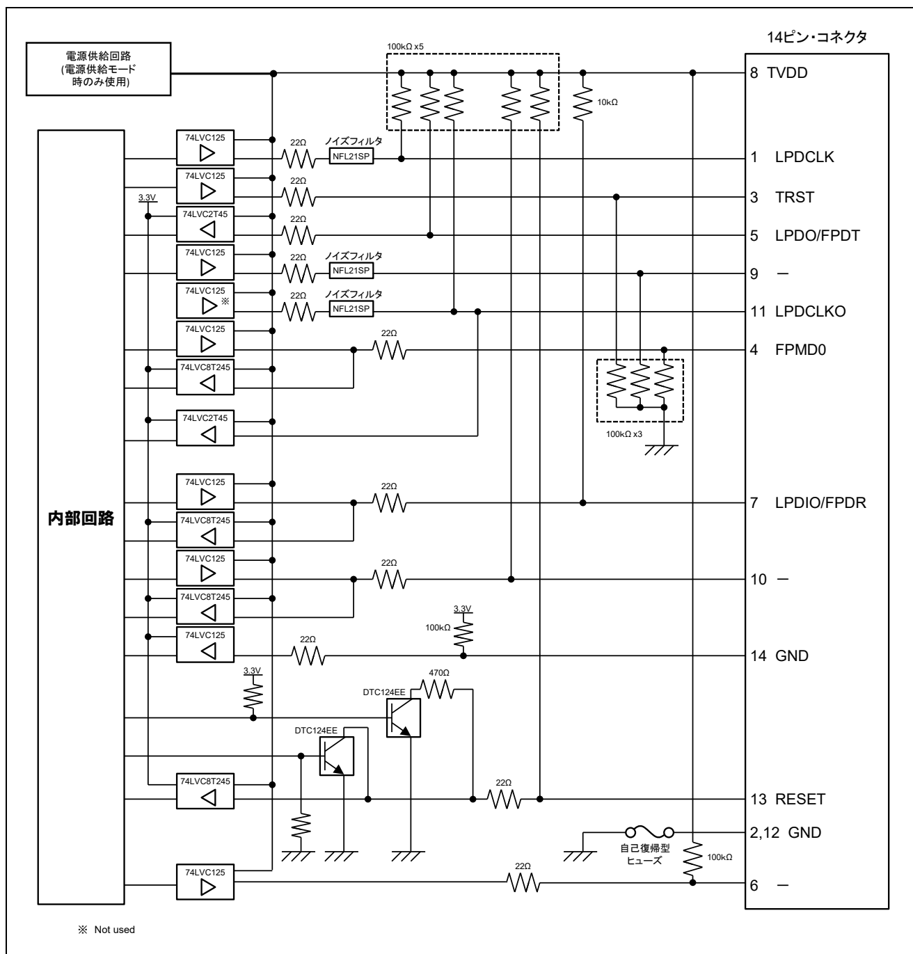
図 5-2 E1/E20 エミュレータ内インタフェース回路(LP4pin、2wireUART)
