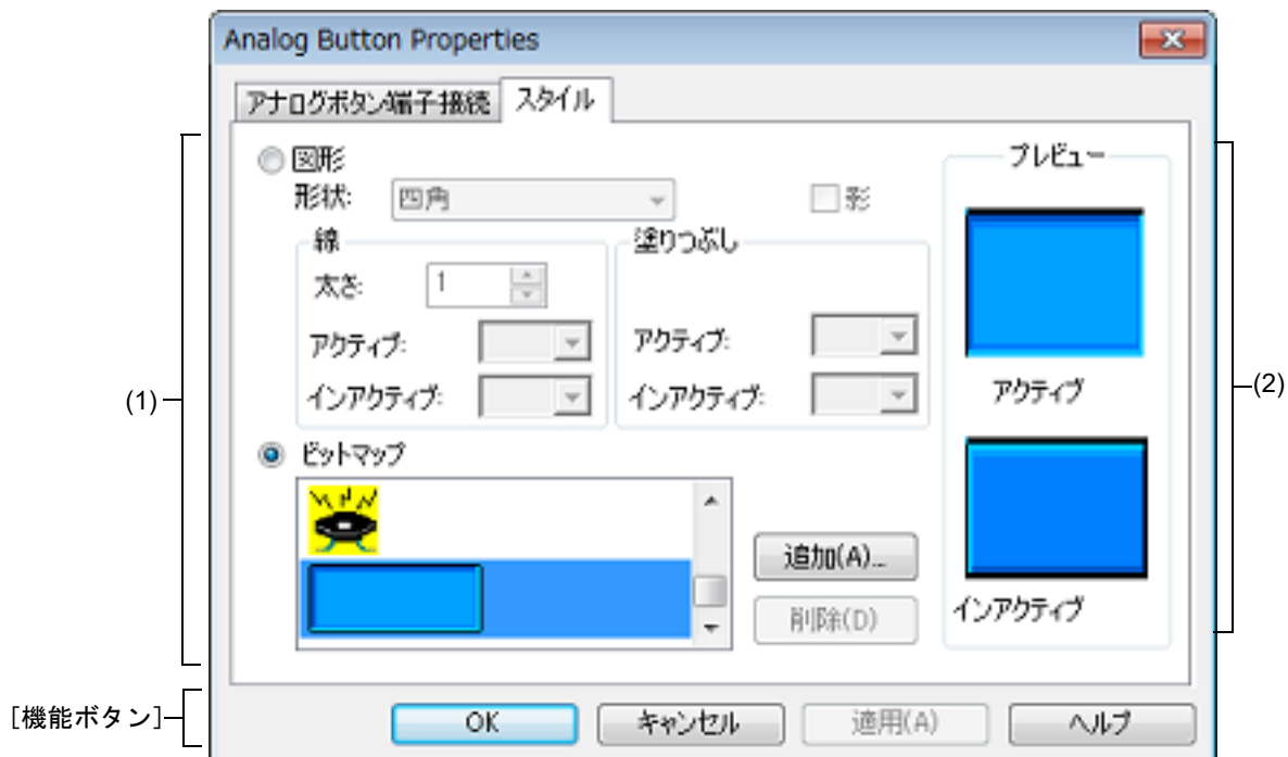
図 A.66 Analog Button Properties ダイアログ : [スタイル] タブ
