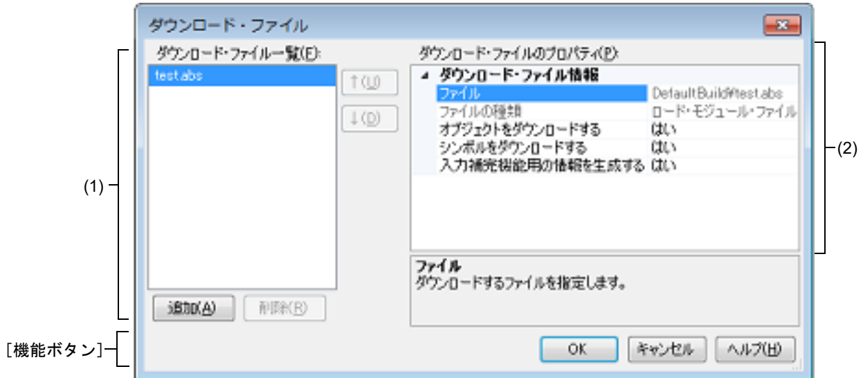
図 A.20 ダウンロード・ファイル ダイアログ
