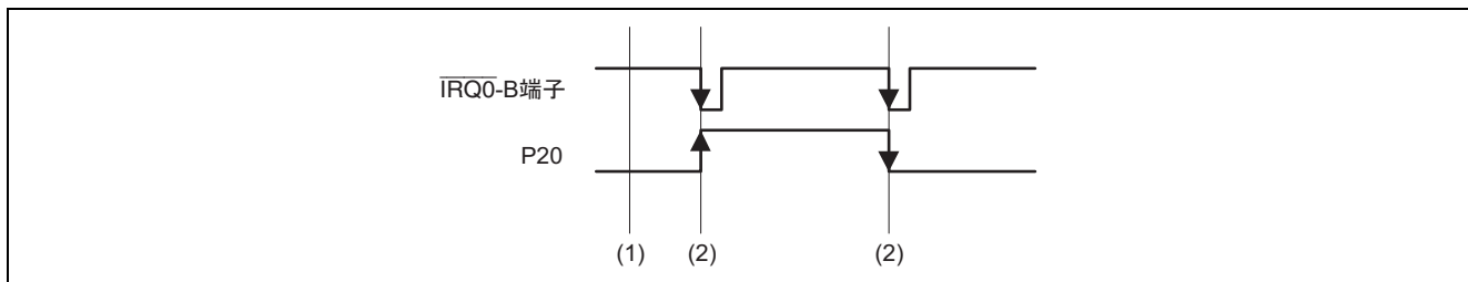
図 4 割り込み制御モード 2 の動作例
