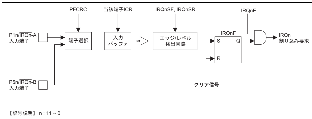
図 2 IRQ n 割り込みのブロック図
