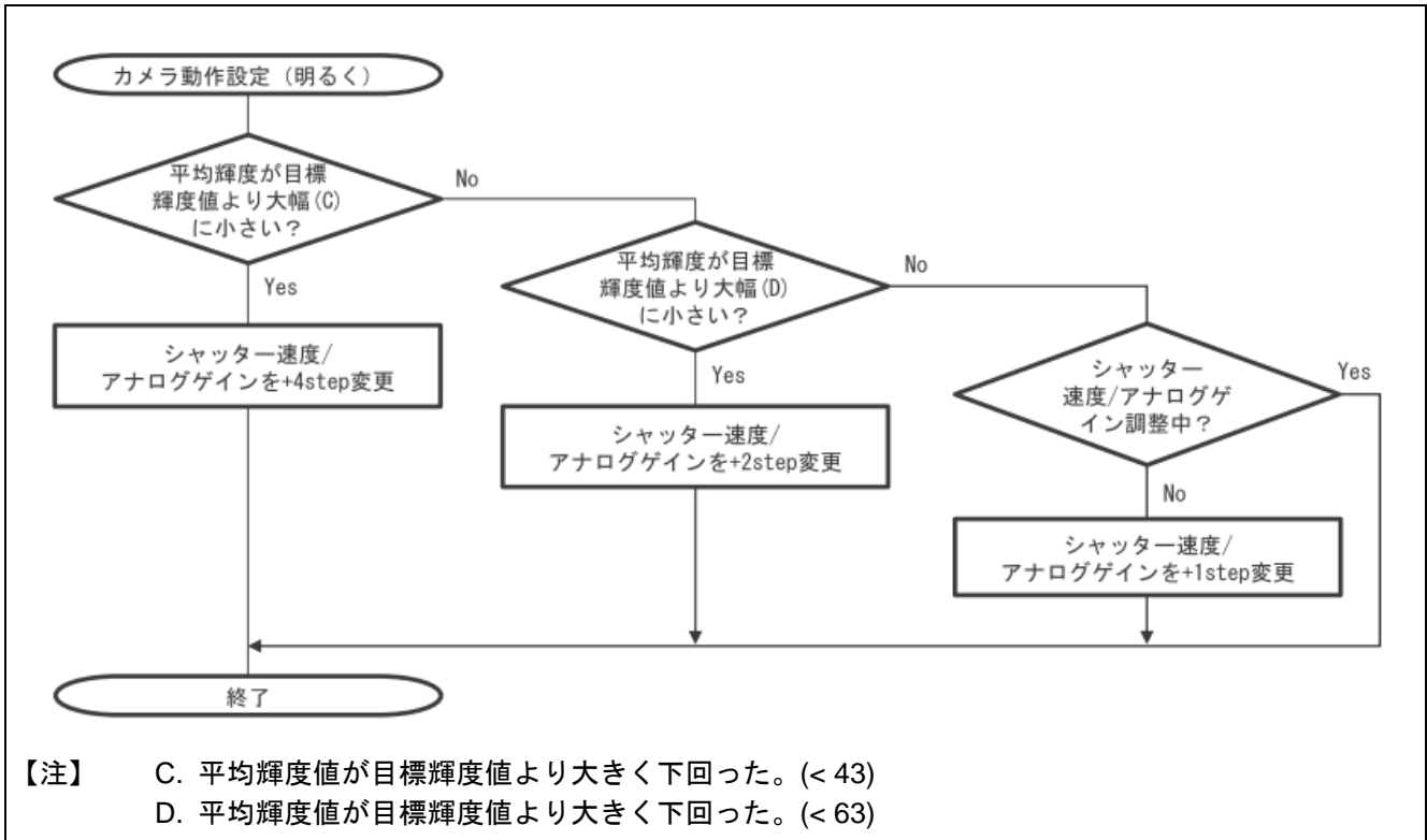
図 4.5 カメラ動作設定(明るく) フローチャート
