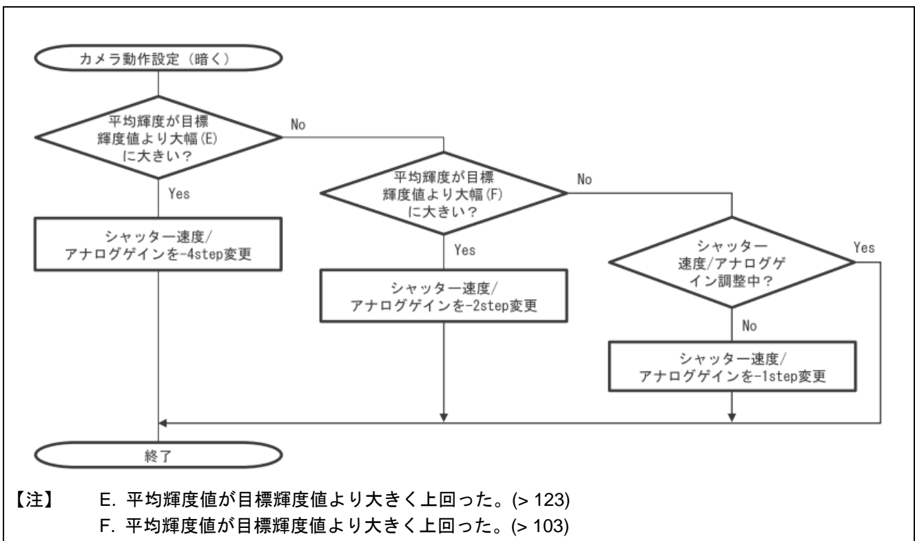
図 4.6 カメラ動作設定(暗く)フローチャート
