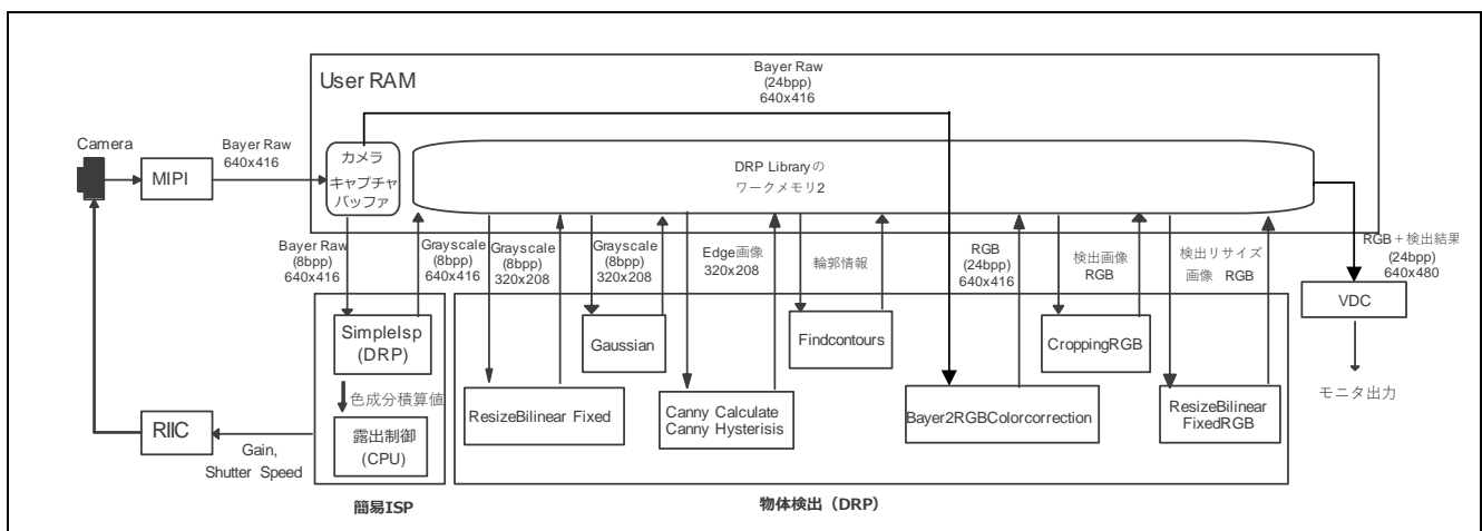
図 4.1 物体検出サンプルプログラムのシステムブロック
