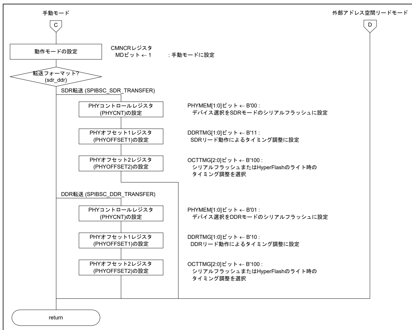
図5.12 SPIBSC 動作モード設定のフローチャート (3/3)
