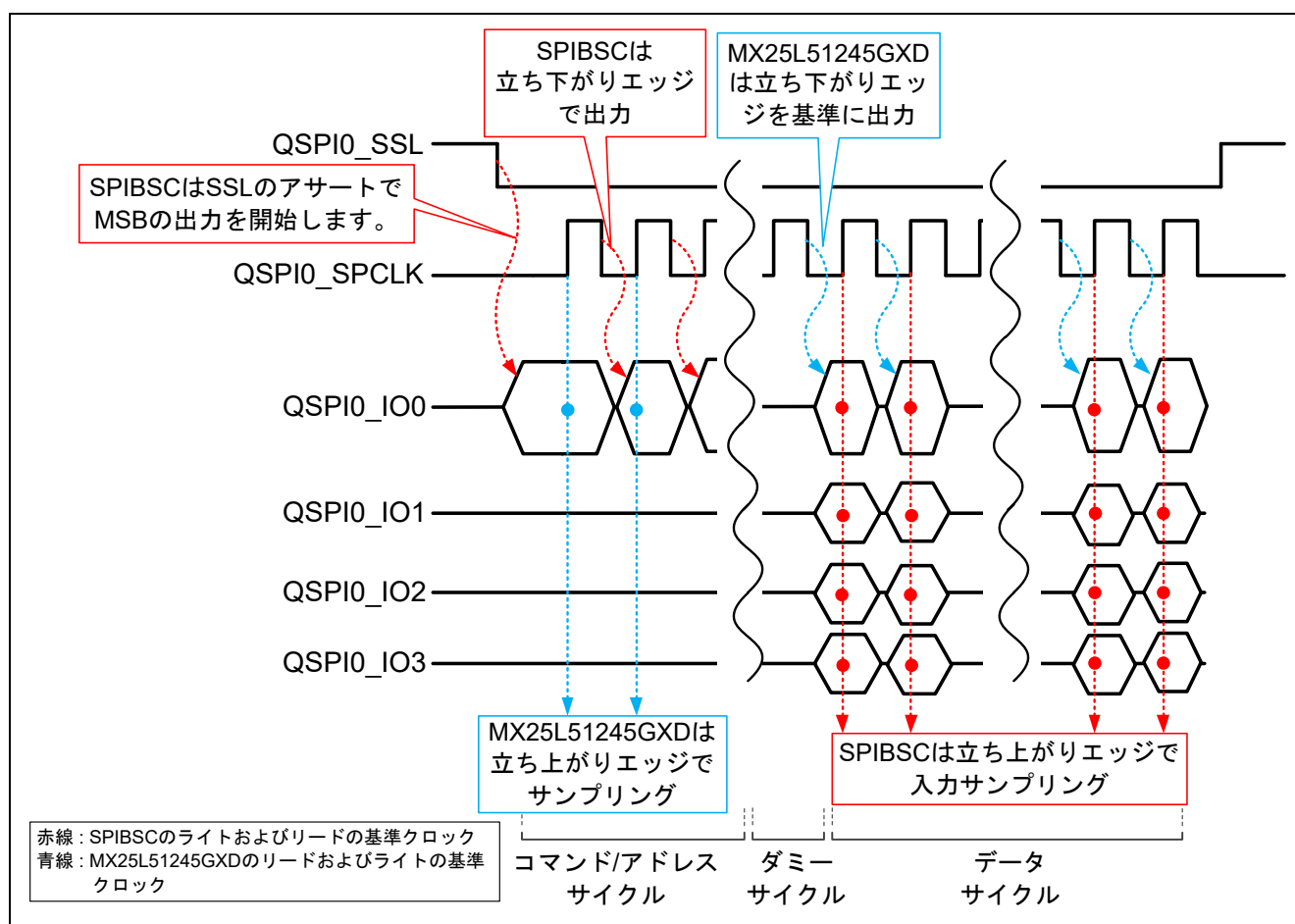
図6.2 SDR 転送のリード動作
