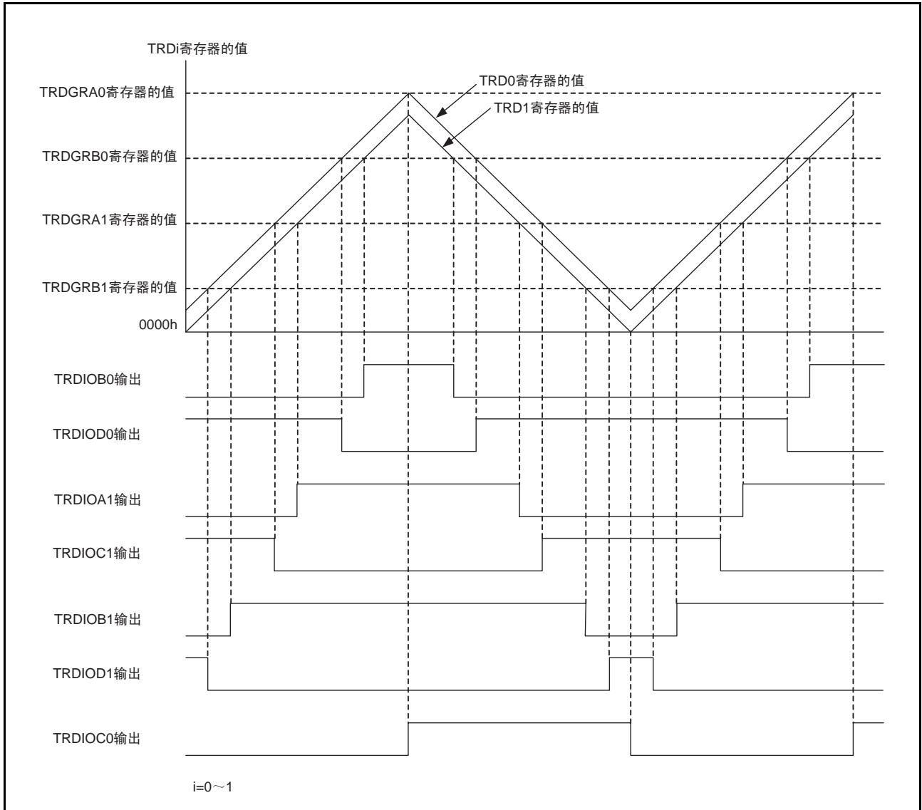
图 13 互补PWM模式的输出模型
