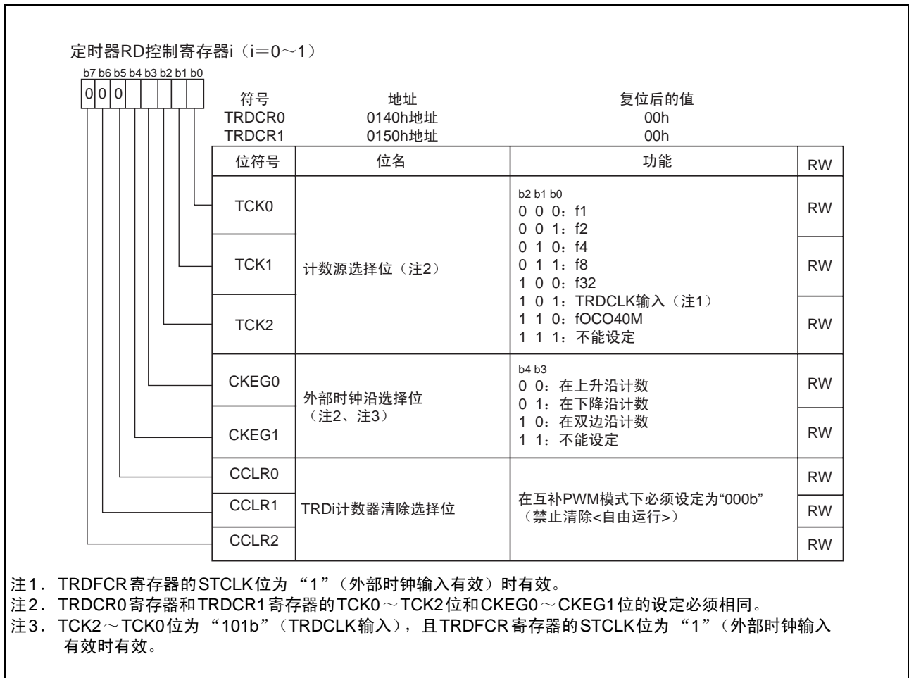
图8 互补PWM模式时的TRDCR0~TRDCR1寄存器
