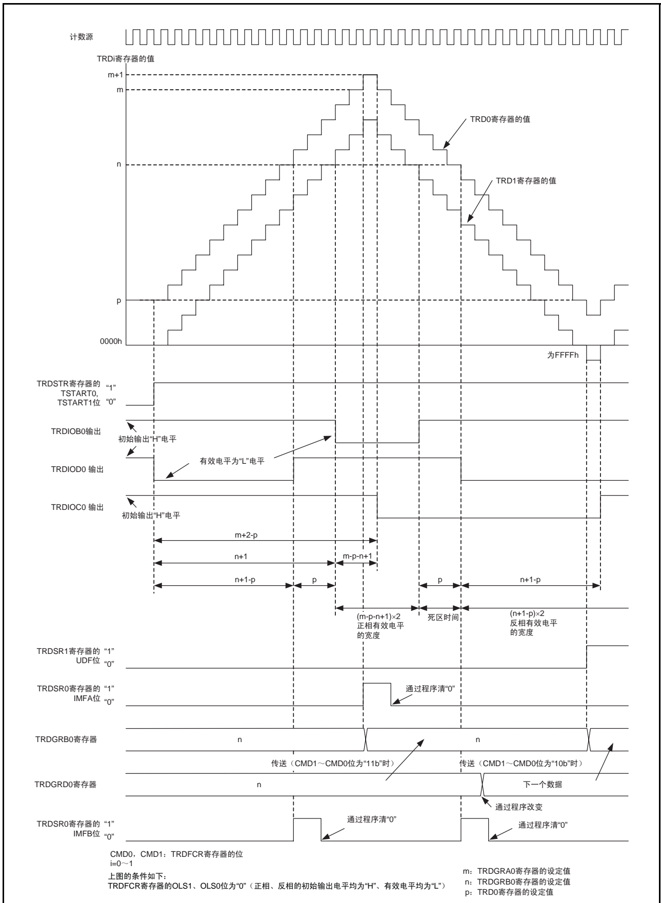
图 14 互补PWM模式的运行示例
