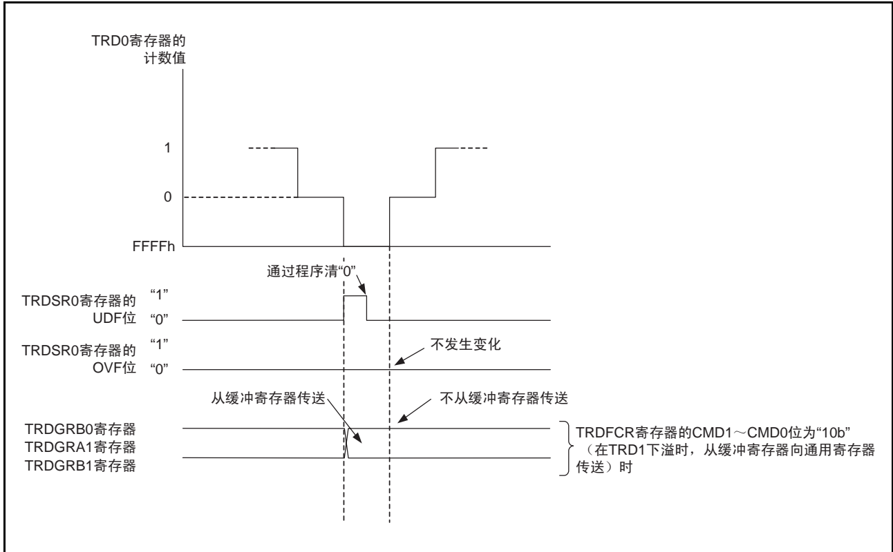
图 17 互补PWM模式 TRD1下溢时的运行
