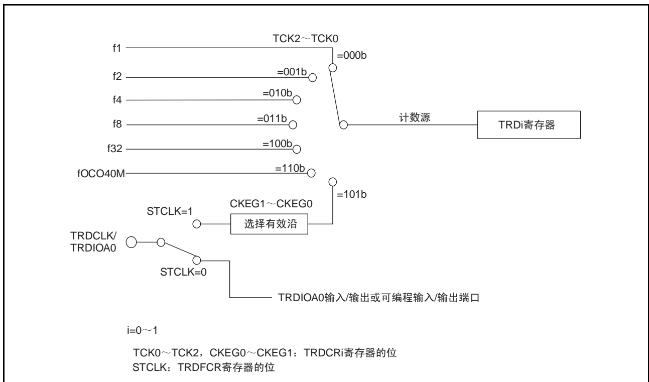
图2 计数源的框图
