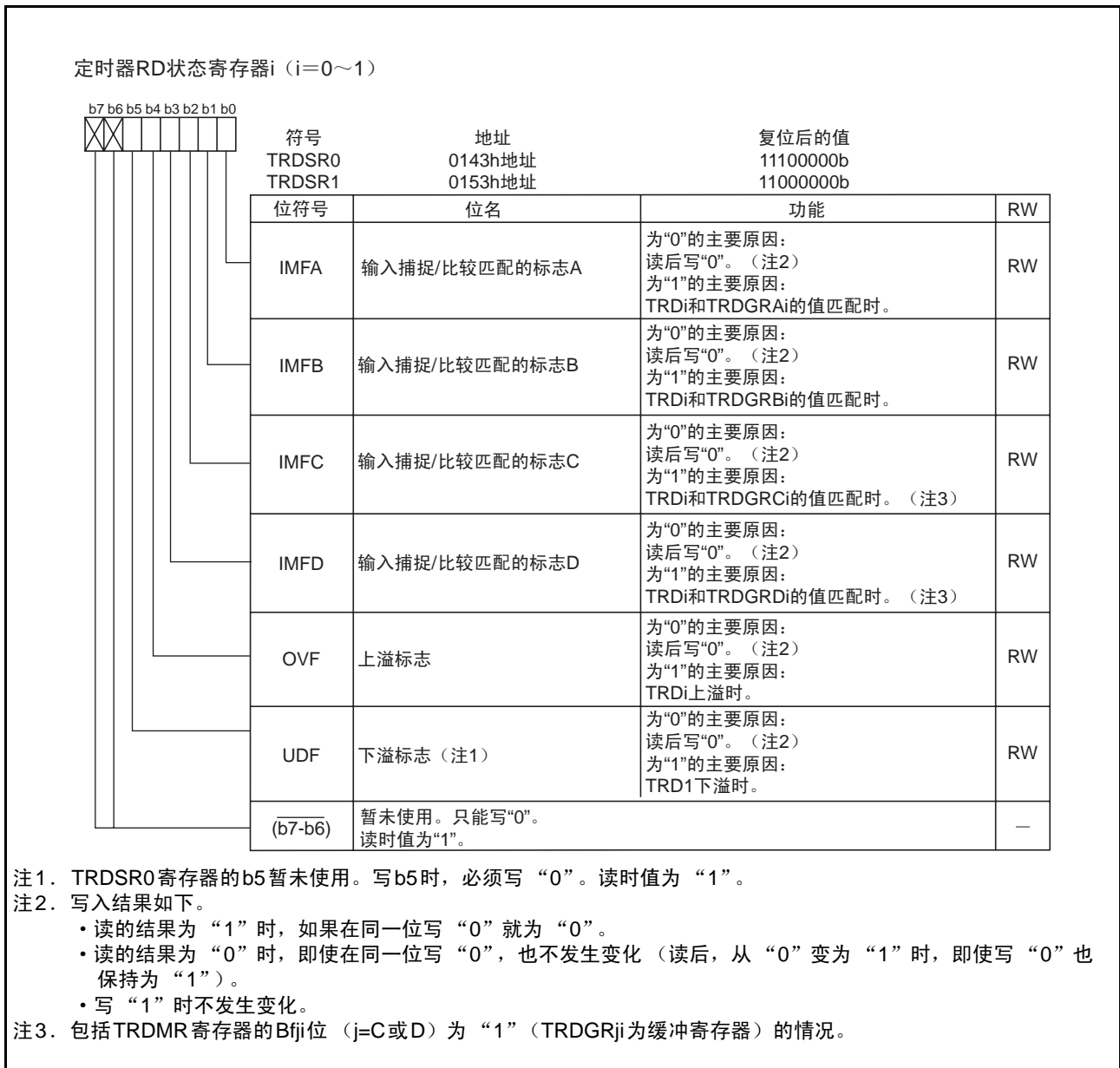
图9 互补PWM模式时的TRDSR0~TRDSR1寄存器
