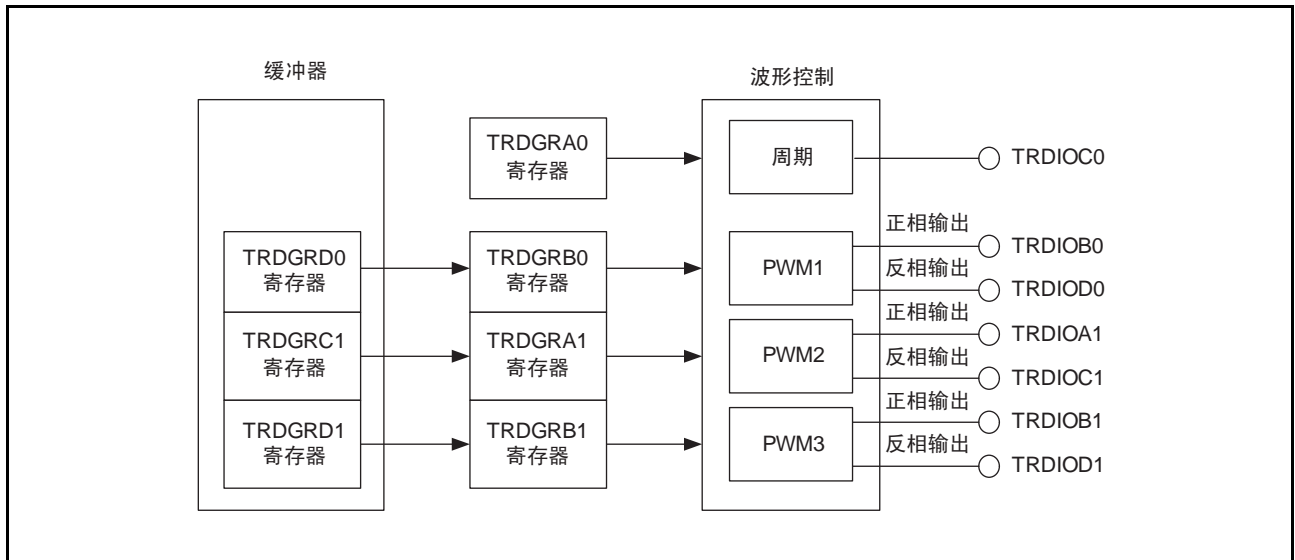
图 4 互补 PWM 模式的框图
