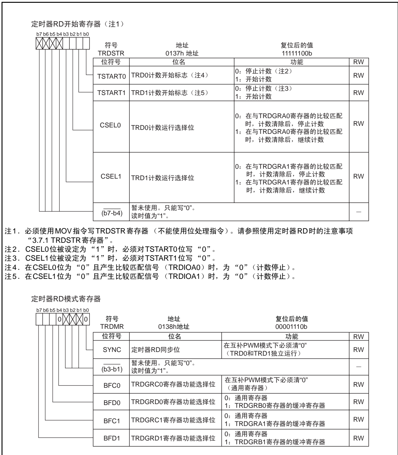
图5 互补PWM模式时的TRDSTR、TRDMR寄存器
