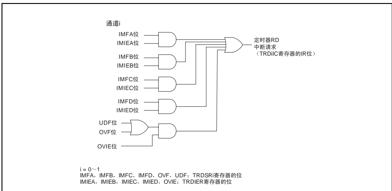
图 15 定时器 RD 中断的框图
