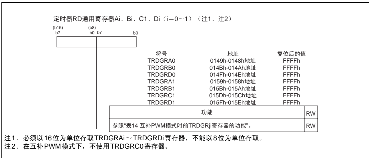
图 12 互补PWM模式时的TRDGRAi、TRDGRBi、TRDGRC1、TRDGRDi寄存器
