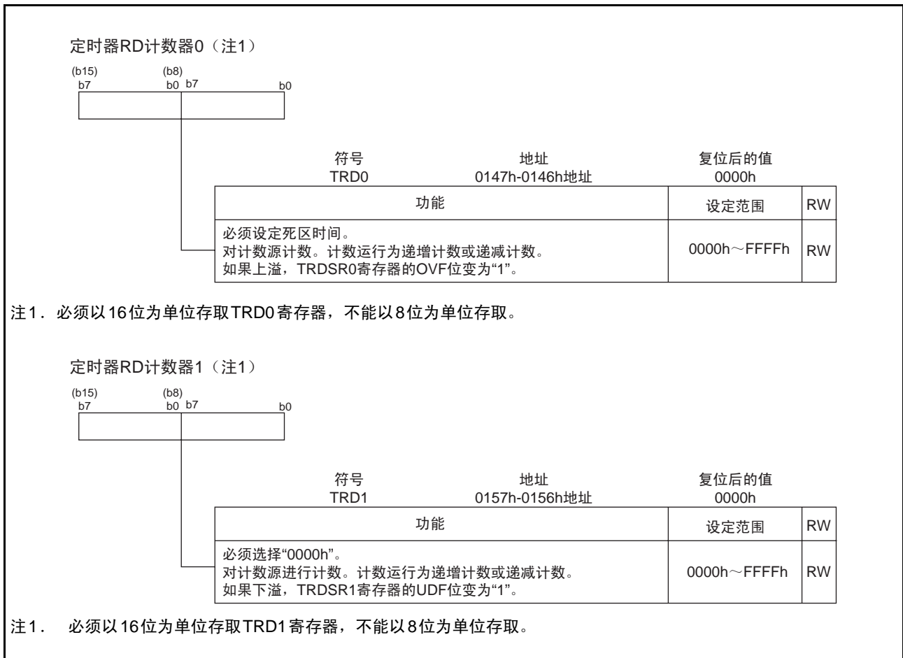
图 11 互补PWM模式时的TRD0~TRD1寄存器
