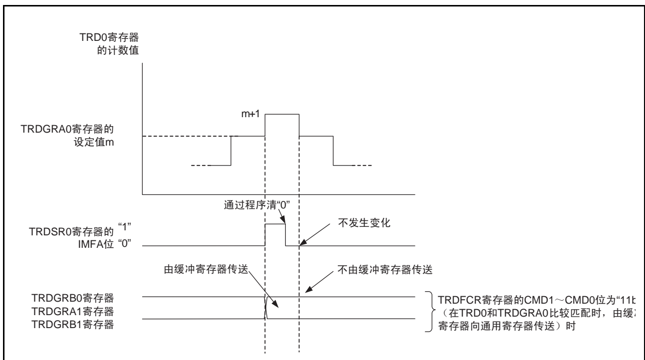
图 16 互补 PWM 模式下 TRD0 和 TRDGRA0 寄存器比较匹配时的运行
