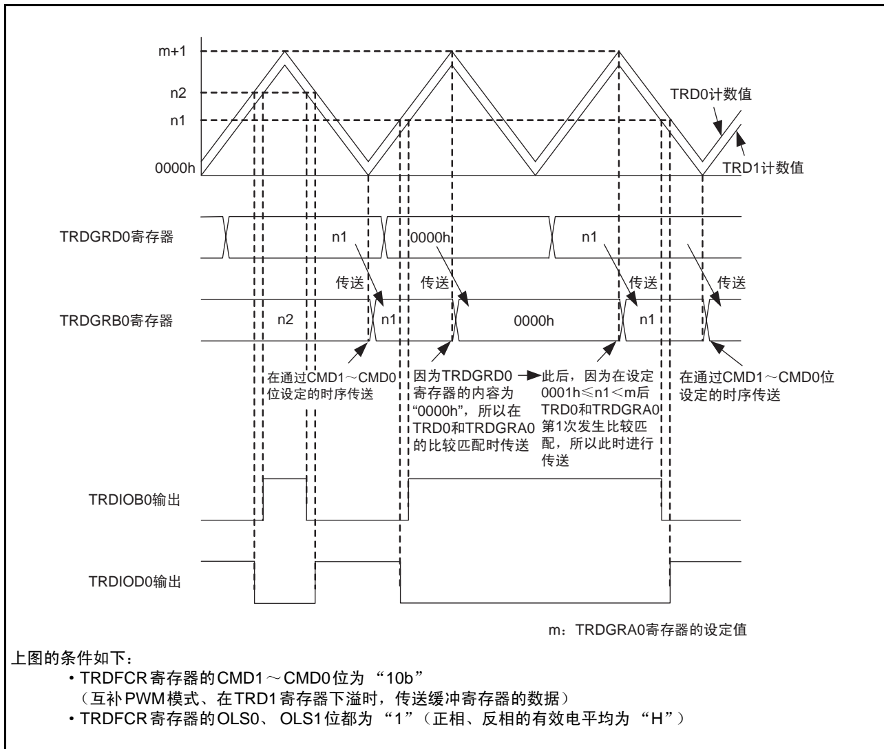
图 19 互补PWM模式时的缓冲寄存器的值为“0000h”时的运行示例
