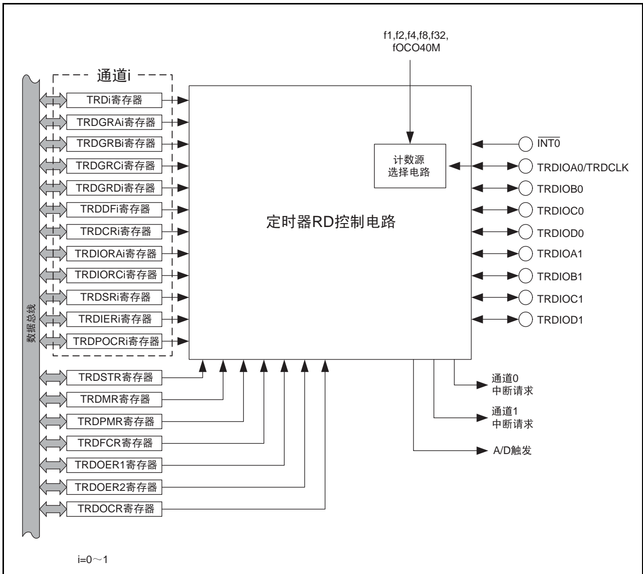
图1 定时器 RD 的框图
