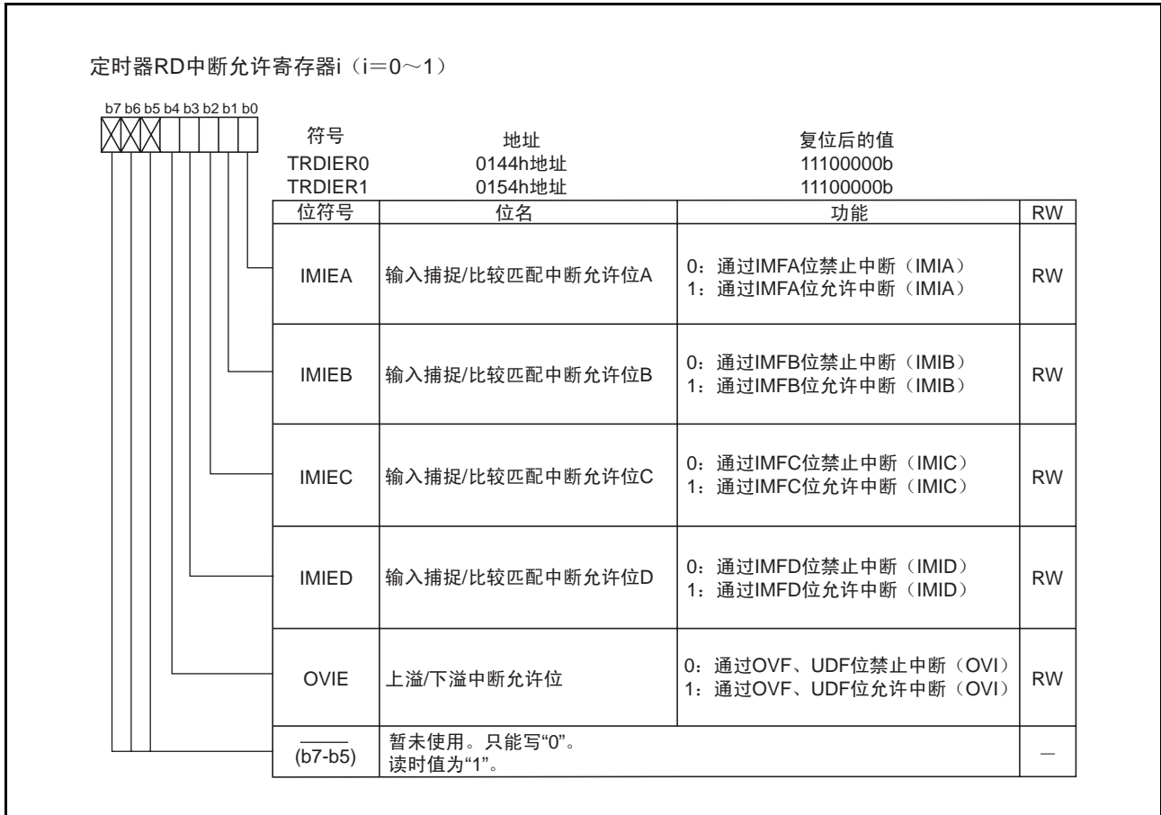
图 10 互补 PWM 模式时的 TRDIER0 ~ TRDIER1 寄存器
