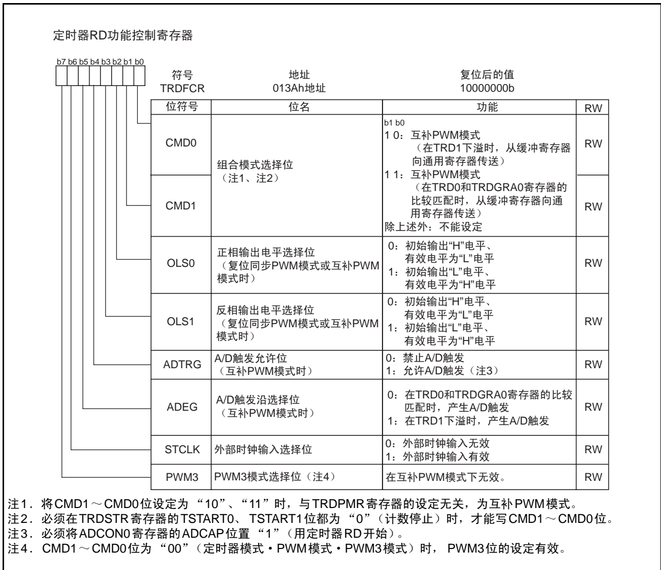
图6 互补PWM模式时的TRDFCR寄存器
