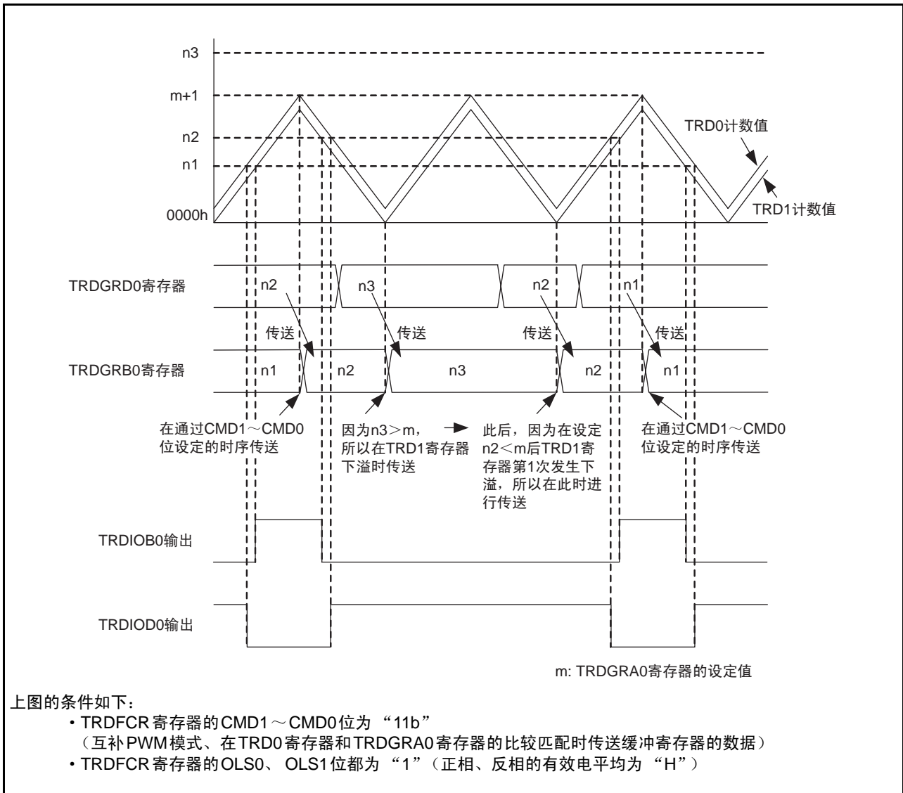
图18 互补PWM模式时的缓冲寄存器的值大于等于TRDGRA0寄存器的值时的运行示例
