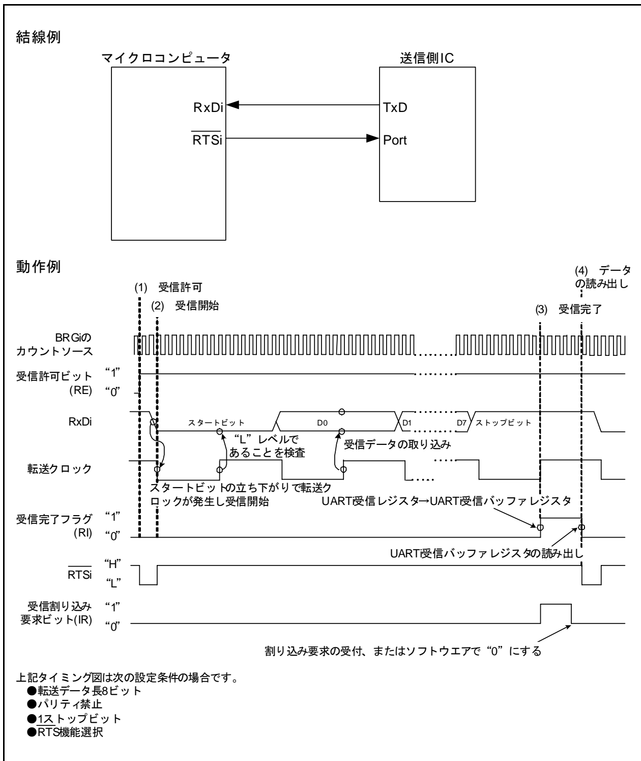
図 4.1 クロック非同期形シリアル I/O モードの受信動作タイミング
