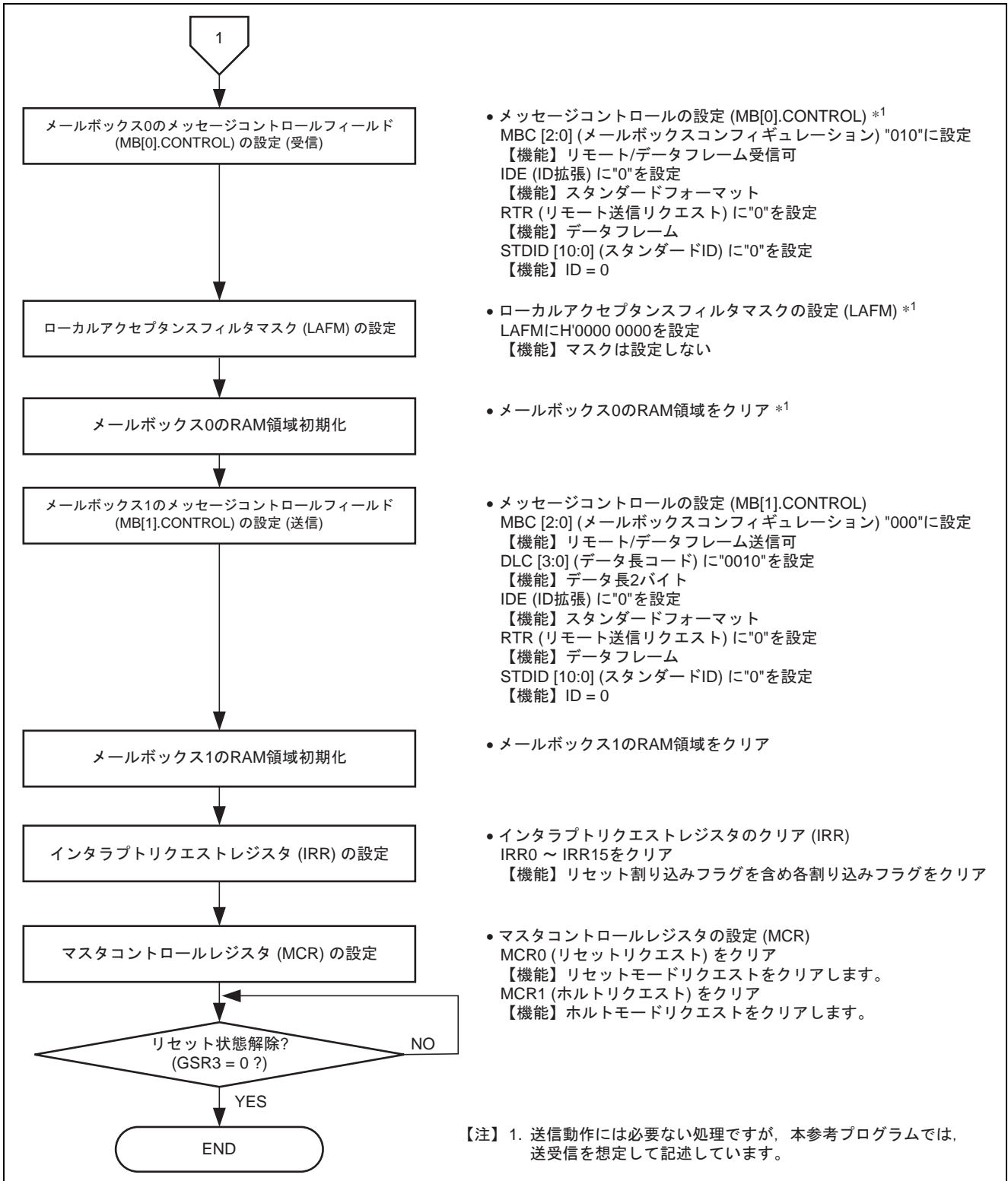
図3 RCAN-TL1の初期設定フロー例 (2)
