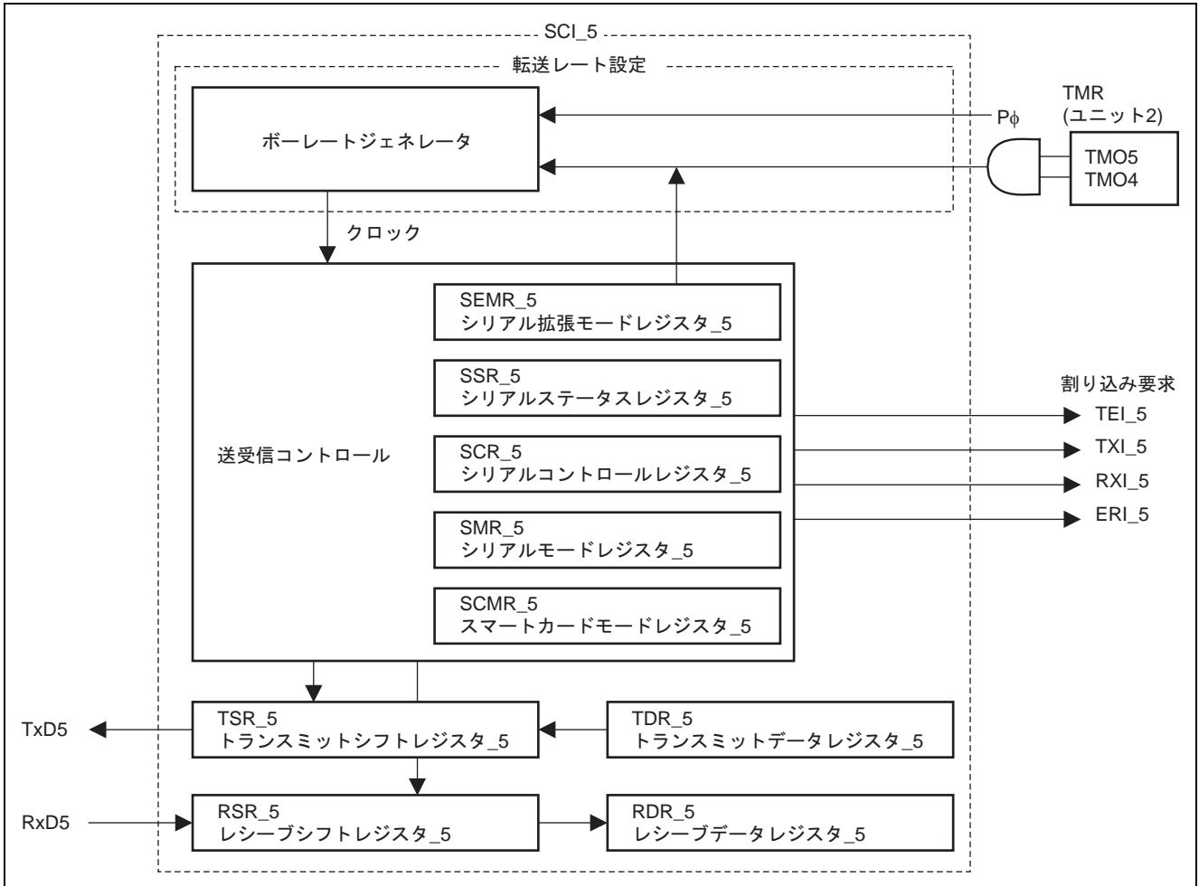
図 2 SCI_5 ブロック図
