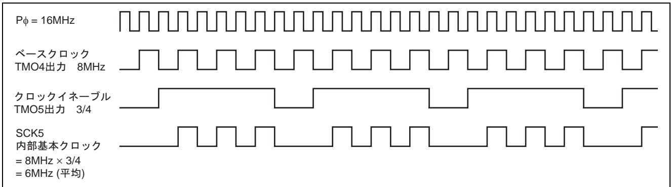
図 9 SCK5 内部基本クロック波形
