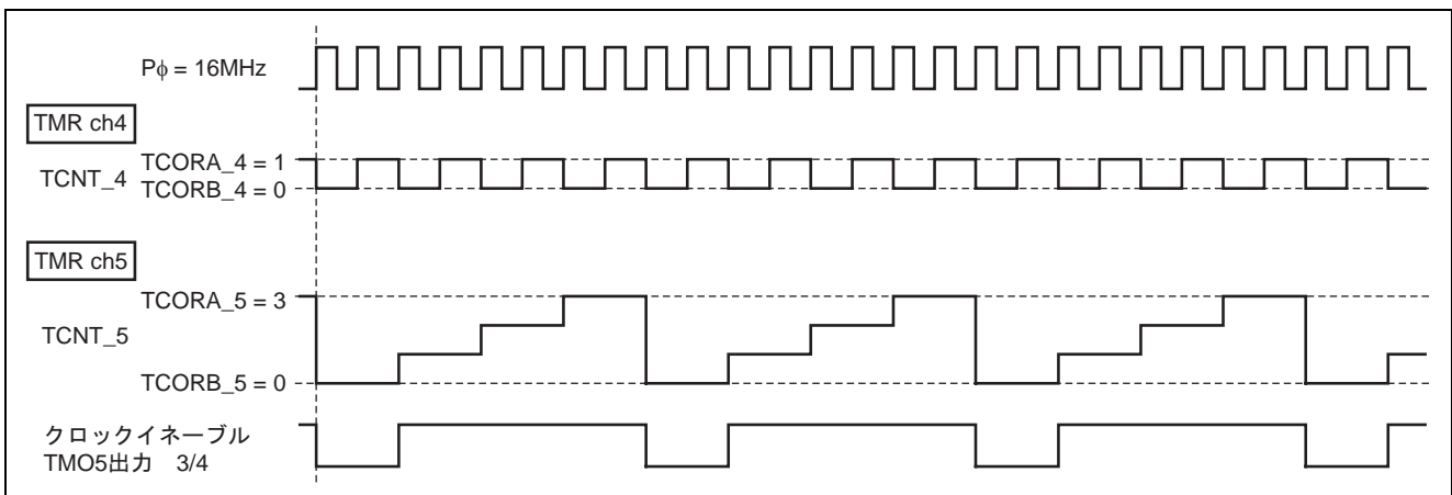
図 8 TMO5 の出力波形
