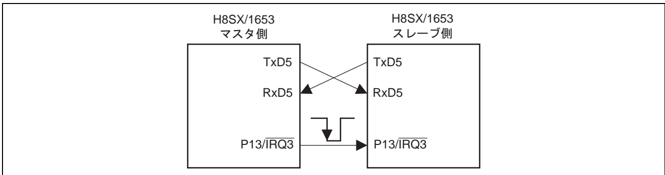
図 1 TMR クロック入力調歩同期式送受信の接続図
