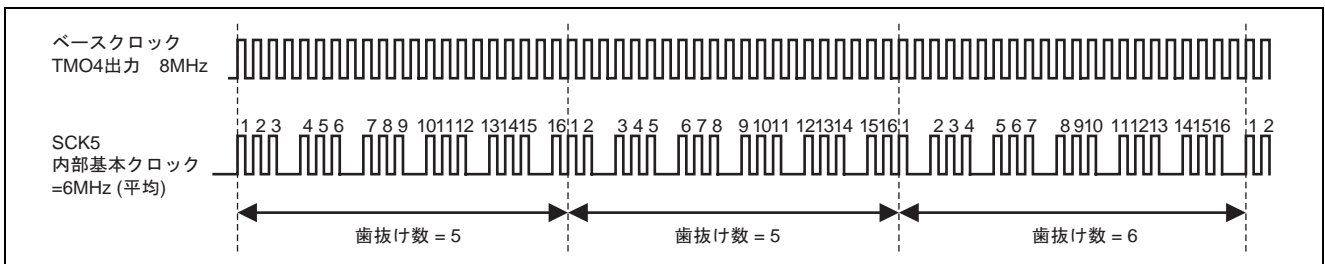
図 10 通信データの 1 ビット期間
