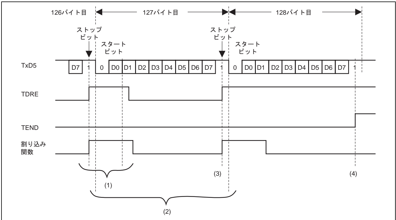
図5 送信動作タイミング
