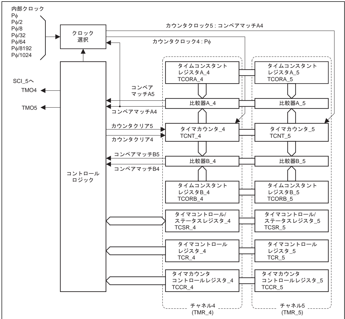
図3 TMR ユニット2ブロック図
