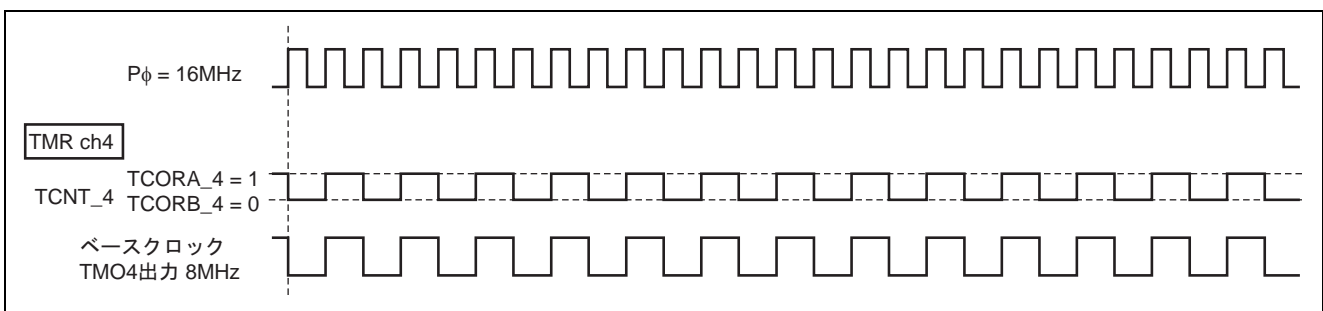
図 7 TMO4 の出力波形
