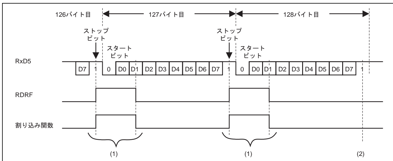
図 6 受信動作タイミング
