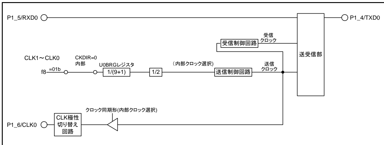
図 3.1 ブロック図
