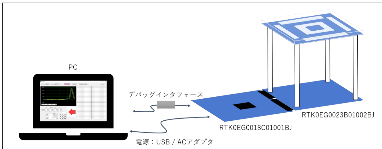
図 2-1 機器接続図
