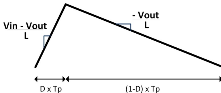
Bild 2: Verlauf des Induktorstroms
