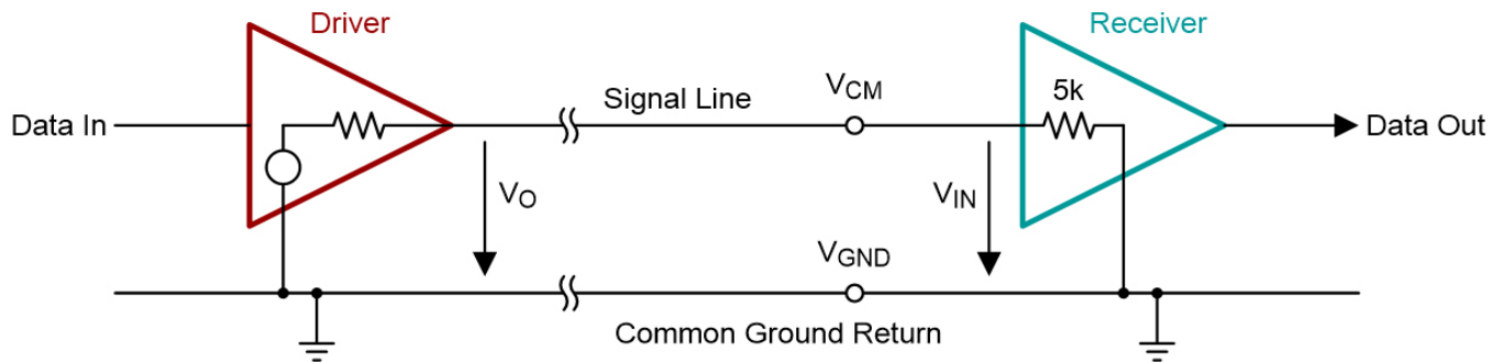
图 1: 单端点对点数据链路
