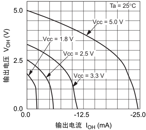
输出特性 ("H"电平)
