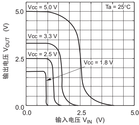
(HD74ALVC1G04)
