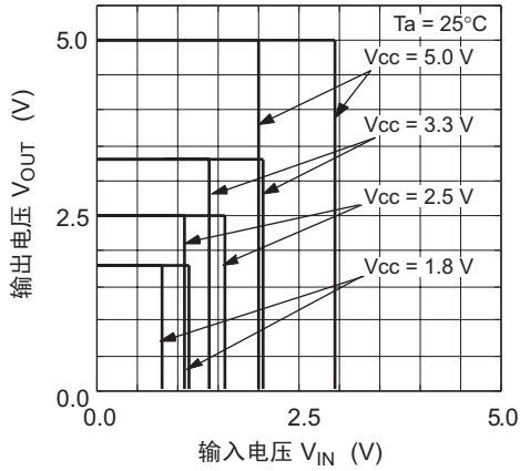
(HD74HC1GU04)
