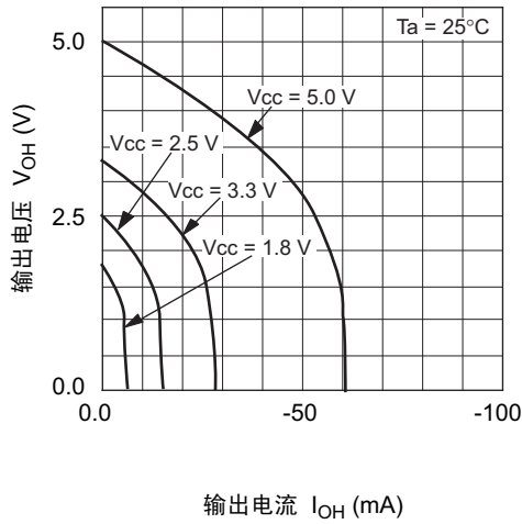
输出特性 ("H"电平)
