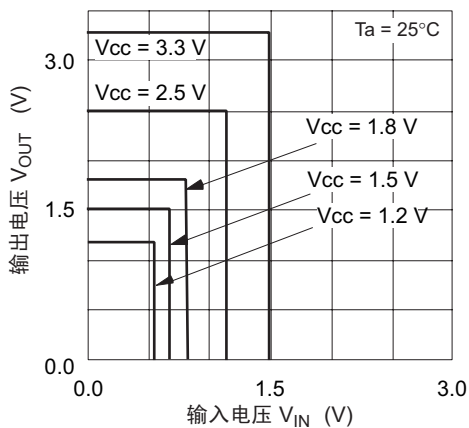
(HD74ALVC1G04)
