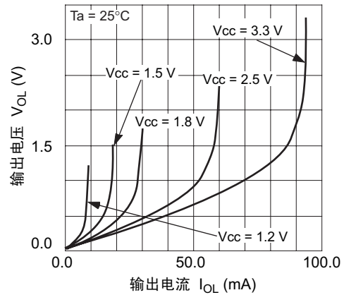
输出特性 ("L"电平)
