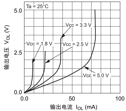
输出特性 ("L"电平)
