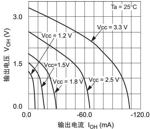
输出特性 ("H"电平)
