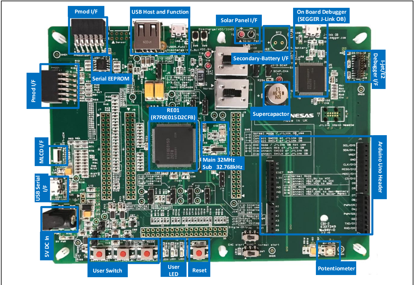
図 2 Evaluation Kit RE01 1500KB 外観図(部品面)
