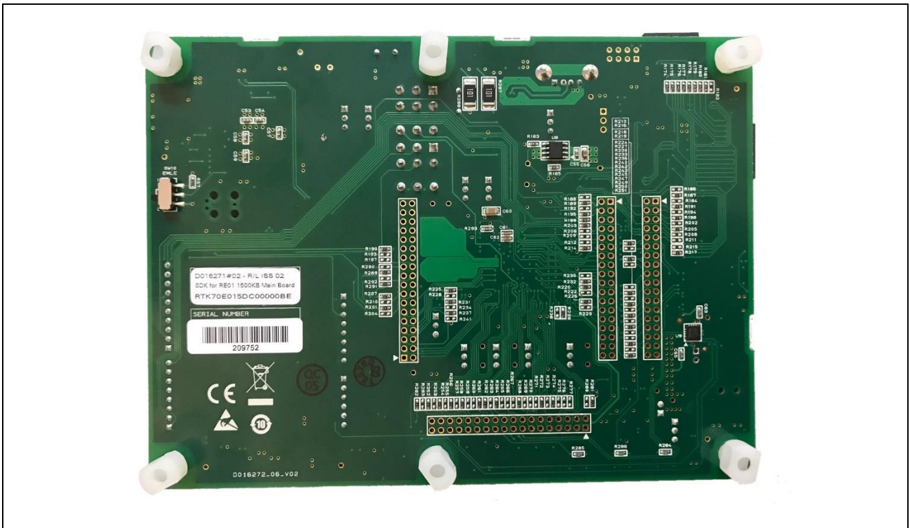
図 3 Evaluation Kit RE01 1500KB 外観図(はんだ面)
