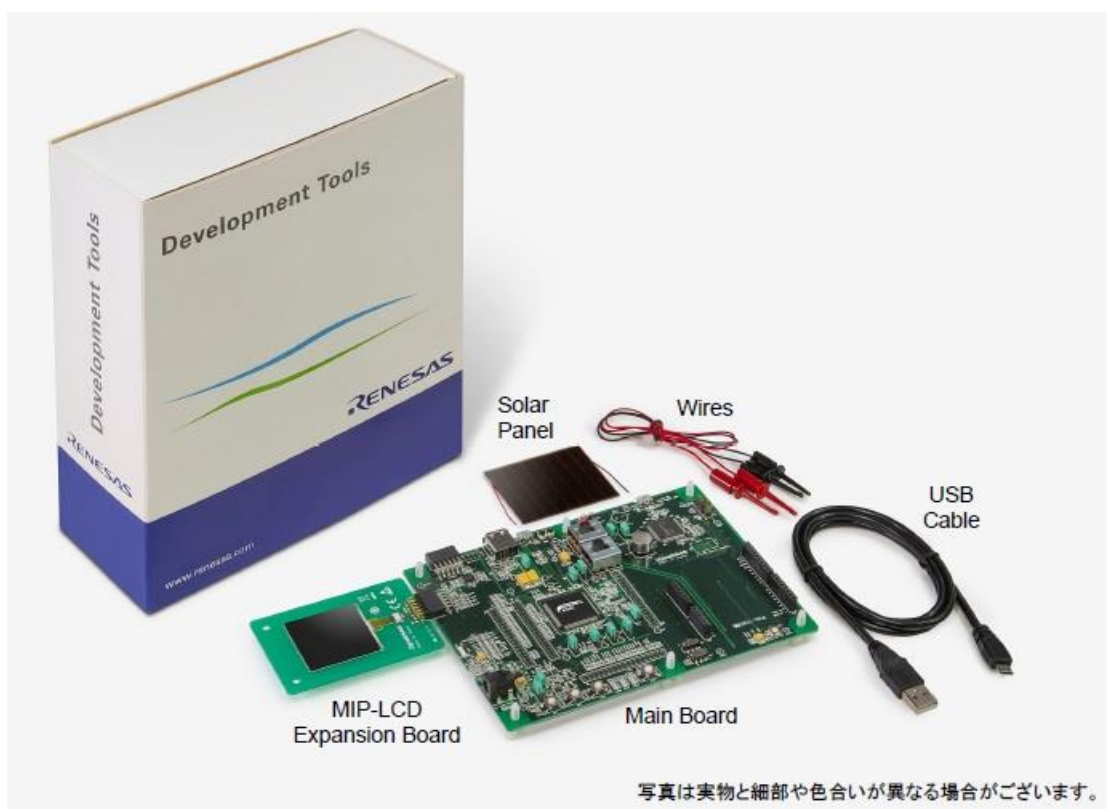
図 1 Evaluation Kit RE01 1500KB
