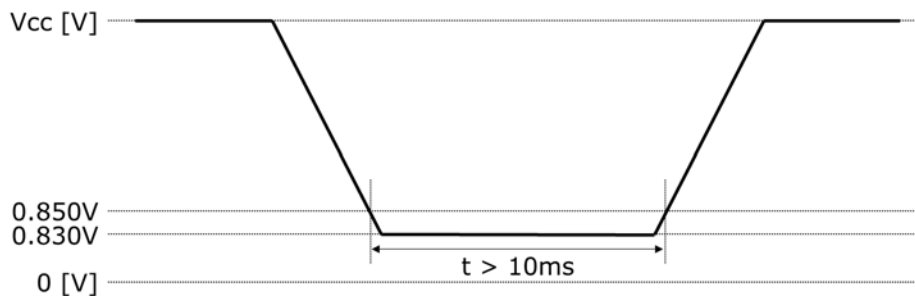
図1. 残電圧のある電源起動波形
