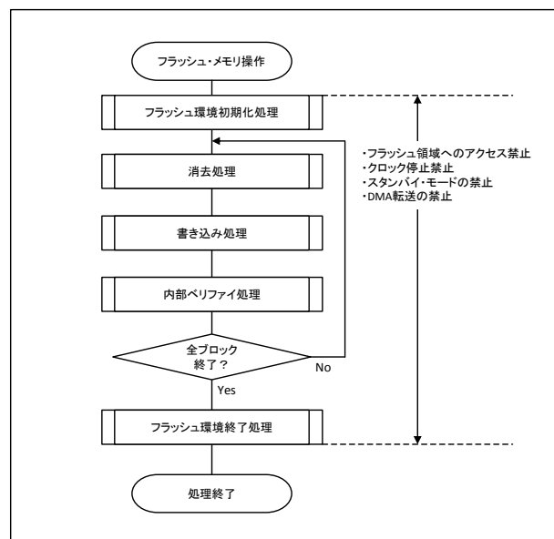
標準セルフ・プログラミング・フロー
