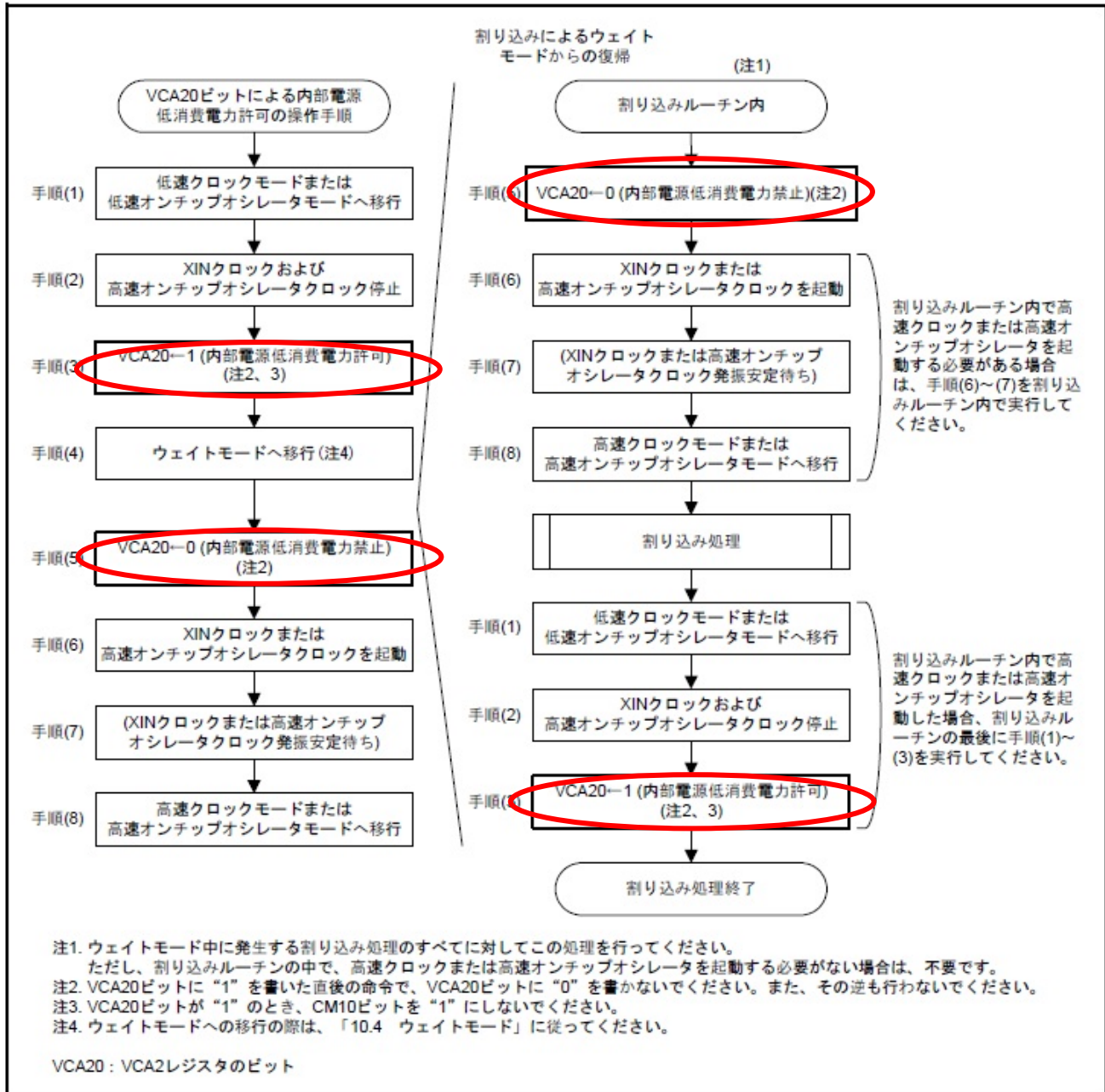
図 10.9 WAIT 命令を実行してウェイトモードにする場合の VCA20 ビットによる内部電源低消費電力操作設定手順
