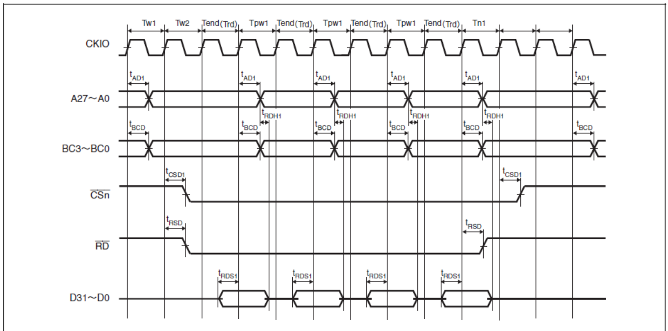
図 31.12 外部アドレス空間基本バスタイミング (ページリードアクセス、外部リードデータ連続アサートモード)
