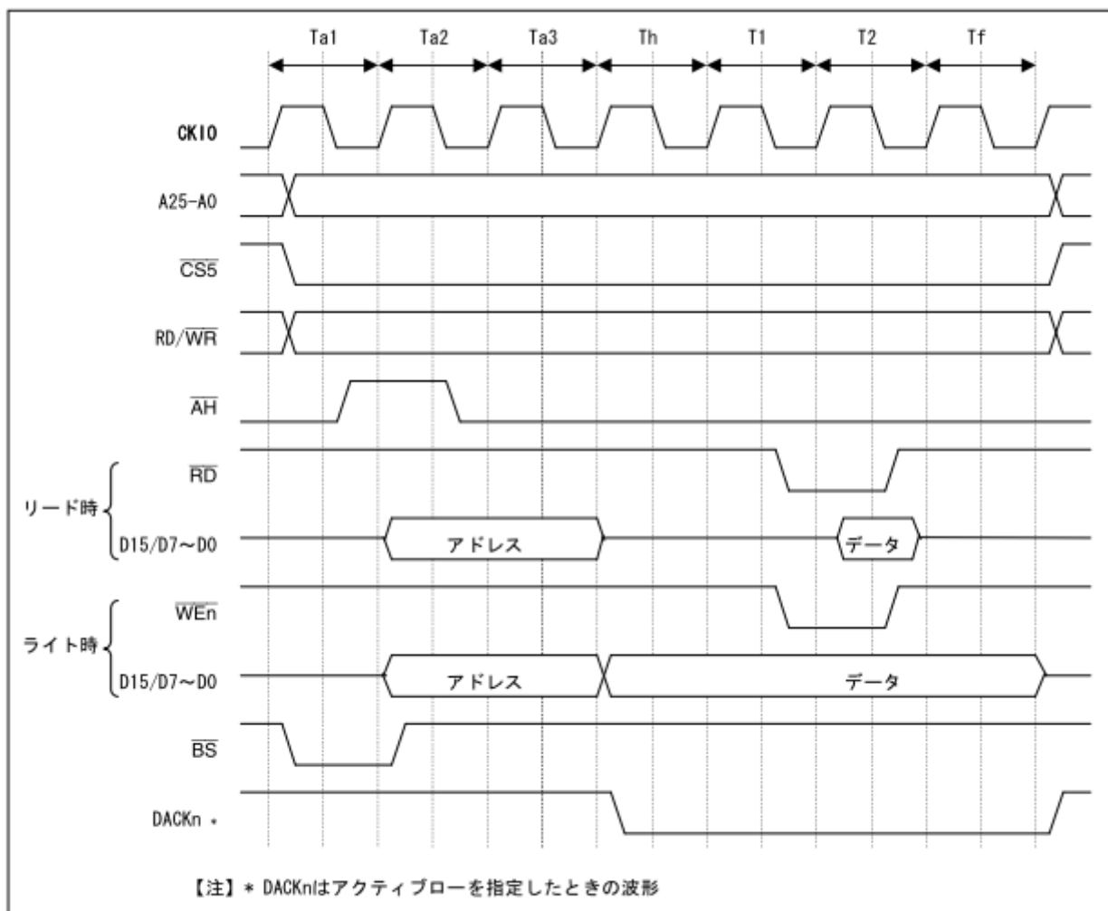
mm (2) MPX空間アクセスタイミング (アドレスサイクルノーウェイト、アサート拡張サイクル1.5、データサイクルノーウェイト、ネゲート拡張サイクル1.5)
