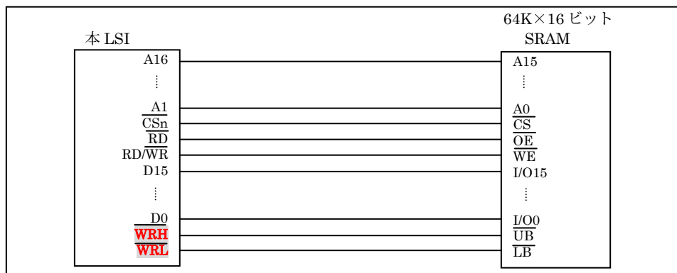
図9.41 16 ビットデータ幅バイト選択付きSRAM 接続例
