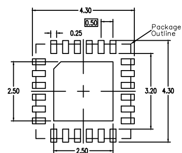
(D1 & P4) 2.50 mm SQ EPAD
