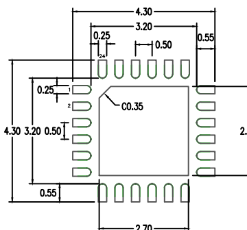
(P6) 2.70 mm SQ EPAD
