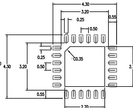
(S4) 2.70 mm SQ EPAD
