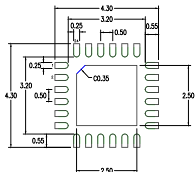
(S1/S2) 2.50 mm SQ EPAD
