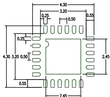
(P1) 2.45 mm SQ EPAD
