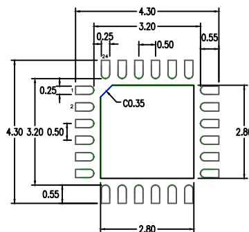
(P2) 2.80 mm SQ EPAD
