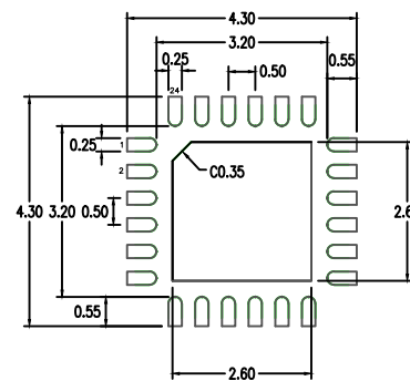
(P3 & S3) 2.60 mm SQ EPAD
