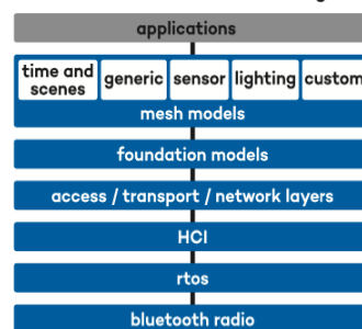
ClarinoxBlue BLE MESH Block Diagram
