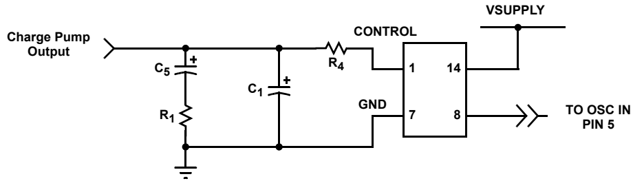
(1) VCXO
