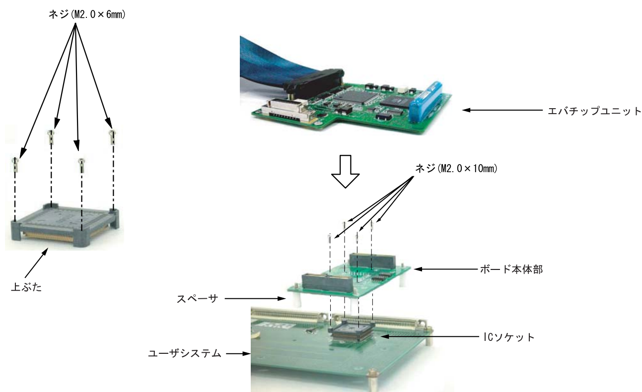
図 1 SH7136 PLQP0080JA-A 用ユーザシステムインタフェースボード
