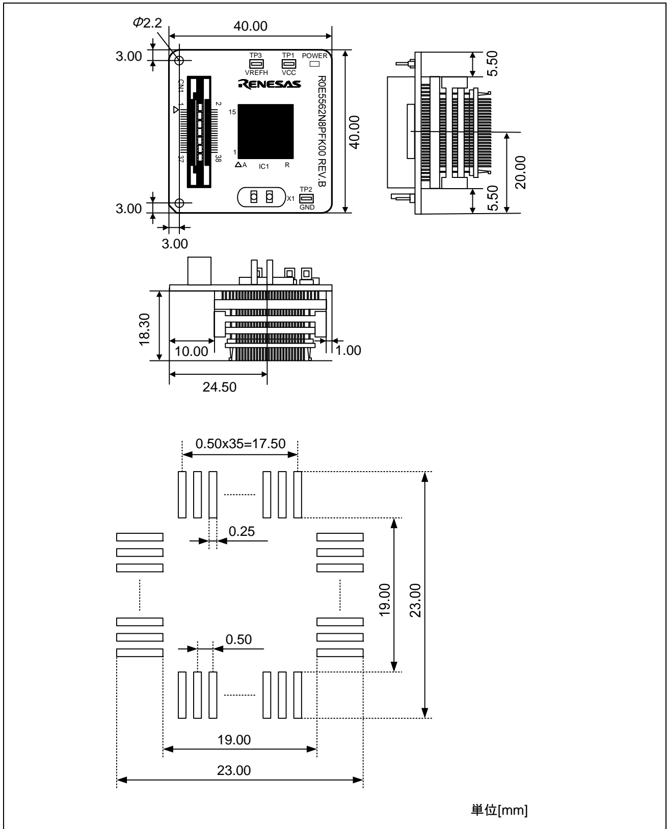
図4 R0E5562N8PFK00 の寸法図及び参考フットパターン
