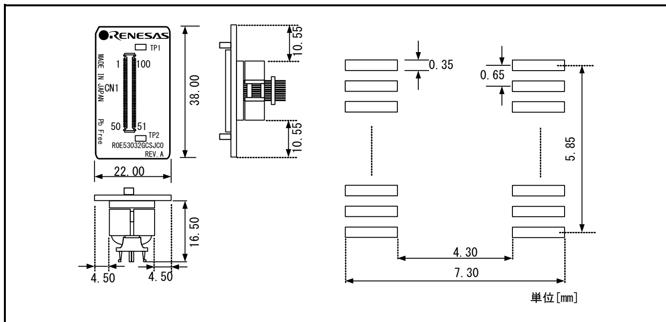
図7.4 R0E53032GCSJC0ユーザシステム接続部の寸法図および参考フットパターン
