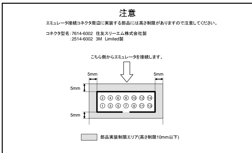
図3 エミュレータ接続基板に対する部品実装制限
