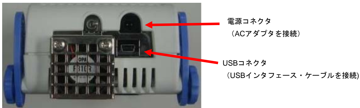
図2-10 コネクタ位置
