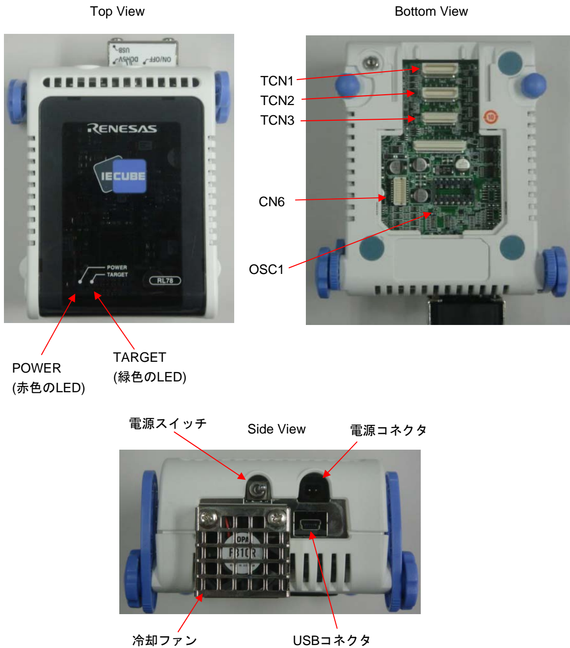
図1-1 QB-RL78G14の各部の名称
