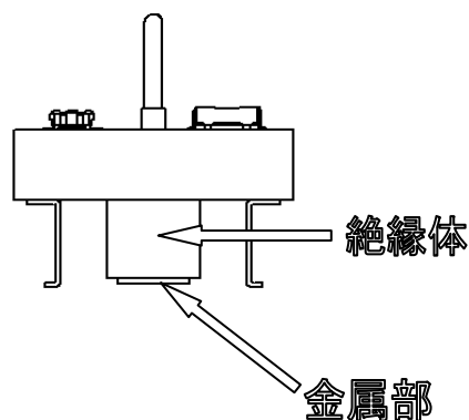
図2-4 TC突起図
