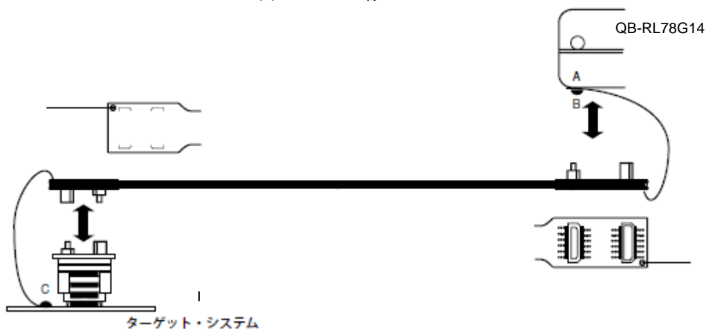
図2-8 GND線
