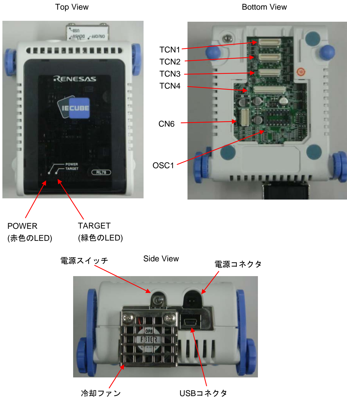
図1-1 QB-RL78F15の各部の名称
