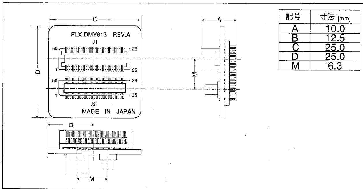
図3 FLX-DMY613の寸法
