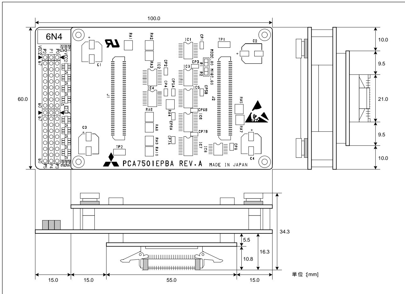
図5.5 エミュレーションプロープ全体寸法図
