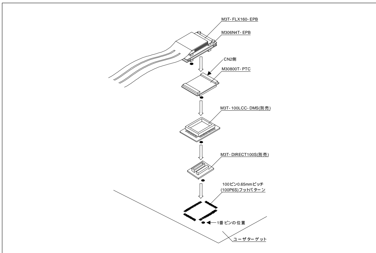
図3.13 100ピン0.65mmピッチフットパターンへの接続(1)
