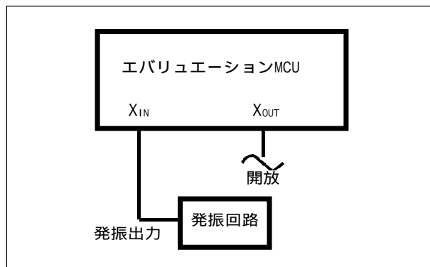
図3.5 ターゲットシステム上発振回路の使用
