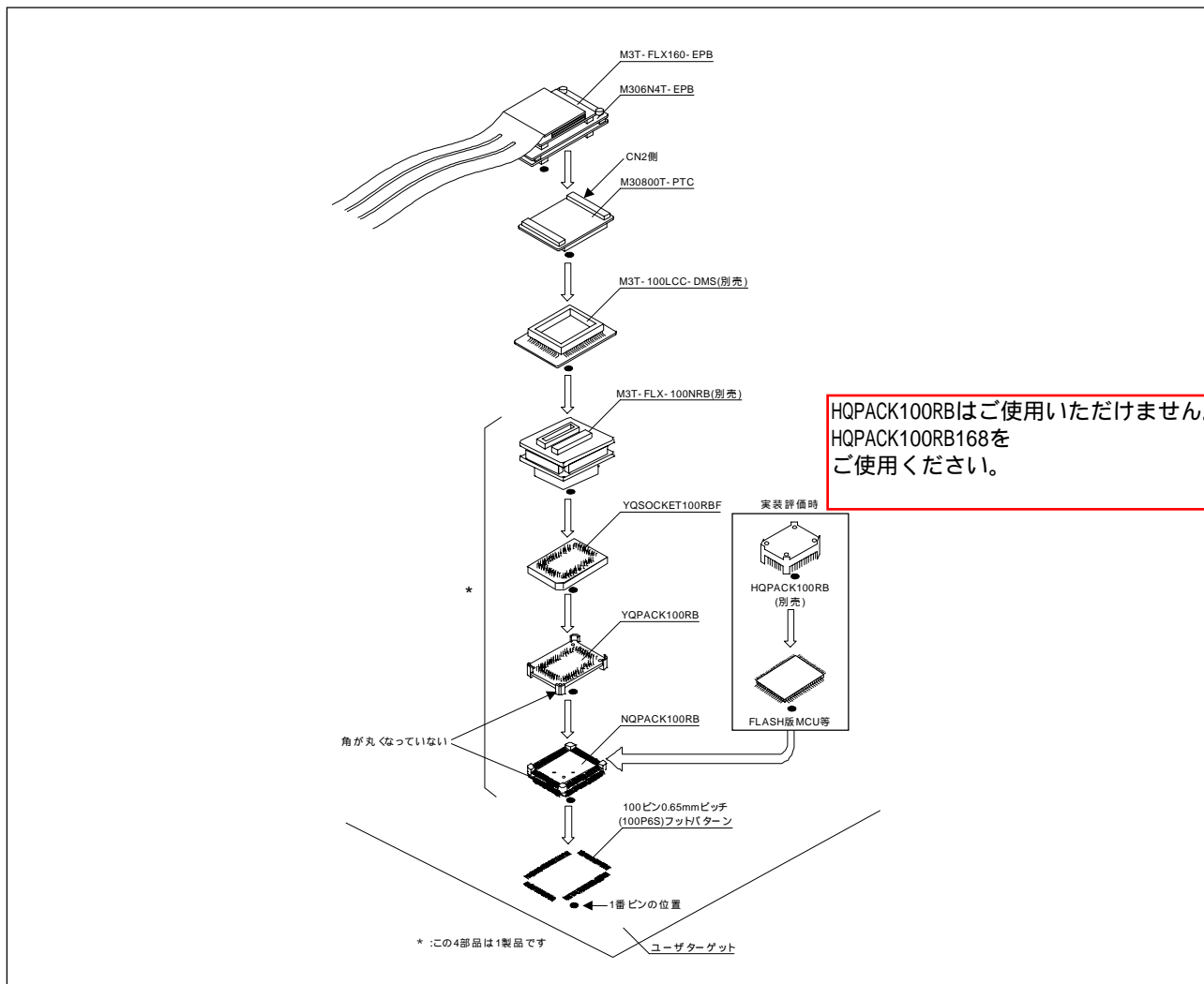
図3.15 100ピン0.65mmピッチフットパターンへの接続(3)
