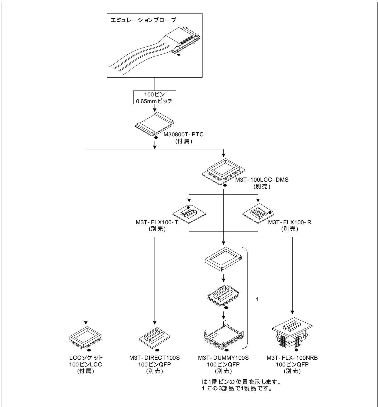
図3.11 本製品とターゲットシステムの接続形態
