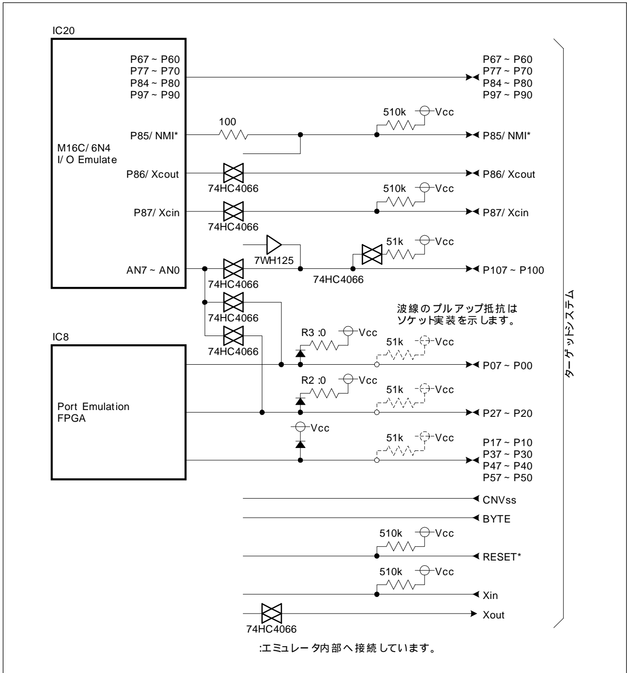
図5.4 接続図
