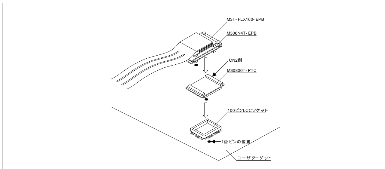
図3.12 100ピンLCCソケットへの接続
