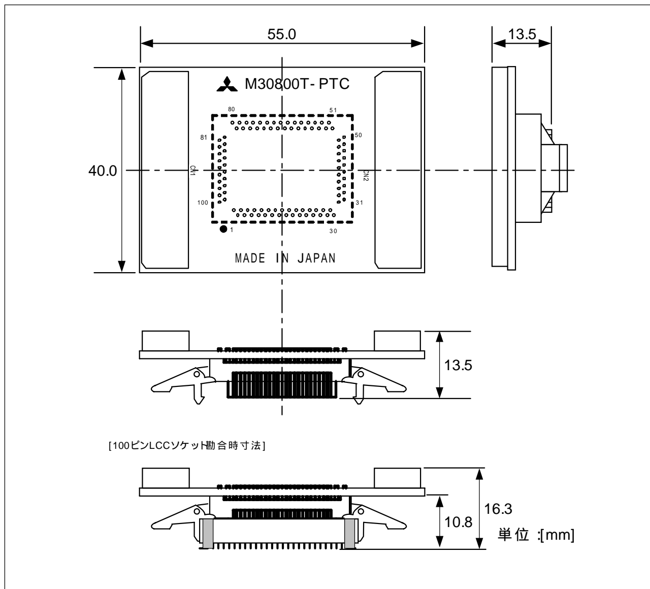
図5.6 変換基板(M30800T-PTC)寸法図
