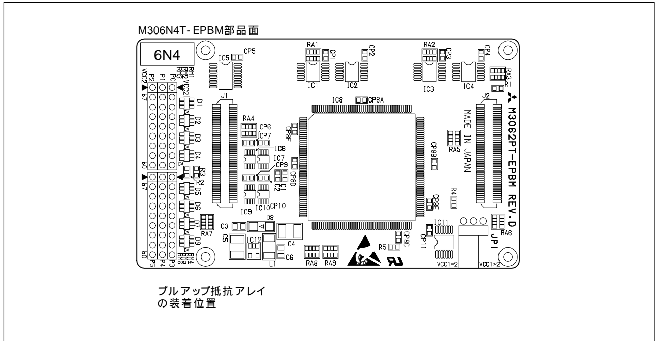
図3.9 プルアップ抵抗アレイの装着位置
