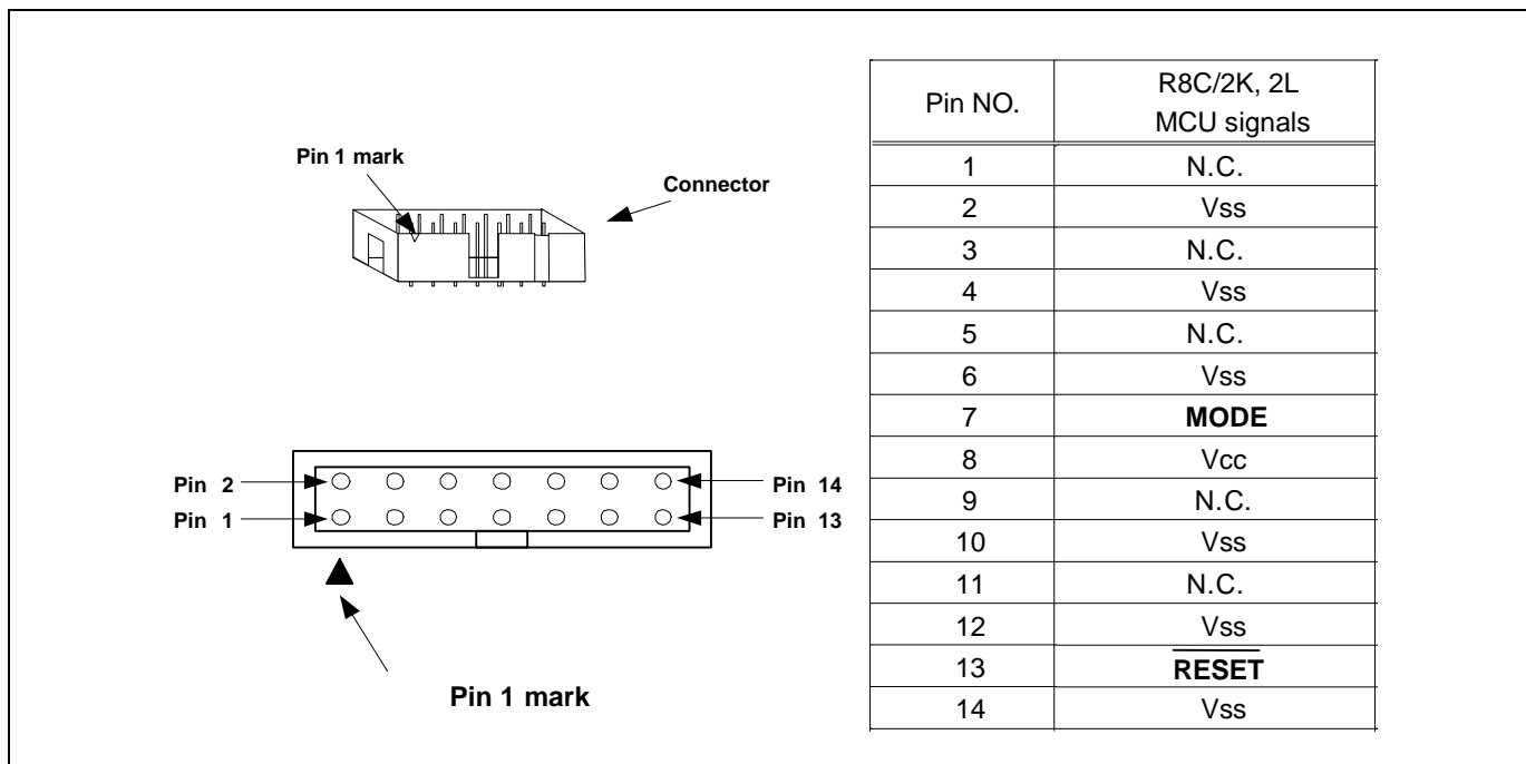
図4.1 E8a 接続コネクタのピン配置
