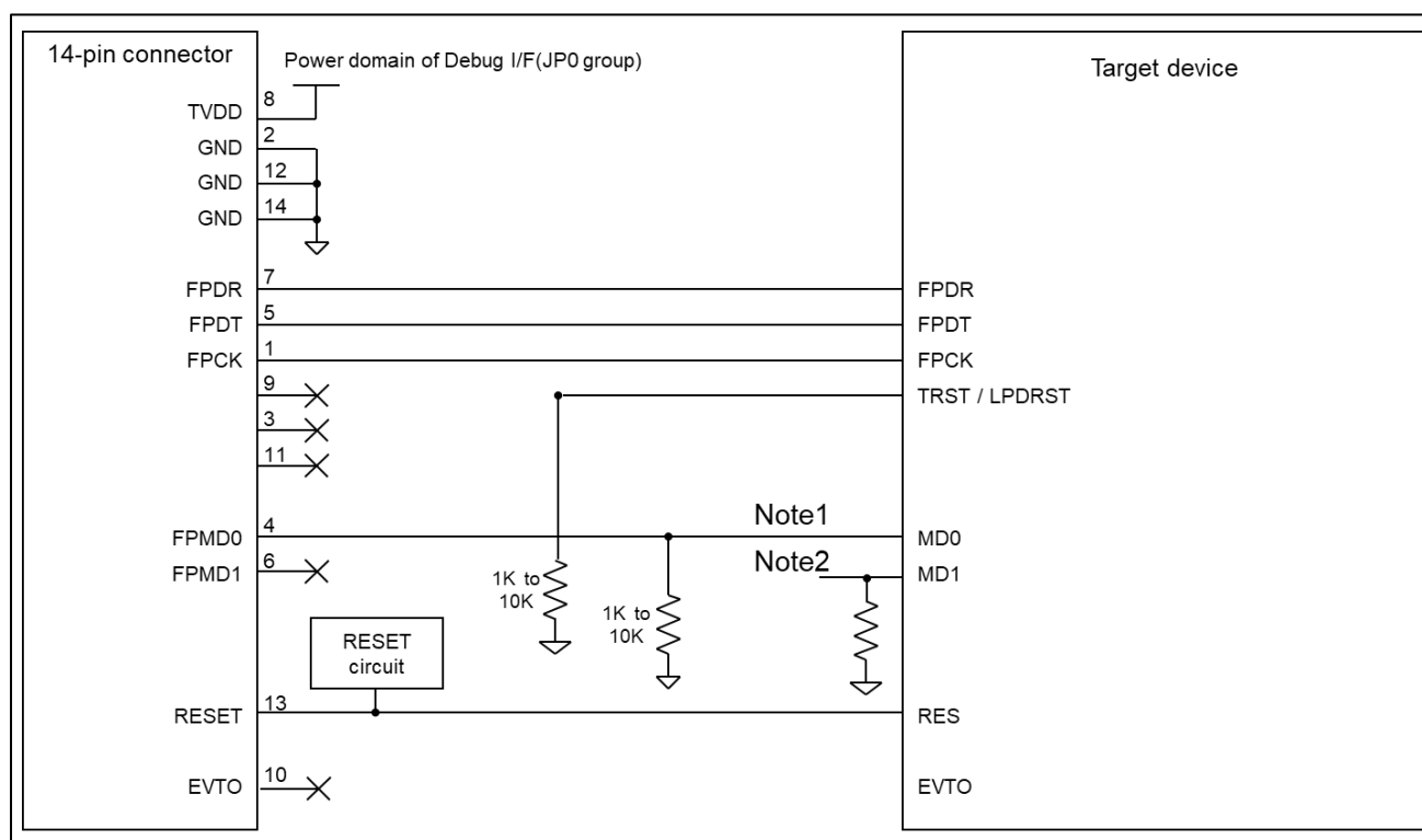
図 2-5 接続例
