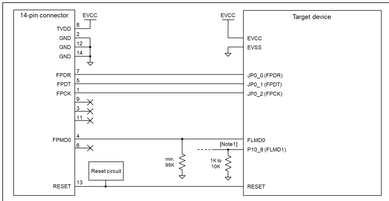
図 2-7 接続例
