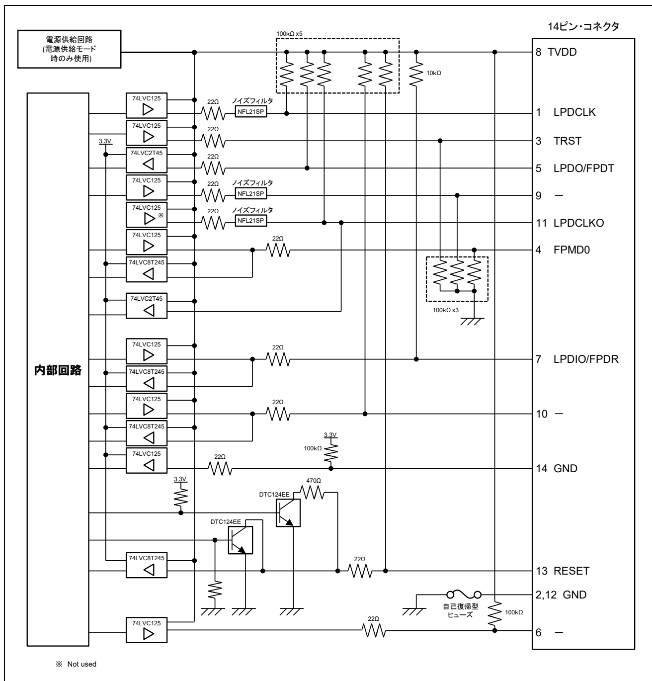
図 5-1 E1/E20 エミュレータ内インタフェース回路(LP1pin、1wireUART)
