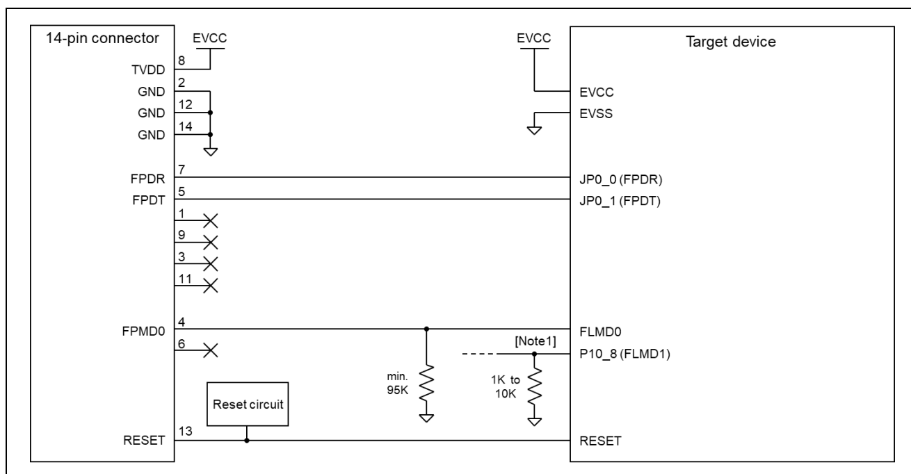
図 2-6 接続例
