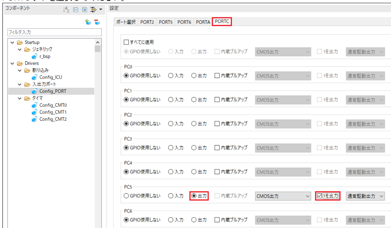
図 4-26 PORTC タブ選択
