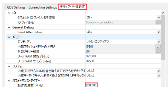
図 6-3 デバッグ・ツール設定
