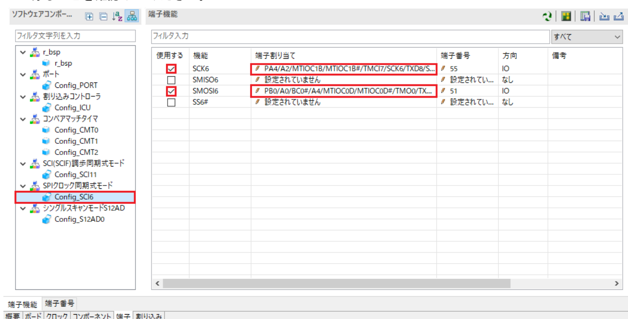
図 4-45 端子設定 - Config_SCI6
