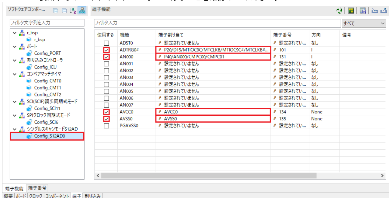
図 4-46 端子設定 - Config_S12AD0
