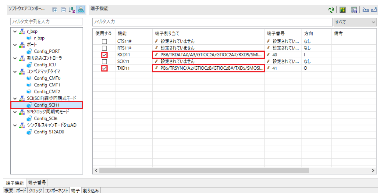
図 4-44 端子設定 - Config_SCI11
