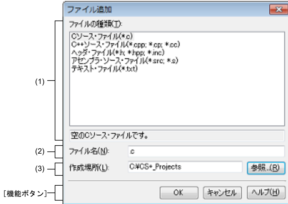
図 A.9 ファイル追加 ダイアログ
