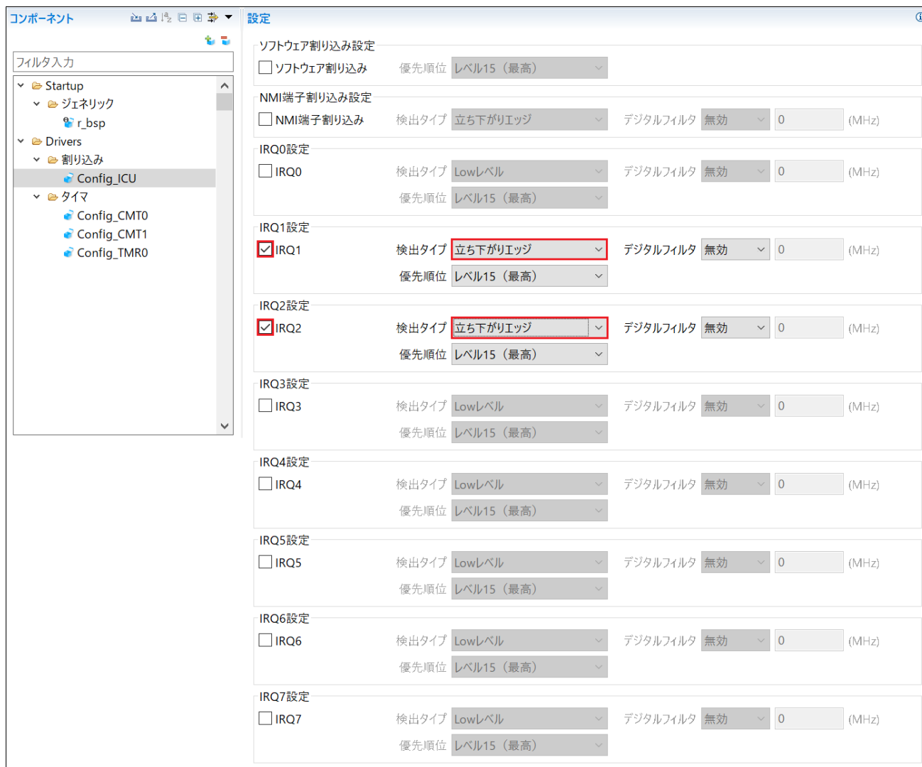
図 4-22: Config_ICU 設定
