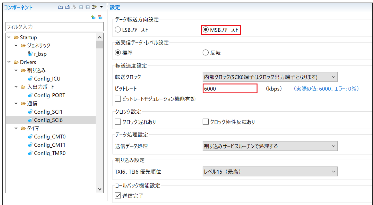
図 4-39: Config_SCI6 設定
