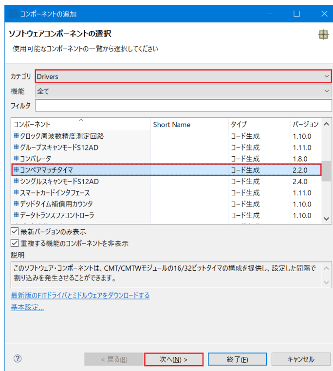
図 4-14: コンペアマッチタイマ選択
