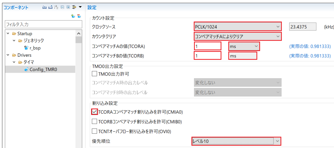
図 4-13: Config_TMR0 設定
