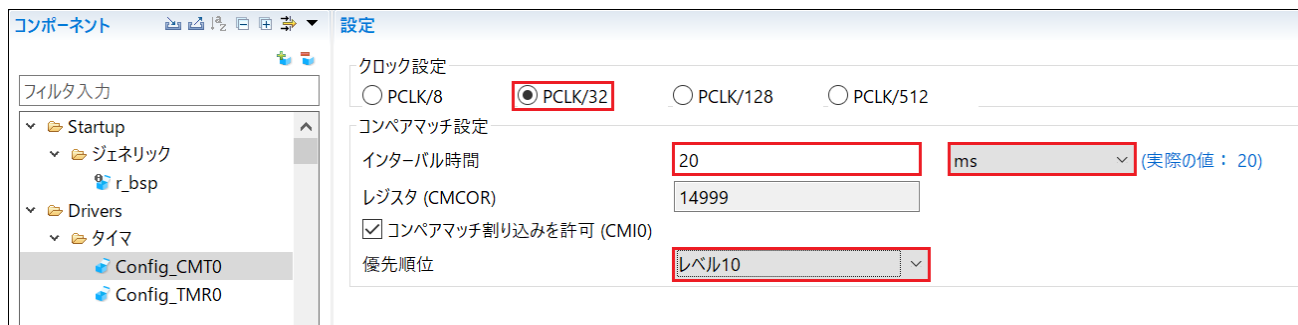
図 4-16: Config_CMT0 設定
