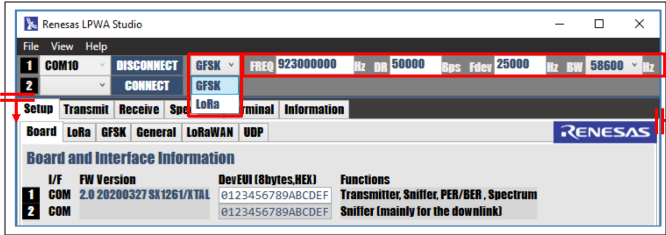
Figure 6. GFSK Parameters
