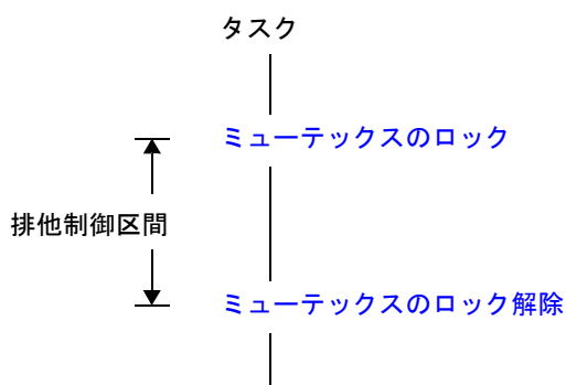
図 7-1 処理の流れ（ミューテックス）
