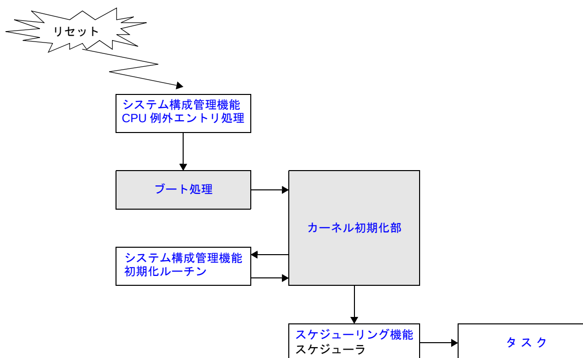
図 15 - 1 処理の流れ（システム初期化処理）
