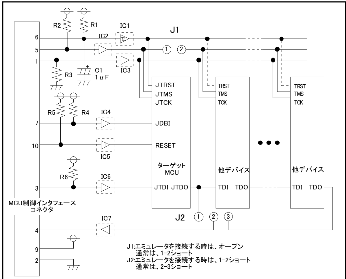
図 3.4 SDI MCU 制御インタフェース回路例
