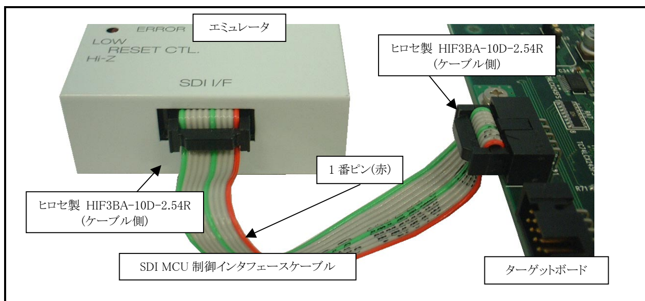
図 3.3 SDI インタフェースケーブルの接続方法
