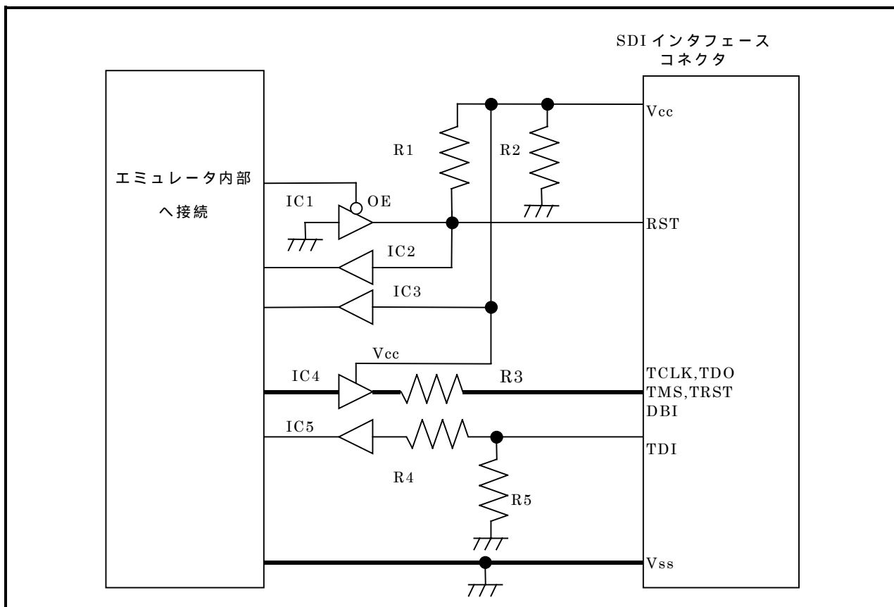
図 3.5 SDI インタフェース部エミュレータ側回路図
