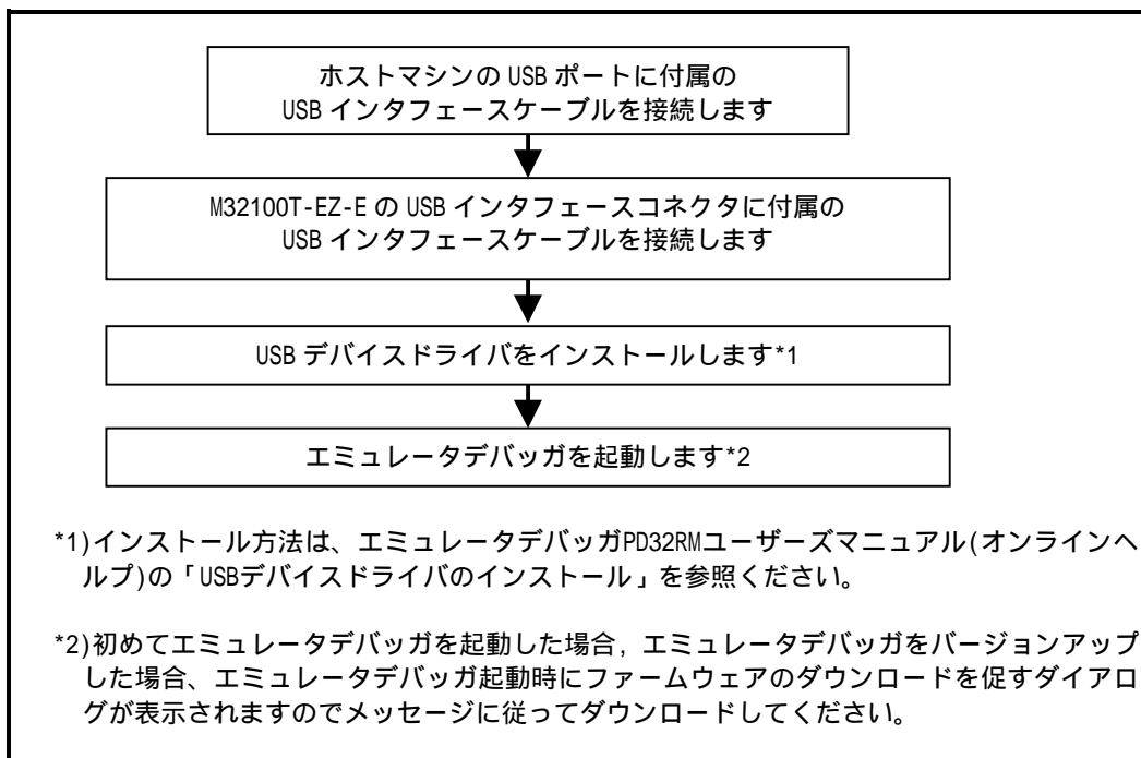
図 3.2 USB インタフェースの接続手順
