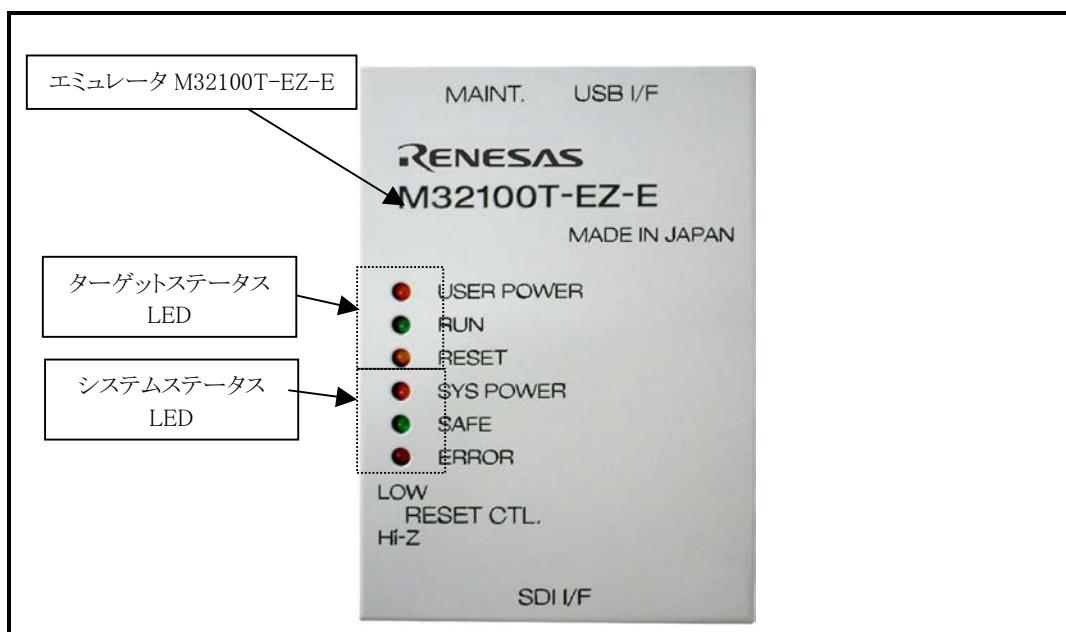
図 2.2 上面パネルの名称
