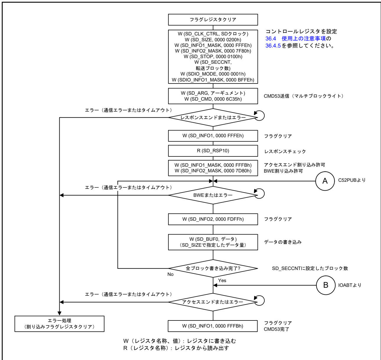
図 36.20 CMD53 マルチブロックライト動作時の IO_RW_EXTENDED コマンドの例
