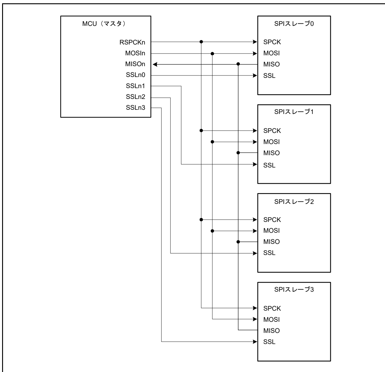
図 32.11 シングルマスタとマルチスレーブの構成例 (MCU はマスタ)
