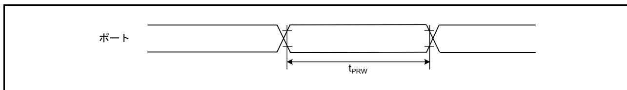
図 50.47 I/Oポート入力タイミング
