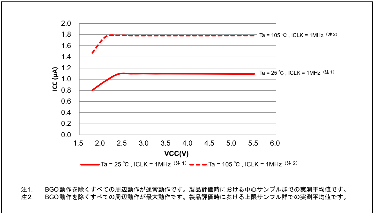
図 50.19 Low-speed モードにおける電圧依存性 (参考データ)
