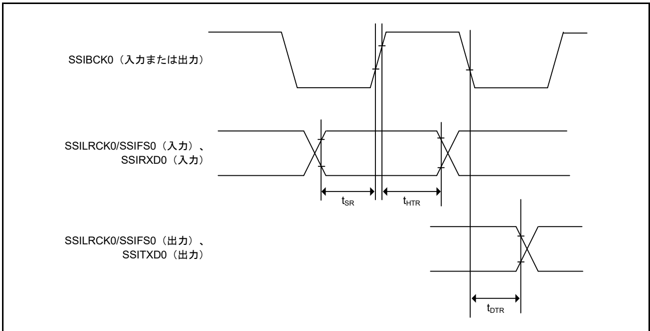
図 50.72 SSIE データ送受信タイミング (SSICR.BCKP = 0)
