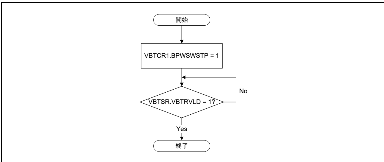
図 12.2 VBTCR1.BPWSWSTP ビットの設定フロー
