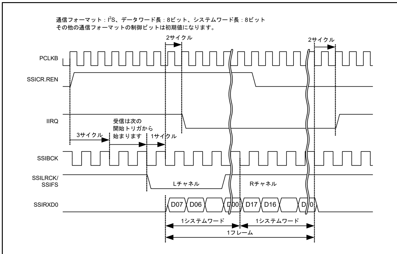
図 35.13 IIRQ 設定タイミング (受信)
