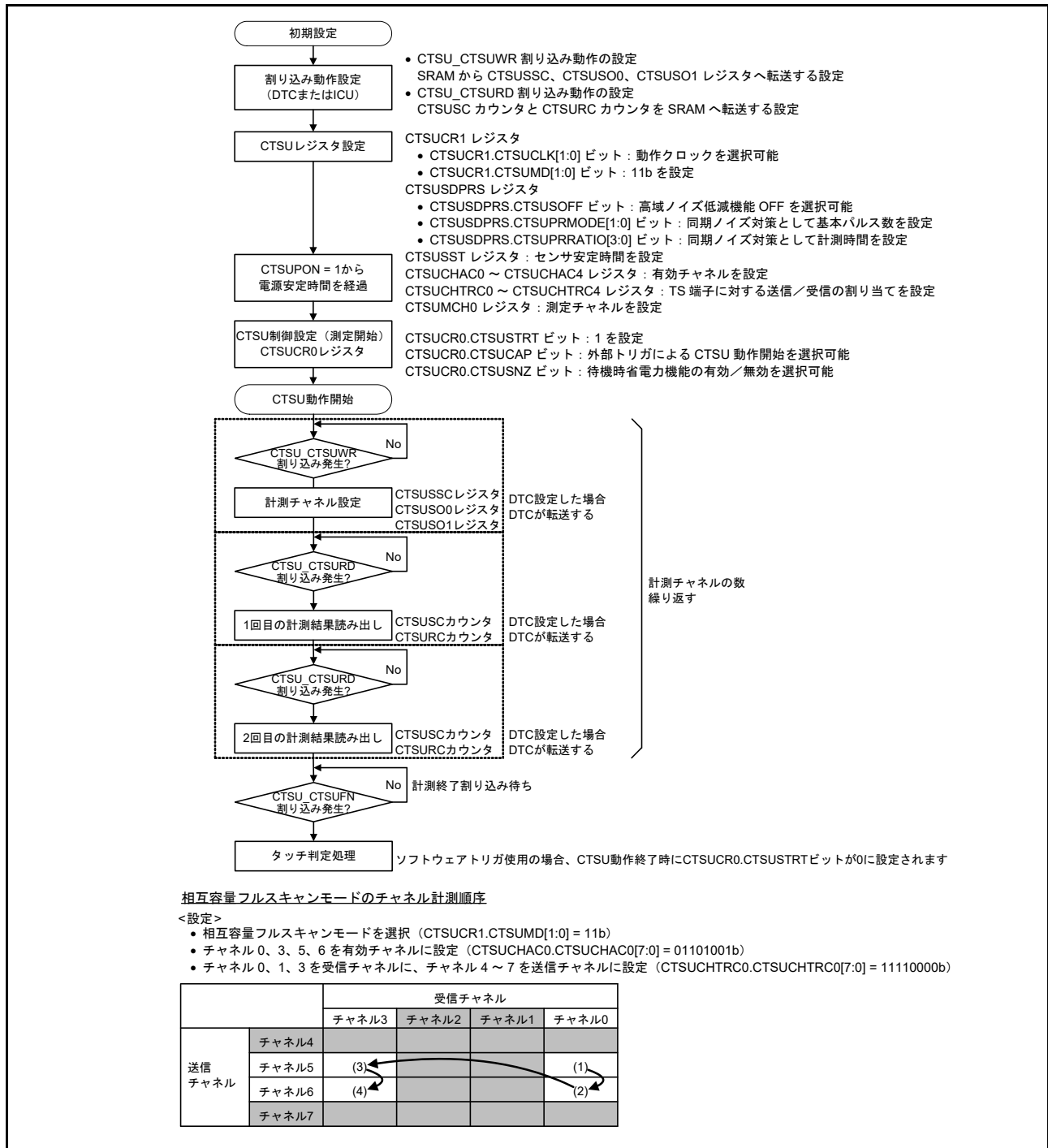
図 44.16 相互容量フルスキャンモードのソフトウェアフローと動作例
