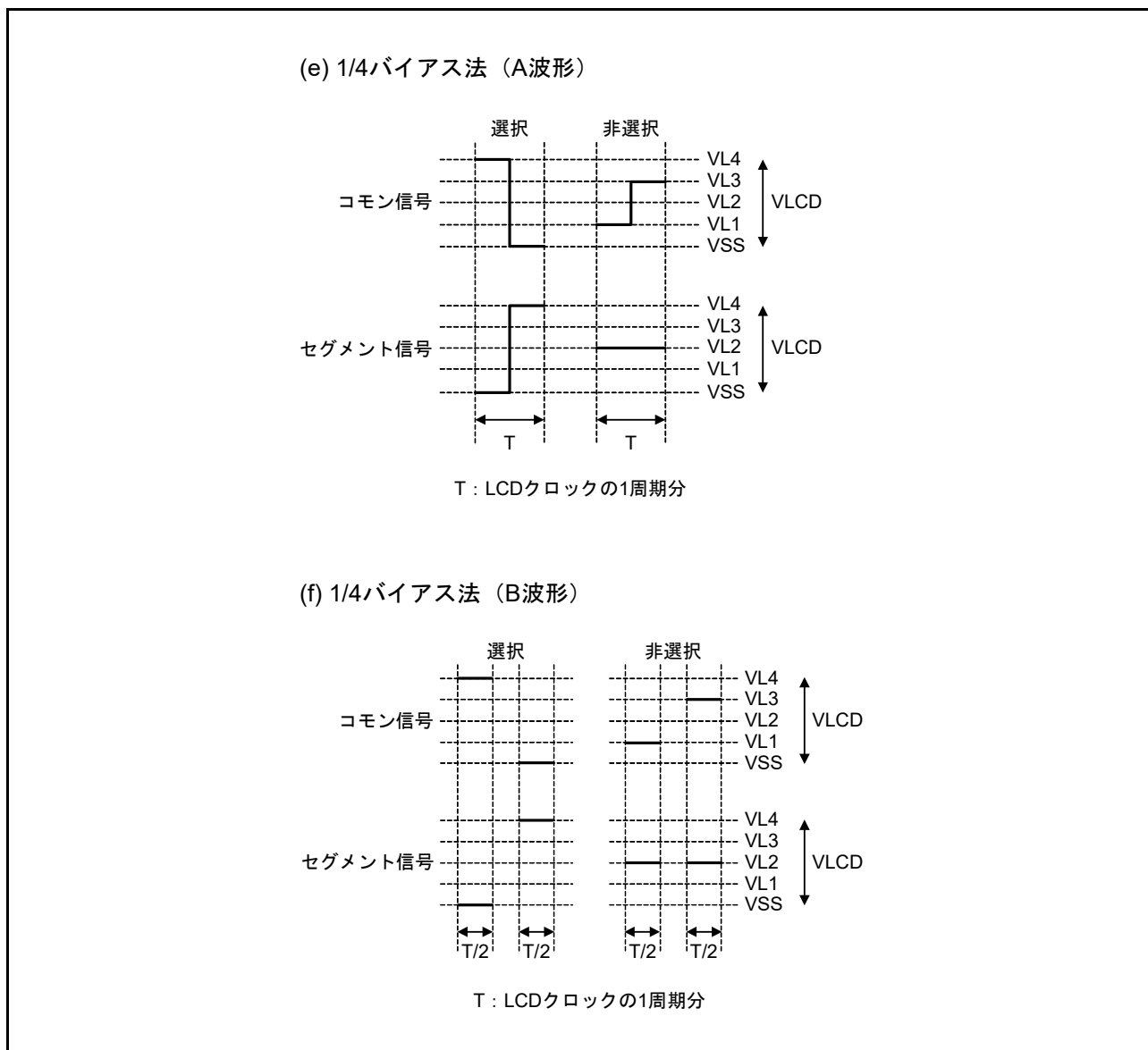
図 48.17 コモン信号とセグメント信号の電圧と位相 (3/3)
