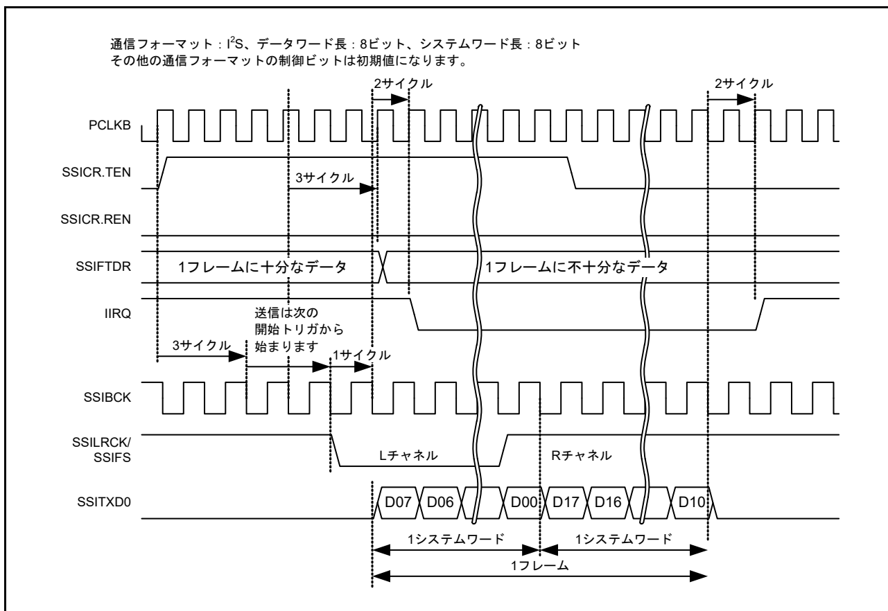
図 35.12 IIRQ 設定タイミング (送信)
