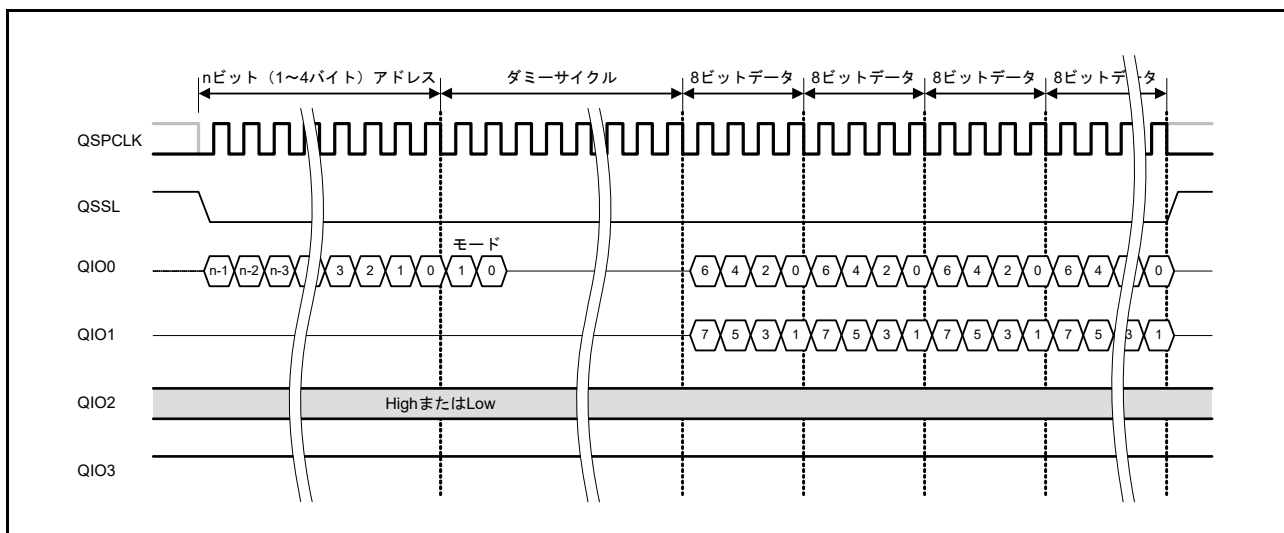
図 33.20 XIP モード時のファストリード Dual 出力バスサイクル
