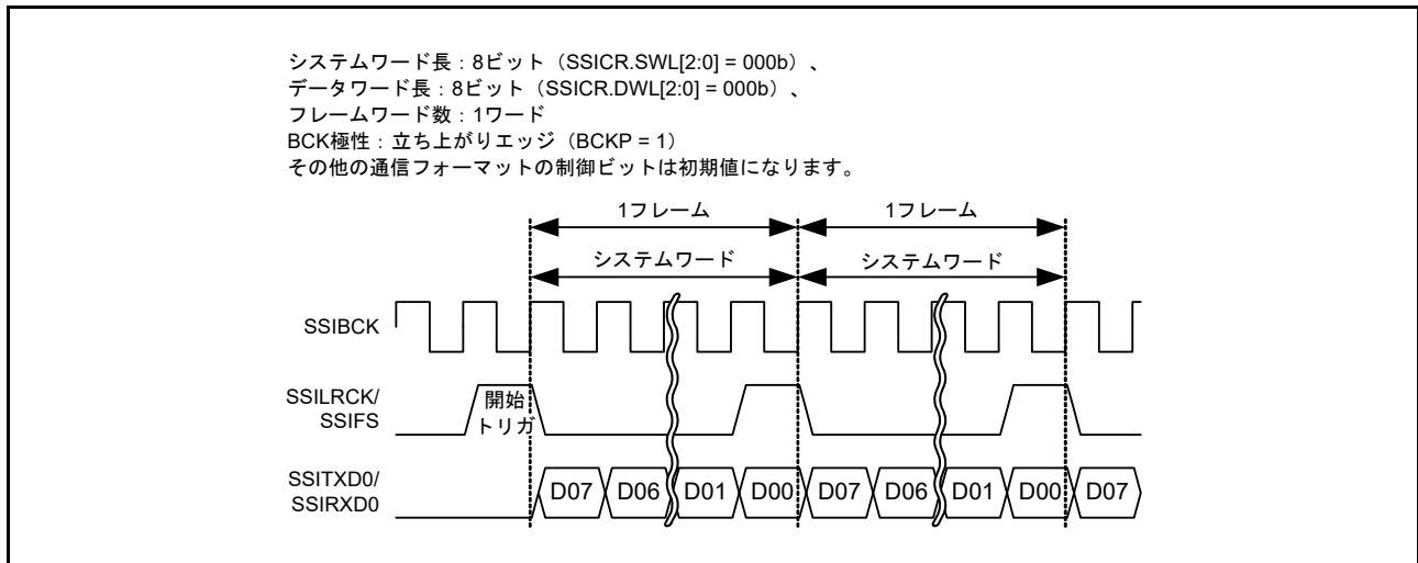
図 35.36 モノラルフォーマットでのショートフレーム (パディングなし、システムワード長 = データワード長)
