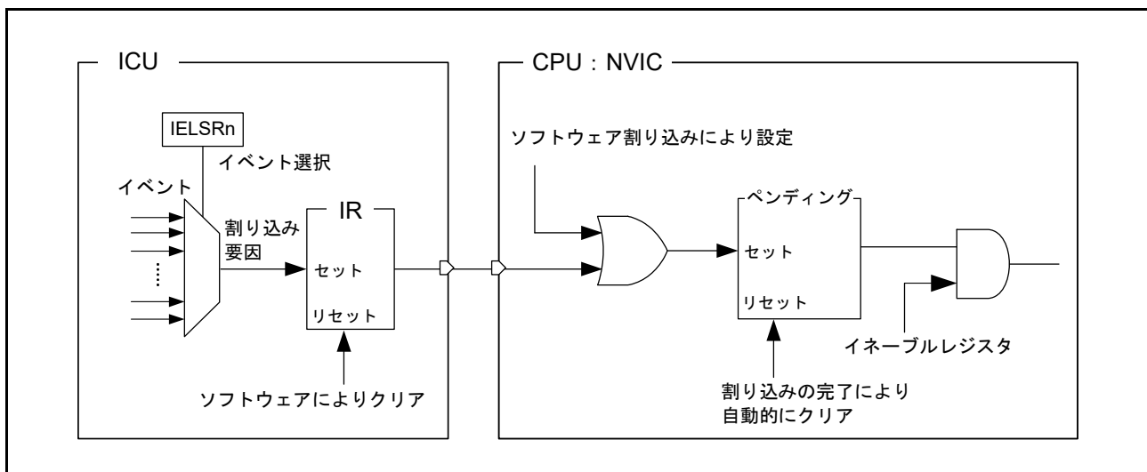
図 14.2 ICU, CPU: NVIC の割り込み経路
