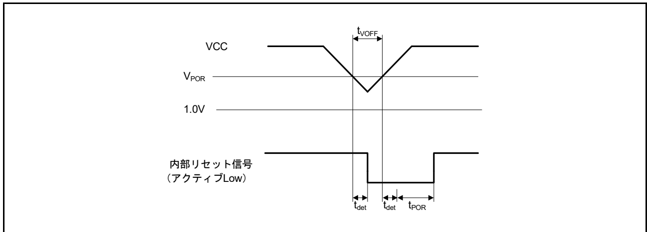
図 50.85 電圧検出リセットタイミング
