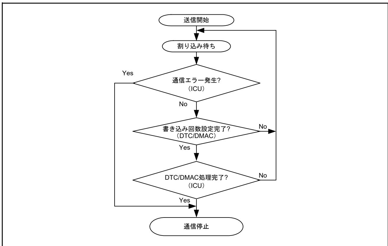
図 35.50 送信手順
