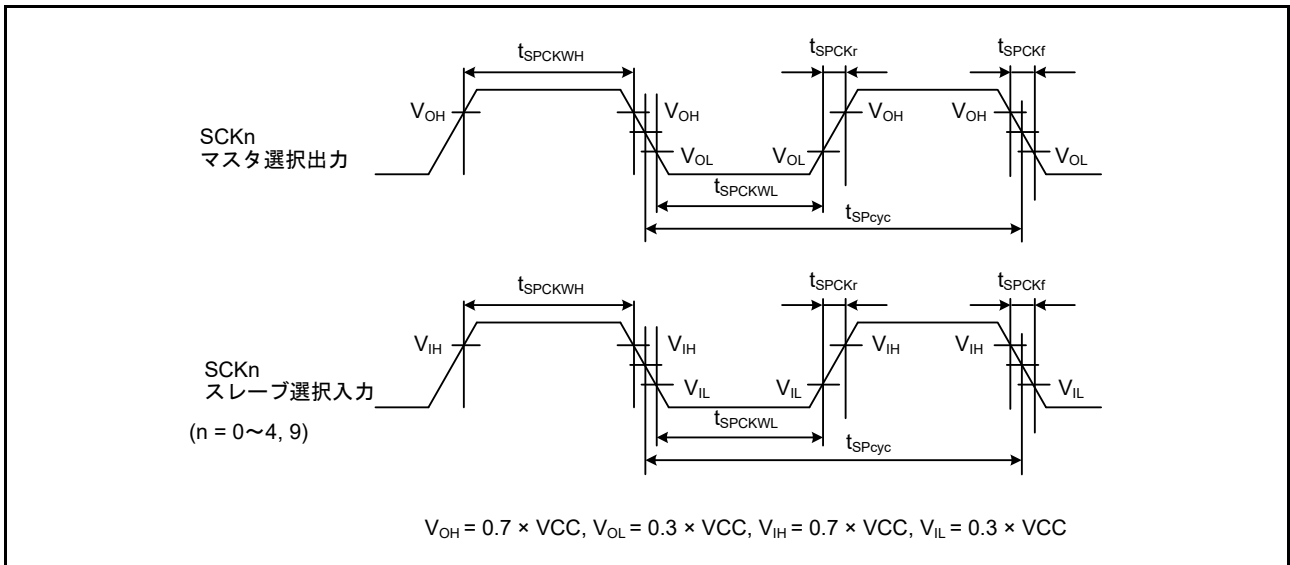
図 50.55 SCI 簡易 SPI モードクロックタイミング
