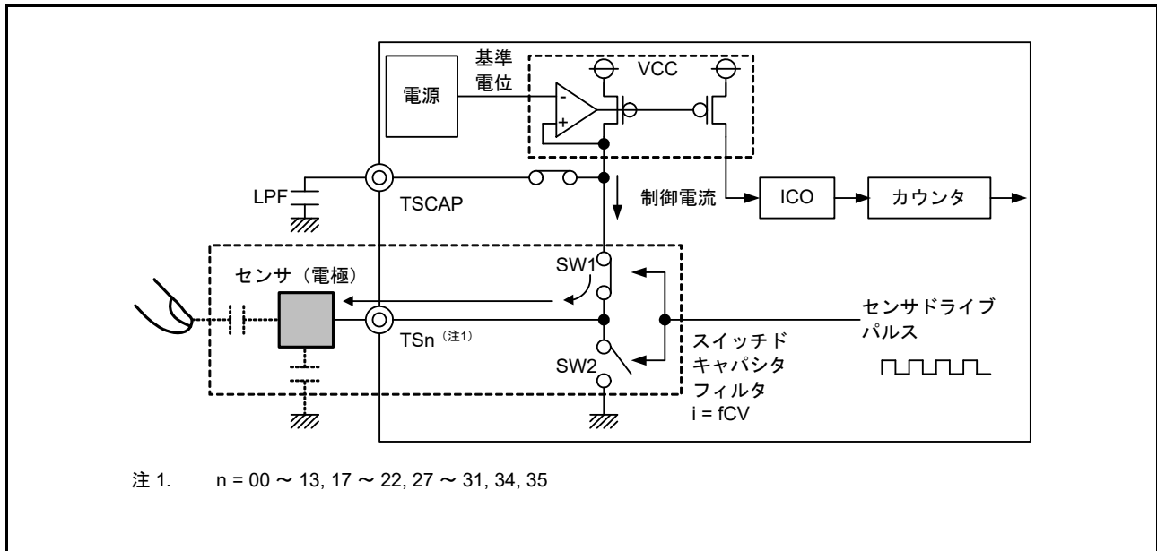
図 44.5 充電動作
