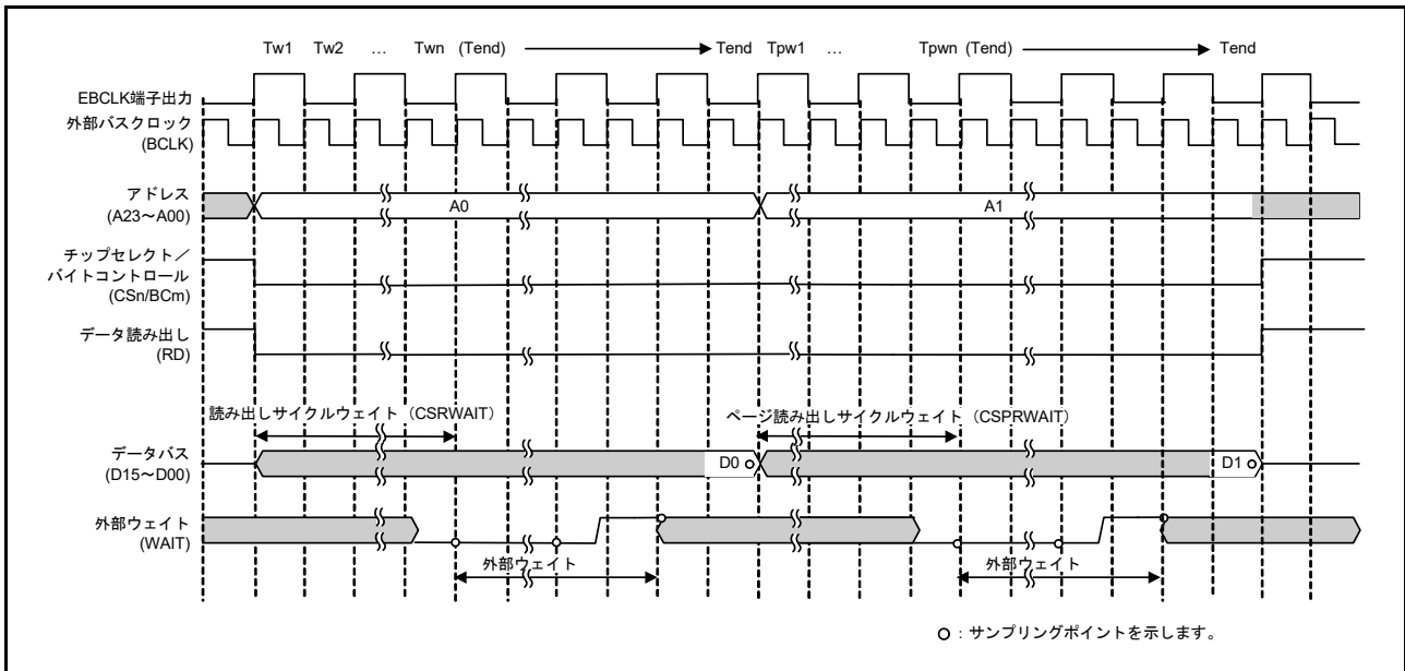
図 15.27 16 ビットバス空間に対するページリードアクセスの外部ウェイトタイミング例 (EBCLK 端子出力選択ビットで BCLK の 2 分周を選択した場合) ( n = 0 \sim 3, m = 0, 1 )
