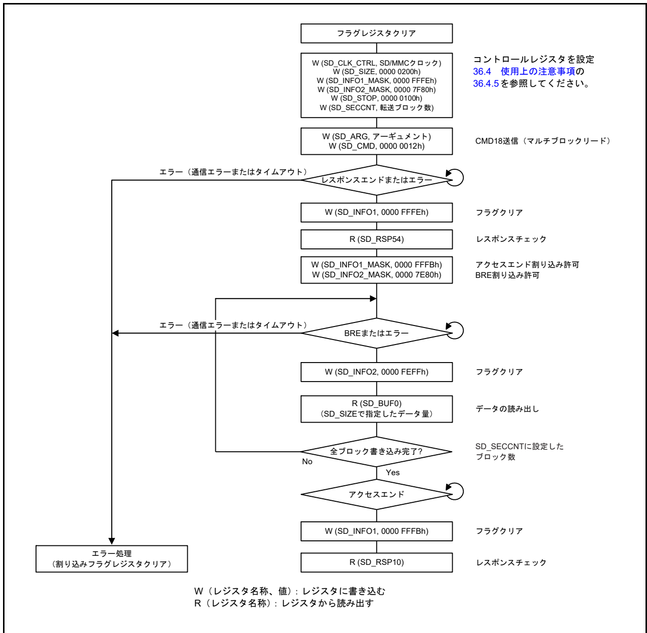
図 36.13 マルチブロックリード動作のフロー例
