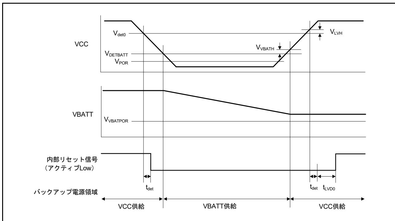
図 50.90 電源切り替えおよびLVD0リセットタイミング
