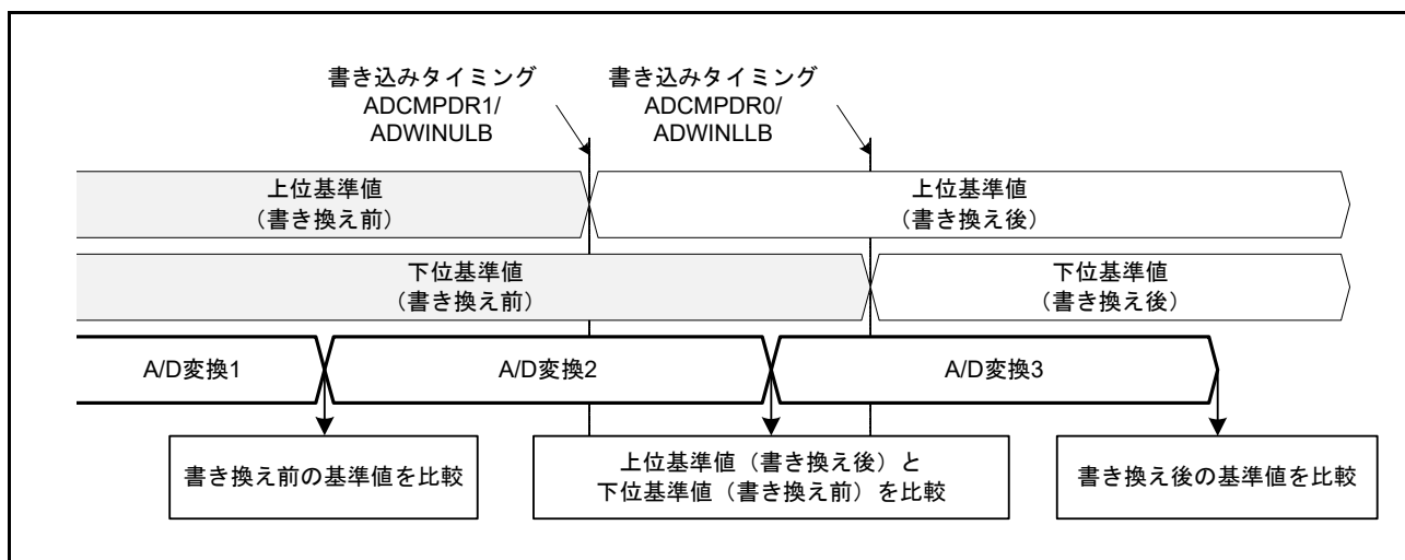
図 38.4 書き換え前後の上側基準値と下側基準値の比較
