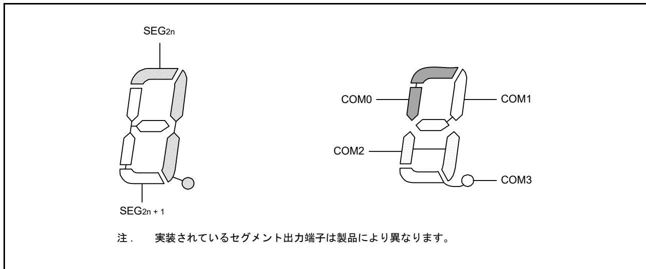
図 48.28 4 時分割 LCD 表示パターンと電極接続
