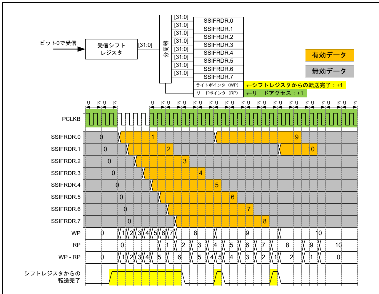
図 35.30 受信 FIFO データレジスタと受信シフトレジスタの構成例および FIFO 動作例
