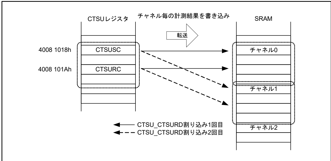
図 44.20 CTSU_CTSURD 割り込みを用いた DTC 転送動作例
