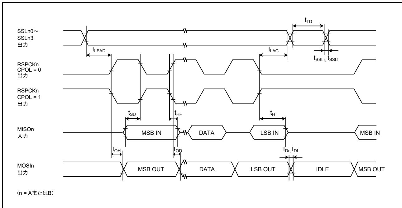
図 50.65 SPI タイミング (マスタ、CPHA = 1) (ビットレート : PCLKA を 2 分周に設定)
