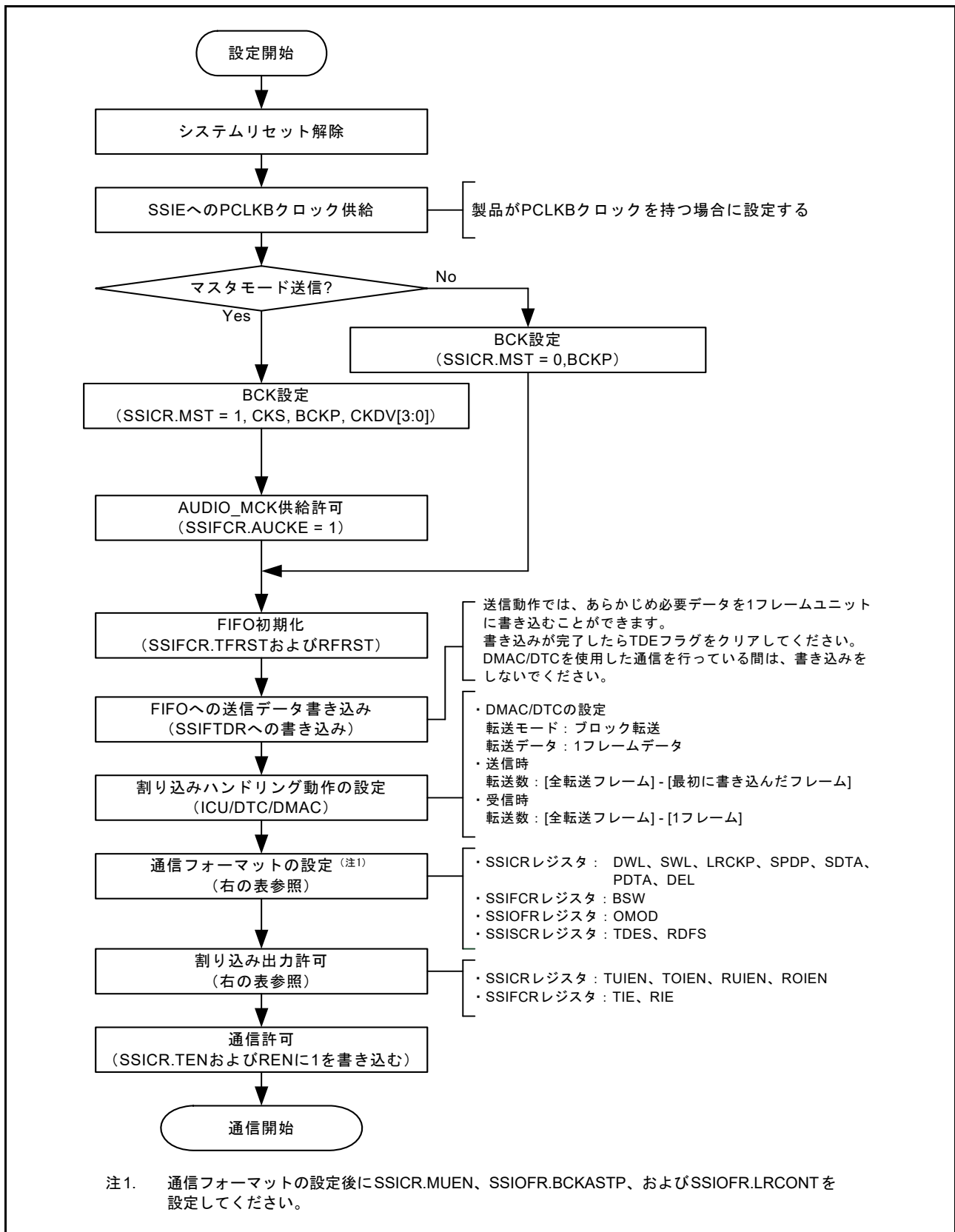
図 35.49 通信開始手順 (CPU 動作手順)
