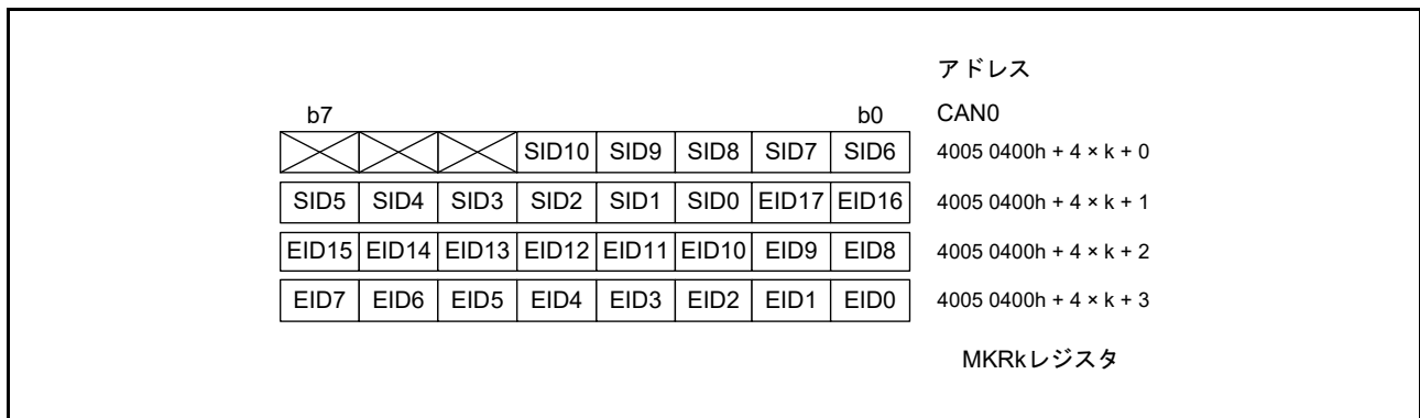
図 31.14 MKR k レジスタの構成 (k = 0 ~ 7)
