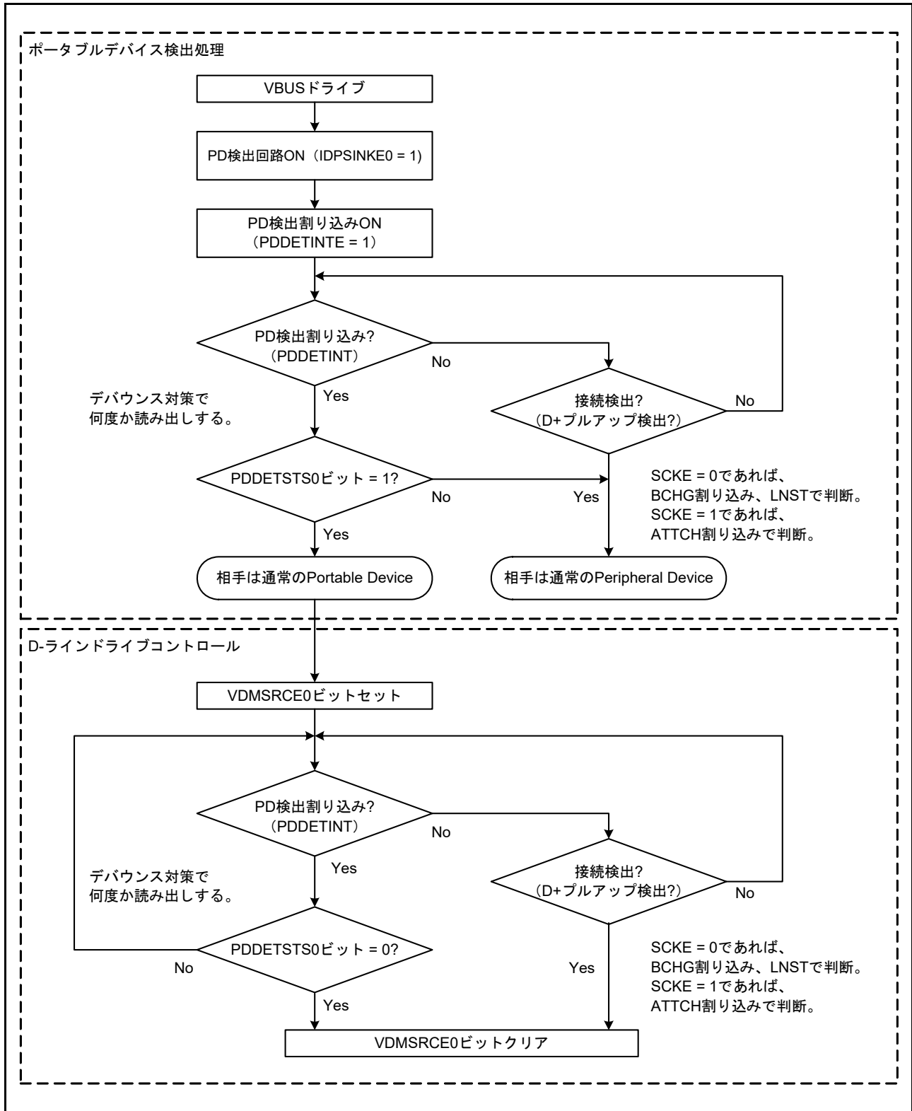
図 28.25 チャージングダウンストリームポートとして動作する場合の処理フロー (ステップ 1～4)
