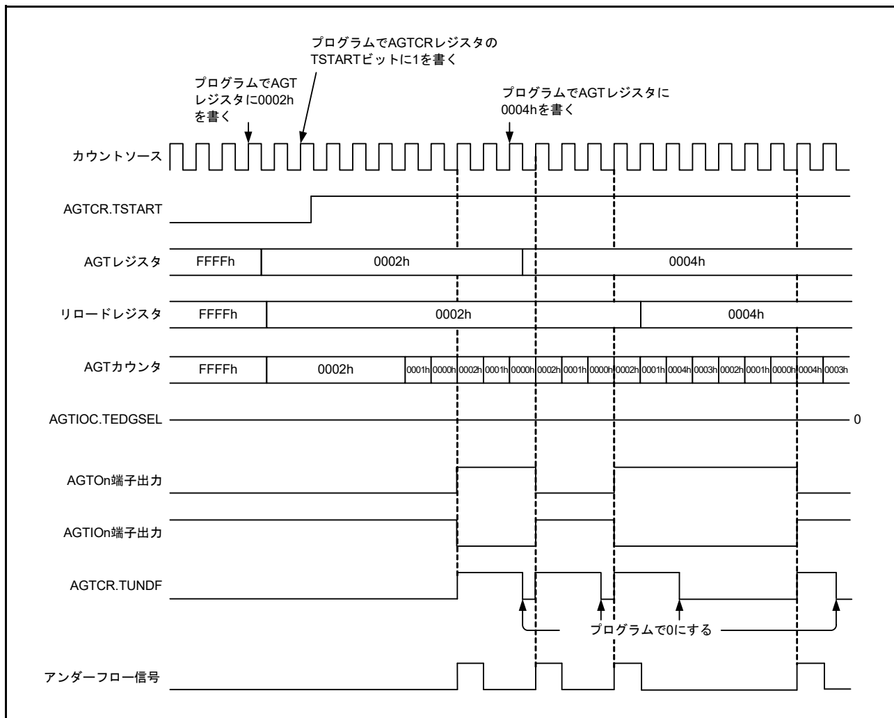
図 24.6 パルス出力モードでの動作例
