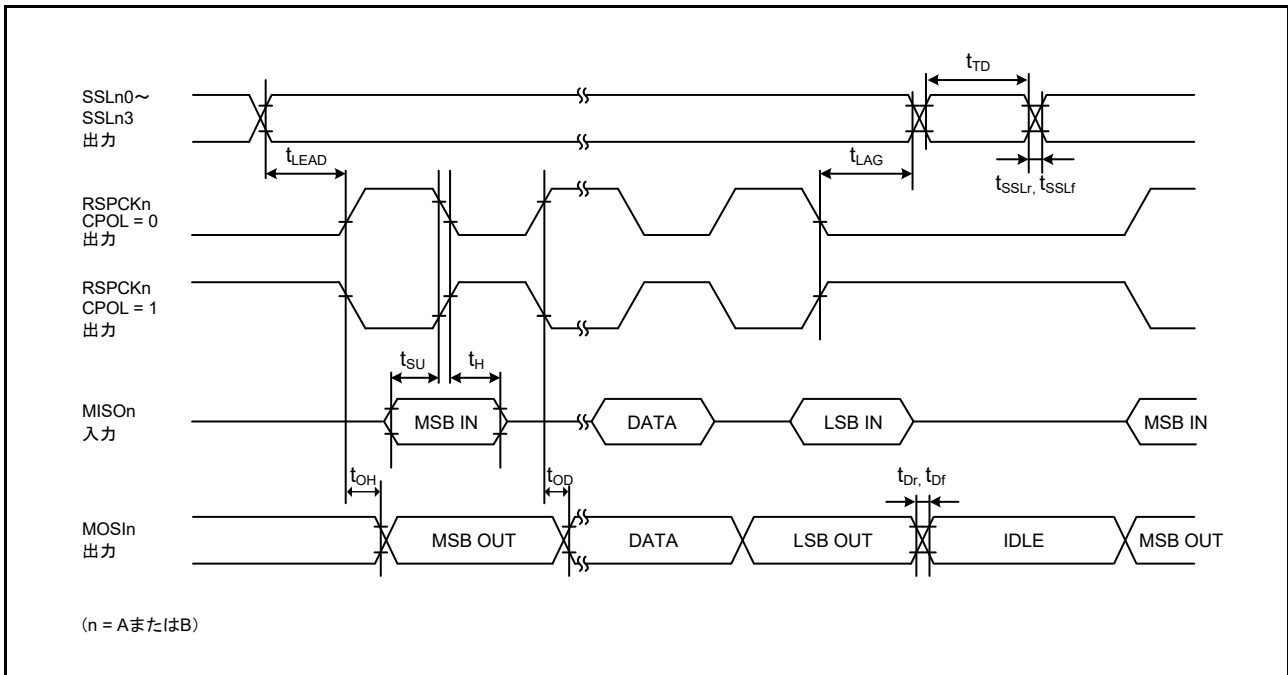
図 50.64 SPI タイミング (マスタ、CPHA = 1) (ビットレート : PCLKA を 2 分周以外に設定)
