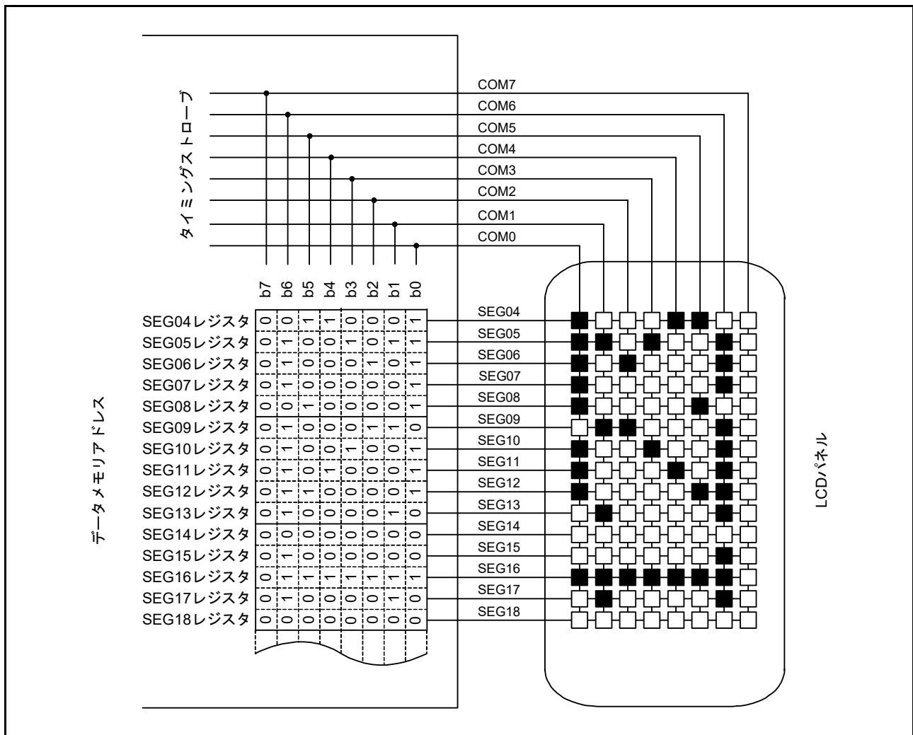
図 48.33 8 時分割 LCD パネルの接続例
