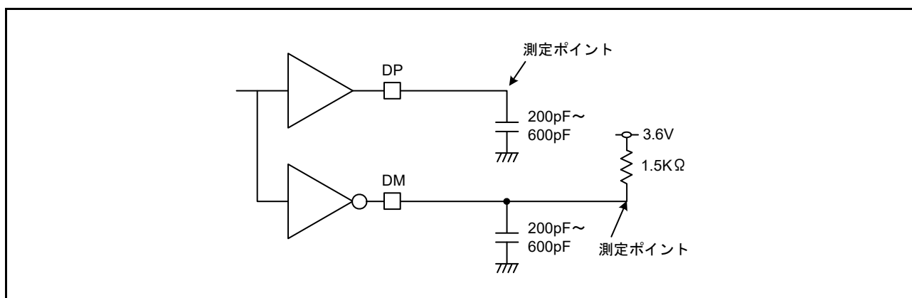
図 50.79 ロースピード (LS) 接続の測定回路
