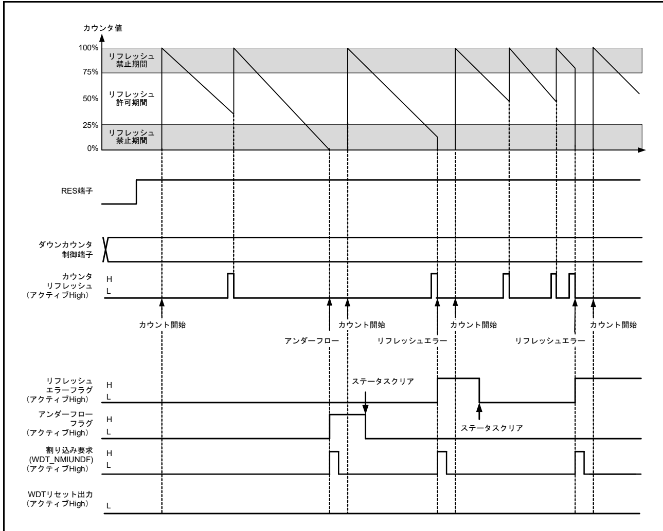
図 26.4 オートスタートモードでの動作例
