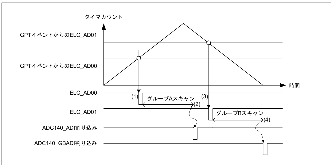
図 38.13 グループスキャンモードの基本動作例 (ELC からの同期トリガ)
