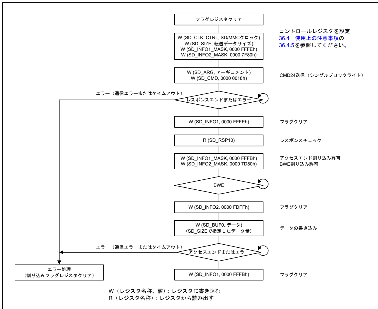
図 36.12 シングルブロックライト動作のフロー例
