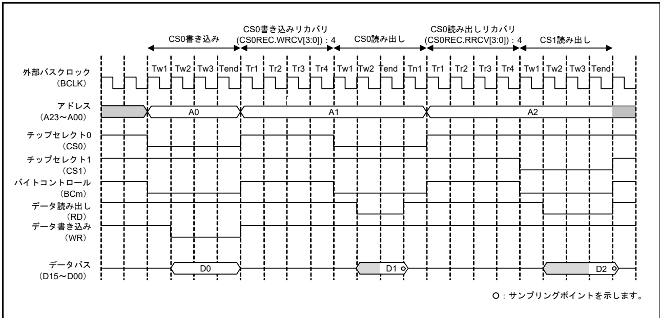
図 15.31 セパレートバスインタフェース時のリカバリサイクルの挿入例 (m = 0, 1)
