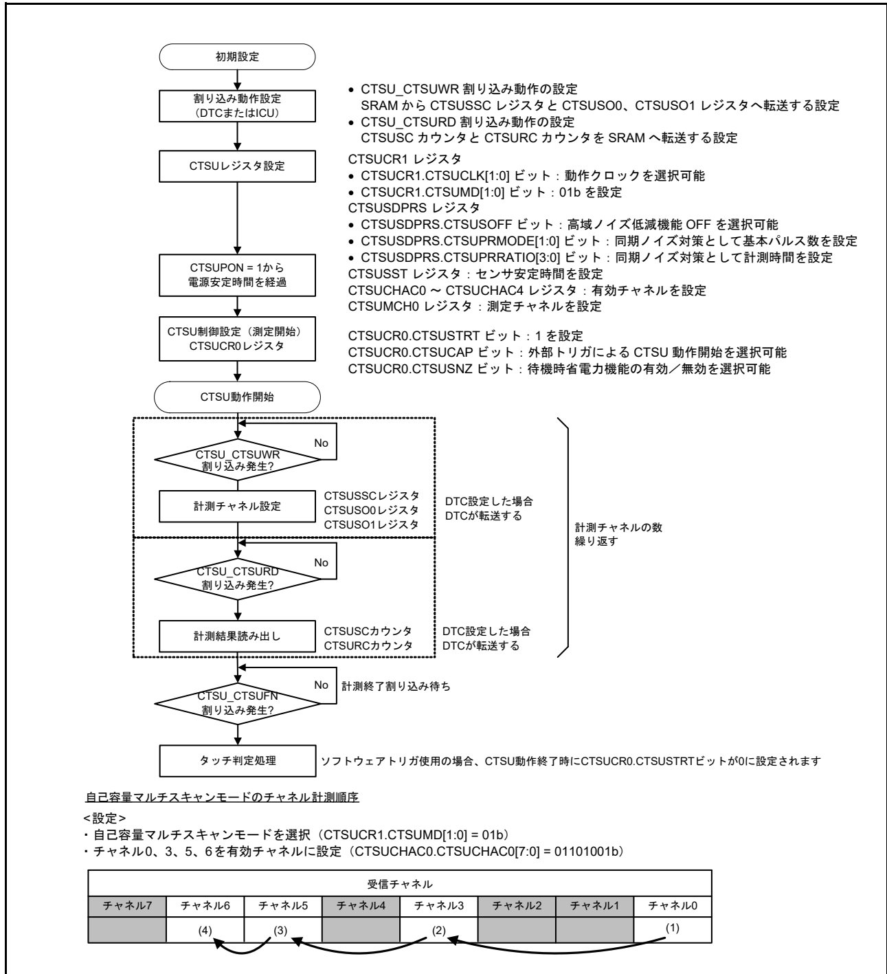
図 44.14 自己容量マルチスキャンモードのソフトウェアフローと動作例
