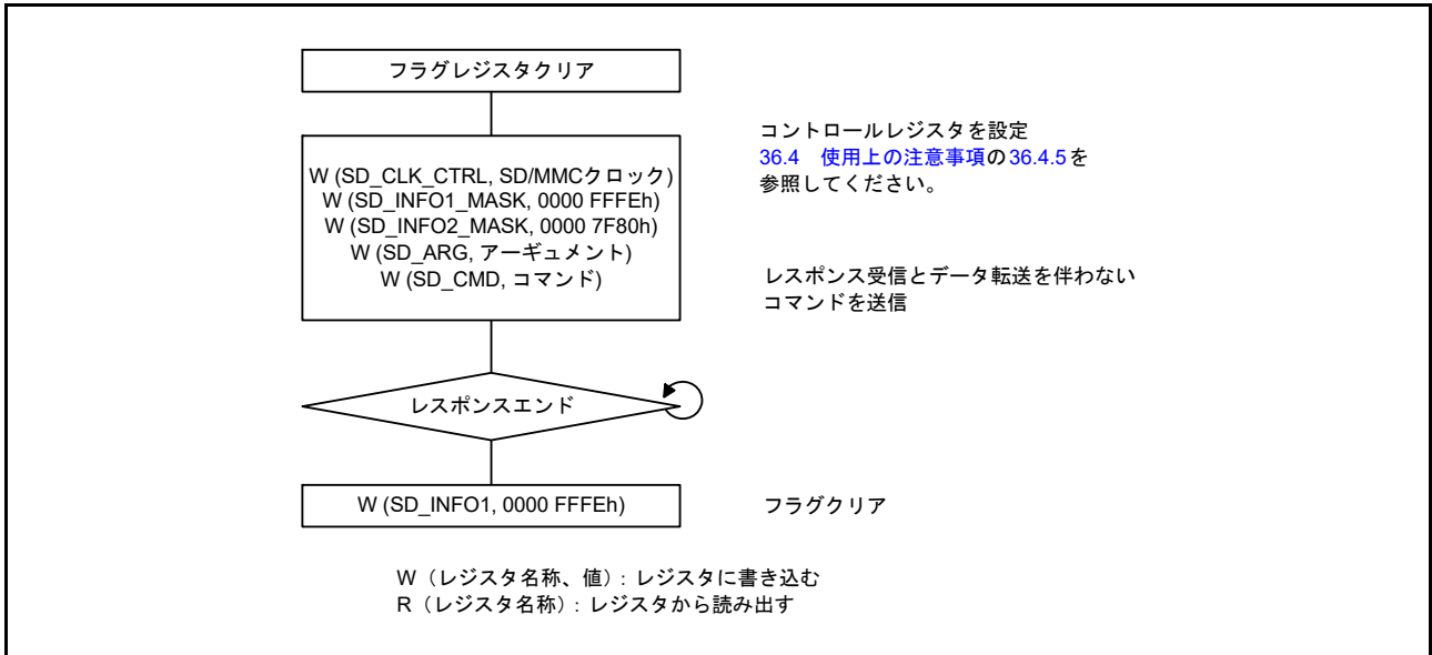
図 36.9 レスポンスおよびデータがないコマンドのフロー例
