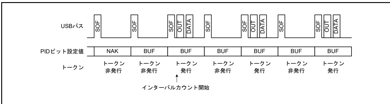
図 28.18 IITV[2:0] = 1 の場合のトークン発行
