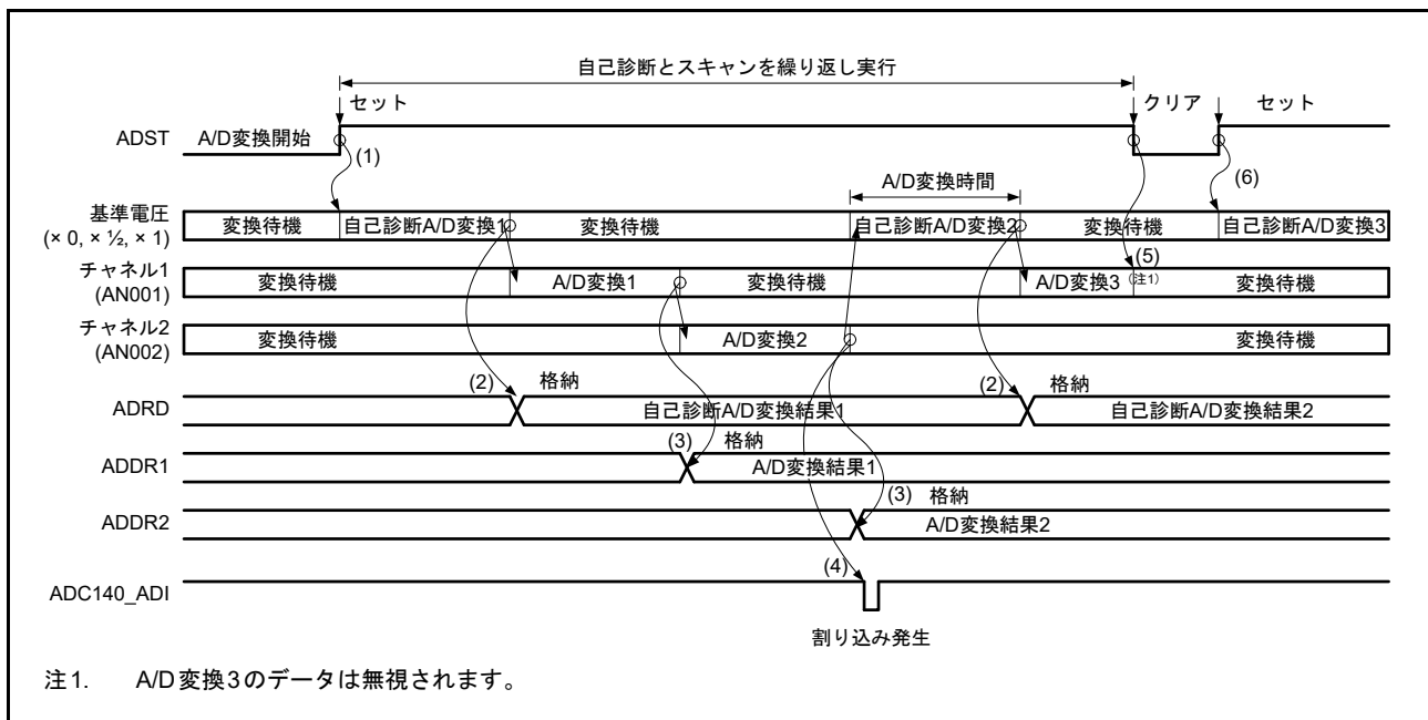
図 38.12 連続スキャンモードの基本動作例 (AN001 および AN002 選択 + 自己診断)
