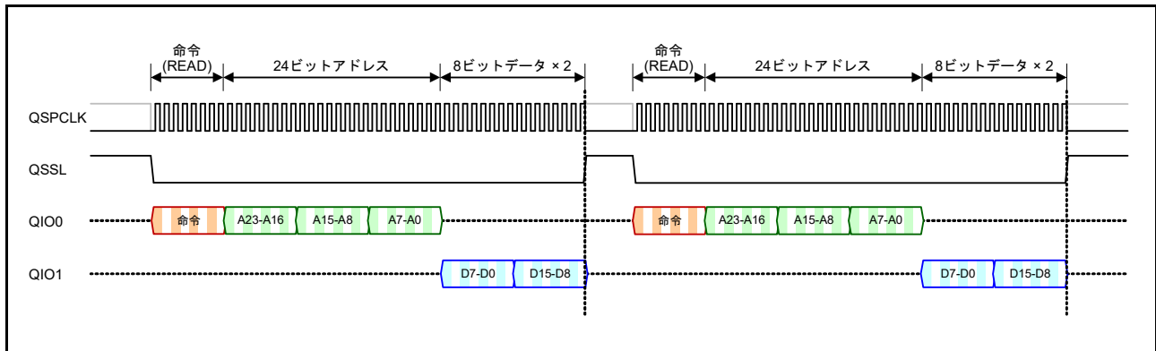
図 33.30 個々の変換に基づく連続データリード動作
