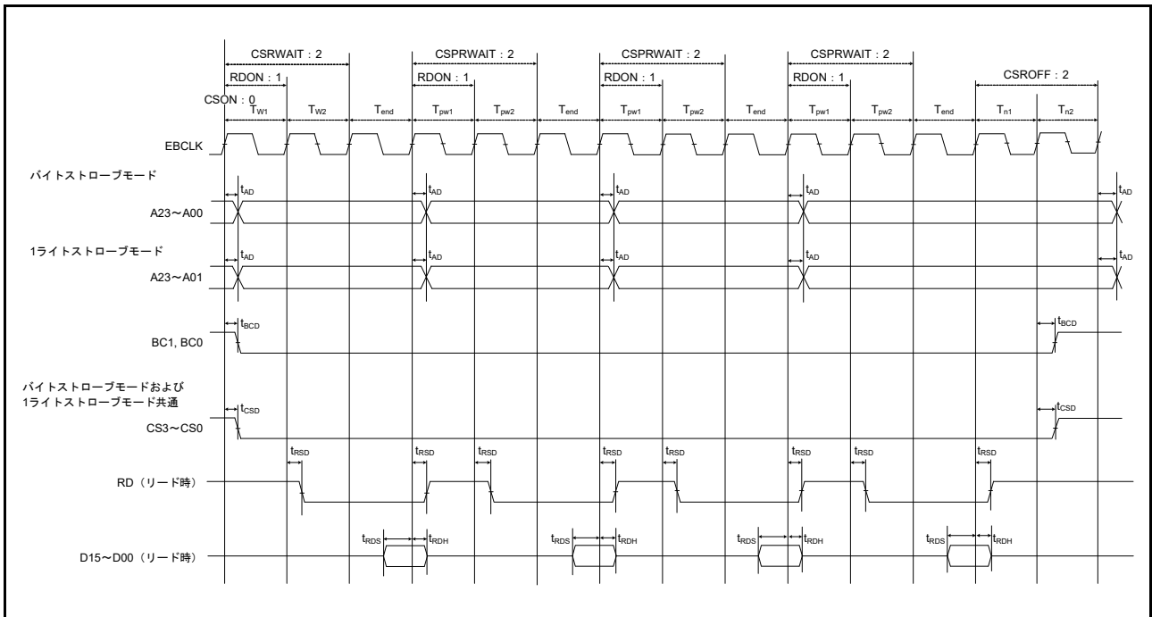
図 50.44 外部バスタイミング/ページリードサイクル (バスクロック同期)
