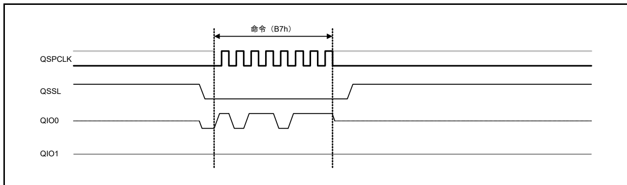
図 33.27 4 バイトモード遷移命令のバスサイクル
