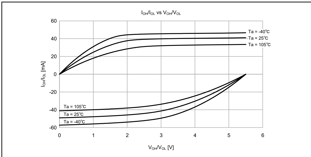
図 50.6 低駆動出力選択時の VCC = 5.5V での V_{OH}/V_{OL} および I_{OH}/I_{OL} 温度特性 (参考データ)
