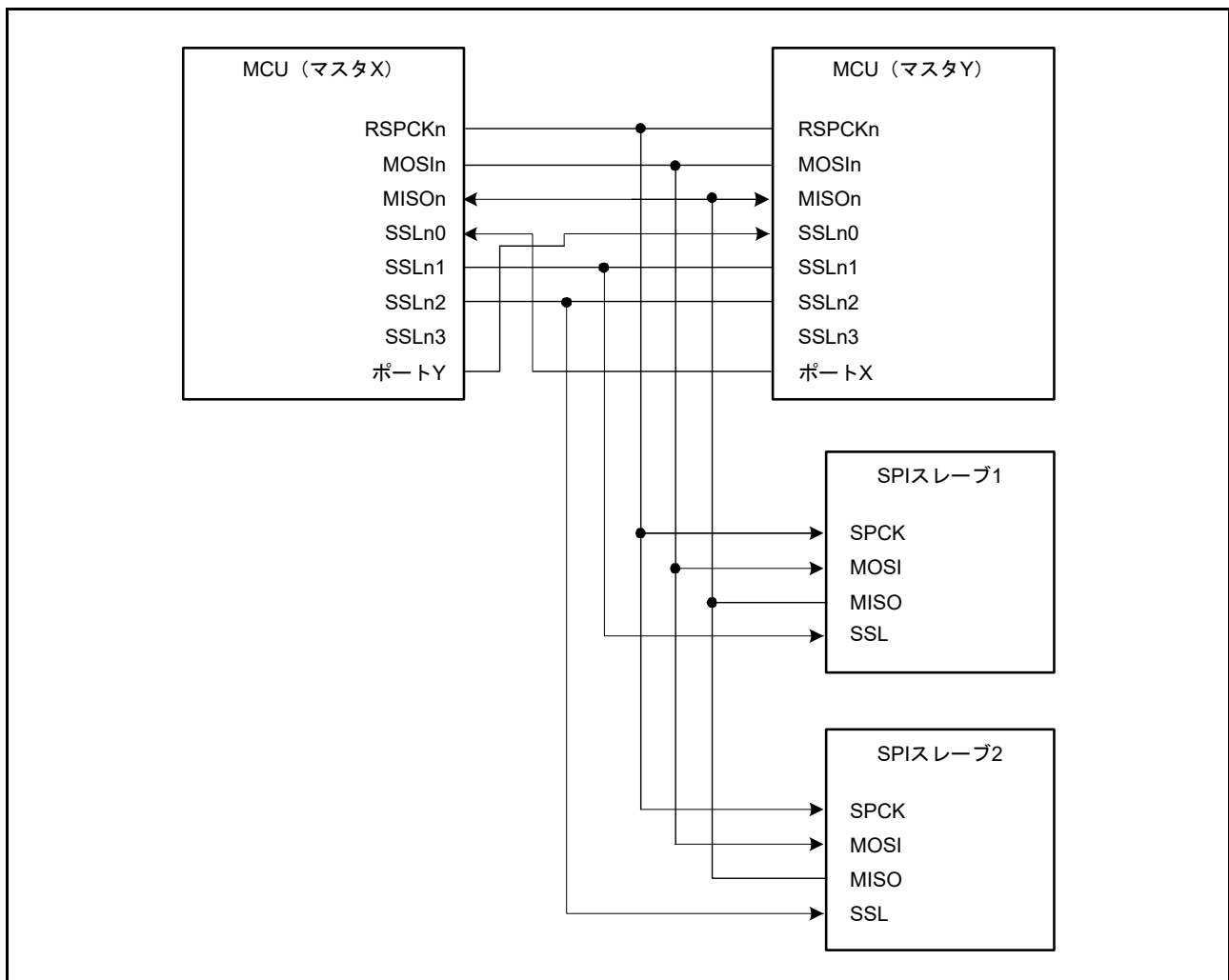
図 32.13 マルチマスタとマルチスレーブの構成例 (MCU はマスタ)
