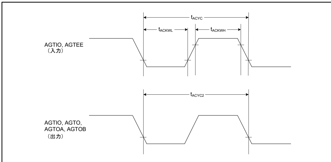
図 50.50 AGT 入出力タイミング
