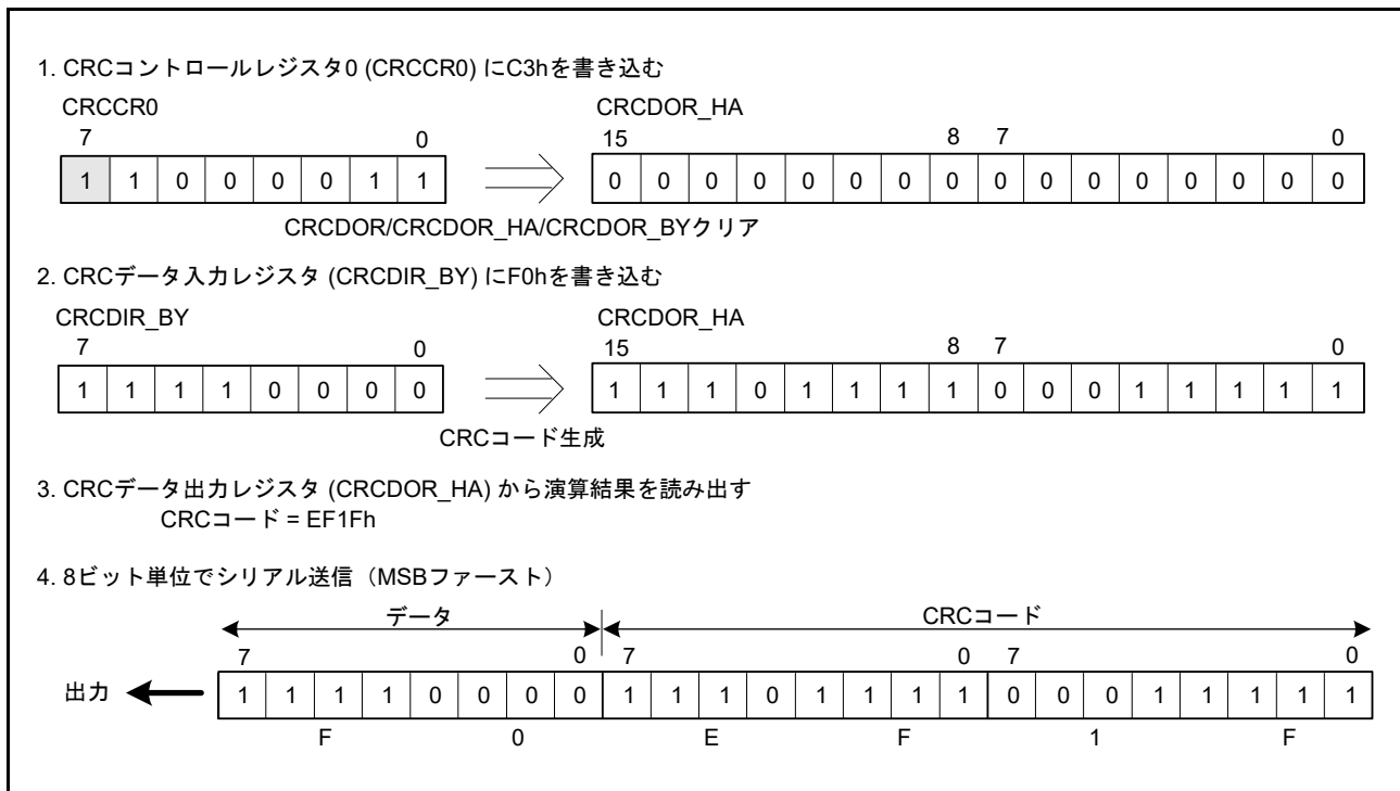
図 34.3 MSB ファーストのデータ送信
