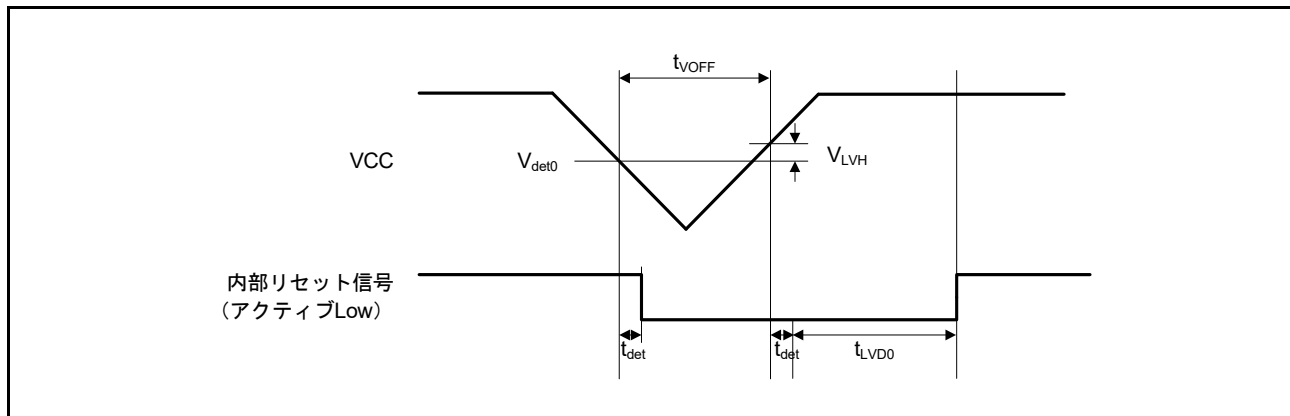
図 50.87 電圧検出回路タイミング ( V_{det0} )
