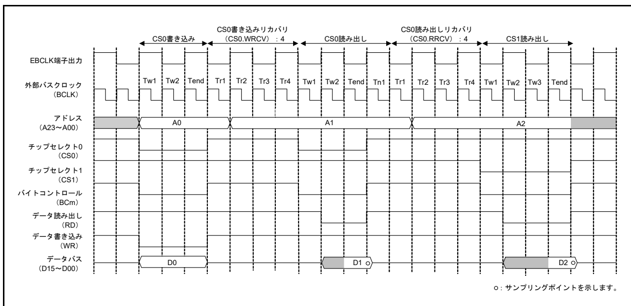
図 15.34 セパレートバスインタフェース時のノーマルアクセスで、EBCLK 端子出力選択ビットで BCLK の 2 分周を設定した場合のリカバリサイクルの動作例 (m = 0, 1)
