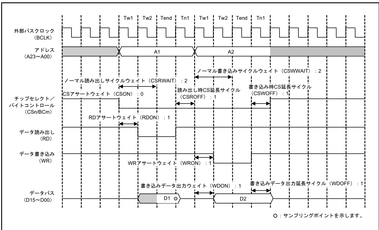
図 15.9 ノーマルアクセスの動作例 (読み出し/書き込み) (n = 0 ~ 3, m = 0, 1)
