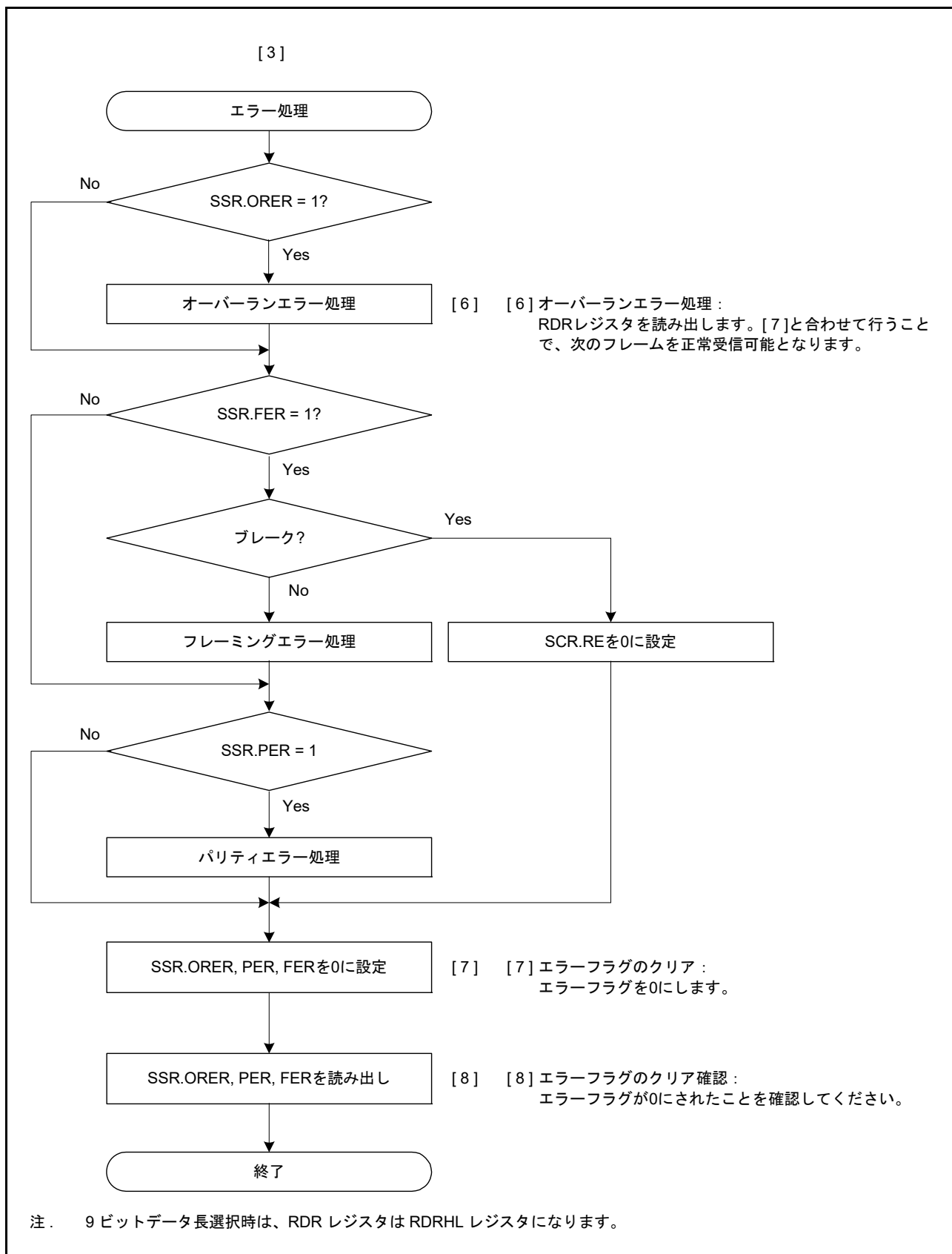
図 29.18 調歩同期式モードにおけるシリアル受信のフローチャート例 (非 FIFO 選択時) (2)
