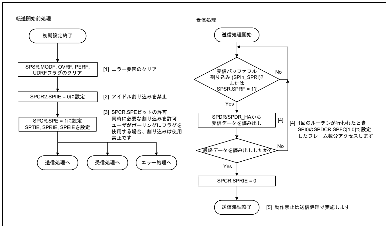
図 32.45 マスタモードでの受信フロー
