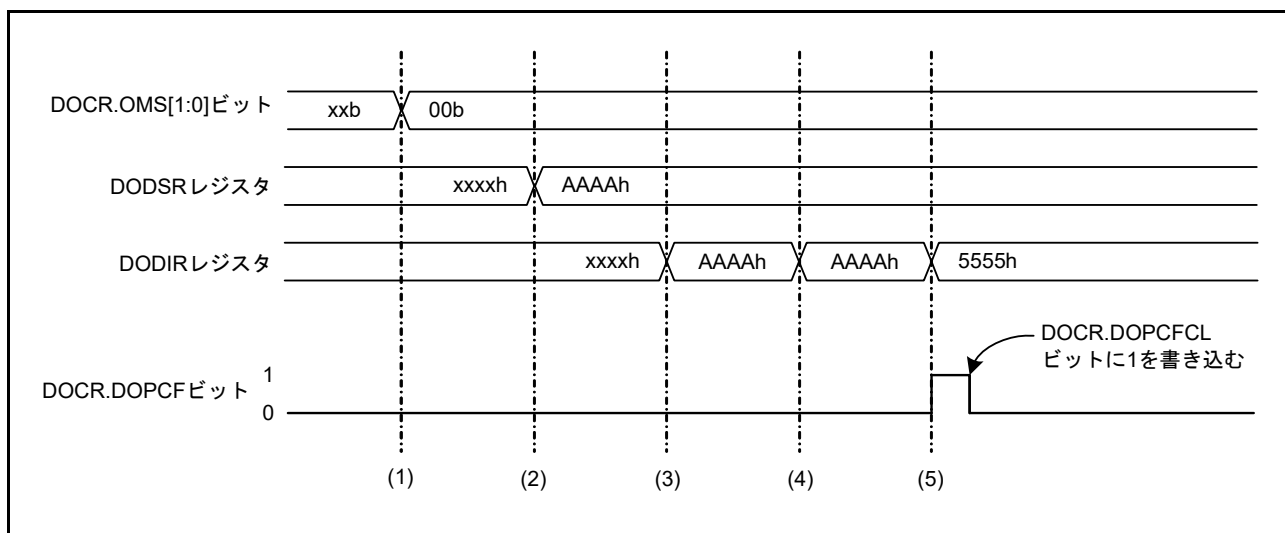
図 45.2 データ比較モードの動作例
