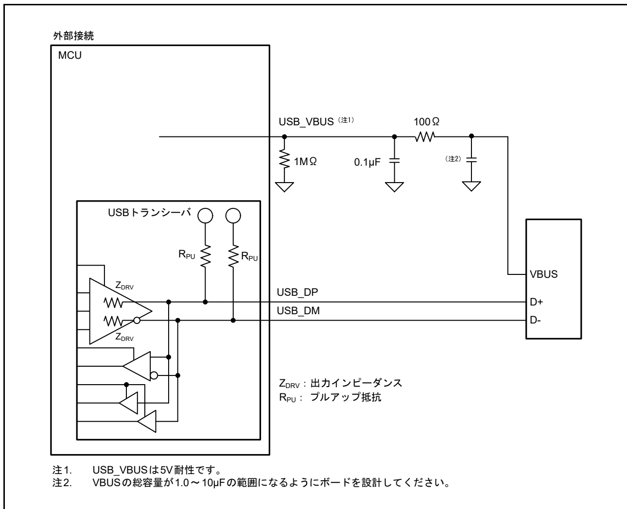
図 28.6 セルフパワー状態でのデバイス接続例
