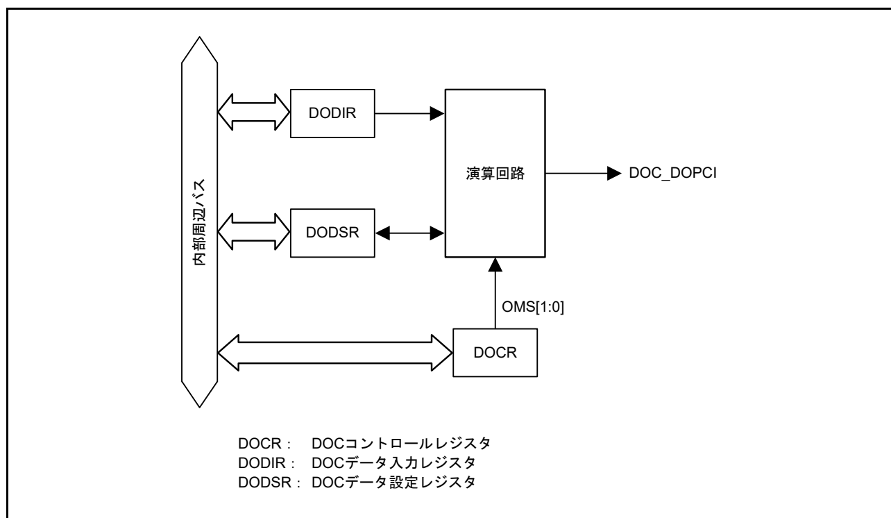
図 45.1 DOC ブロック図
