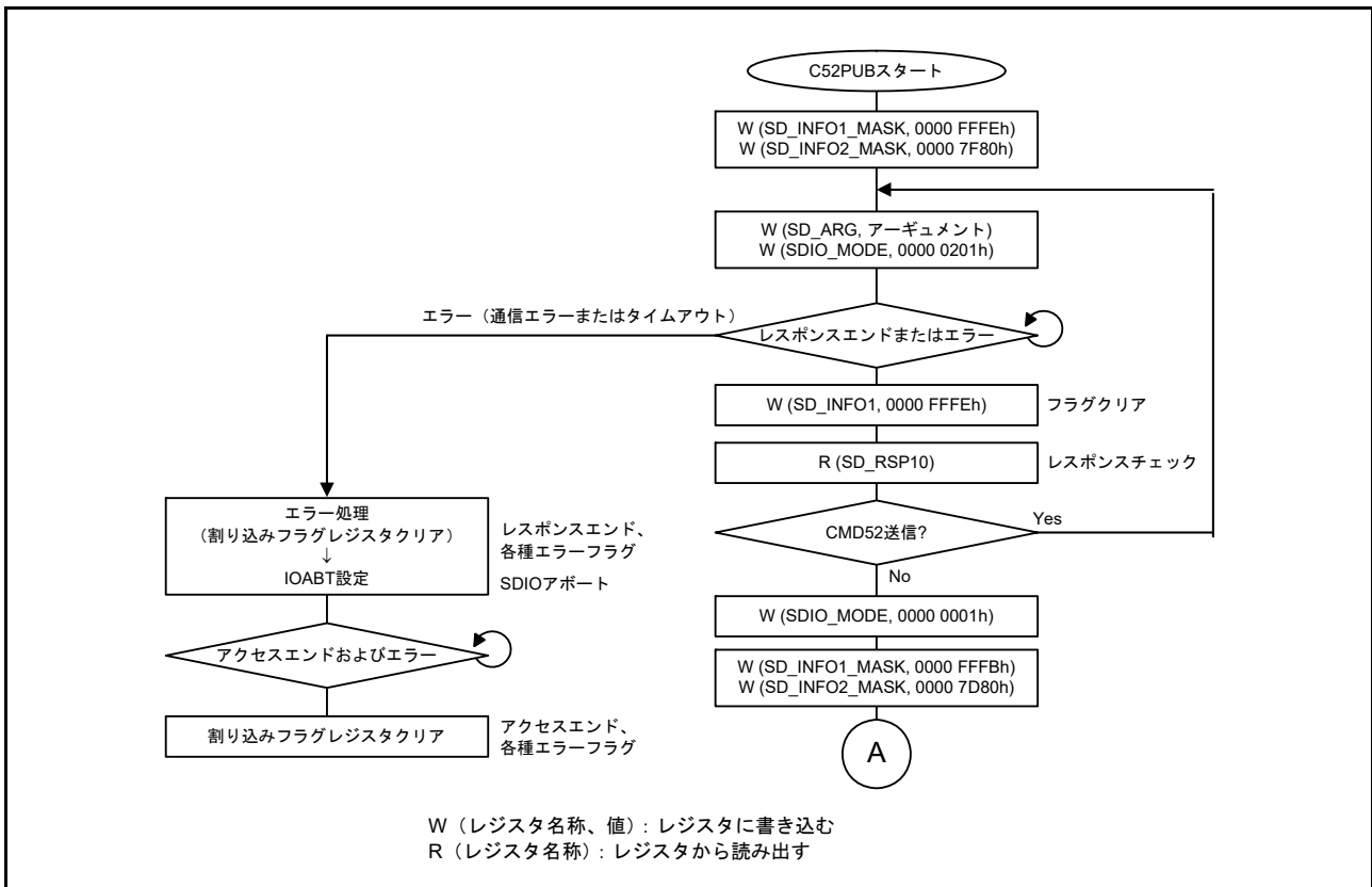
図 36.22 CMD53 マルチブロックライト時に CMD52 (SDIO none abort) が送信される場合のフロー
