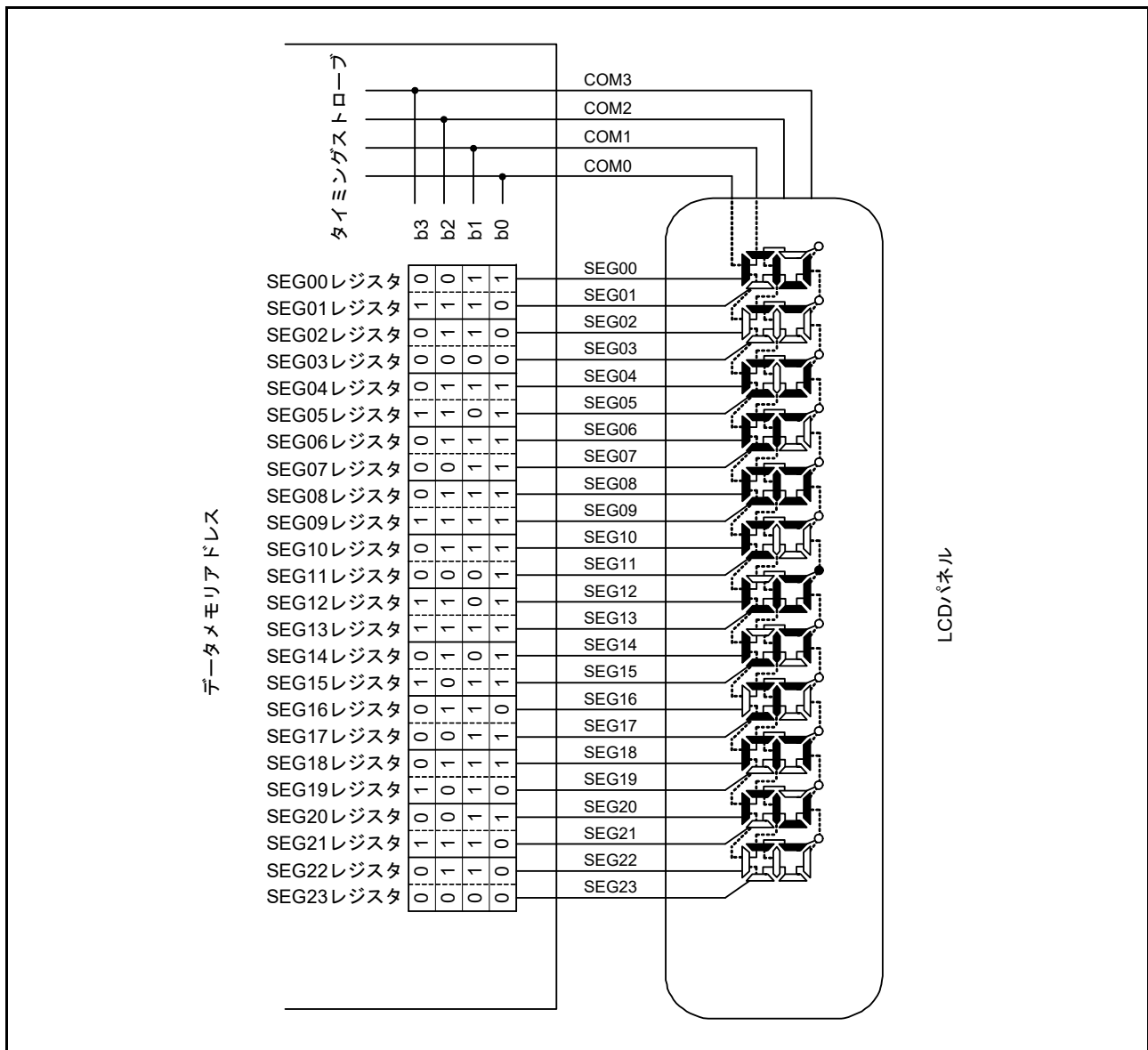
図 48.29 4 時分割 LCD パネルの接続例
