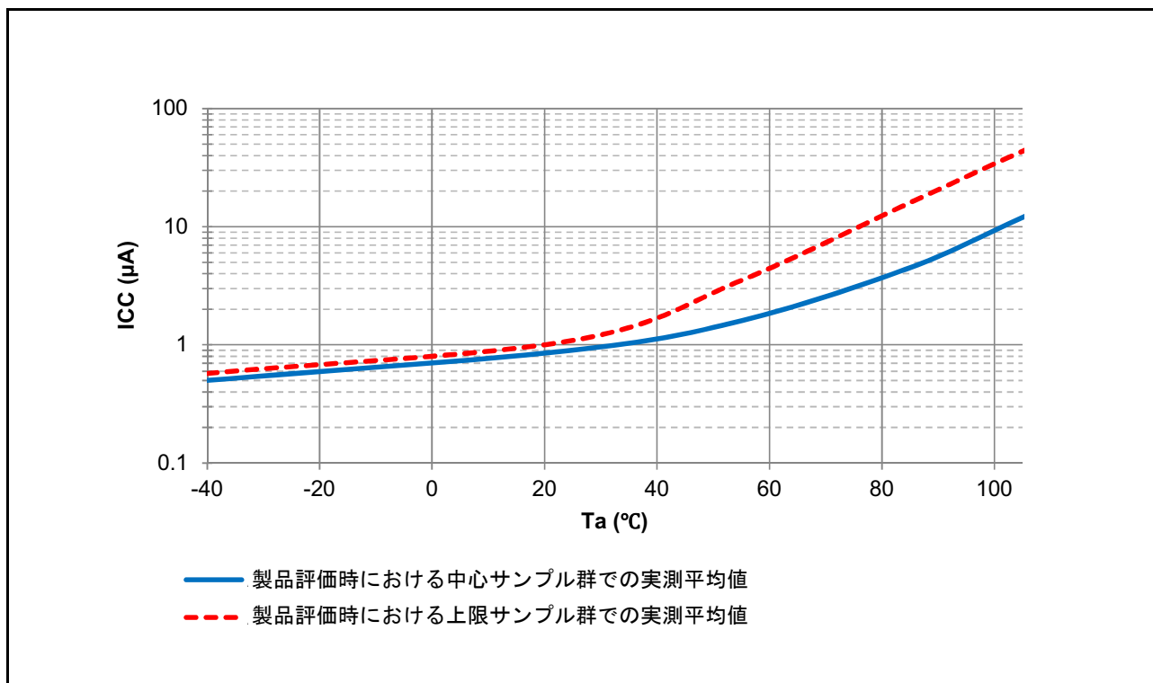
図 50.22 48KB SRAM がオンのソフトウェアスタンバイモード時の温度依存性 (参考データ)
