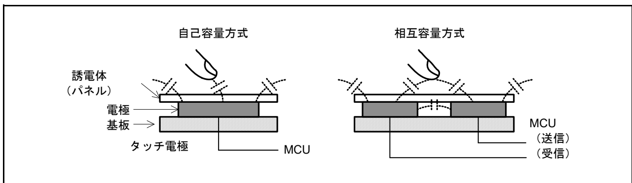
図 44.2 自己容量方式と相互容量方式
