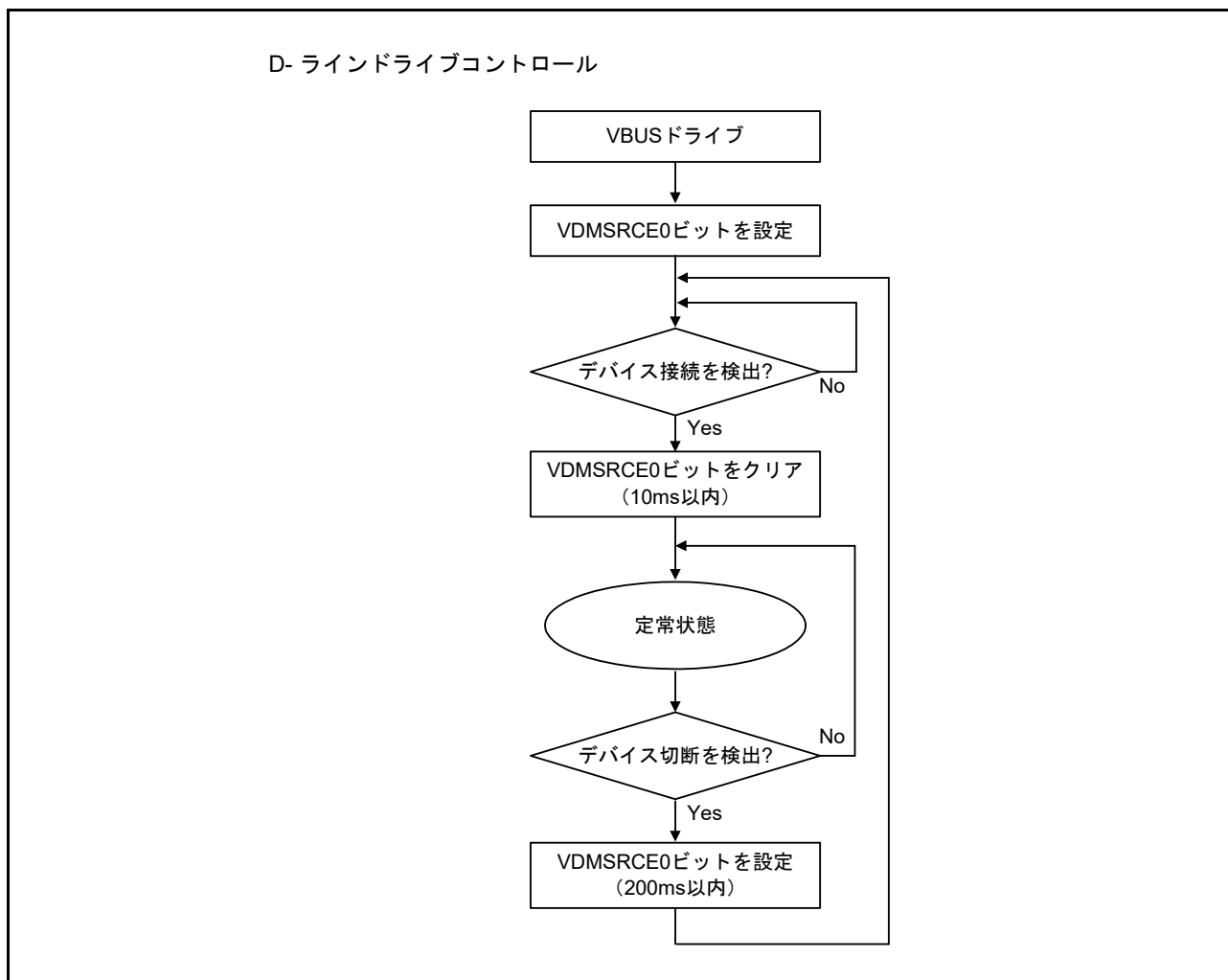
図 28.26 チャージングダウンストリームポートとして動作する場合の処理フロー (ステップ a ~ b)
