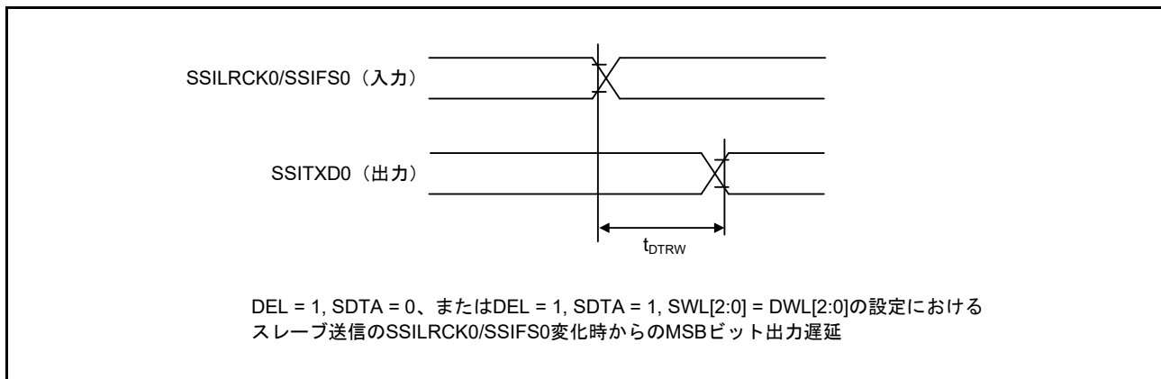
図 50.74 SSILRCK0/SSIFS0 変化時からの SSIE データ出力遅延
