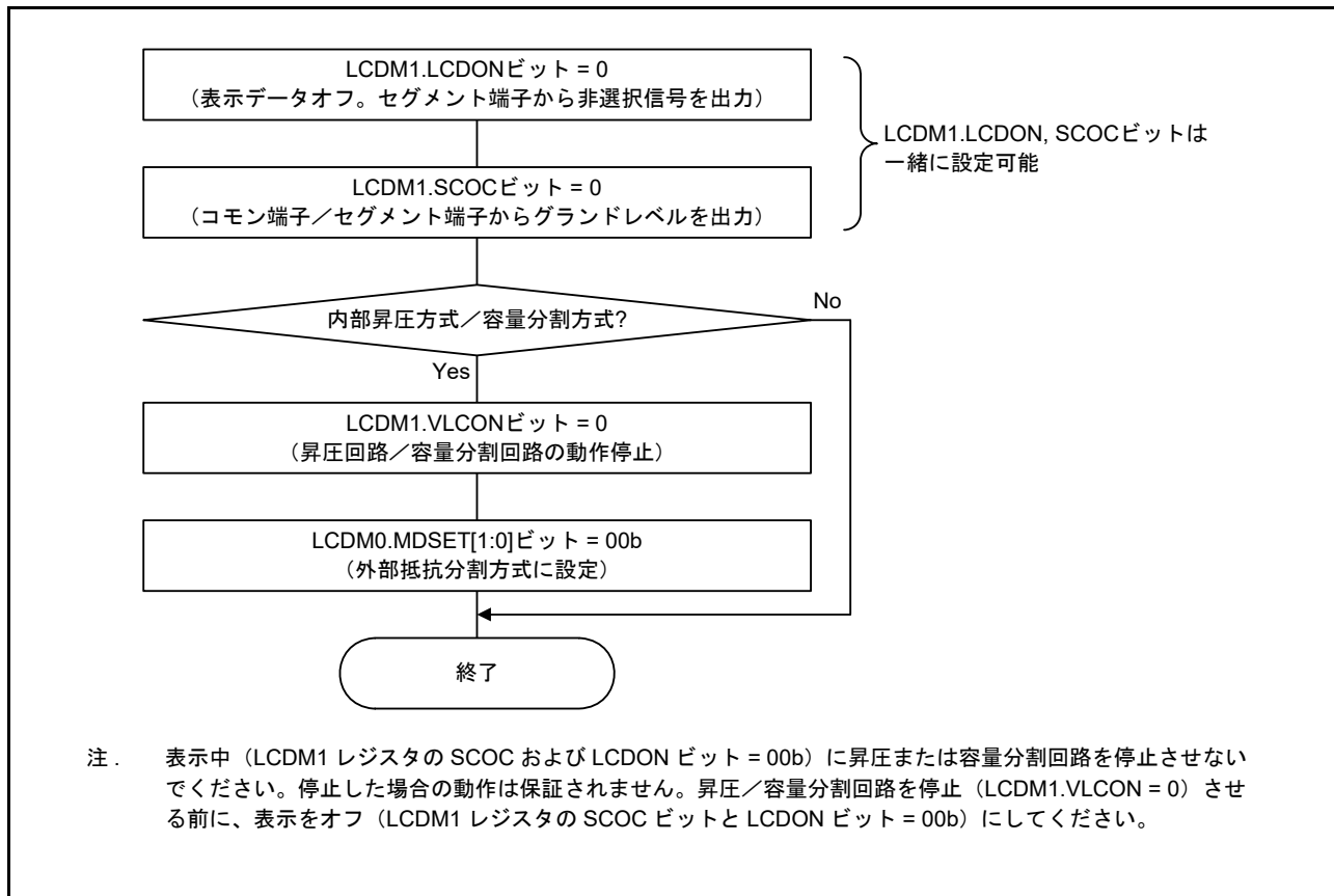
図 48.8 通常液晶波形 (A または B) 表示での動作停止手順
