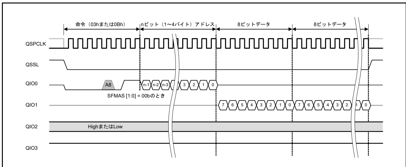
図 33.16 標準リードバスサイクル
