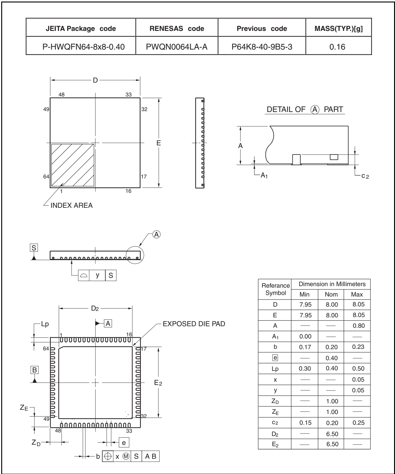
図 2.7 QFN 64 ピン
