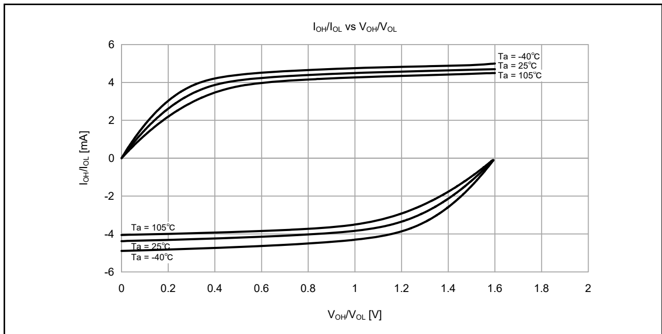
図 50.8 中駆動出力選択時の VCC = 1.6V での V OH /V OL および I OH /I OL 温度特性 (参考データ)
