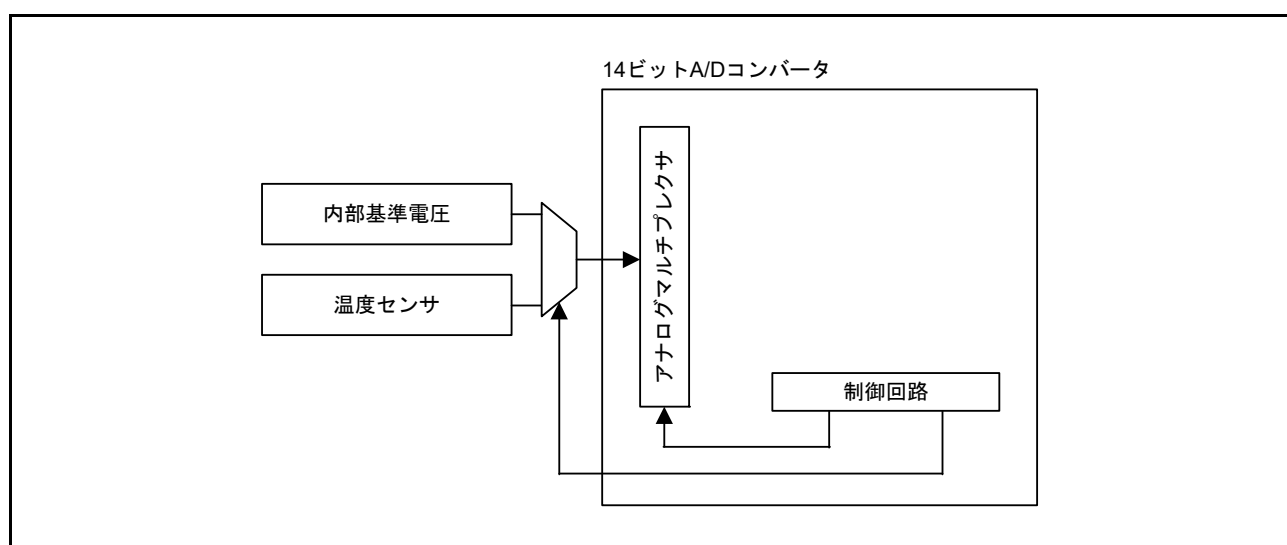
図 40.1 温度センサのブロック図
