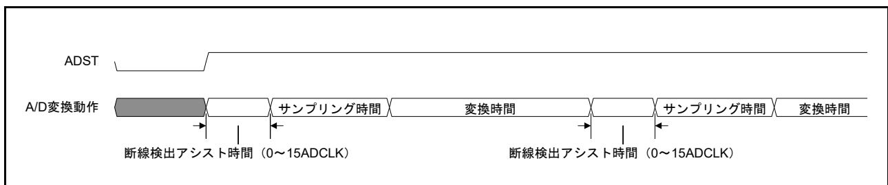
図 38.26 断線検出アシスト機能を使用した場合の A/D 変換動作図
