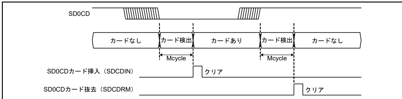
図 36.7 SD_BUF0 レジスタからの読み出し
