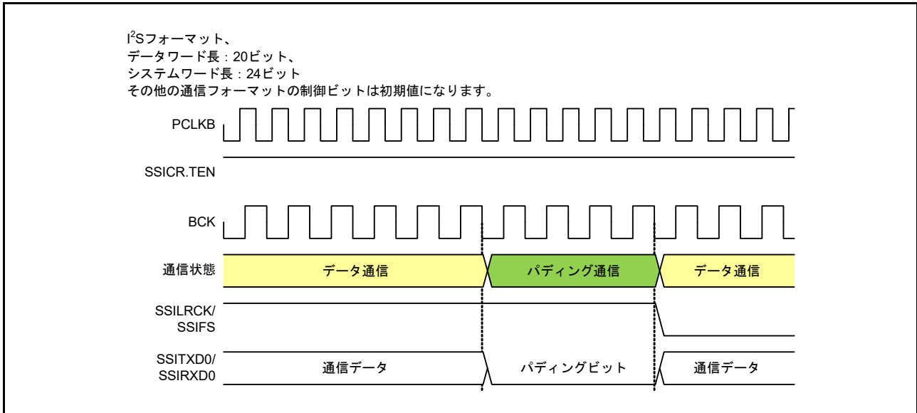
図 35.45 データ通信からパディング通信への遷移
