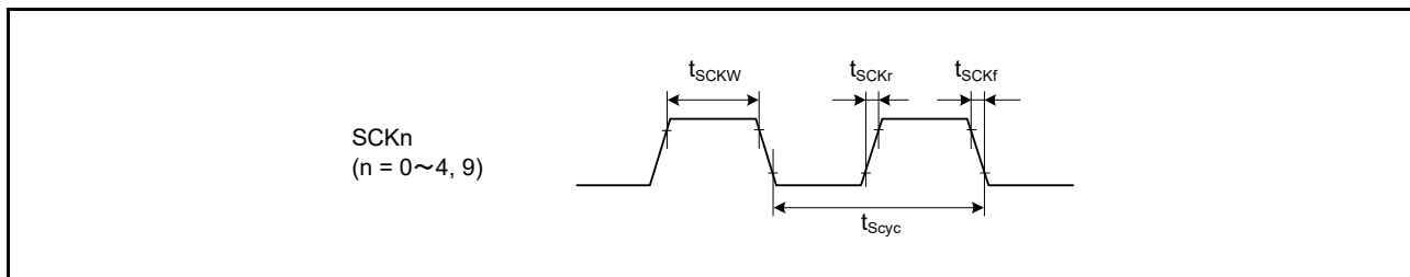
図 50.53 SCK クロック入力タイミング
