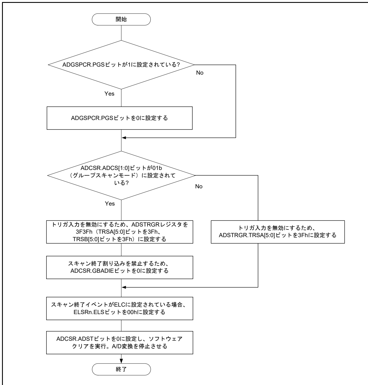
図 38.31 ソフトウェアによる ADCSR.ADST ビットのクリア手順
