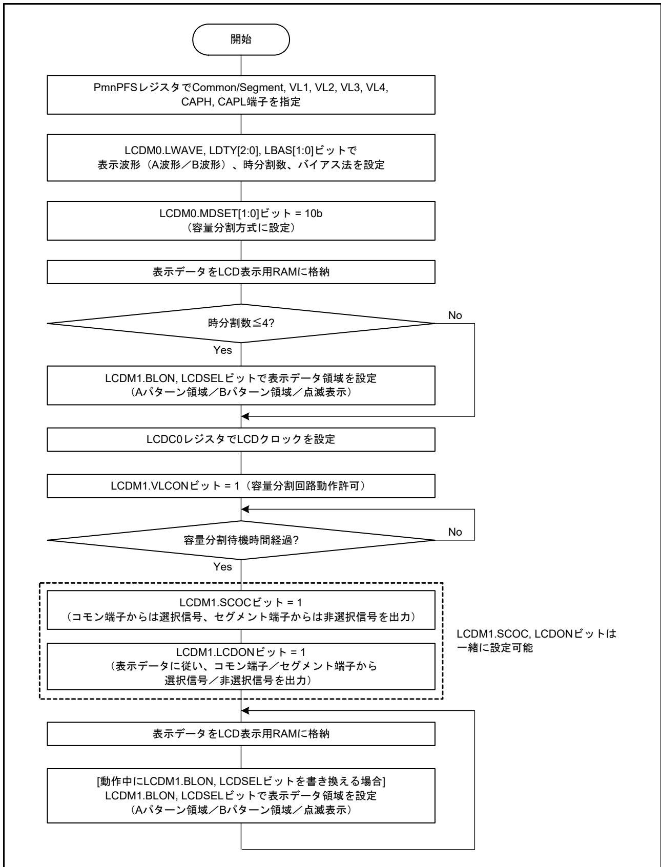
図 48.7 通常液晶波形表示での容量分割方式の設定手順
