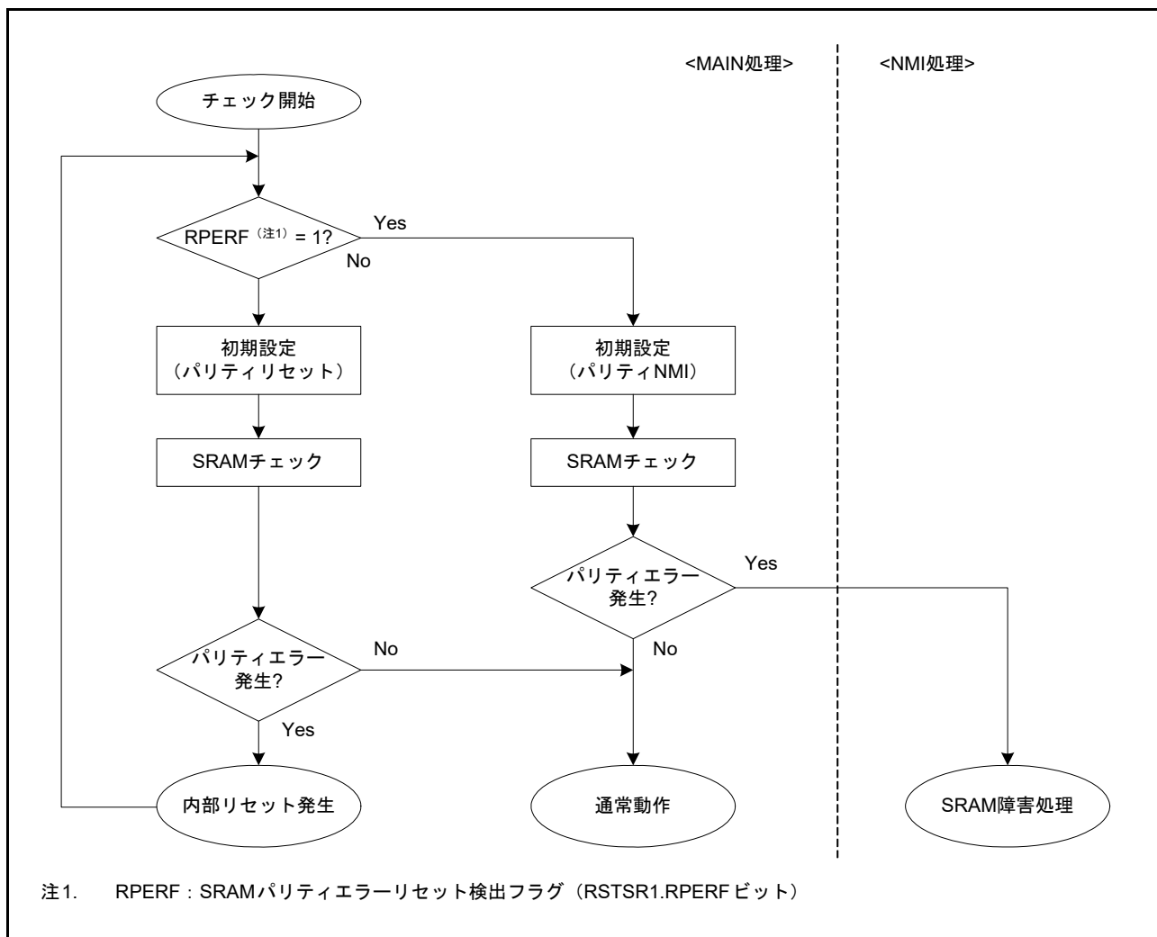
図 46.2 SRAM パリティリセット許可の場合の SRAM パリティチェックのフロー
