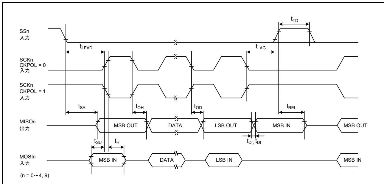
図 50.58 SCI 簡易 SPI モードタイミング (スレーブ、CKPH = 1)
