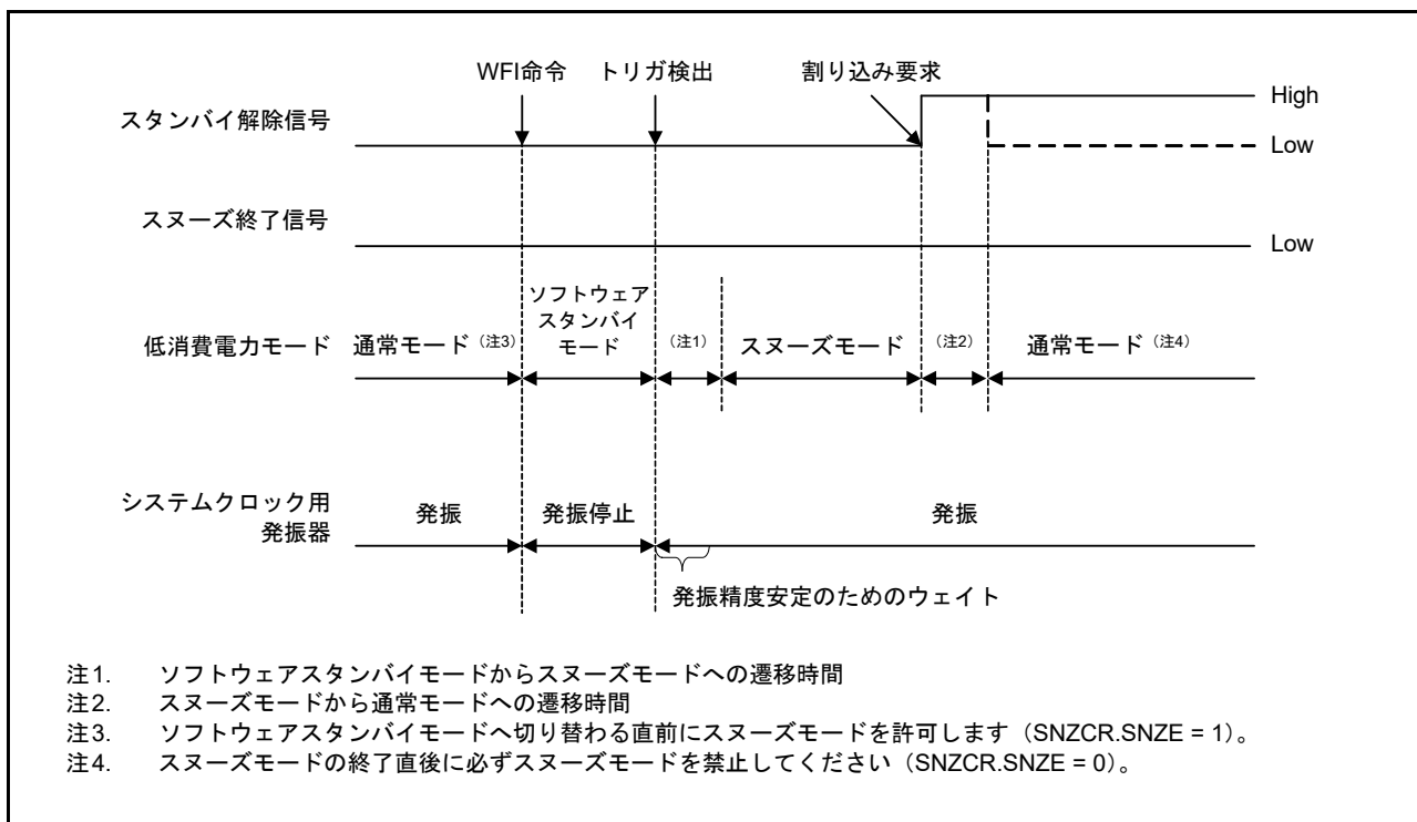
図 11.9 割り込み要求信号が発生する場合のスヌーズモードの解除
