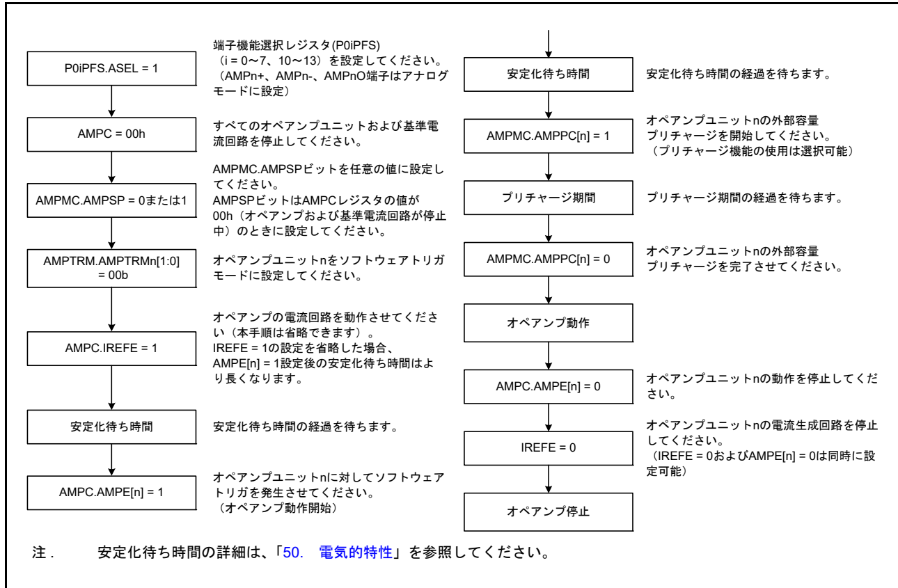
図 41.7 ソフトウェアトリガモードでの OPAMP 起動および停止手順
