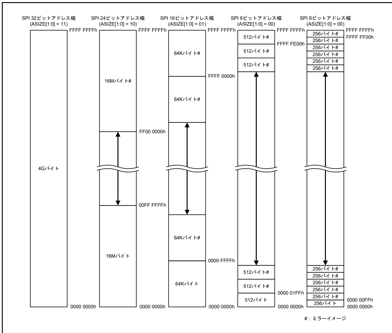
図 33.3 SPI 空間のメモリマップ
