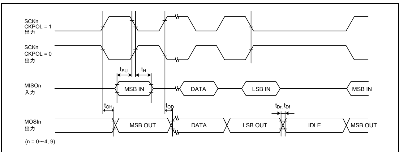
図 50.57 SCI 簡易 SPI モードタイミング (マスタ、CKPH = 0)
