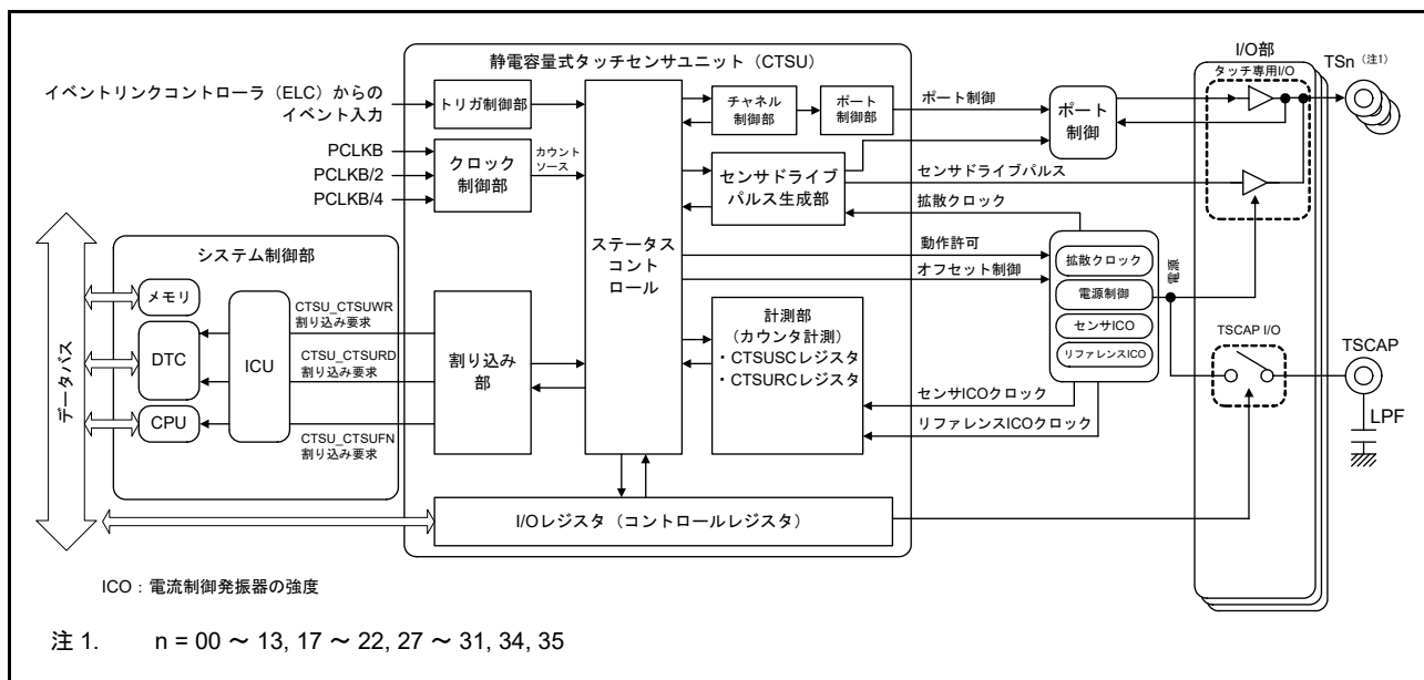
図 44.3 CTSUSのブロック図
