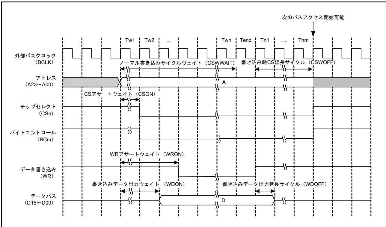
図 15.8 ノーマルライトアクセスのバスタイミング (1ライトストローブモード) (n = 0 ~ 3, m = 0, 1)
