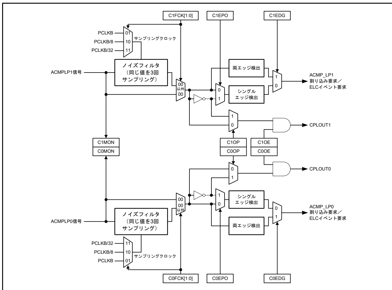
図 42.5 ノイズフィルタおよびエッジ検出の構成
