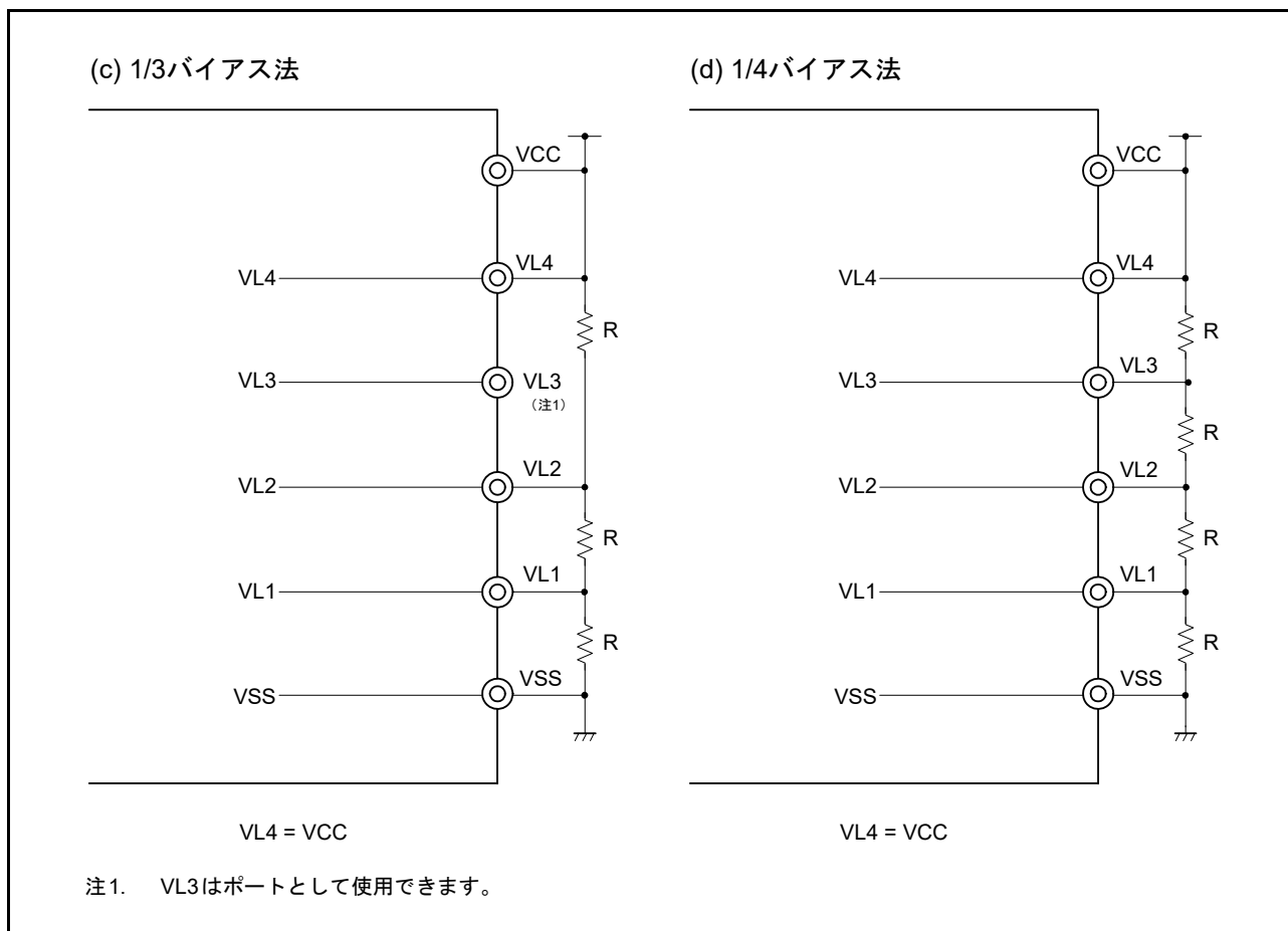
図 48.10 LCD 駆動電源の接続例（外部抵抗分割方式）(2/2)
