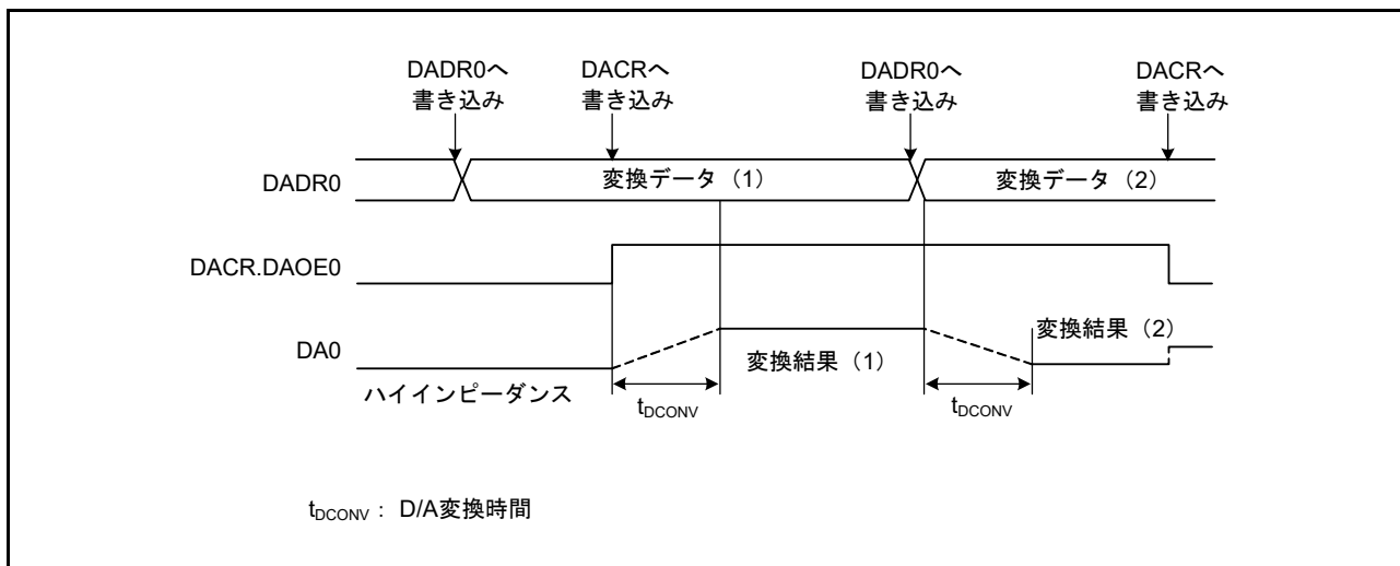
図 39.2 DAC12 の動作例
