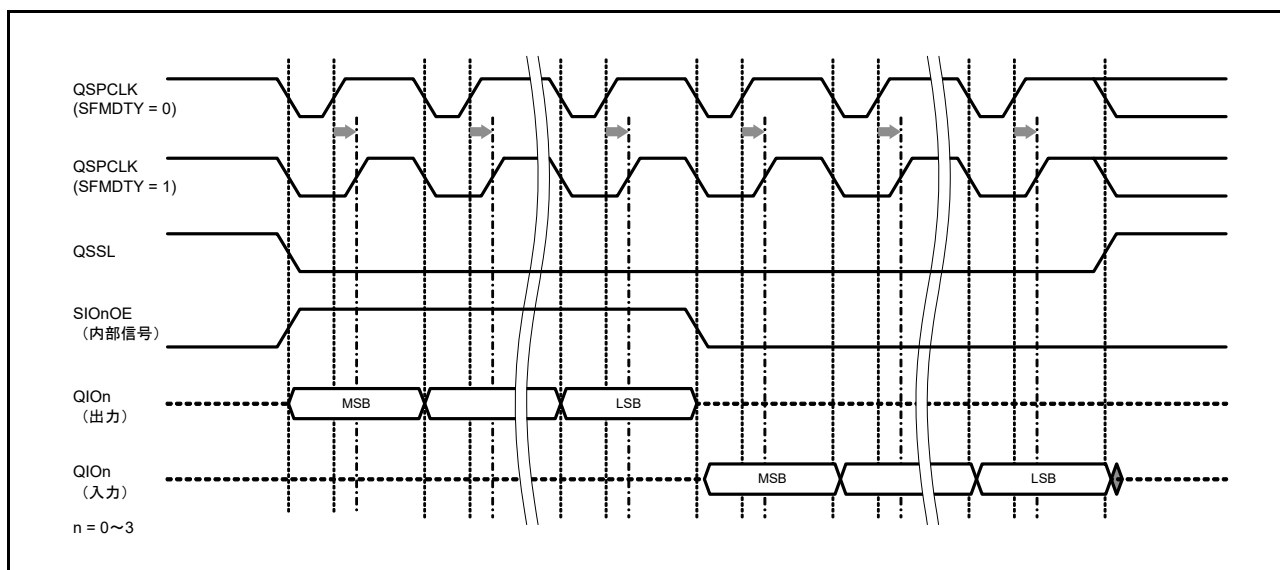
図 33.9 PCLKA を 3 逡倍した場合の SFMDTY ビットを使用した QSPCLK 信号デューティ比補正例
