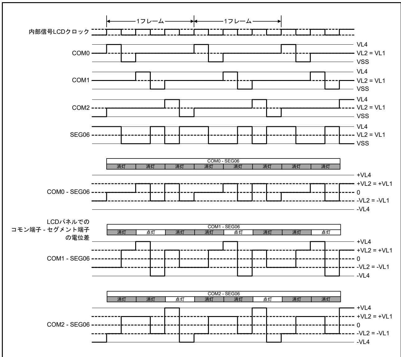
図 48.26 1/2 バイアス法を用いた SEG06 と各コモン信号との間の 3 時分割 LCD 駆動波形例
