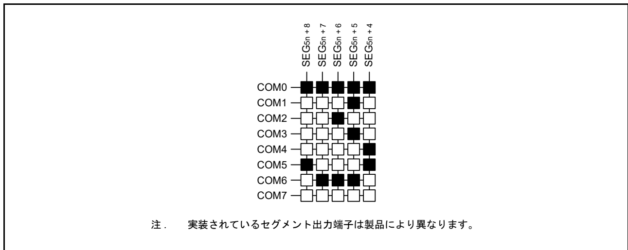
図 48.32 8 時分割 LCD 表示パターンと電極接続
