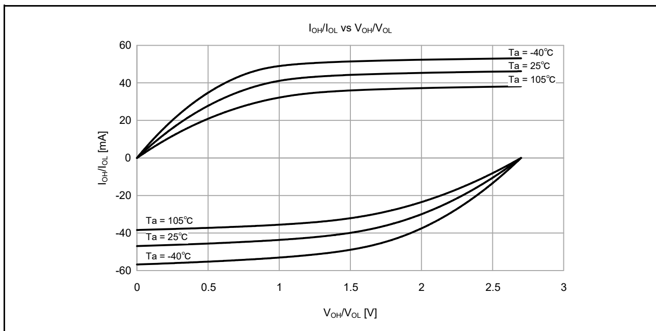
図 50.13 中駆動出力選択時の VCC = 2.7V での V OH /V OL および I OH /I OL 温度特性 (参考データ)
