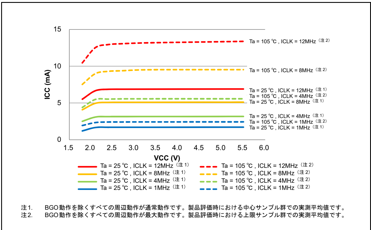
図 50.18 Middle-speed モードにおける電圧依存性 (参考データ)
