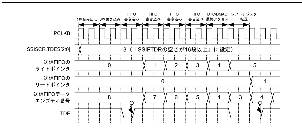
図 35.27 TDE の設定およびクリアのタイミング図
