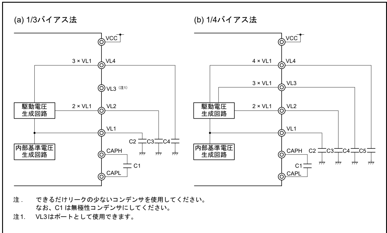
図 48.11 LCD 駆動電源の接続例 (内部昇圧方式)
