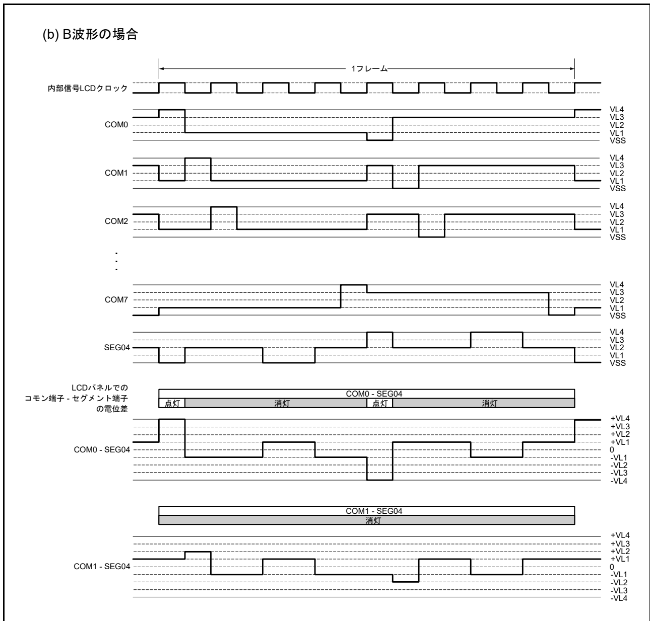
図 48.35 1/4 バイアス法を用いた SEG04 と各コモン信号との間の 8 時分割 LCD 駆動波形例 (2/2)
