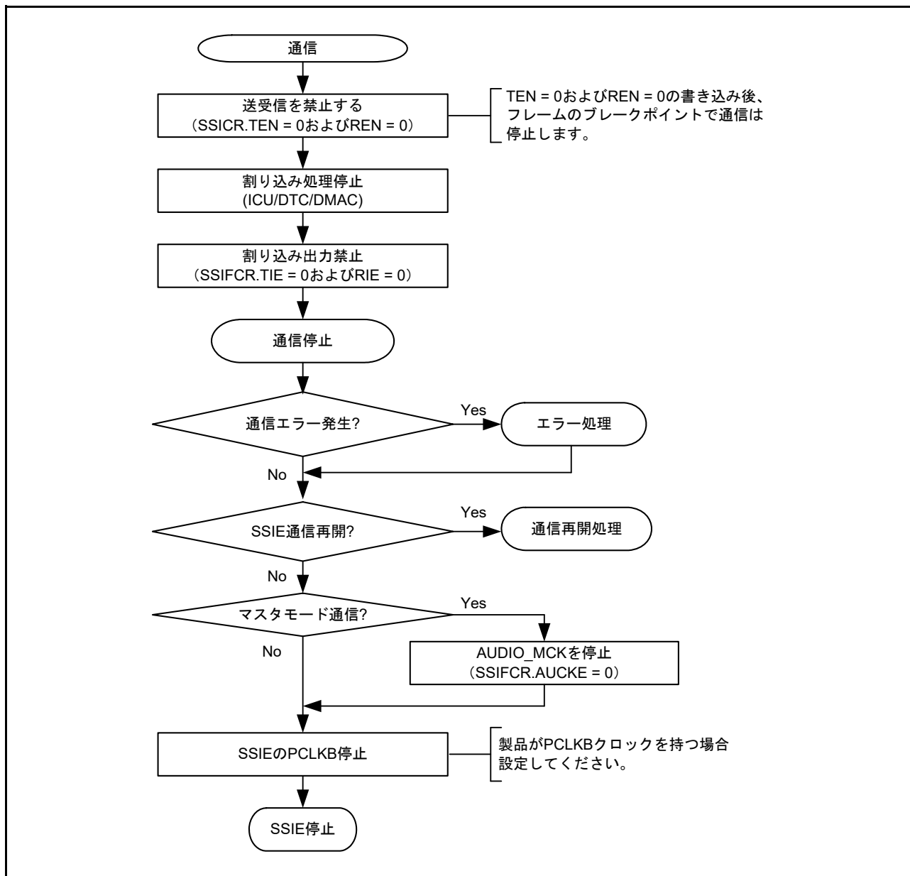
図 35.52 通信停止手順 (CPU 動作)
