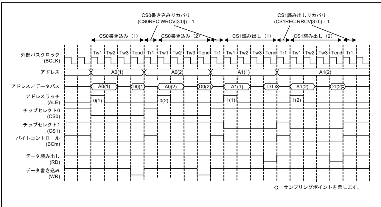
図 15.36 アドレス/データマルチプレクス I/O インタフェース時のバスアクセスが分割された場合のリカバリサイクルの挿入例 (m = 0, 1)
