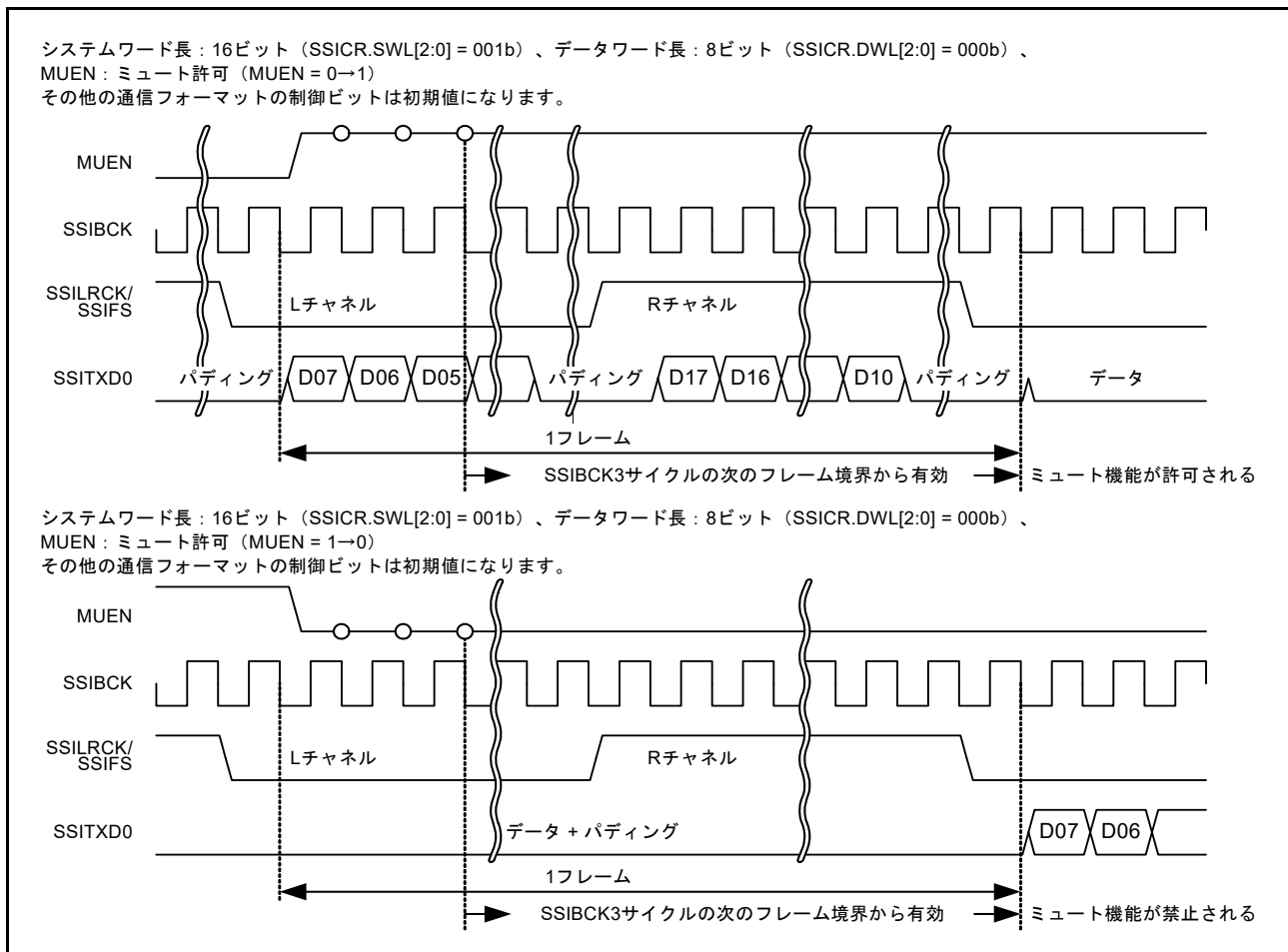
図 35.4 ミュート機能設定時の送信データ
