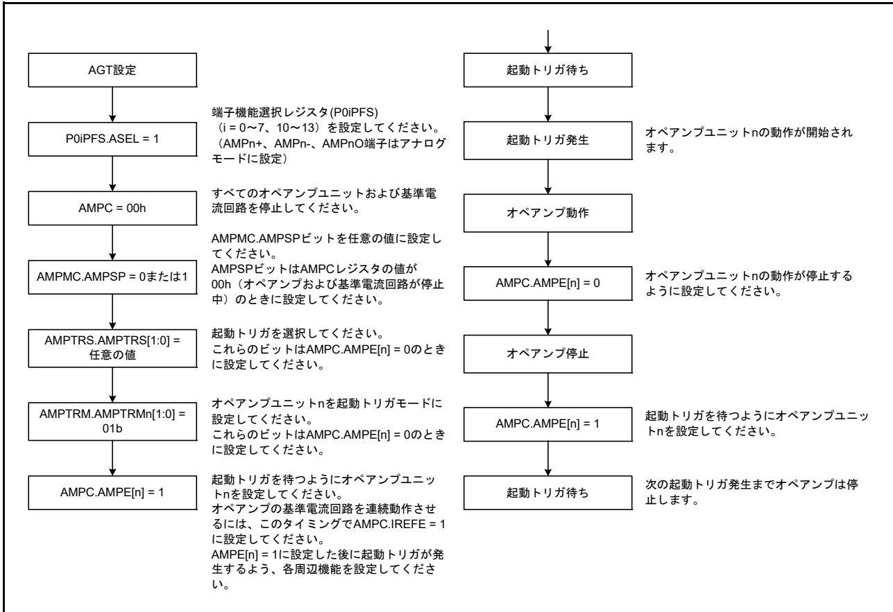
図 41.8 起動トリガモードでの OPAMP 起動および停止手順
