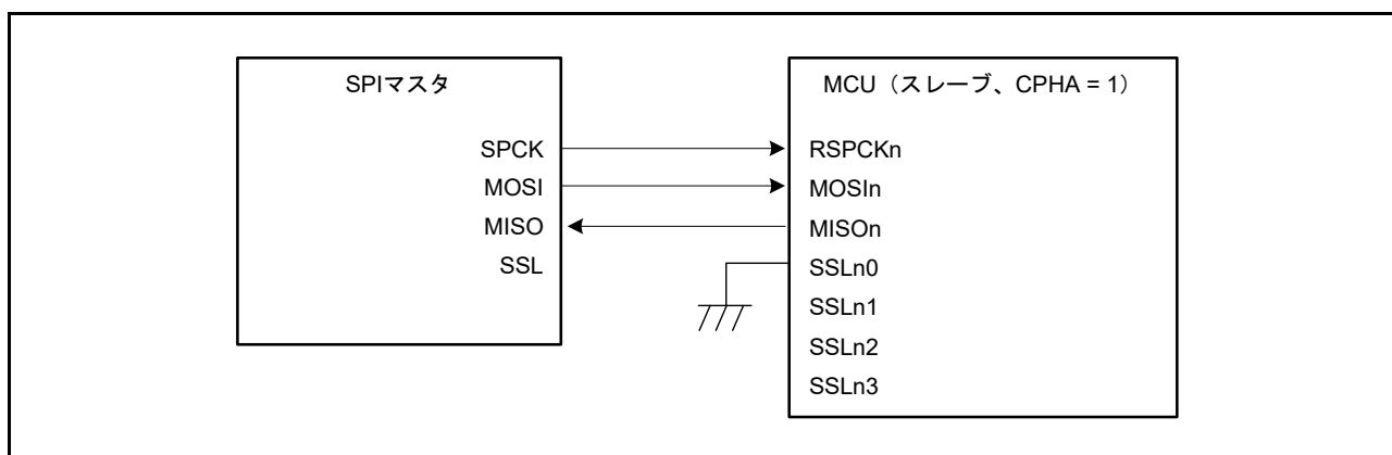
図 32.10 シングルマスタとシングルスレーブの構成例 (MCU はスレーブ、CPHA = 1)
