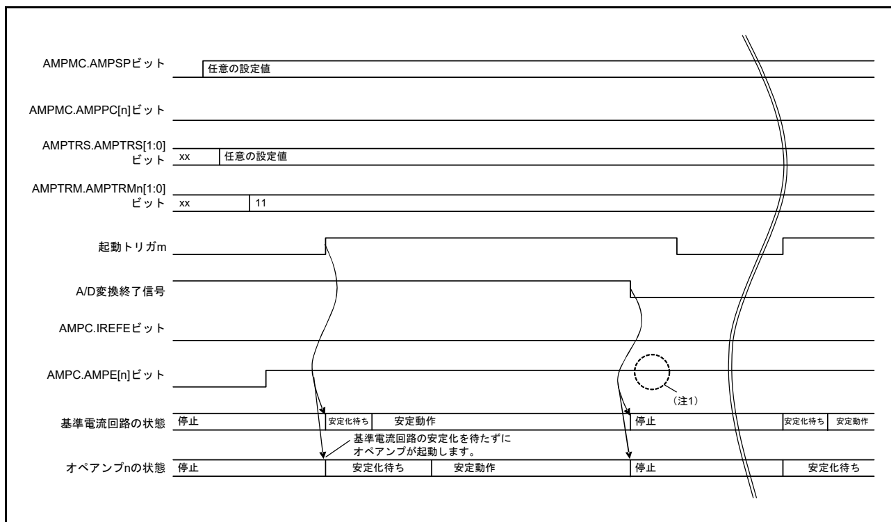
図 41.5 オペアンプの制御動作 (起動および A/D トリガモード (1)) (基準電流回路およびオペアンプを起動トリガによって起動し、A/D 変換終了 (トリガ) によって停止する場合)
