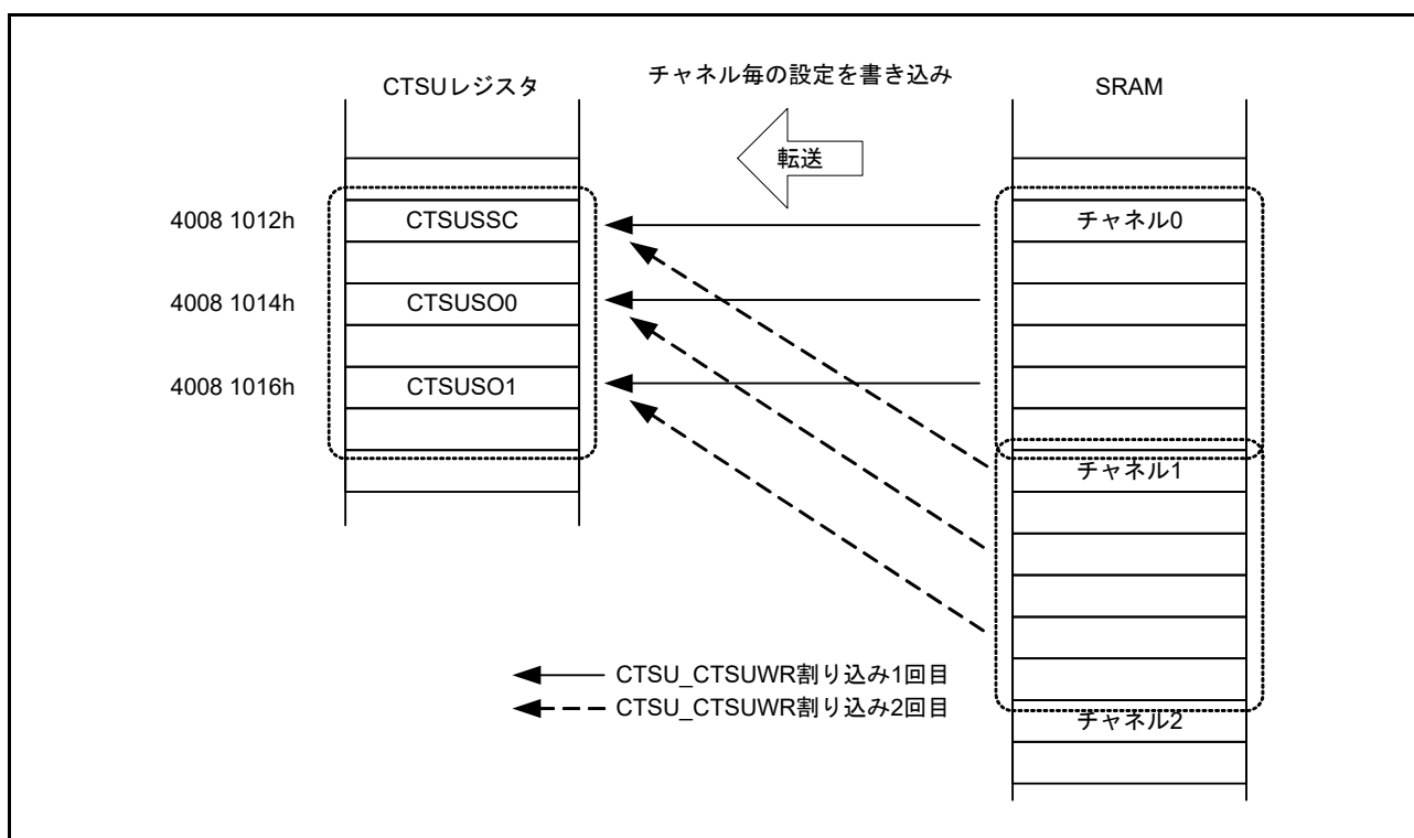
図 44.19 CTSUS_CTSUWR 割り込みを用いた DTC 転送動作例
