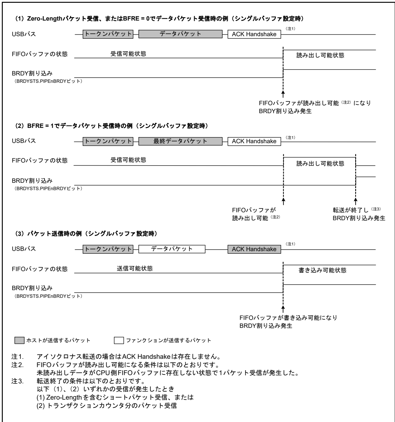
図 28.12 BRDY 割り込みの発生タイミング
