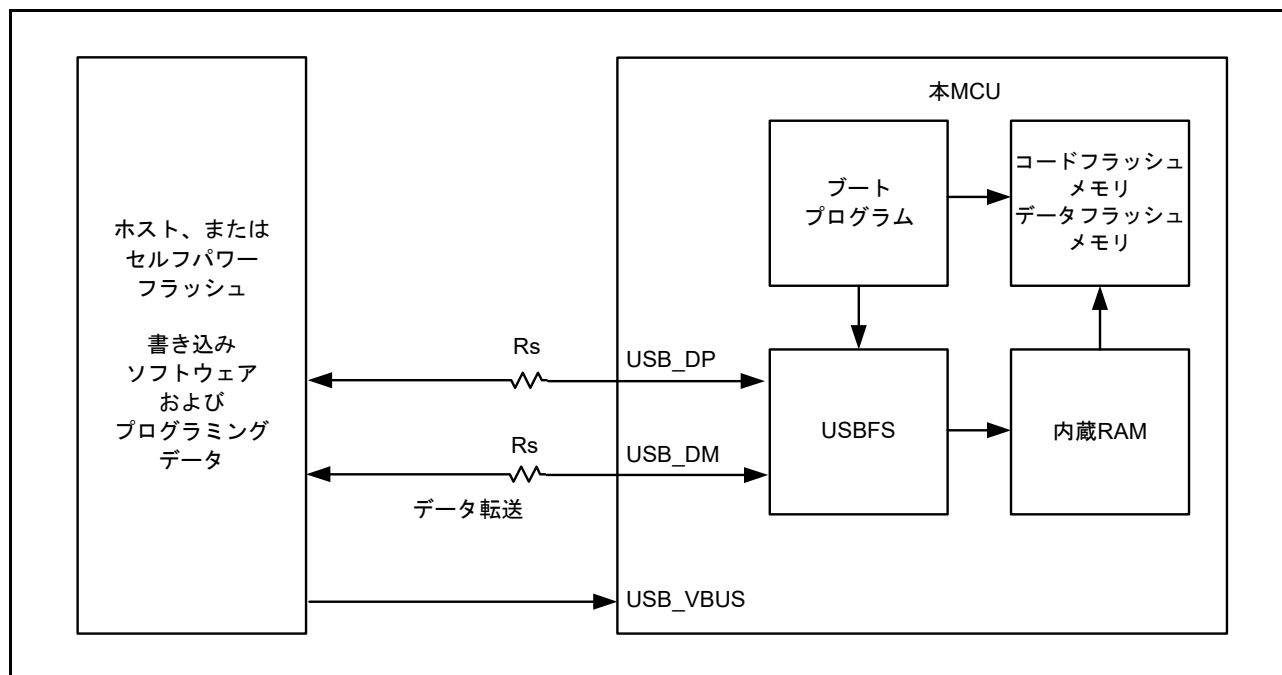
図 47.10 USB ブートモード時のシステム構成
