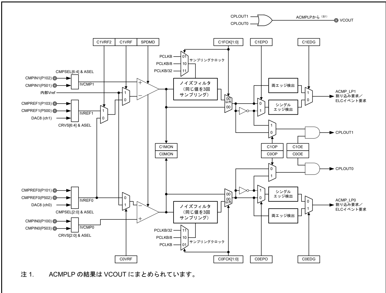
図 42.1 ウィンドウ機能無効時の ACMPLP ブロック図
