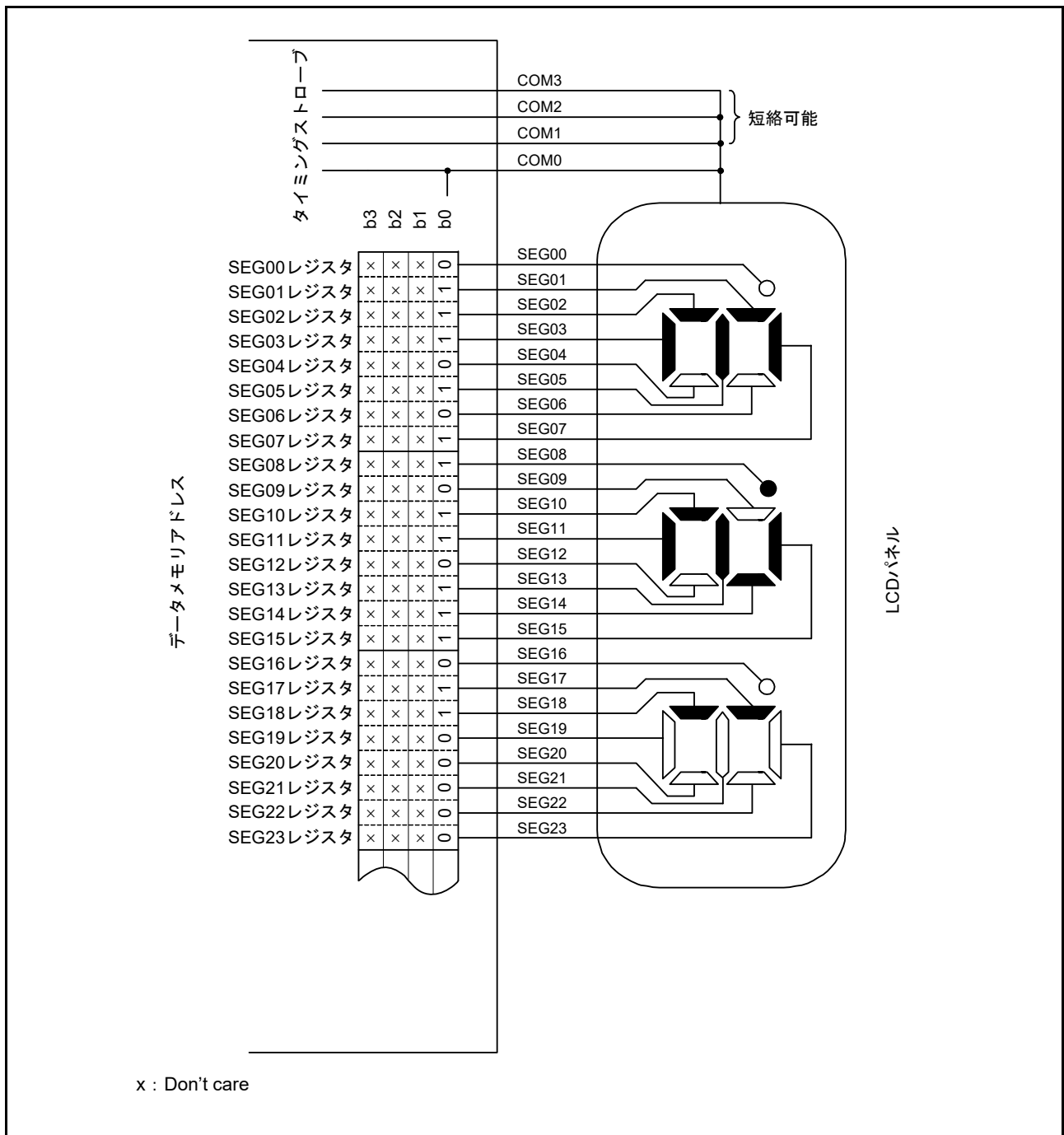
図 48.19 スタティック LCD パネルの接続例
