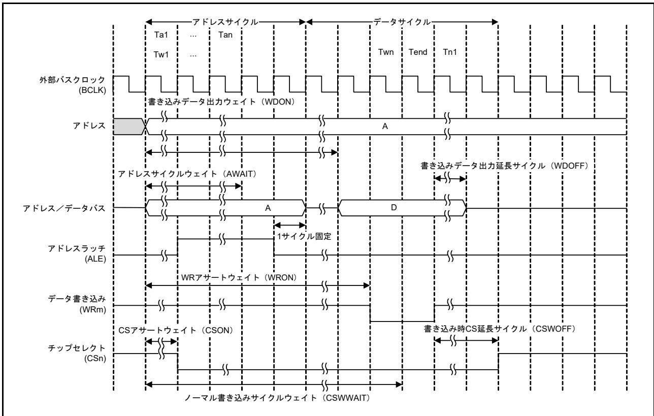
図 15.24 アドレス/データマルチプレクス I/O インタフェース時のライトアクセスの動作例 (m = 0, 1)
