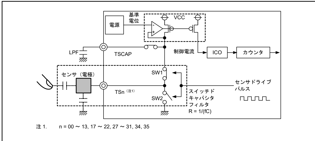
図 44.4 計測部回路
