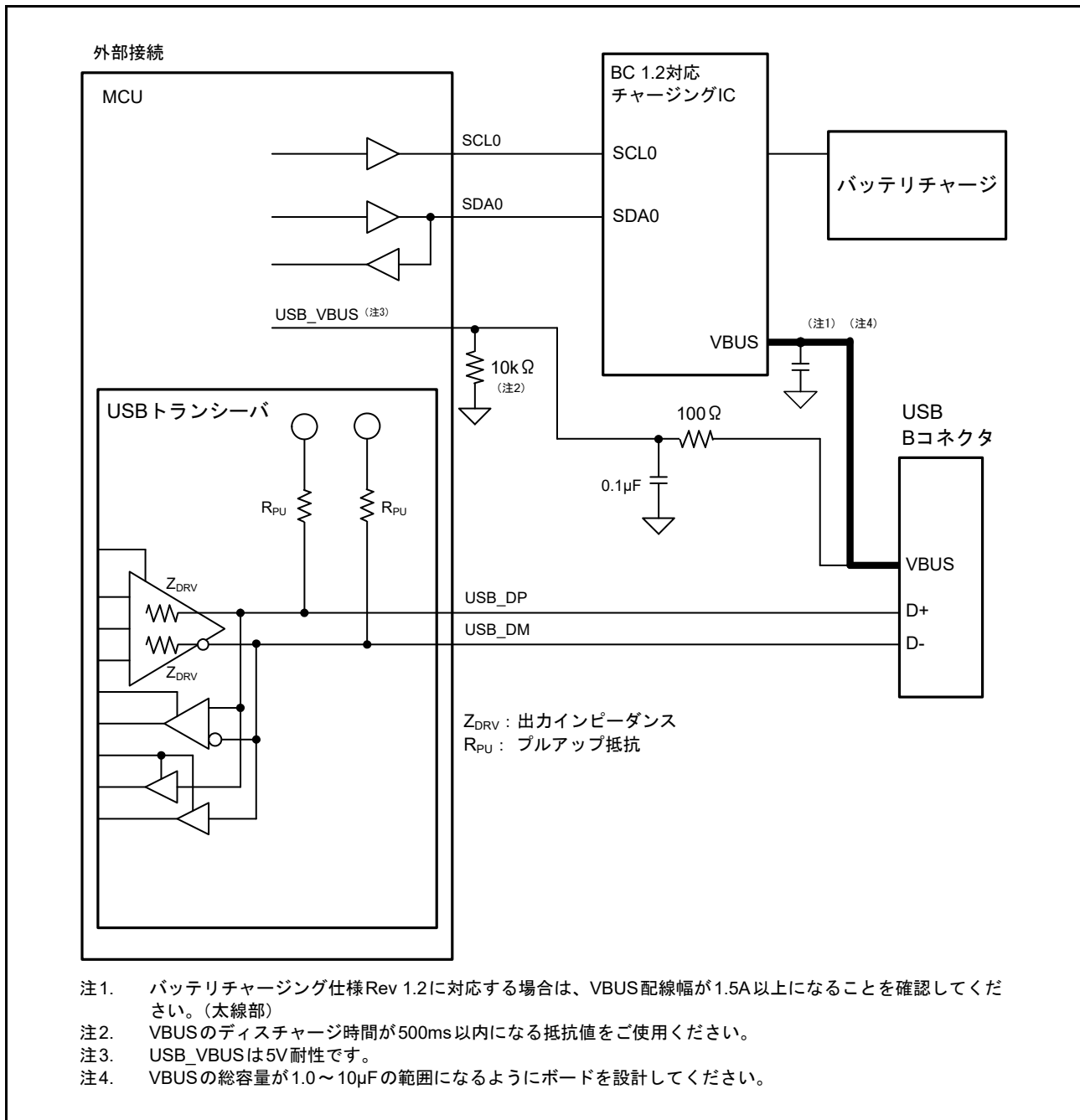
図 28.10 バッテリーチャージング仕様リビジョン 1.2 に対応したファンクション接続例
