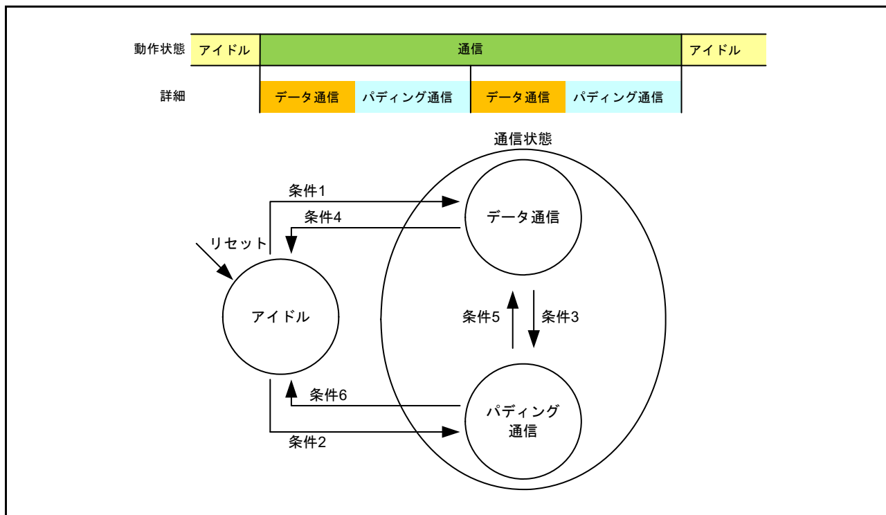
図 35.42 通信の状態遷移
