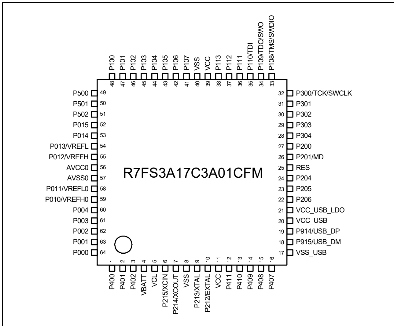
図 1.8 64-pin LQFP のピン配置図 (上面図)
