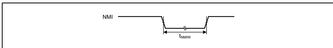
図 50.38 NMI 割り込み入力タイミング
