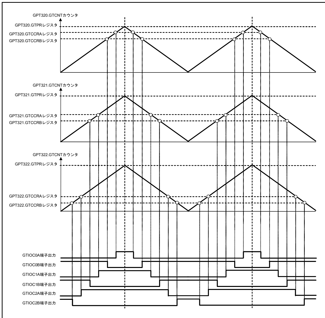
図 23.64 三角波 3 相相補 PWM 出力例
