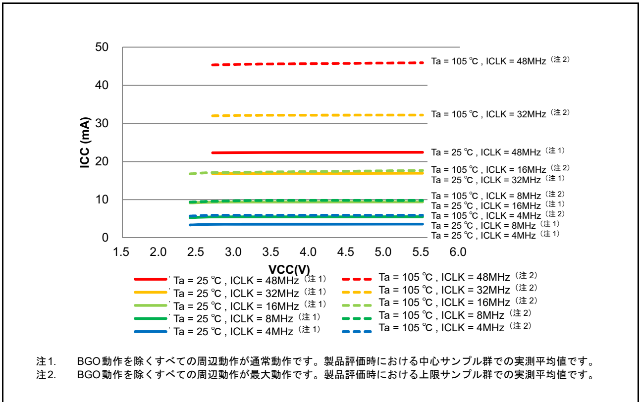
図 50.17 High-speed モードにおける電圧依存性 (参考データ)
