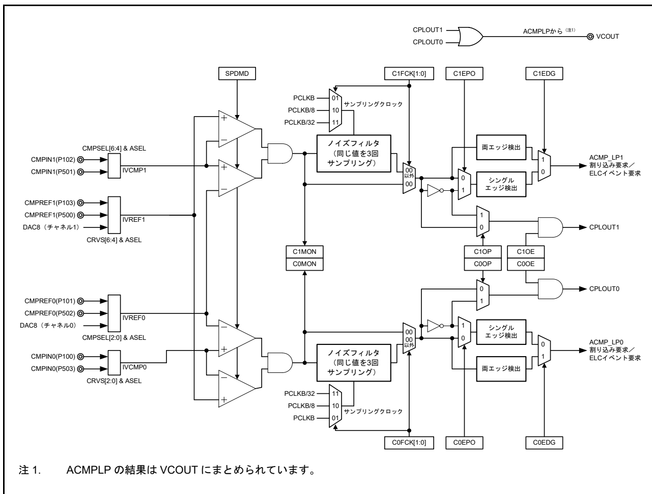
図 42.2 ウィンドウ機能有効時の ACMPLP ブロック図
