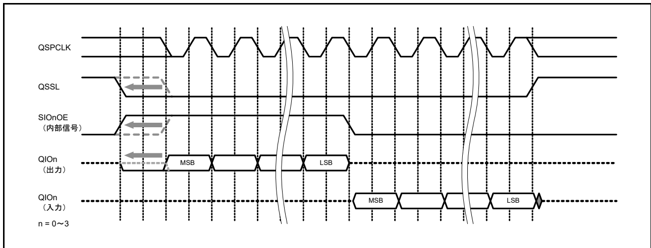
図 33.10 SFMSLD ビットを使用した QSSL 信号のセットアップ時間調整
