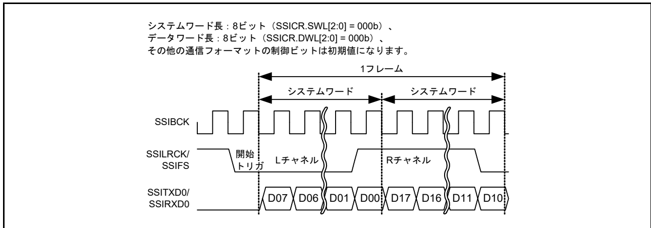
図 35.35 I 2 S フォーマット (パディングなし、システムワード長 = データワード長)
