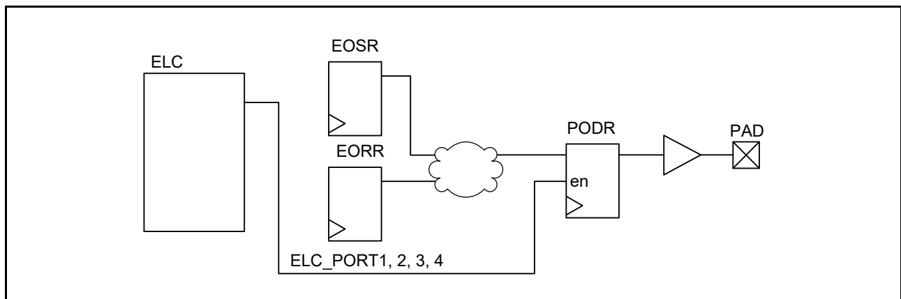
図 20.3 イベントポート出力データ
