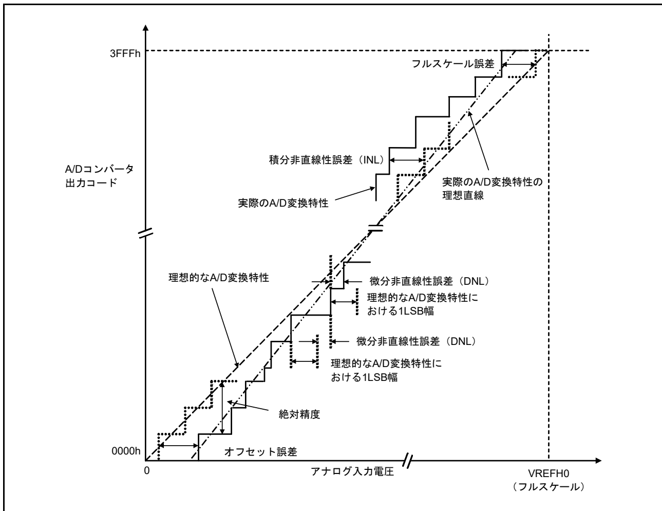
図 50.82 14 ビット A/D コンバータ 特有用語の解説図
