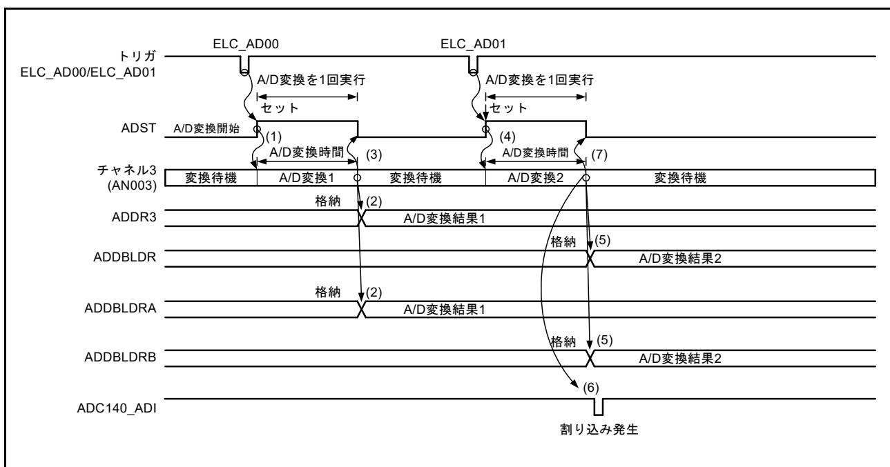
図 38.10 ダブルトリガモードの拡張動作例 (1) (AN003 を2重化選択および ELC_AD00/ELC_AD01 選択)
