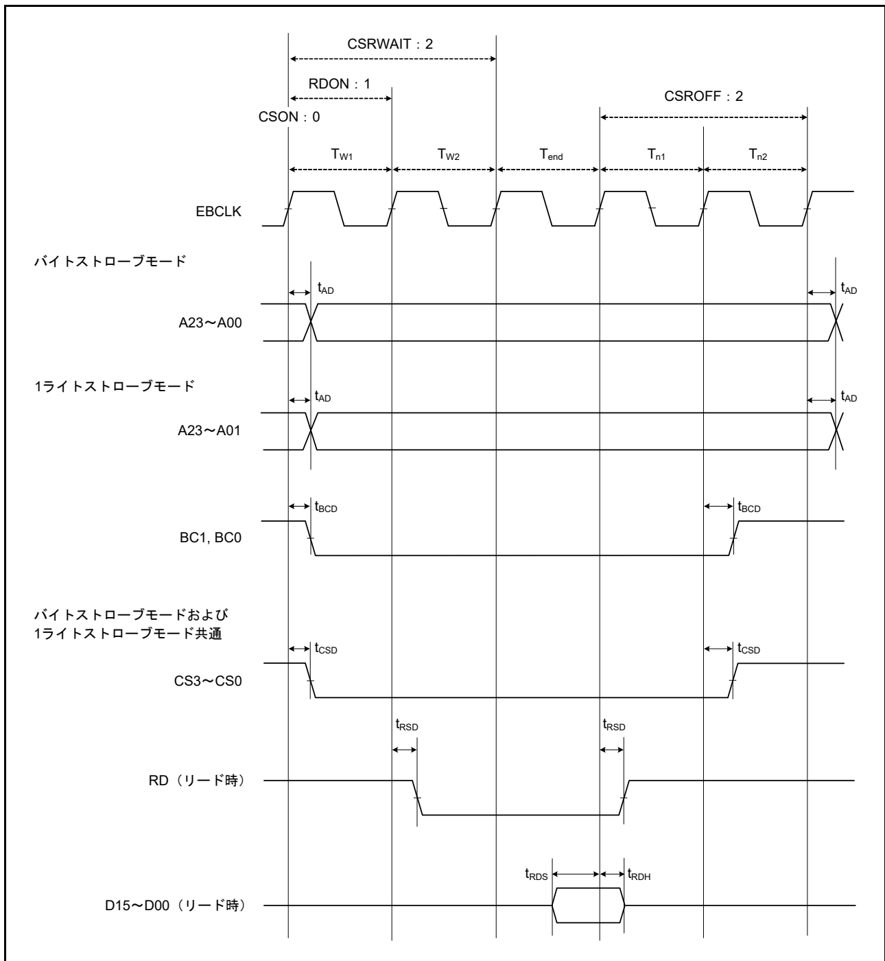
図 50.42 外部バスタイミング/ノーマルリードサイクル (バスクロック同期)
