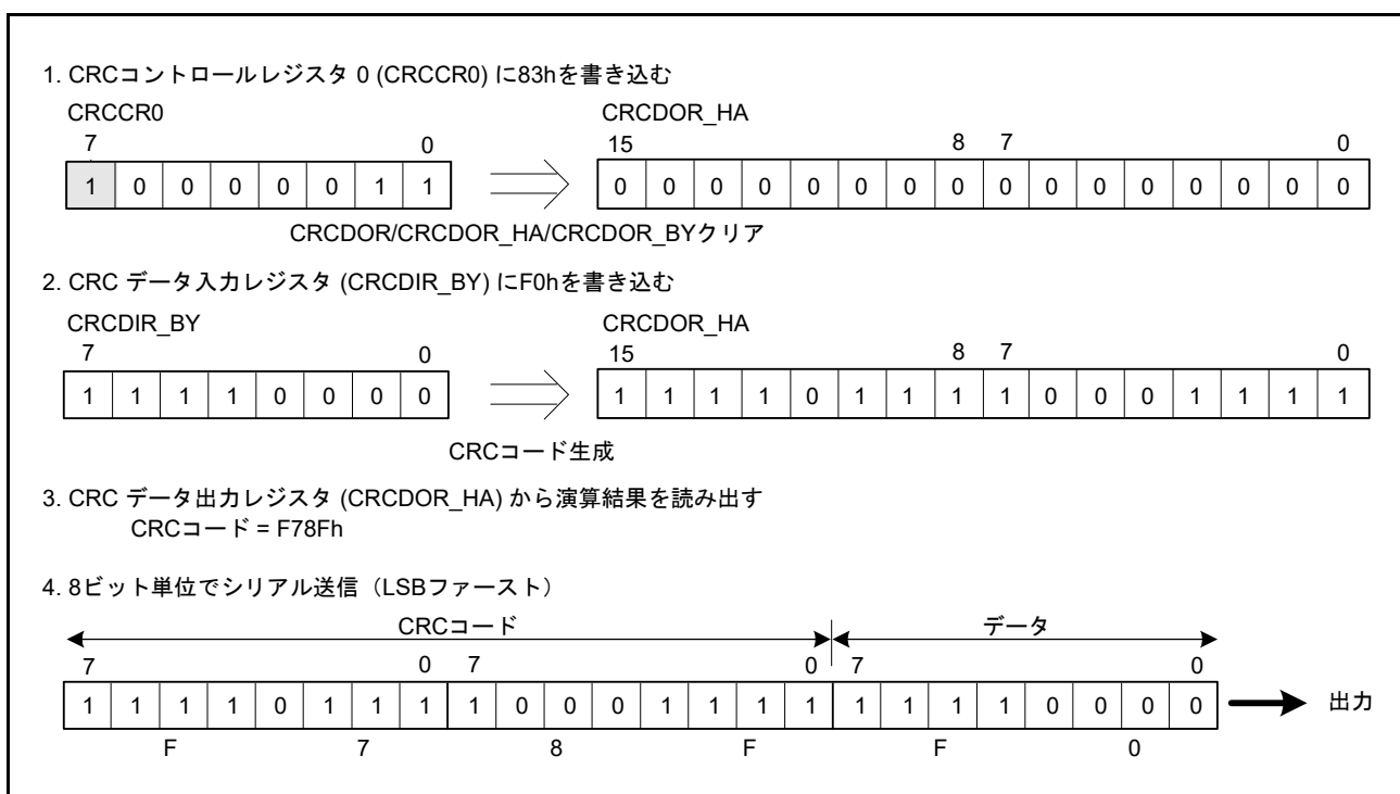
図 34.2 LSB ファーストのデータ送信
