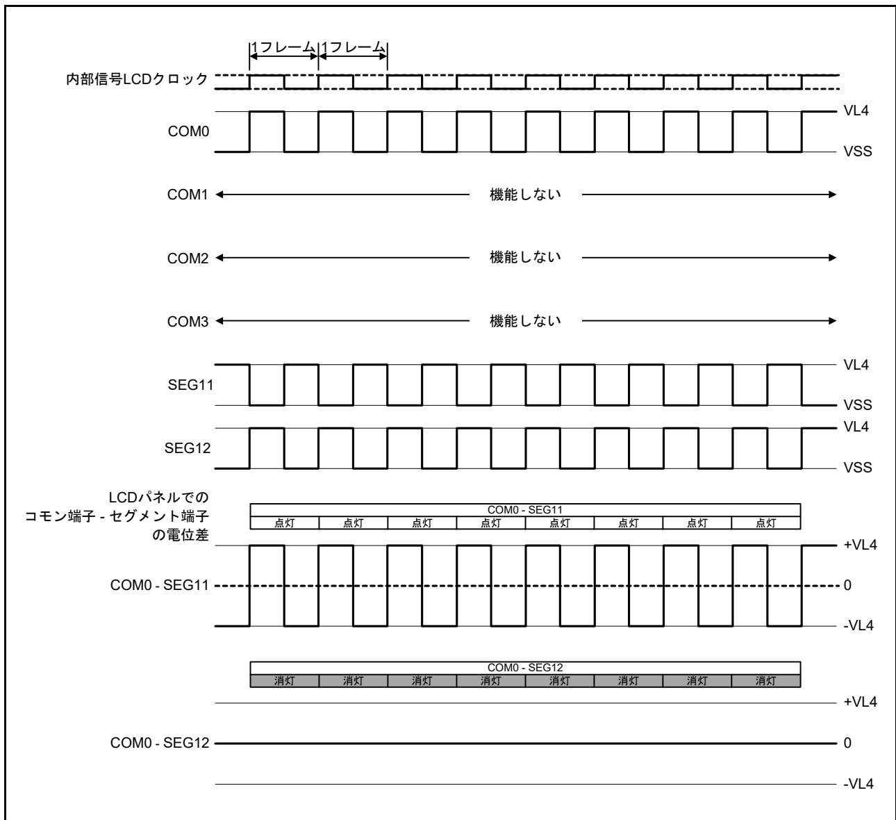
図 48.20 SEG11、SEG12、COM0 のスタティック LCD 駆動波形例
