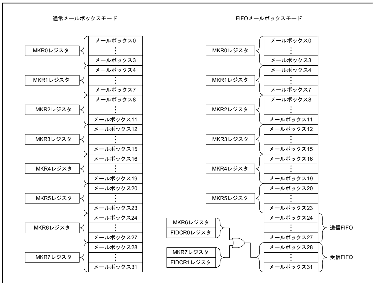
図 31.16 マスクレジスタとメールボックスの関係
