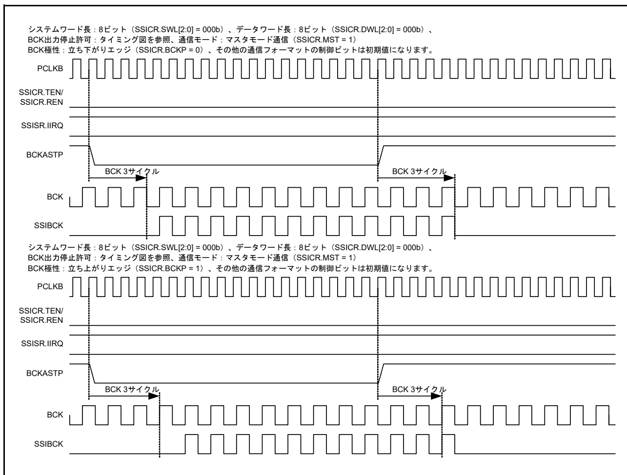
図 35.32 BCKASTP ビットの動作例 (アイドル状態の場合)
