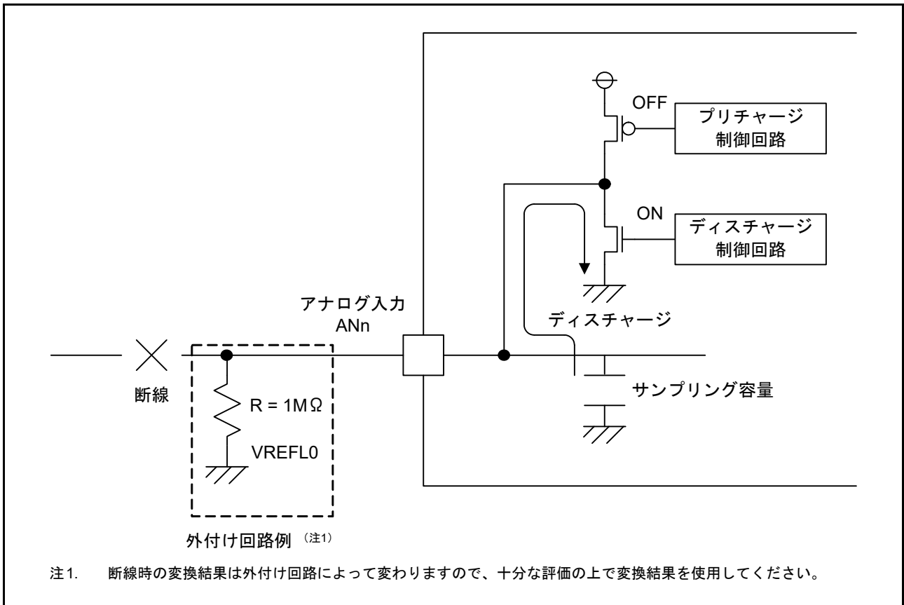
図 38.28 ディスチャージを選択した場合の断線検出例
