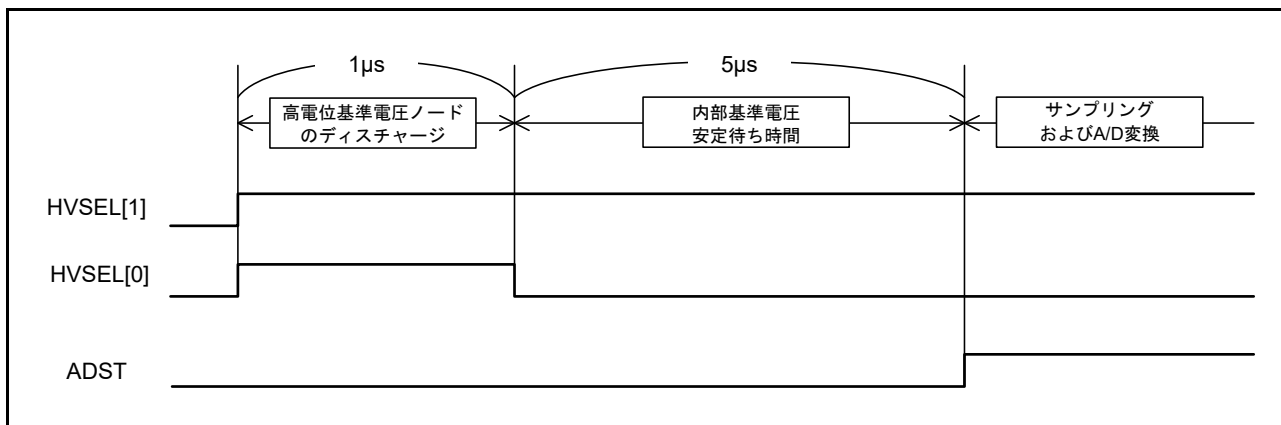
図 38.30 高電位基準電圧に内部基準電圧を選択する手順
