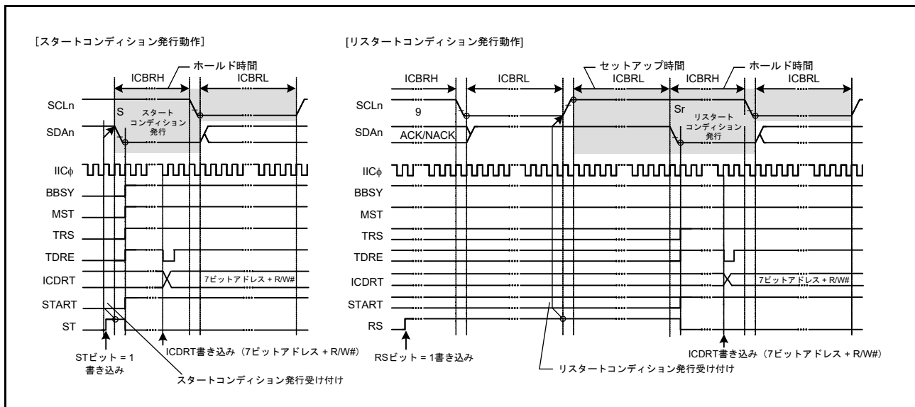
図 30.45 スタートコンディション/リスタートコンディション発行動作タイミング (ST、RS ビット使用)
