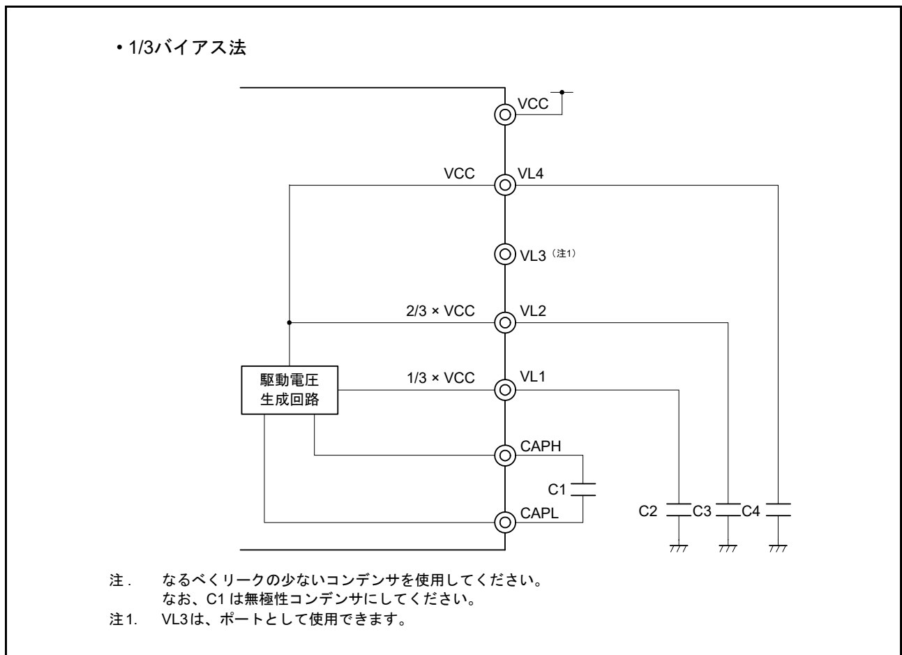
図 48.12 LCD 駆動電源の接続例 (容量分割方式)
