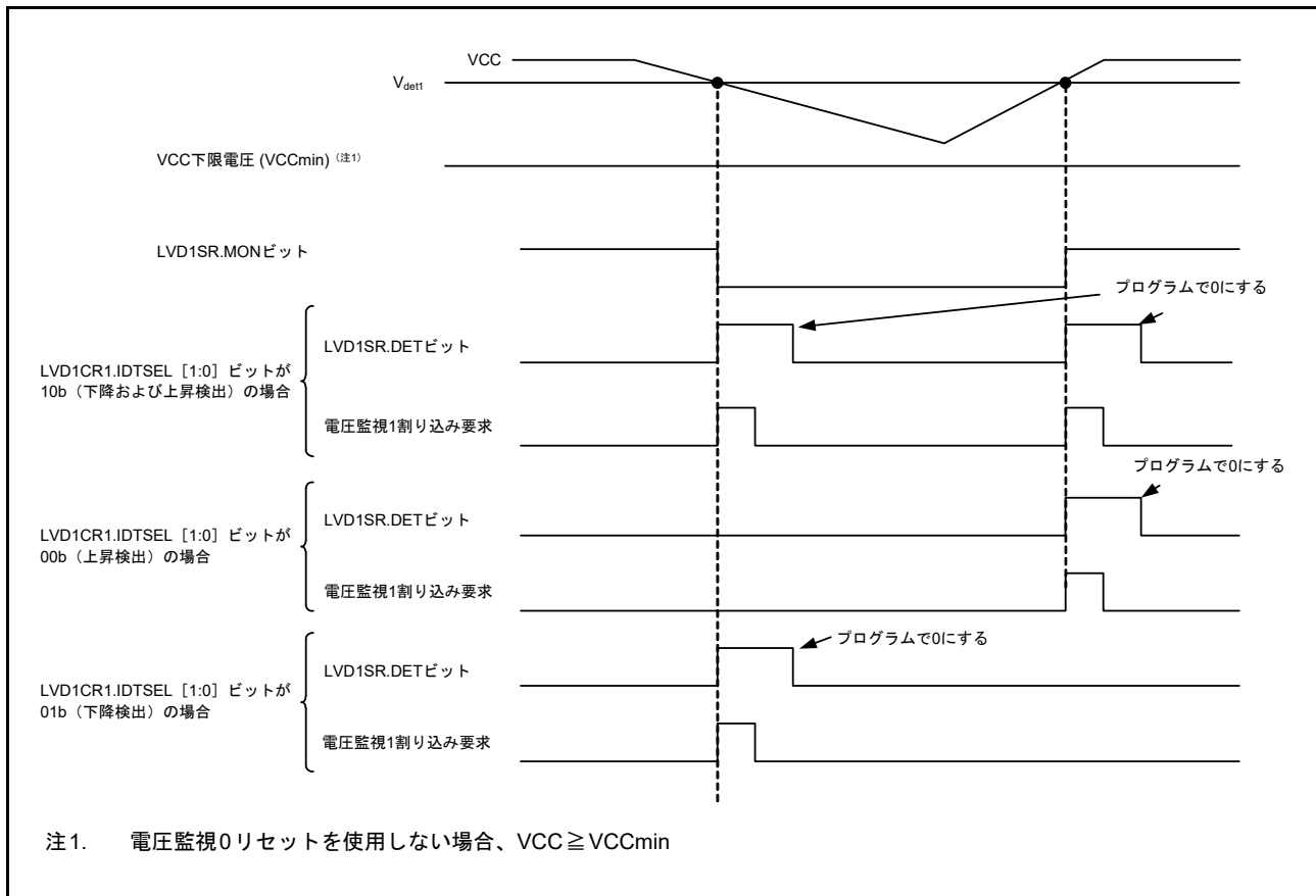
図 8.5 電圧監視 1 割り込みの動作例
