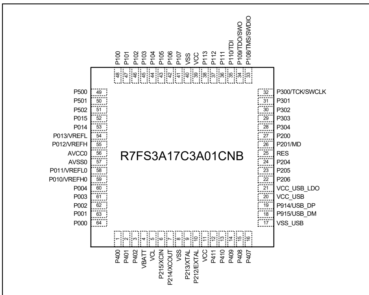
図 1.9 64-pin QFN のピン配置図 (上面図)
