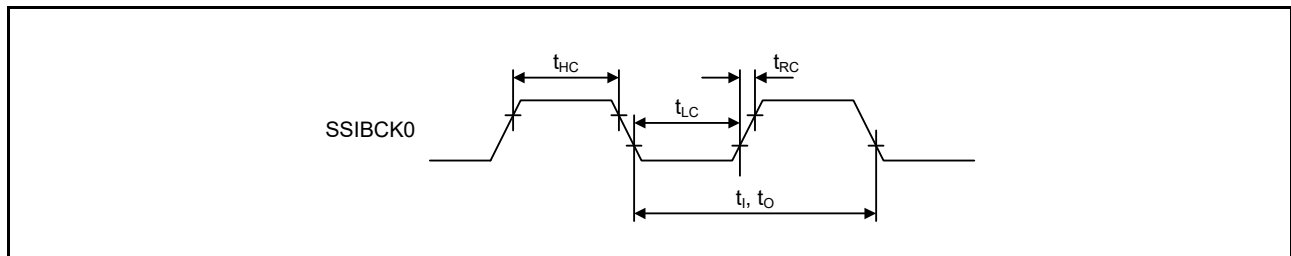
図 50.71 SSIE クロック入出力タイミング
