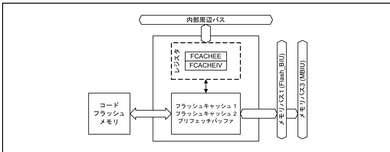
図 47.4 FCACHE のブロック図
