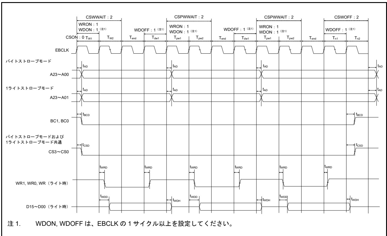
図 50.45 外部バスタイミング/ページライトサイクル (バスクロック同期)
