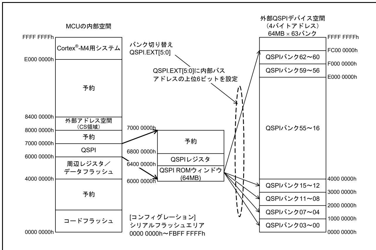
図 33.2 デフォルト領域設定および AHB 空間メモリマップ
