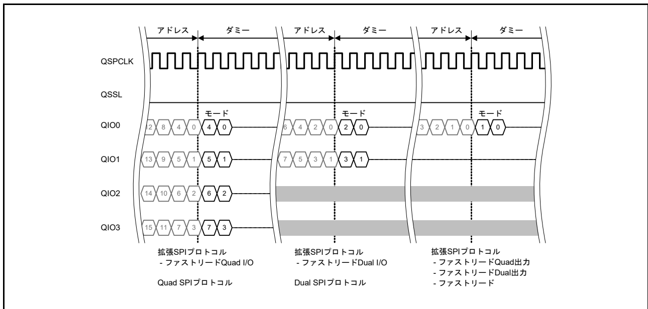
図 33.33 XIP モード制御データ
