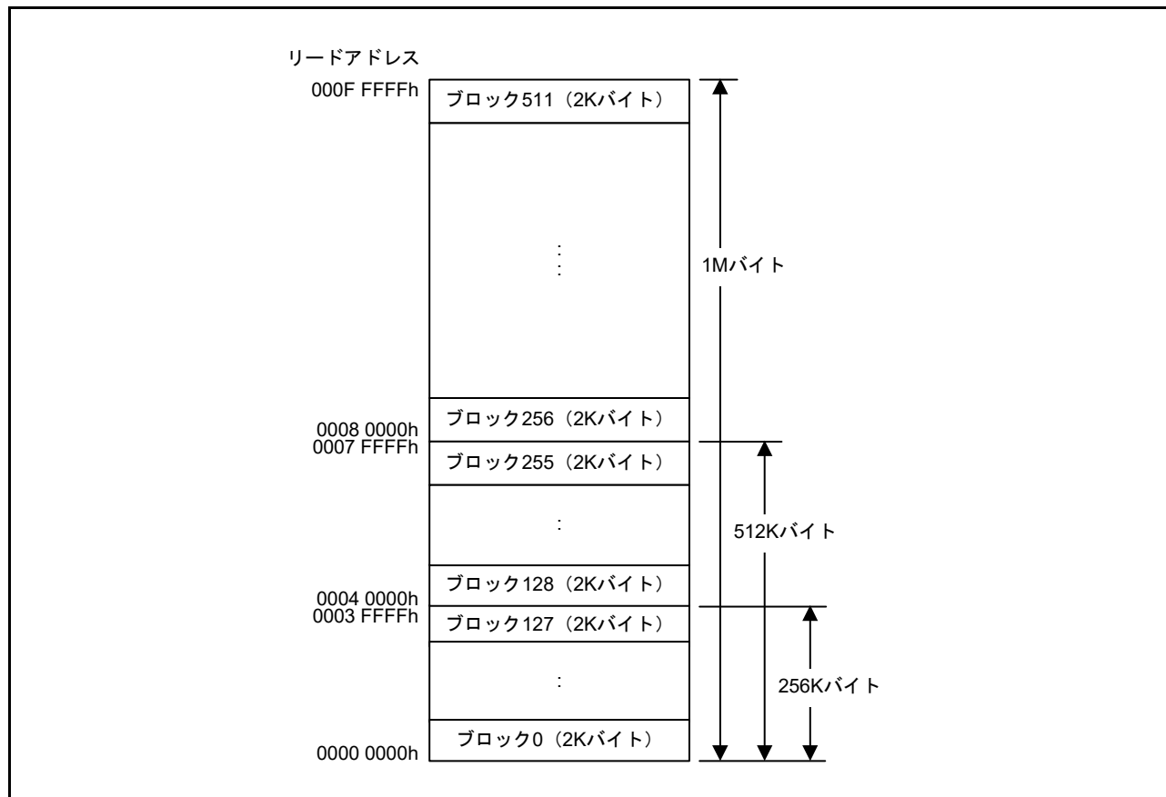
図 47.2 コードフラッシュメモリマッピング
