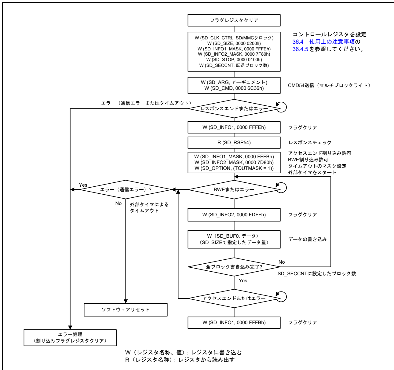
図 36.15 外付けタイマによるマルチブロックライト動作のフロー例
