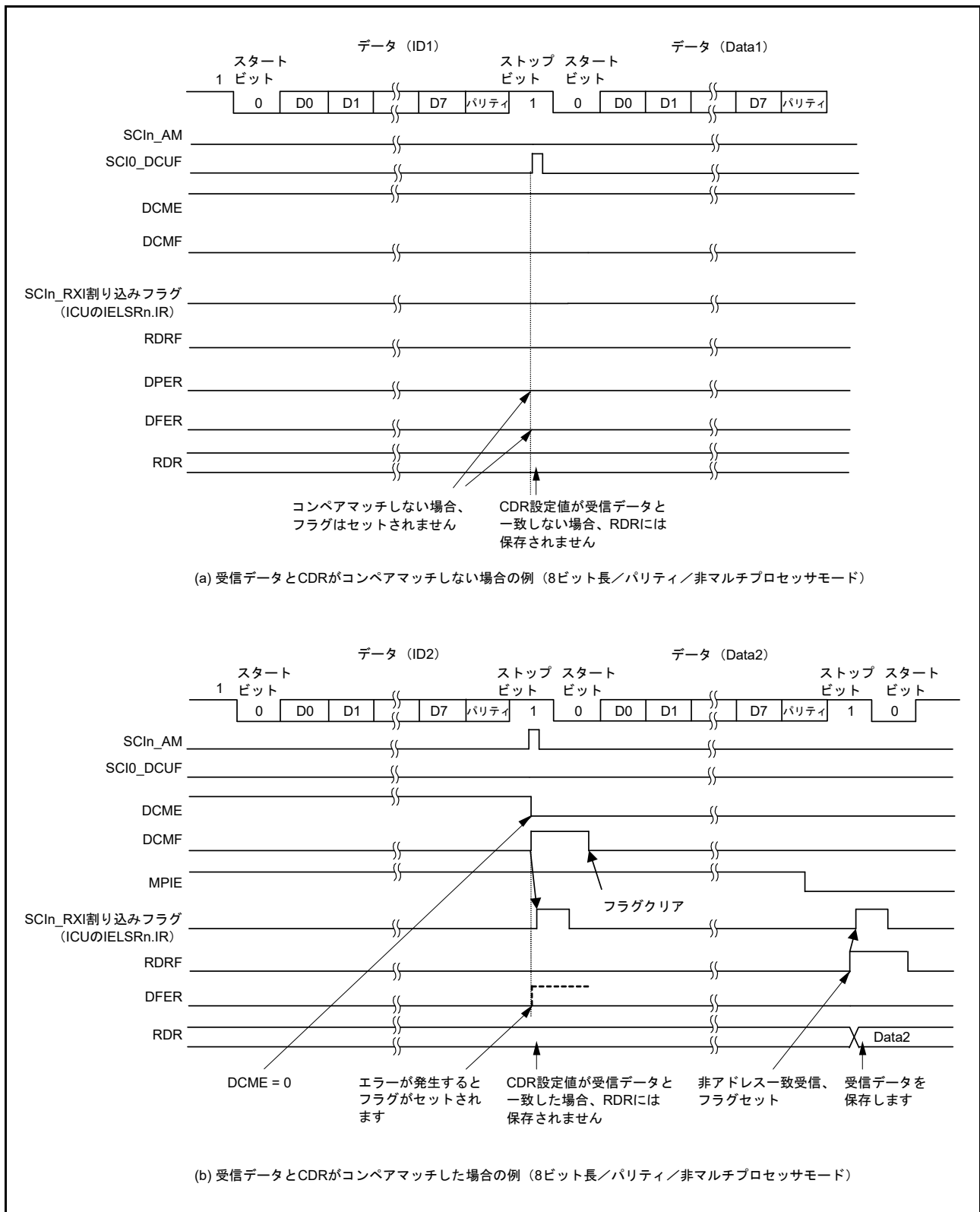
図 29.5 アドレス一致検出の例 (1) (非マルチプロセッサモード)
