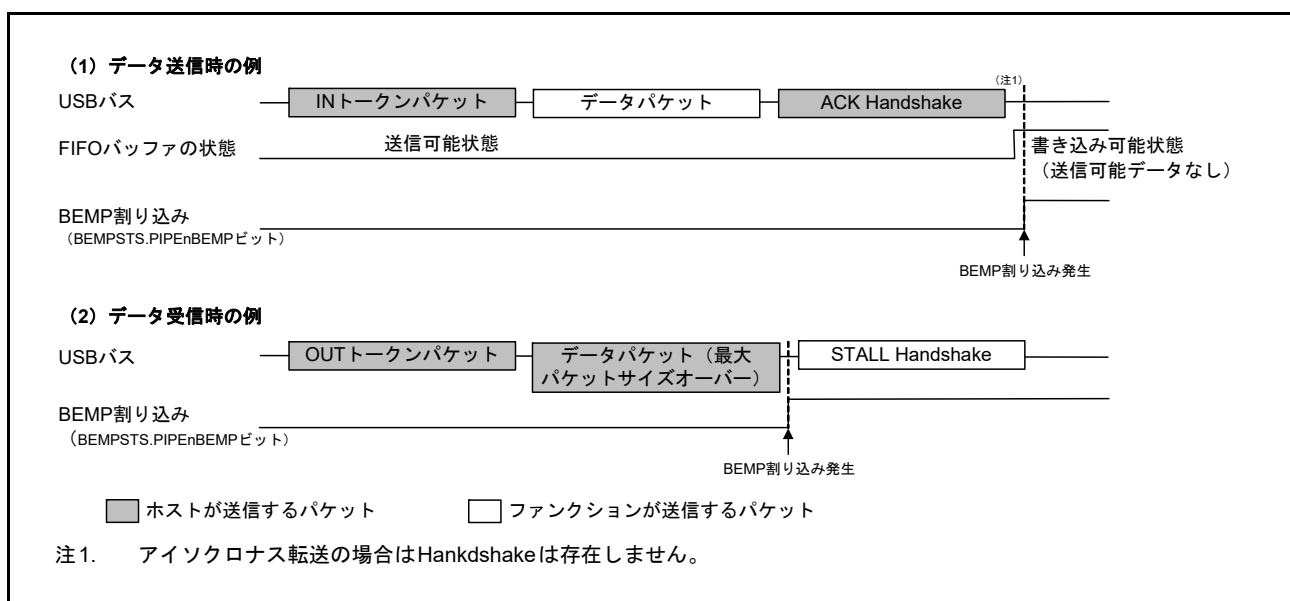
図 28.14 デバイスコントローラモード時の BEMP 割り込みの発生タイミング
