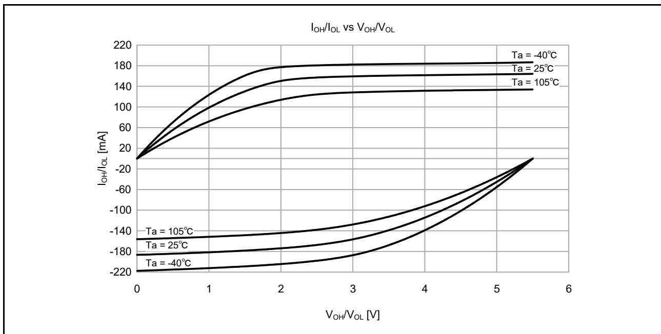
図 50.15 中駆動出力選択時の VCC = 5.5V での V_{OH}/V_{OL} および I_{OH}/I_{OL} 温度特性 (参考データ)
