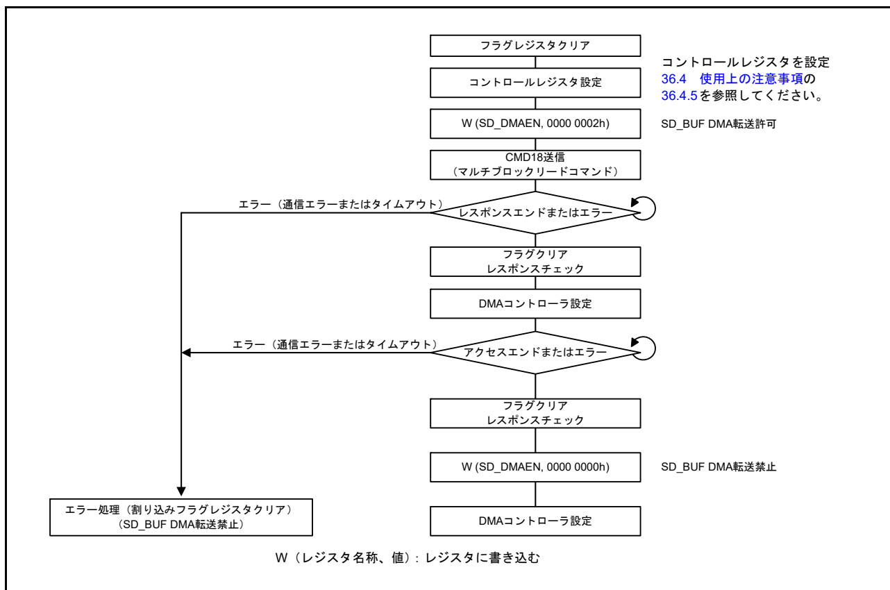
図 36.23 SD_BUF DMA リード動作の例
