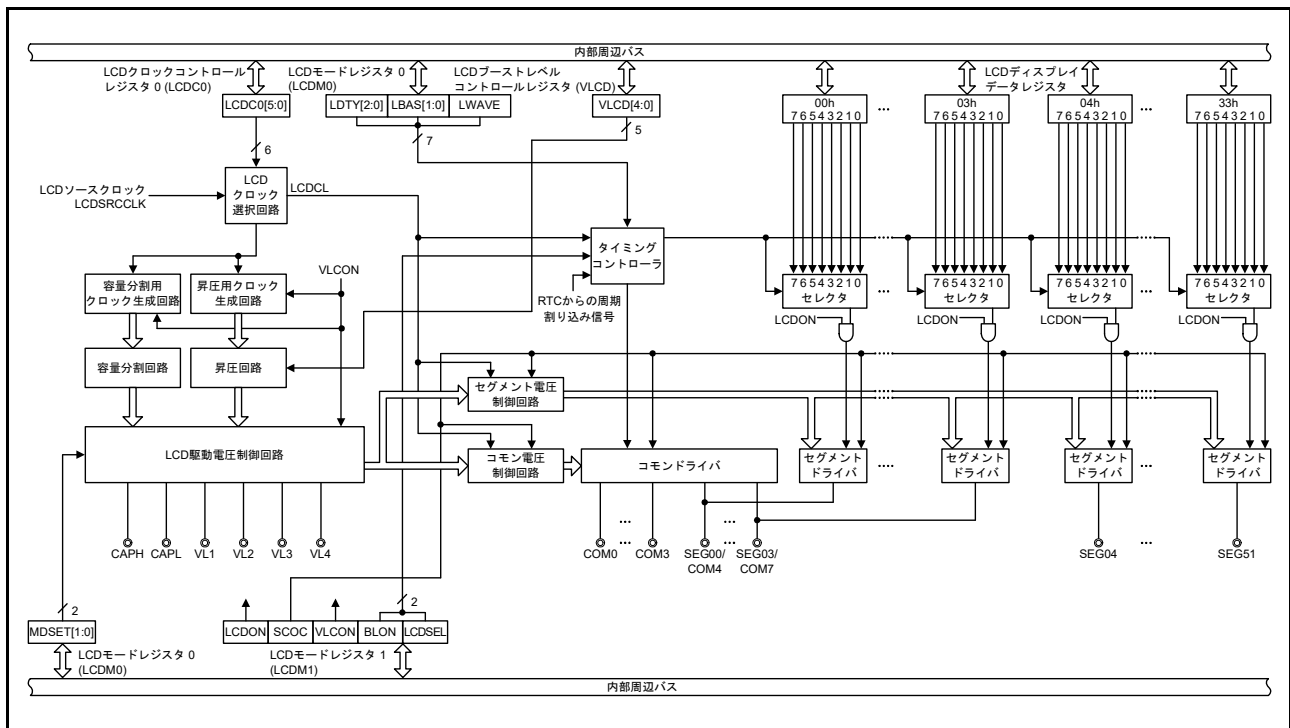
図 48.1 SLCDC のブロック図
