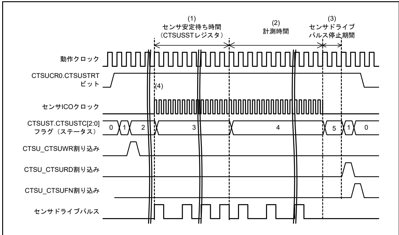
図 44.18 センサ安定待ちと計測のタイミング
