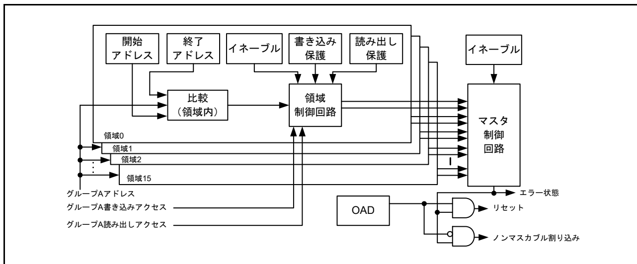
図 16.4 バスマスタ MPU のグループ A
