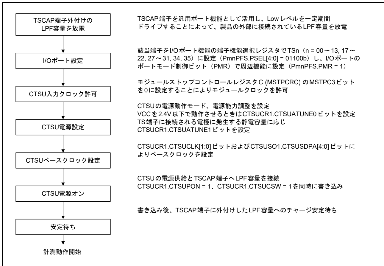
図 44.9 CTSUS 初期設定フロー
