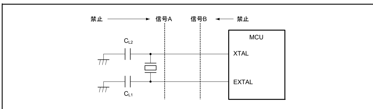
図 9.8 発振回路部のボード設計での信号ルーティング (メインクロック発振器の場合、サブクロック発振器も同様)
