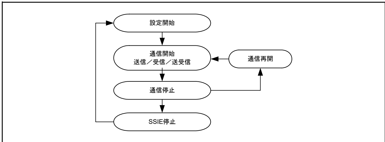
図 35.48 SSIE 通信動作
