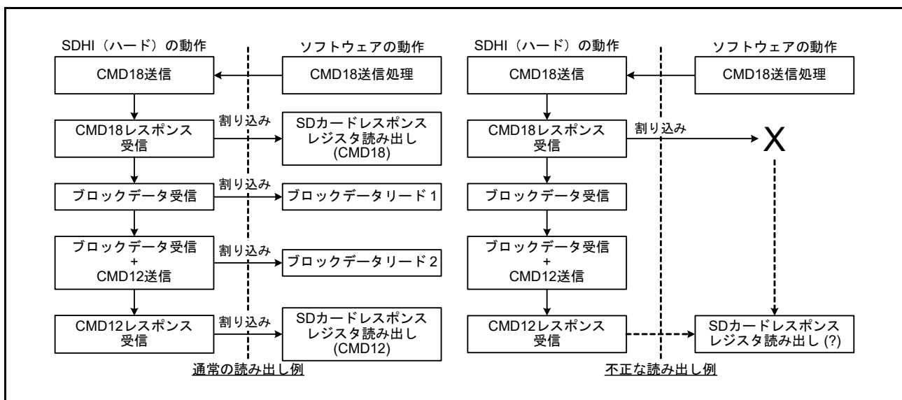
図 36.25 マルチブロックリード動作のフローチャート (2 ブロック)
