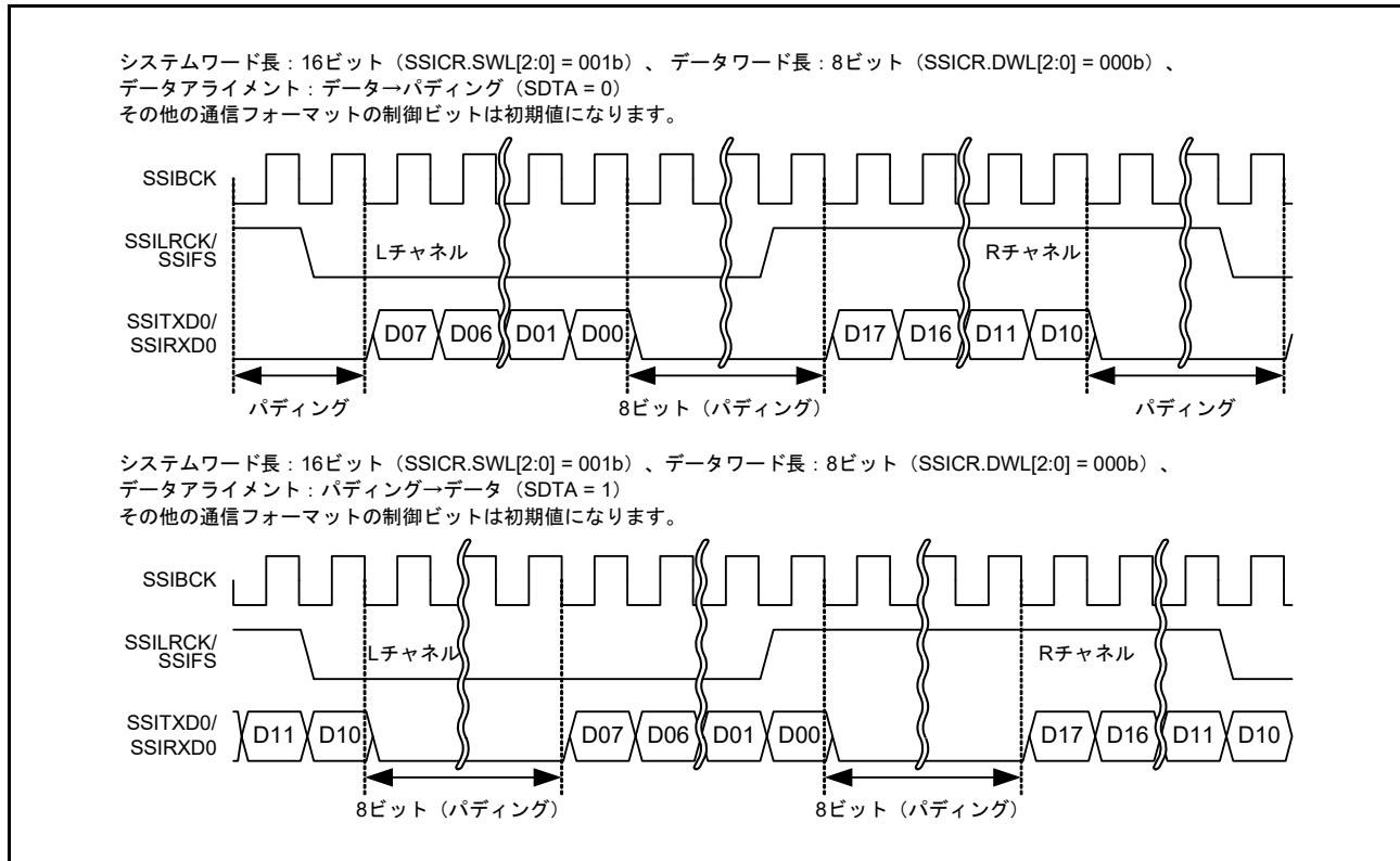
図 35.9 パディングビットのあるシリアルデータのアライメント設定
