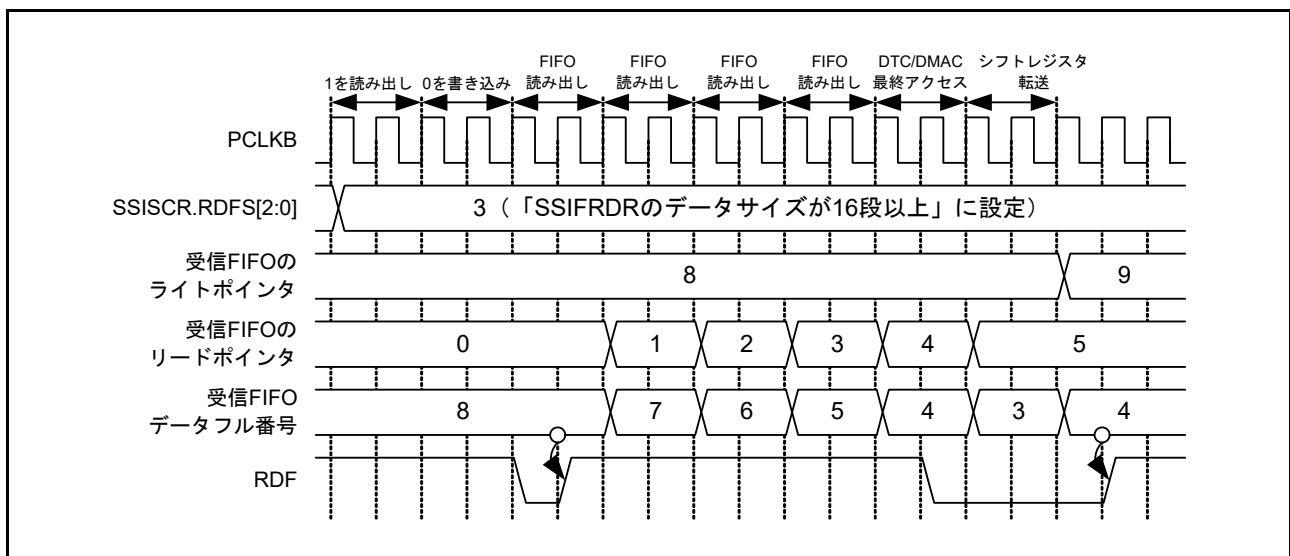
図 35.26 RDF の設定およびクリアのタイミング図
