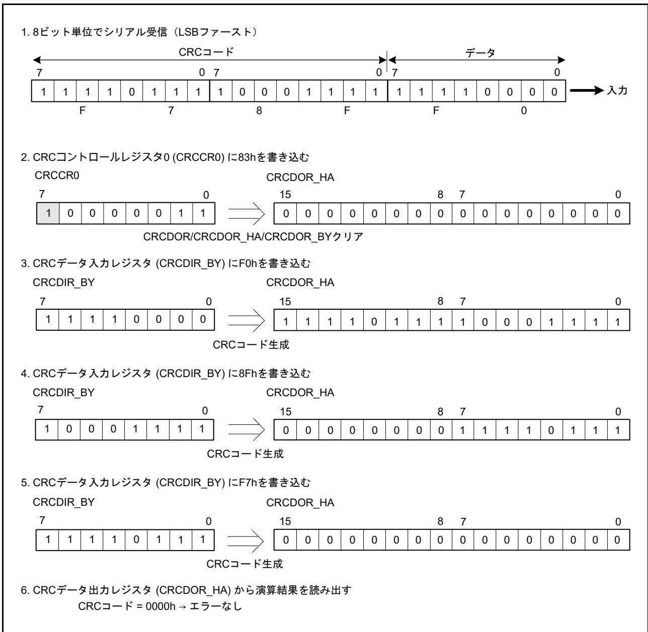
図 34.4 LSB ファーストのデータ受信
