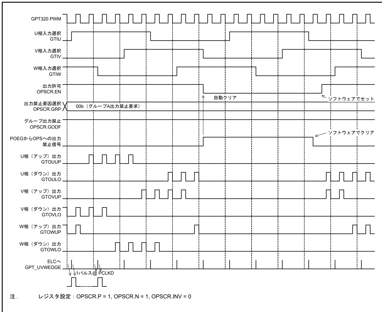
図 23.80 グループ出力禁止制御動作例
