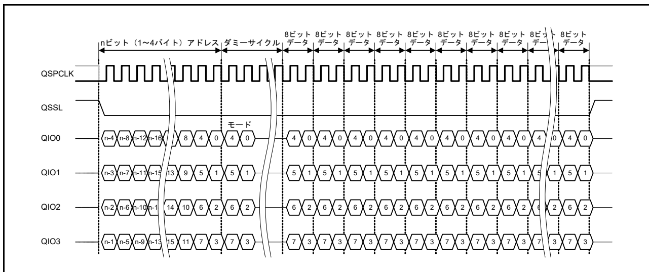
図 33.26 XIP モード時のファストリード Quad I/O バスサイクル
