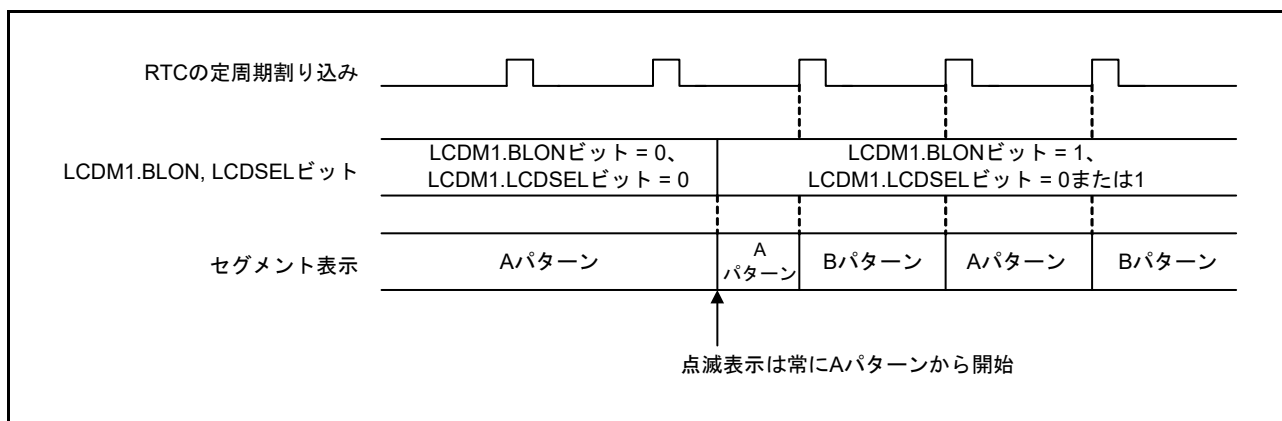
図 48.3 Aパターン表示から点滅表示への切り替え動作
