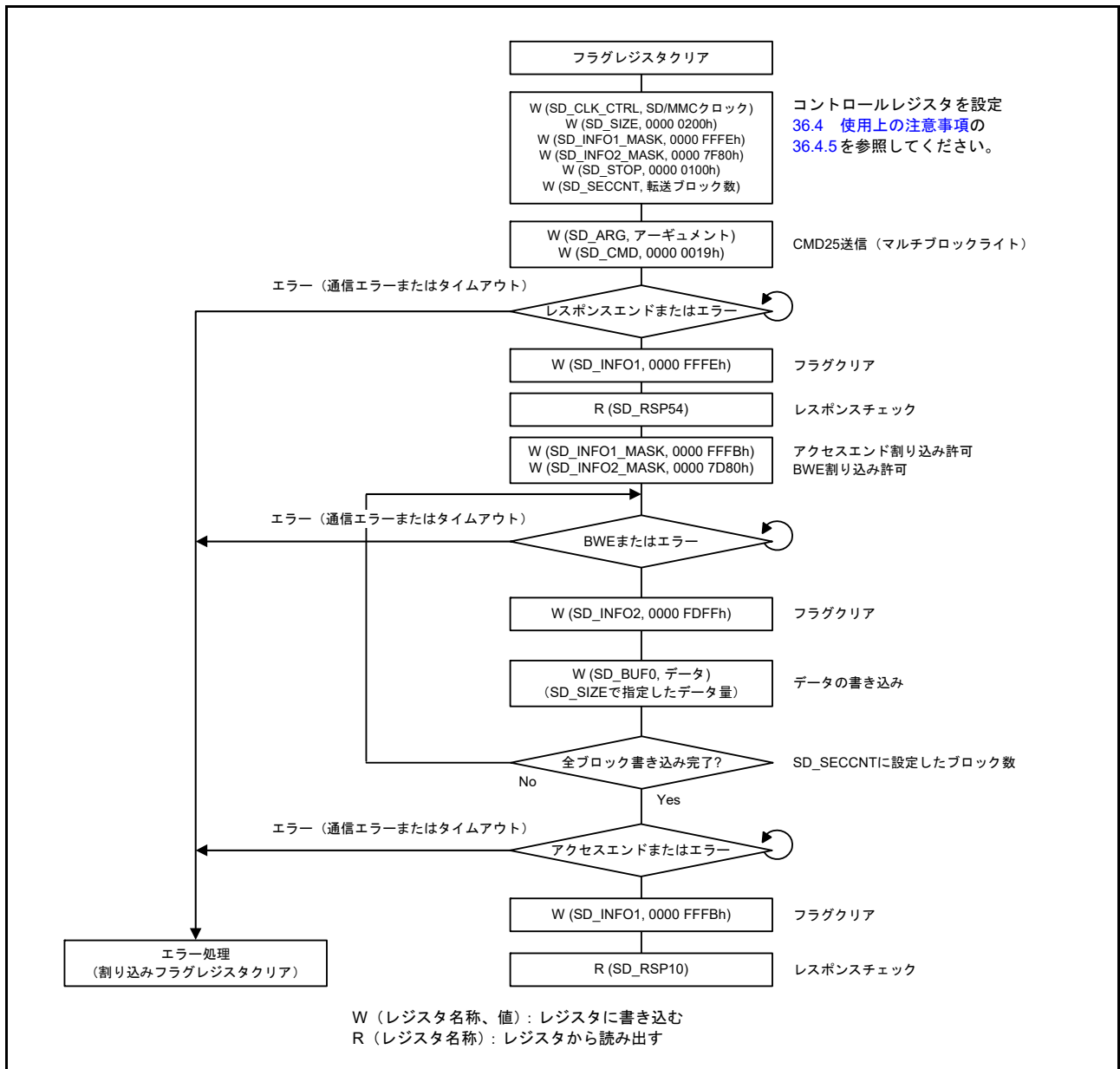
図 36.14 内蔵タイマによるマルチブロックライト動作のフロー例
