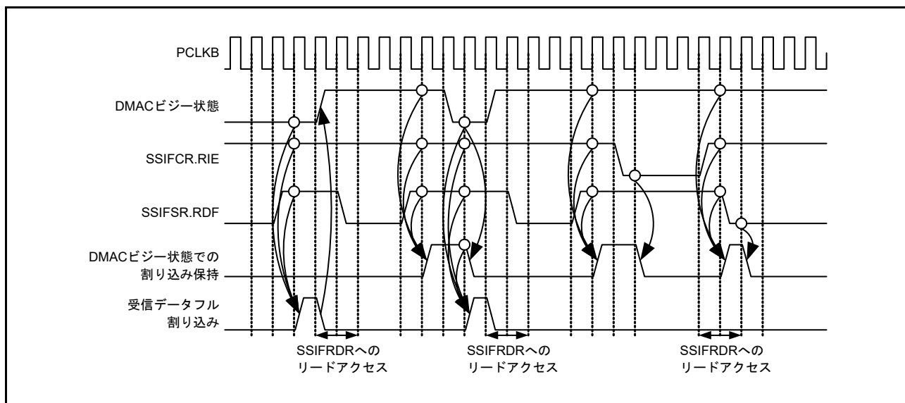
図 35.20 受信データフル割り込みのタイミング
