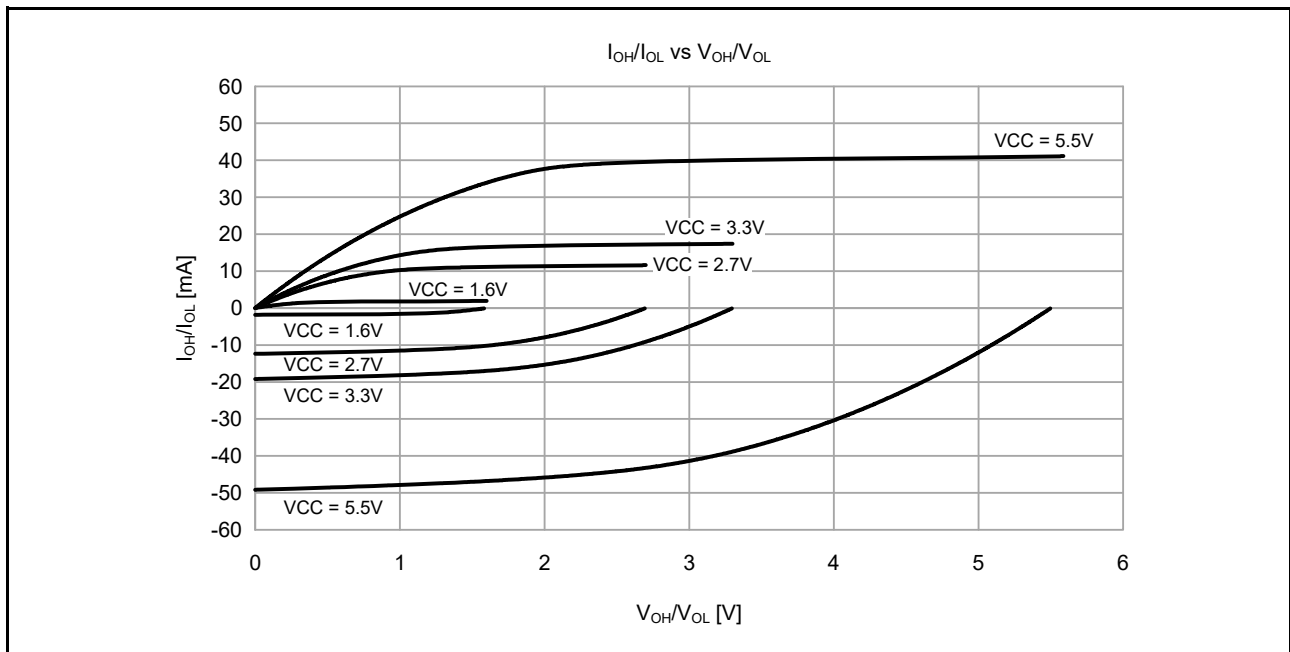
図 50.2 低駆動出力選択時の Ta = 25 °Cでの V OH /V OL および I OH /I OL 電圧特性 (参考データ)
