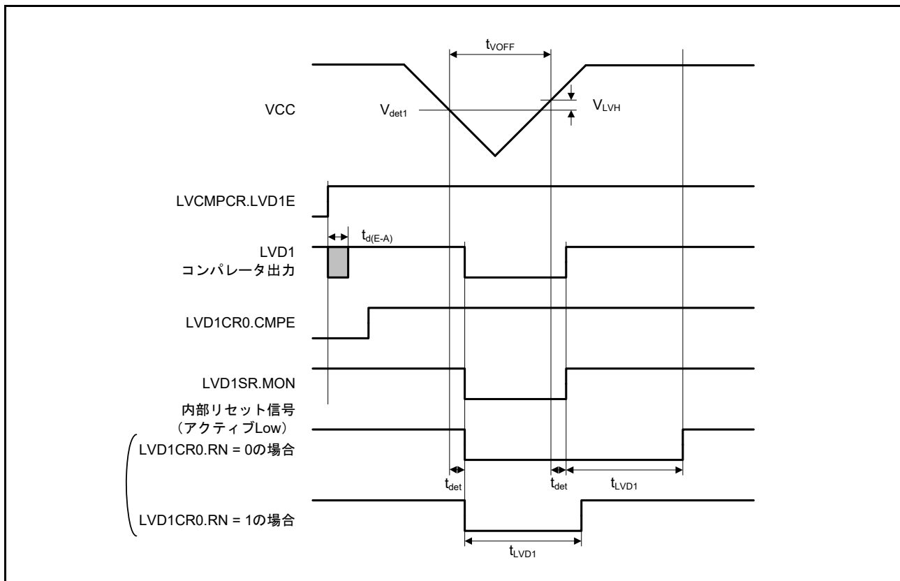
図 50.88 電圧検出回路タイミング ( V_{det1} )
