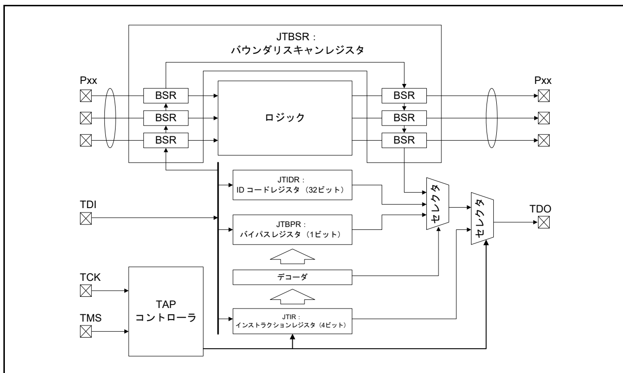
図 37.1 バウンダリスキャン機能のブロック図
