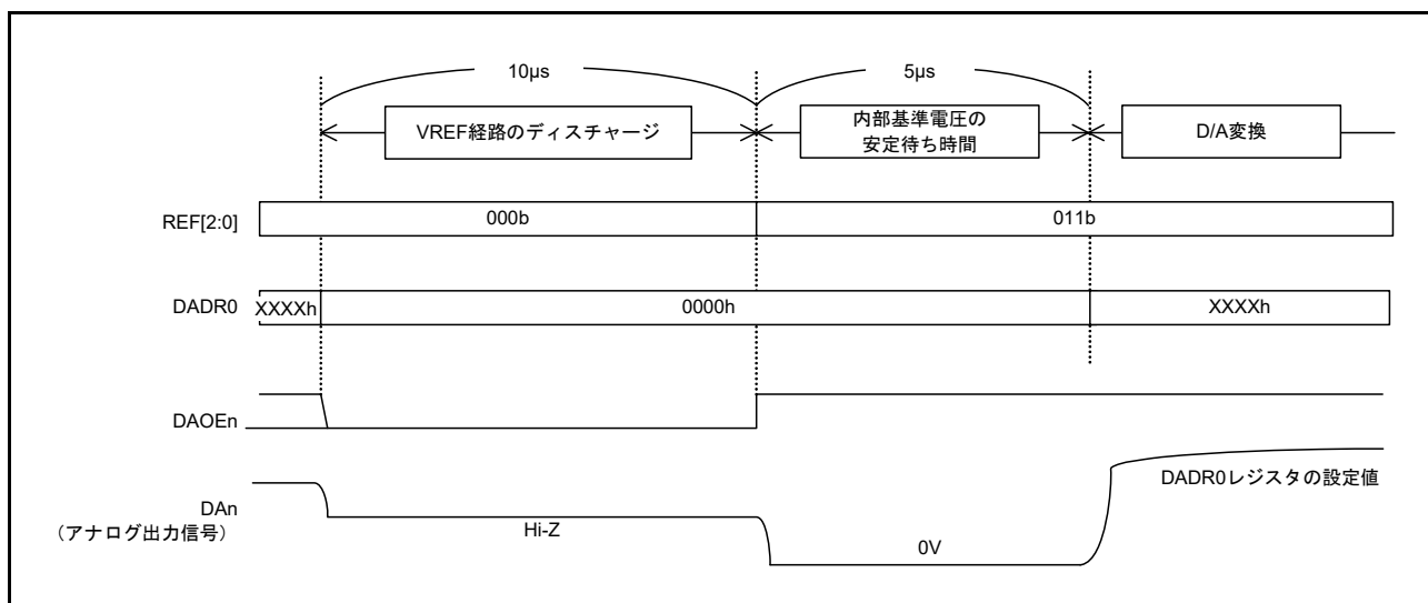
図 39.5 内部基準電圧を基準電圧に選択する手順
