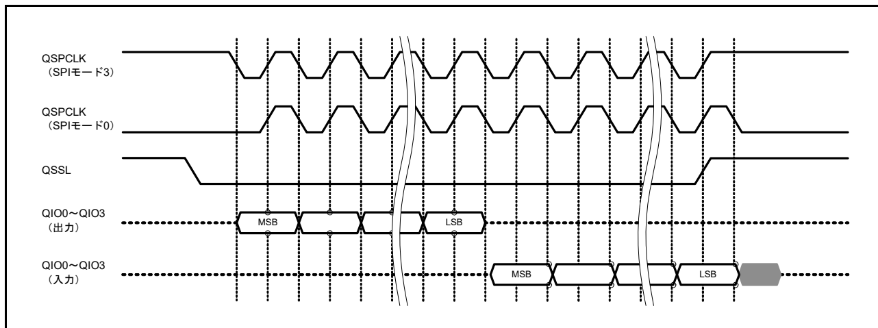
図 33.8 シリアルインタフェースの基本タイミング
