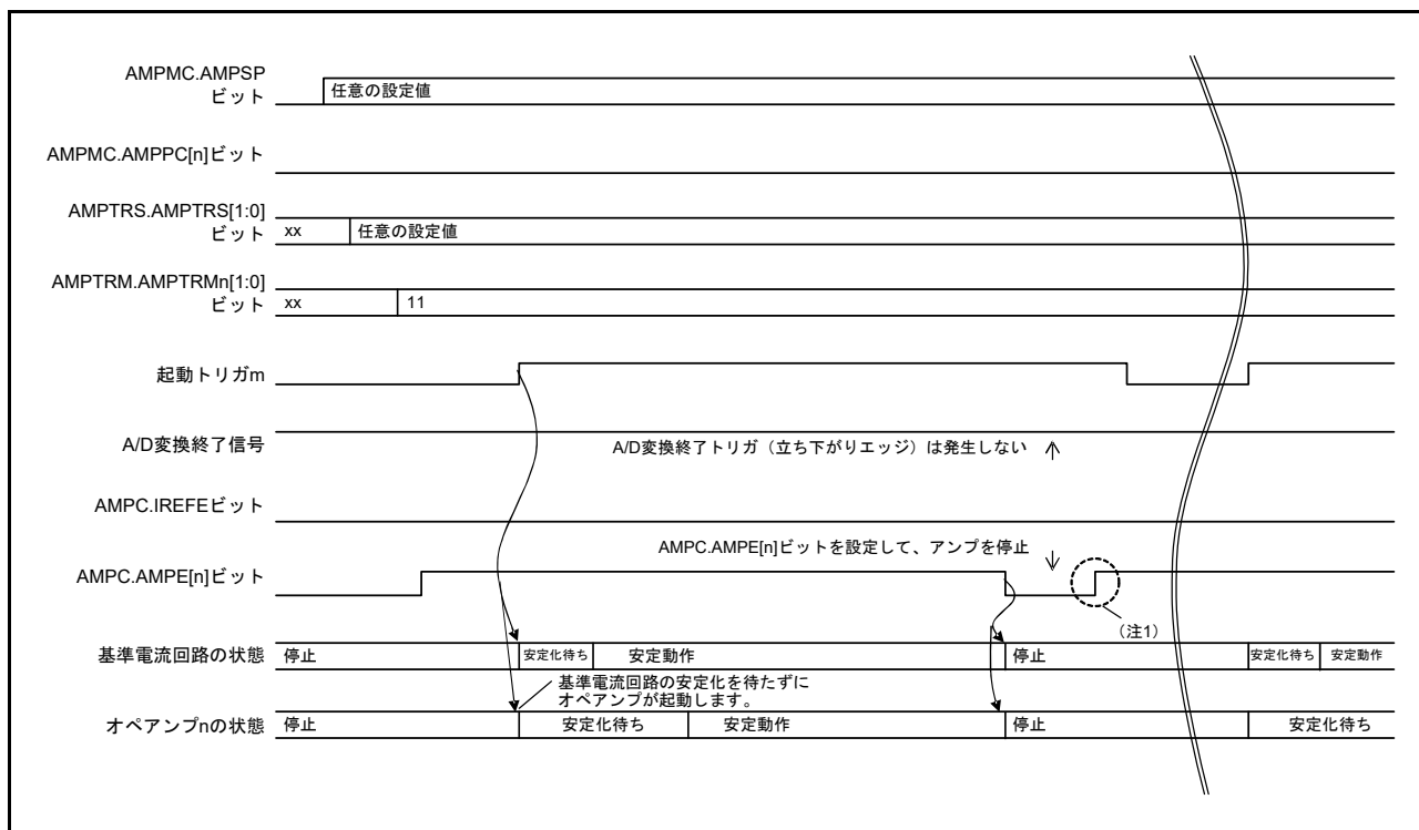
図 41.6 オペアンプの制御動作 (起動および A/D トリガモード (2)) (基準電流回路およびオペアンプを起動トリガによって起動し、AMPC レジスタの設定によって基準電流回路およびオペアンプを停止する場合)
