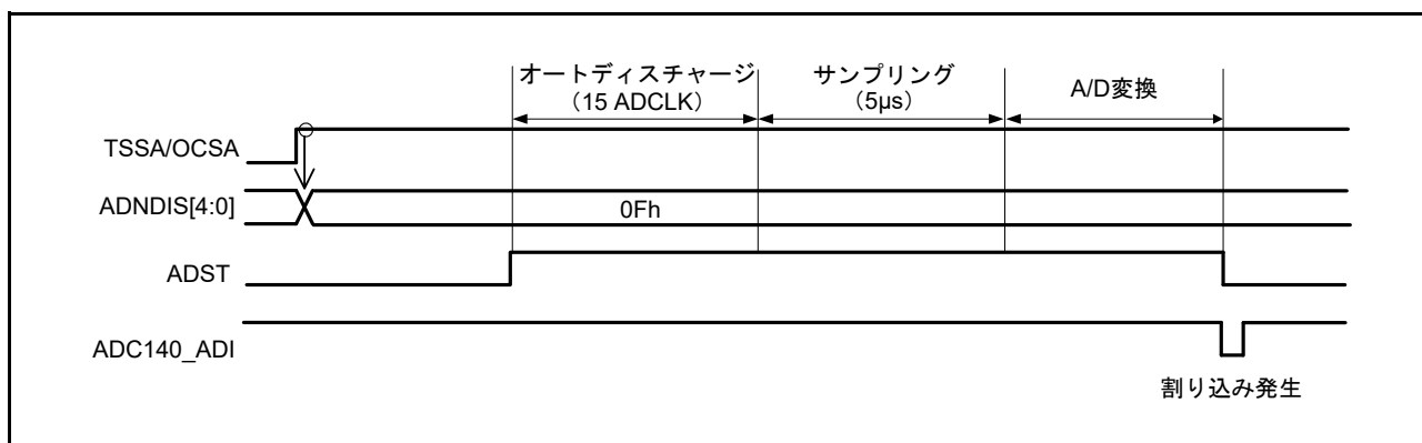
図 38.8 シングルスキャンモードの基本動作例 (AN000、温度センサ出力または内部基準電圧選択)
