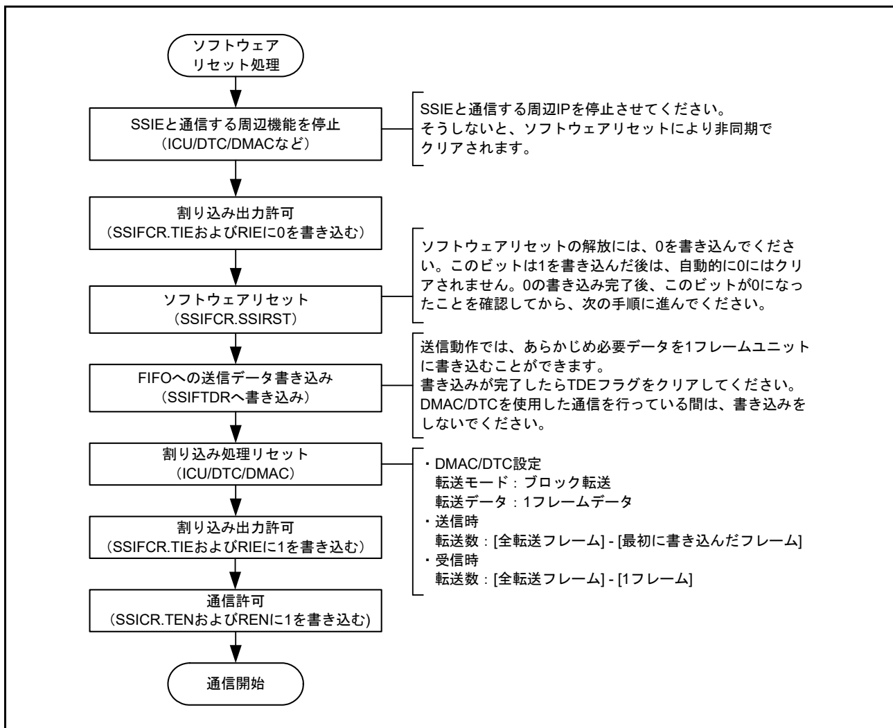
図 35.57 ソフトウェアリセット手順 (CPU 動作)
