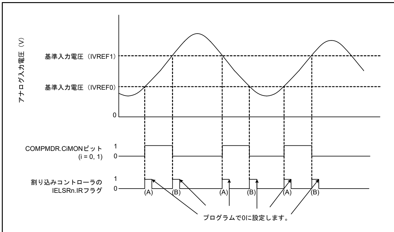
図 42.4 ウィンドウ機能有効時の ACMPLP i (i = 0, 1) の動作例
