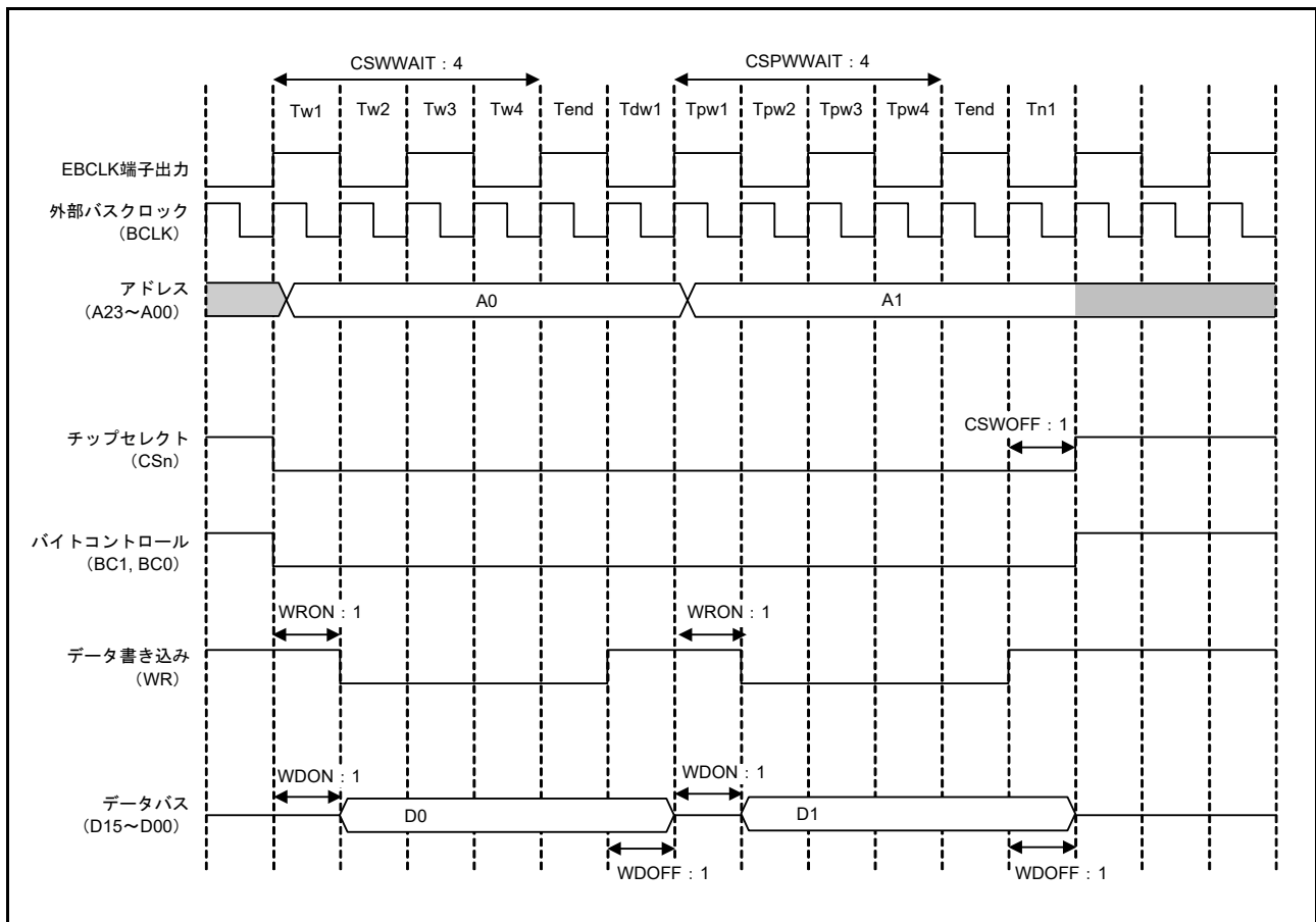
図 15.22 1 ライトストロブモード時のページライトアクセスの動作例 (EBCLK 端子出力選択ビットで BCLK の 2 分周を選択した場合、および 1 転送要求に対して 2 回バスアクセスが発生する場合) (n = 0 ~ 3)
