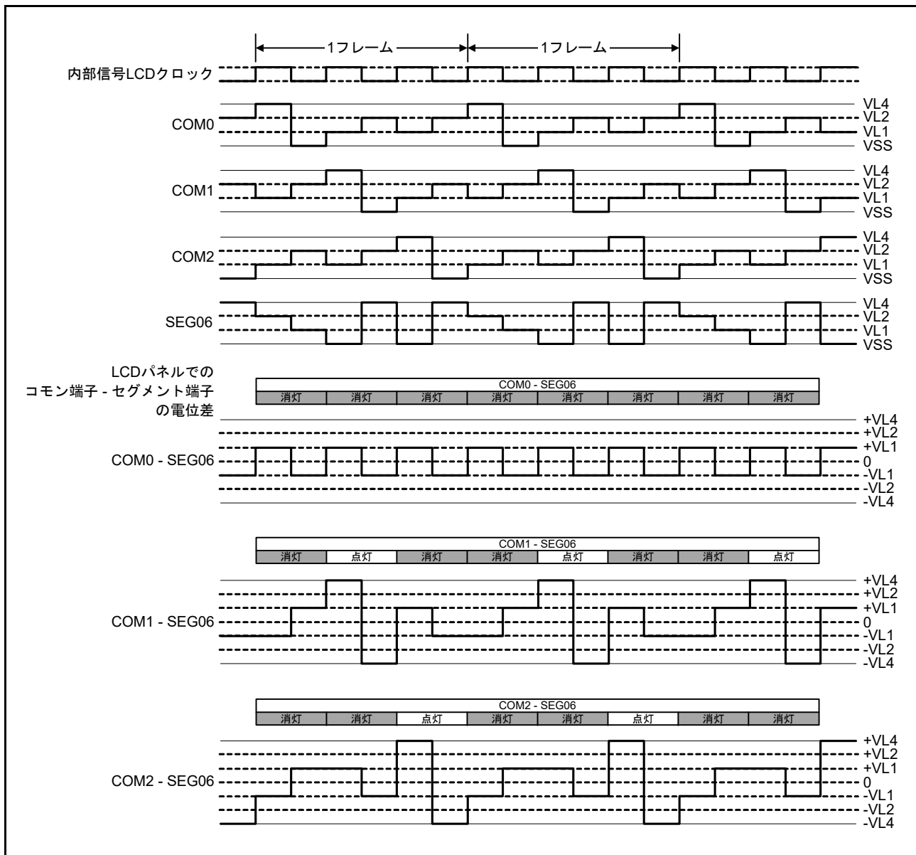
図 48.27 1/3 バイアス法を用いた SEG06 と各コモン信号との間の 3 時分割 LCD 駆動波形例
