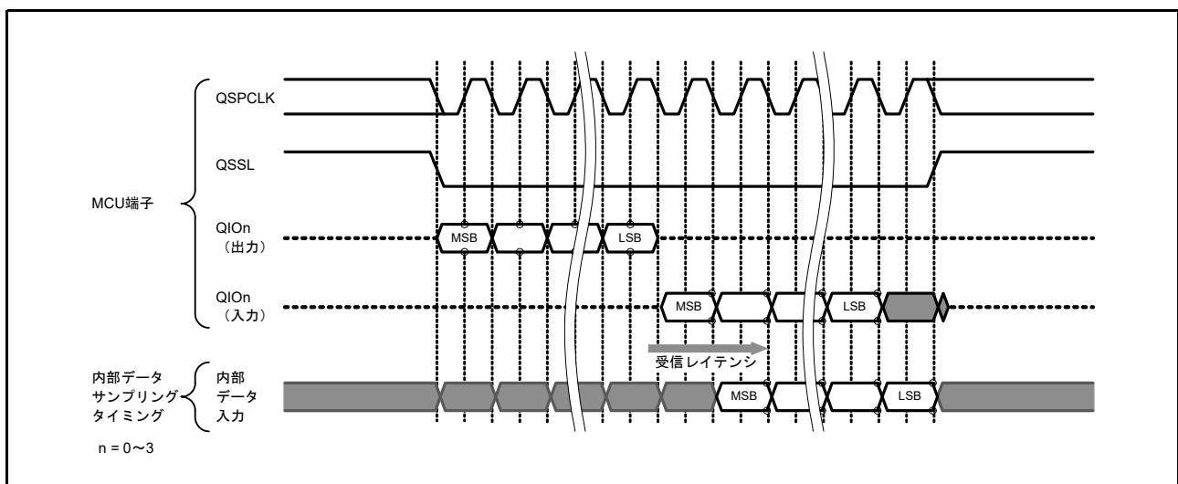
図 33.15 受信レイテンシ
