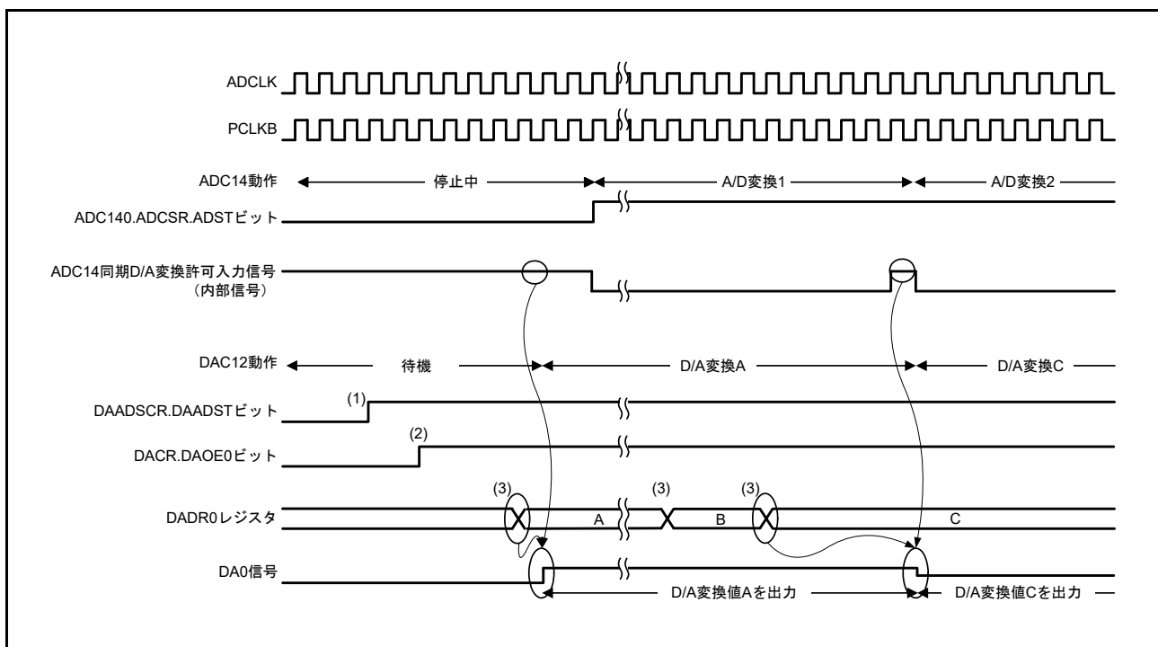
図 39.3 DAC12をADC14に同期して変換する例
