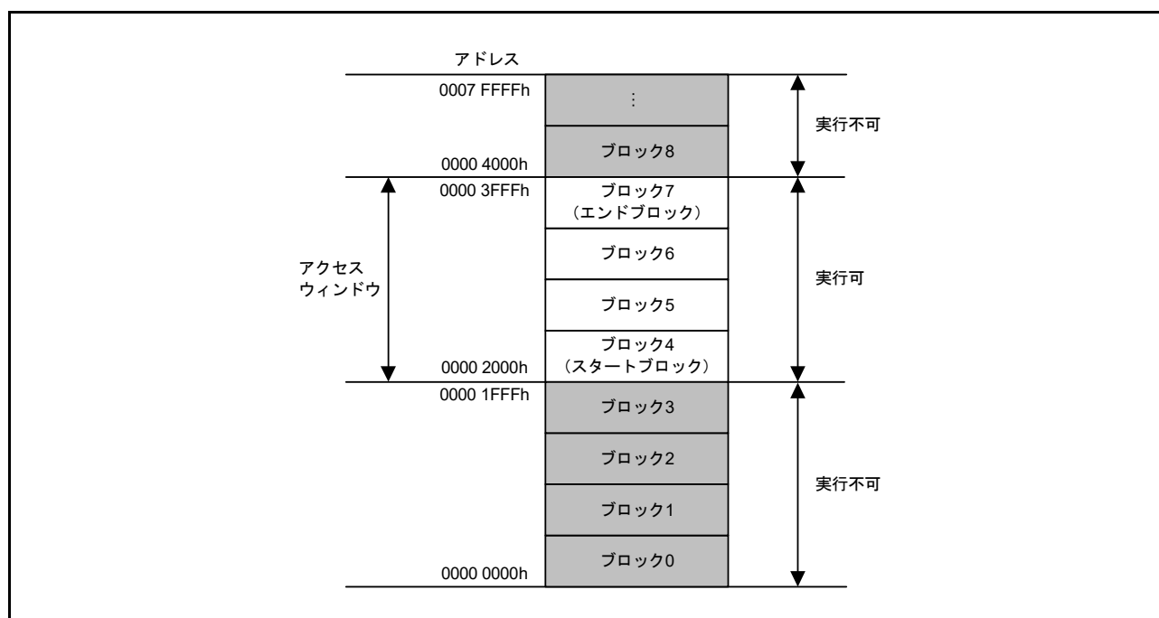
図 47.8 フラッシュ領域プロテクションの概要
