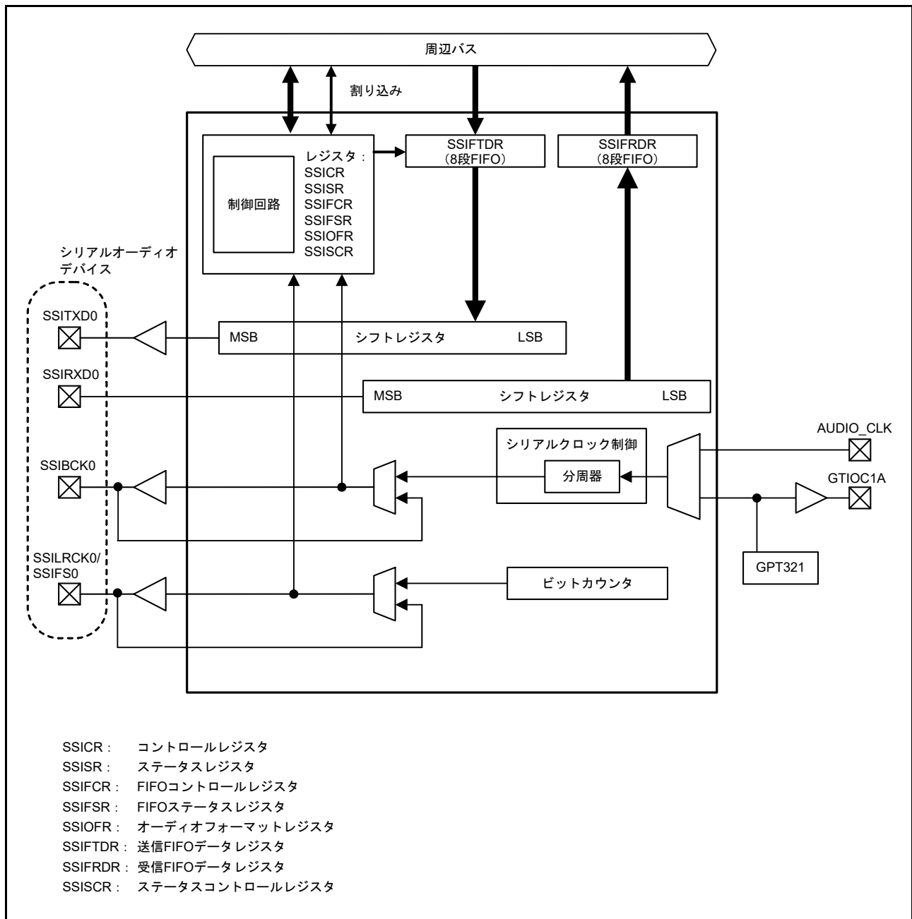
図 35.2 SSIE ブロック図 (SSIE0)
