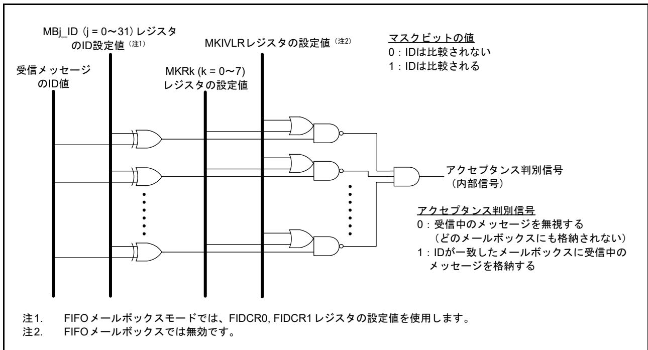
図 31.17 アクセプタンスフィルタ機能
