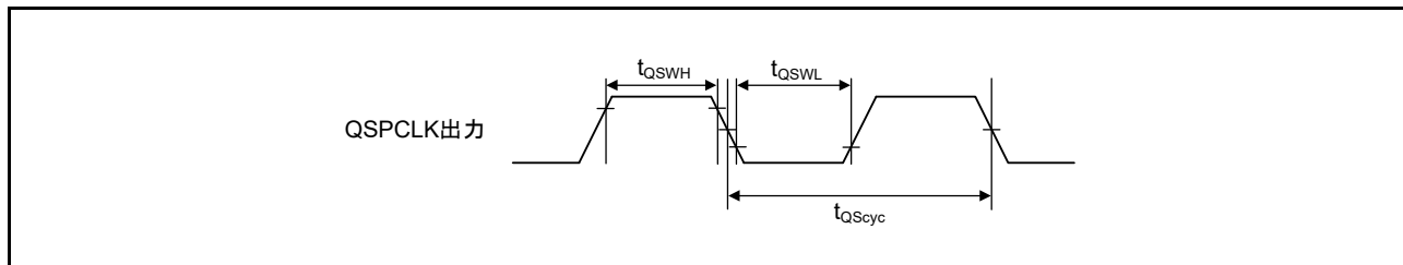
図 50.68 QSPI クロックタイミング
