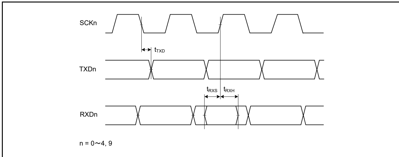
図 50.54 クロック同期式モードにおける SCI 入出力タイミング
