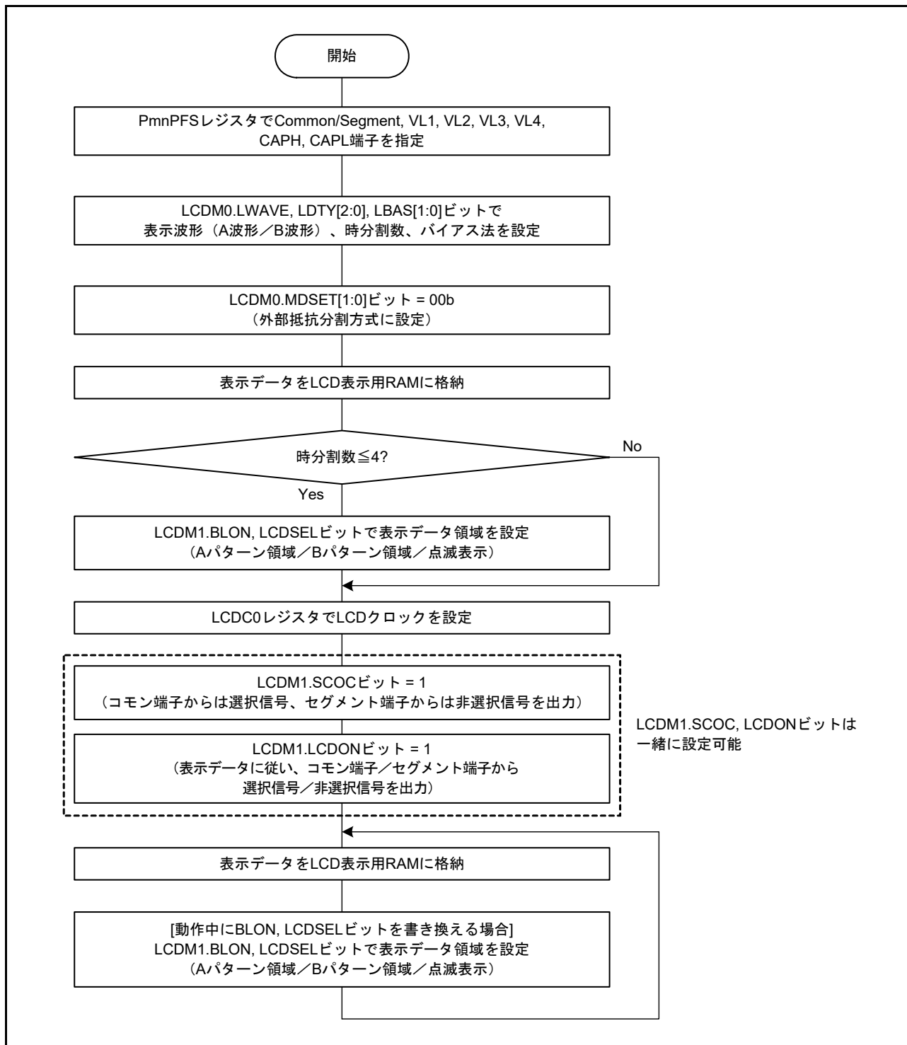
図 48.5 通常液晶波形表示での外部抵抗分割方式の設定手順
