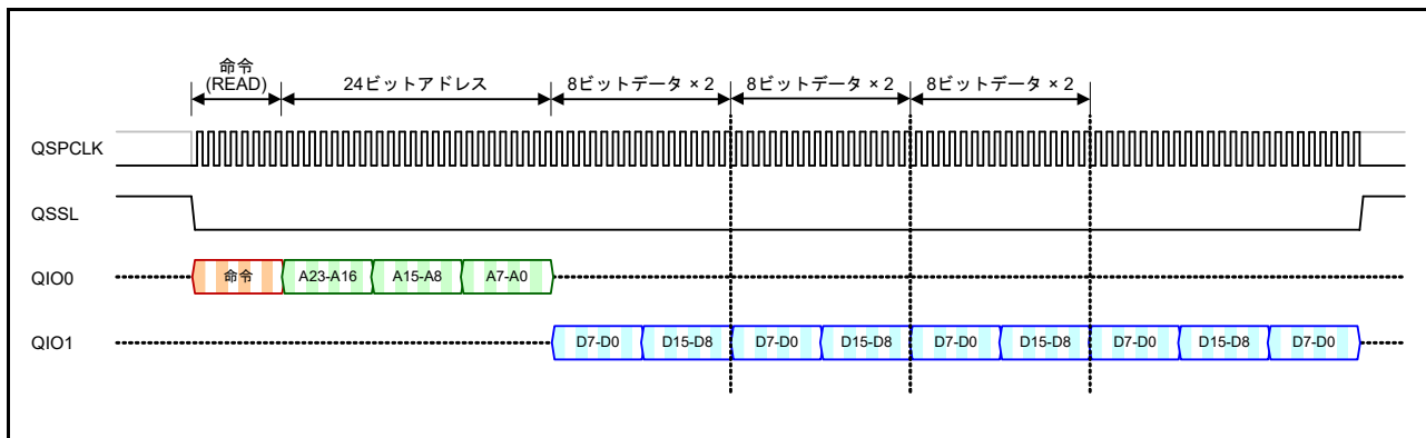
図 33.31 プリフェッチ機能を使用した連続データリード動作
