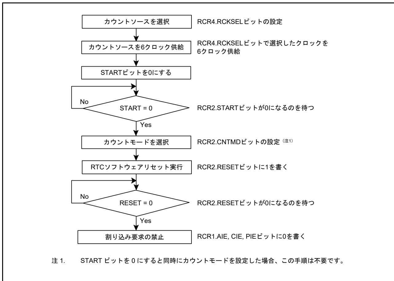
図 25.14 初期化手順
