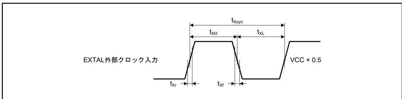
図 50.27 EXTAL 外部クロック入力タイミング
