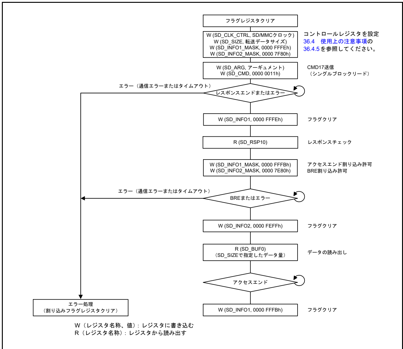
図 36.11 シングルブロックリード動作のフロー例
