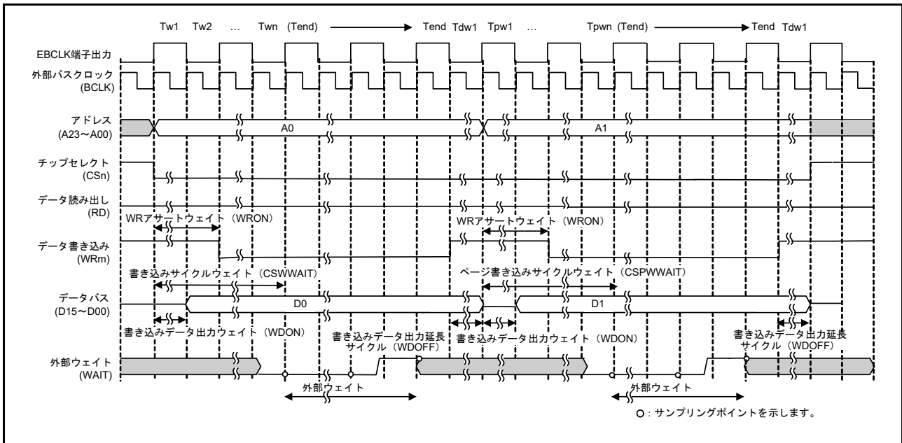
図 15.29 バイトストローブモード時の 16 ビットバス空間に対するページライトアクセスの外部ウェイトタイミング例 (EBCLK 端子出力選択ビットで BCLK の 2 分周を選択した場合) (n = 0 ~ 3, m = 0, 1)
