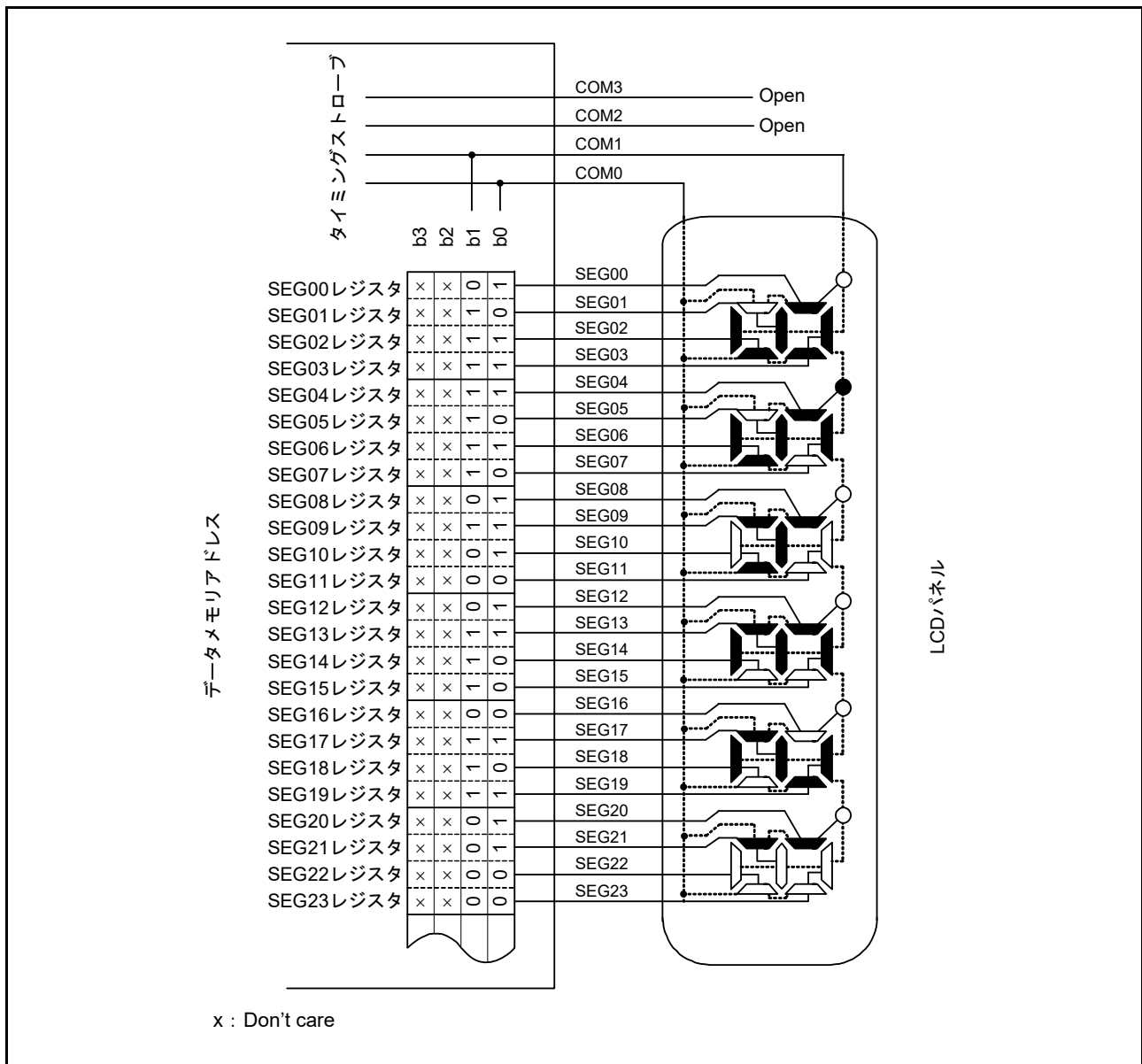
図 48.22 2 時分割 LCD パネルの接続例
