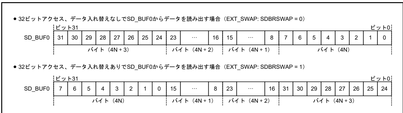
図 36.6 SD_BUF0 レジスタからの読み出し
