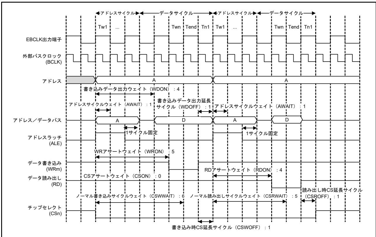
図 15.25 アドレス/データマルチプレクス I/O インタフェース時のバスタイミング例 (m = 0, 1)
