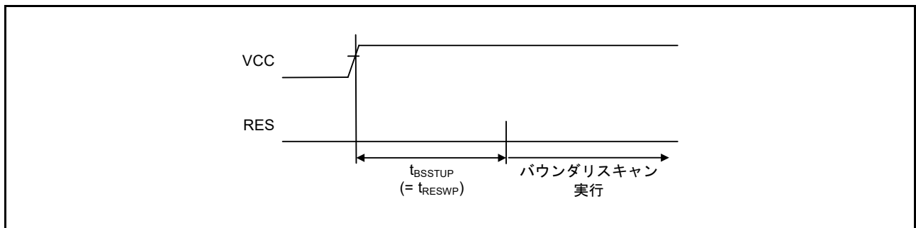
図 50.96 パウンダリスキャン回路起動タイミング
