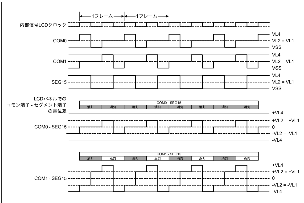
図 48.23 1/2 バイアス法を用いた SEG15 と各コモン信号との間の 2 時分割 LCD 駆動波形例
