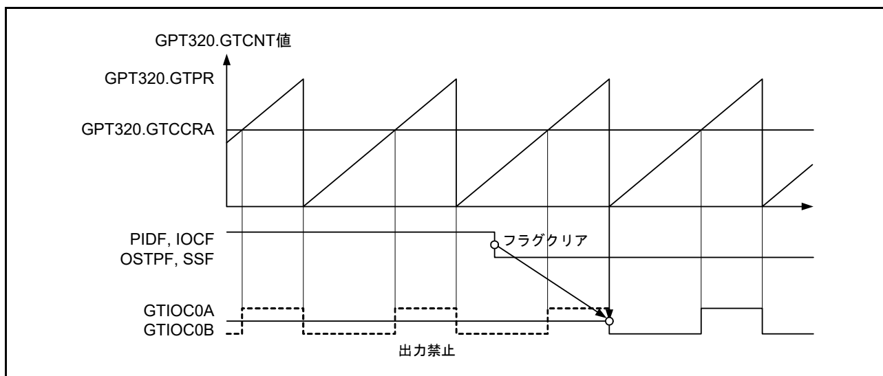
図 22.3 GPT 端子出力の出力禁止状態の解除タイミング
