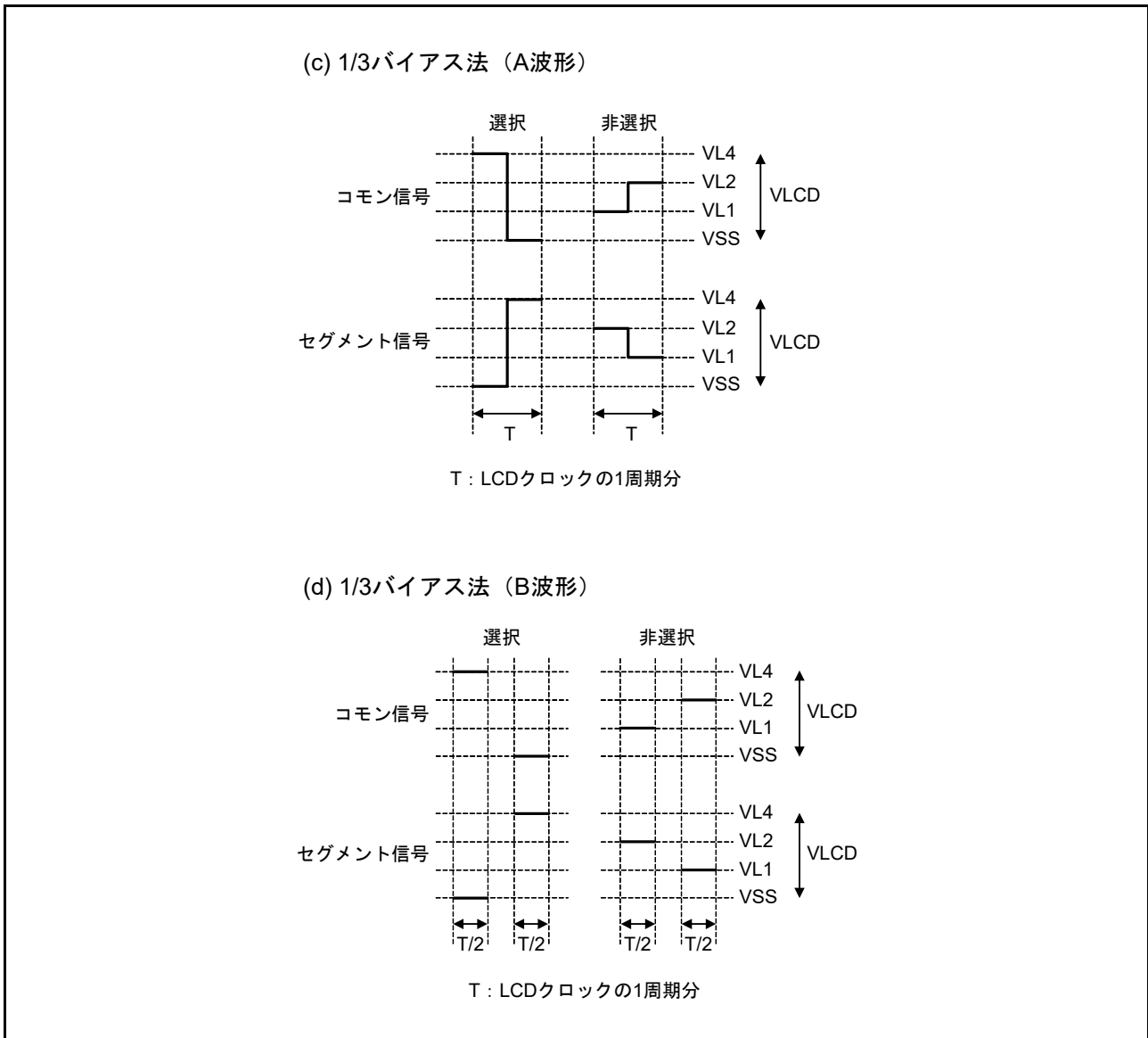
図 48.16 コモン信号とセグメント信号の電圧と位相 (2/3)
