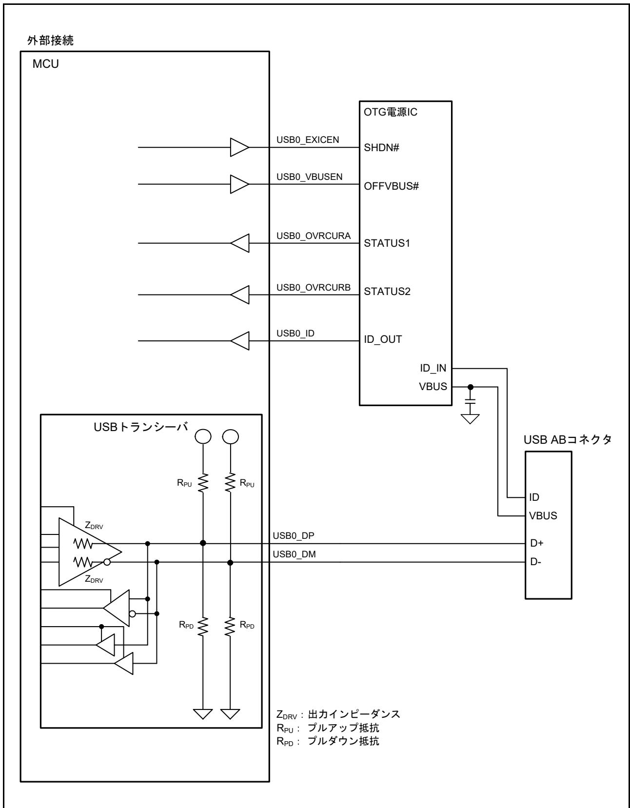
図 28.5 セルフパワー状態での OTG 接続例
