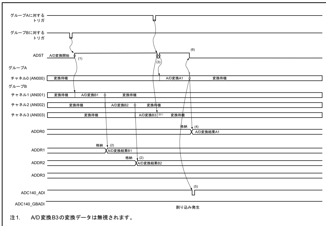
図 38.19 グループ A 優先制御の動作例 (4) (ADGSPCR.GBRSCN = 0, ADGSPCR.GBRP = 0 の場合)
