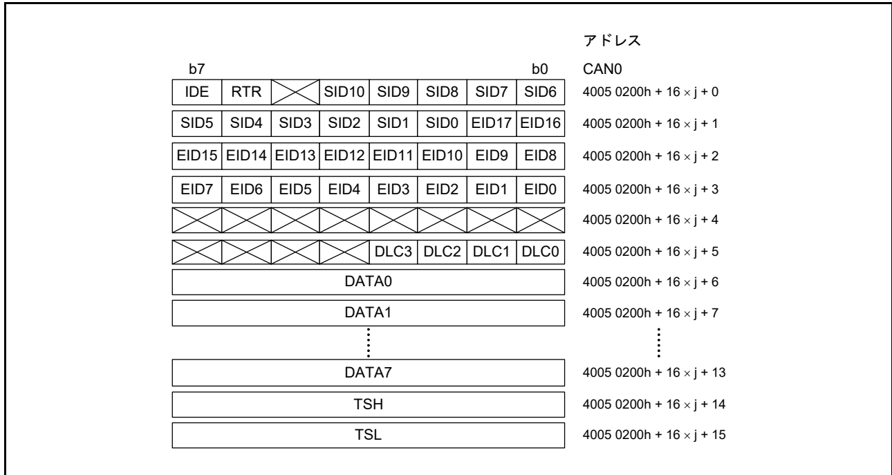
図 31.13 メールボックスレジスタの構成 (j = 0 ~ 31)
