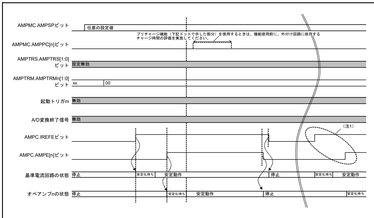
図 41.3 オペアンプの制御動作 (ソフトウェアトリガモードによる制御) (ソフトウェアトリガモードによって基準電流回路およびオペアンプを起動/停止する場合)
