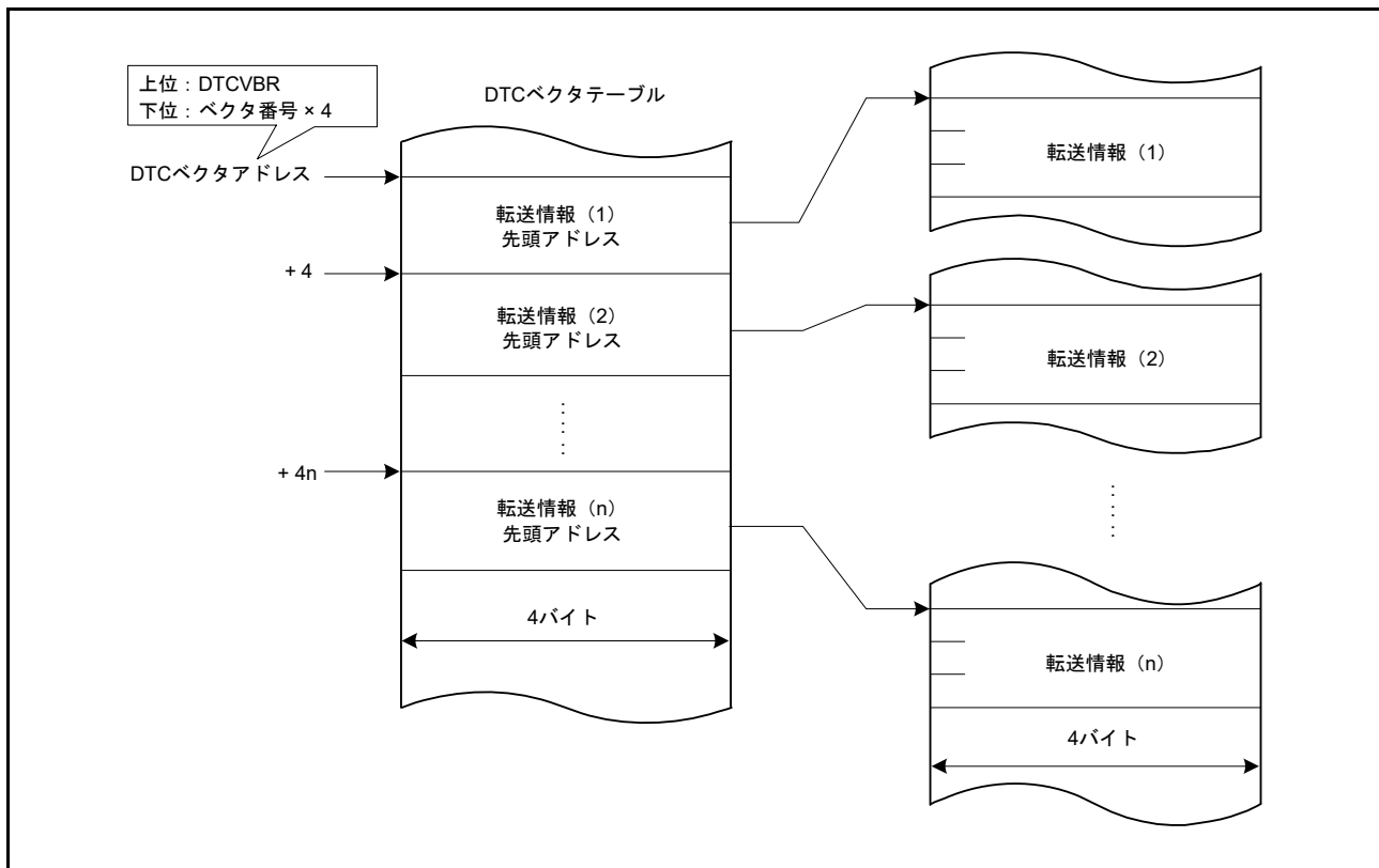
図 18.2 DTC ベクタテーブルと転送情報
