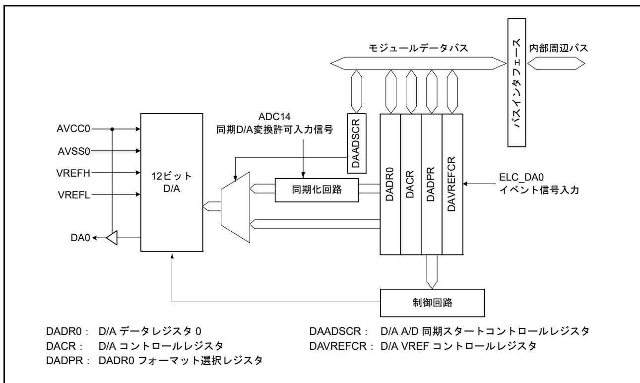
図 39.1 DAC12のブロック図
