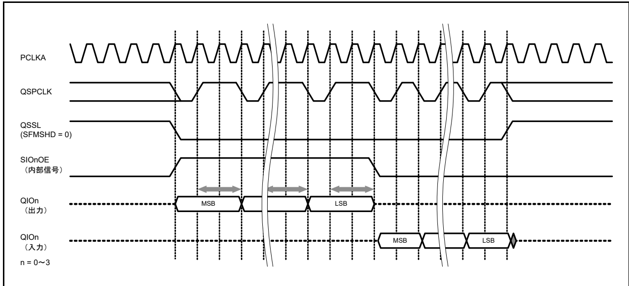
図 33.14 SFMOHW ビットを使用したシリアルデータ出力のホールド時間調整
