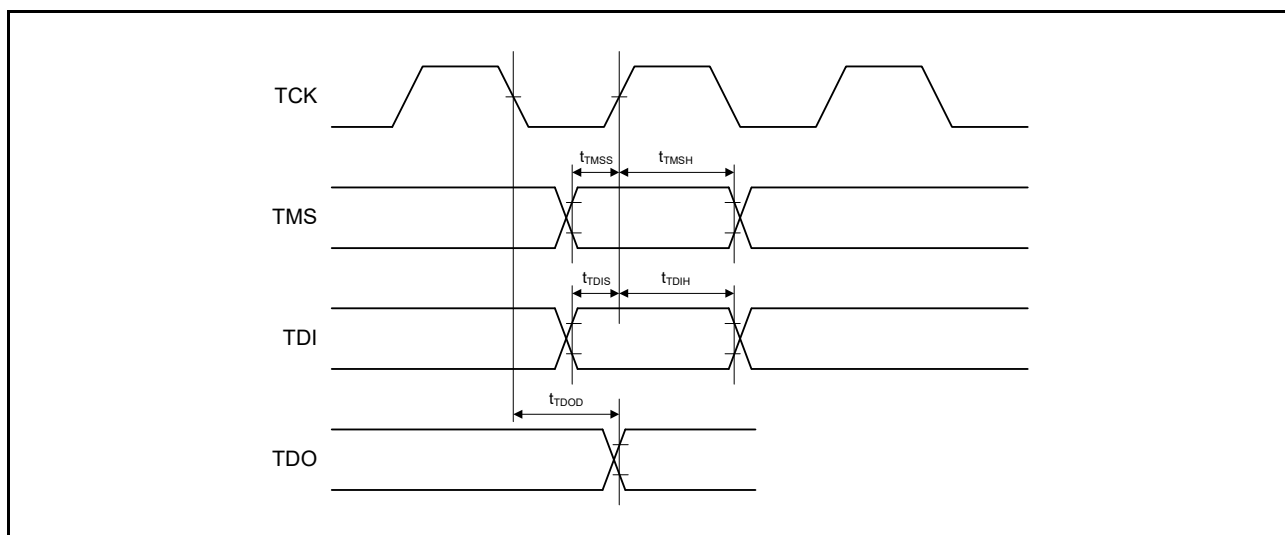
図 50.95 バウンダリスキャン入出力タイミング
