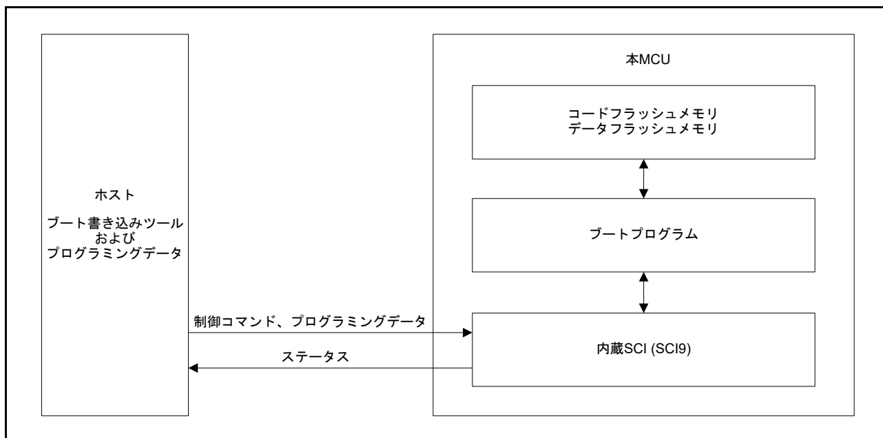
図 47.9 SCI ブートモード時のシステム構成
