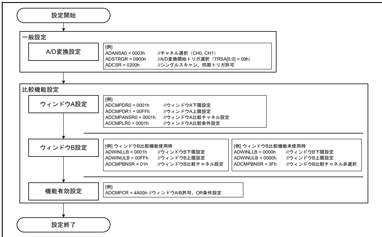
図 38.22 コンペア機能のイベント出力使用時の設定例
