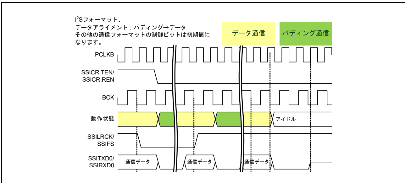
図 35.46 データ通信からの停止 (パディングビットあり)
