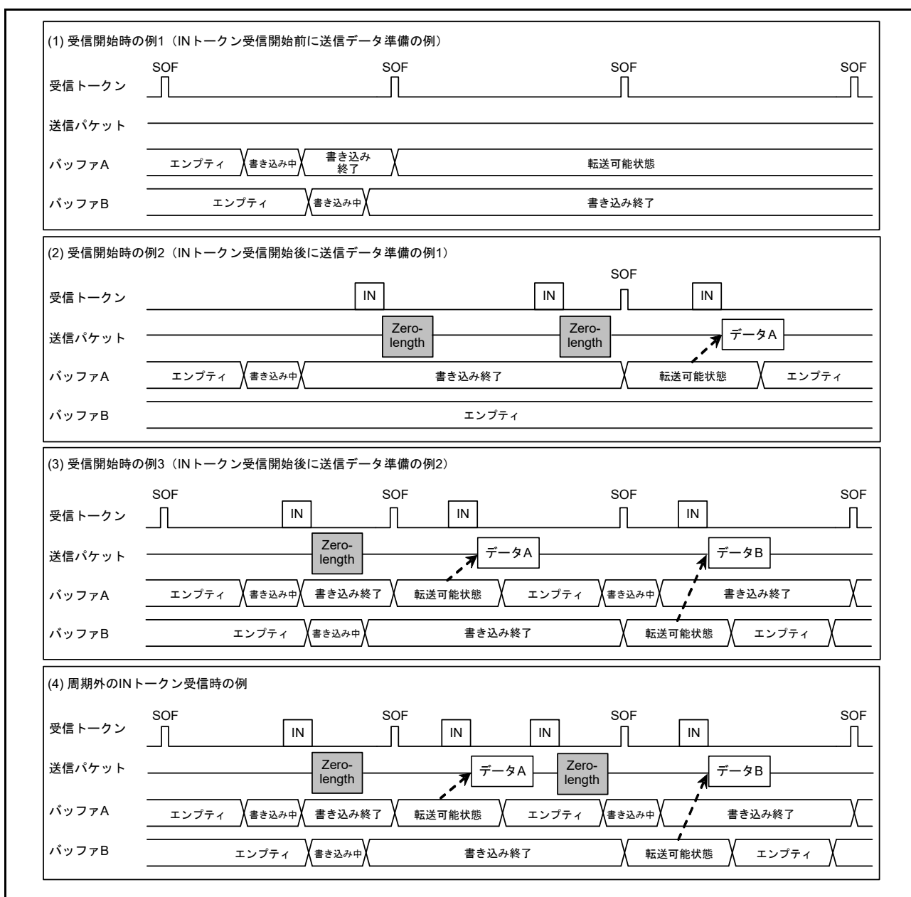
図 28.21 データセットアップ動作例
