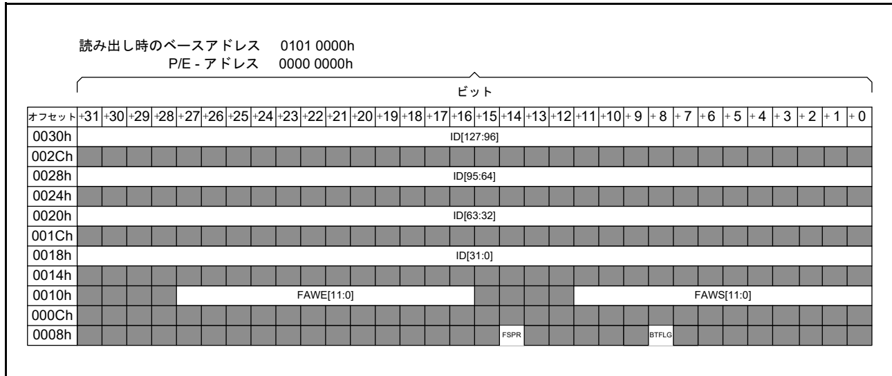
図 47.6 構成領域ビットマップ
