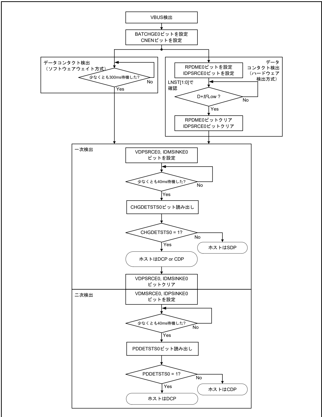
図 28.24 ポータブルデバイスとして動作時の処理フロー
