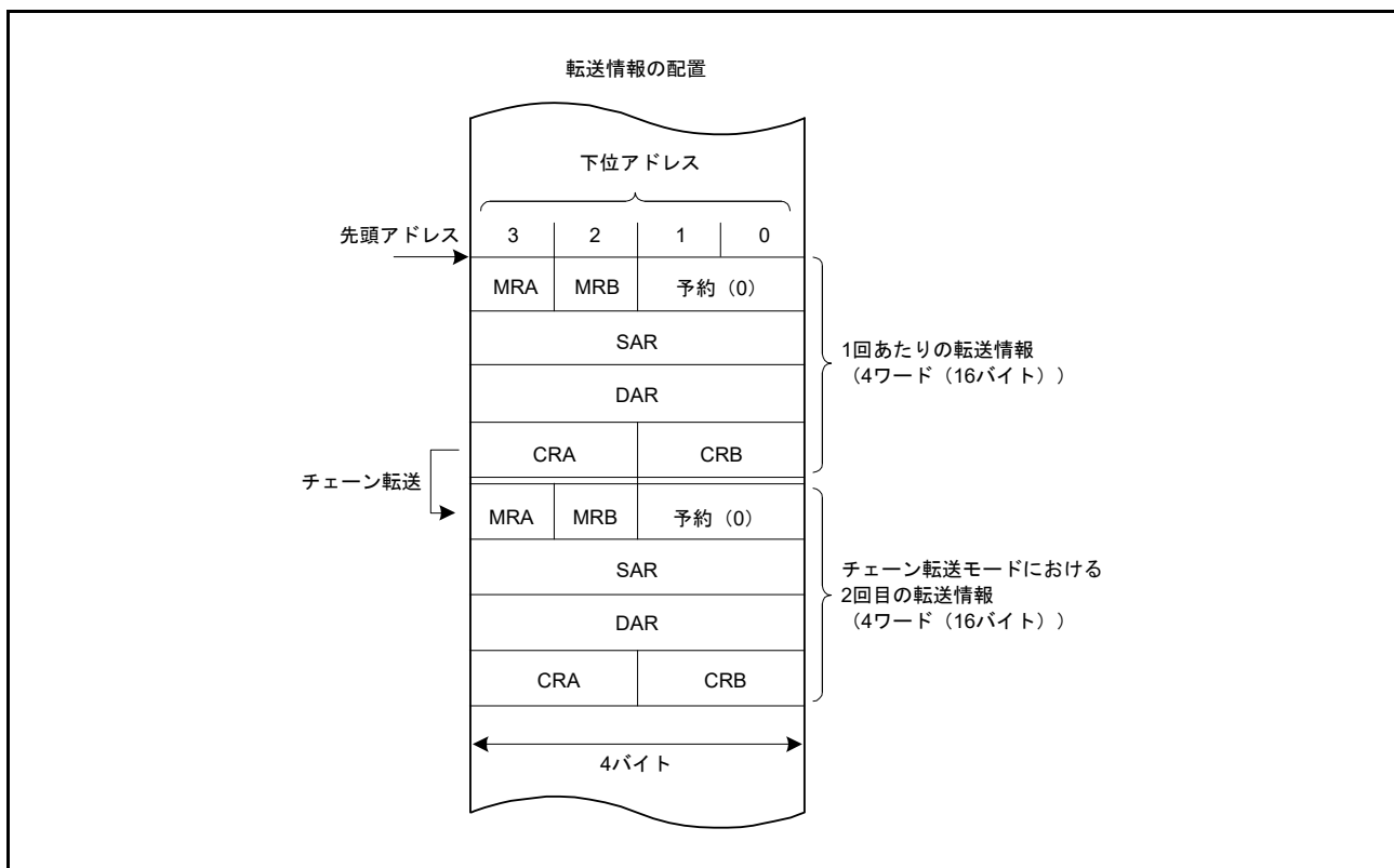
図 18.3 SRAM 領域上の転送情報の配置
