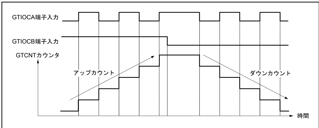
図 23.70 位相計数モード2 動作例 (C)
