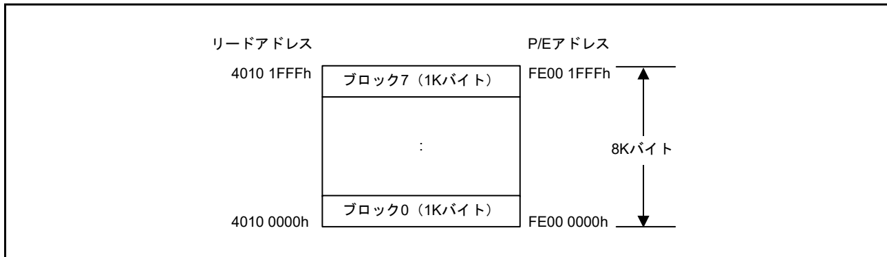
図 47.3 データフラッシュメモリマッピング
