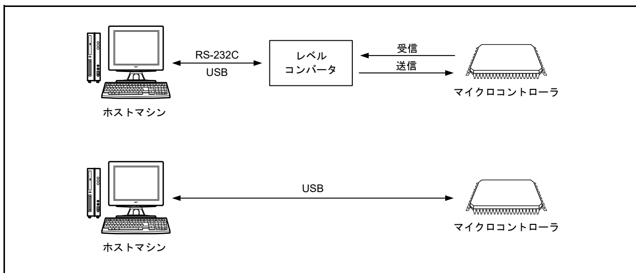
図 47.11 フラッシュメモリにプログラムを書き込むための環境
