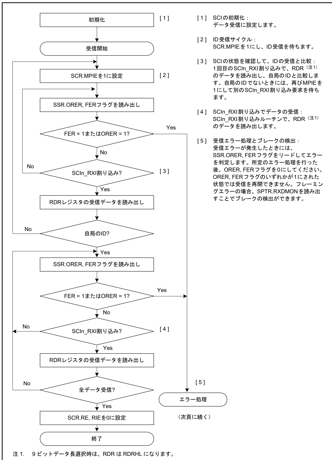
図 29.27 マルチプロセッサシリアル受信のフローチャート例 (1) (非 FIFO 選択時)
