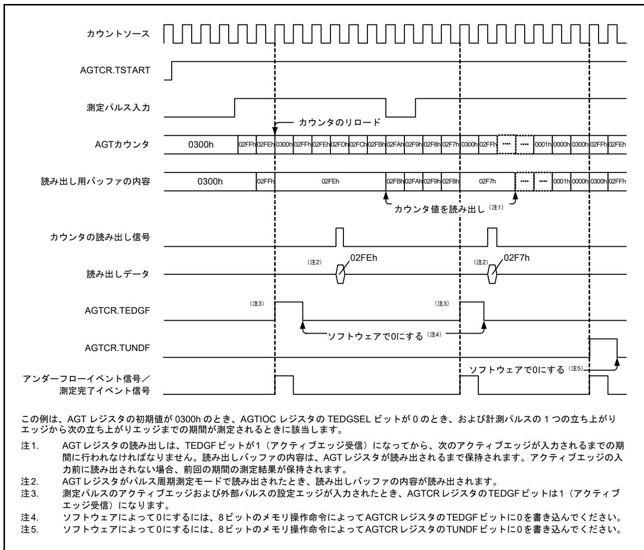
図 24.10 パルス周期測定モードでの動作例
