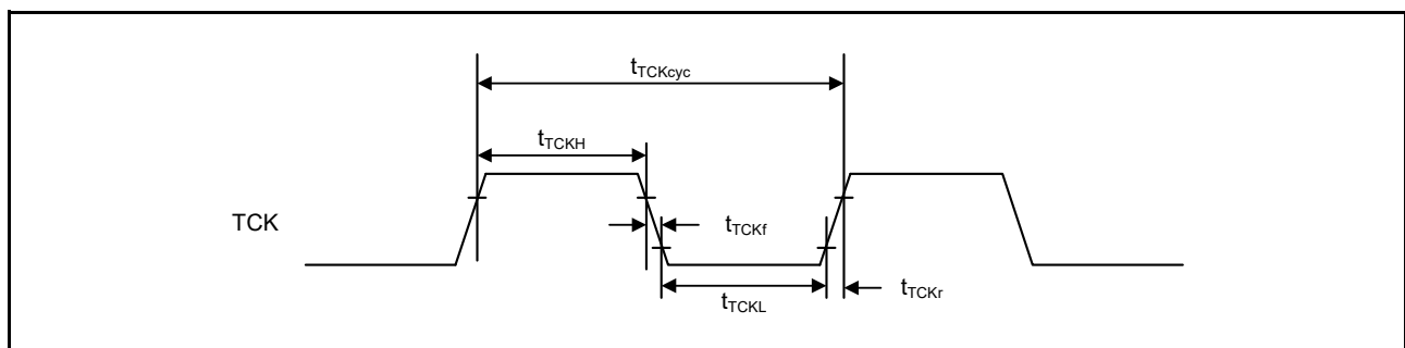
図 50.97 JTAG TCK タイミング
