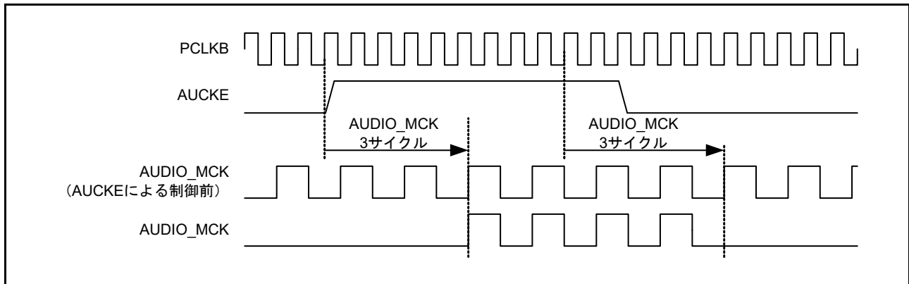
図 35.23 AUDIO_MCK の停止/再開
