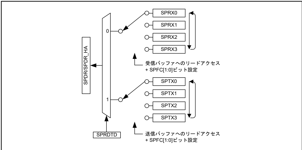
図 32.6 読み出し時の SPDR/SPDR_HA レジスタの構成図 (SPI0 の場合)
