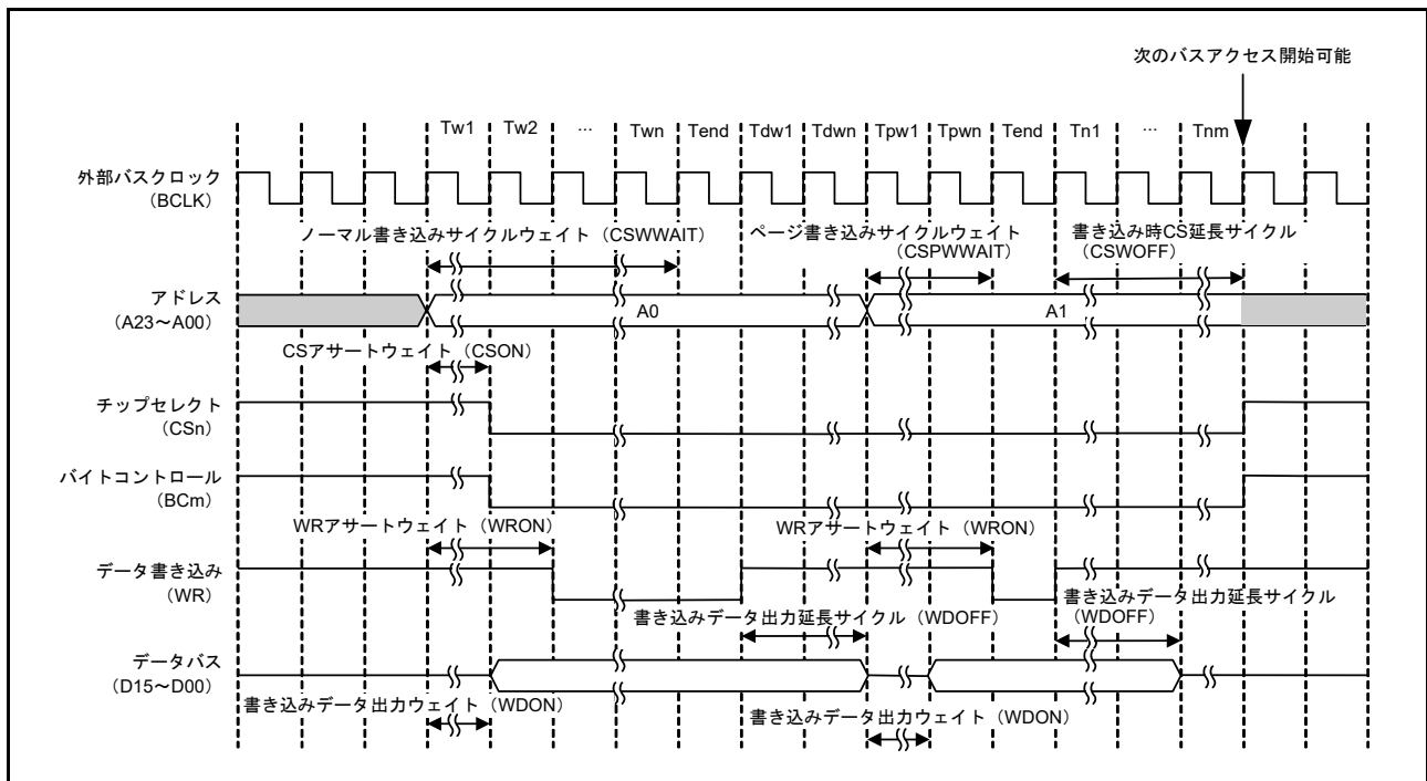
図 15.18 ページライトアクセスのタイミング (n = 0 ~ 3, m = 0, 1)
