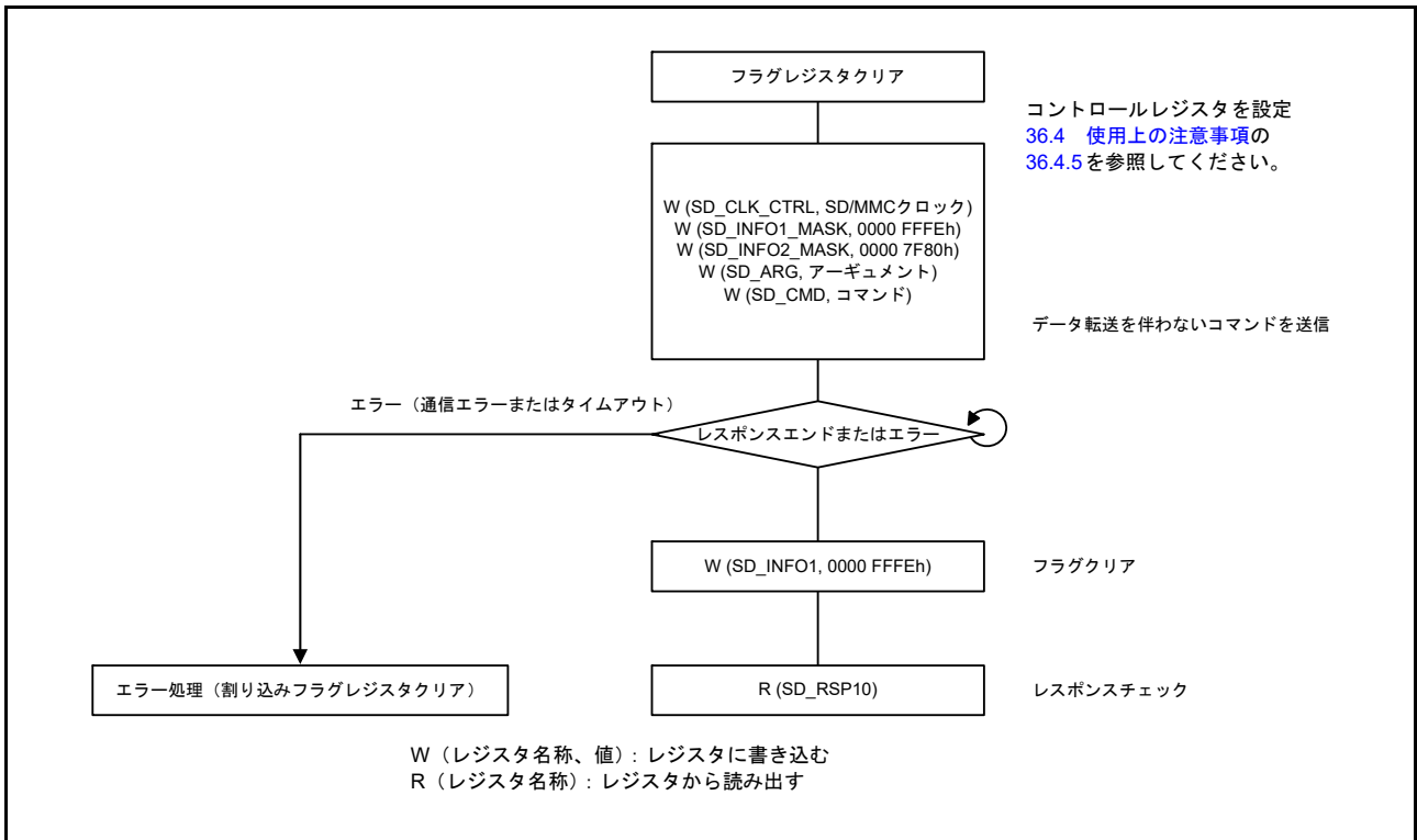
図 36.10 データがないコマンドのフロー例
