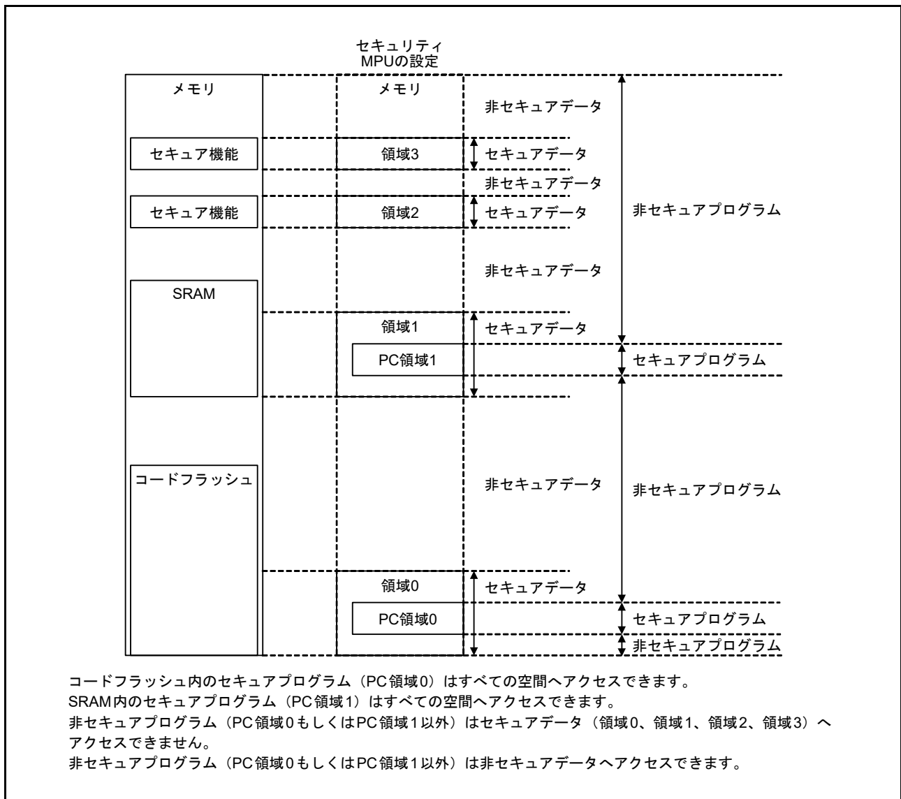
図 16.11 セキュリティ MPU の使用例
