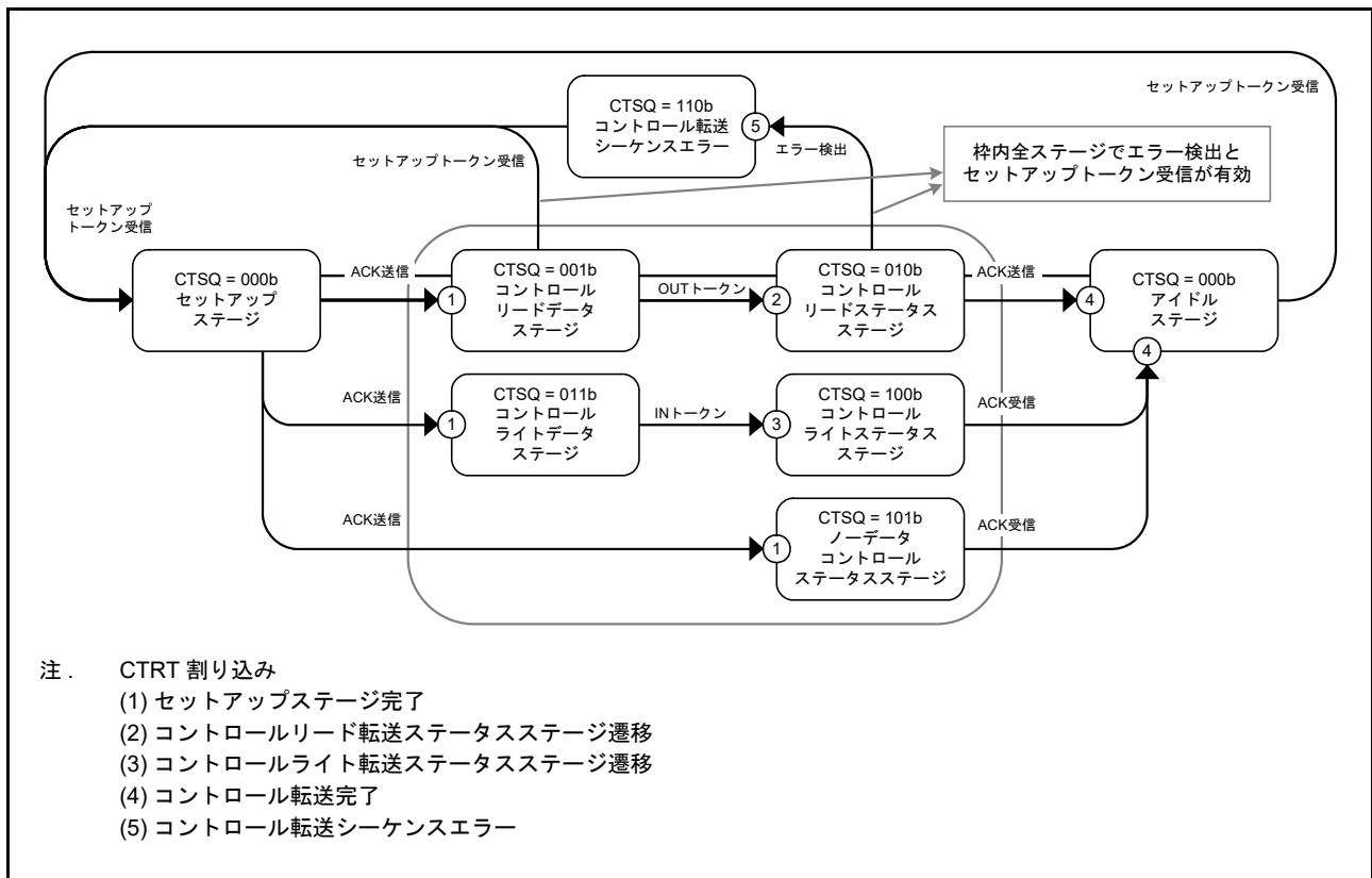
図 28.16 コントロール転送ステージの遷移
