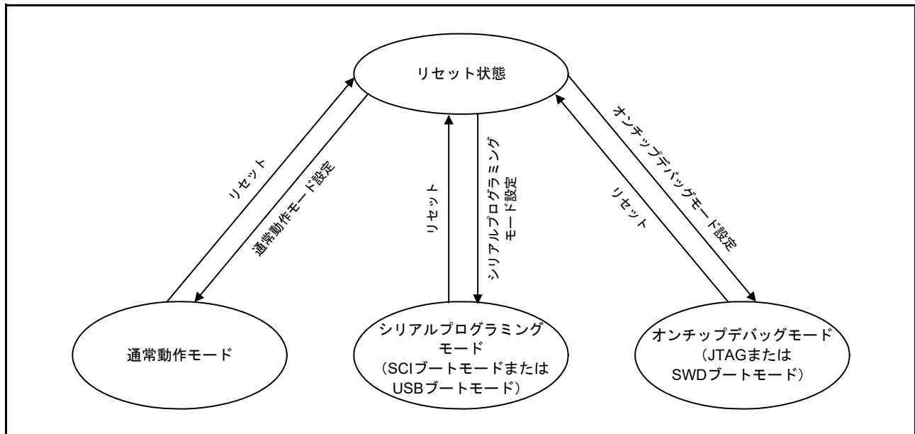
図 47.5 フラッシュメモリに関するモード遷移図
