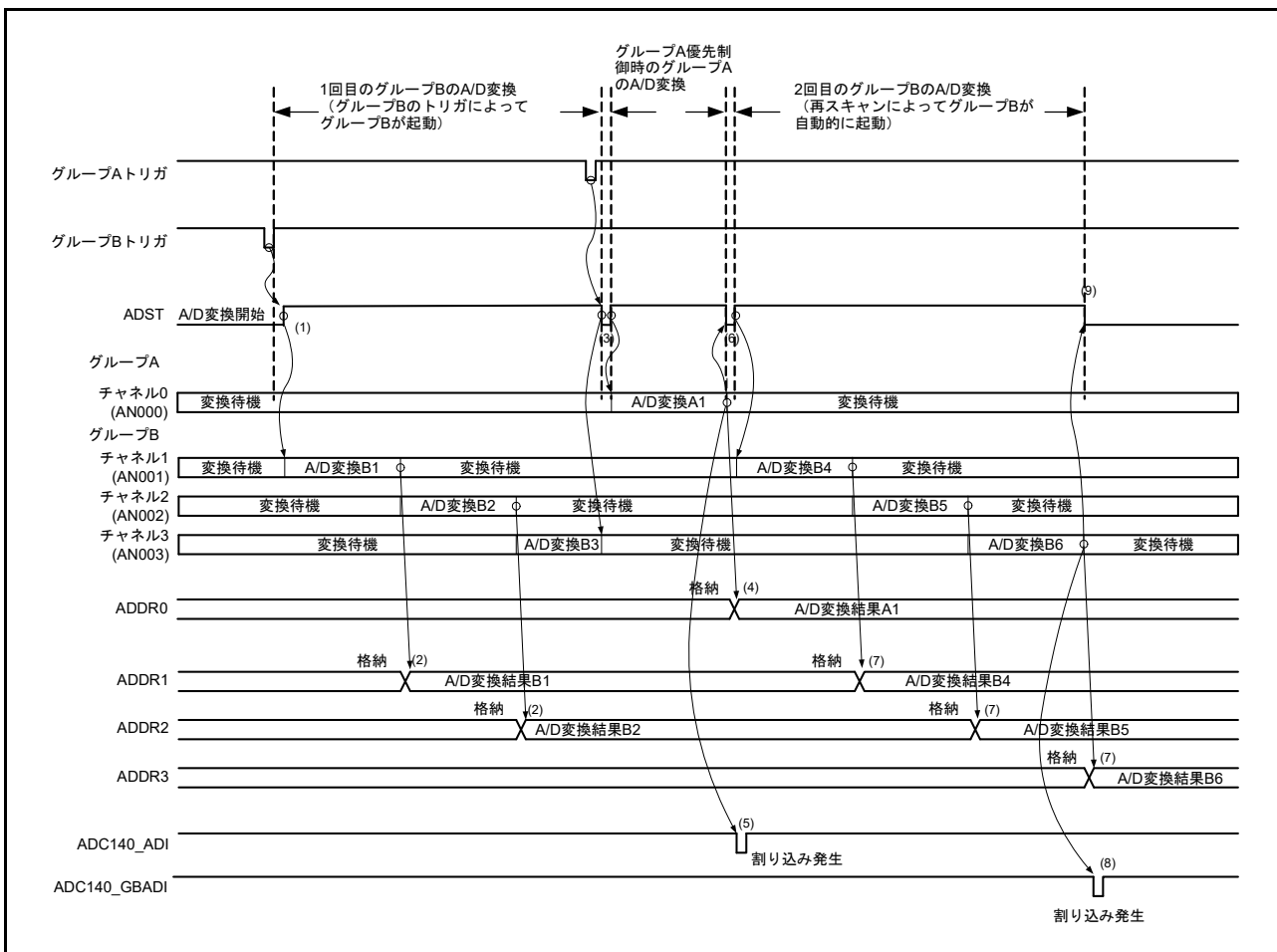
図 38.16 グループ A 優先制御の動作例 (1) (ADGSPCR.GBRSCN = 1, ADGSPCR.GBRP = 0 の場合)
