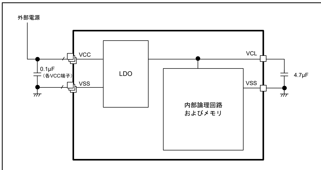
図 49.1 LDOモード設定
