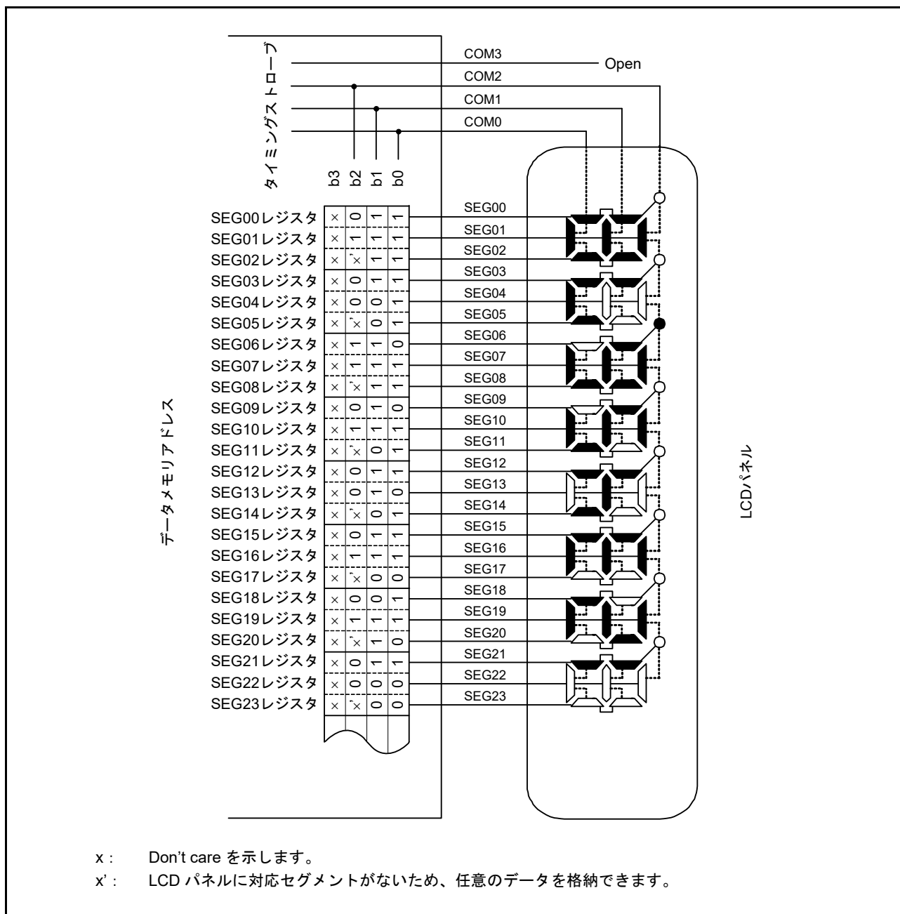
図 48.25 3 時分割 LCD パネルの接続例
