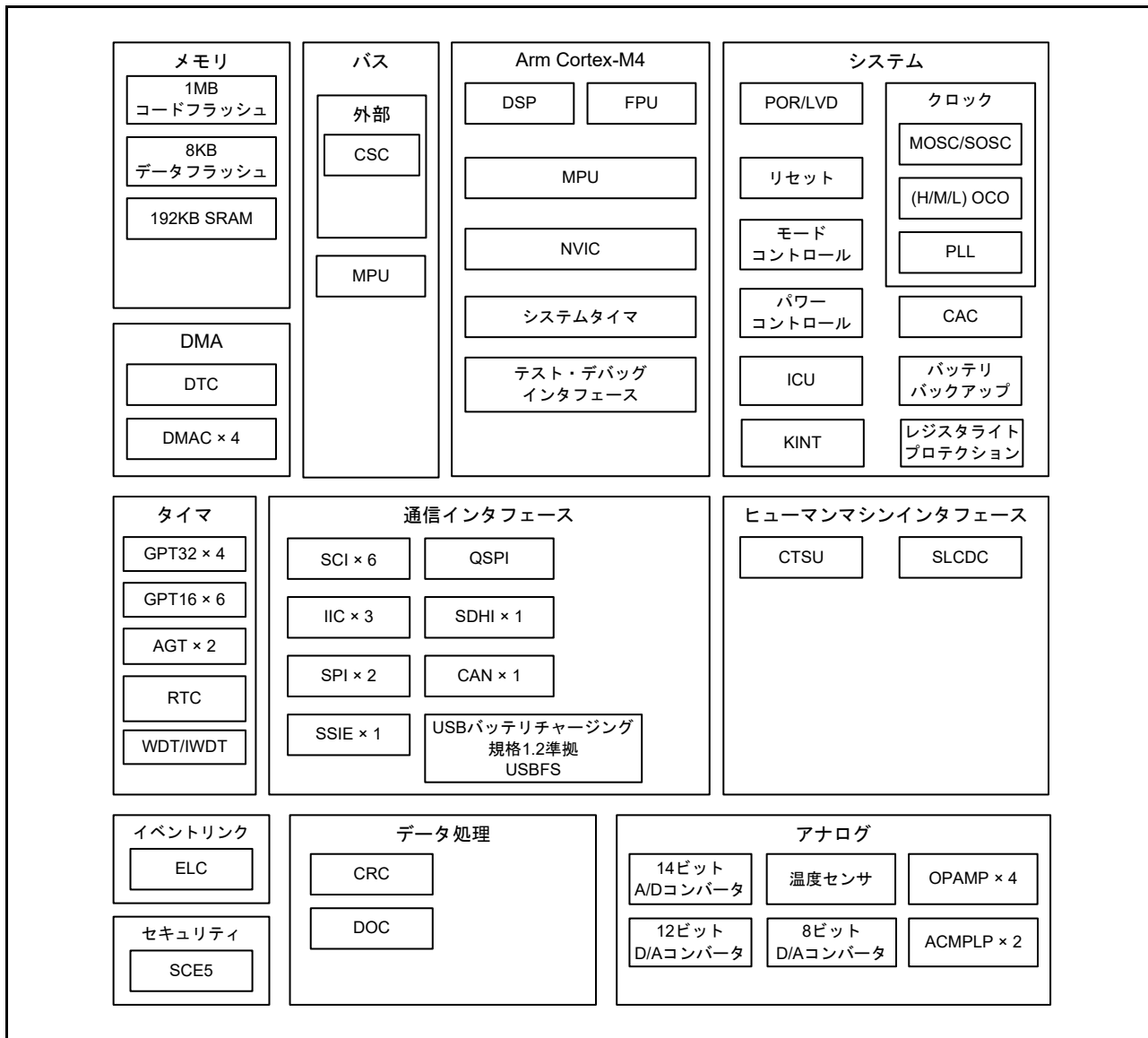
図 1.1 ブロック図
