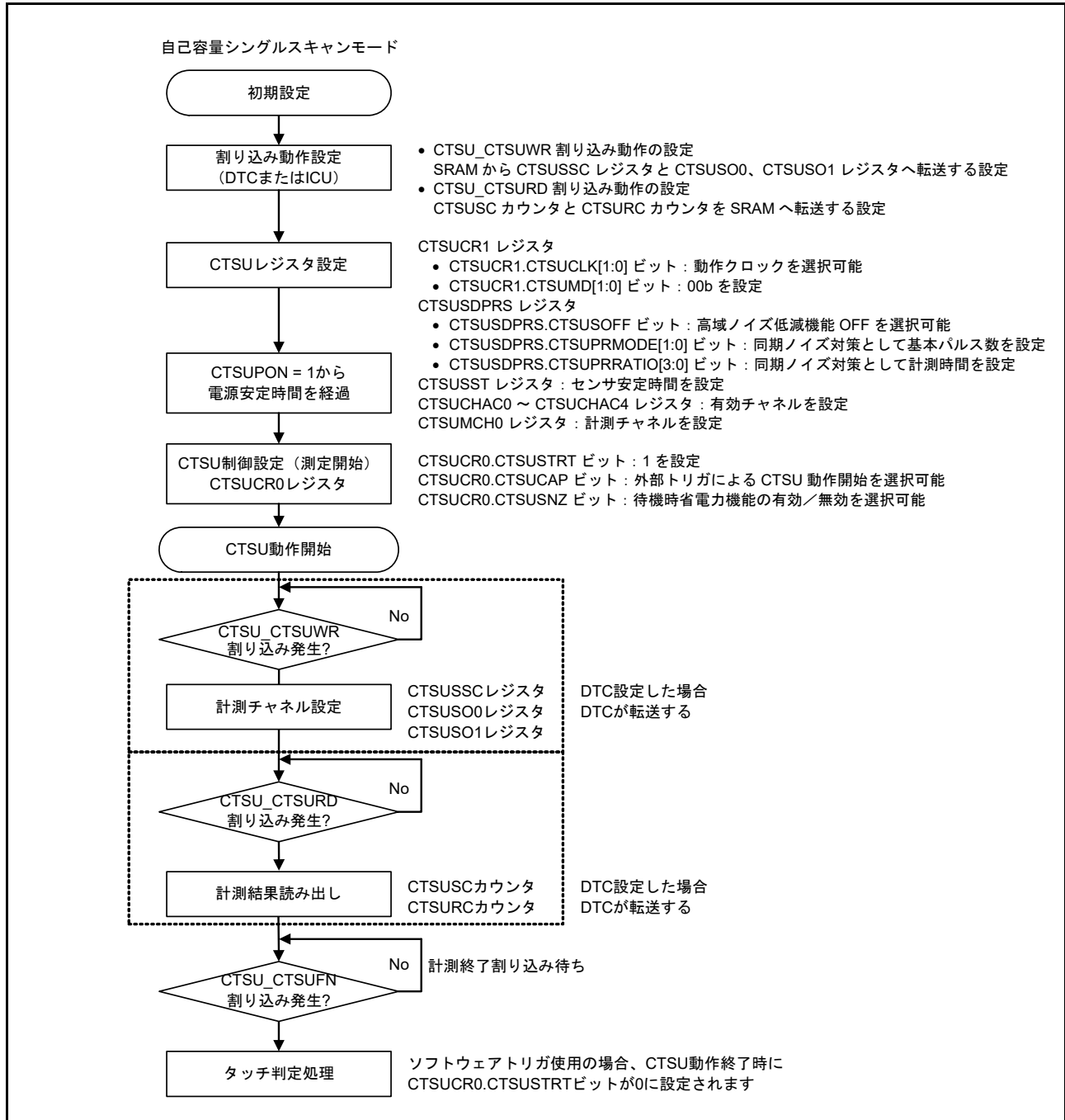
図 44.12 自己容量シングルスキャンモードのソフトウェアフローと動作例
