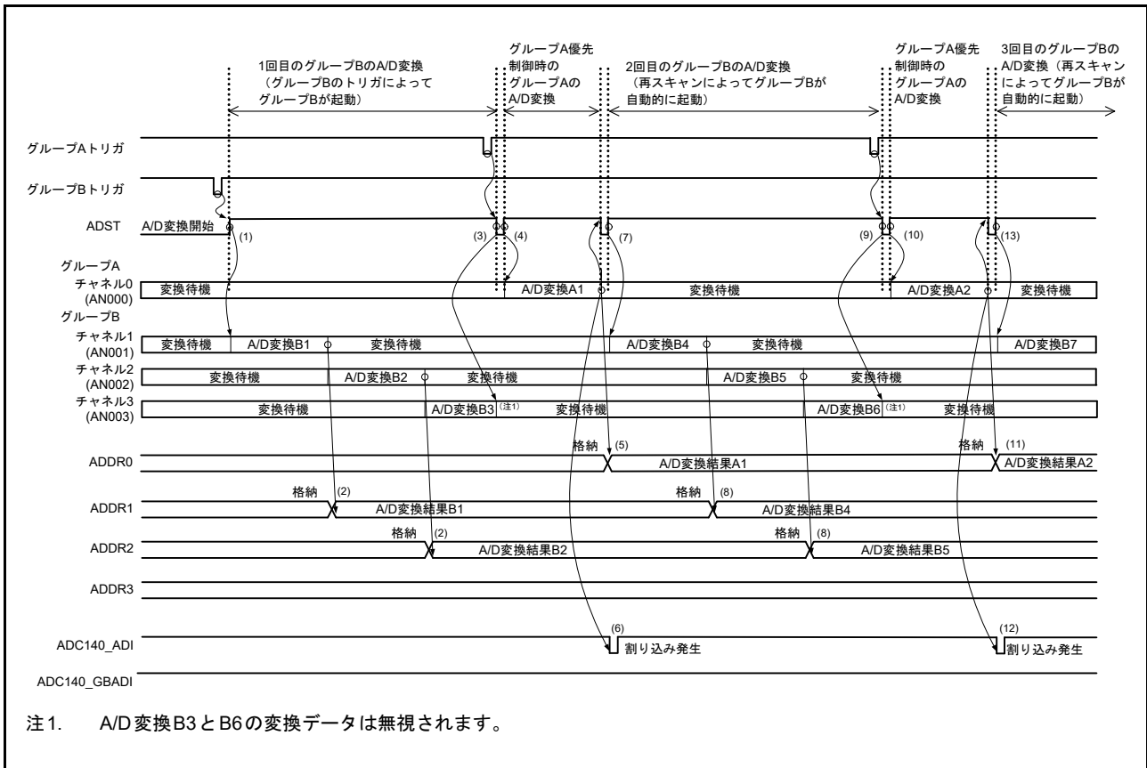
図 38.17 グループ A 優先制御の動作例 (2) (ADGSPCR.GBRSCN = 1, ADGSPCR.GBRP = 0 の場合)
