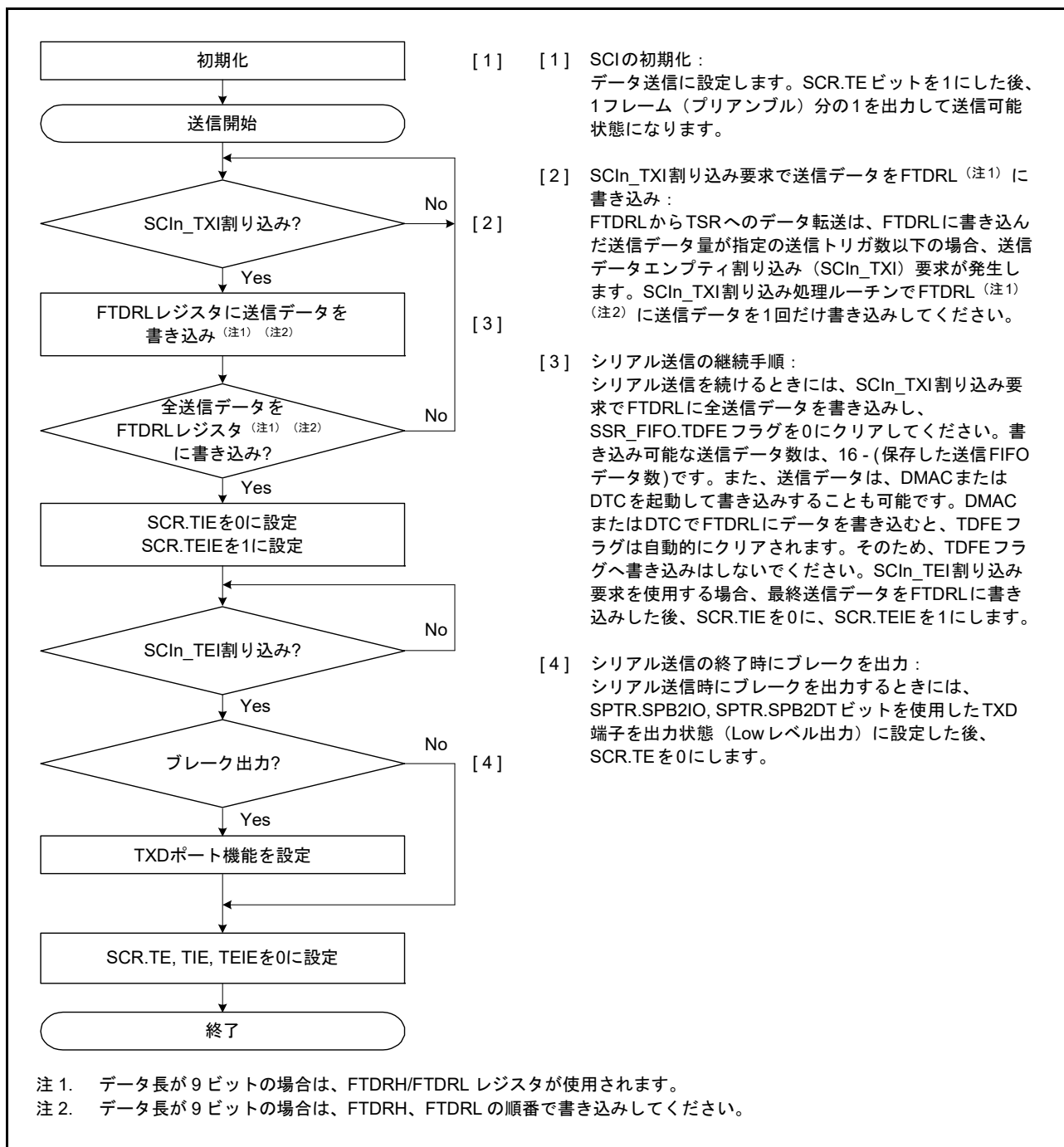
図 29.14 調歩同期式モードにおけるシリアル送信のフローチャート例（FIFO 選択時）
