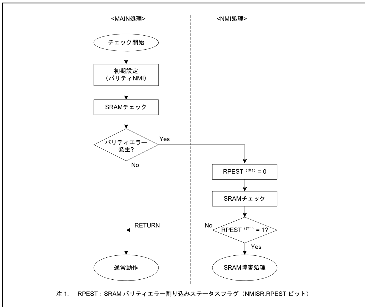
図 46.3 SRAM パリティ割り込み許可の場合の SRAM パリティチェックのフロー
