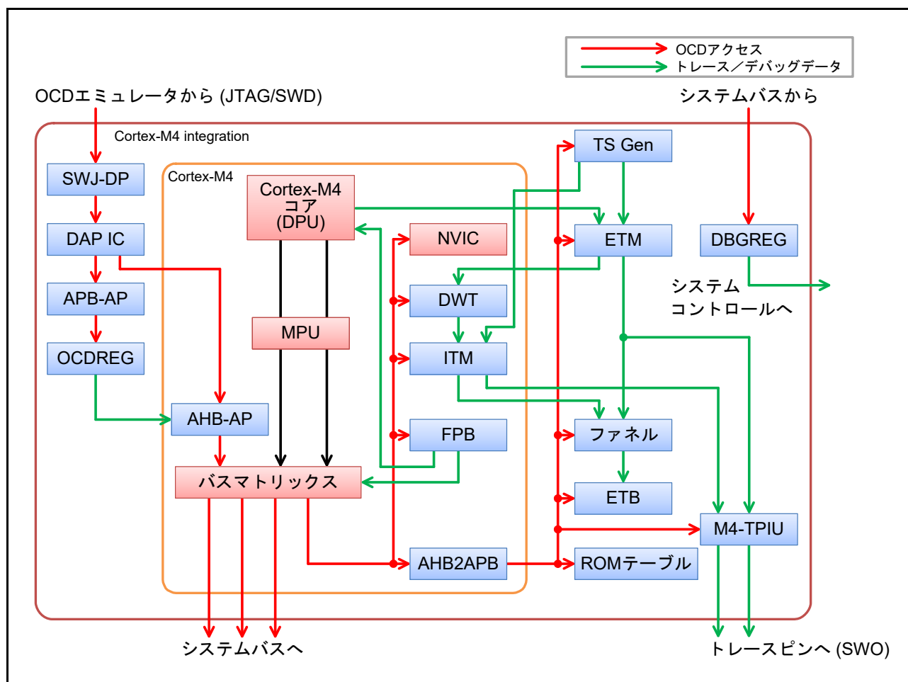
図 2.1 Cortex-M4 CPU ブロック図
