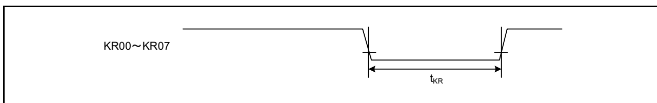
図 50.52 キー割り込み入力タイミング
