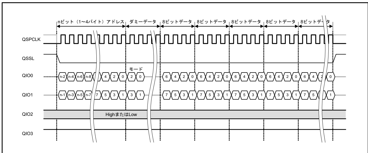
図 33.22 XIP モード時のファストリード Dual I/O バスサイクル
