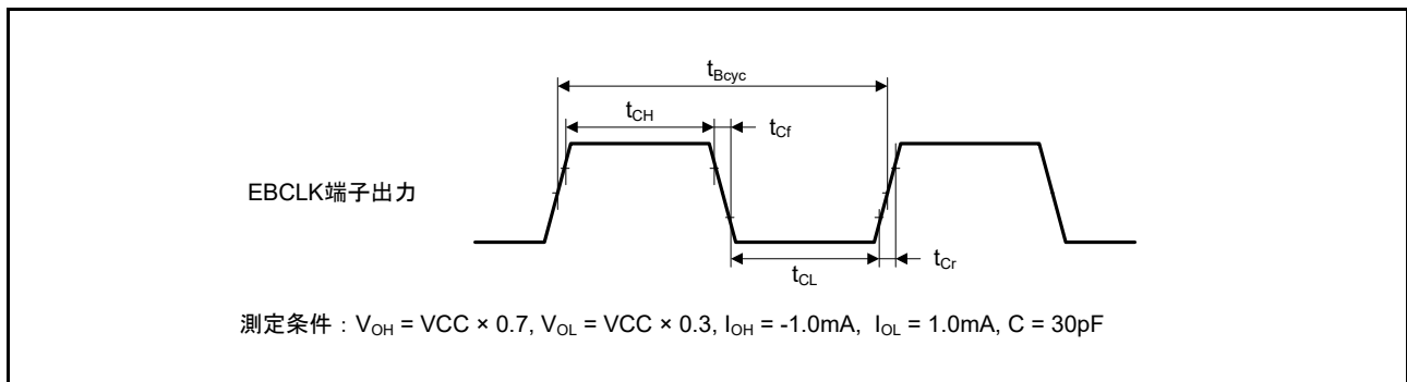
図 50.26 EBCLK 端子出力タイミング
