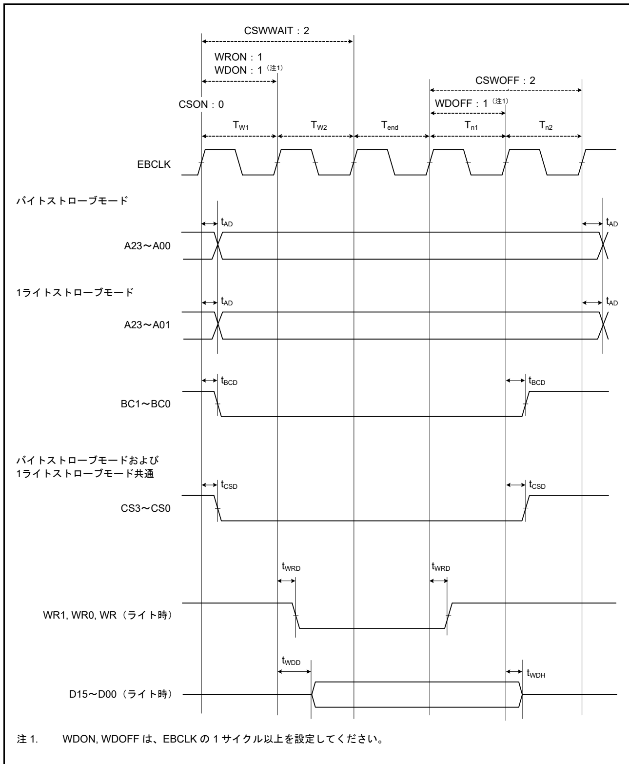
図 50.43 外部バスタイミング/ノーマルライトサイクル (バスクロック同期)
