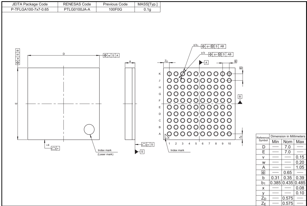
図 2.4 LGA 100 ピン
