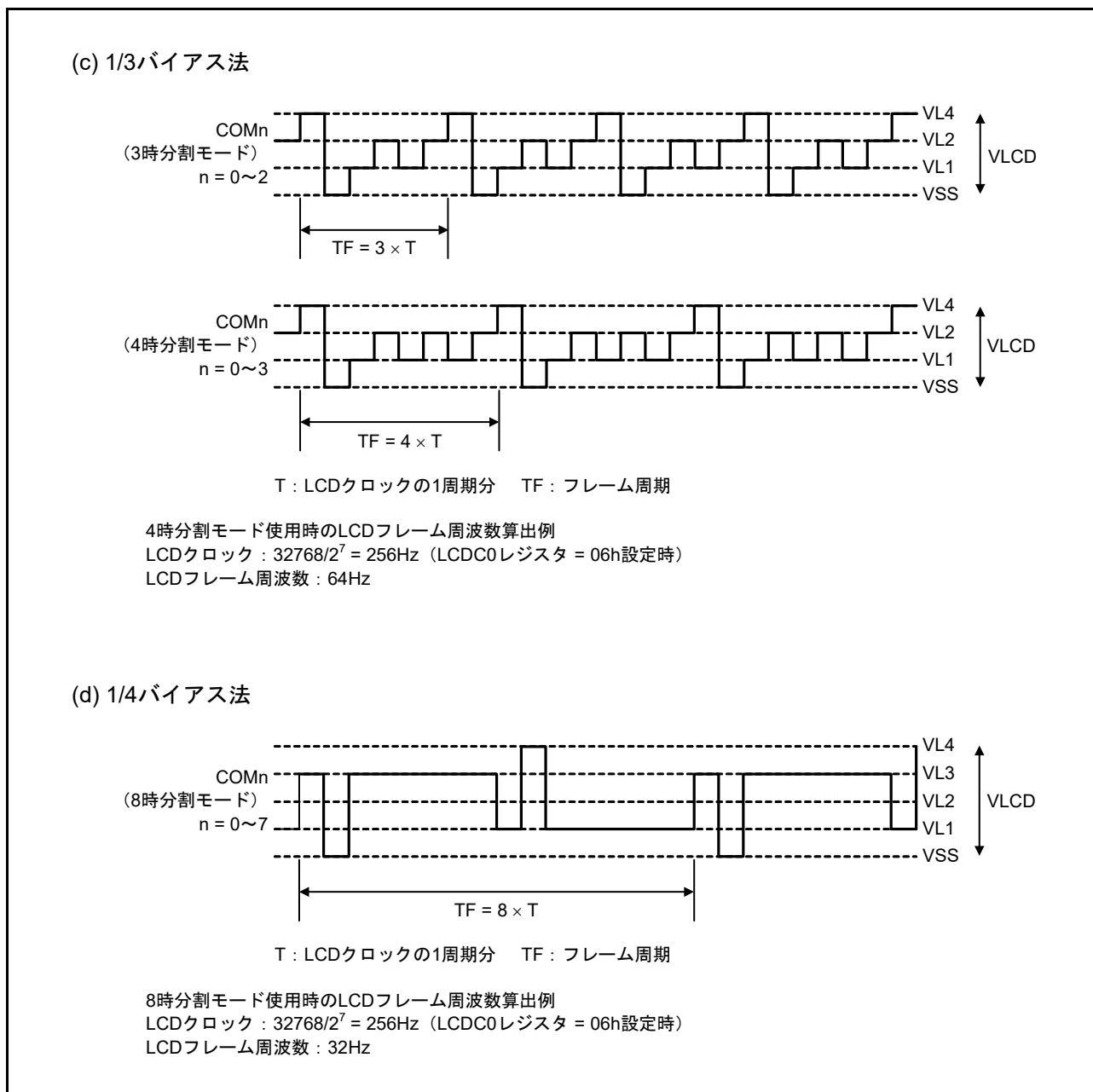
図 48.14 コモン信号波形 (2/2)
