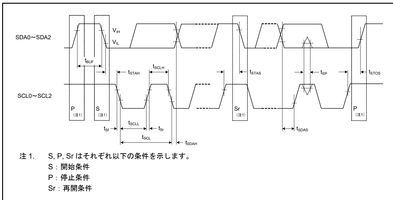
図 50.70 I 2 C バスインタフェース入出カタイミング
