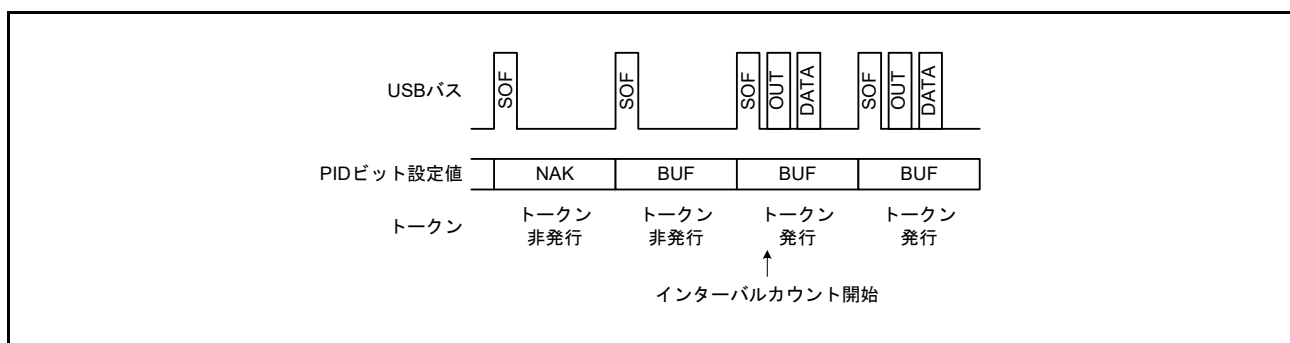
図 28.17 IITV[2:0] = 0 の場合のトークン発行
