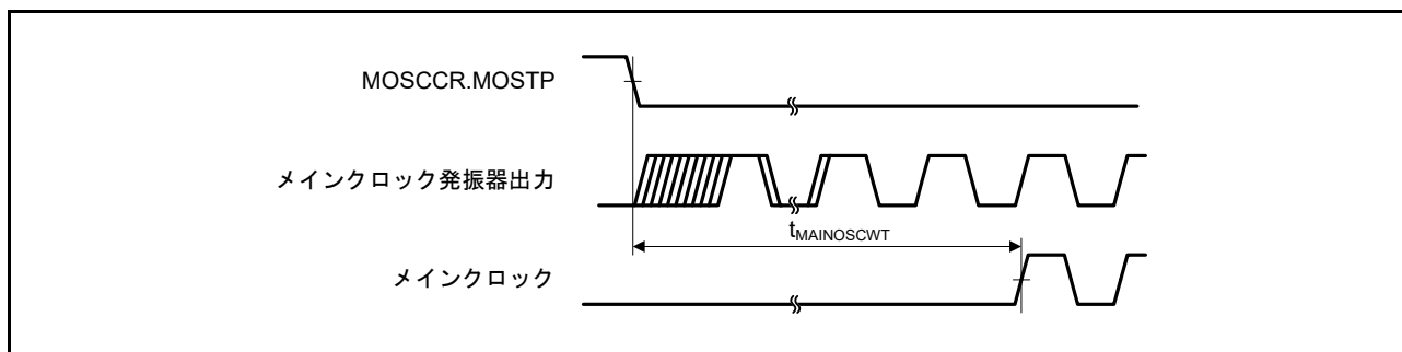
図 50.30 メインクロック発振開始タイミング
