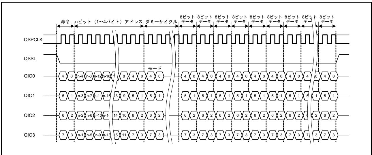
図 33.7 Quad-SPI プロトコル例 (ファストリード)
