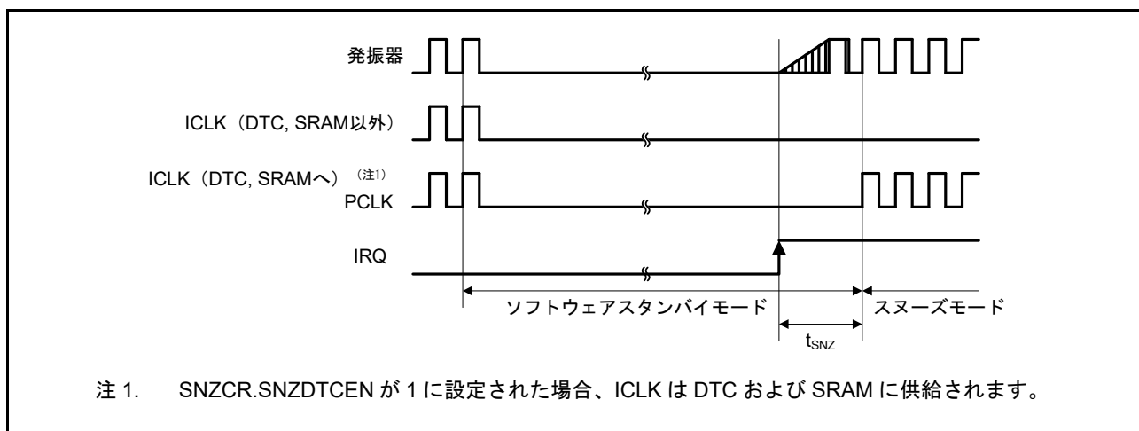
図 50.37 ソフトウェアスタンバイモードからスヌーズモードへの復帰タイミング
