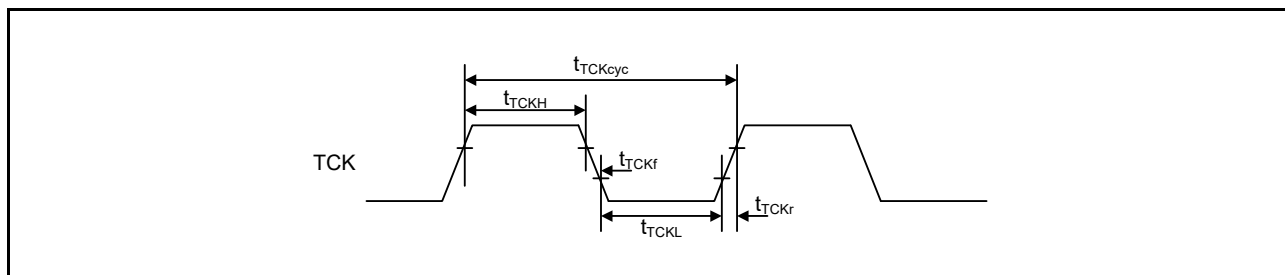
図 50.94 バウンダリスキャン TCK タイミング
