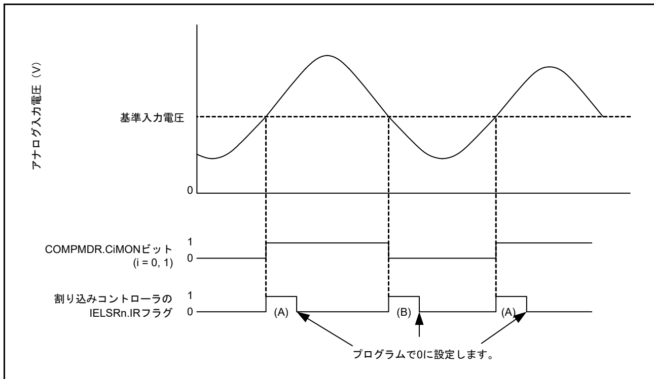
図 42.3 ウィンドウ機能無効時の ACMPLPi (i = 0, 1) の動作例
