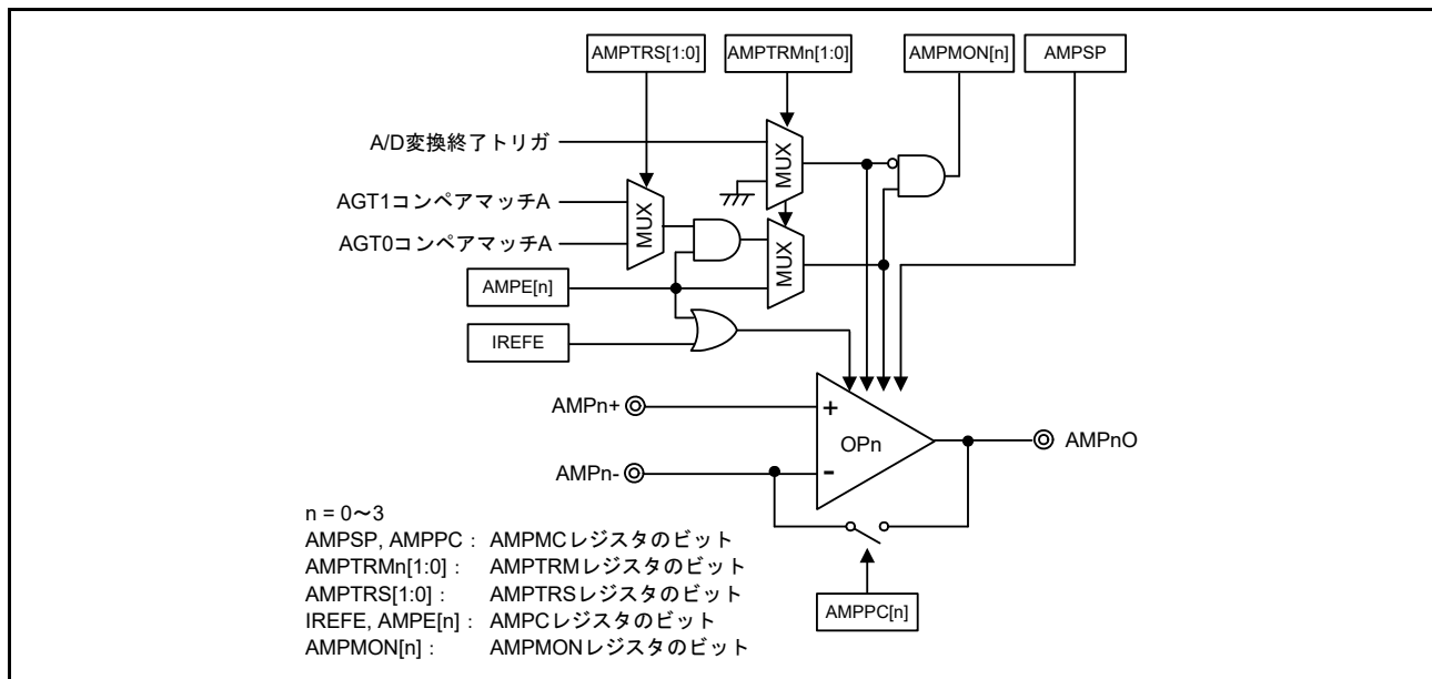
図 41.1 オペアンプのブロック図
