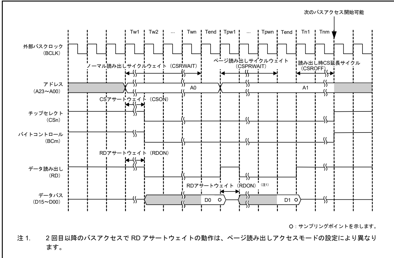
図 15.17 ページリードアクセスのタイミング (n = 0 ~ 3, m = 0, 1)
