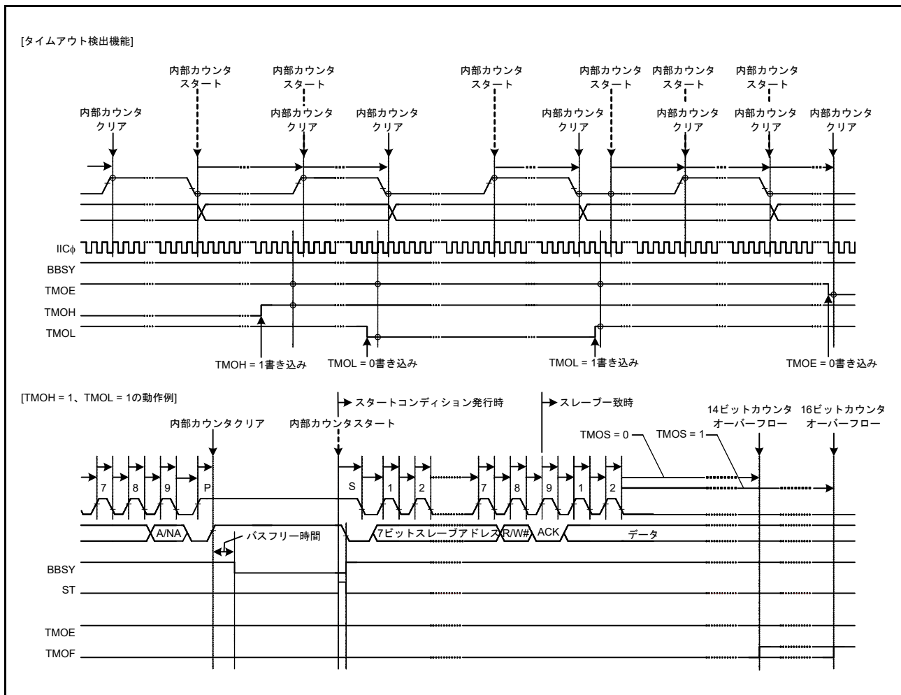
図 30.48 タイムアウト検出機能 (TMOE、TMOS、TMOH、TMOL ビット使用)
