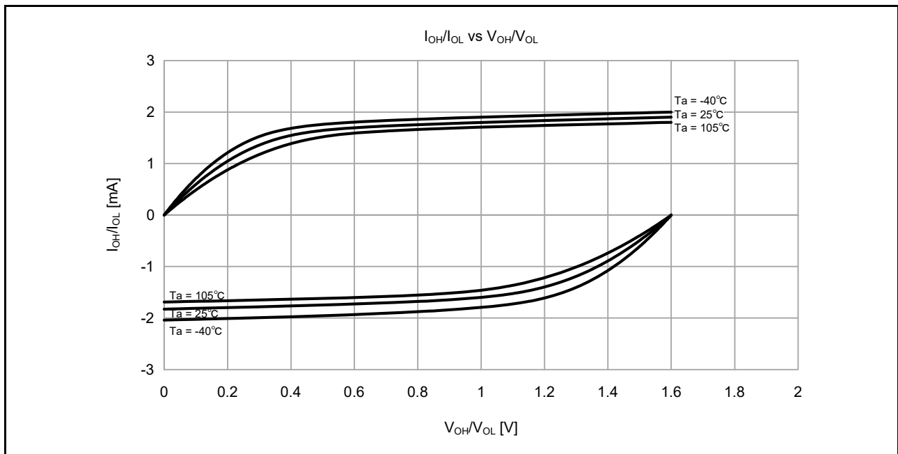
図 50.3 低駆動出力選択時の VCC = 1.6V での V OH /V OL および I OH /I OL 温度特性 (参考データ)
