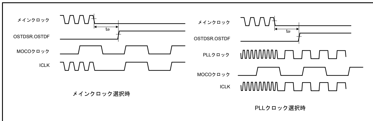
図 50.84 発振停止検出タイミング
