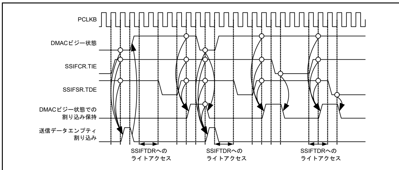
図 35.21 送信データエンプティ割り込みのタイミング
