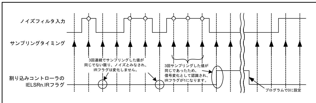
図 42.6 ノイズフィルタおよび割り込みの動作例
