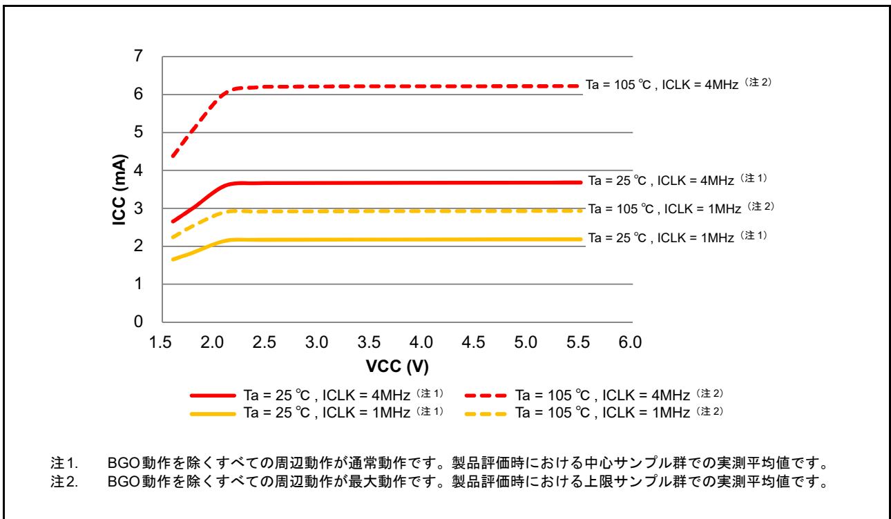
図 50.20 Low-voltage モードにおける電圧依存性 (参考データ)
