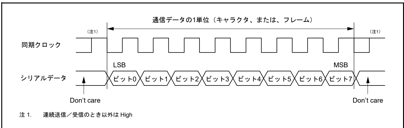
図 29.31 クロック同期式シリアル通信のデータフォーマット (LSB ファーストの並び順の場合)
