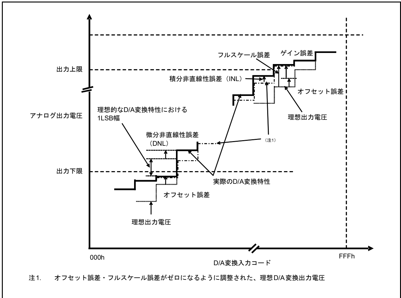
図 50.83 D/A コンバータ特性用語の解説図
