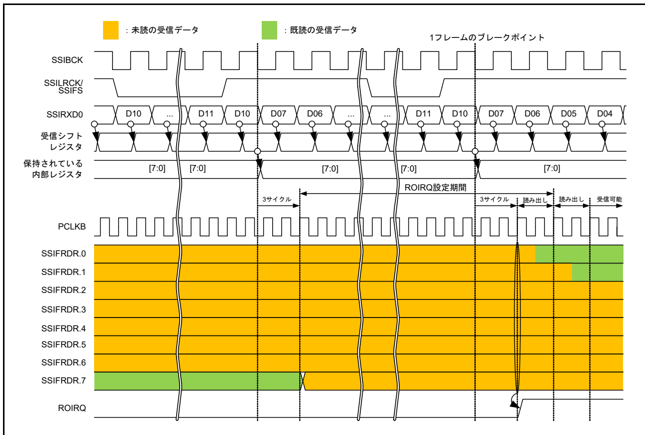
図 35.14 ROIRQ 設定タイミング
