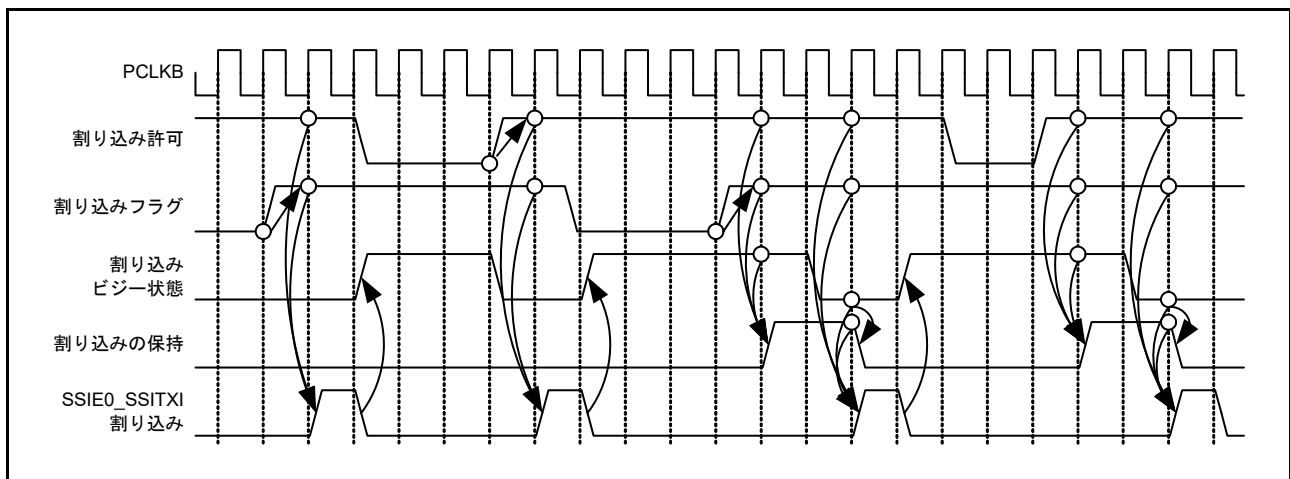
図 35.56 SSIE0_SSITXI 割り込みのタイミング図
