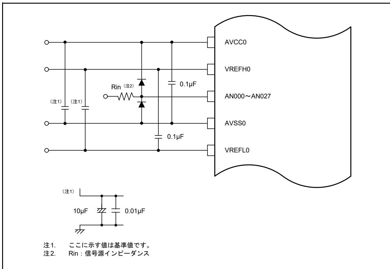
図 38.32 アナログ入力用保護回路例
