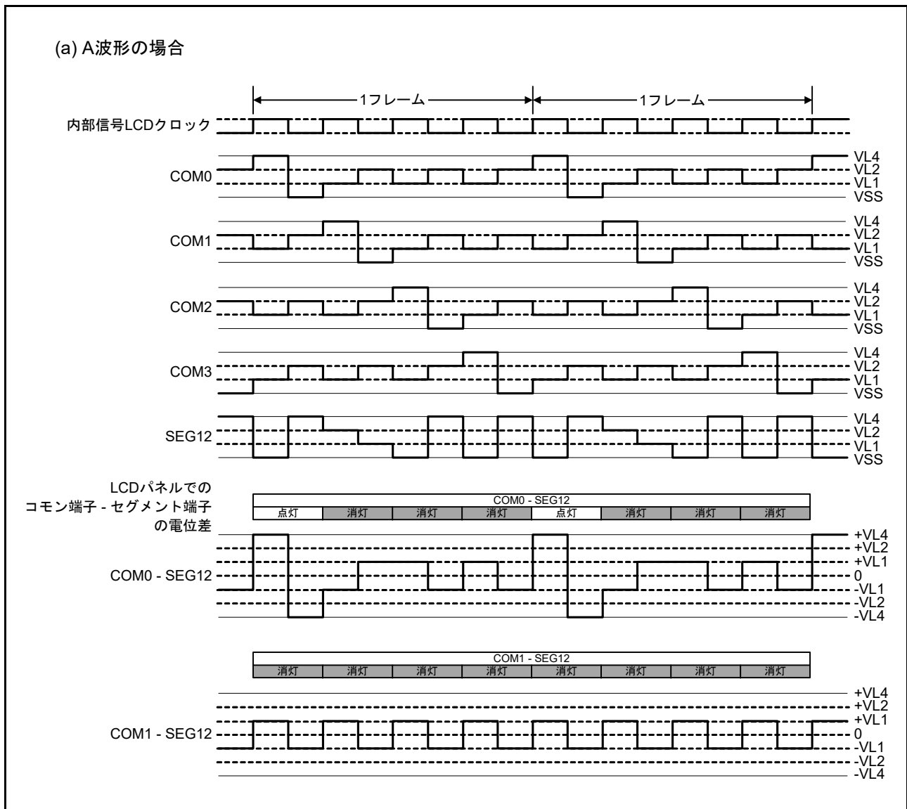
図 48.30 1/3 バイアス法を用いた SEG12 と各コモン信号との間の 4 時分割 LCD 駆動波形例 (1/2)
