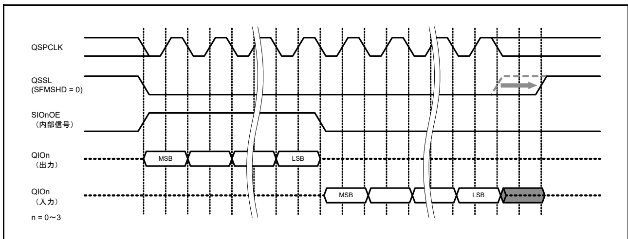
図 33.11 SFMSHD ビットを使用した QSSL 信号のホールド時間調整
