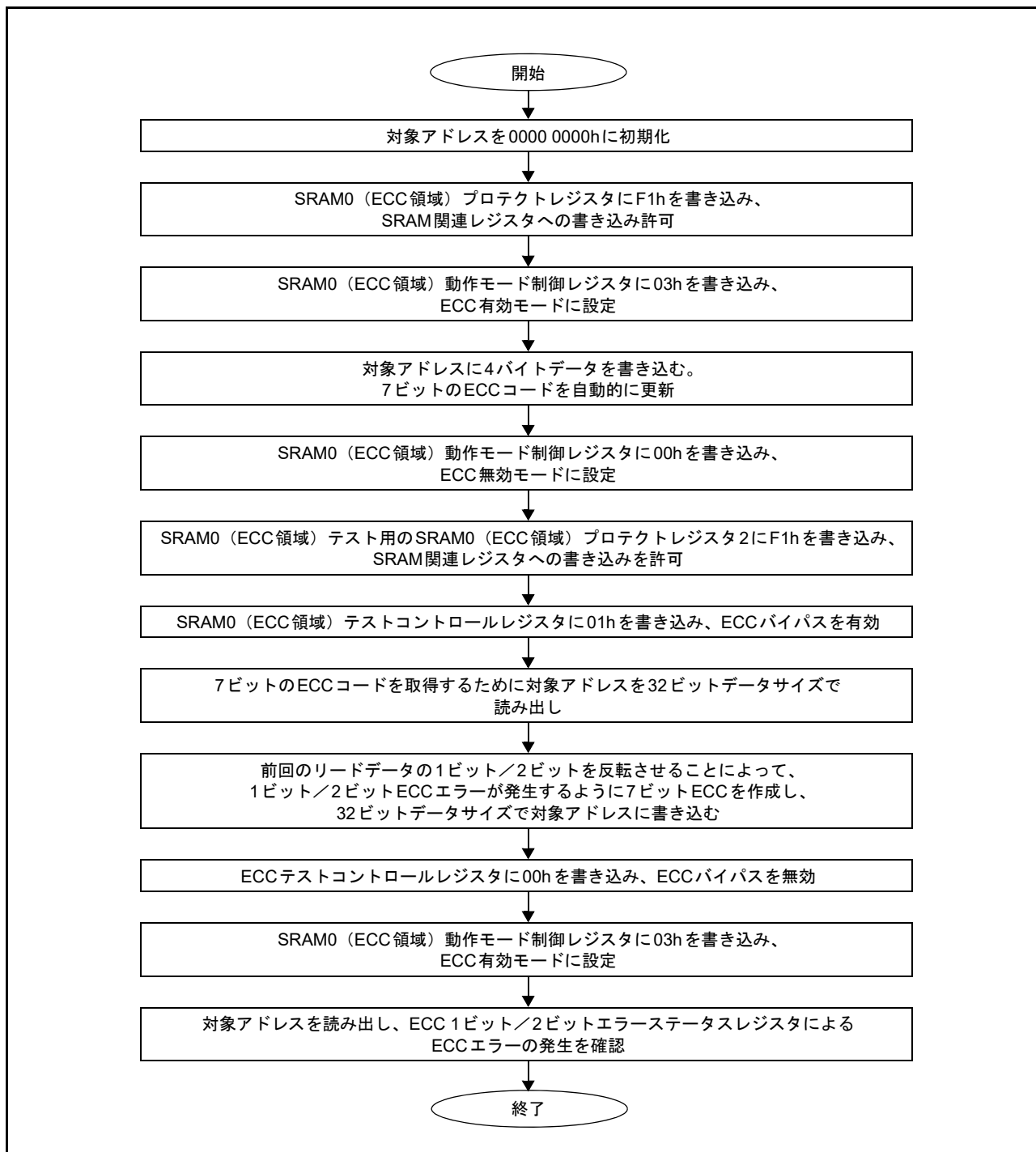
図 46.1 ECC デコーダのテスト方法
