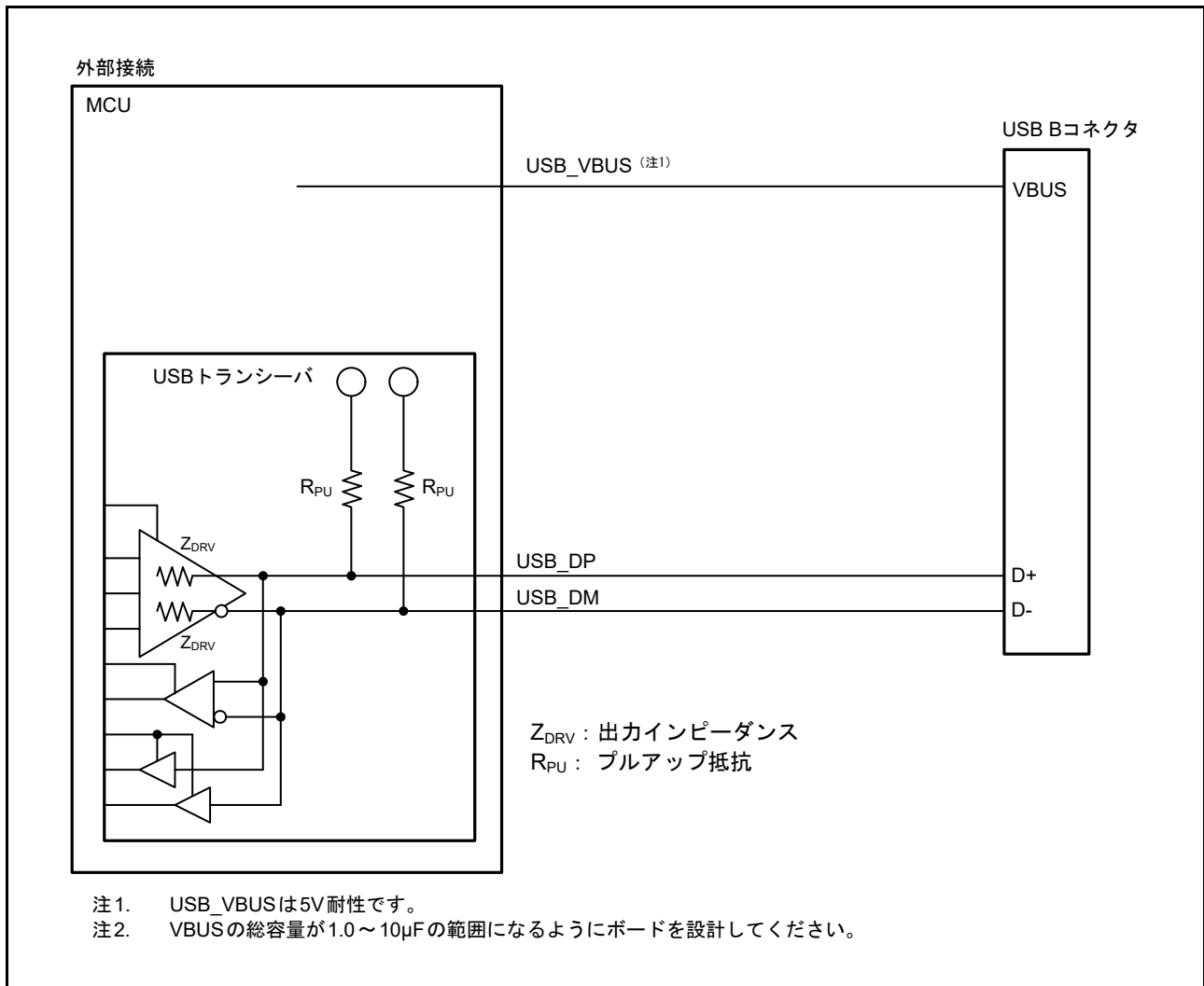
図 28.9 バスパワー状態 2 でのデバイス接続例
