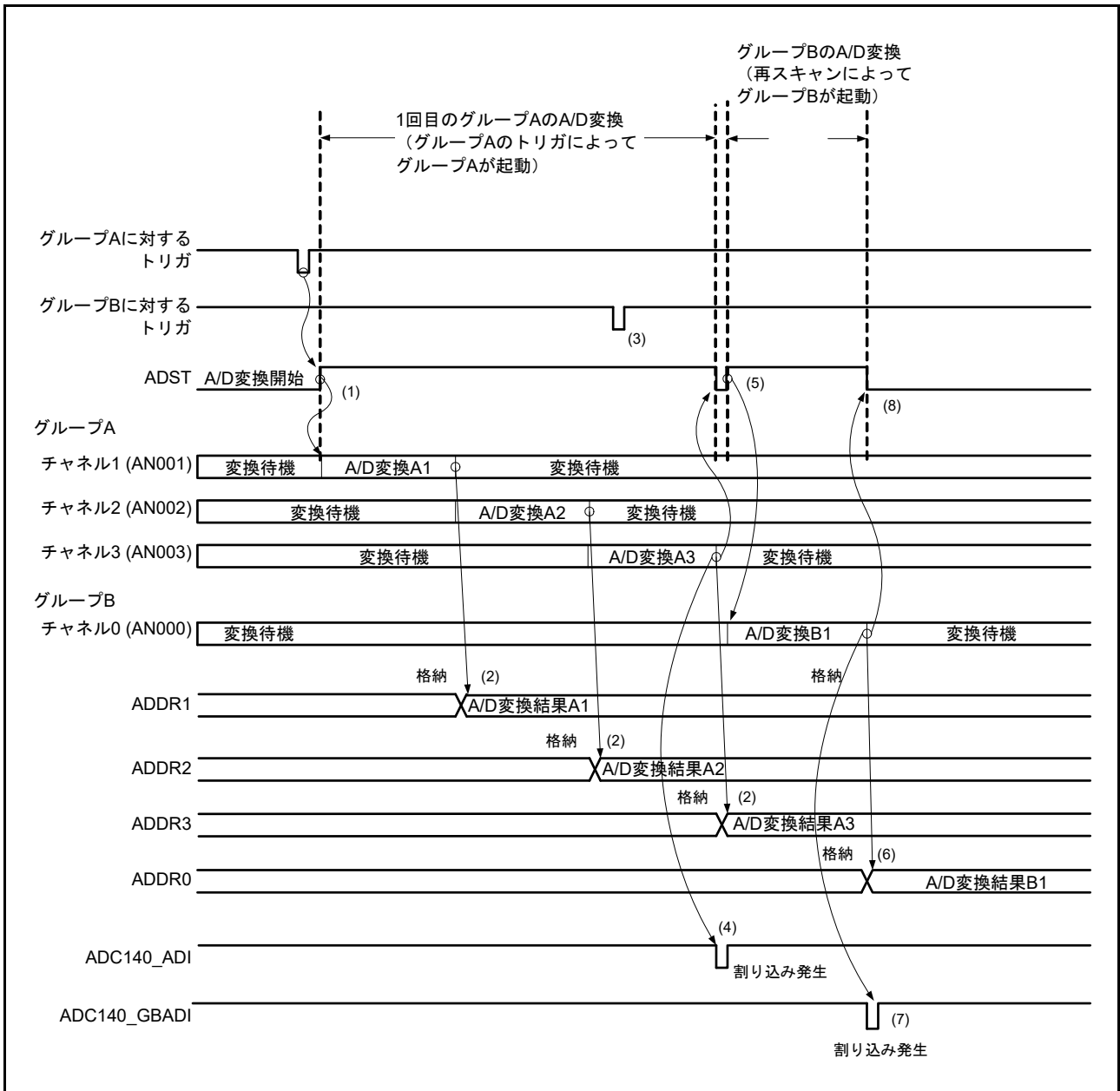
図 38.18 グループ A 優先制御の動作例 (3) (ADGSPCR.GBRSCN = 1, ADGSPCR.GBRP = 0 の場合)
