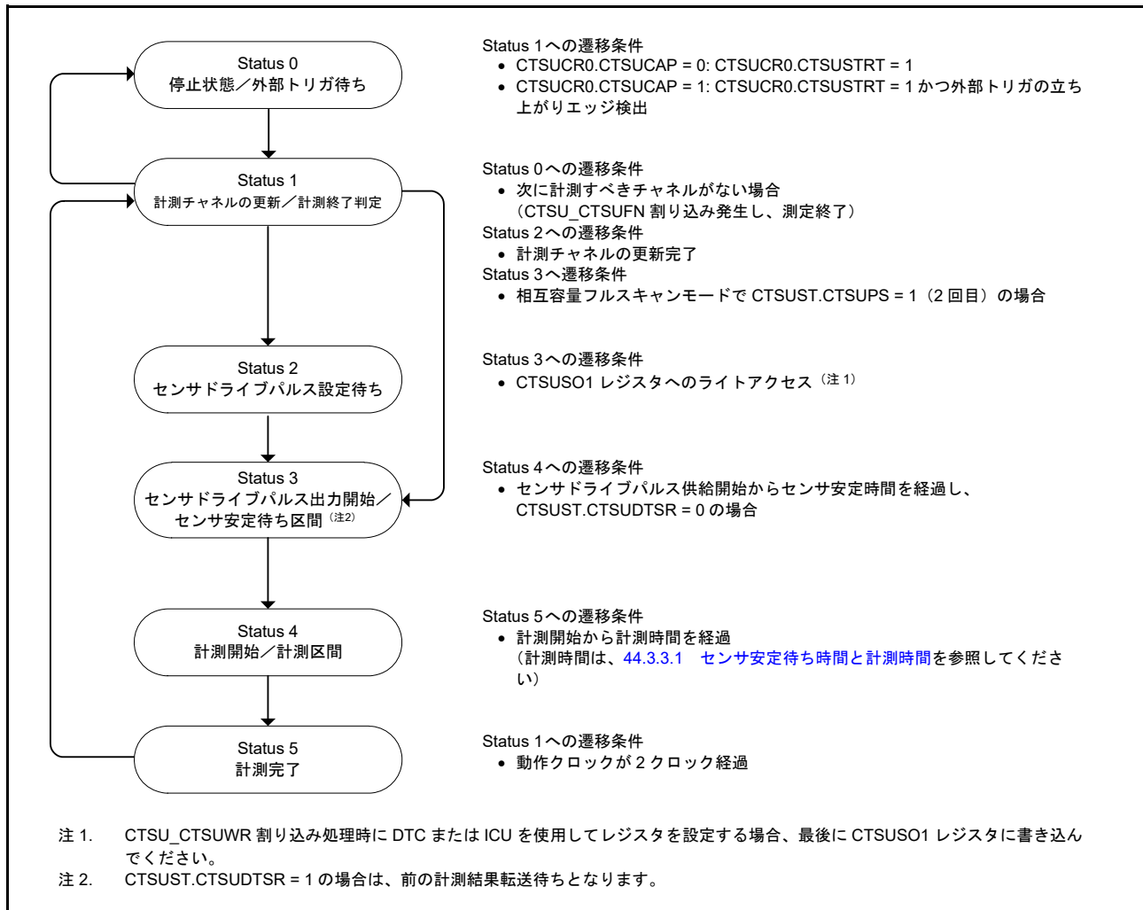
図 44.11 ステータス動作遷移図
