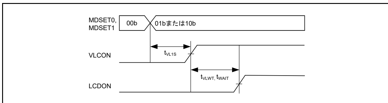
図 50.93 LCD 基準電圧セットアップ時間、昇圧待機時間、容量分割待機時間
