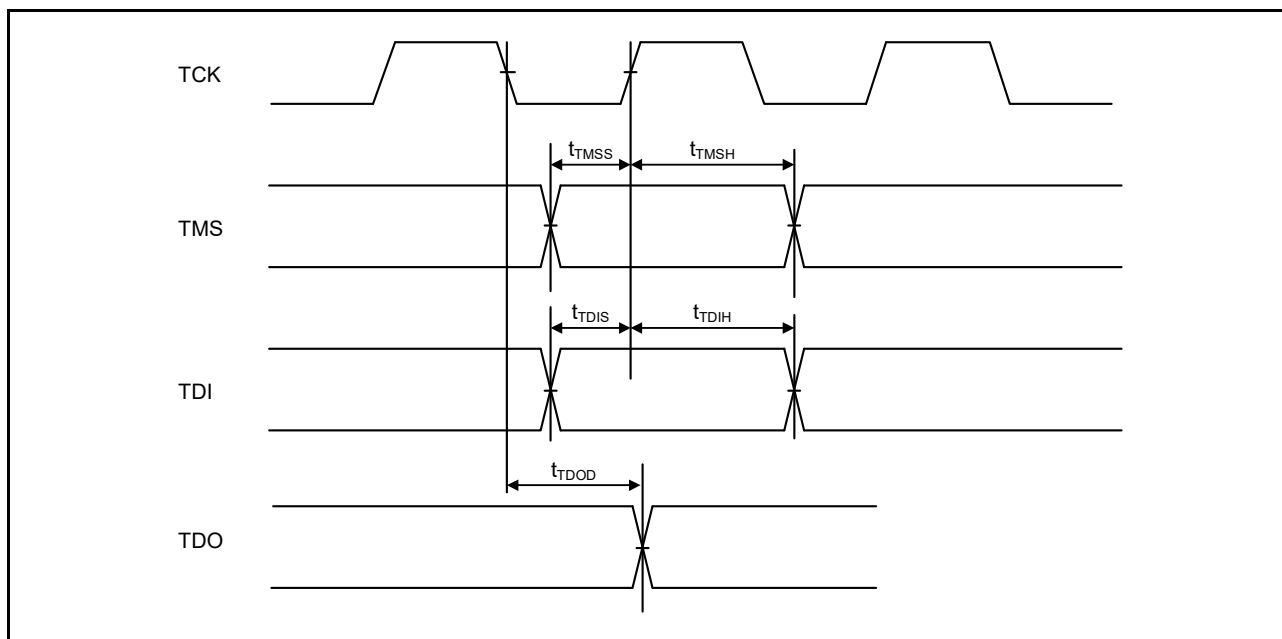
図 50.98 JTAG 入出カタイミング
