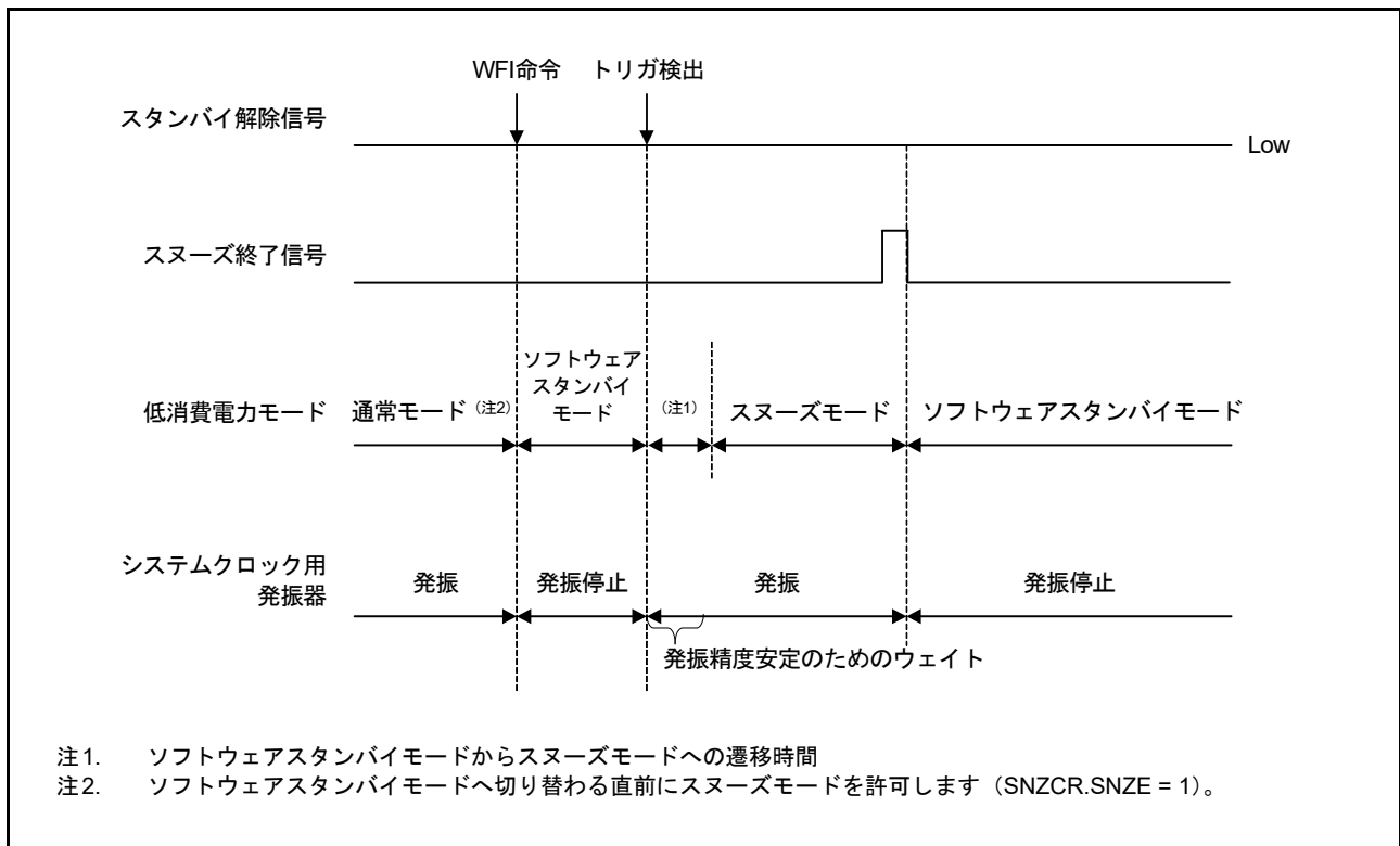
図 11.10 割り込み要求信号が発生しない場合のスヌーズモードの解除
