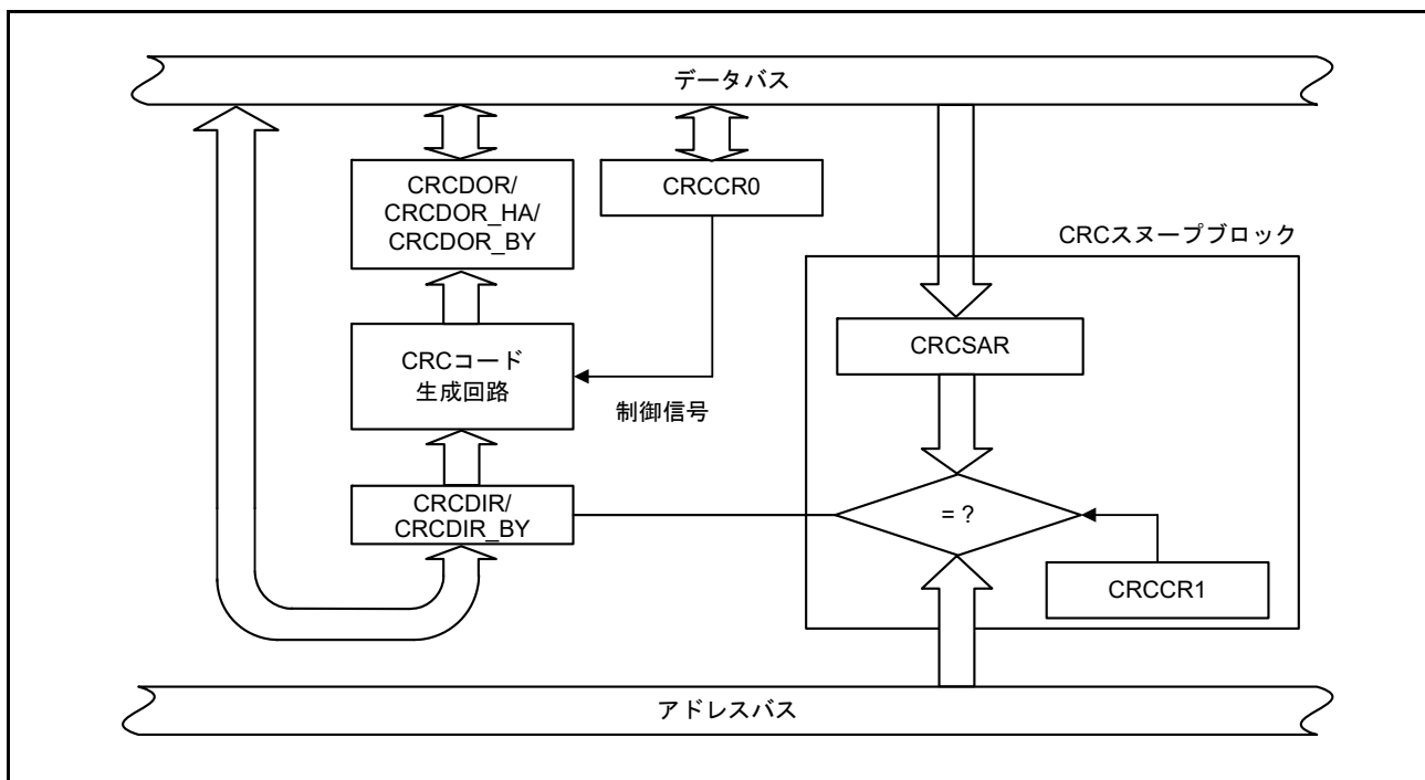
図 34.1 CRC 演算器のブロック図
