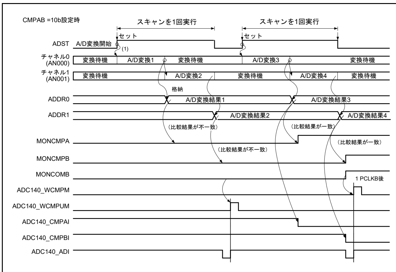
図 38.23 コンペア機能のイベント出力動作例 (AN000 と AN001 を比較)
