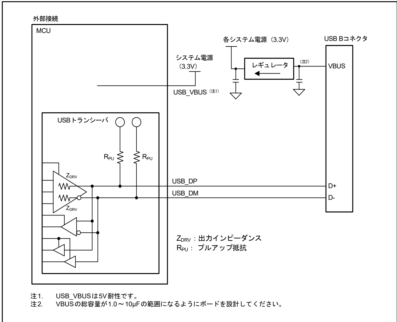
図 28.8 バスパワー状態 1 でのデバイス接続例
