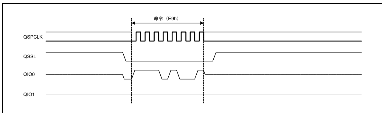
図 33.28 4 バイトモード解除命令のバスサイクル
