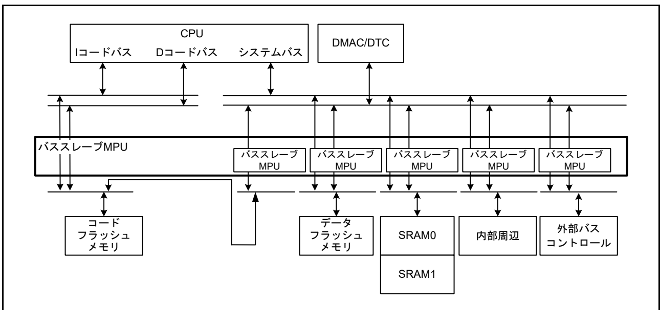
図 16.9 バススレーブ MPU のブロック図
