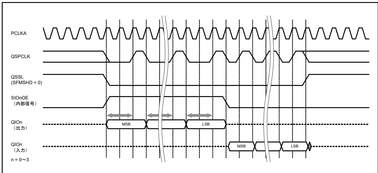
図 33.13 SFMOSW ビットを使用したシリアルデータ出力のセットアップ時間調整
