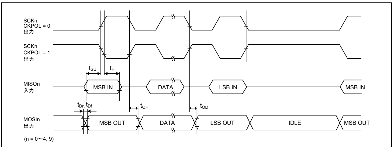
図 50.56 SCI 簡易 SPI モードタイミング (マスタ、CKPH = 1)
