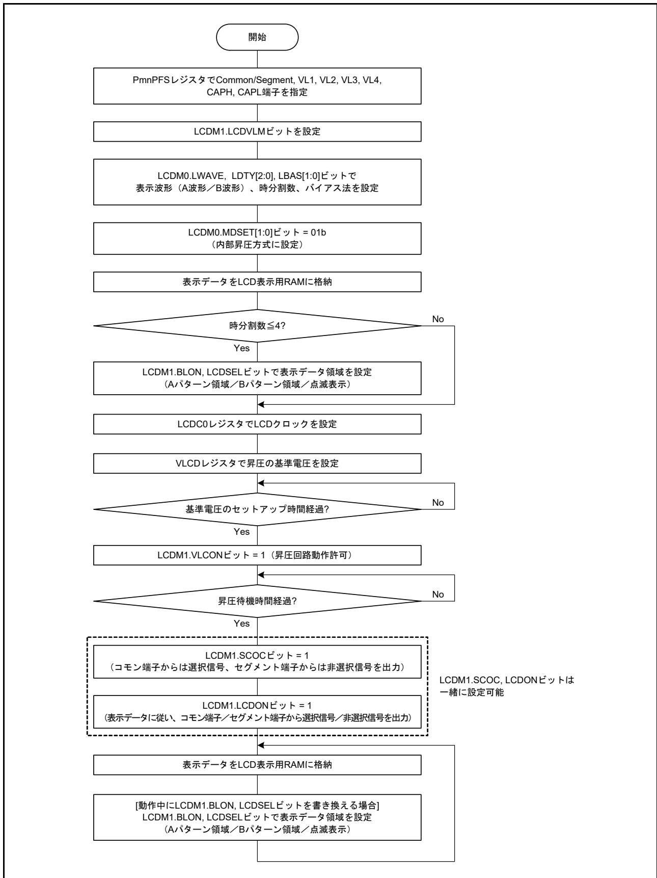
図 48.6 通常液晶波形表示での内部昇圧方式の設定手順
