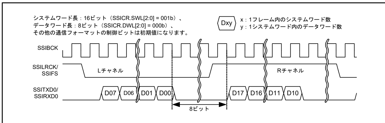
図 35.34 パディングビットの転送例 (I 2 S フォーマット、システムワード長>データワード長)
