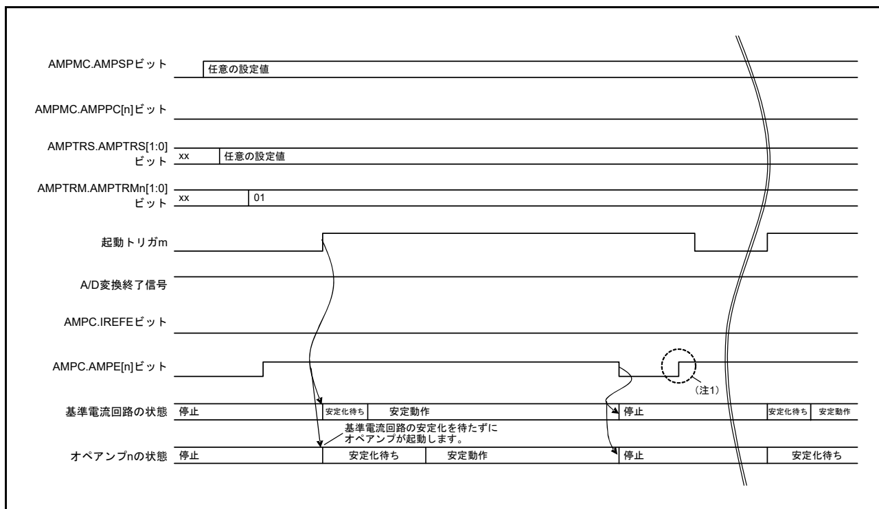
図 41.4 オペアンプの制御動作 (起動トリガモードによる起動) (基準電流回路およびオペアンプを起動トリガによって起動し、AMPC レジスタ設定によって停止する場合)
