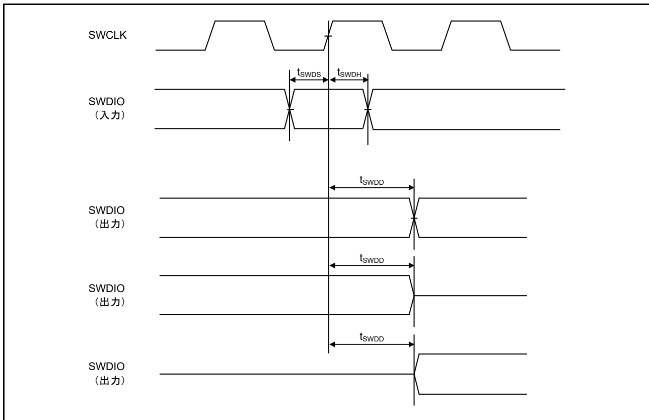
図 50.100 SWD 入出力タイミング
