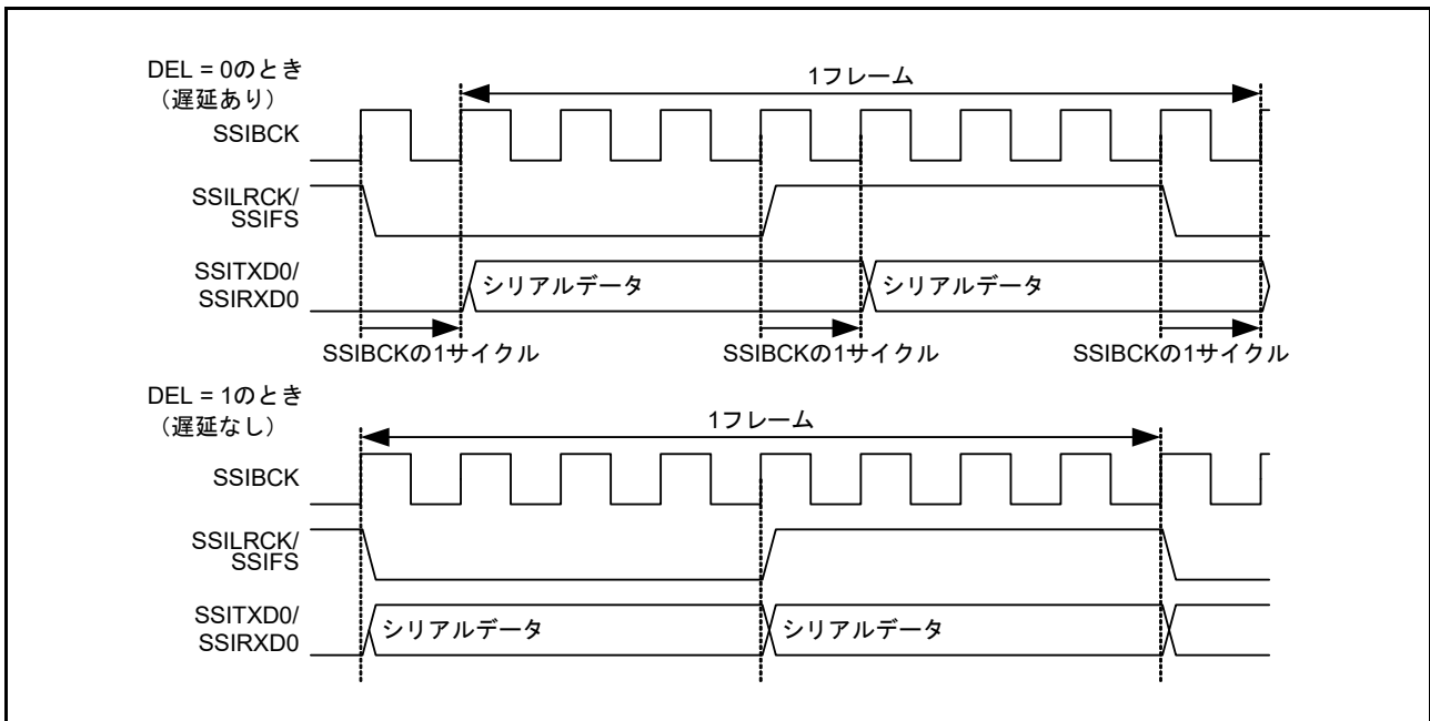
図 35.6 シリアルデータディレイの設定
