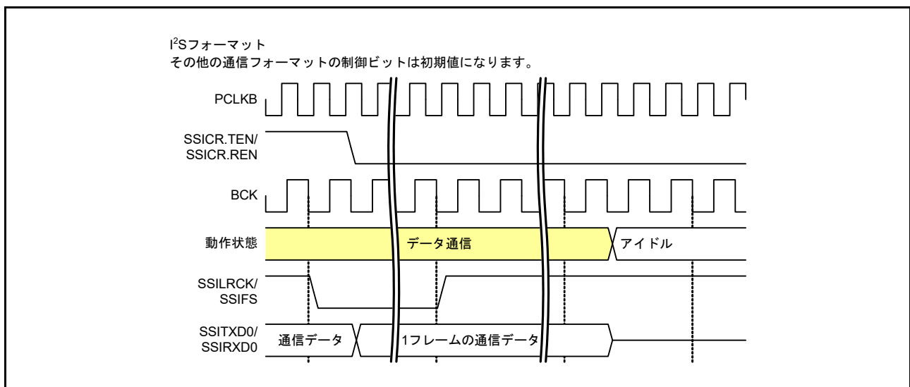
図 35.44 データ通信からの停止 (パディングビットなし)
