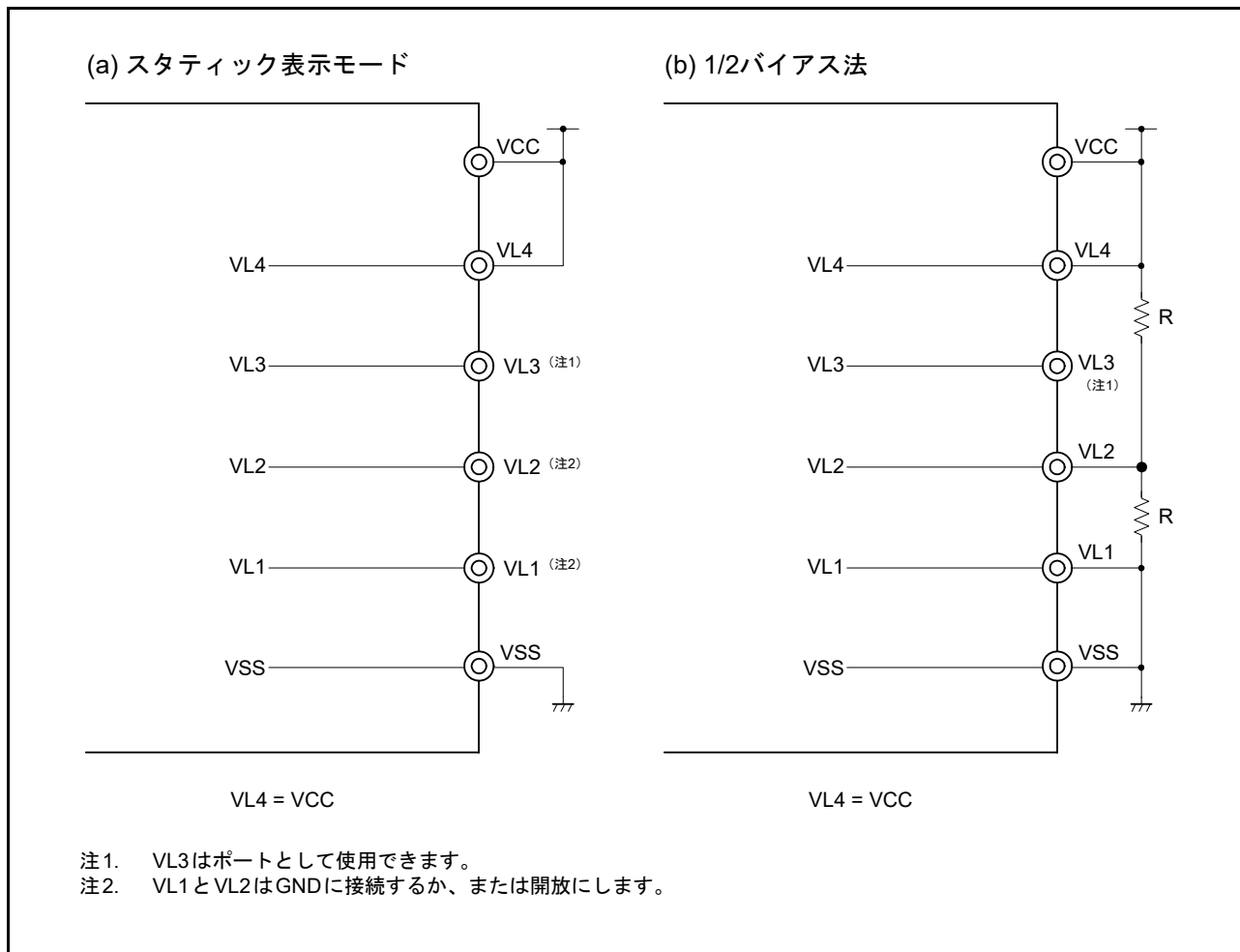
図 48.9 LCD 駆動電源の接続例 (外部抵抗分割方式) (1/2)
