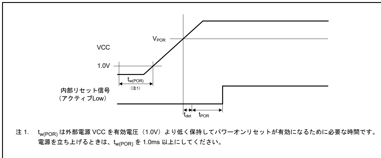
図 50.86 パワーオンリセットタイミング
