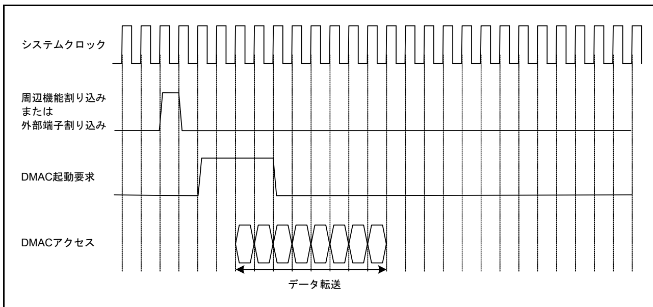
図 17.11 DMAC 動作タイミング例 2: 周辺モジュールまたは外部割り込み入力端子からの割り込みによる DMA 起動 (ブロック転送モードでブロックサイズ = 4 の場合)
