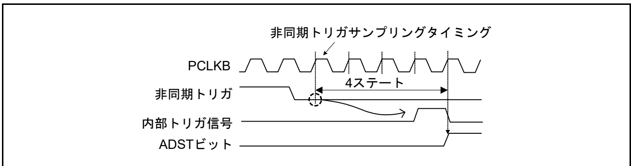
図 38.29 非同期トリガ入力タイミング
