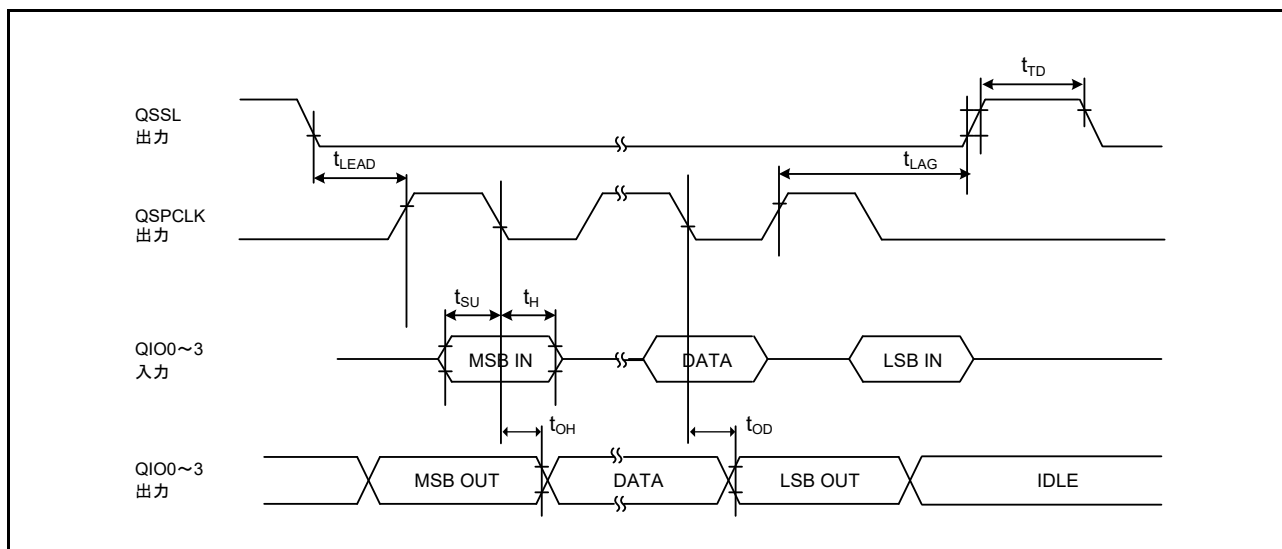
図 50.69 送受信タイミング
