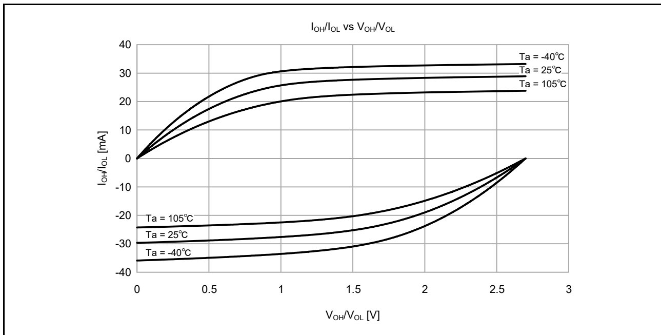
図 50.9 中駆動出力選択時の VCC = 2.7V での V_{OH}/V_{OL} および I_{OH}/I_{OL} 温度特性 (参考データ)
