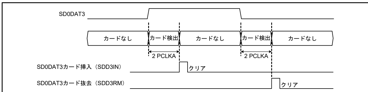
図 36.8 SD0DAT3 による SD カード検出
