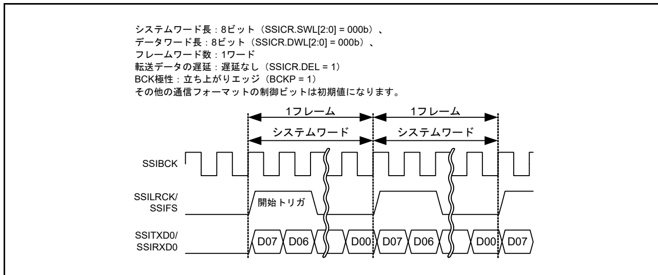
図 35.38 モノラルフォーマットでのロングフレーム (パディングなし)
