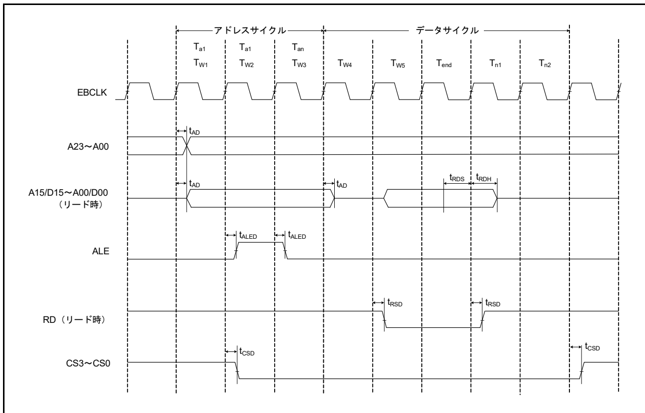
図 50.40 アドレス/データマルチプレクスバスのリードアクセスタイミング
