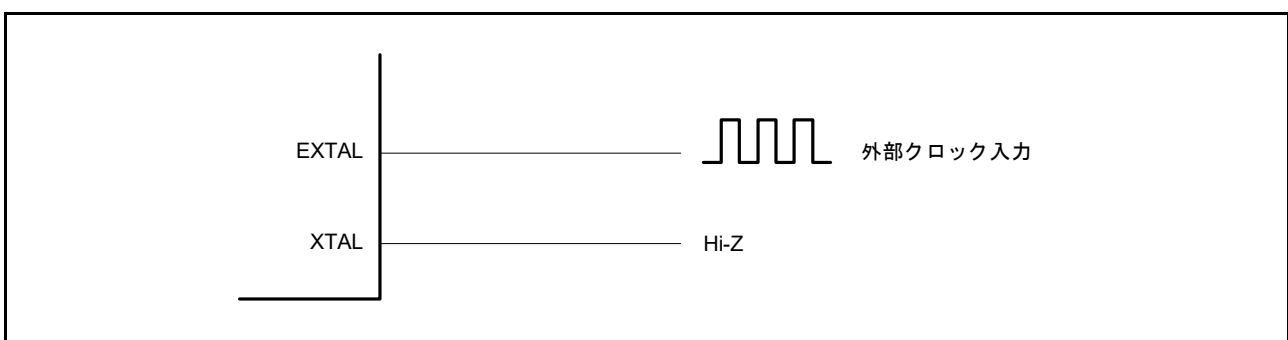
図 9.5 外部クロックの等価回路
