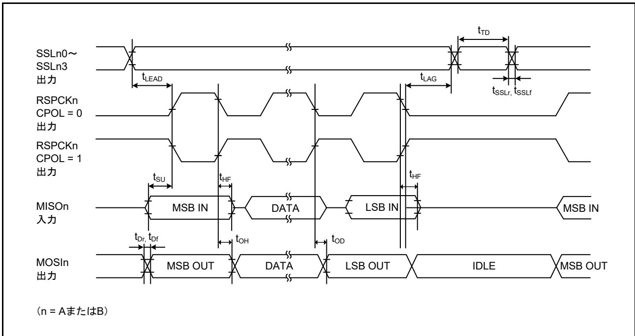
図 50.63 SPI タイミング (マスタ、CPHA = 0) (ビットレート : PCLKA を 2 分周に設定)
