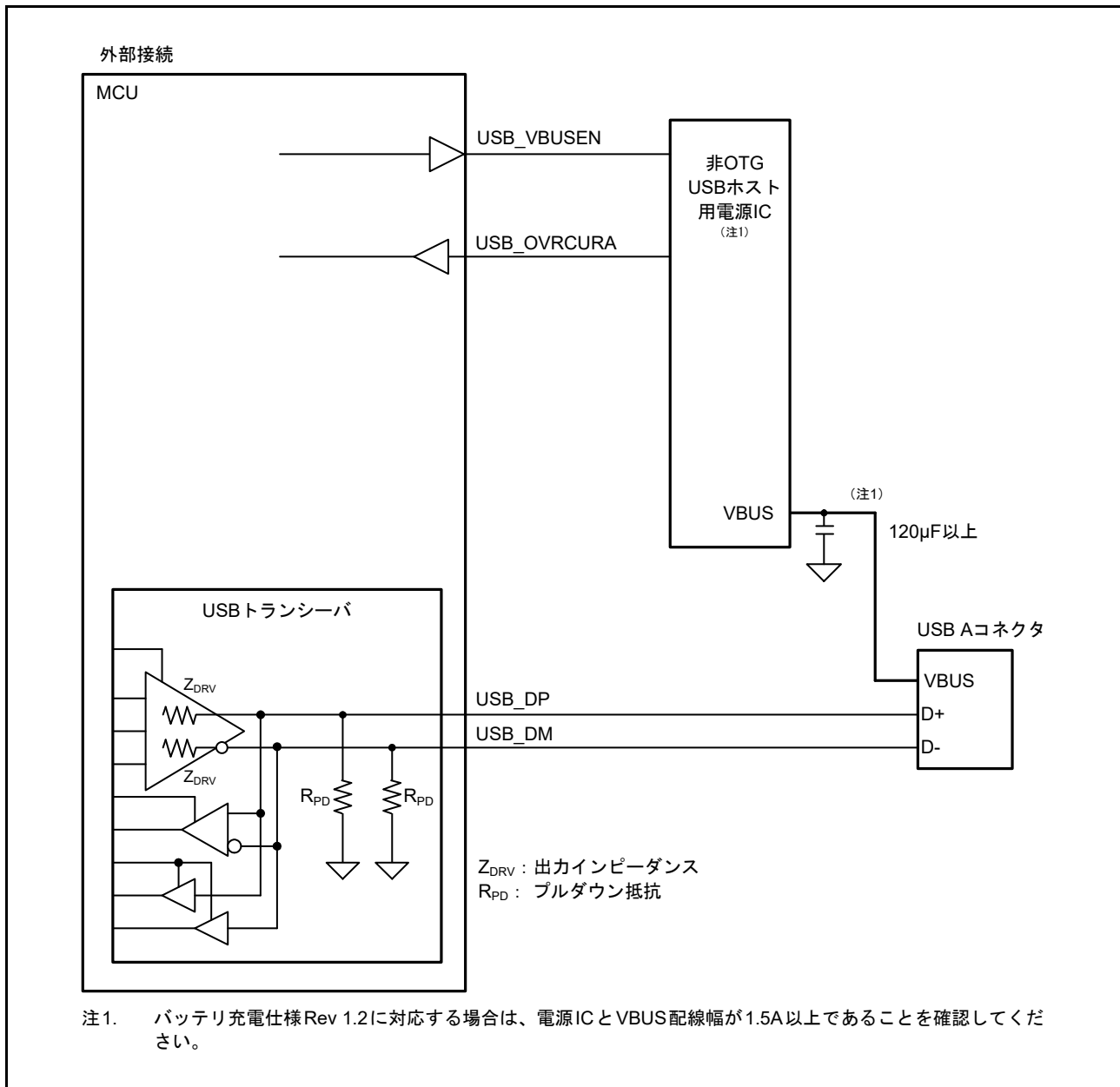
図 28.7 ホスト接続例
