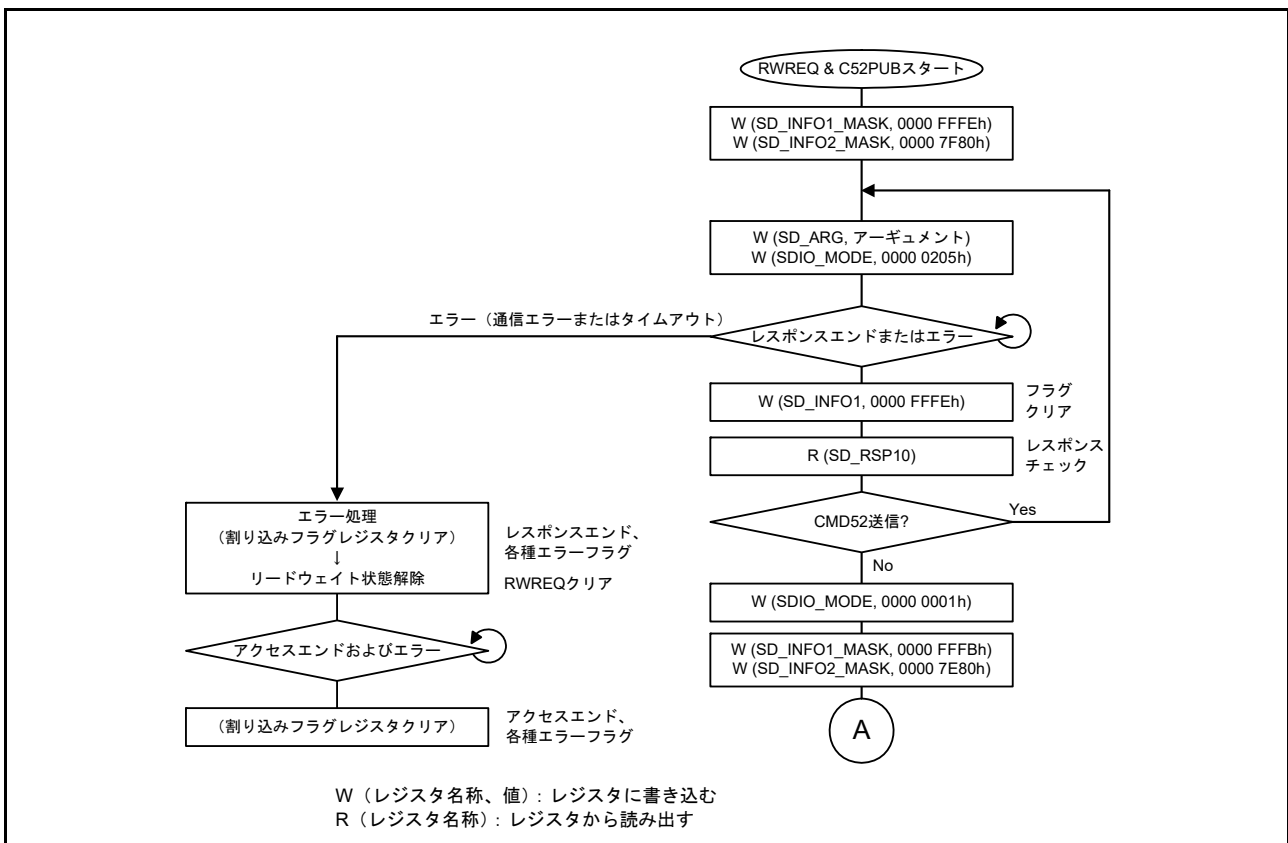
図 36.19 SD ホストインタフェースが Read Wait 状態で、CMD53 マルチブロックリード時に CMD52 (SDIO none abort) が送信される場合のフロー
