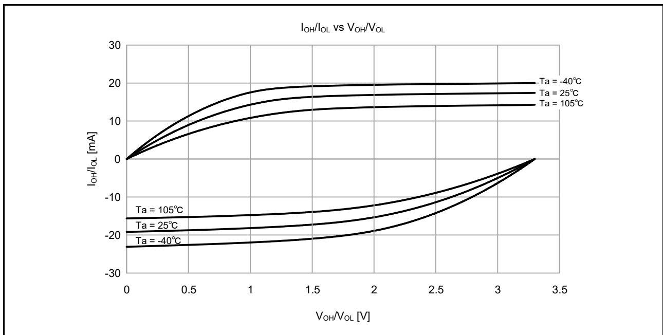
図 50.5 低駆動出力選択時の VCC = 3.3V での V_{OH}/V_{OL} および I_{OH}/I_{OL} 温度特性 (参考データ)
