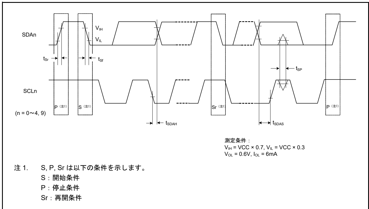
図 50.60 SCI 簡易 IIC モードタイミング
