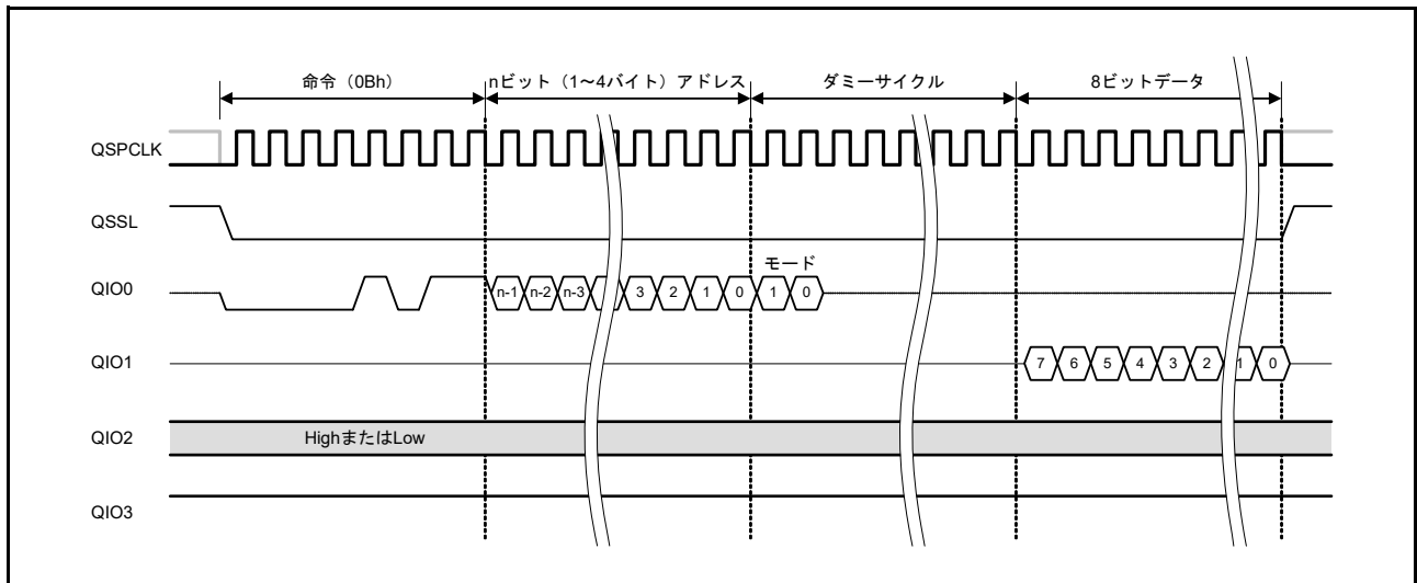
図 33.17 ファストリードバスサイクル
