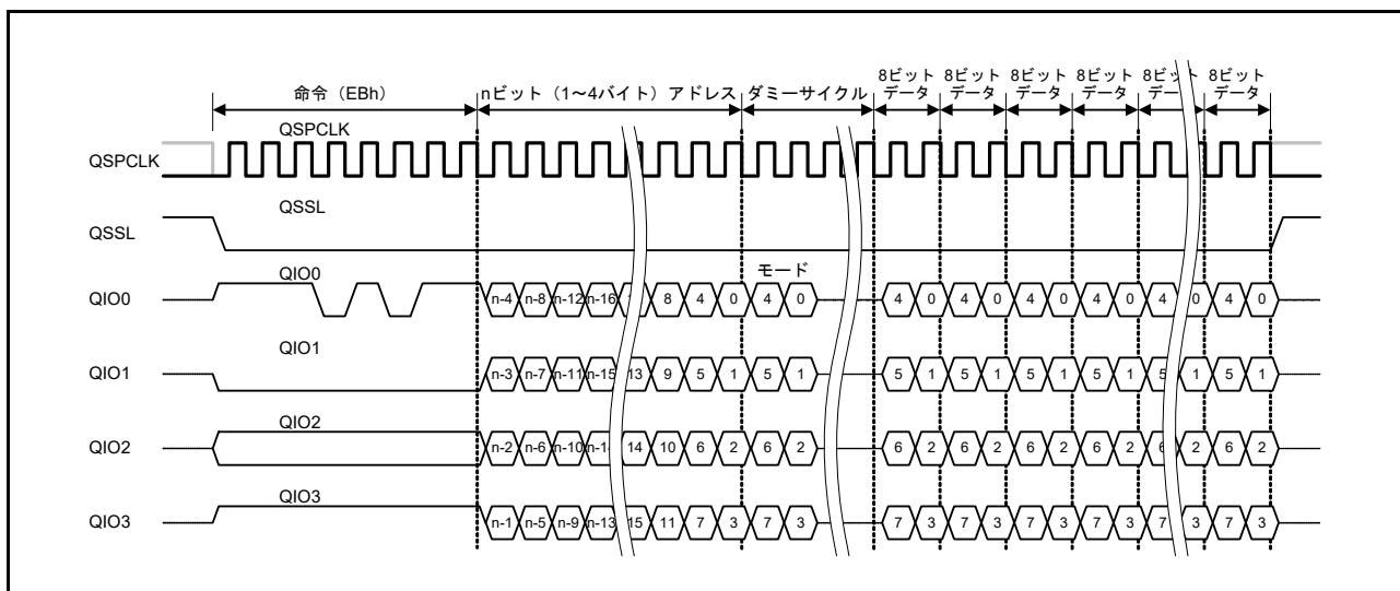
図 33.25 ファストリード Quad I/O バスサイクル
