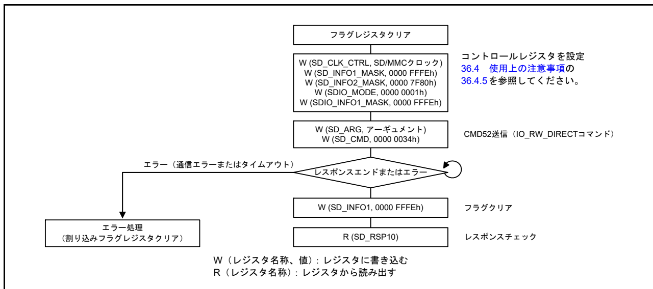
図 36.16 IO_RW_DIRECT コマンド (CMD52) 動作の例
