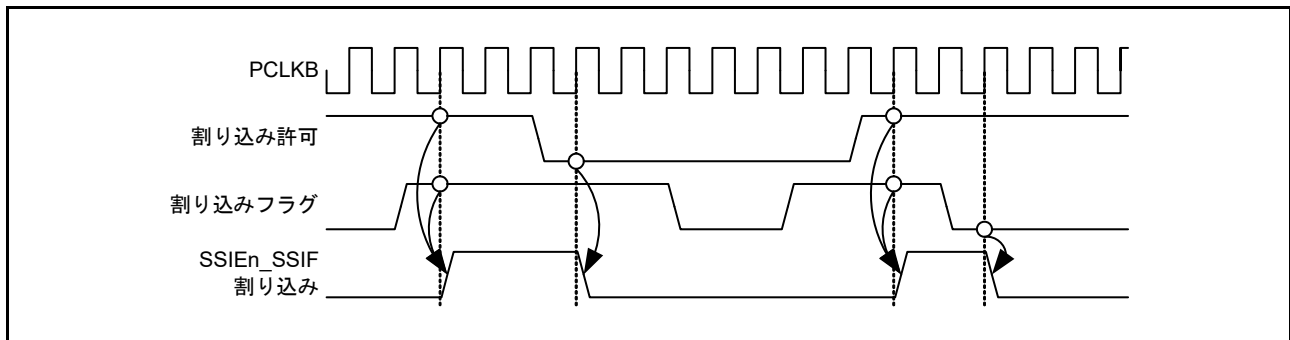
図 35.55 割り込み要因共通のタイミング図 (SSIE0_SSIF)
