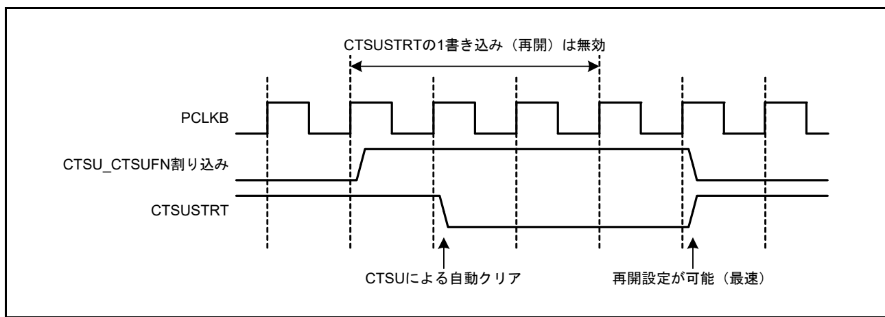
図 44.21 再開時の注意事項
