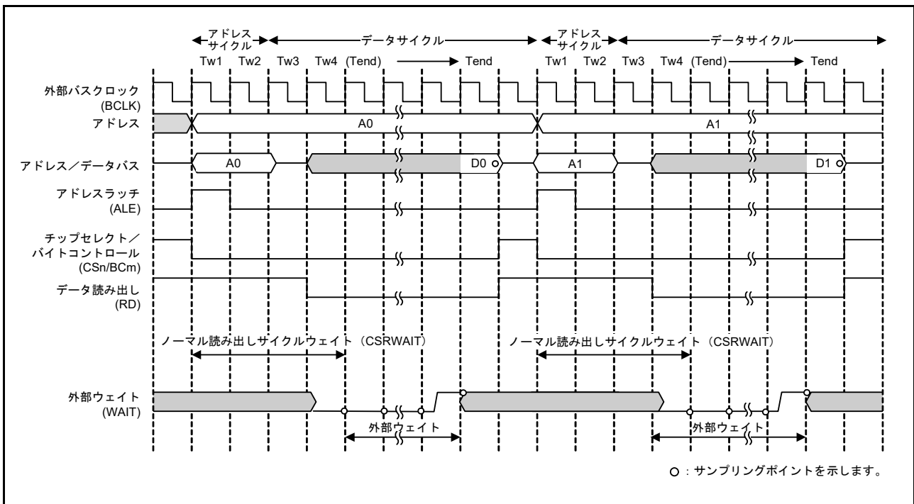
図 15.30 アドレス/データマルチプレクス I/O インタフェース時の外部ウェイト挿入のタイミング例 (m = 0, 1)
