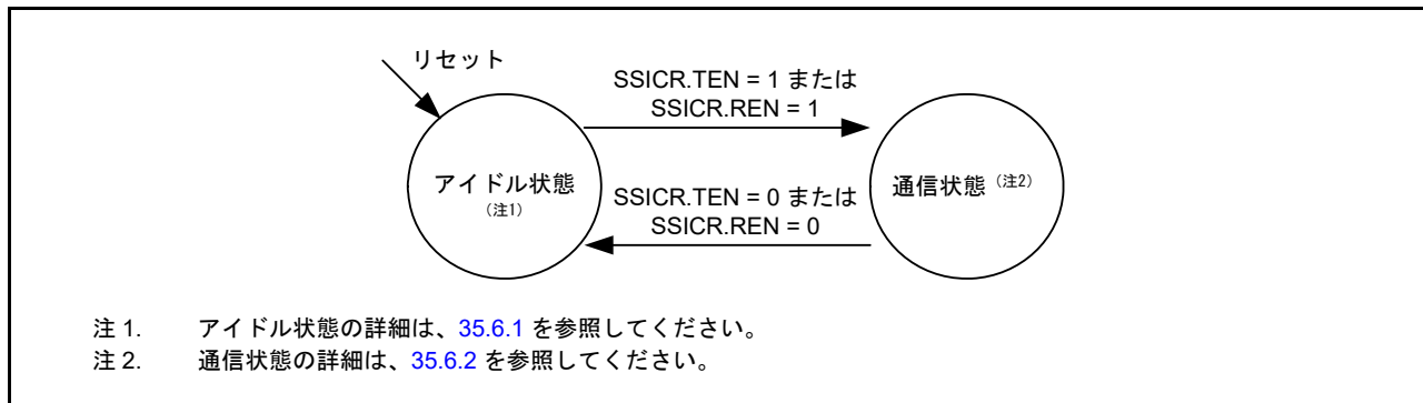
図 35.39 SSIE の状態遷移
