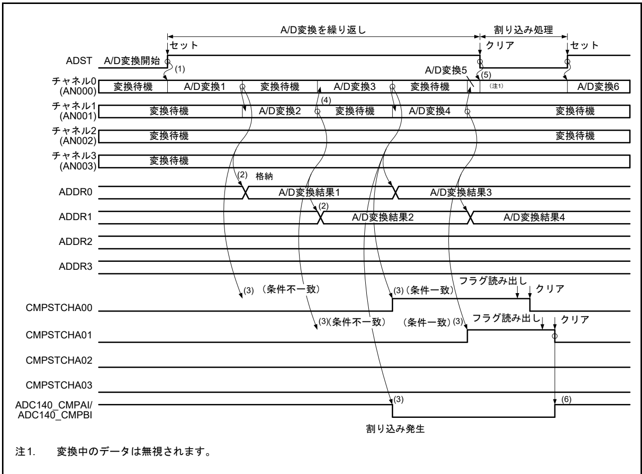
図 38.21 コンペア機能の動作例 (AN000 ~ AN003 を比較)
