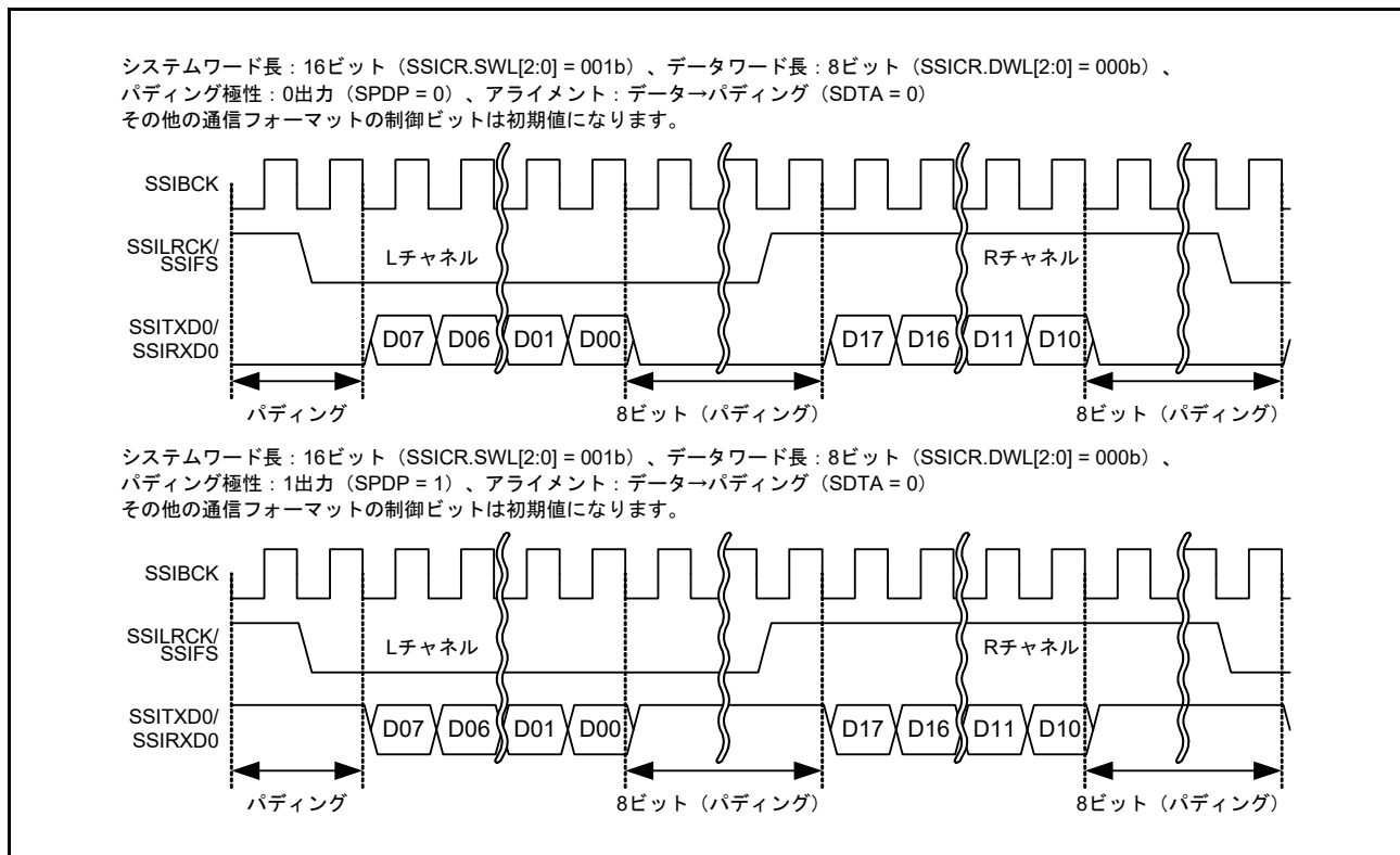
図 35.10 パディングビット極性
