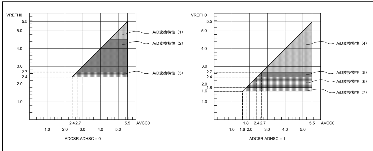
図 50.80 AVCC0 ~ VREFH0 電圧範囲
