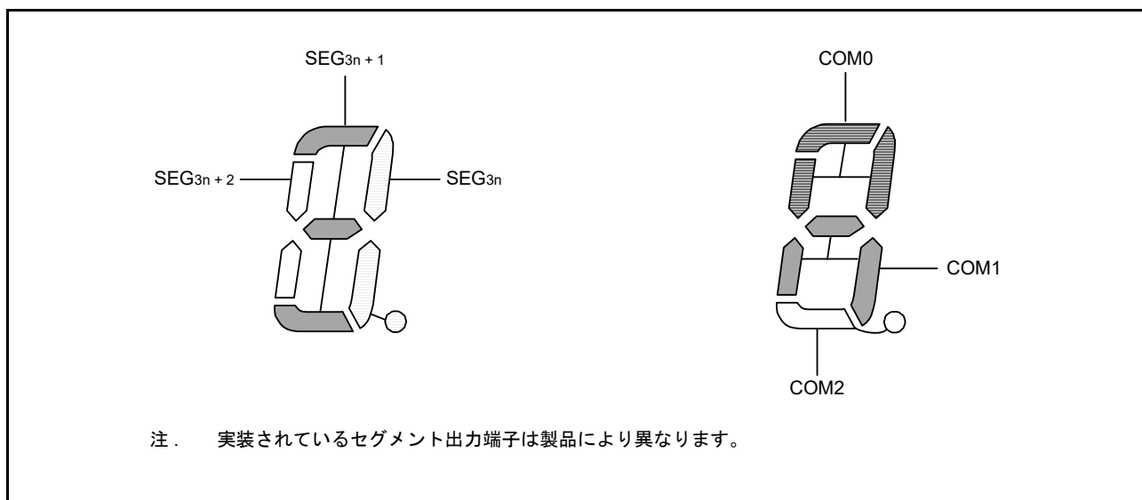
図 48.24 3 時分割 LCD 表示パターンと電極接続
