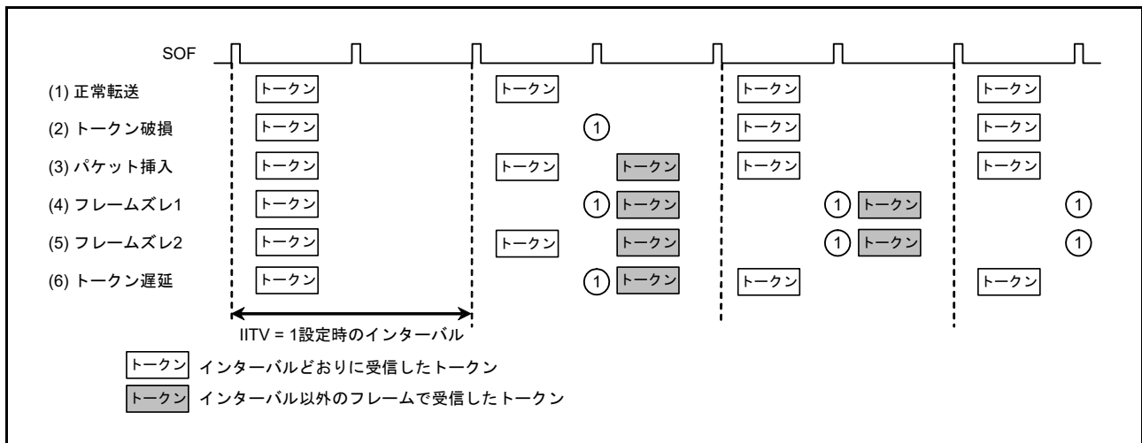
図 28.23 IITV = 1 の場合のインターバルエラー発生例
