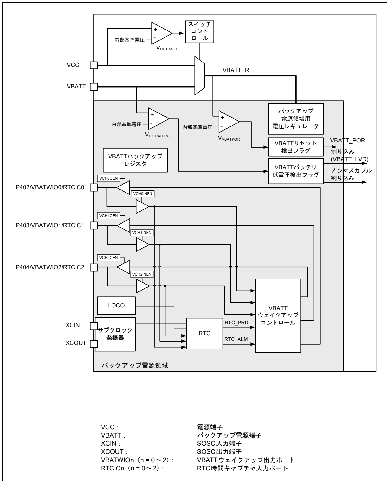
図 12.1 バッテリバックアップ機能の構成
