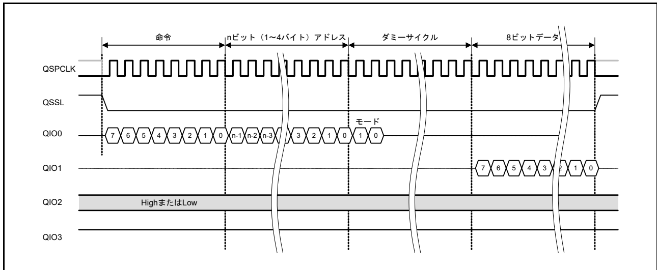
図 33.4 拡張 SPI プロトコル例 1 (ファストリード)
