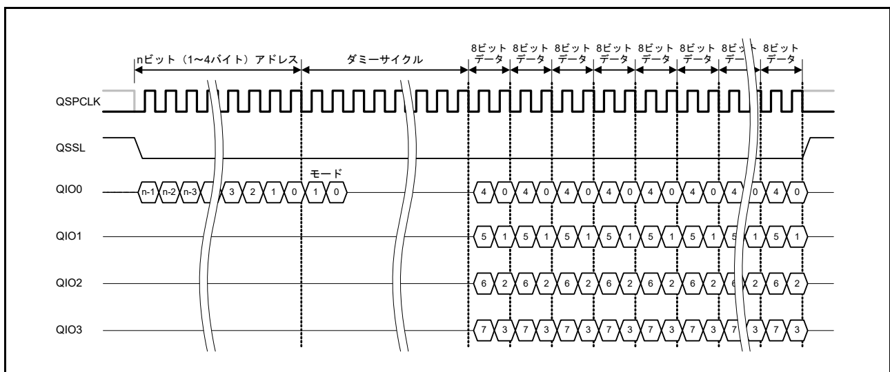
図 33.24 XIP モード時のファストリード Quad 出力バスサイクル
