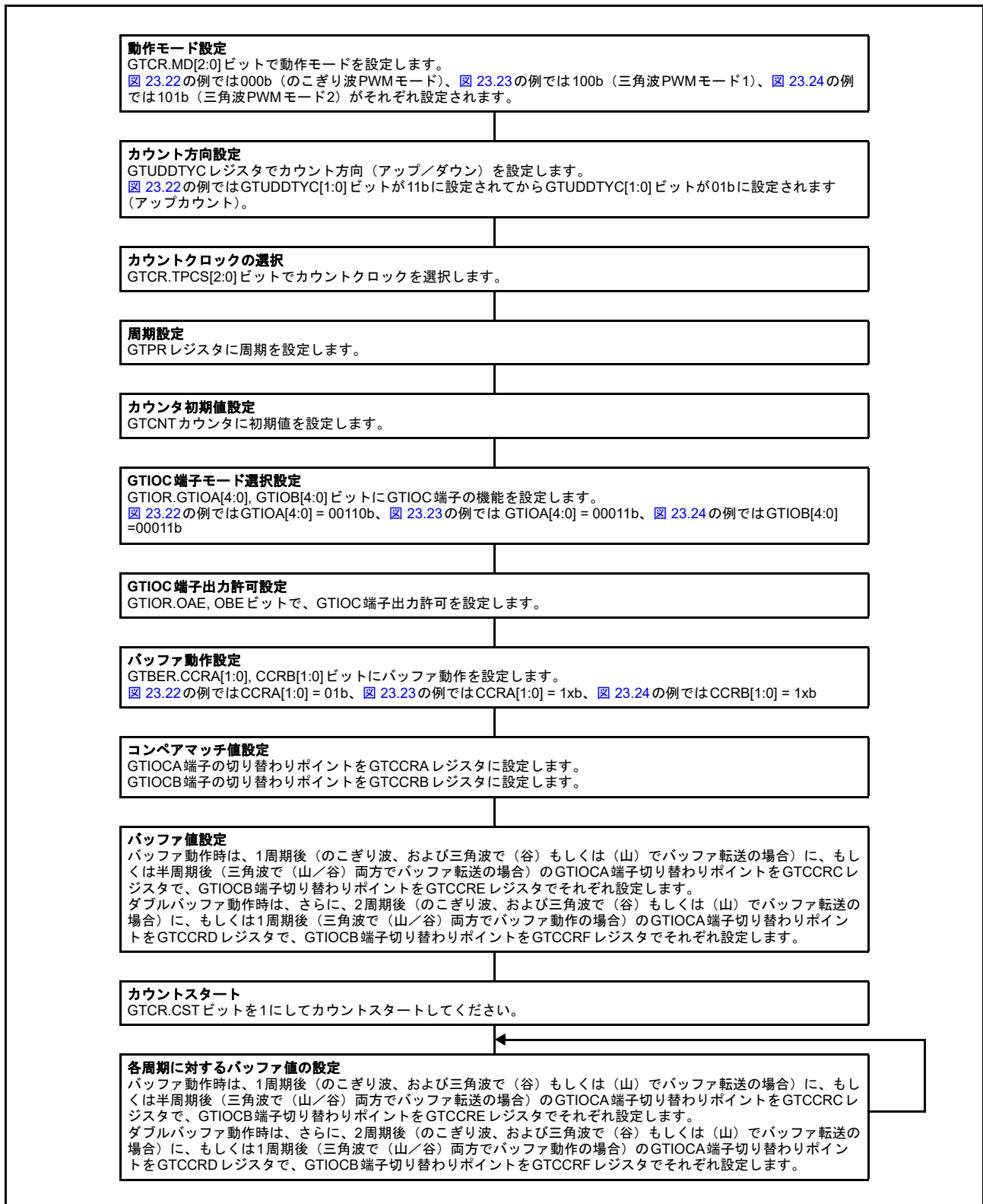
図 23.25 GTCRA、GTCCRB レジスタのバッファ動作の設定例 (アウトプットコンペア時)
