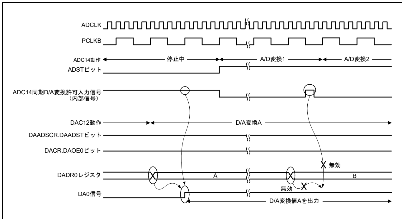
図 39.4 DAC12 が ADC14 同期 D/A 変換許可入力信号を取り込めない場合の例
