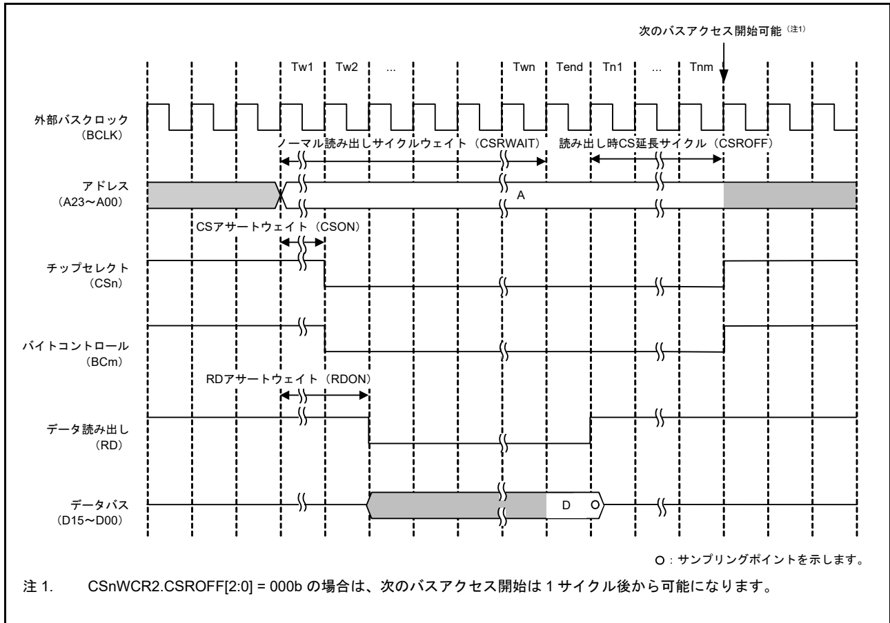
図 15.7 ノーマルリードアクセスのバスタイミング (n = 0 ~ 3, m = 0, 1)
