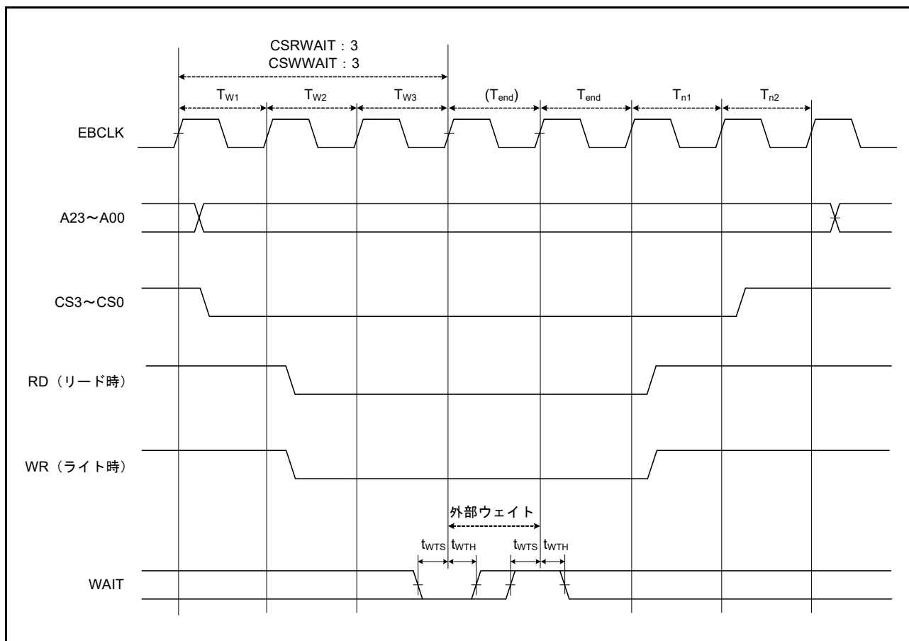
図 50.46 外部バスタイミング/外部ウェイト制御
