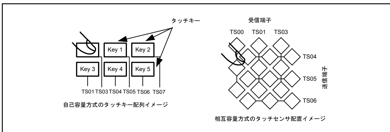
図 44.8 自己容量方式と相互容量方式の概要
