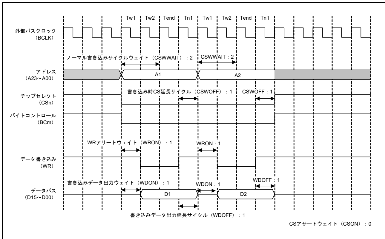
図 15.11 ノーマルライトアクセスの動作例 (1 転送要求に対して 2 回バスアクセスが発生する場合 : 1 ライトストローブモード時) (n = 0 ~ 3, m = 0, 1)
