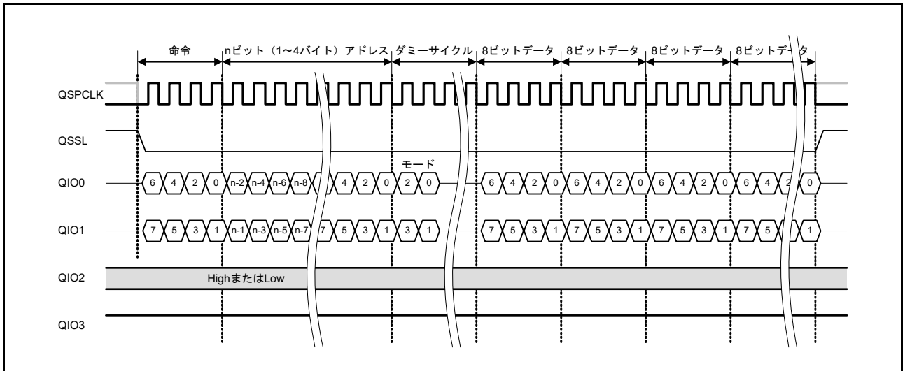
図 33.6 Dual-SPI プロトコル例 (ファストリード)
