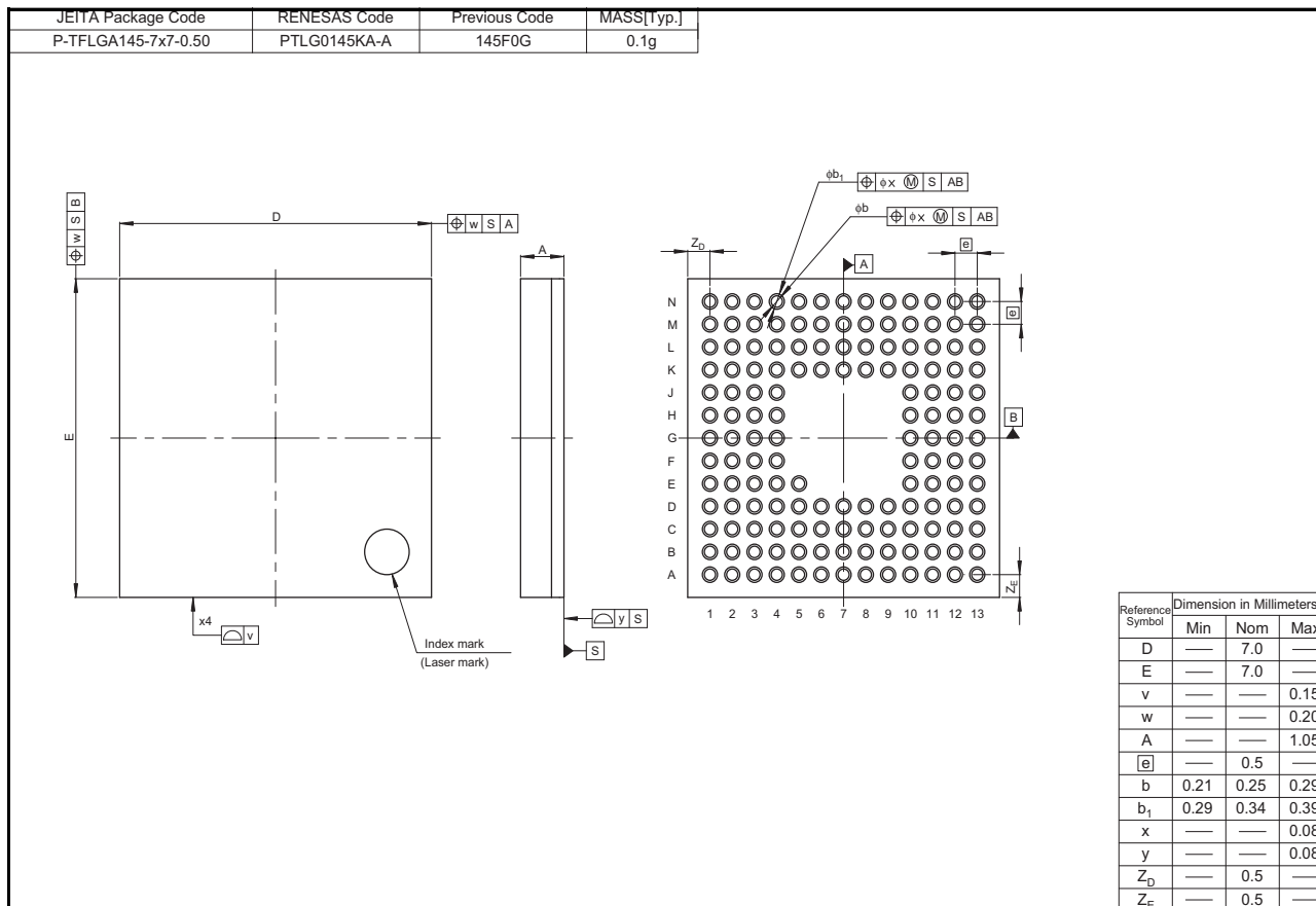
図 2.1 LGA 145 ピン
