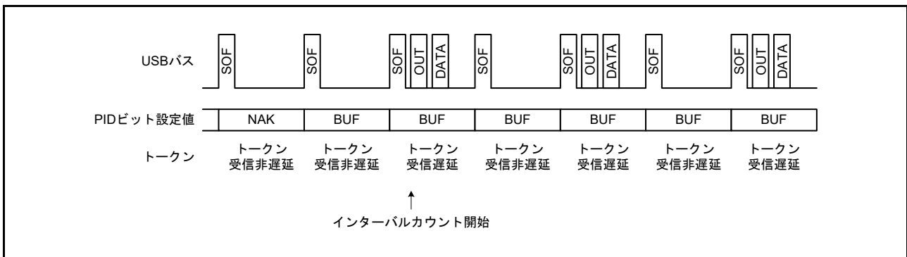
図 28.20 フレームと予想されるトークン受信の関係 (IITV[2:0] ≠ 0 の場合)
