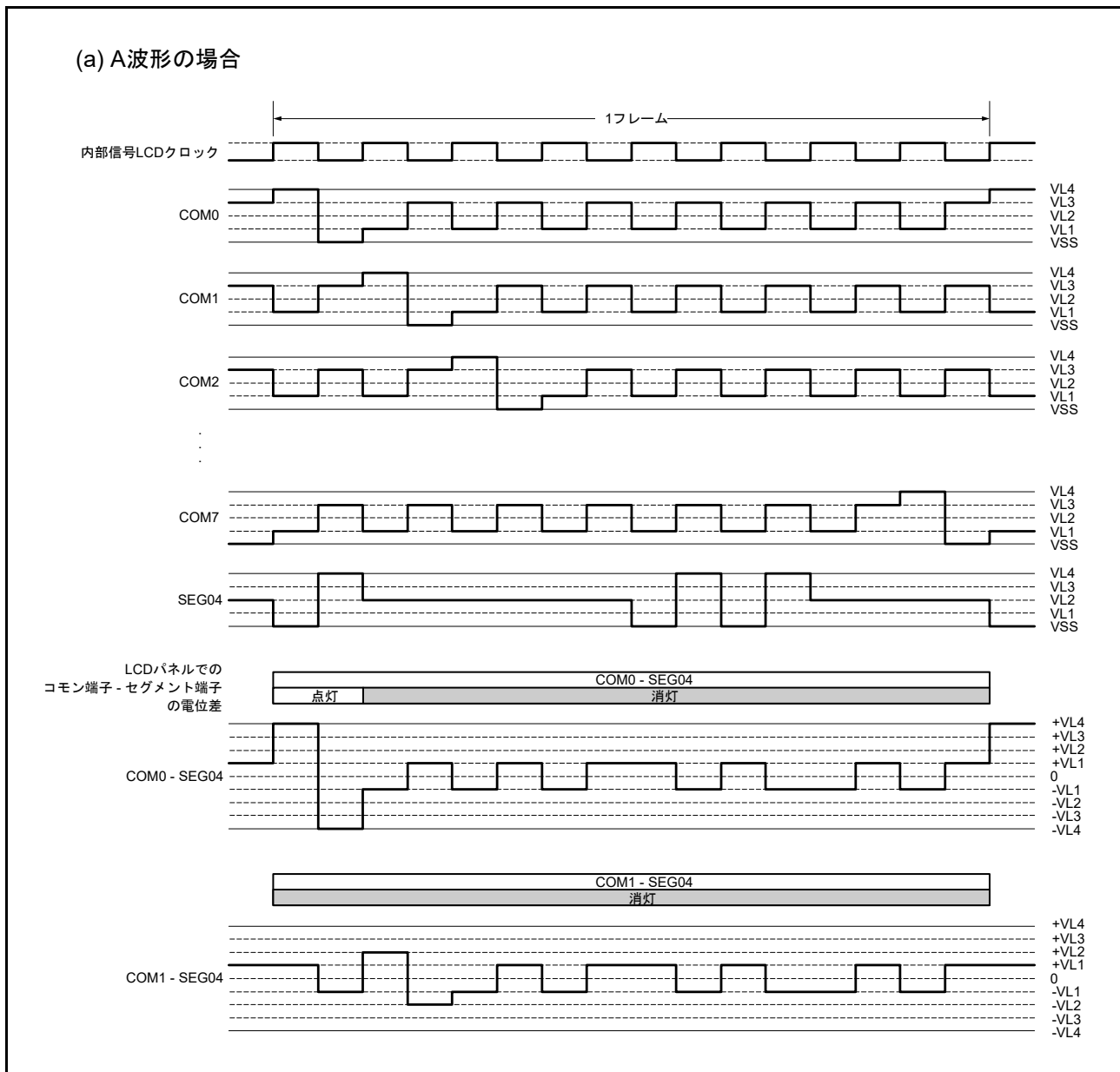
図 48.34 1/4 バイアス法を用いた SEG04 と各コモン信号との間の 8 時分割 LCD 駆動波形例 (1/2)
