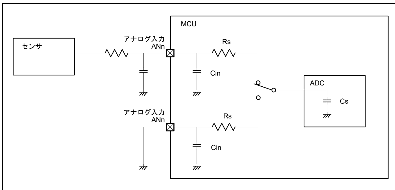
図 50.81 アナログ入力の等価回路
