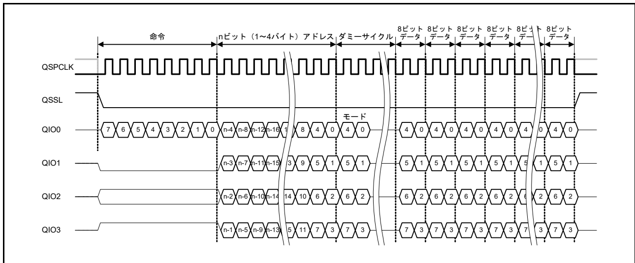
図 33.5 拡張 SPI プロトコル例 2 (ファストリード Quad I/O)
