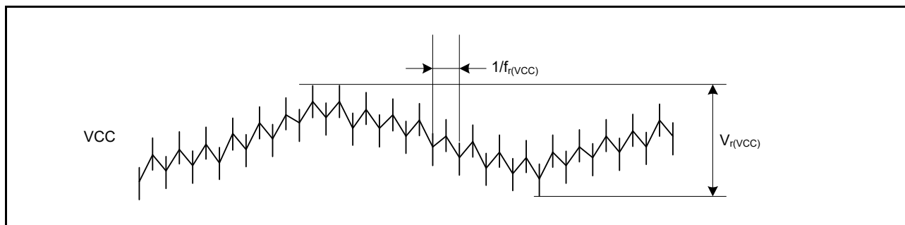
図 50.25 リップル波形
