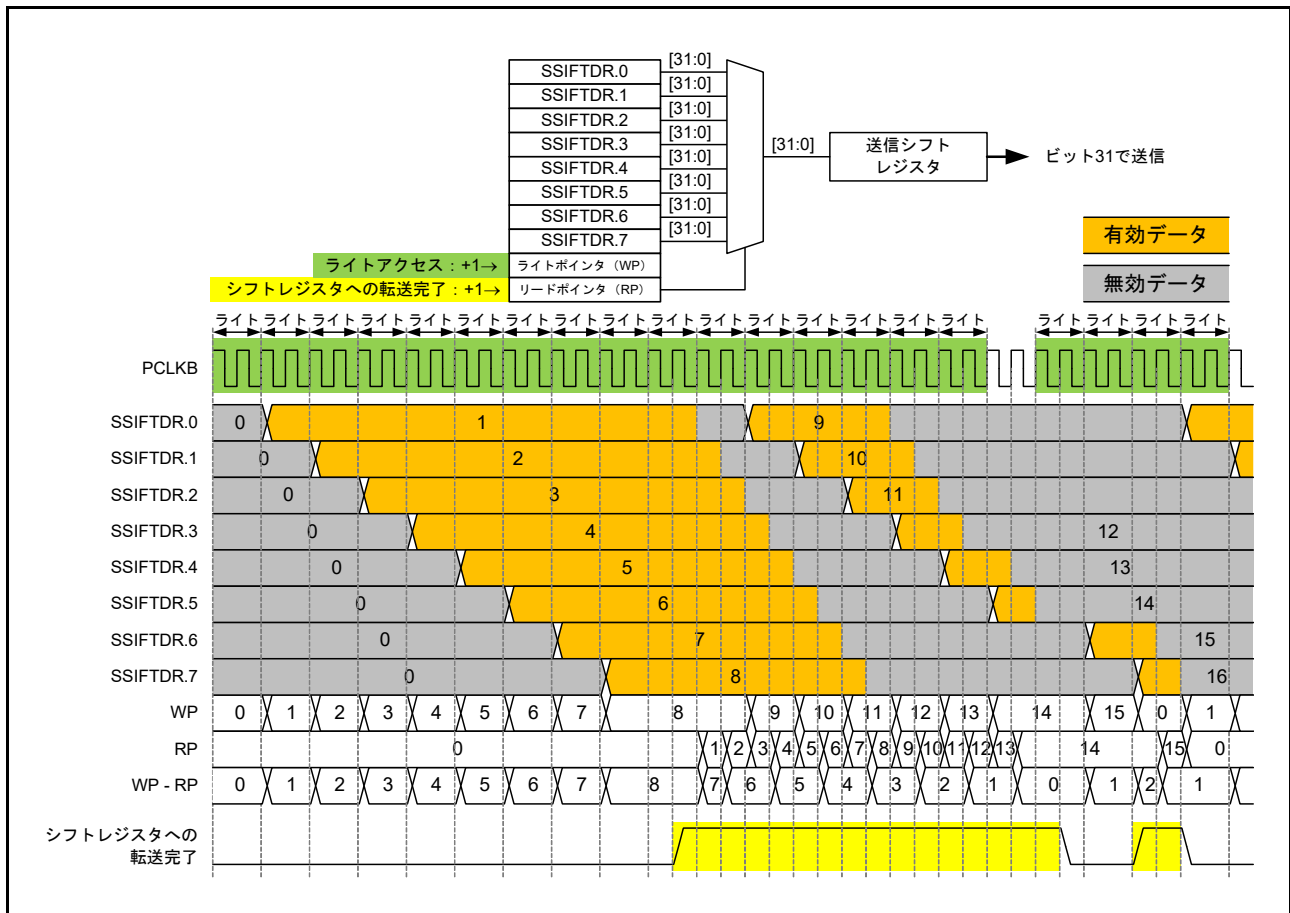
図 35.29 送信 FIFO データレジスタと送信シフトレジスタの構成例および FIFO 動作例
