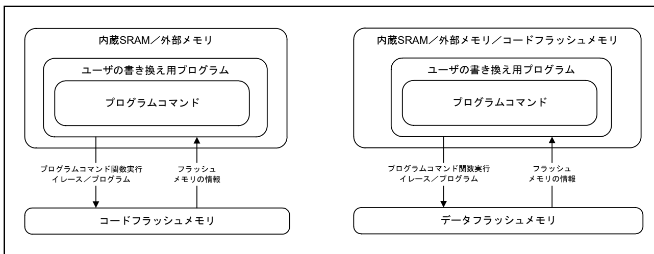
図 47.12 セルフプログラミングの概念
