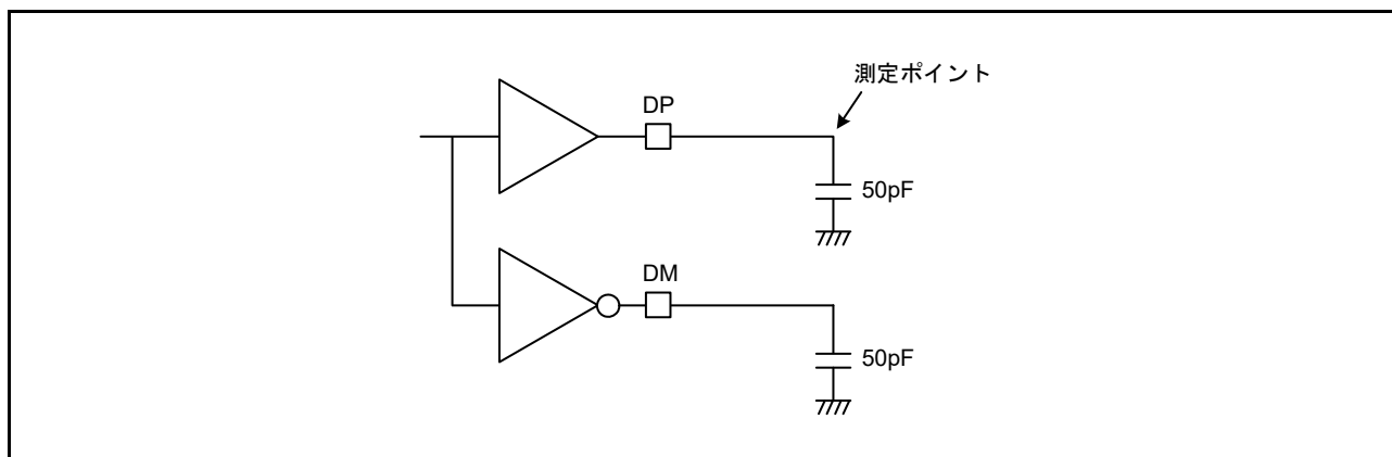
図 50.78 フルスピード (FS) 接続の測定回路
