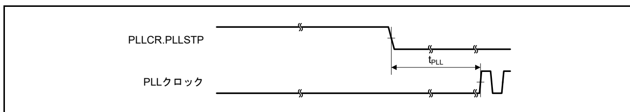
図 50.31 PLL クロック発振開始タイミング (メインクロックの発振安定後に PLL を動作させたとき)
