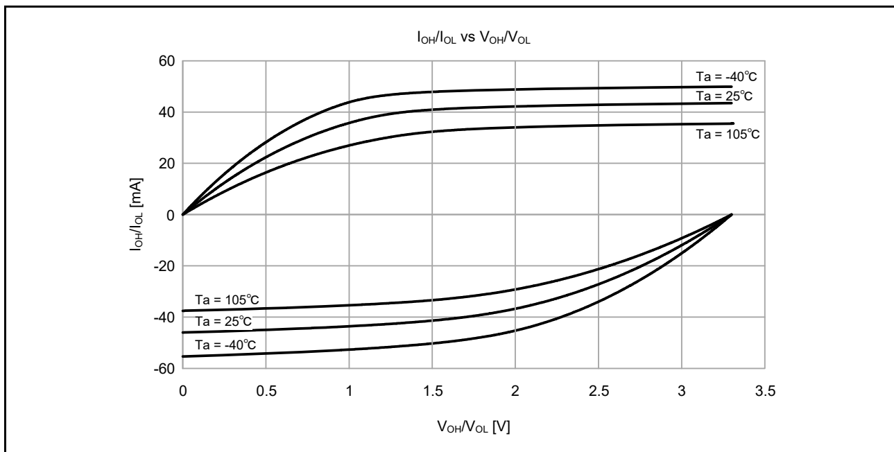
図 50.10 中駆動出力選択時の VCC = 3.3V での V_{OH}/V_{OL} および I_{OH}/I_{OL} 温度特性 (参考データ)
