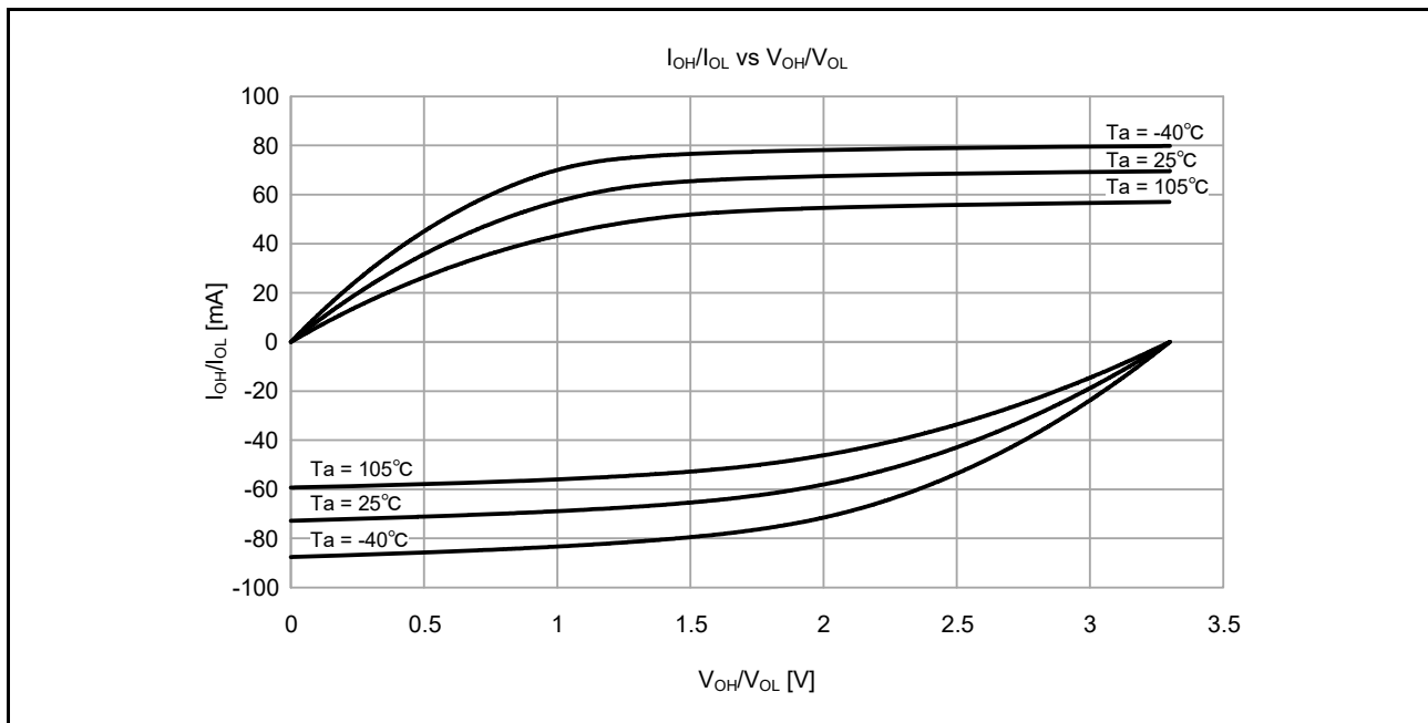
図 50.14 中駆動出力選択時の VCC = 3.3V での V_{OH}/V_{OL} および I_{OH}/I_{OL} 温度特性 (参考データ)
