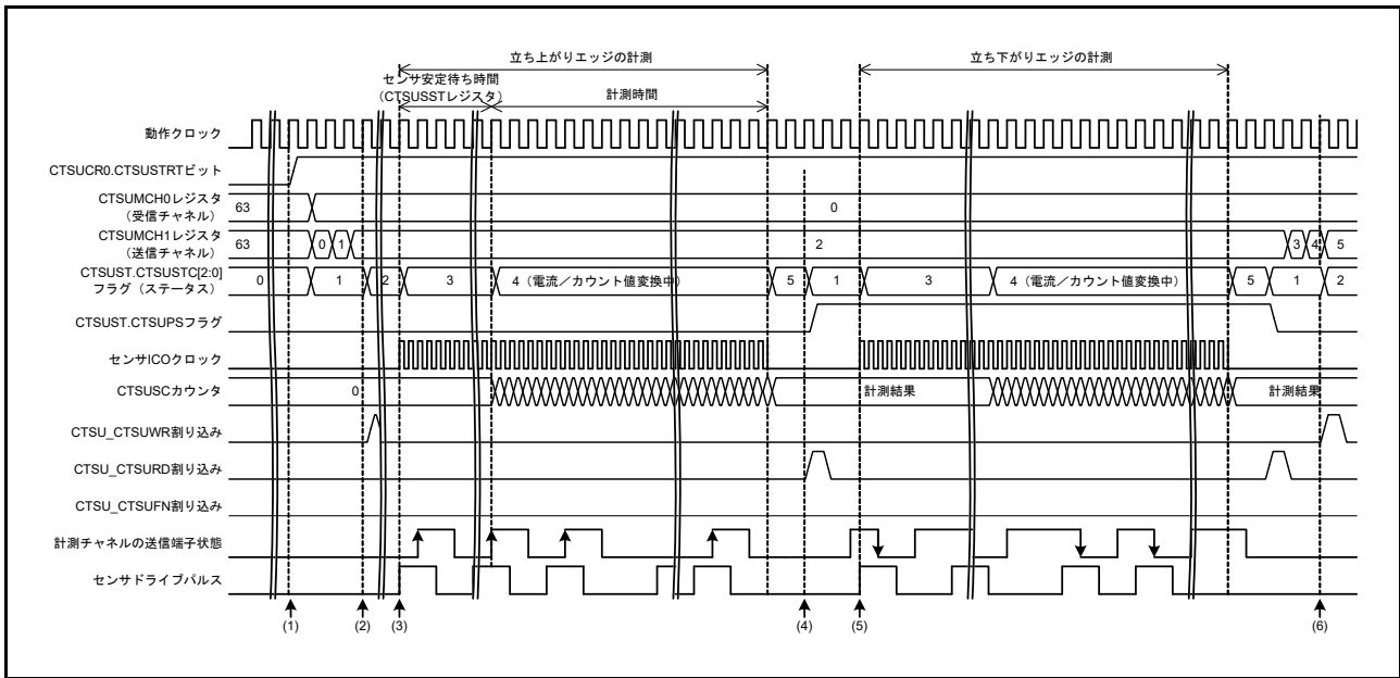
図 44.17 相互容量フルスキャンモードのタイミング (計測開始条件がソフトウェアトリガの場合)
