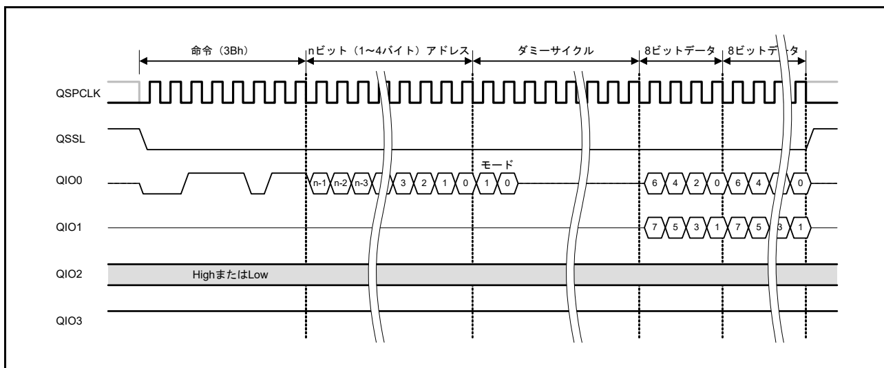
図 33.19 ファストリード Dual 出力バスサイクル
