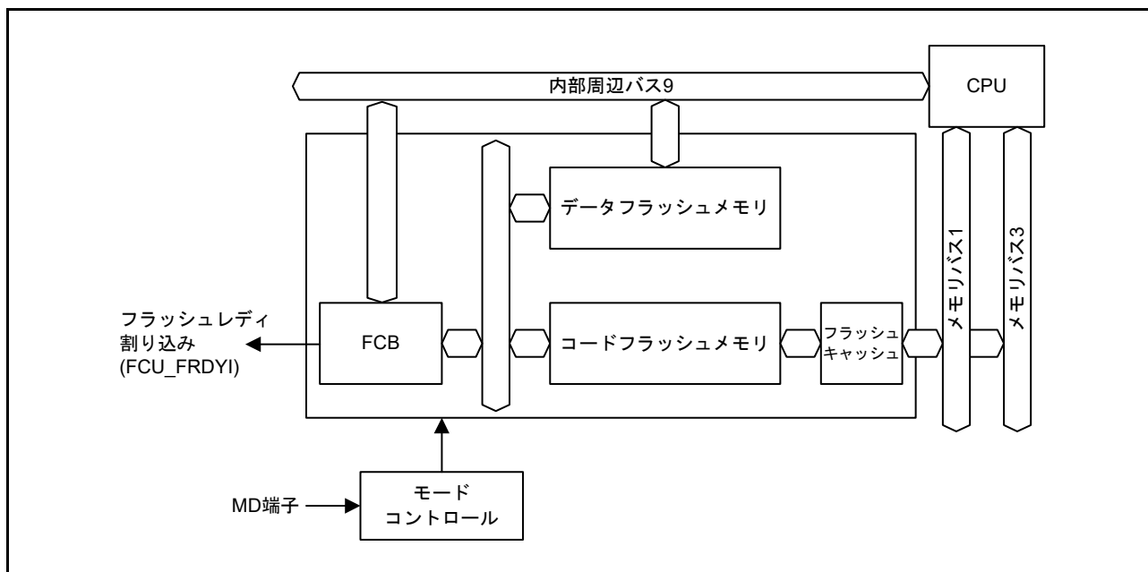
図 47.1 フラッシュメモリ関連モジュールのブロック図
