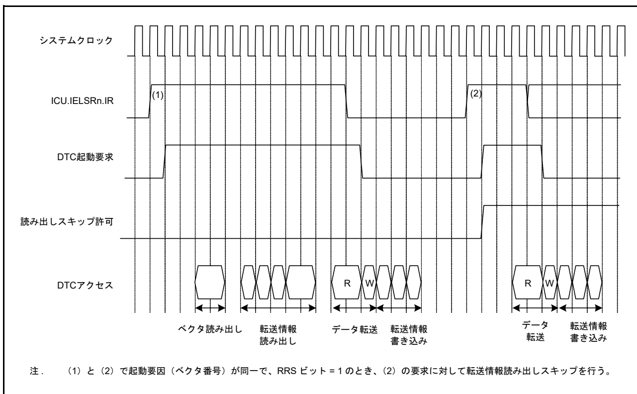
図 18.12 転送情報の読み出しスキップ時の動作例 (ベクタ、転送情報、転送先データが SRAM にあり、転送元データが周辺モジュールにある場合)
