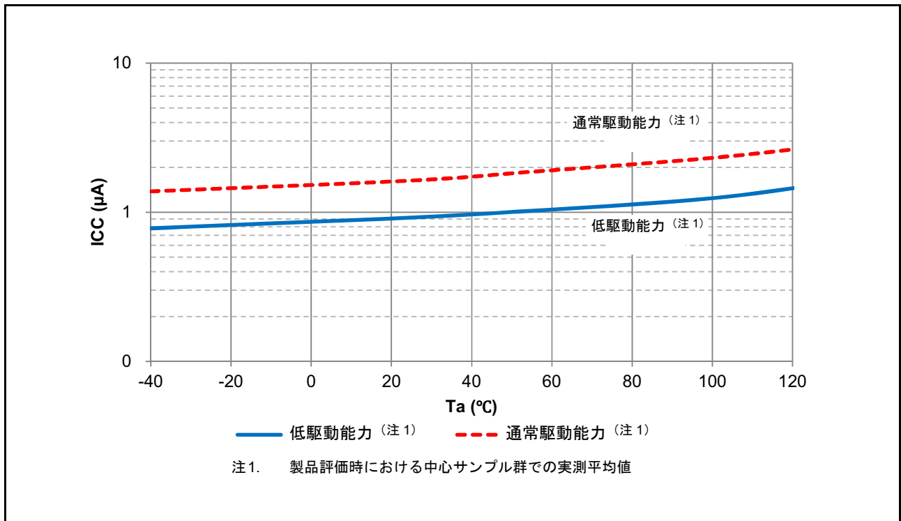
図 50.24 VCC オフ時の RTC 動作の温度依存性 (参考データ)
