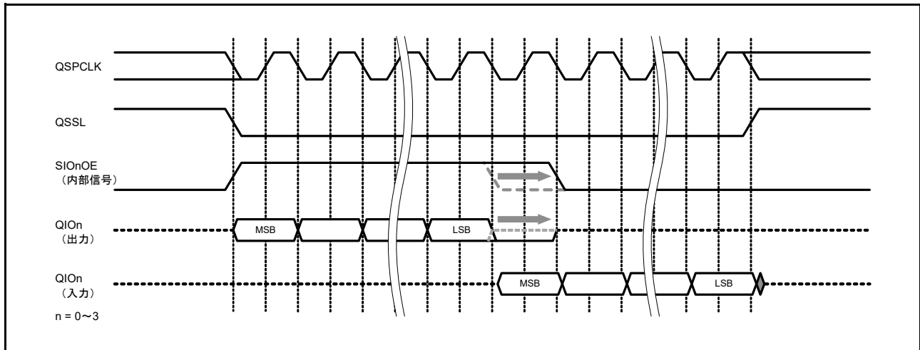
図 33.12 SFMOEX ビットを使用した出力許可ホールド時間調整
