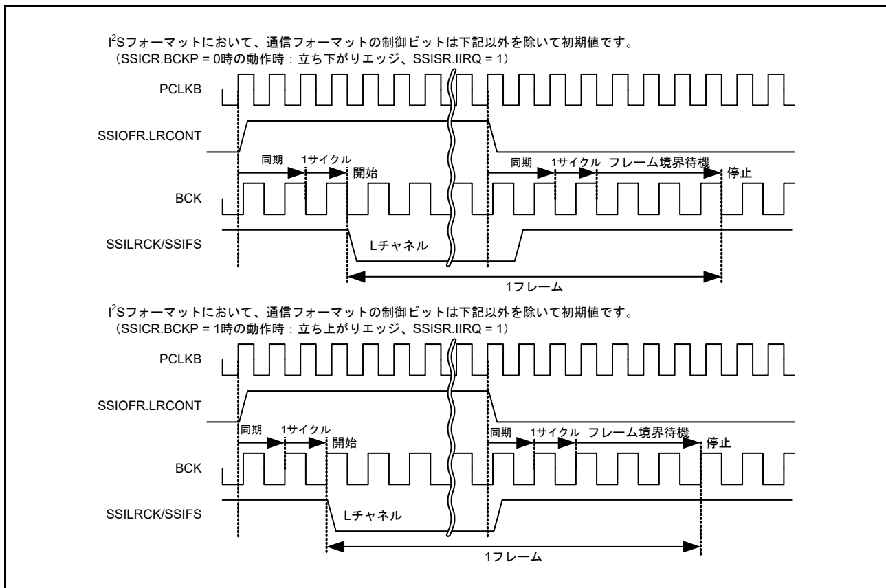
図 35.40 SSIOFR.LRCONT ビットによる LR クロック/フレーム同期継続の禁止例
