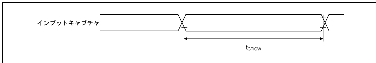
図 50.49 GPT インプットキャプチャタイミング
