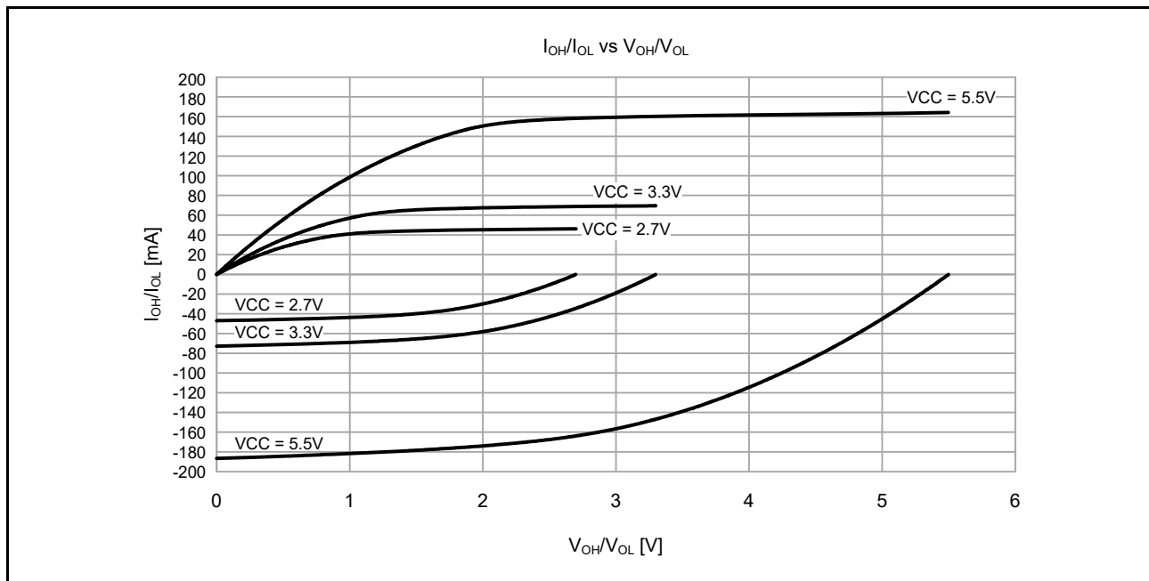
図 50.12 中駆動出力選択時の Ta = 25 °Cでの V OH /V OL および I OH /I OL 電圧特性 (参考データ)
