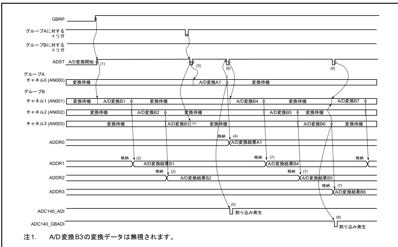
図 38.20 グループ A 優先制御の動作例 (5) (ADGSPCR.GBRP = 1 の場合)
