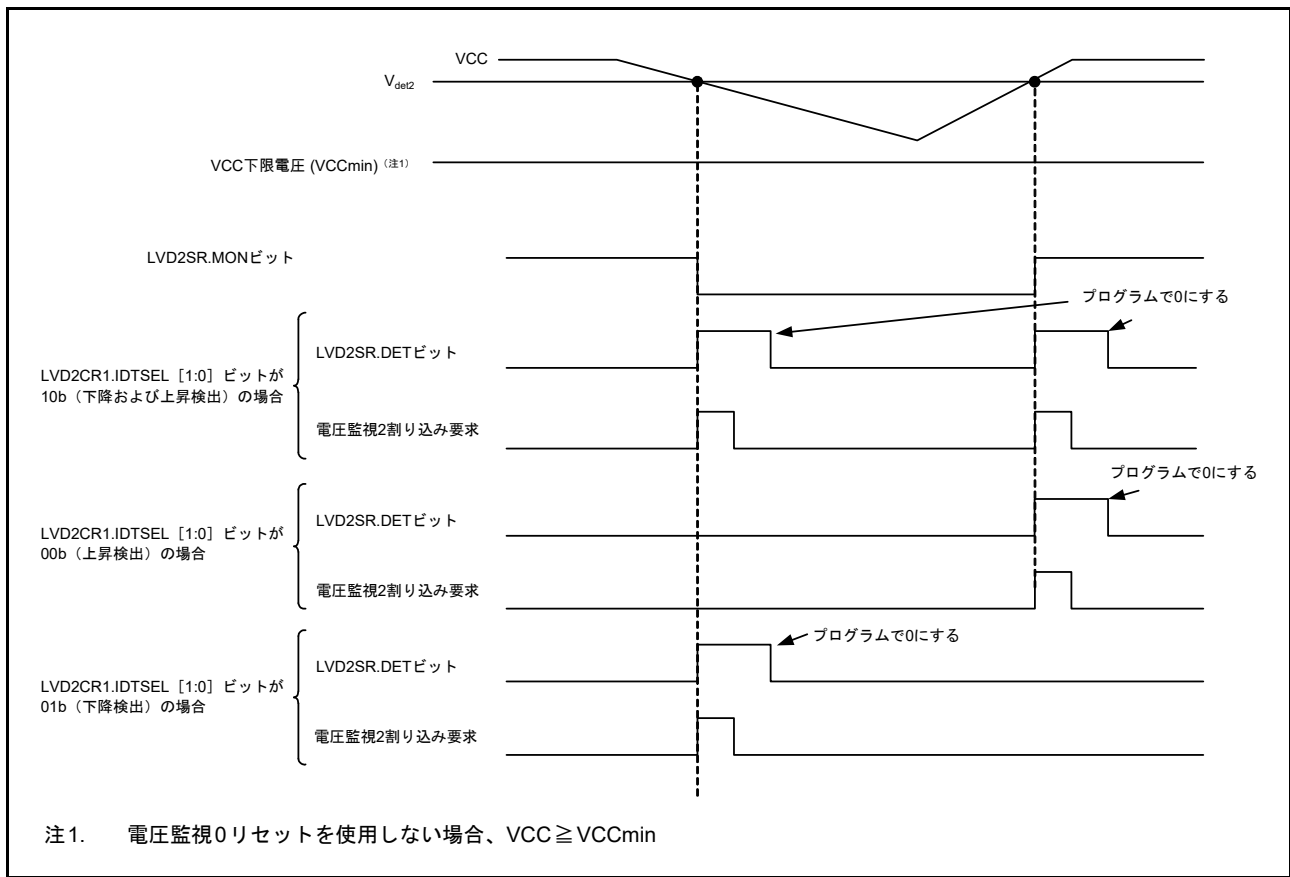
図 8.6 電圧監視 2 割り込みの動作例
