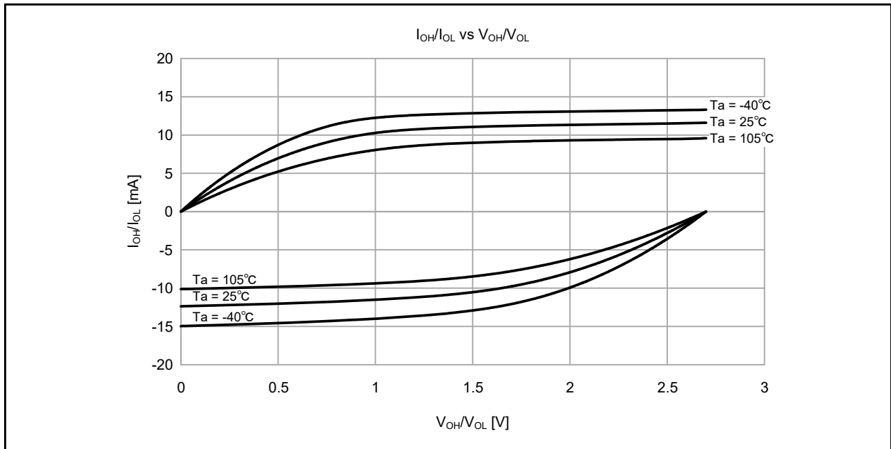
図 50.4 低駆動出力選択時の VCC = 2.7V での V_{OH}/V_{OL} および I_{OH}/I_{OL} 温度特性 (参考データ)
