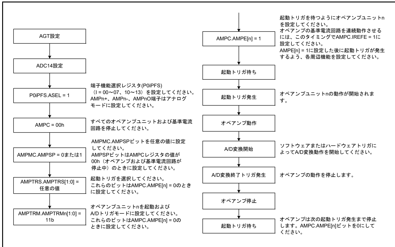
図 41.9 起動トリガによるオペアンプ起動と A/D 変換終了トリガによるオペアンプ停止手順
