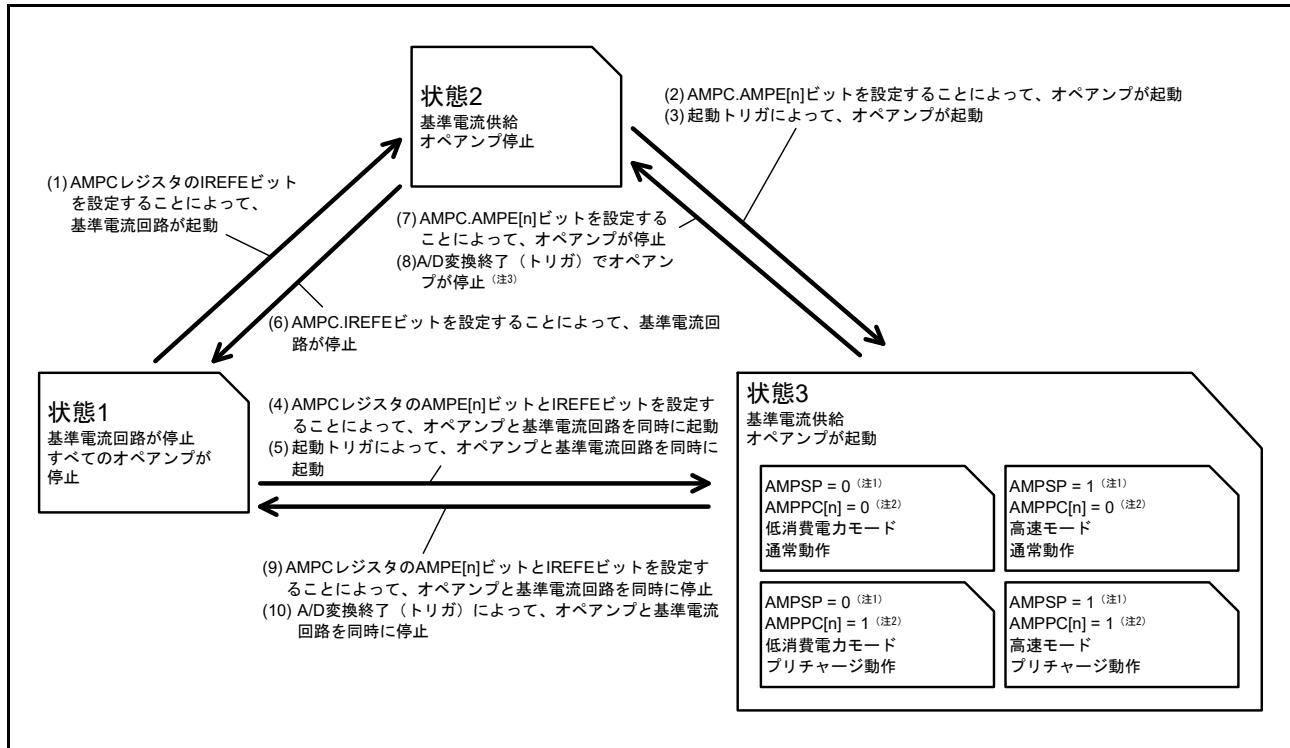
図 41.2 オペアンプの状態遷移
