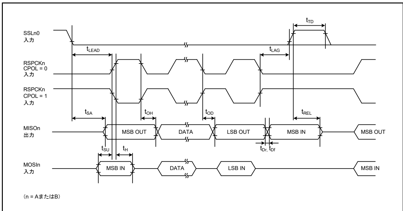
図 50.66 SPI タイミング (スレーブ、CPHA = 0)
