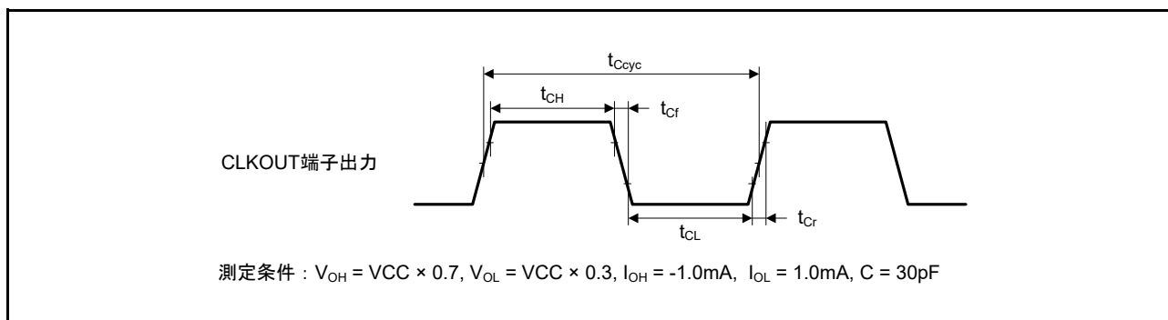
図 50.76 CLKOUT 出力タイミング
