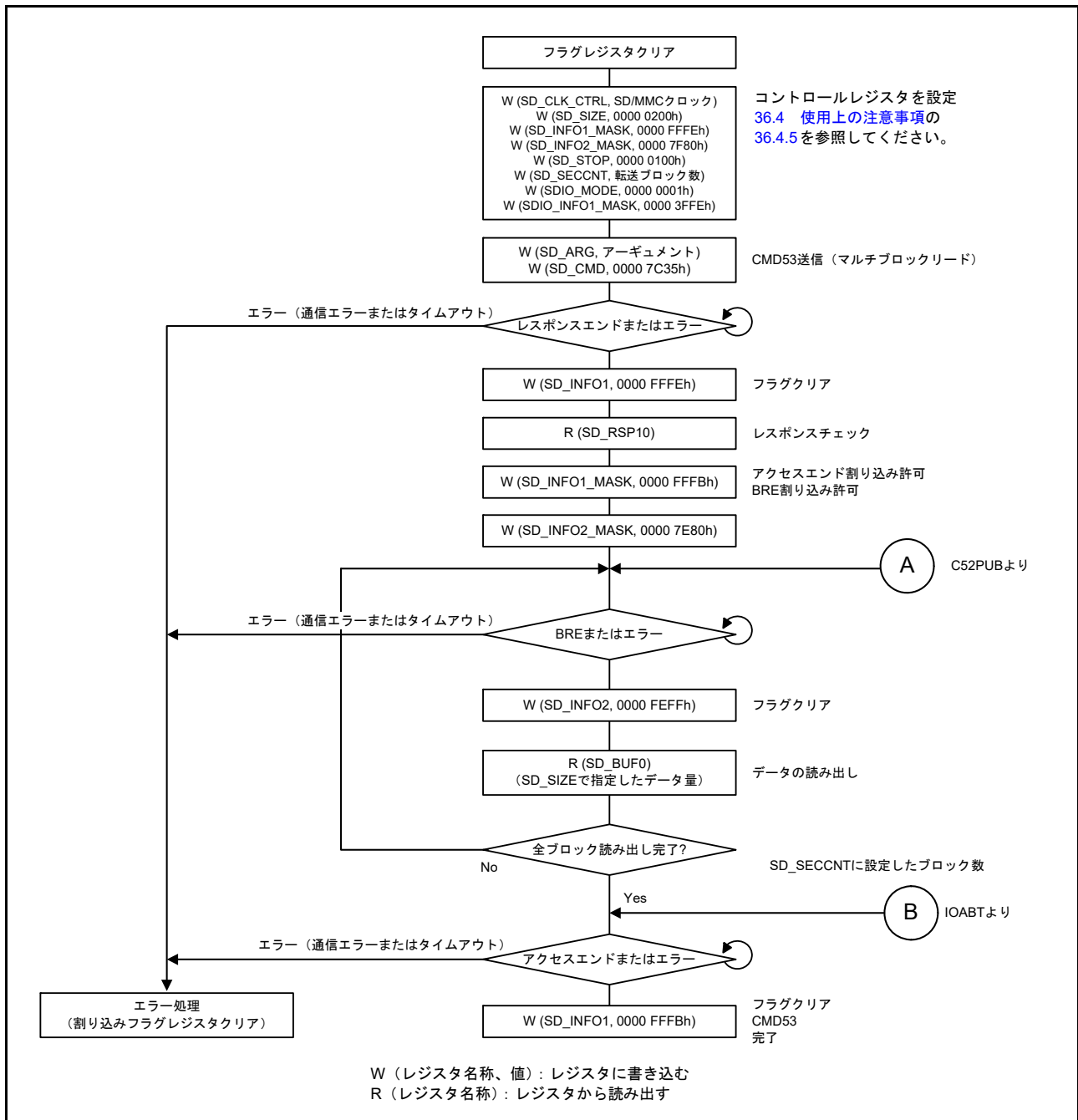
図 36.17 マルチブロックリード動作の IO_RW_EXTENDED コマンド (CMD53) の例
