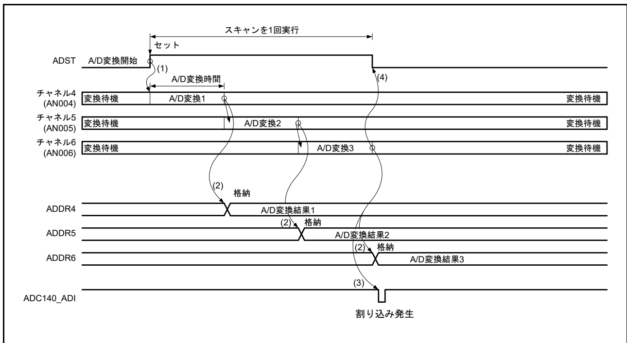
図 38.6 シングルスキャンモードの基本動作例 (AN004 ~ AN006 選択)
