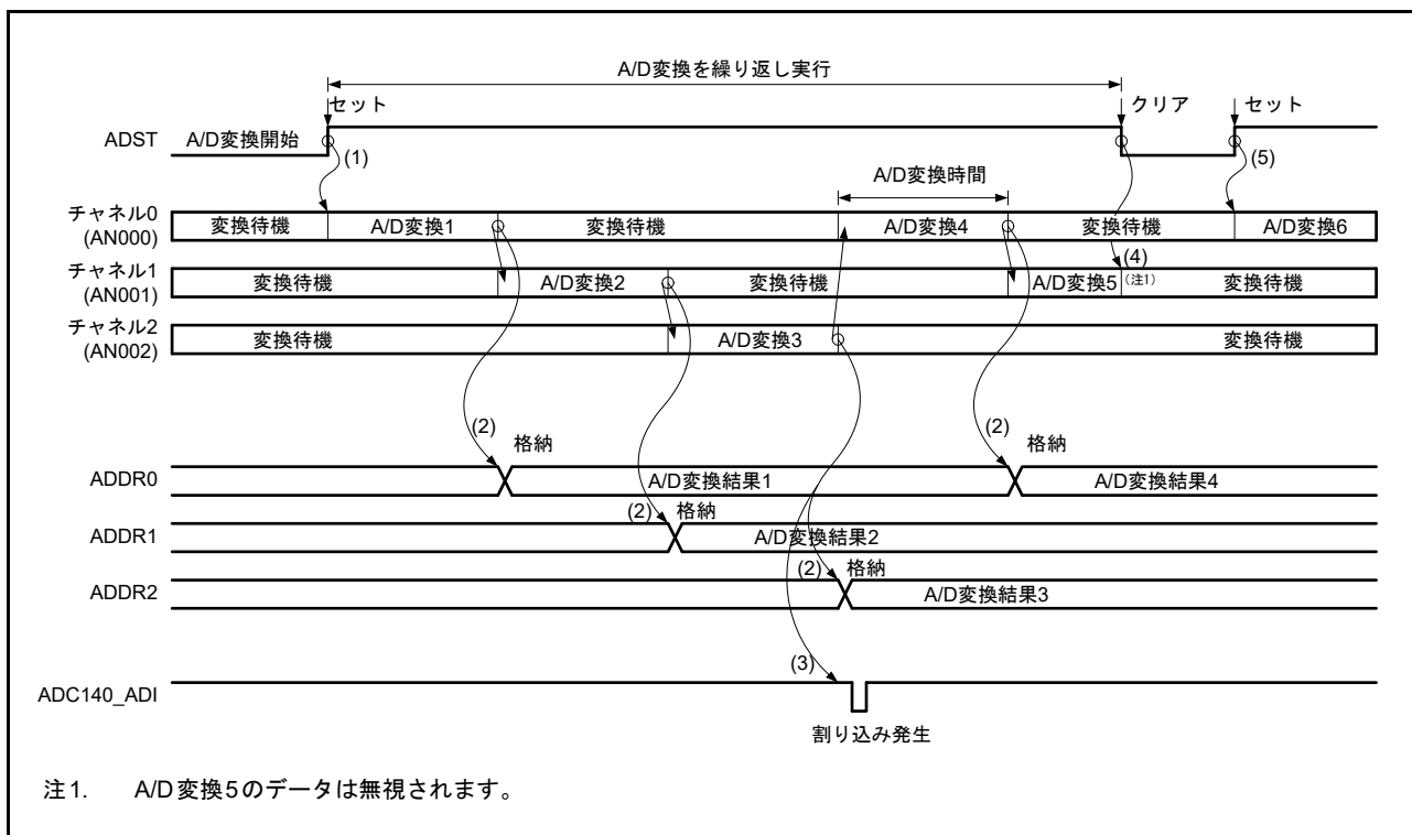
図 38.11 連続スキャンモードの基本動作例 (AN000 ~ AN002 選択)
