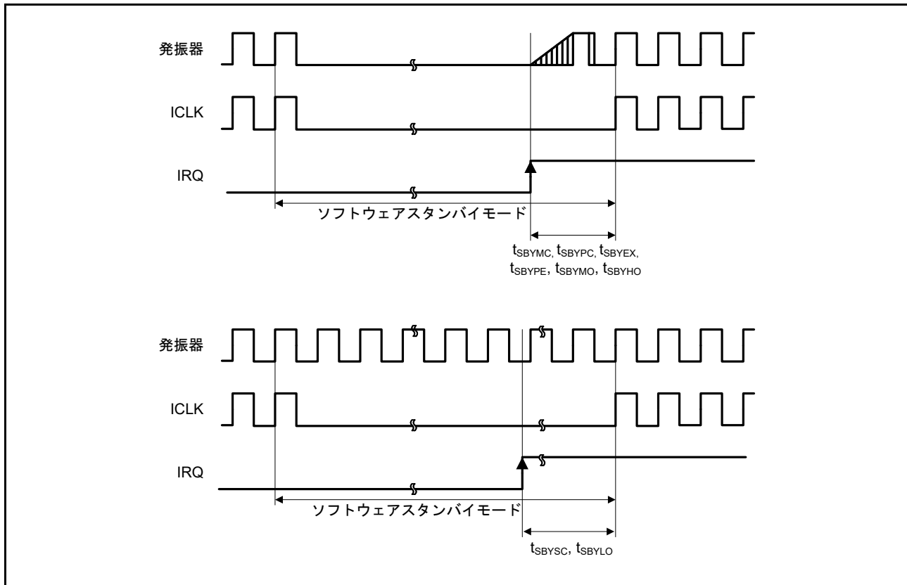
図 50.36 ソフトウェアスタンバイモード解除タイミング
