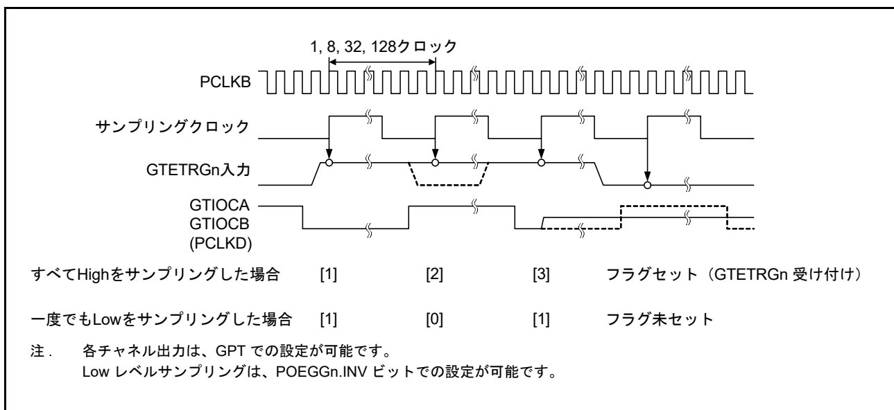
図 22.2 デジタルフィルタの動作例
