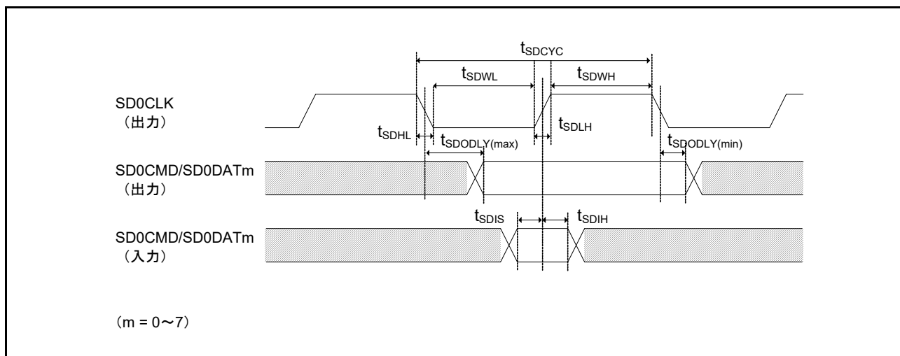
図 50.75 SD/MMC ホストインタフェース信号タイミング
