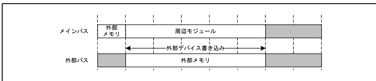
図 15.37 ライトバッファ機能使用時の動作例
