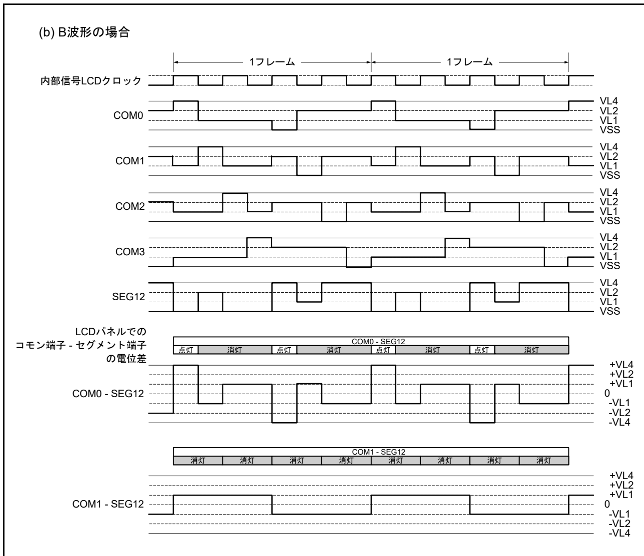
図 48.31 1/3 バイアス法を用いた SEG12 と各コモン信号との間の 4 時分割 LCD 駆動波形例 (2/2)
