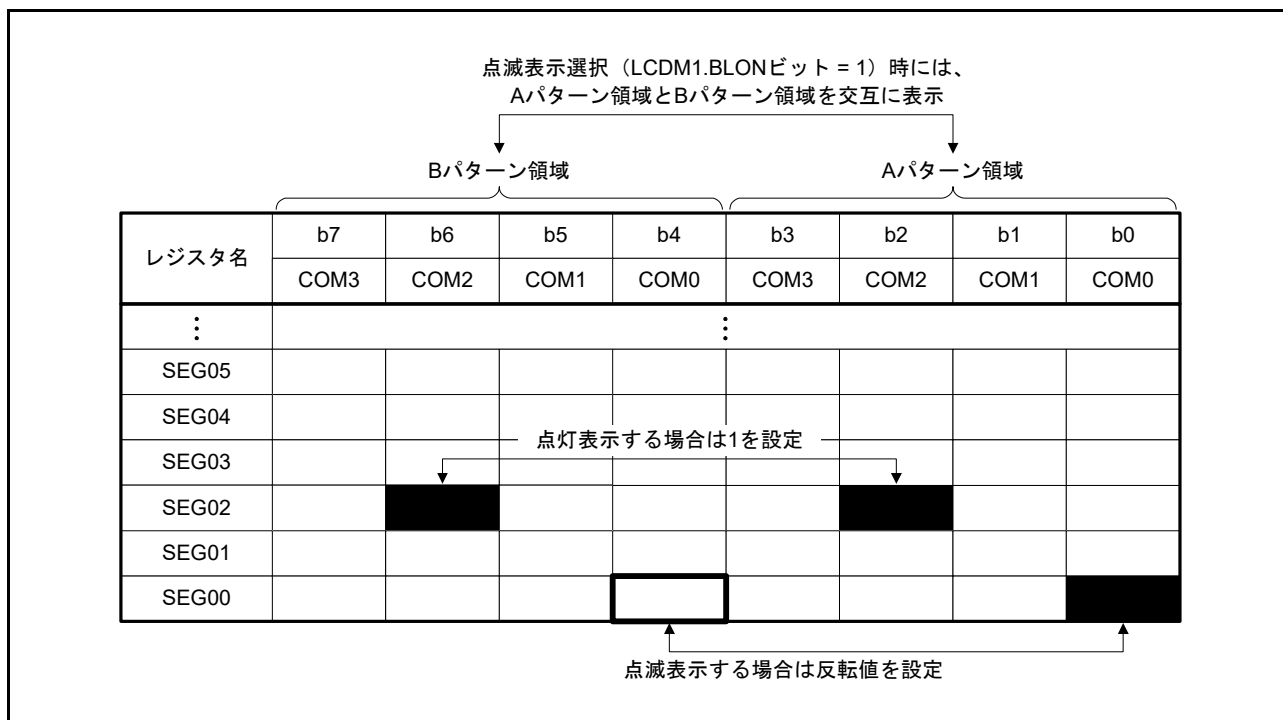
図 48.2 パターン切り替え時の LCD 表示データレジスタの設定例
