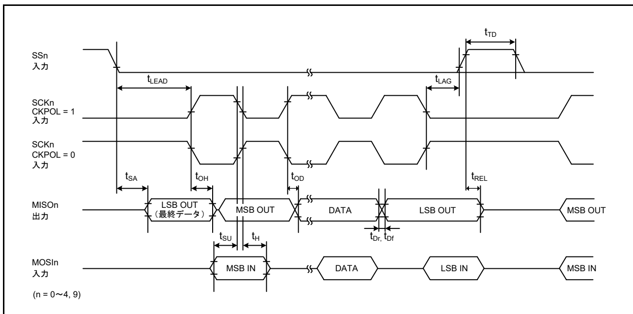
図 50.59 SCI 簡易 SPI モードタイミング (スレーブ、CKPH = 0)
