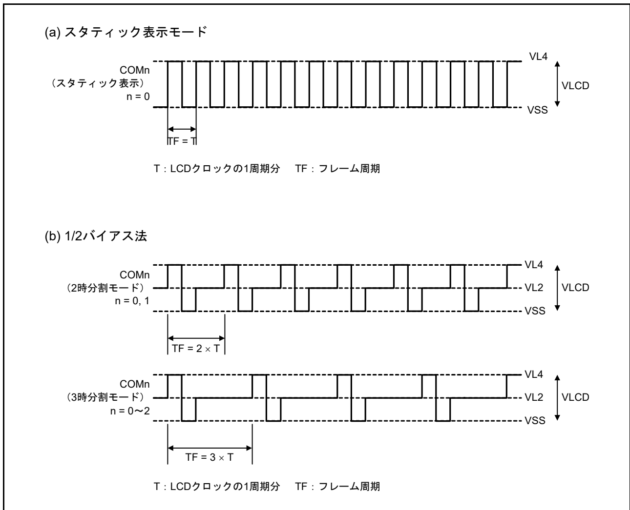
図 48.13 コモン信号波形 (1/2)
