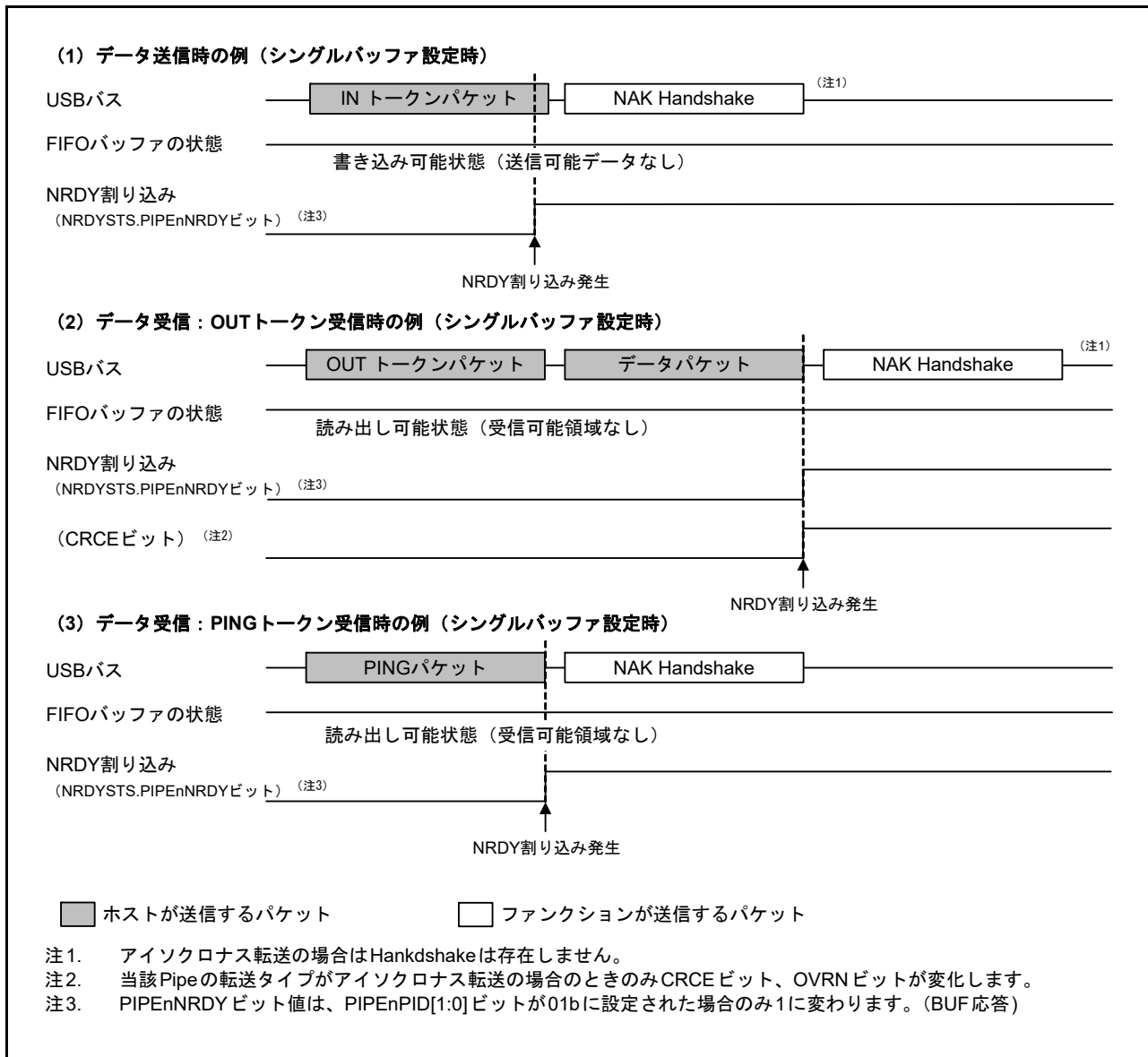
図 28.13 デバイスコントローラモードにおける NRDY 割り込みの発生タイミング
