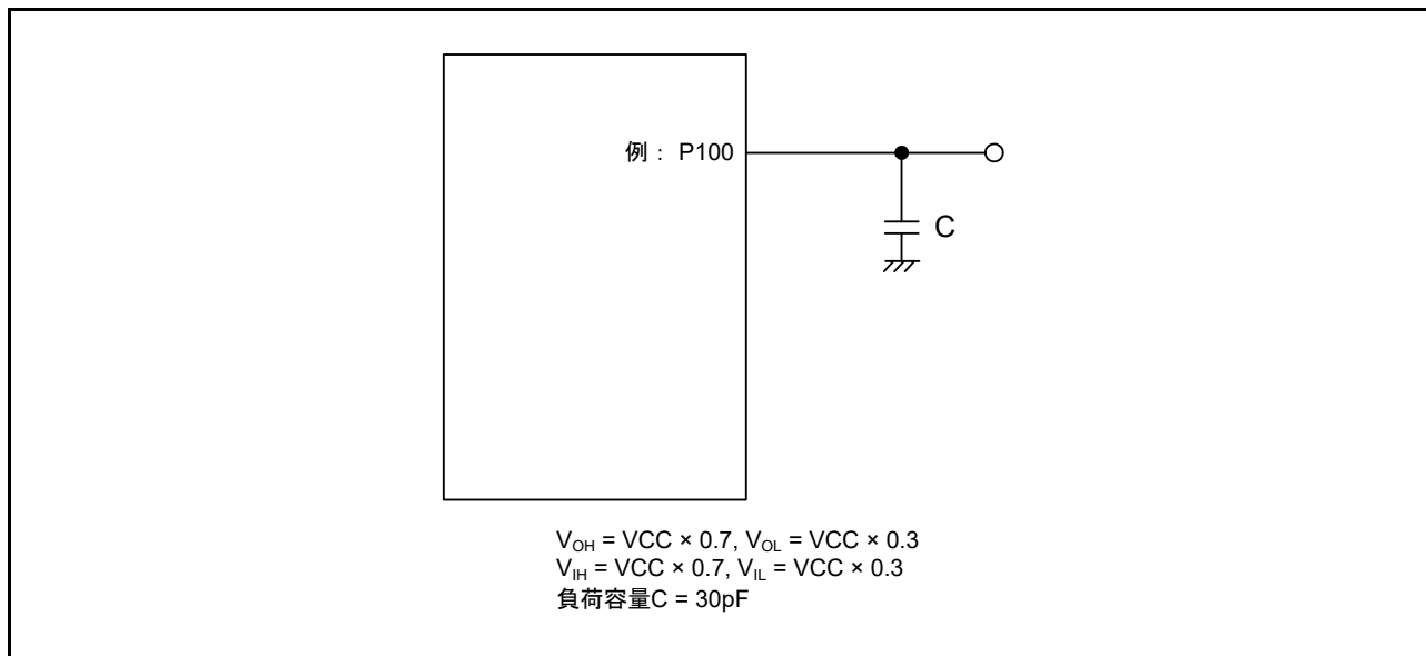
図 50.1 入出力タイミング計測条件
