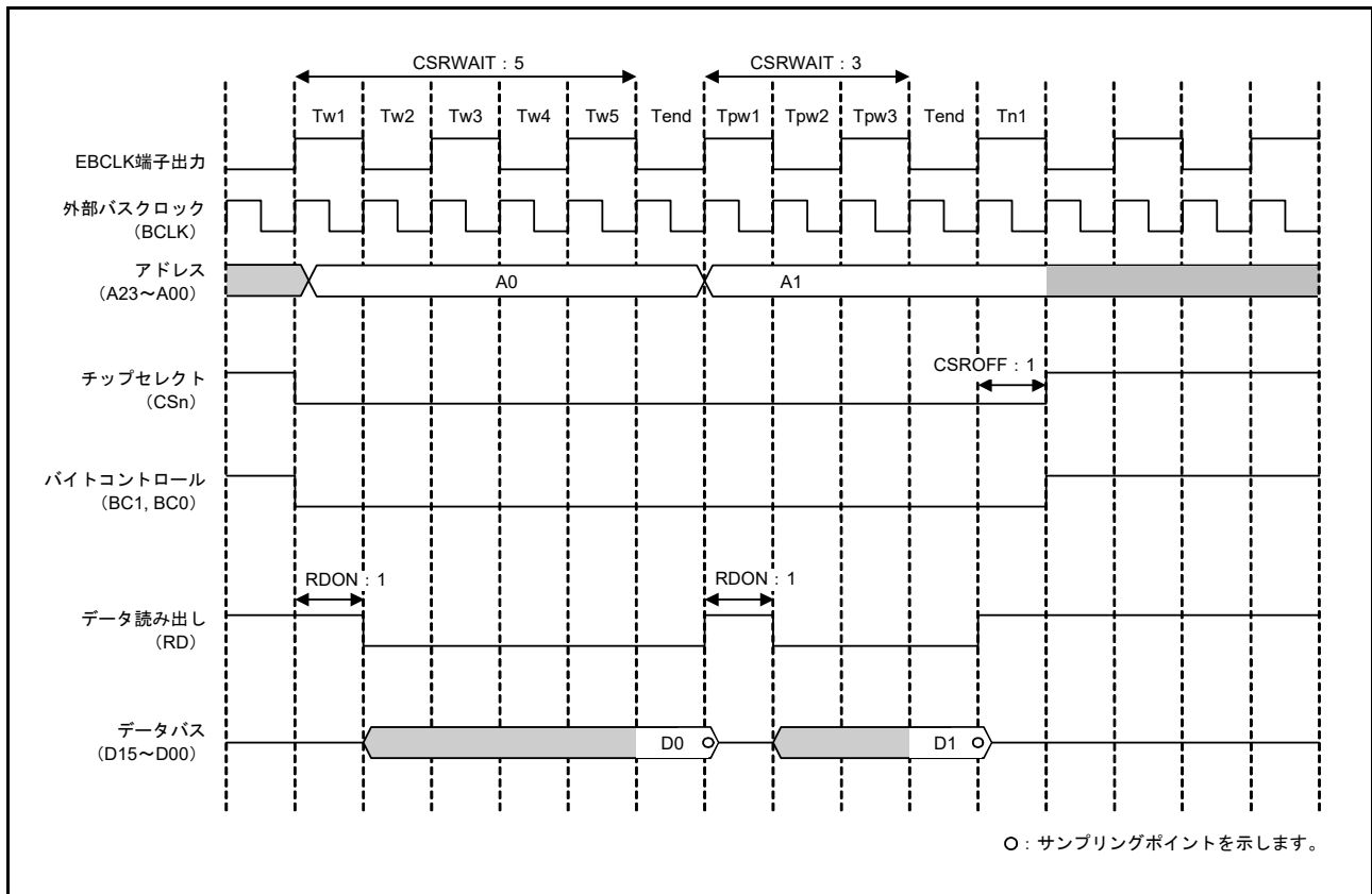
図 15.21 ページリードアクセスの動作例 (EBCLK 端子出力選択ビットで BCLK の 2 分周を選択した場合、および 1 転送要求に対して 2 回バスアクセスが発生する場合) (n = 0 ~ 3)
