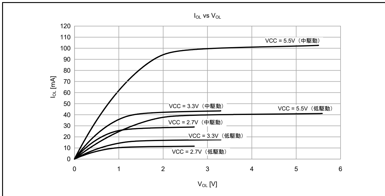
図 50.16 Ta = 25 °Cでの V OH /V OL および I OH /I OL 電圧特性
