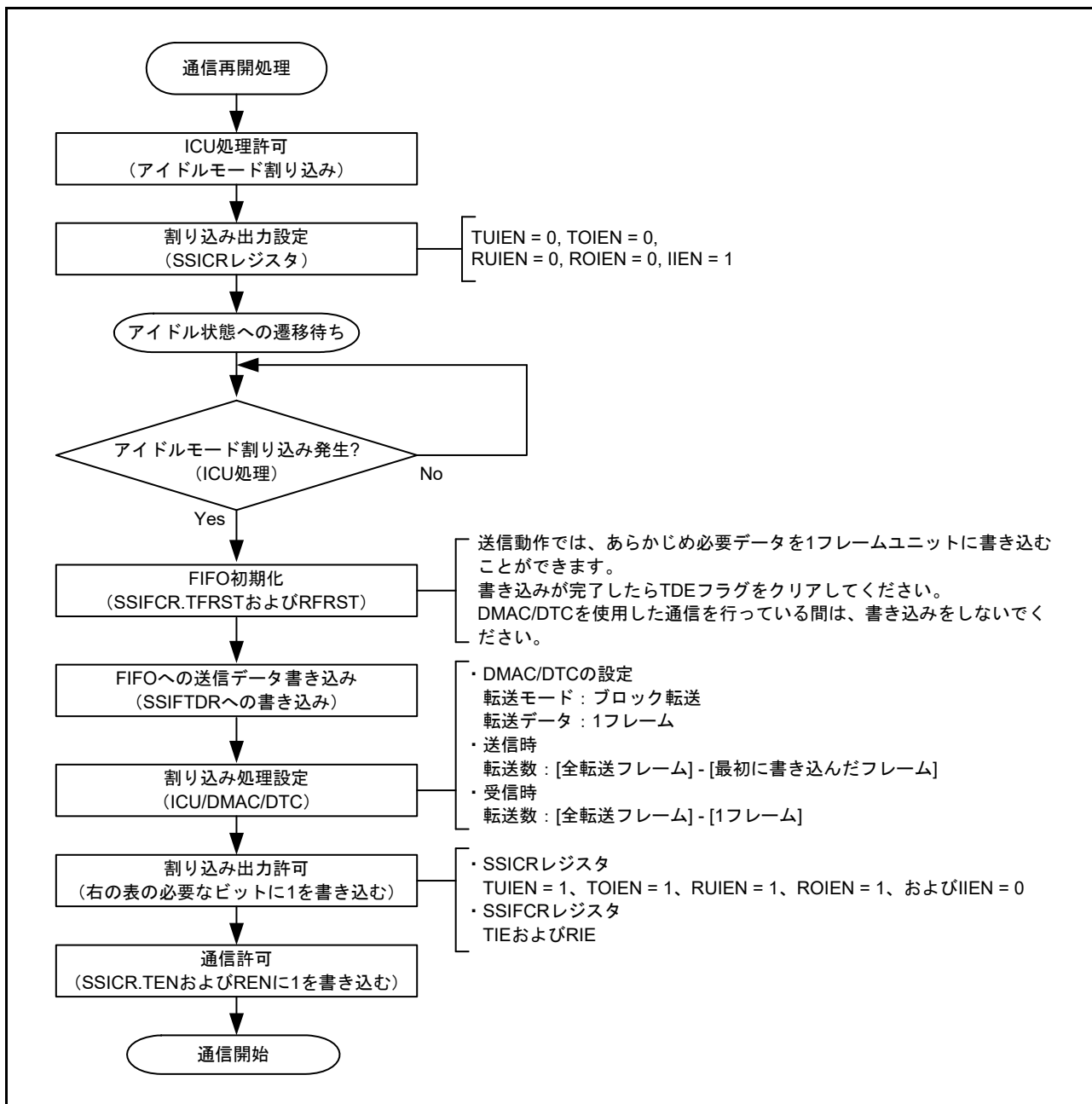
図 35.54 通信再開手順 (CPU 動作)
