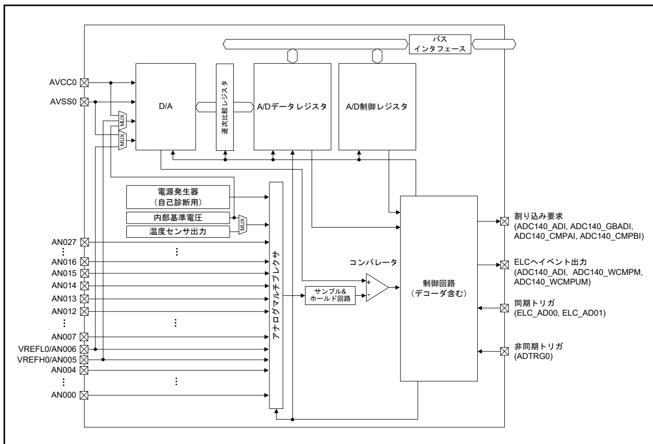
図 38.1 ADC14 のブロック図
