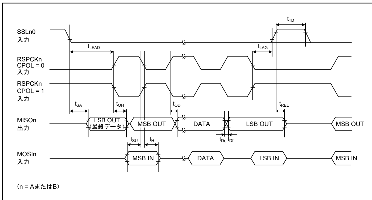
図 50.67 SPI タイミング (スレーブ、CPHA = 1)
