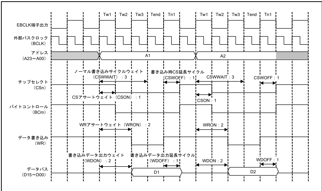
図 15.14 ノーマルライトアクセスの動作例 (EBCLK 端子出力選択ビットで BCLK の 2 分周を選択した場合) ( n = 0 \sim 3, m = 0, 1 )
