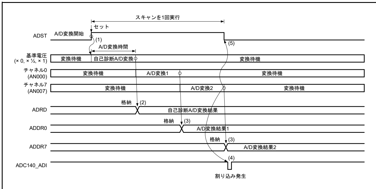
図 38.7 シングルスキャンモードの基本動作例 (AN000、AN007 選択 + 自己診断)
