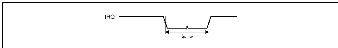
図 50.39 IRQ 割り込み入力タイミング
