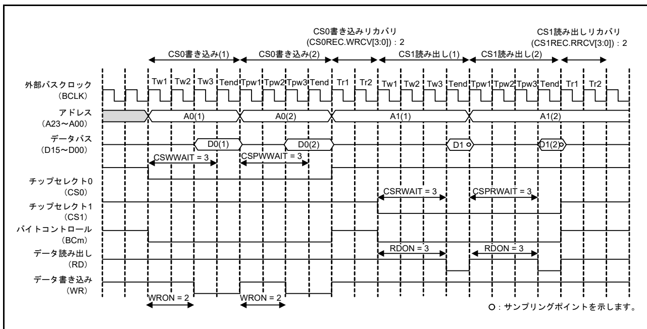
図 15.33 セパレートバスインタフェース時のページアクセスで、バスアクセスが分割された場合のリカバリサイクルの挿入例 (m = 0, 1)
