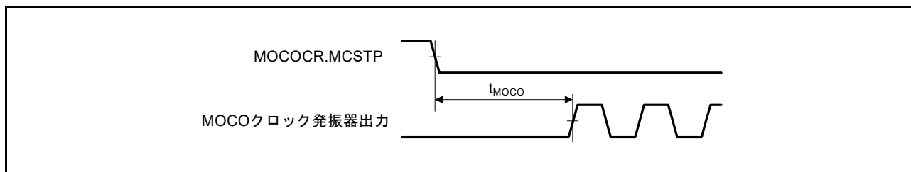
図 50.33 MOCO クロック発振開始タイミング
