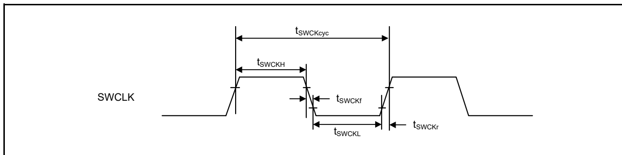
図 50.99 SWD SWCLK タイミング
