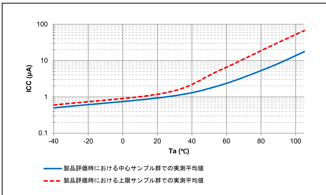
図 50.23 すべての SRAM がオンのソフトウェアスタンバイモード時の温度依存性 (参考データ)
