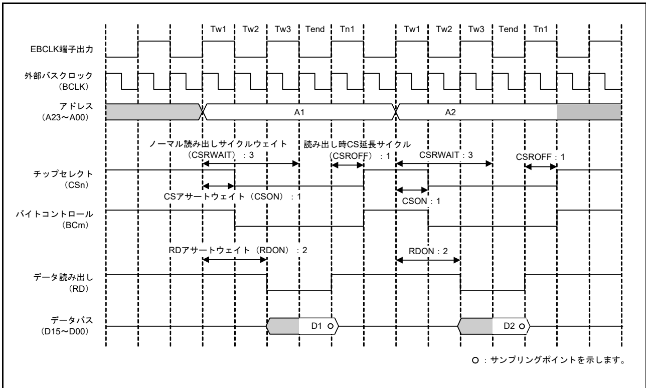
図 15.13 ノーマルリードアクセスの動作例 (EBCLK 端子出力選択ビットで BCLK の 2 分周を選択した場合) ( n = 0 \sim 3, m = 0, 1 )
