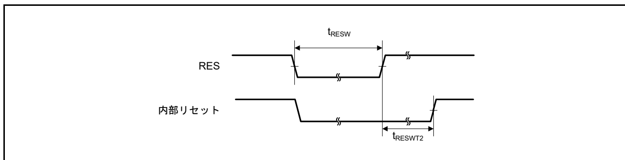
図 50.35 リセット入力タイミング (1)
