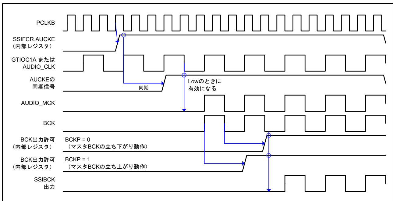
図 35.24 システムリセットからマスタモード通信開始までの動作のタイミング図
