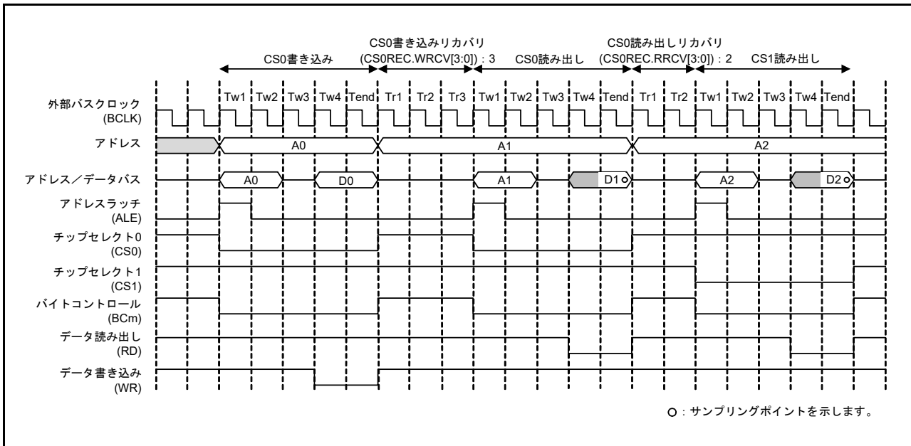
図 15.35 アドレス/データマルチプレクス I/O インタフェース時のリカバリサイクルの挿入例 (m = 0, 1)
