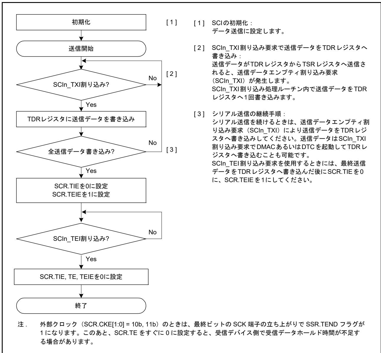
図 29.37 クロック同期式モードにおけるシリアル送信のフローチャート例 (非 FIFO 選択時)
