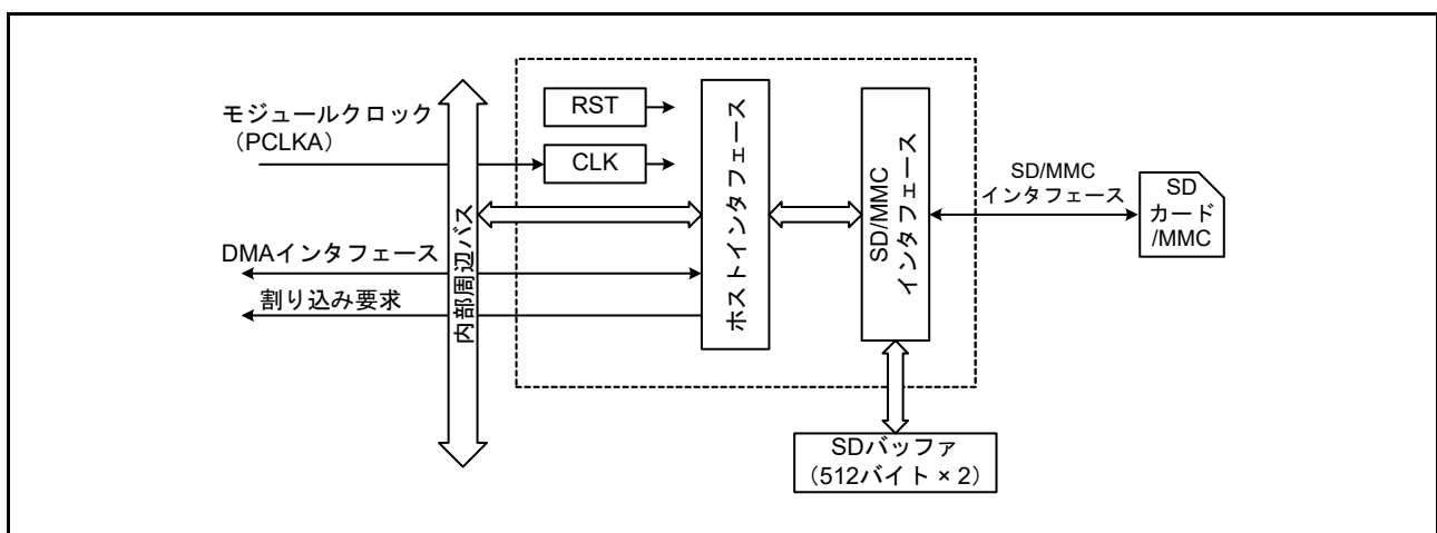
図 36.1 SD/MMCホストインタフェースのブロック図
