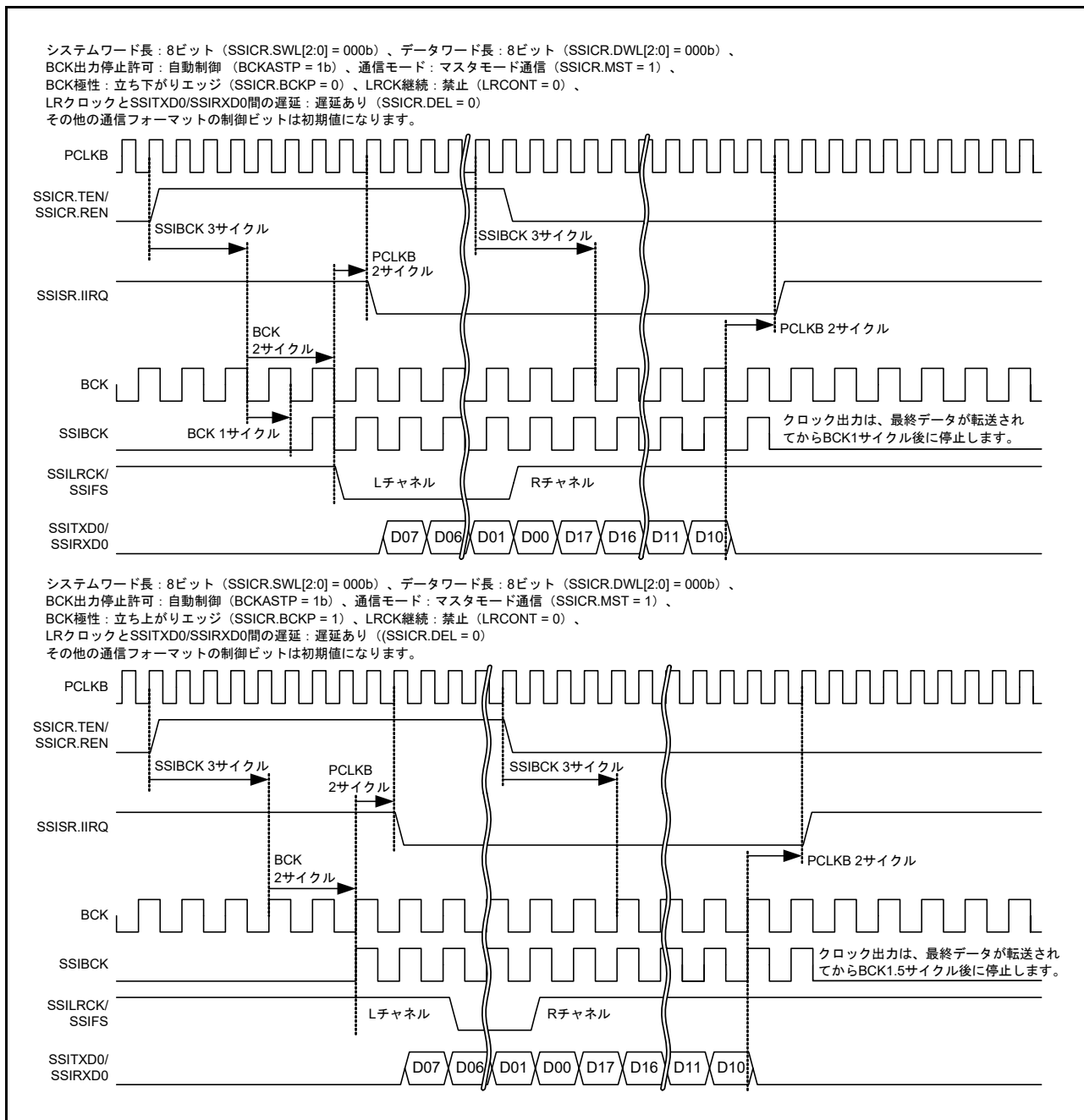
図 35.33 BCKASTP ビットの動作例 (BCKASTP = 1 での通信の場合)
