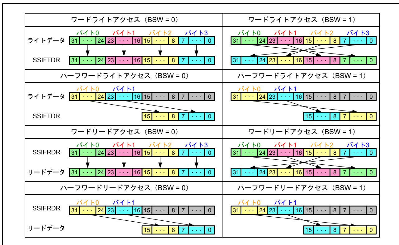
図 35.22 バイトスワップの動作例
