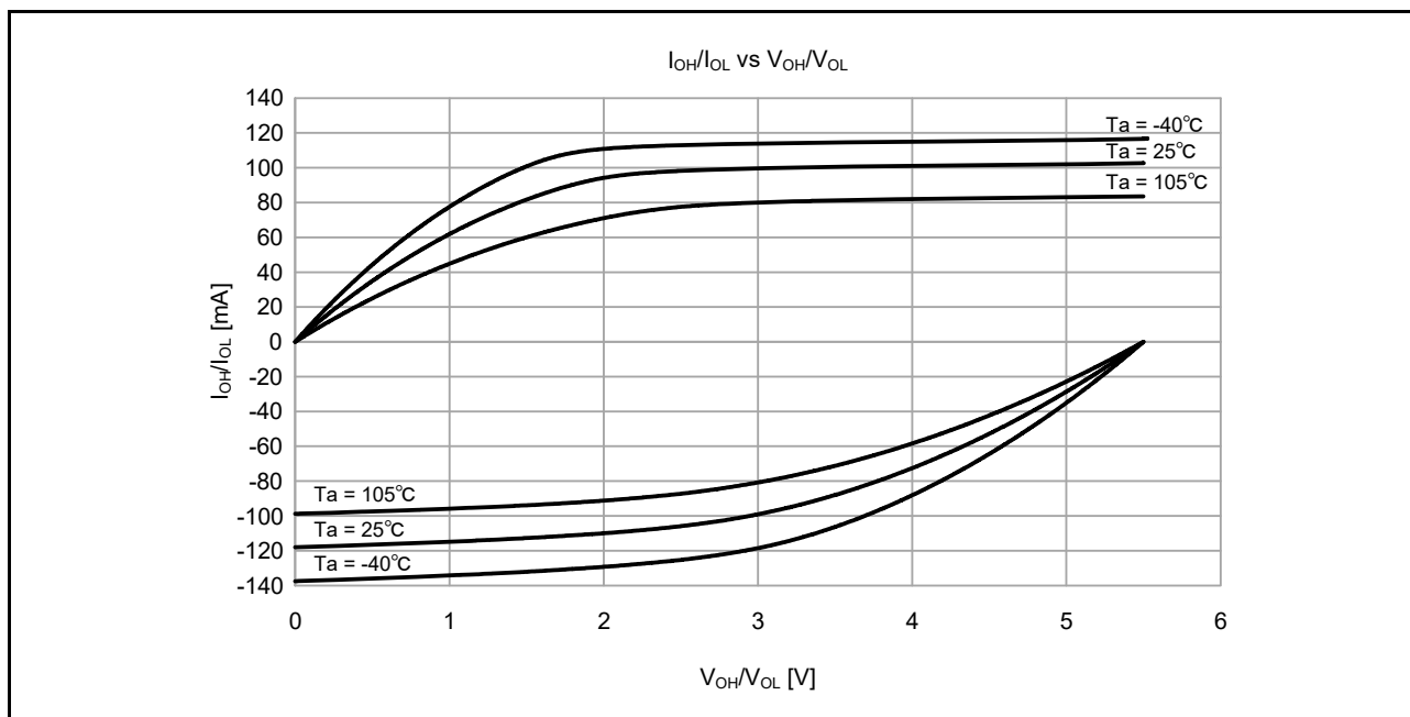
図 50.11 中駆動出力選択時の V_{CC} = 5.5\text{V} での V_{OH}/V_{OL} および I_{OH}/I_{OL} 温度特性 (参考データ)
