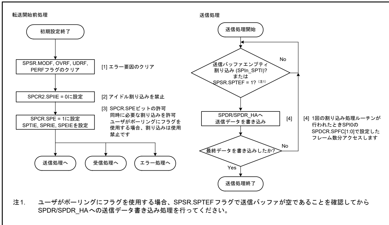
図 32.48 スレーブモードでの送信フロー
