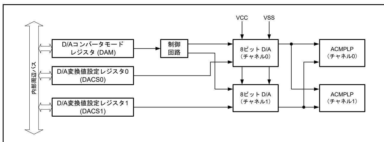
図 43.1 8ビットD/Aコンバータのブロック図
