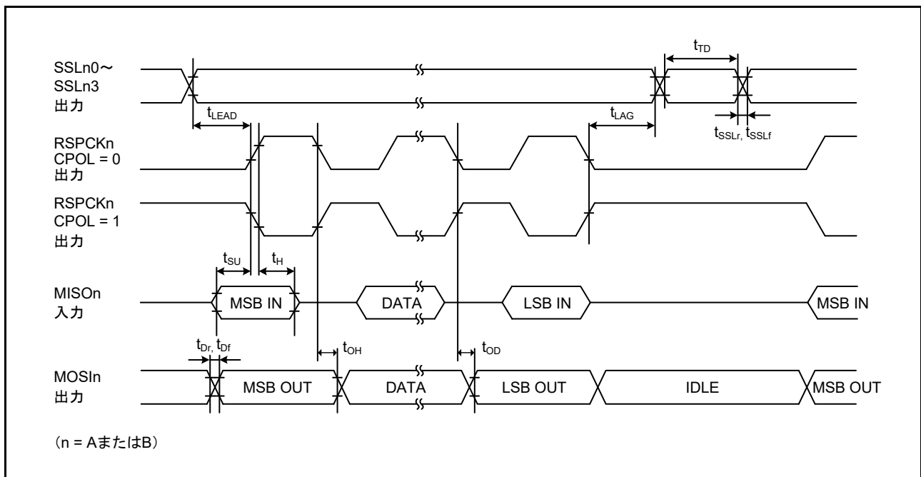
図 50.62 SPI タイミング (マスタ、CPHA = 0) (ビットレート : PCLKA を 2 分周以外に設定)
