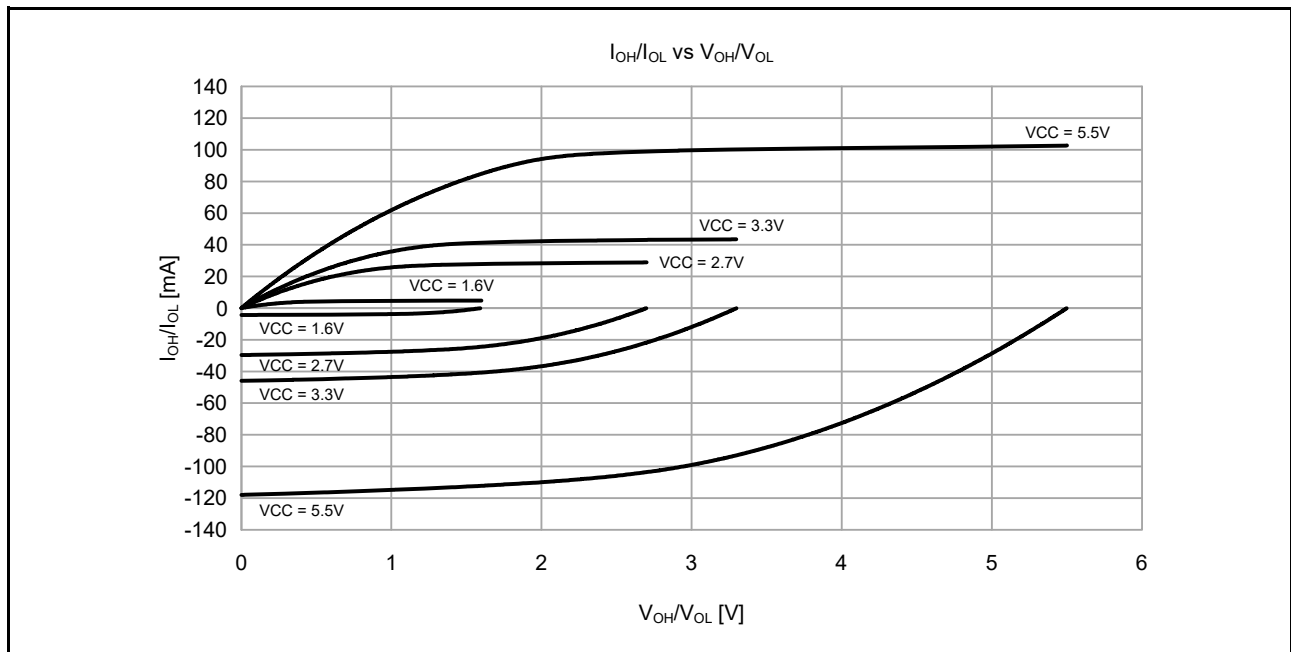
図 50.7 中駆動出力選択時の Ta = 25 °Cでの V OH /V OL および I OH /I OL 電圧特性 (参考データ)
