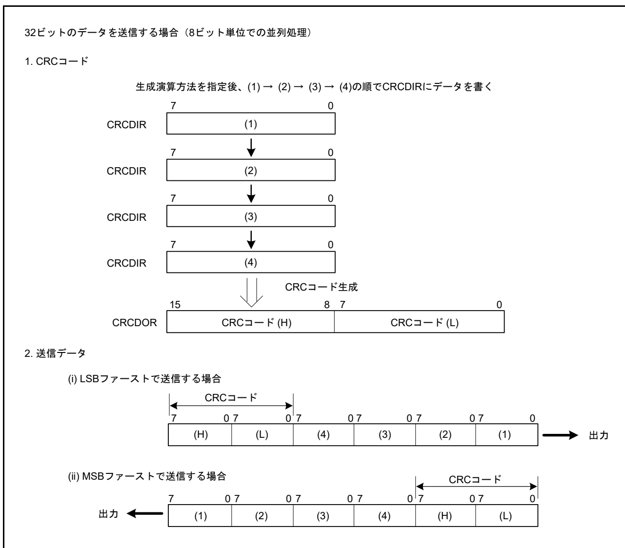
図 34.6 LSB ファーストと MSB ファーストのデータ送信
