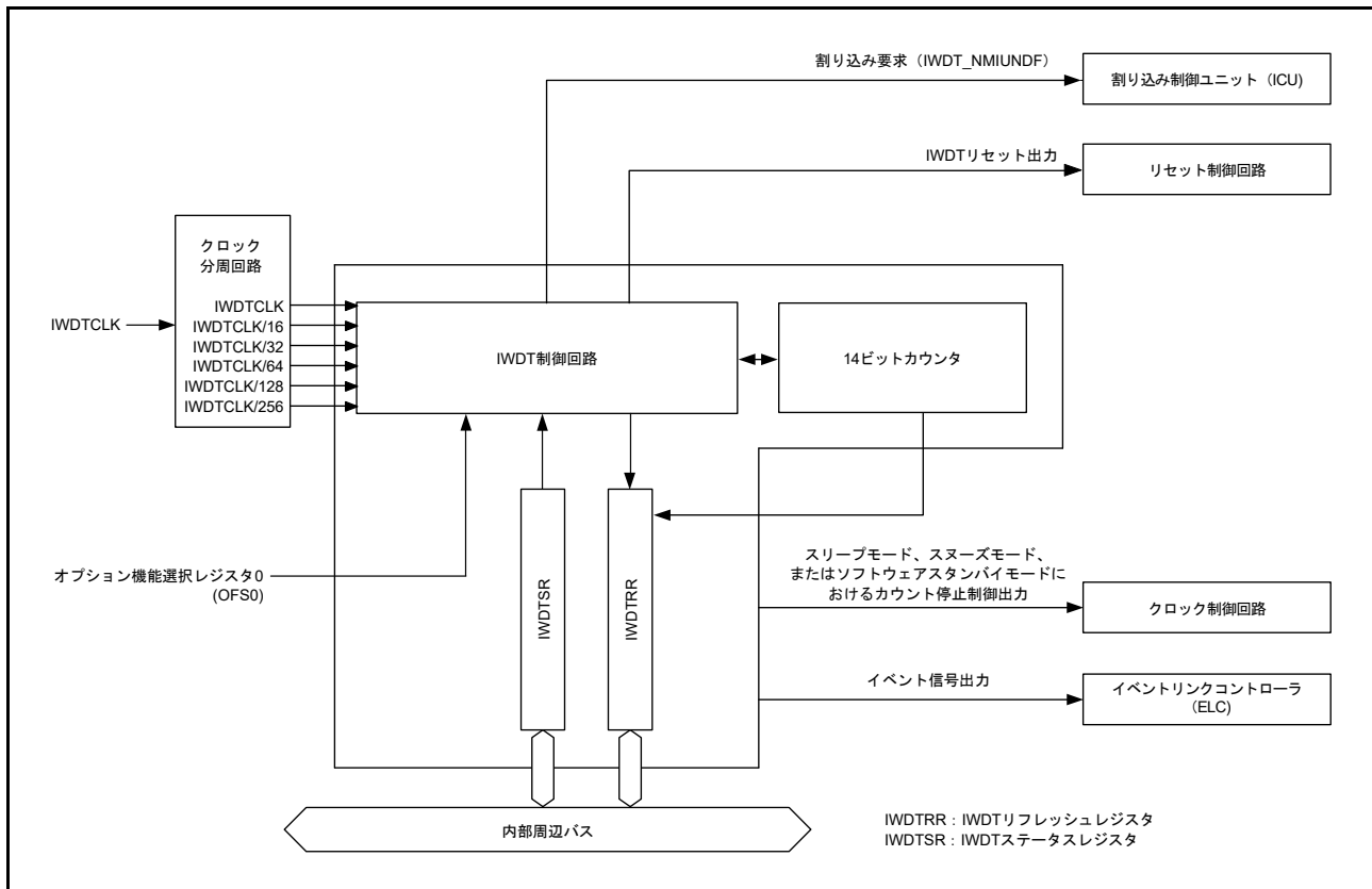
図 27.1 IWDT のブロック図
