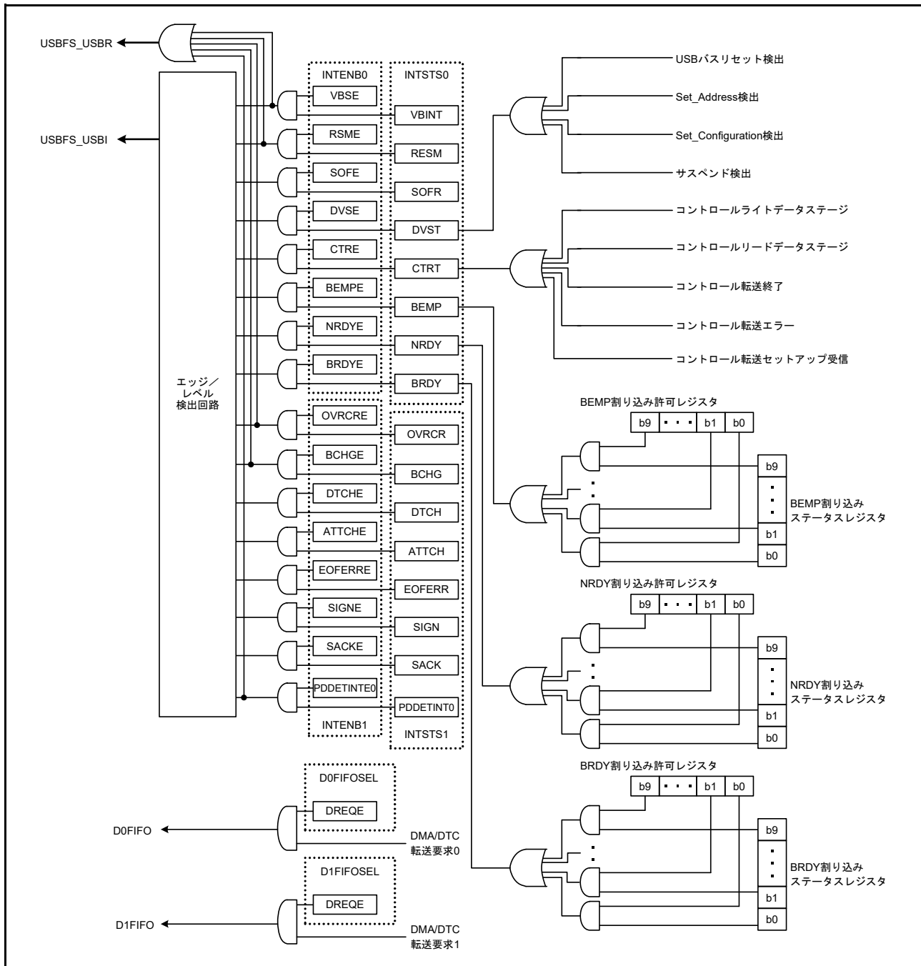
図 28.11 USBFS の割り込みに関連する回路
