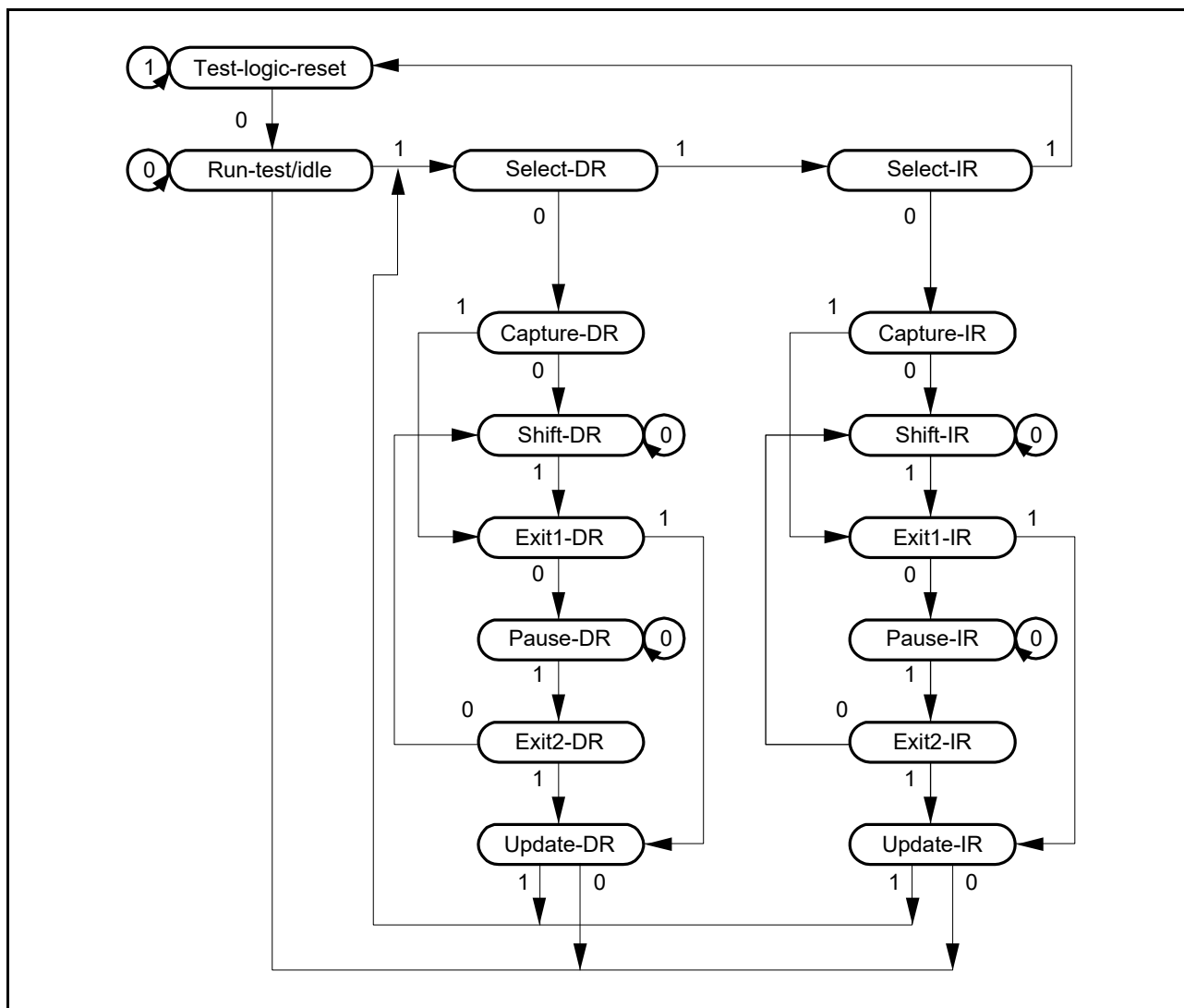
図 37.2 TAP コントローラの状態遷移図
