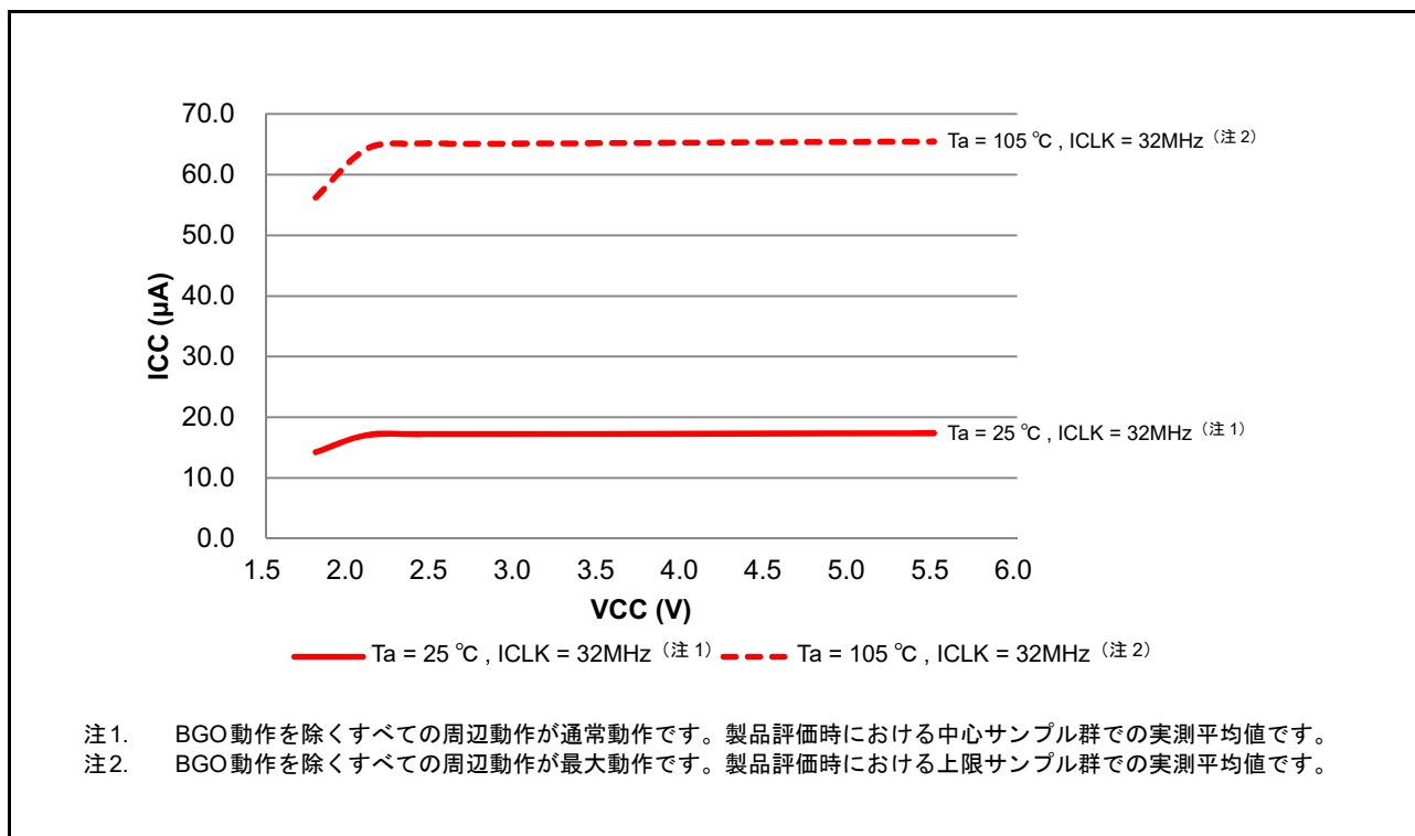
図 50.21 Subosc-speed モードにおける電圧依存性 (参考データ)
