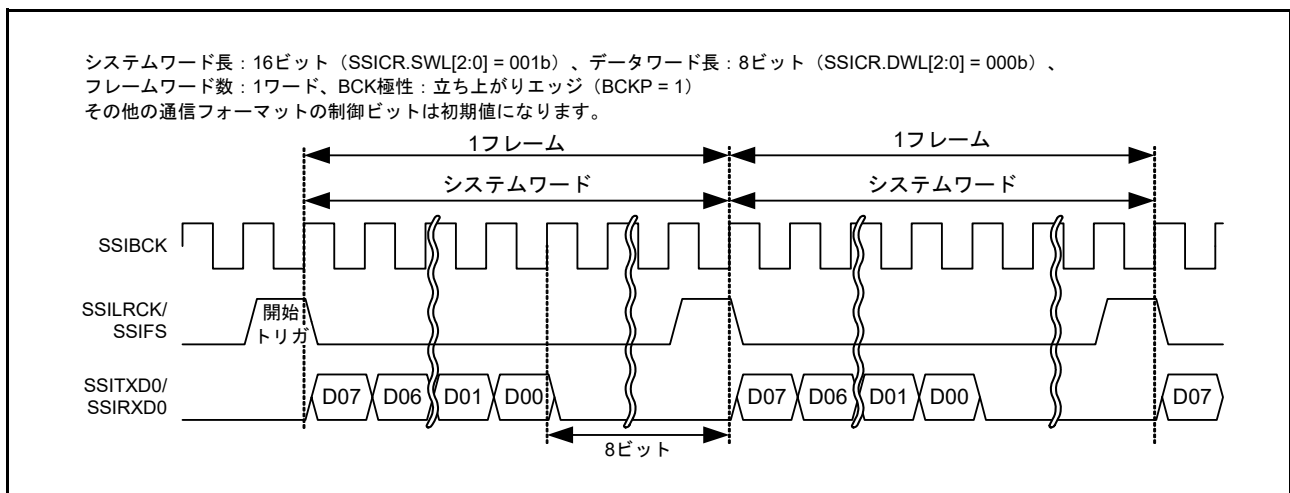
図 35.37 モノラルフォーマットでのショートフレーム (パディングあり、システムワード長 > データワード長)
