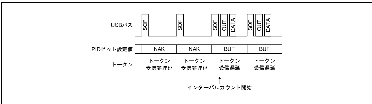
図 28.19 フレームと予想されるトークン受信の関係 (IITV[2:0] = 0 の場合)
