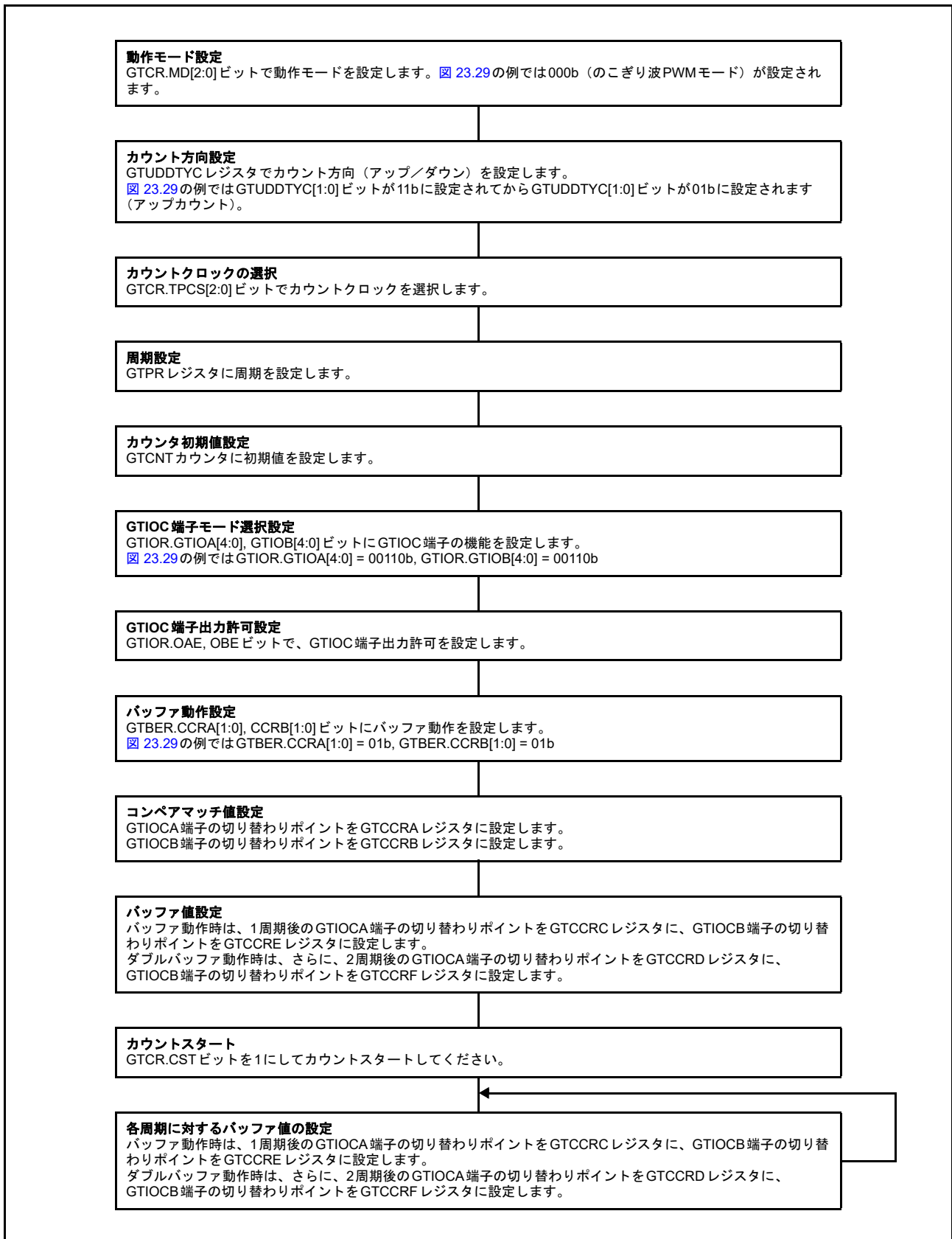
図 23.30 のこぎり波 PWM モードの設定例
