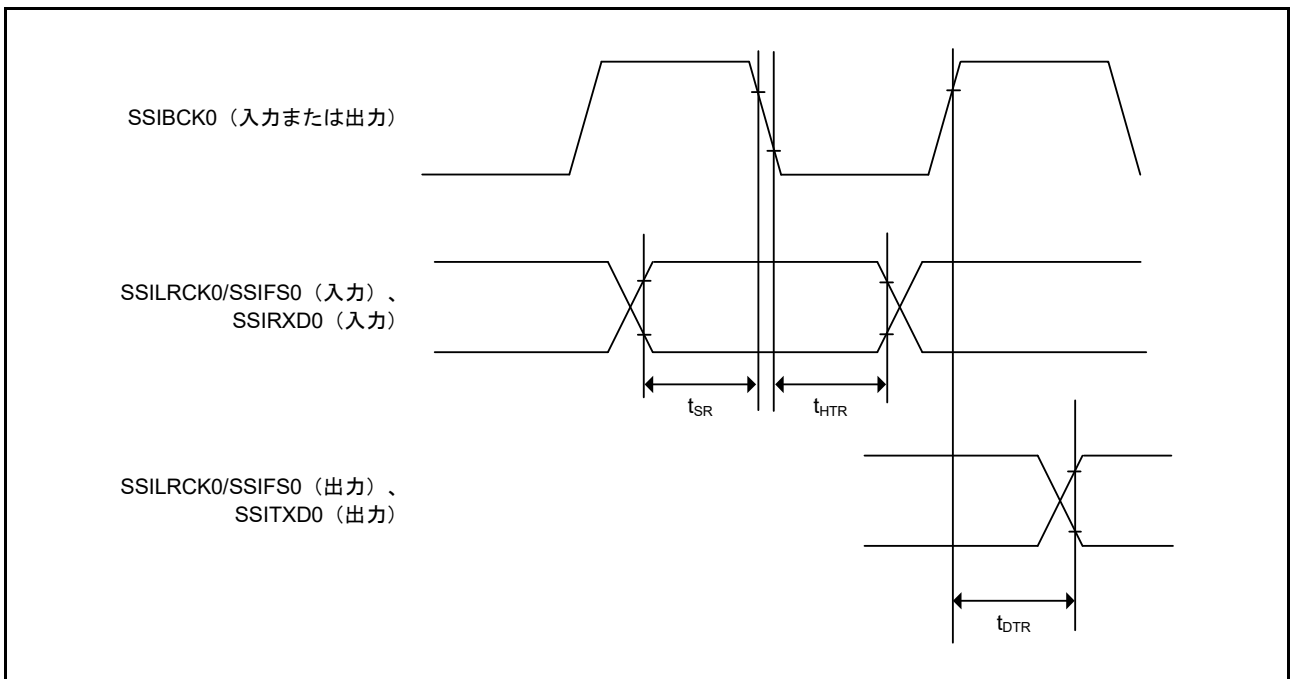
図 50.73 SSIE データ送受信タイミング (SSICR.BCKP = 1)
