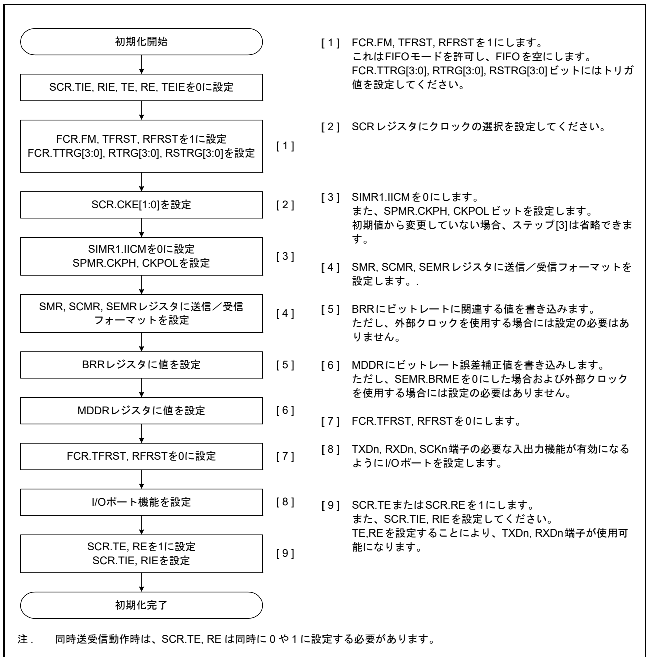
図 29.33 SCIの初期化フローチャート例 (クロック同期式モードまたはFIFO選択時)
