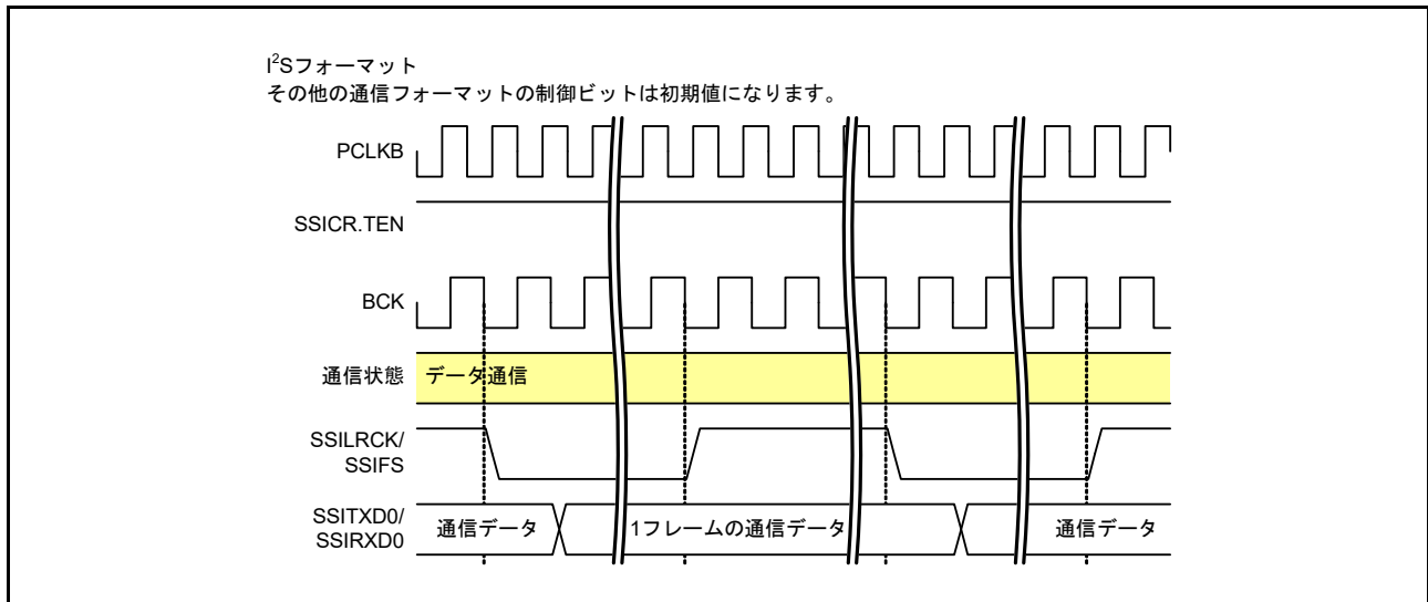
図 35.43 データ通信の継続
