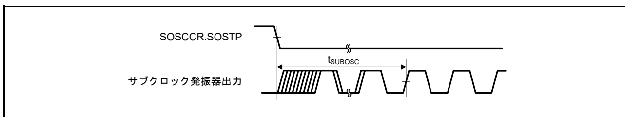
図 50.32 サブクロック発振開始タイミング
