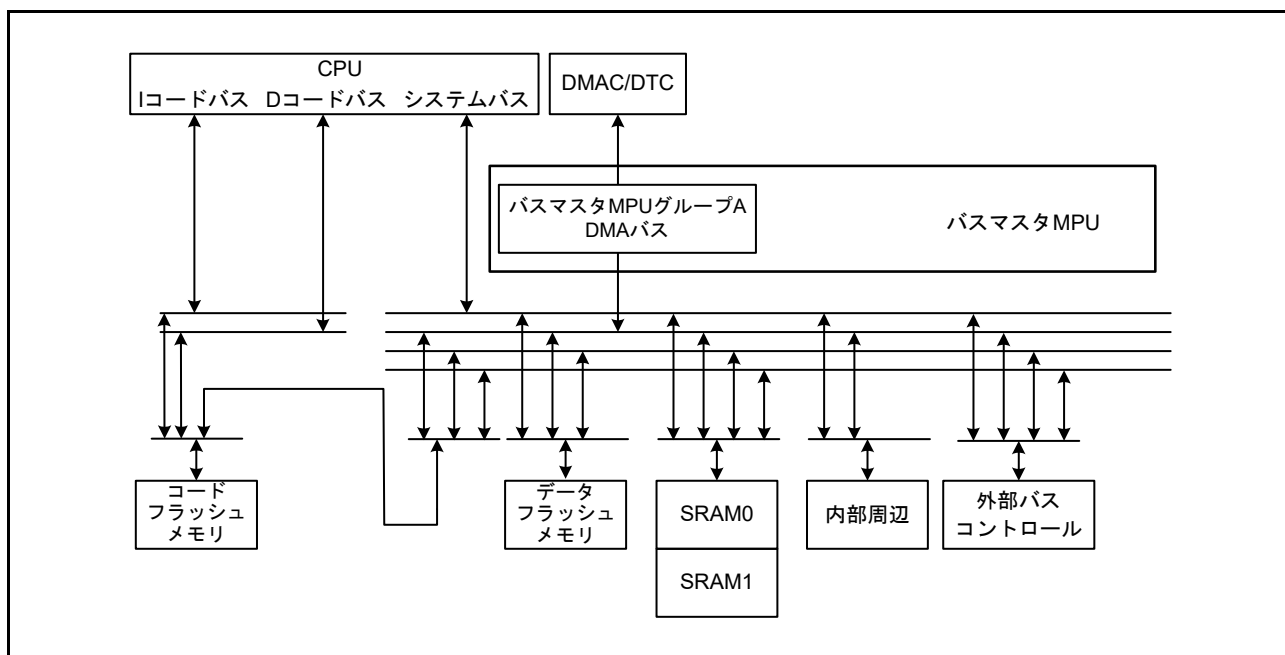
図 16.3 バスマスタ MPU のブロック図
