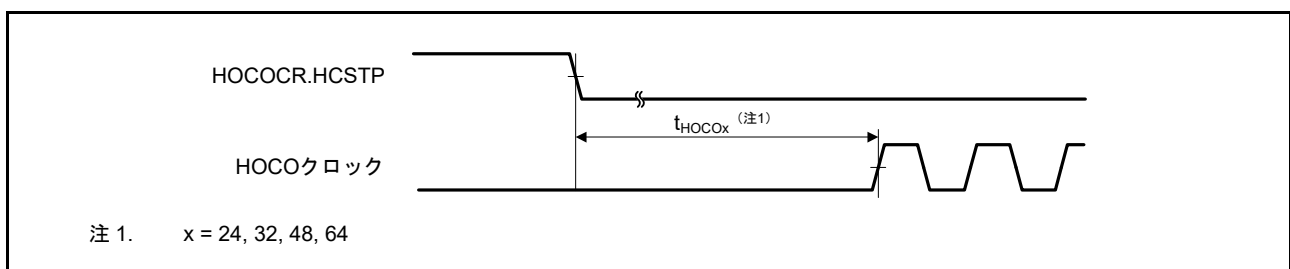
図 50.29 HOCO クロック発振開始タイミング (HOCOCR.HCSTP ビット設定による開始)
