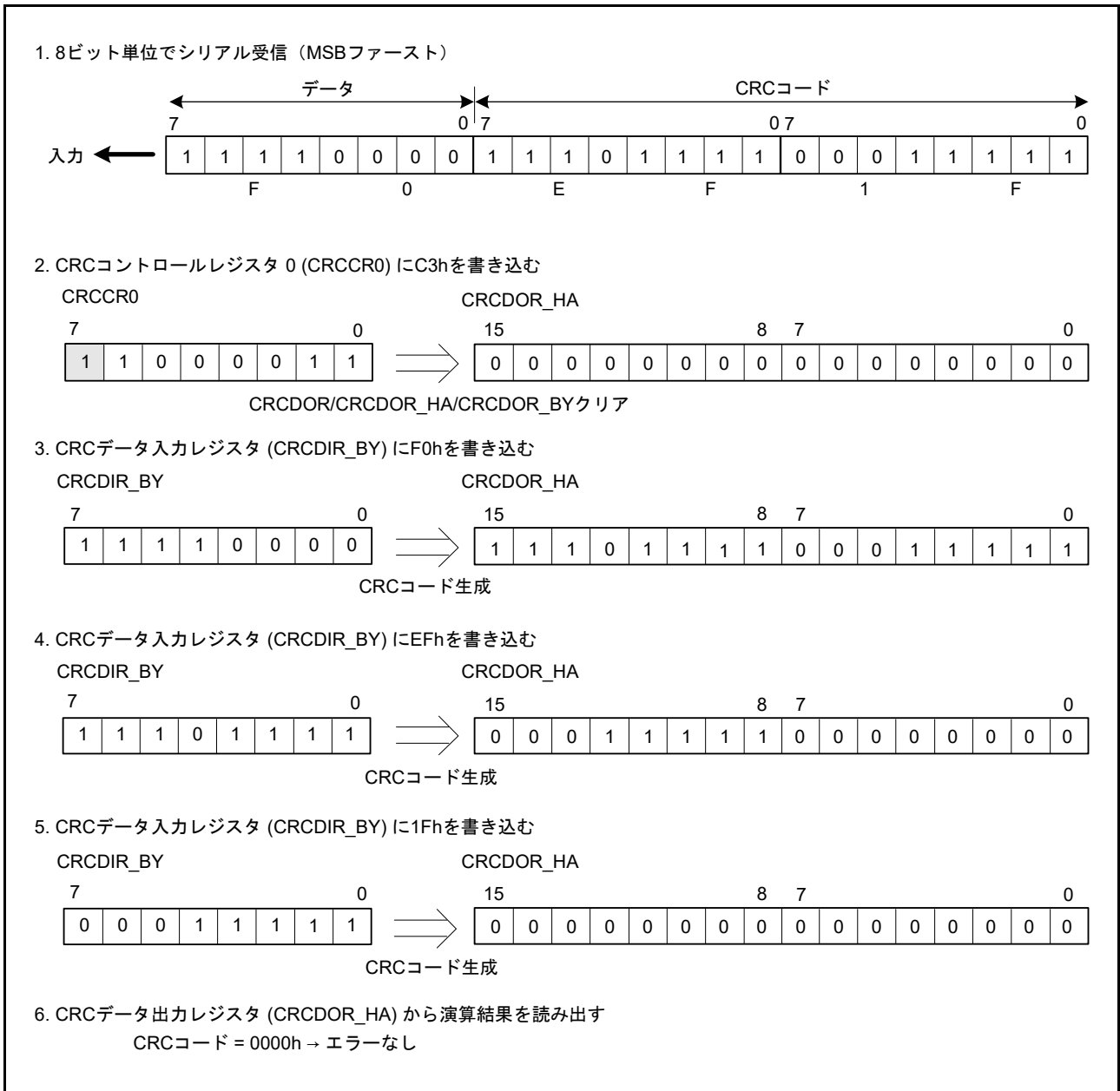
図 34.5 MSB ファーストのデータ受信
