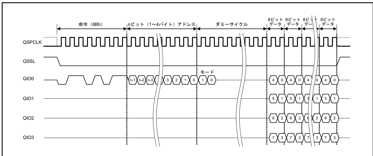
図 33.23 ファストリード Quad 出力バスサイクル
