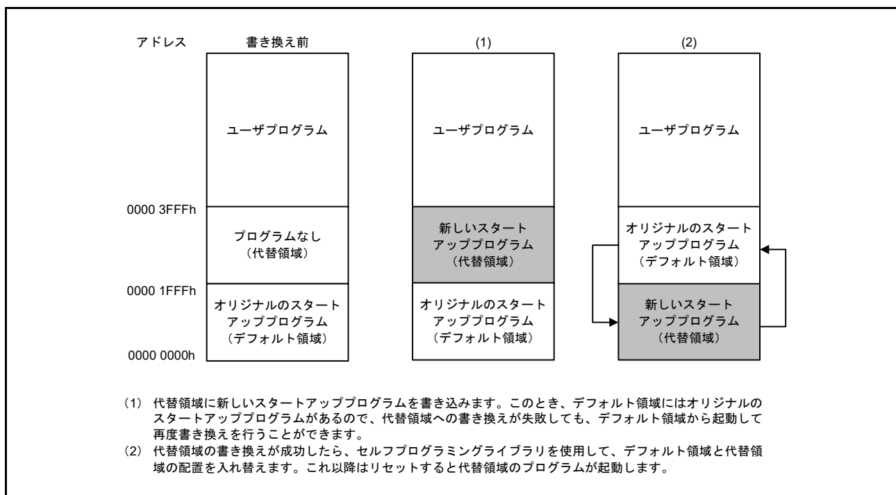
図 47.7 スタートアッププログラムプロテクションの概要
