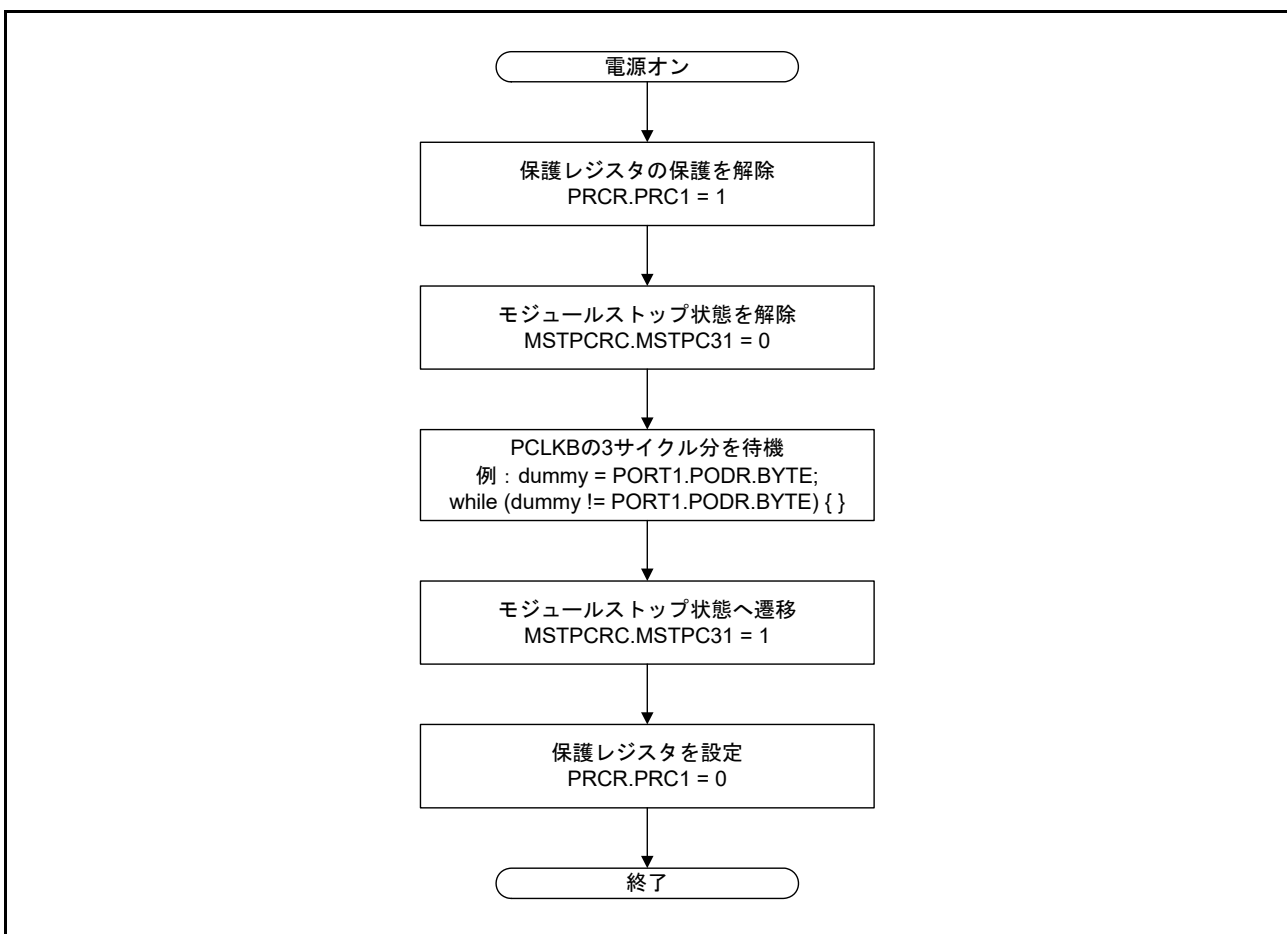
図 11.13 未使用回路の初期設定フロー例
