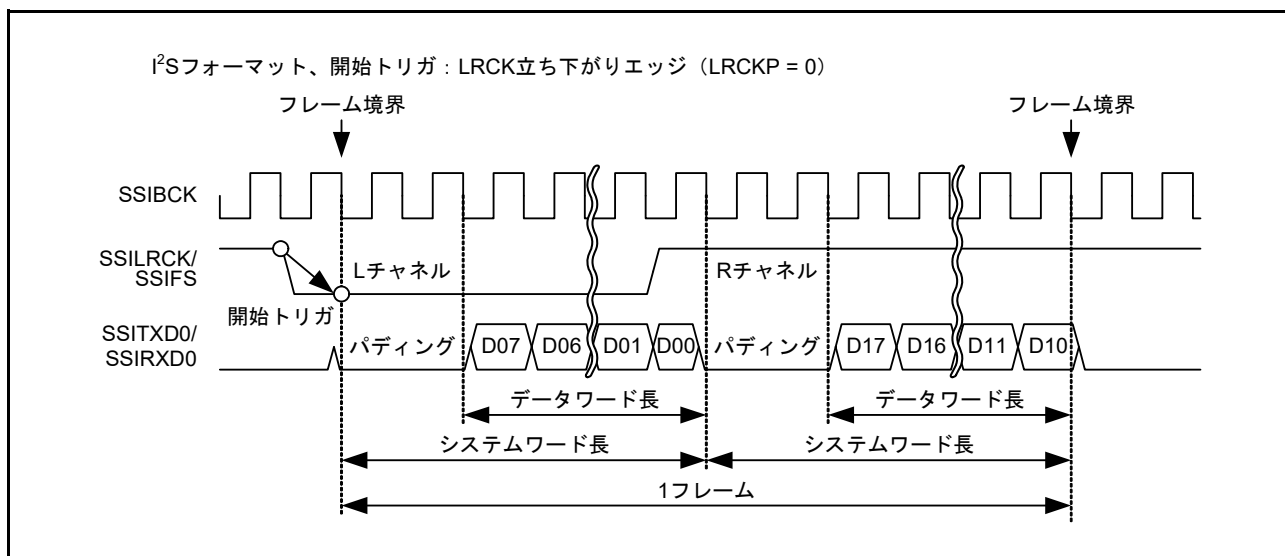
図 35.1 SSIE 通信フォーマット
