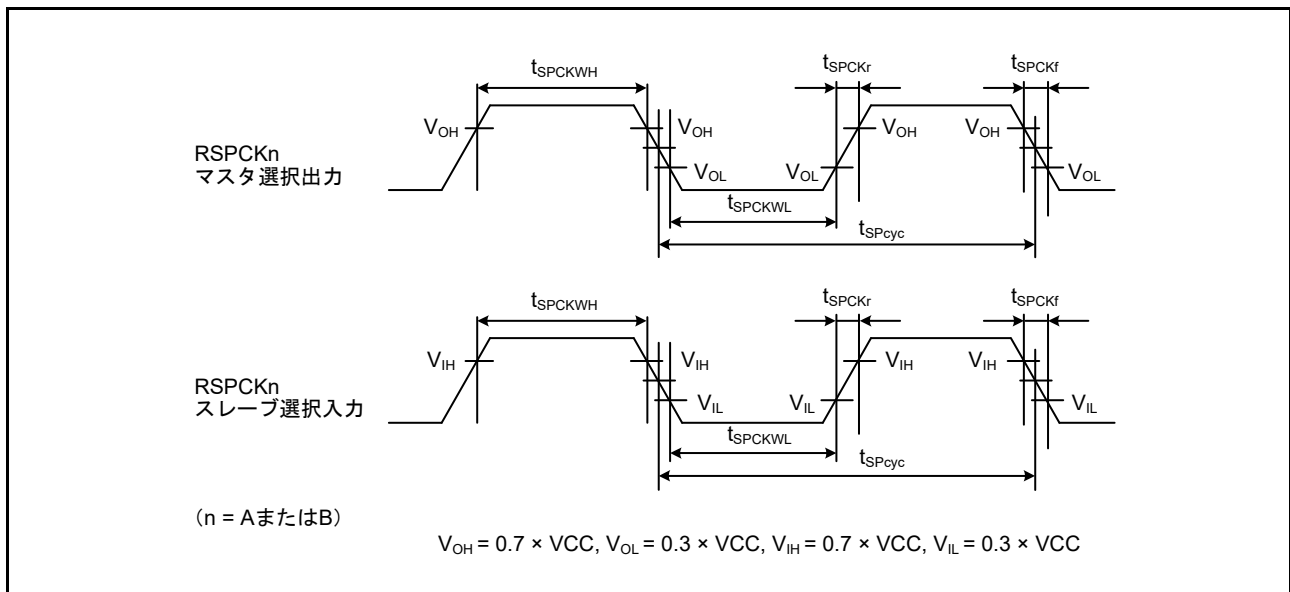
図 50.61 SPI クロックタイミング
