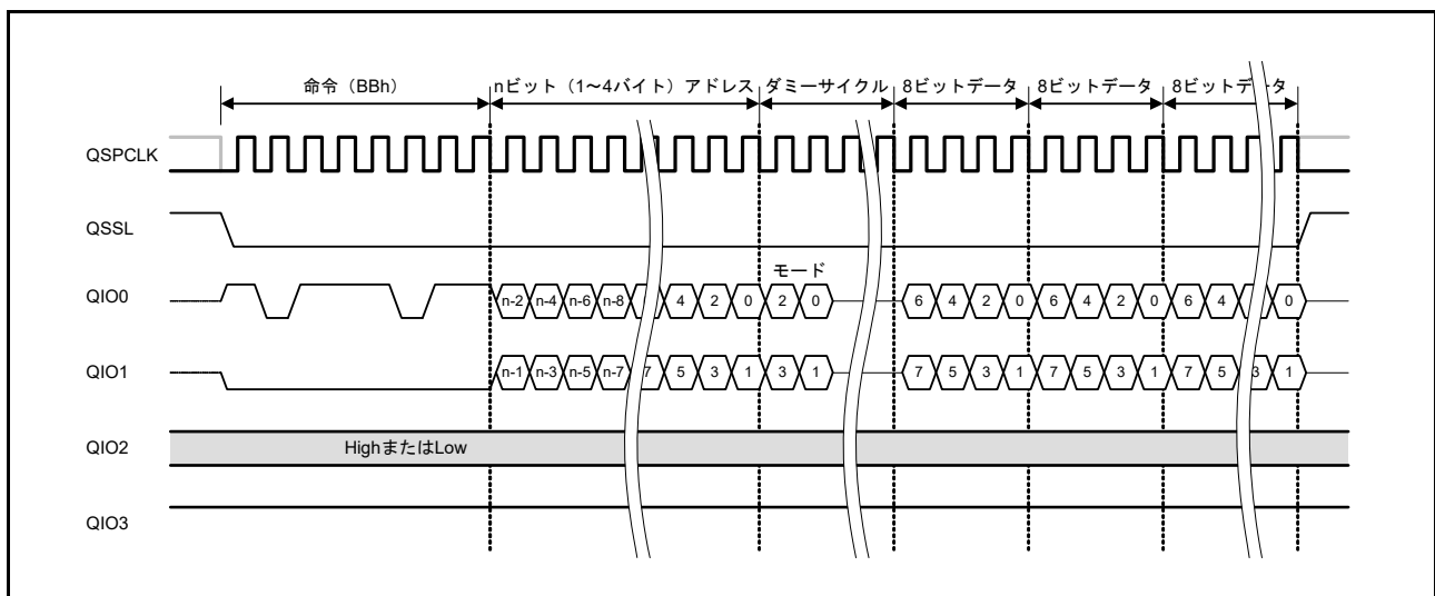
図 33.21 ファストリード Dual I/O バスサイクル
