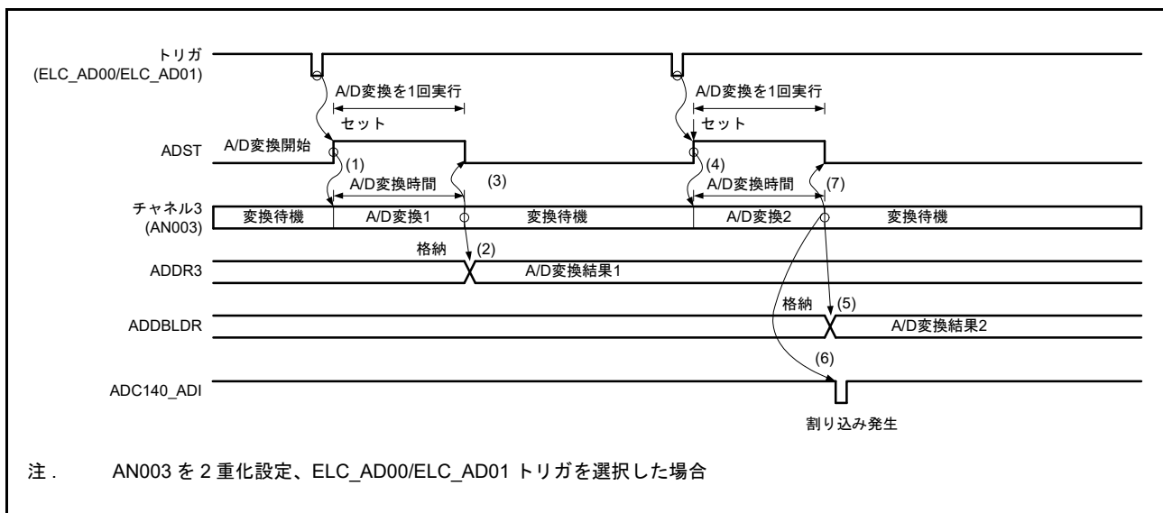
図 38.9 シングルスキャンモードの動作例 (ダブルトリガモード選択、AN003を2重化)
