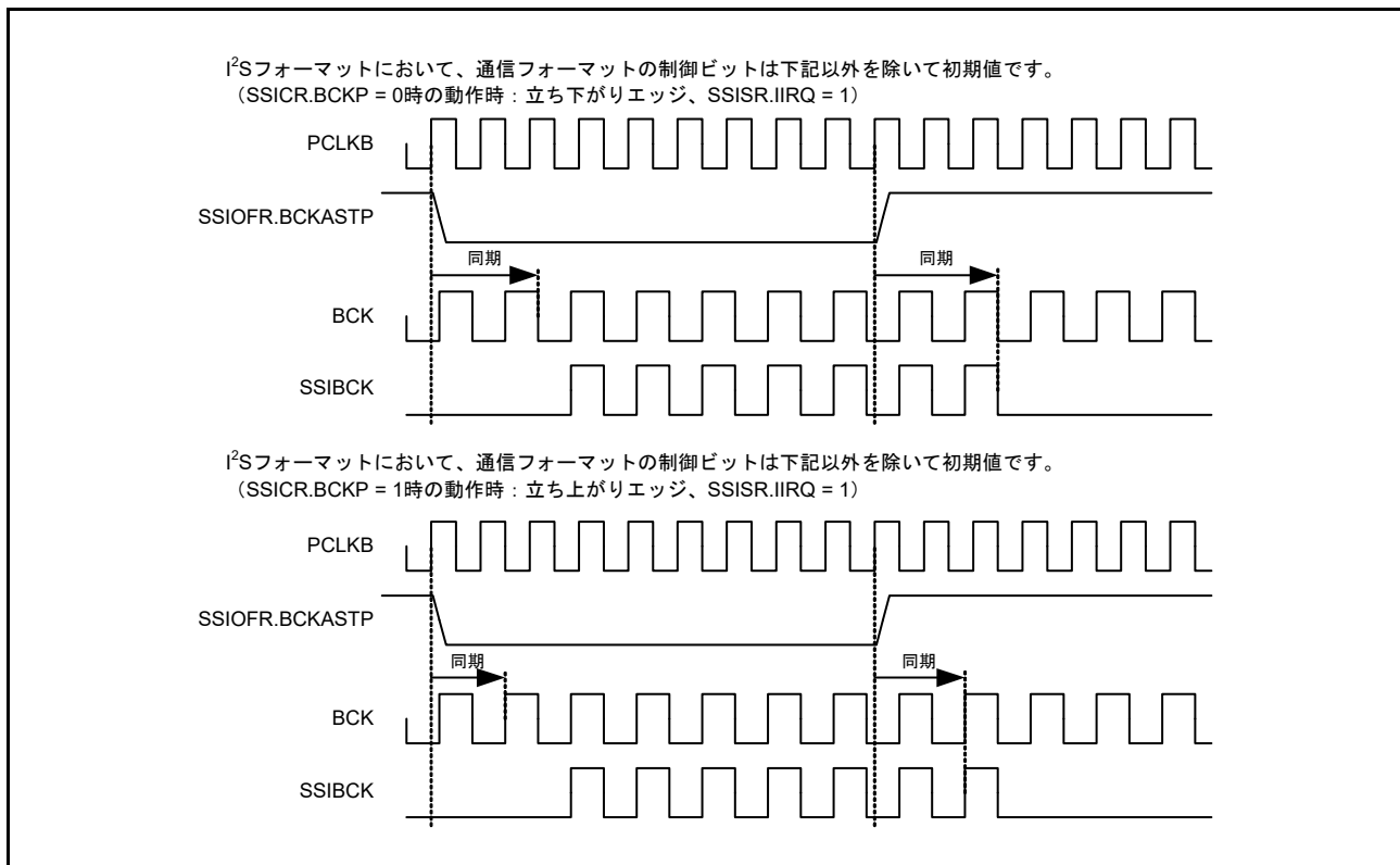
図 35.41 SSIOFR.BCKASTP ビットによる SSIBCK 出力の停止例
