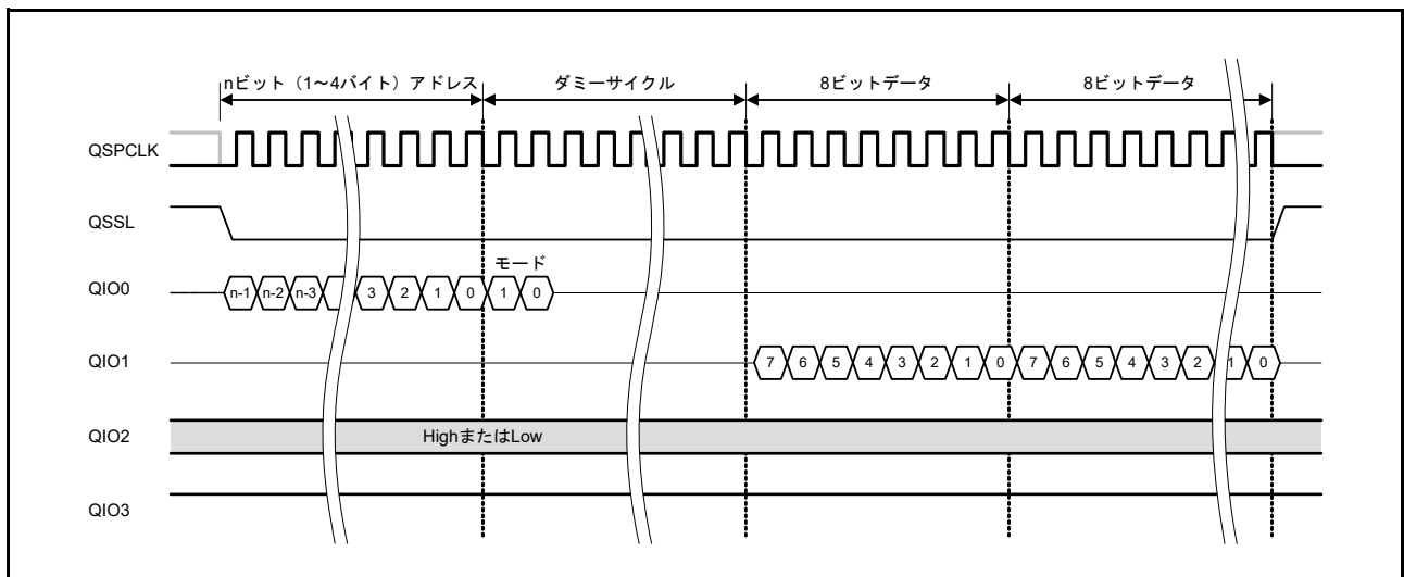
図 33.18 XIP モード時のファストリードバスサイクル
