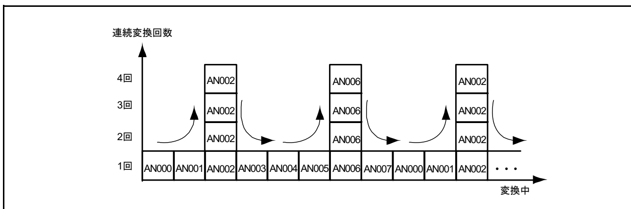
図 38.2 ADADC.ADC[2:0] = 011b、ADADS0.ADS02 = 1、ADADS0.ADS06 = 1 選択時のスキャン変換シーケンス
