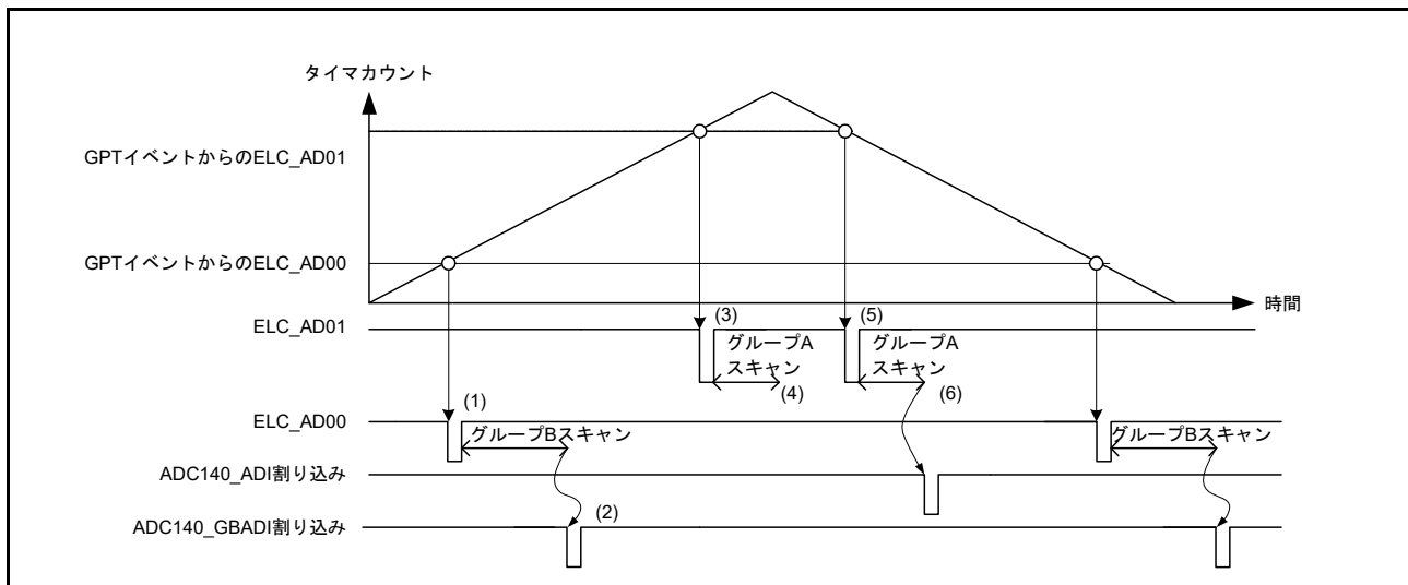
図 38.14 グループスキャンモードかつダブルトリガモード設定時の動作 (ELC からの同期トリガ)
