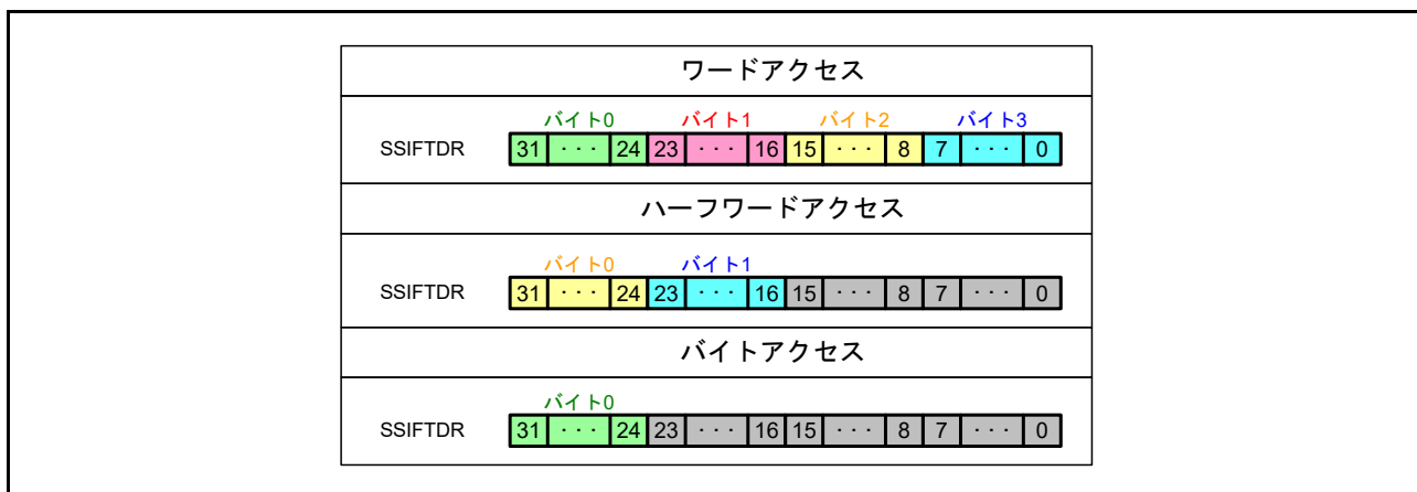
図 35.28 送信 FIFO データレジスタへのレジスタアクセス例
