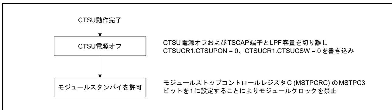
図 44.10 CTSUS 停止フロー
