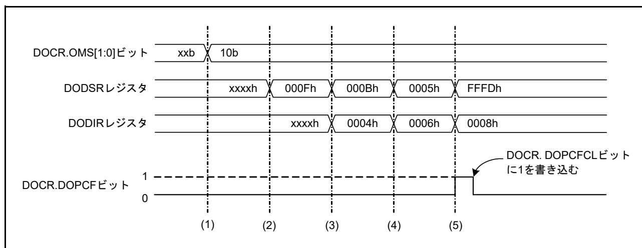
図 45.4 データ減算モードの動作例
