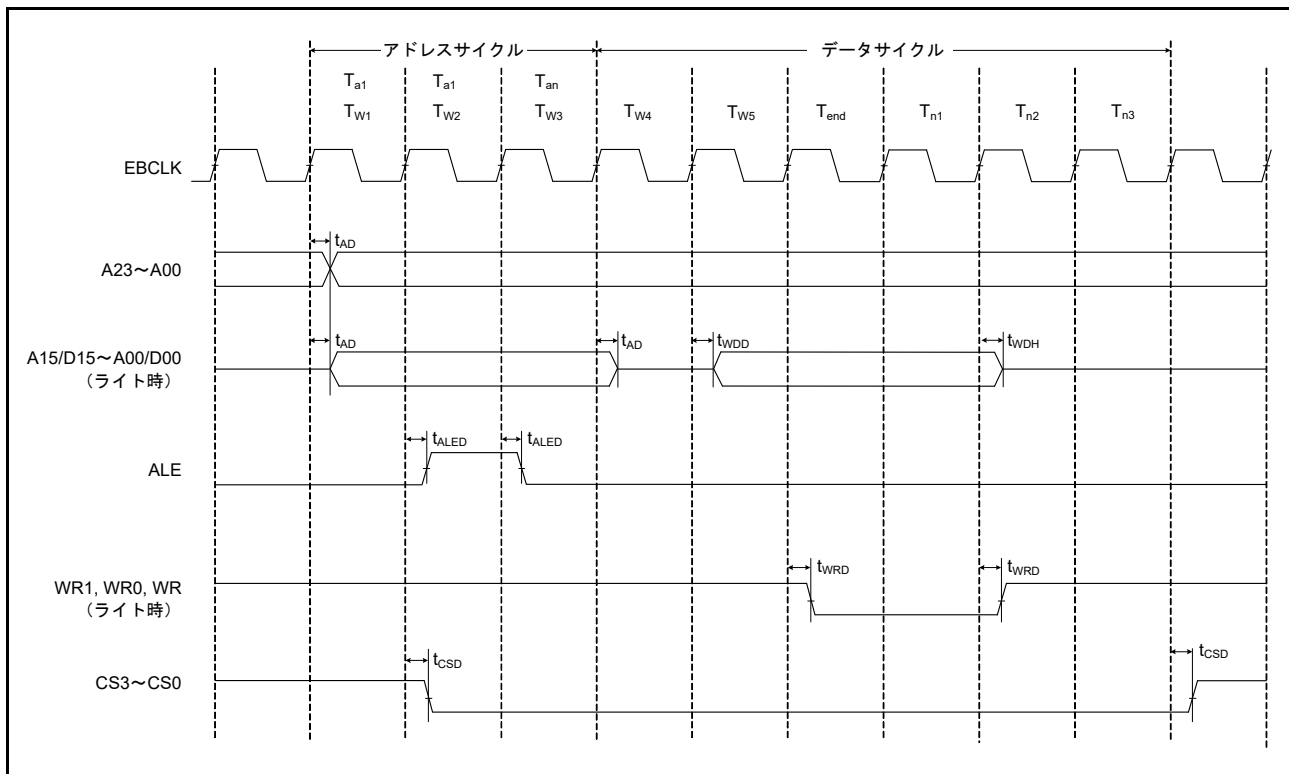
図 50.41 アドレス/データマルチプレクスバスのライトアクセスタイミング
