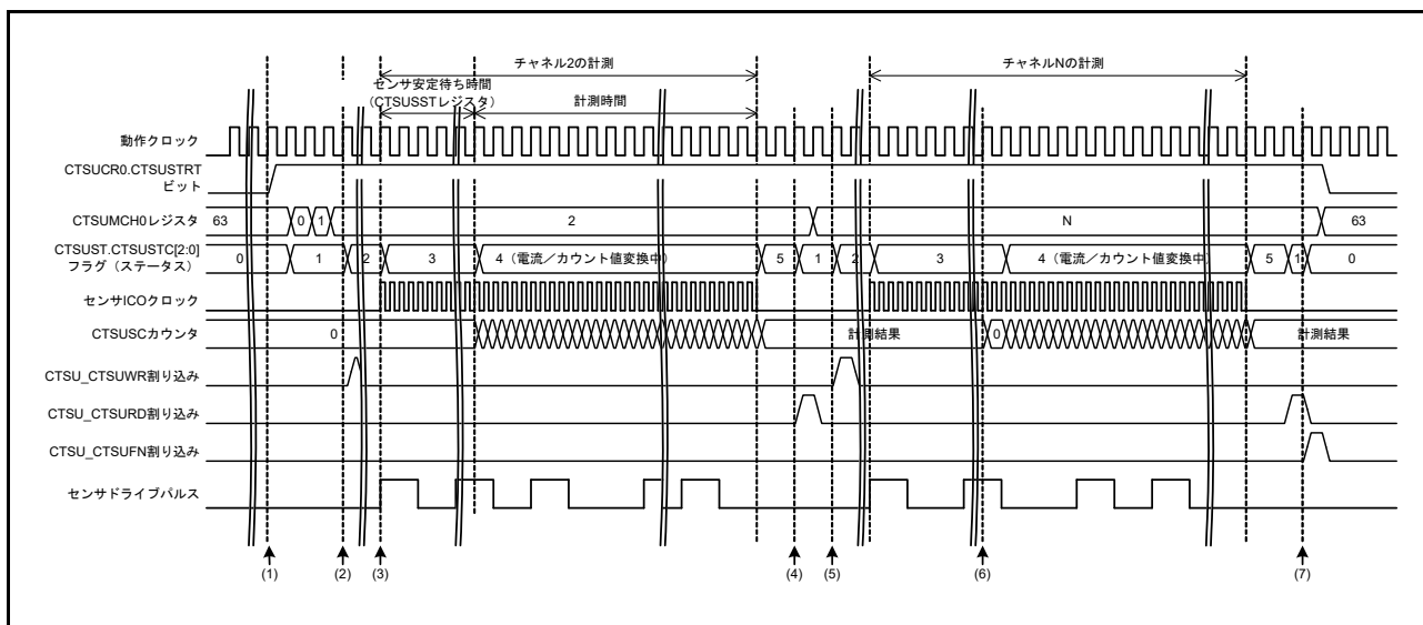
図 44.15 自己容量マルチスキャンモードのタイミング (計測開始条件がソフトウェアトリガの場合)
