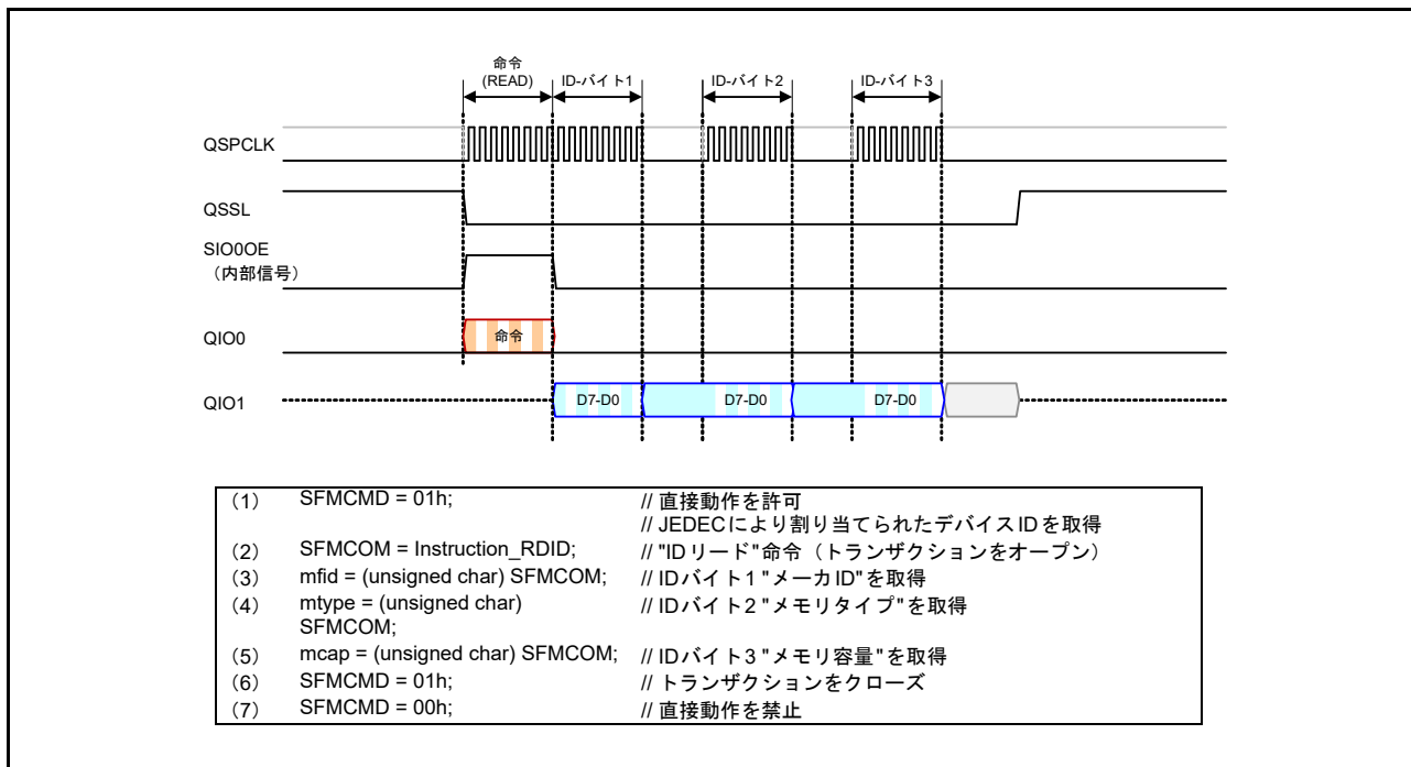
図 33.34 ID リードの直接通信タイミング例
