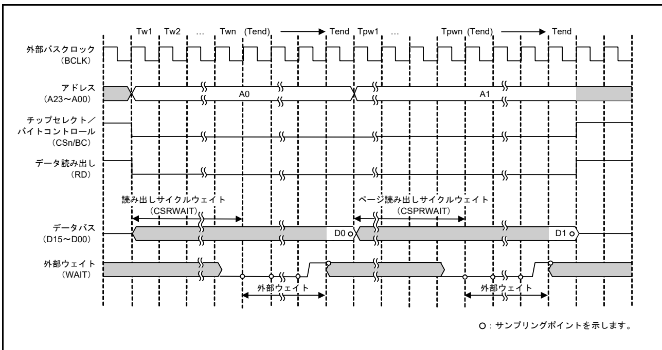
図 15.26 16 ビットバス空間に対するページリードアクセスの外部ウェイトタイミング例 (EBCLK 端子出力選択ビットで BCLK の 1 分周を選択した場合) (n = 0 ~ 3, m = 0, 1)
