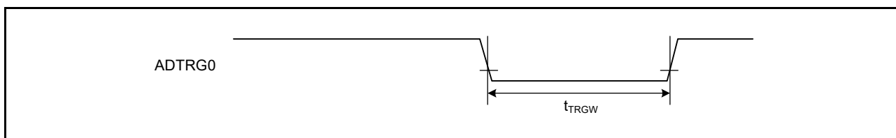
図 50.51 ADC14 トリガ入力タイミング
