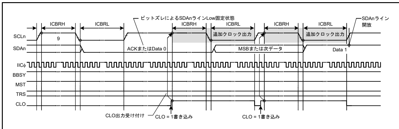
図 30.49 SCL クロック追加出力機能 (CLO ビット使用)
