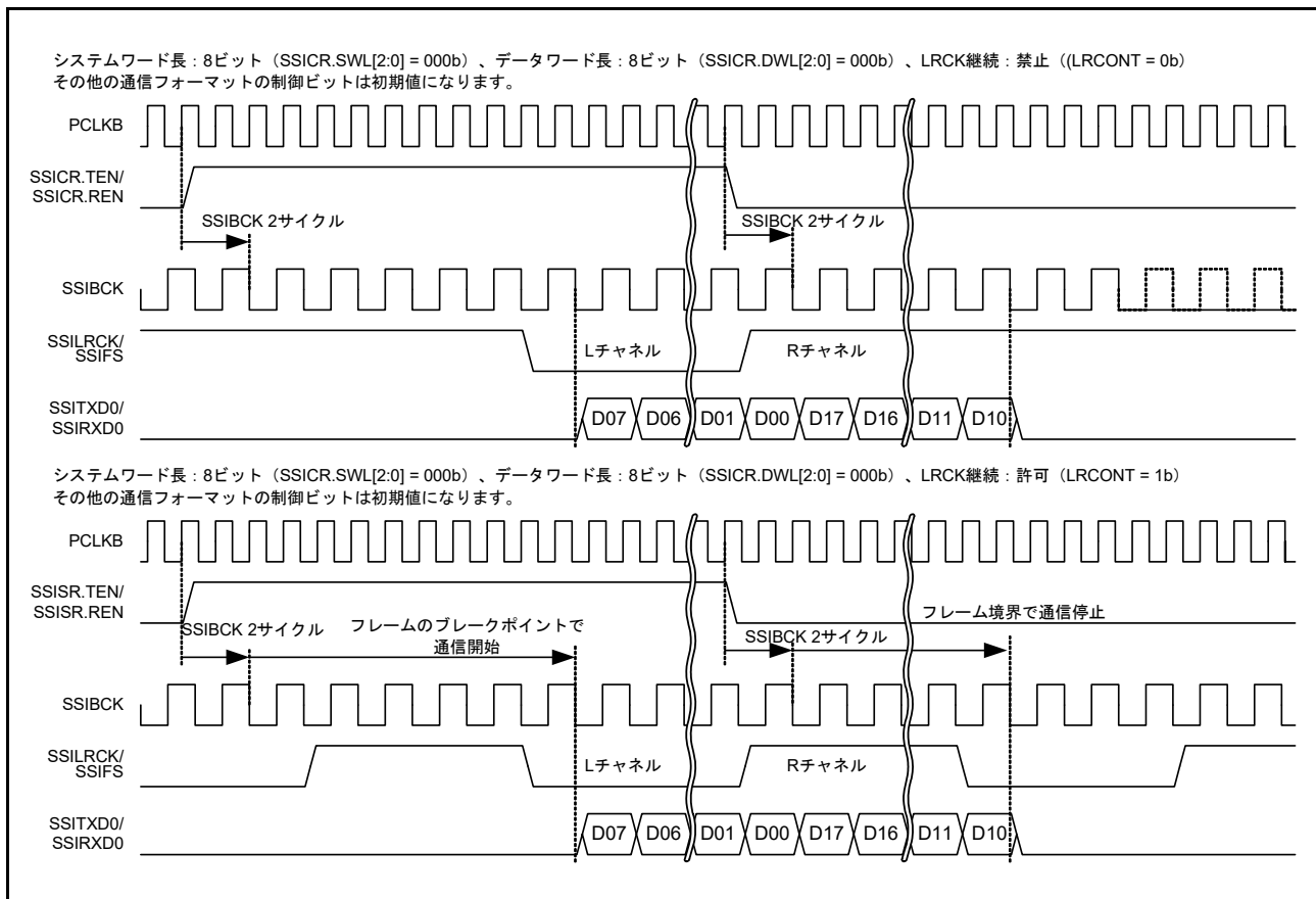
図 35.31 LR クロック/フレーム同期継続の動作例
