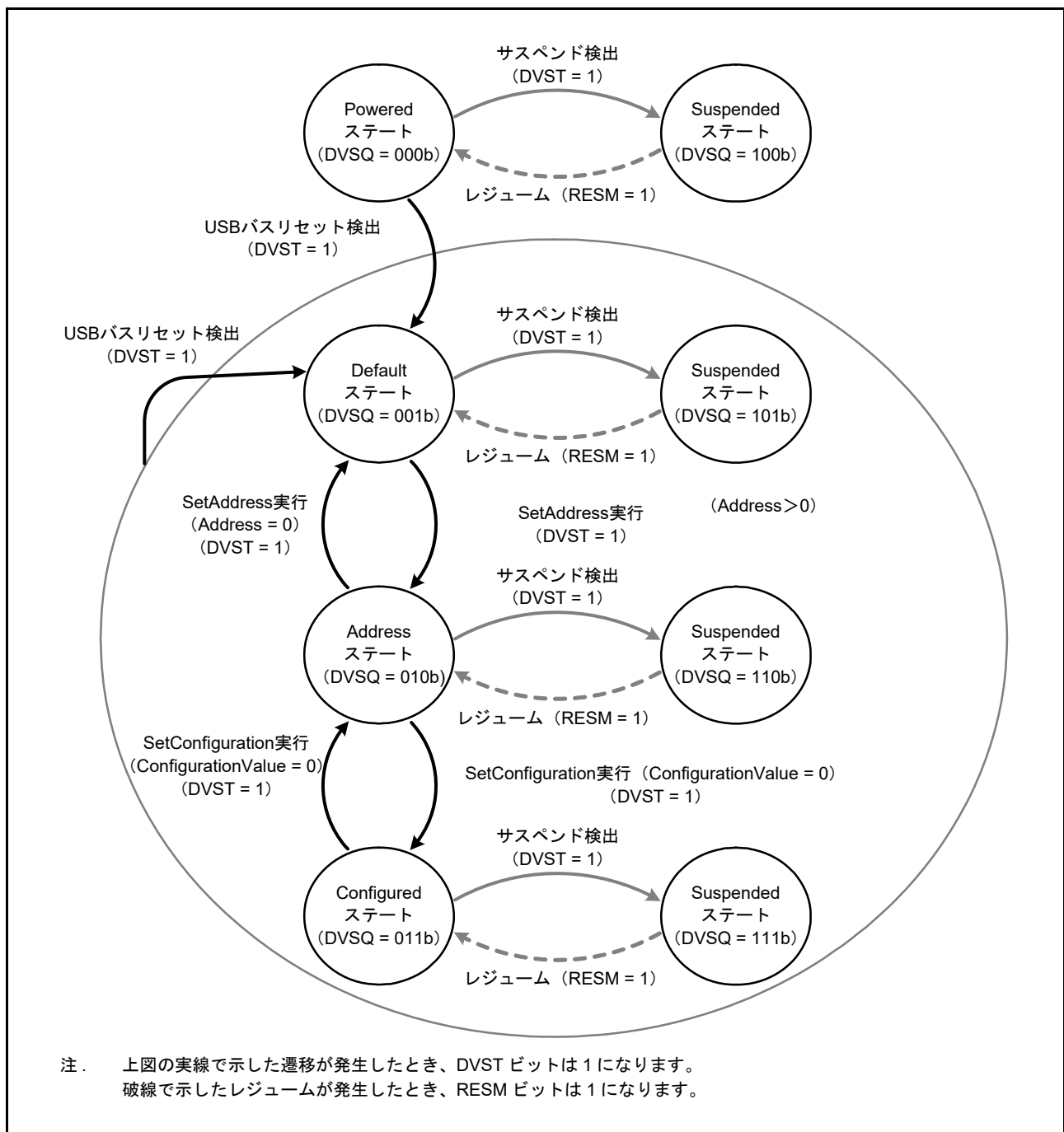
図 28.15 デバイスステートの遷移
