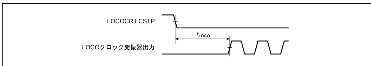
図 50.28 LOCO クロック発振開始タイミング
