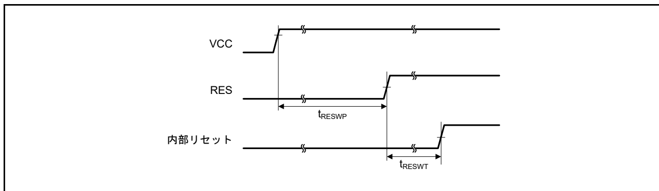
図 50.34 電源投入時リセット入力タイミング
