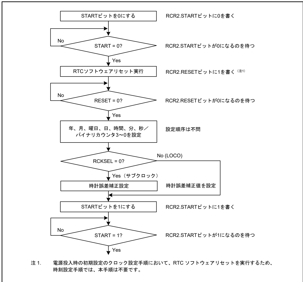
図 25.4 時刻の設定
