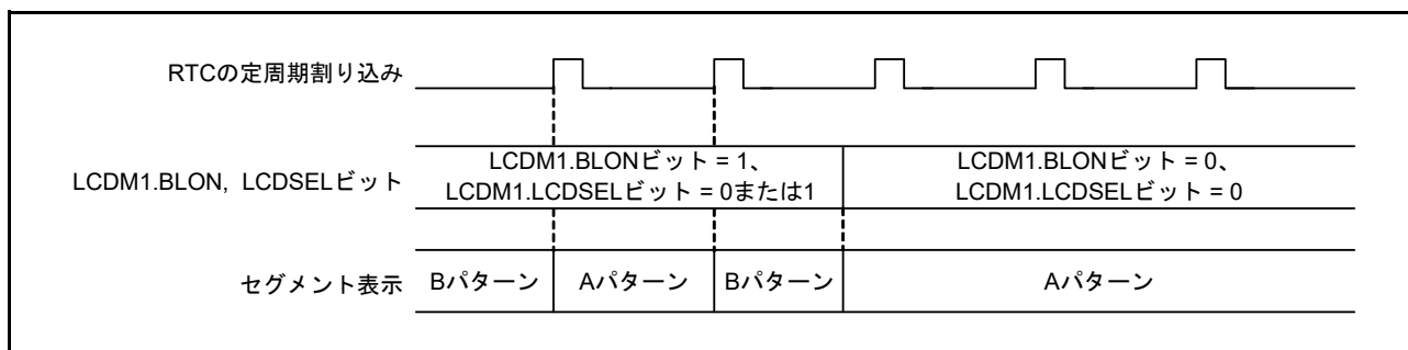
図 48.4 点滅表示から Aパターン表示への切り替え動作
