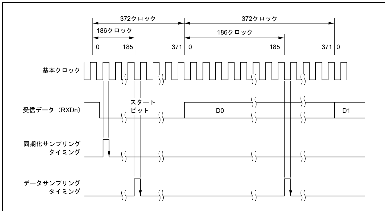
図 29.49 スマートカードインタフェースモード時の受信データサンプリングタイミング (ビットレートの372倍のクロック周波数の場合)
