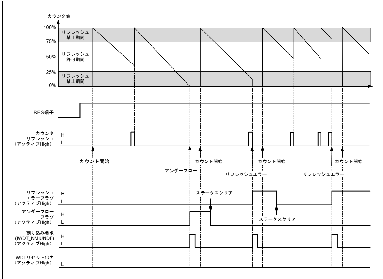
図 27.3 オートスタートモードでの動作例
