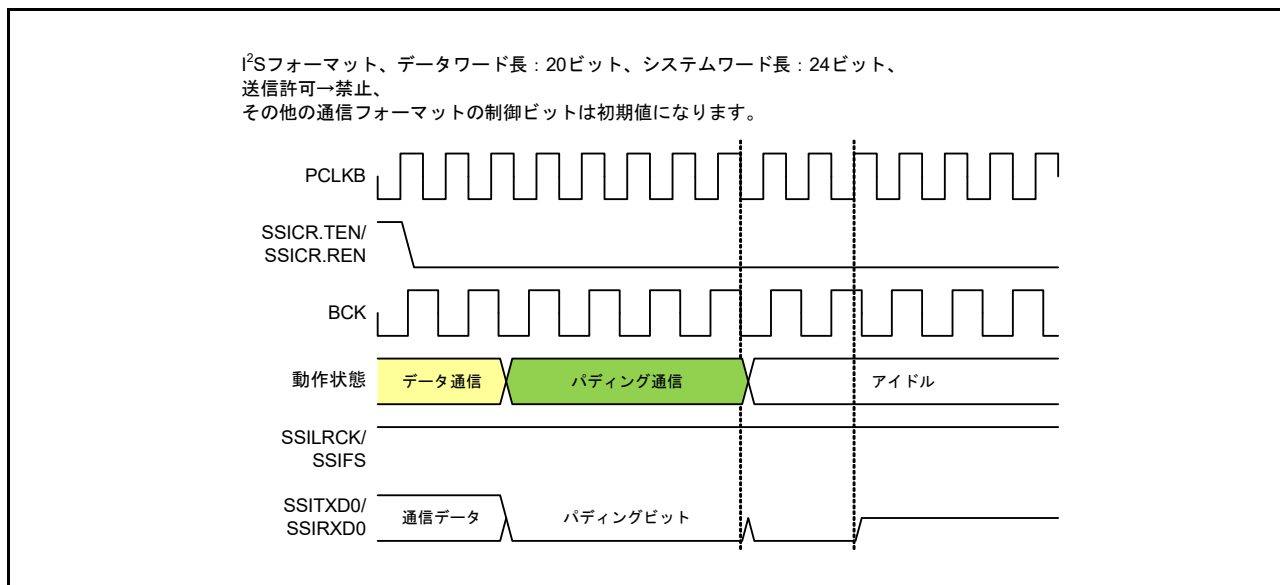
図 35.47 パディング通信からの停止
