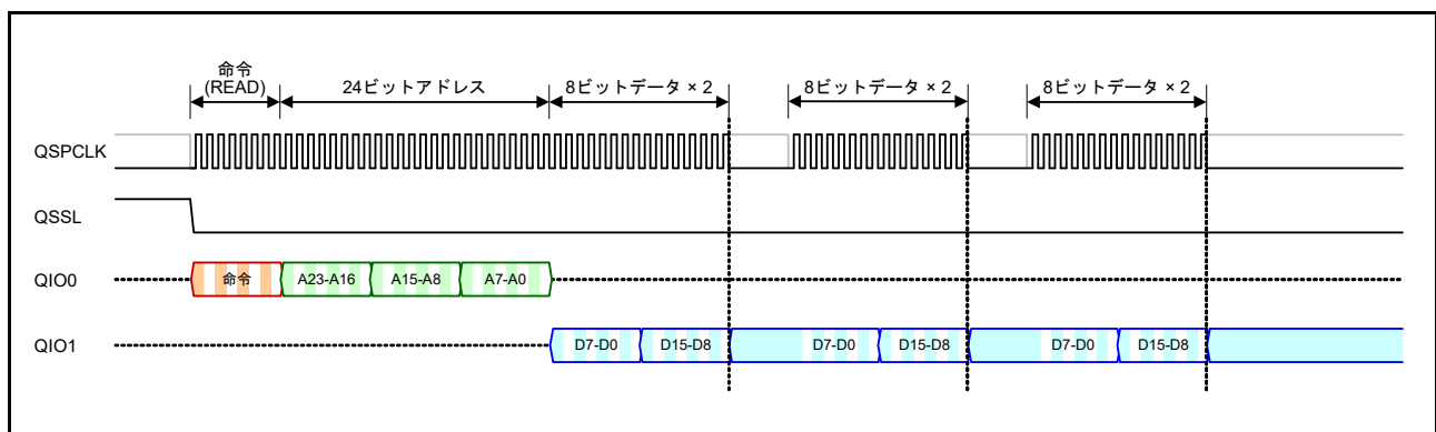
図 33.32 SPI バスサイクル拡張を使用した連続データリード動作
