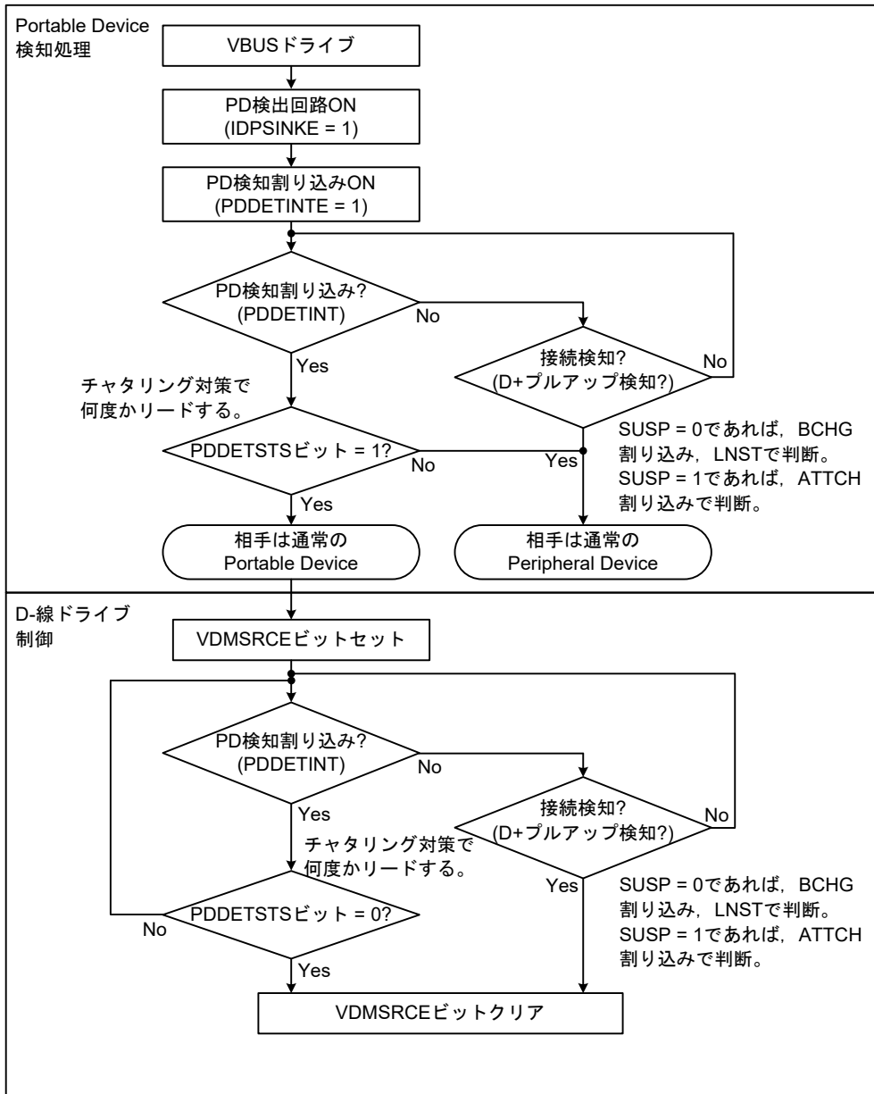
図14-68 Charging Downstream Portとしての処理フロー ( (1) ~ (4) の処理)
