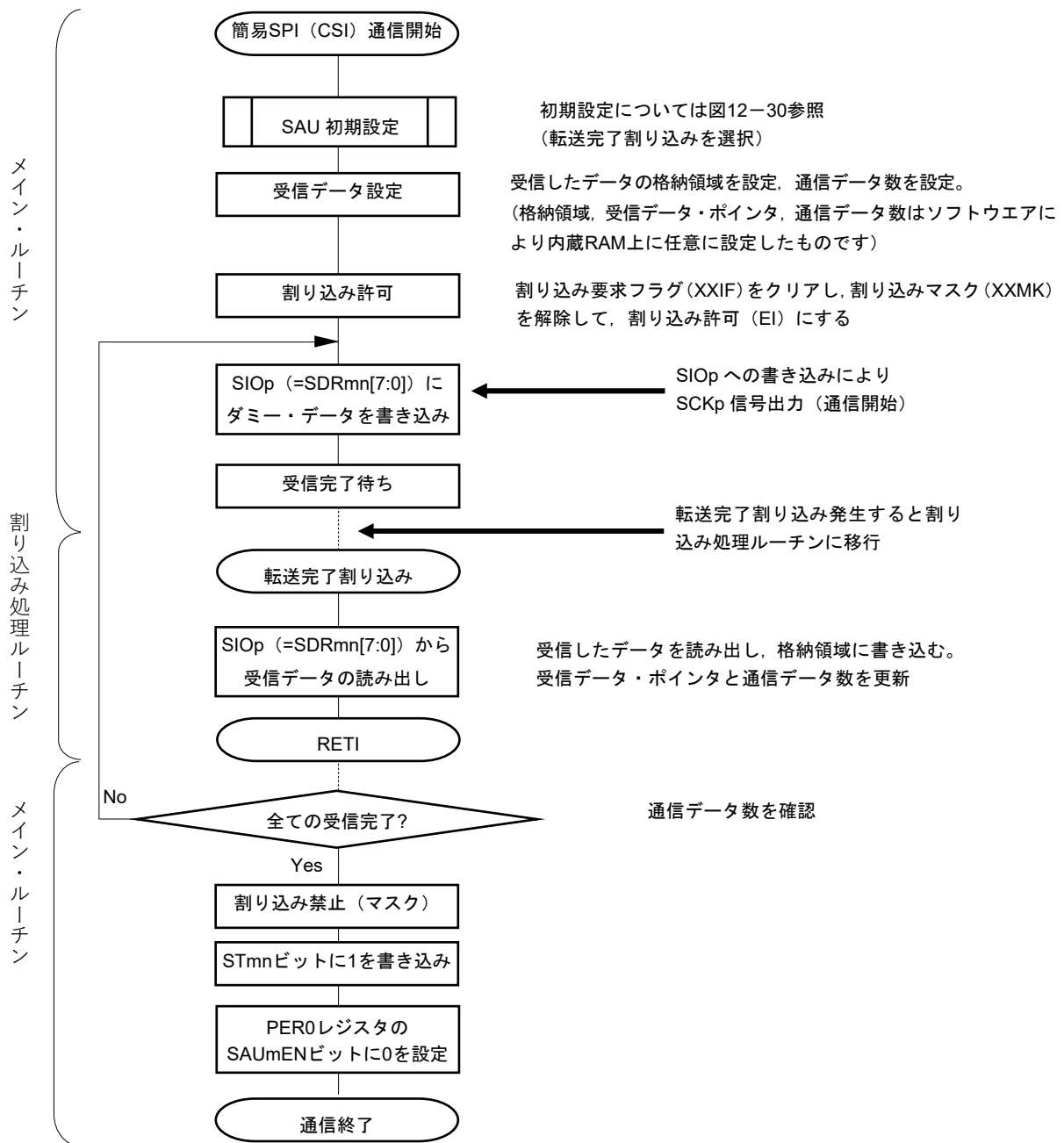
図12-34 マスタ受信（シングル受信モード時）のフロー・チャート
