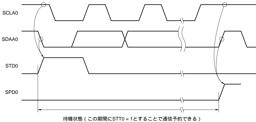
図13-26 通信予約受け付けタイミング
