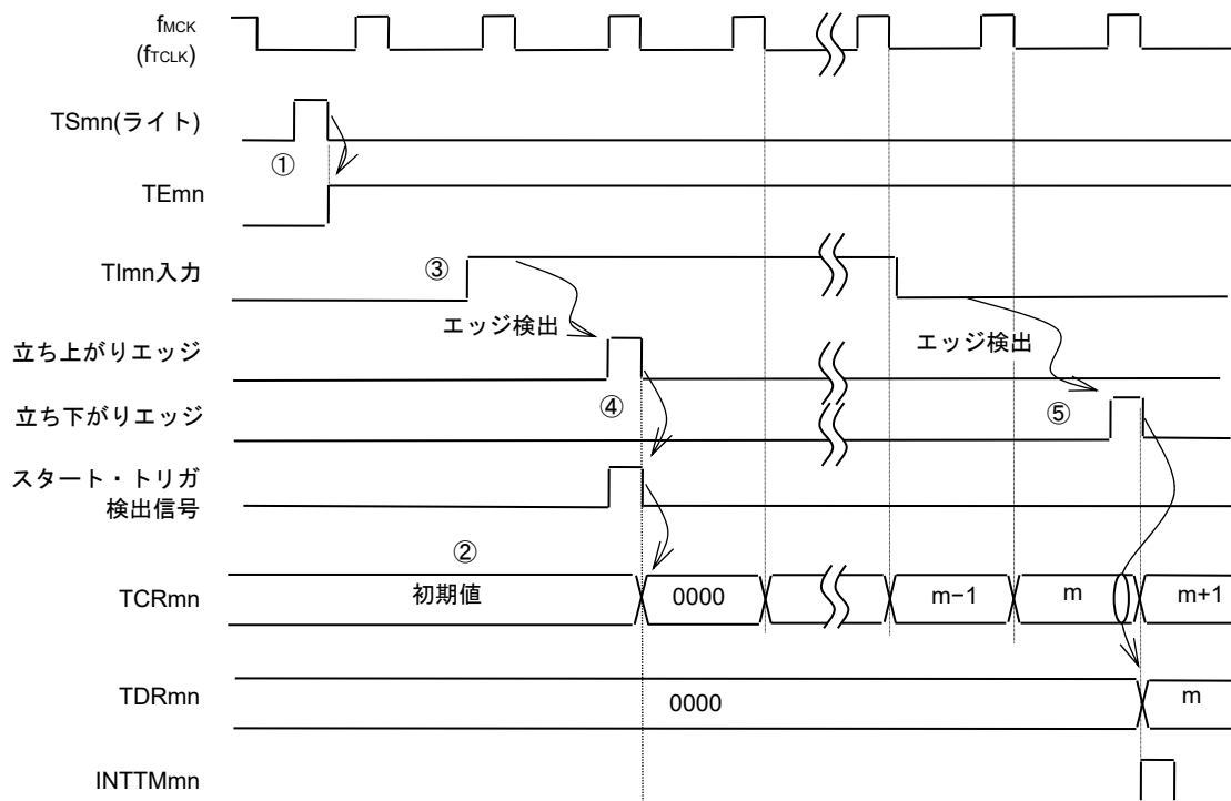
図6-27 動作タイミング（キャプチャ&amp;ワンカウント・モード：ハイ・レベル幅測定）
