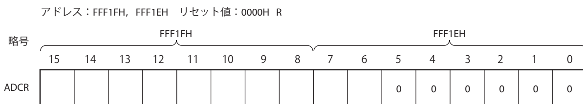
図11-9 10ビットA/D変換結果レジスタ (ADCR) のフォーマット
