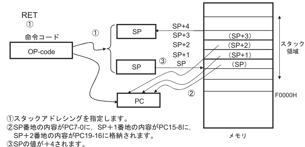
図3-35 RETの例
