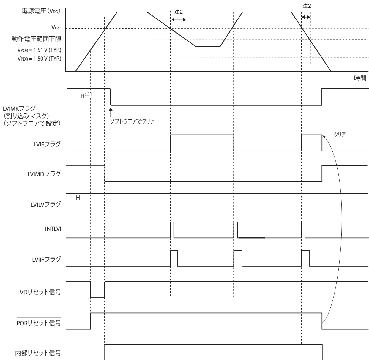
図22-6 割り込み信号発生タイミング (オプション・バイトのLVIMDS1, LVIMDS0 = 0, 1)
