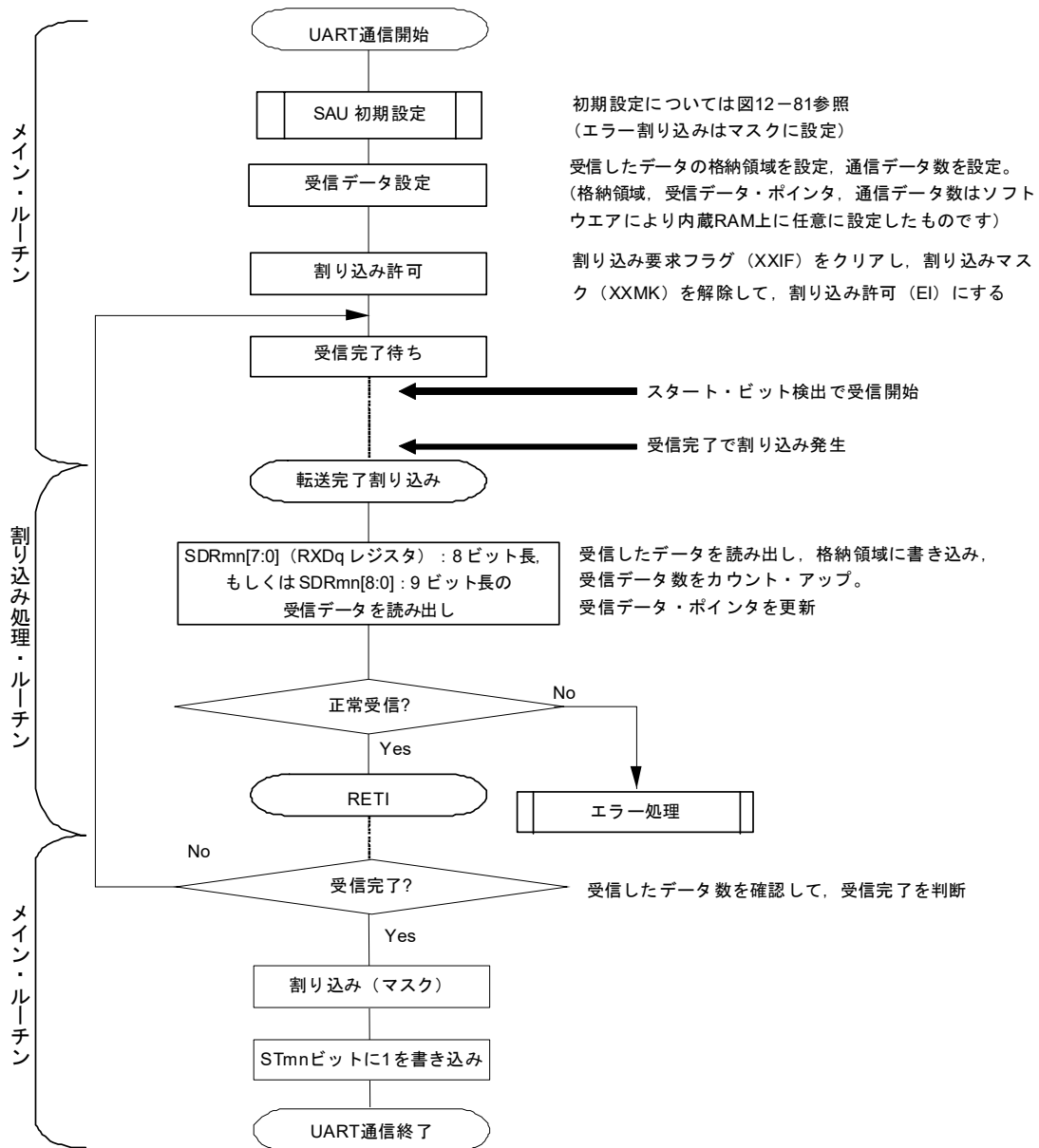
図12-85 UART受信のフロー・チャート
