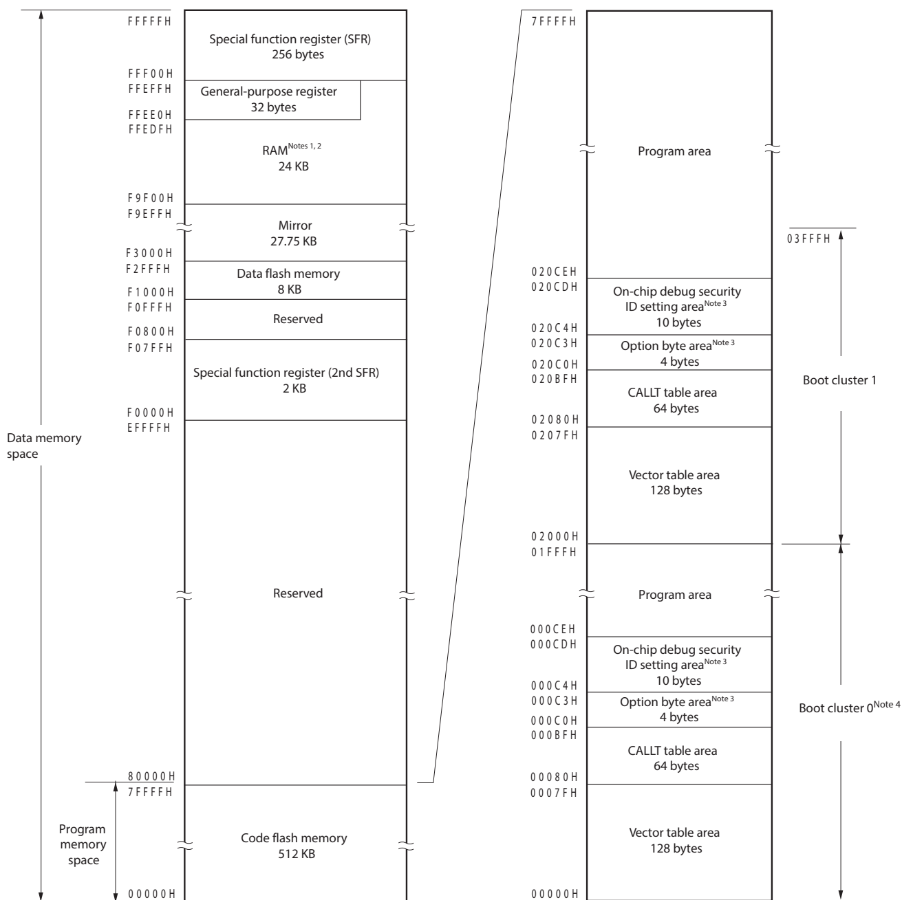
Figure 3-9. Memory Map (R5F10DPL, R5F10DSL)
