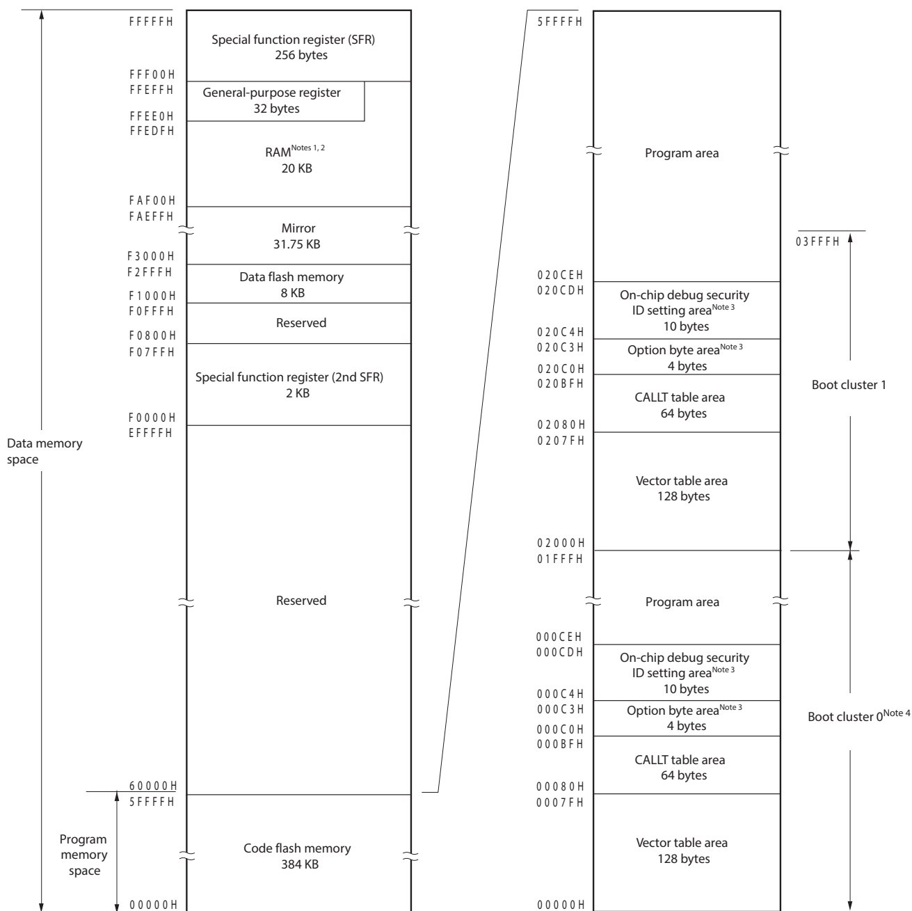
Figure3-8. Memory Map (R5F10DPK, R5F10DSK)
