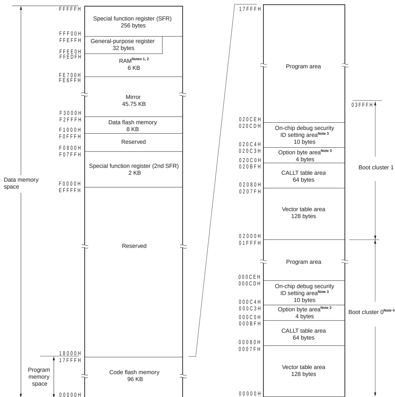
Figure 3-5. Memory Map (R5F10DMF, R5F10DPF)
