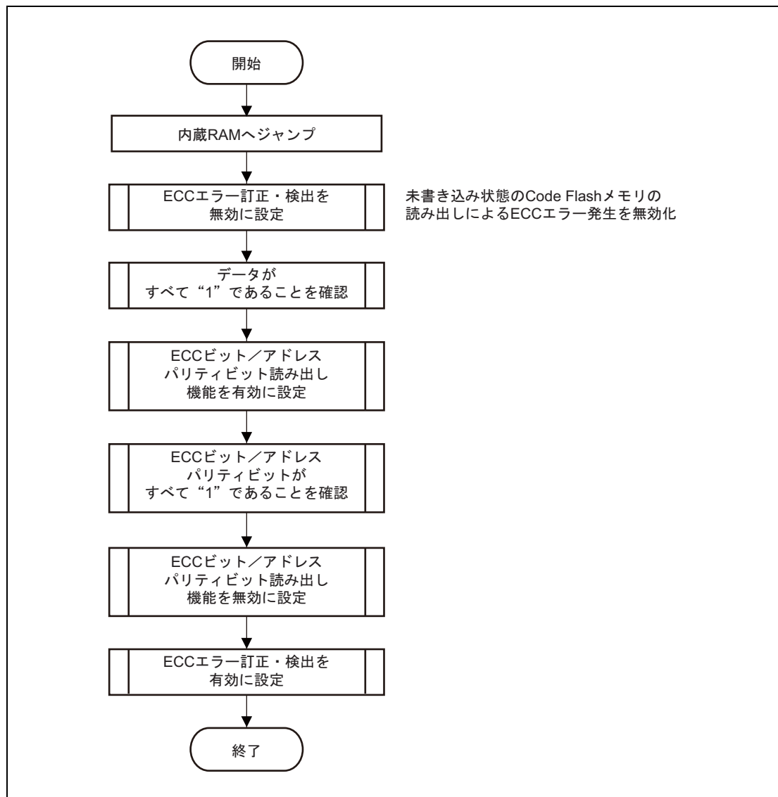
図 8.1 Code Flash メモリのブランクチェック方法
