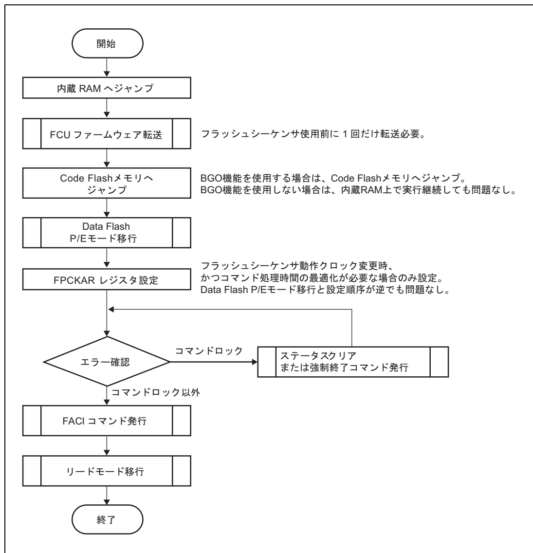
図 6.2 Data Flash P/E モード使用時の概略フロー
