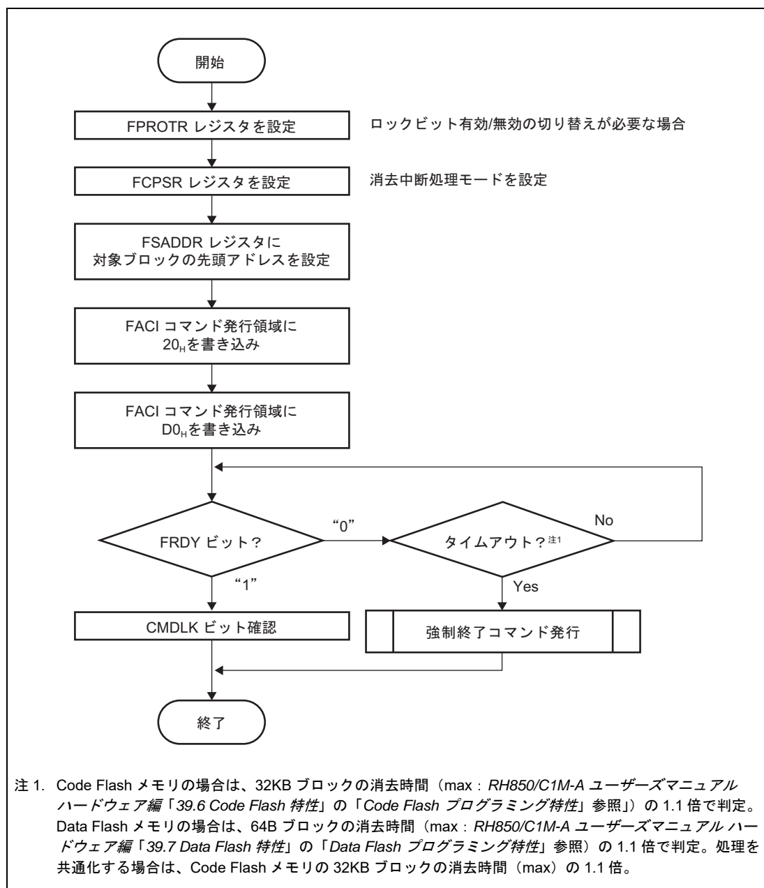
図 6.12 ブロックイレーズコマンドの使用法
