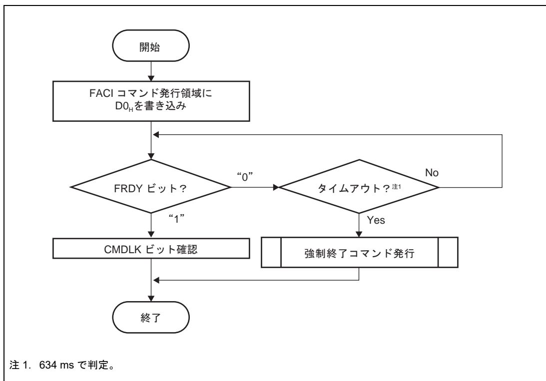
図 6.17 P/E レジュームコマンドの使用方法
