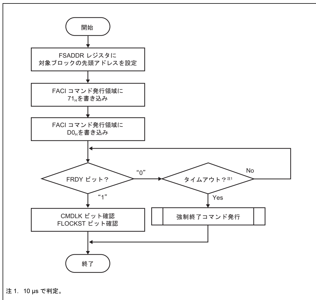
図 6.24 ロックビットリードコマンドの使用法
