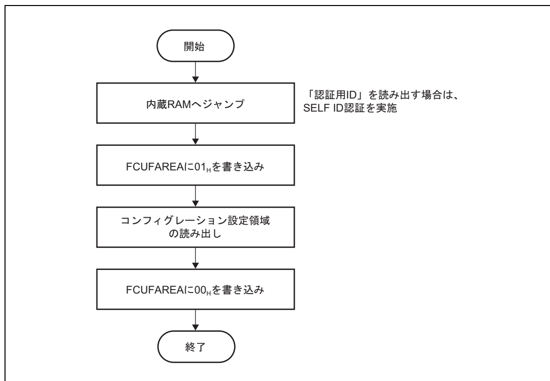
図 6.22 コンフィグレーション設定領域の読み出しフロー
