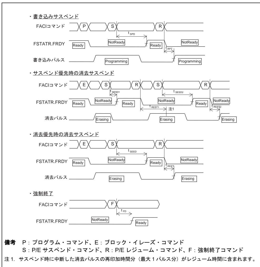
図 10.2 サスペンド/レジューム/強制終了タイミング
