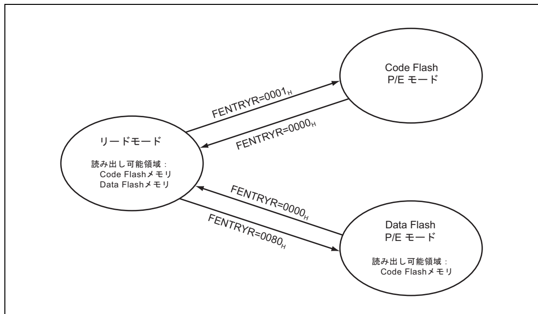
図 5.1 フラッシュシーケンサのモード
