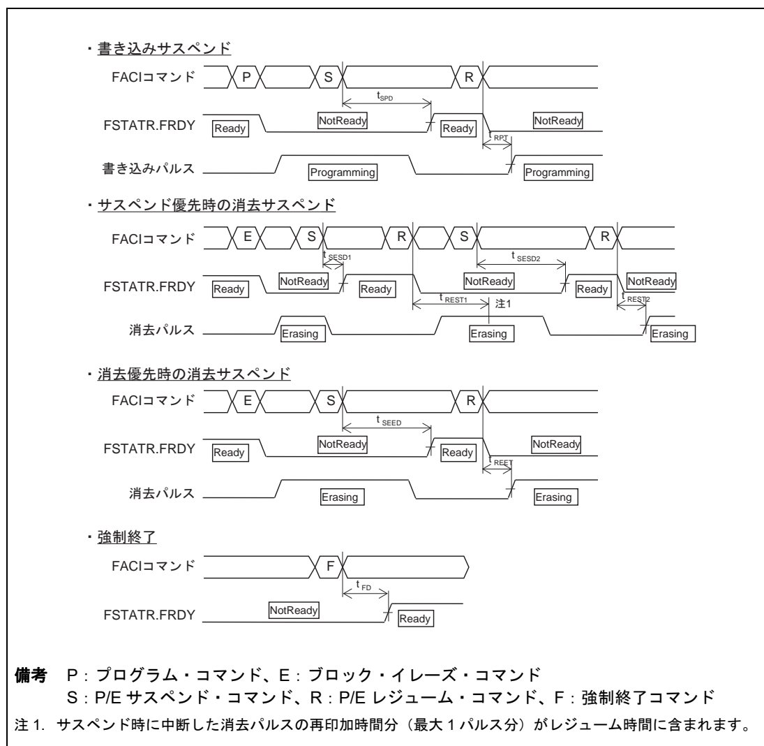
図 10.1 サスペンド/レジューム/強制終了タイミング
