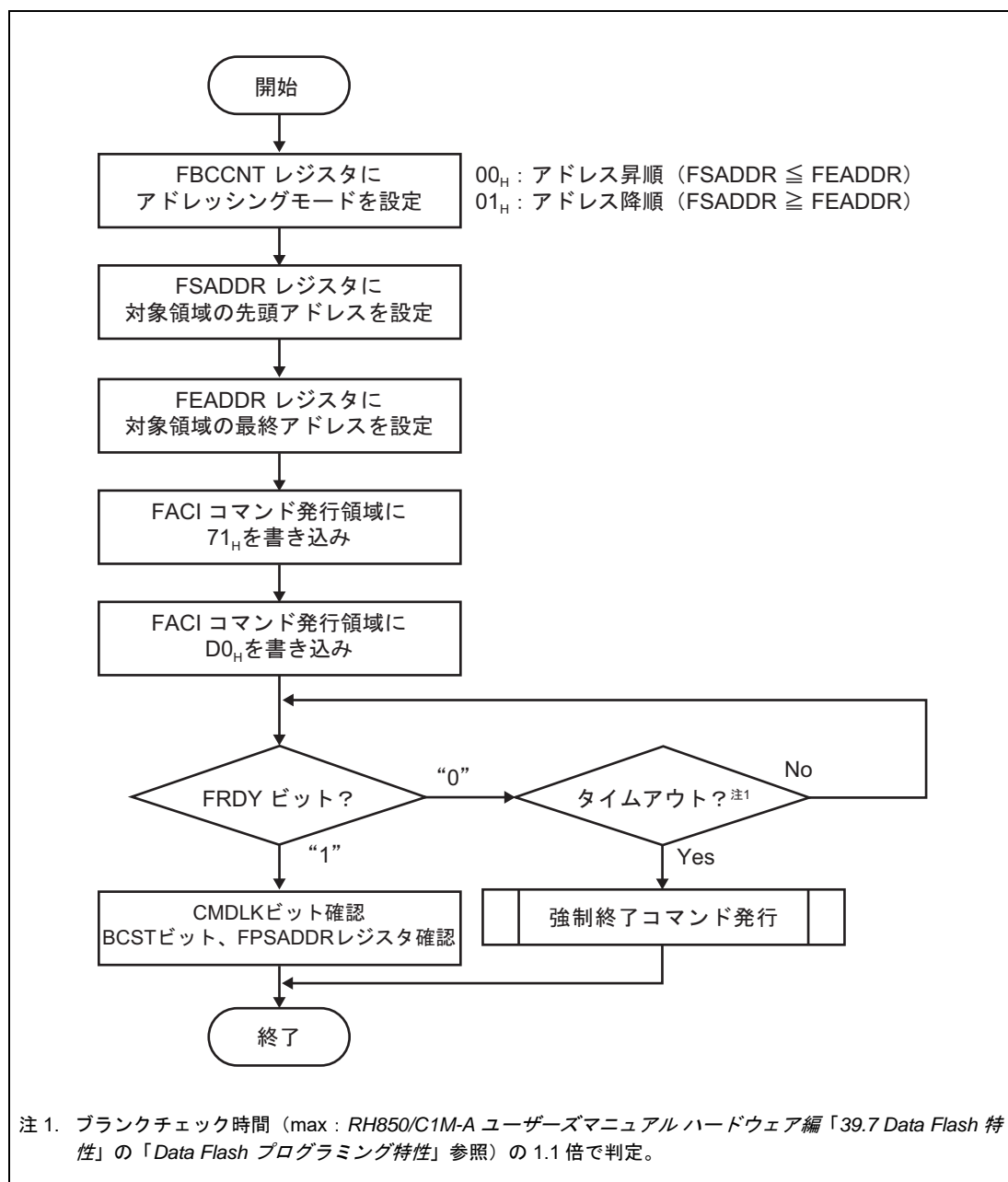
図 6.20 ブランクチェックコマンドの使用法
