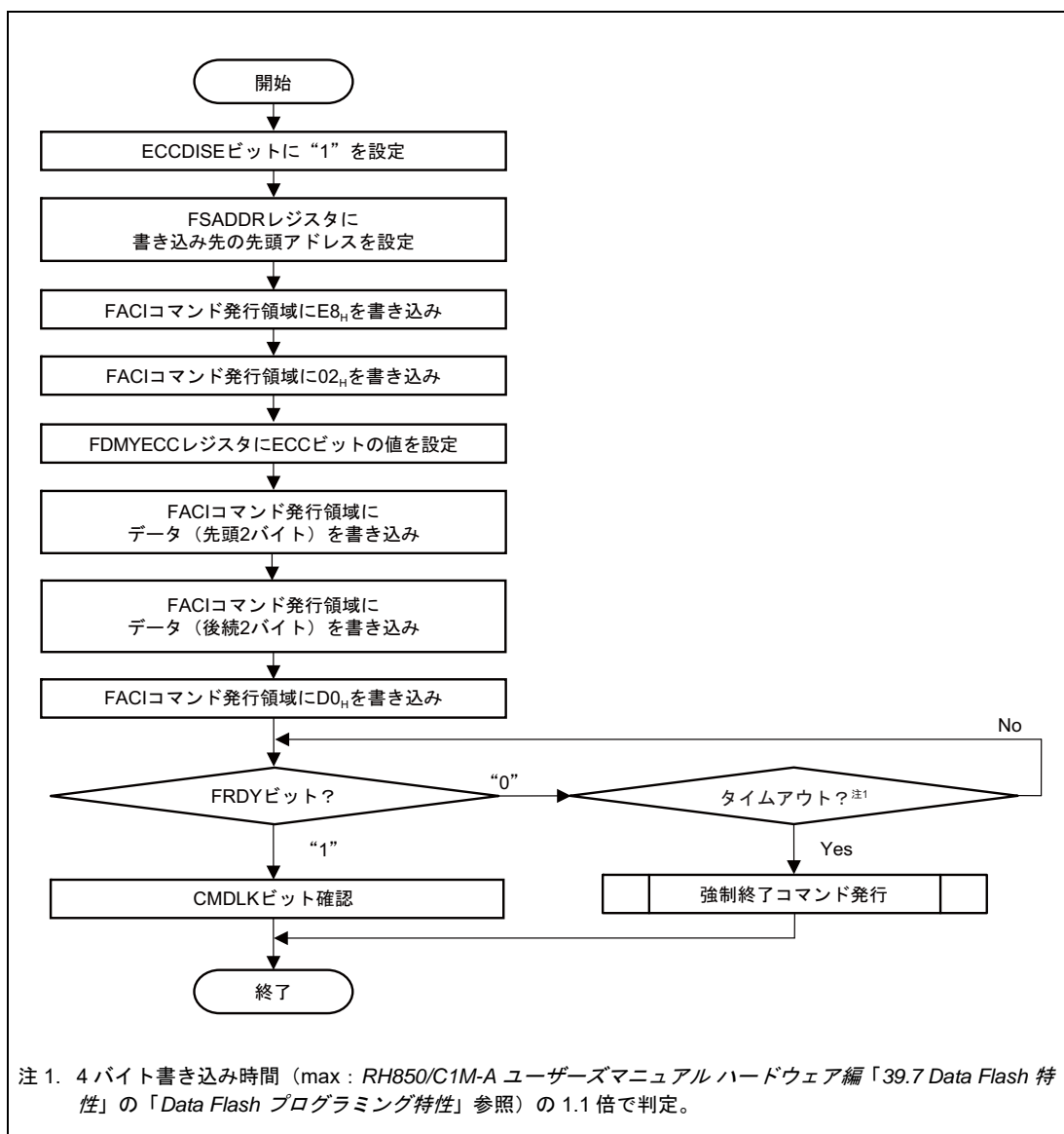
図 6.29 Data Flash メモリの ECC エラー注入方法
