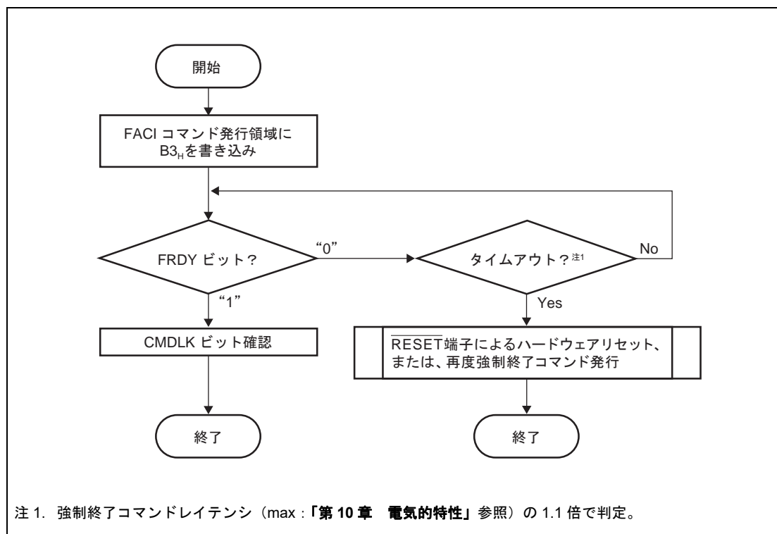
図 6.19 強制終了コマンドの使用方法
