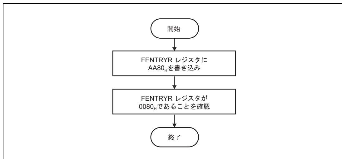
図 6.6 Data Flash P/E モード移行フロー
