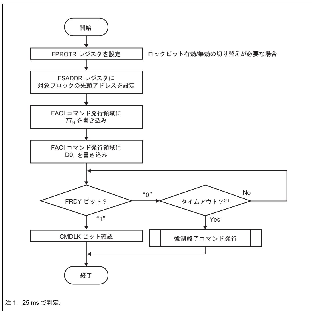
図 6.23 ロックビットプログラムコマンドの使用法
