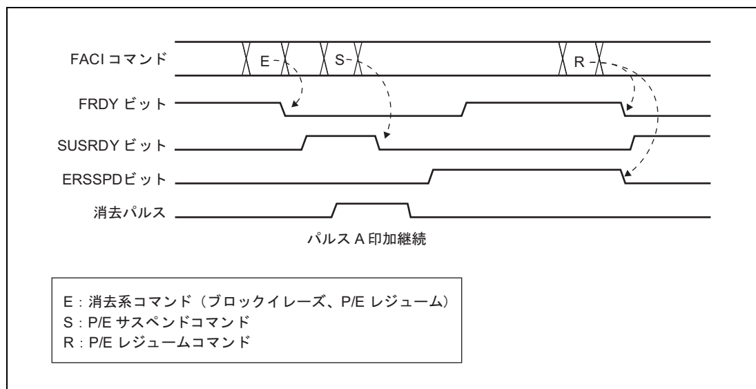
図 6.16 消去処理の中断動作（消去優先モード）
