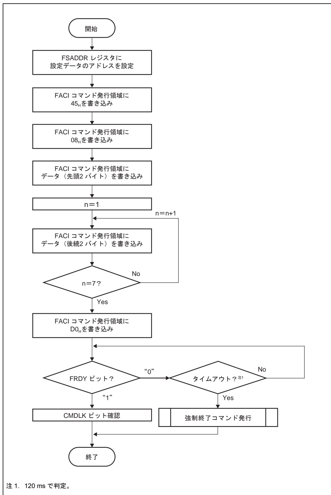
図 6.25 OTP 設定コマンドの使用方法
