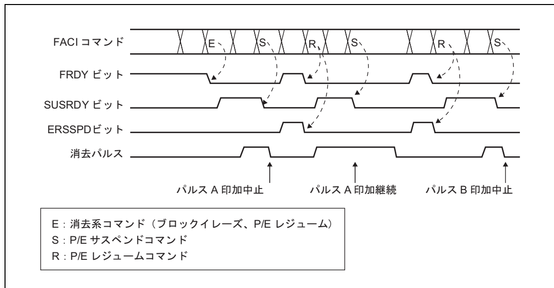
図 6.15 消去処理の中断動作 (サスペンド優先モード)
