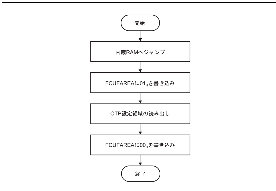
図 6.27 OTP 設定領域の読み出しフロー
