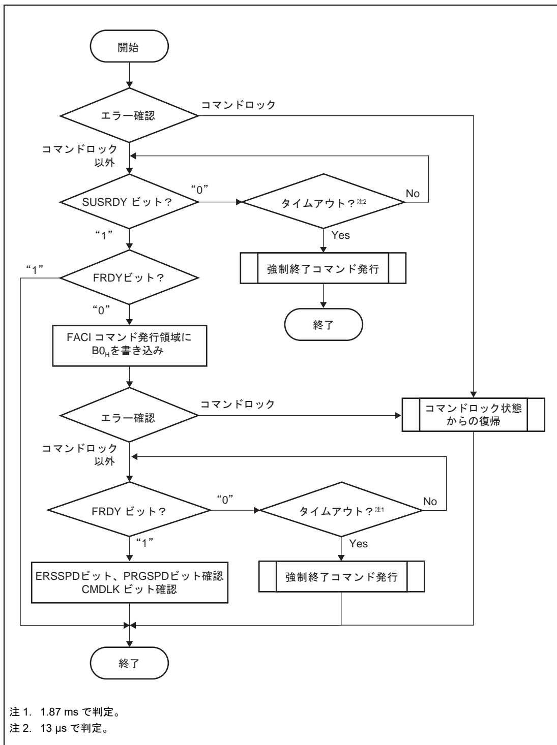
図 6.13 P/E サスペンドコマンドの使用方法
