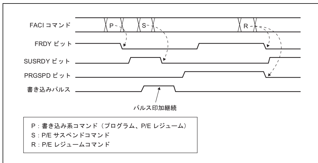
図 6.14 書き込み処理の中断動作
