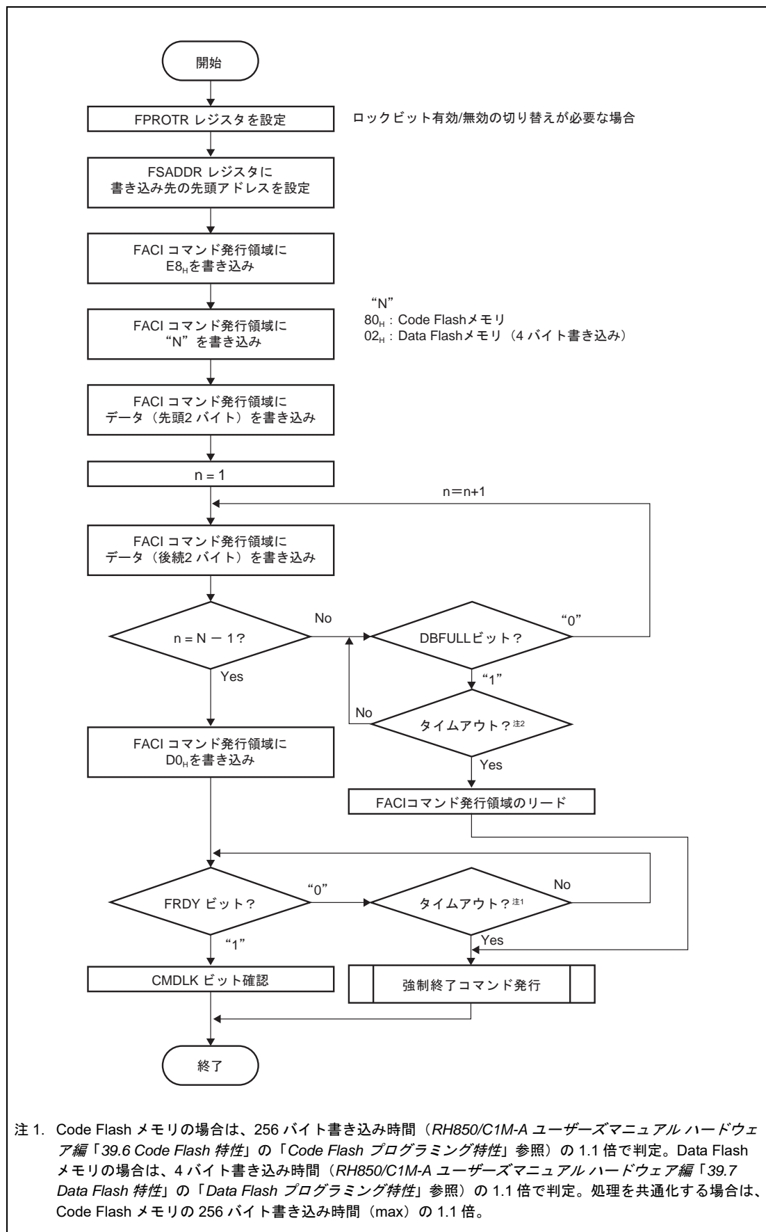
図 6.10 プログラムコマンドの使用方法
