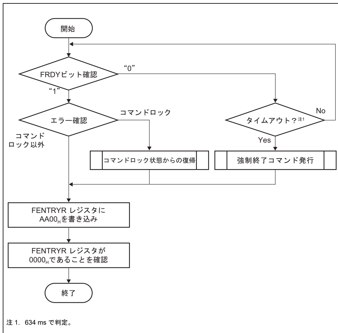
図 6.7 リードモード移行フロー
