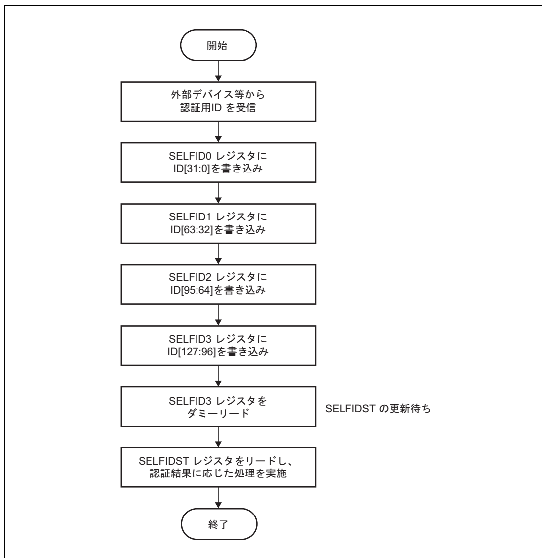
図 6.8 ID 比較のフロー
