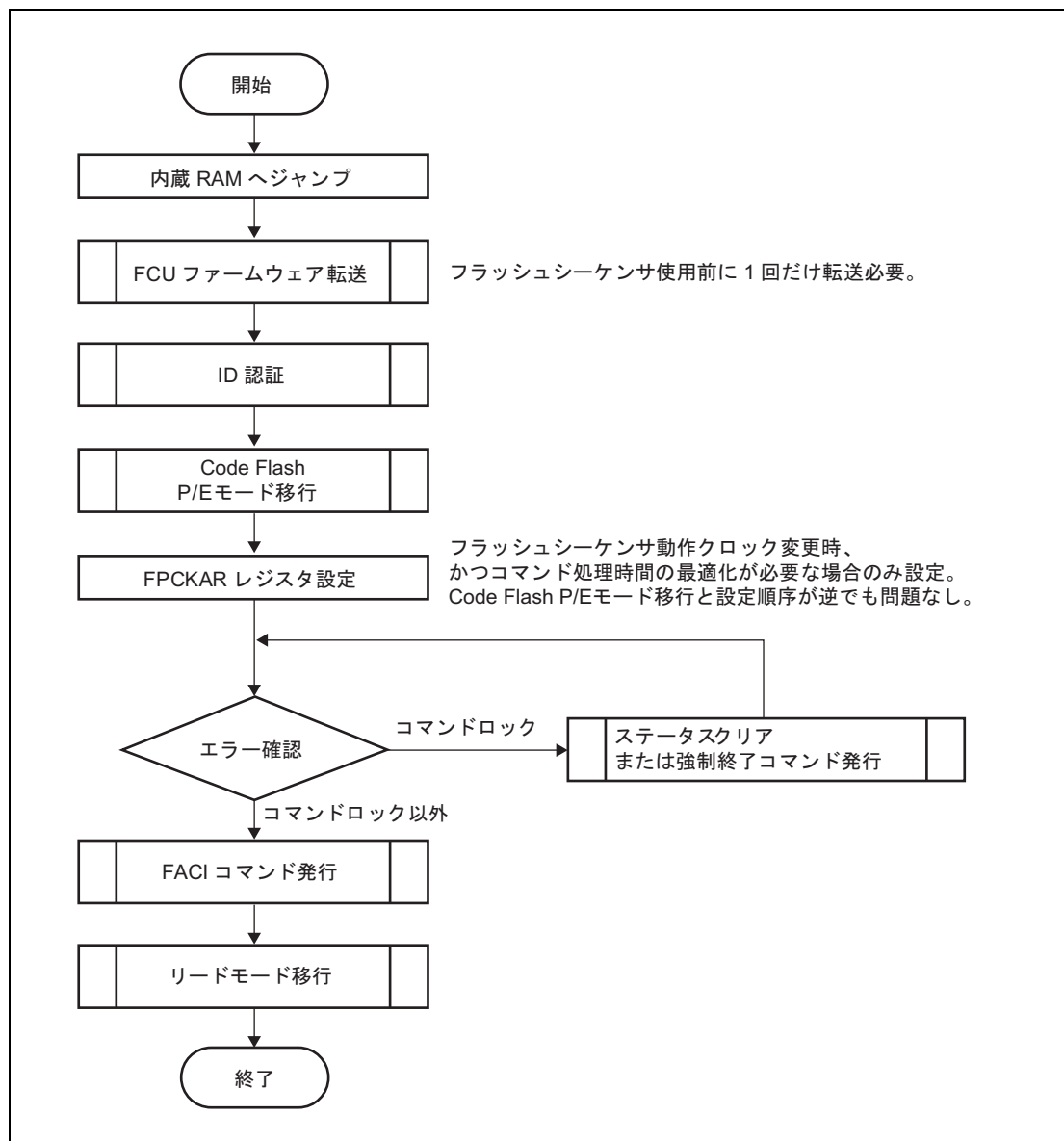
図 6.1 Code Flash P/E モード使用時の概略フロー
