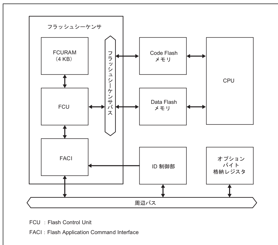
図 2.1 フラッシュメモリ関連モジュールの構成図
