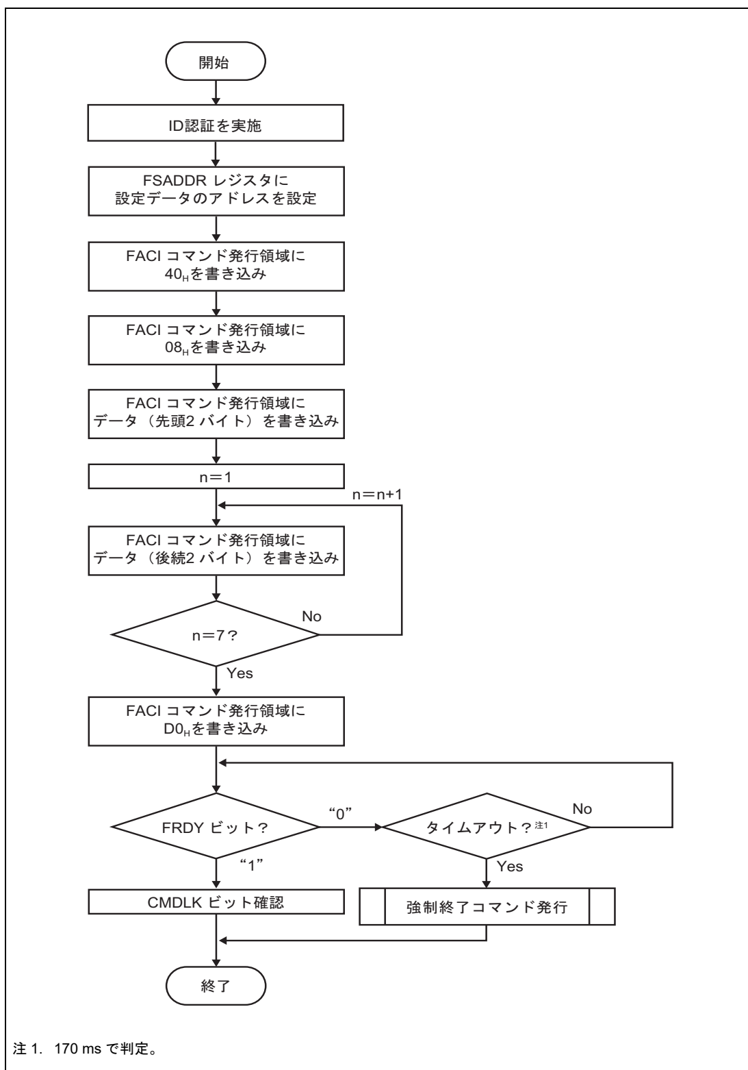
図 6.21 コンフィグレーション設定コマンドの使用法
