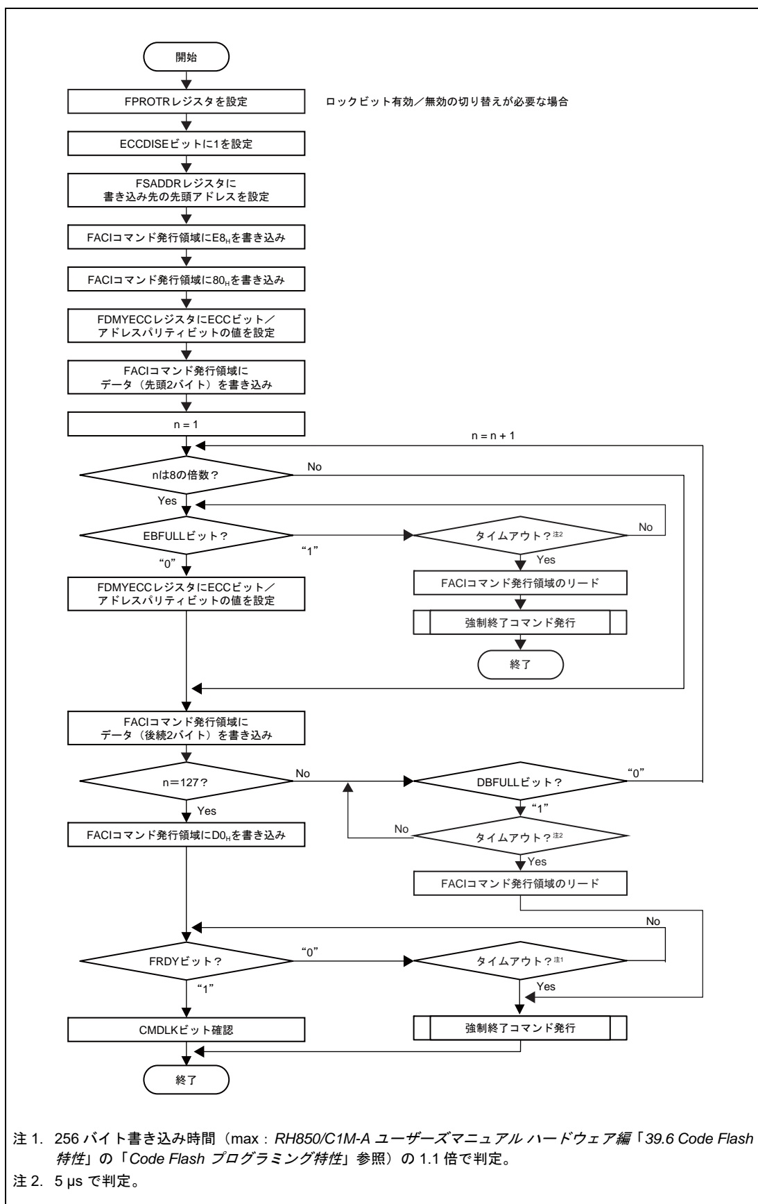
図 6.28 Code Flash メモリの ECC エラー注入方法
