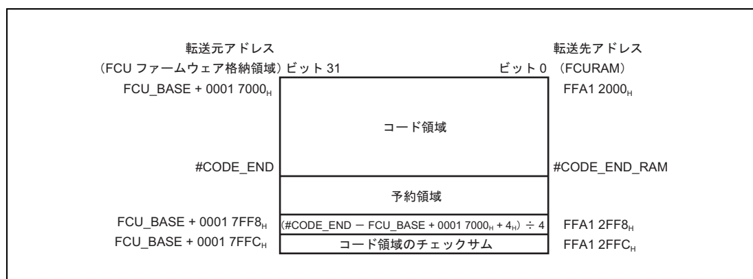
図 6.4 FCU ファームウェアの構成
