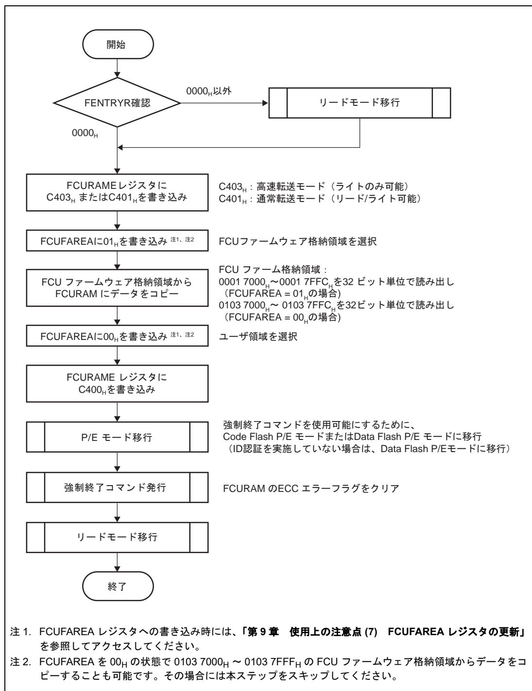
図 6.3 FCU ファームウェア転送フロー
