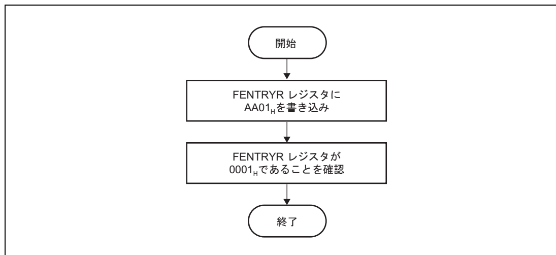
図 6.5 Code Flash P/E モード移行フロー
