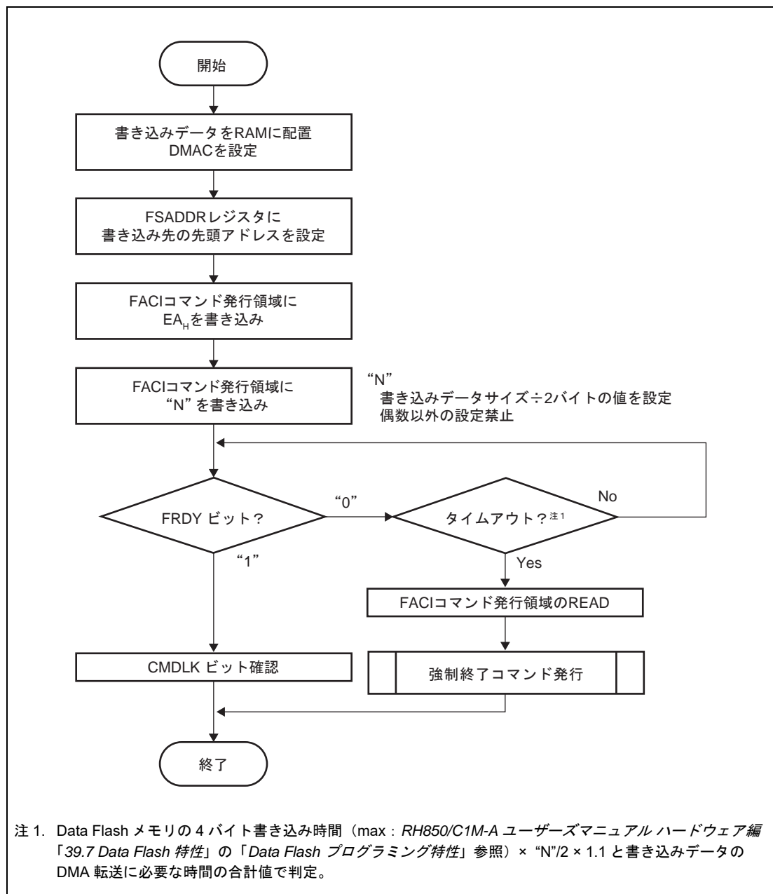
図 6.11 DMA プログラムコマンドの使用法
