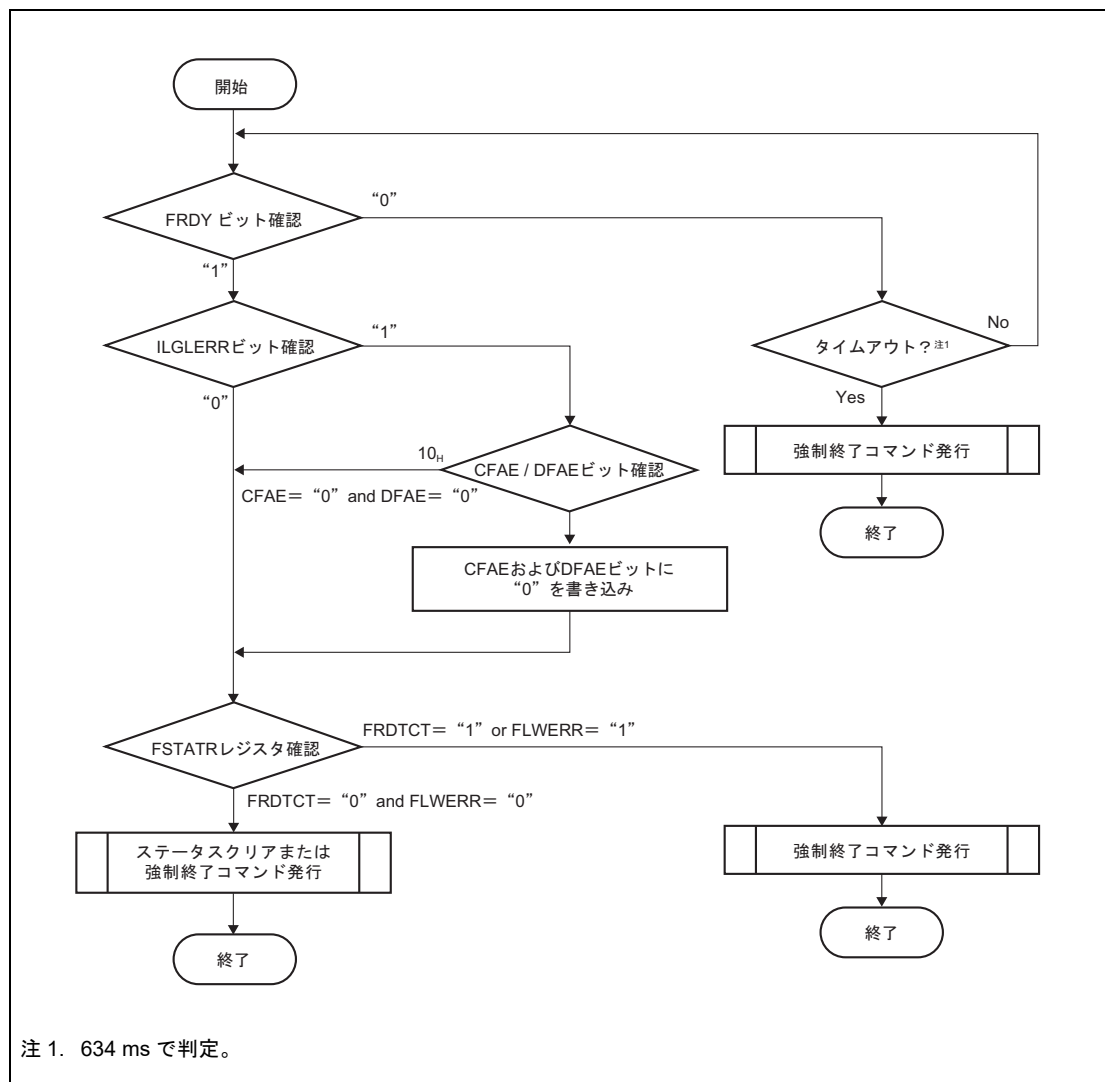
図 6.9 コマンドロック状態からの復帰方法
